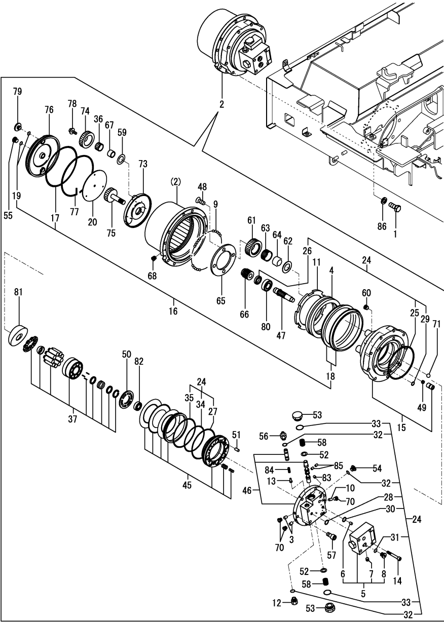
Fig.57. TRAVEL MOTOR
