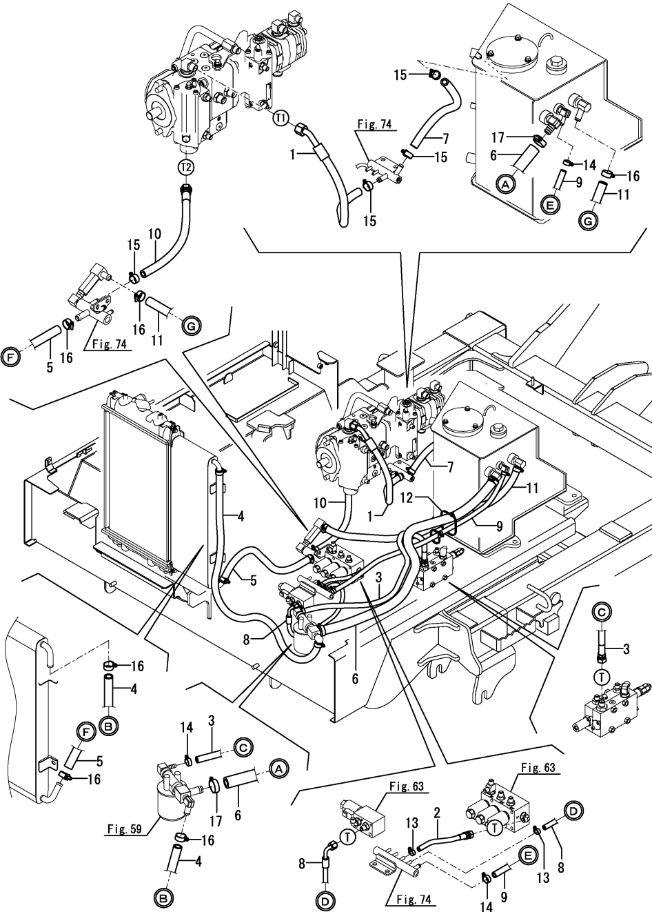
Fig.77. RETURN
