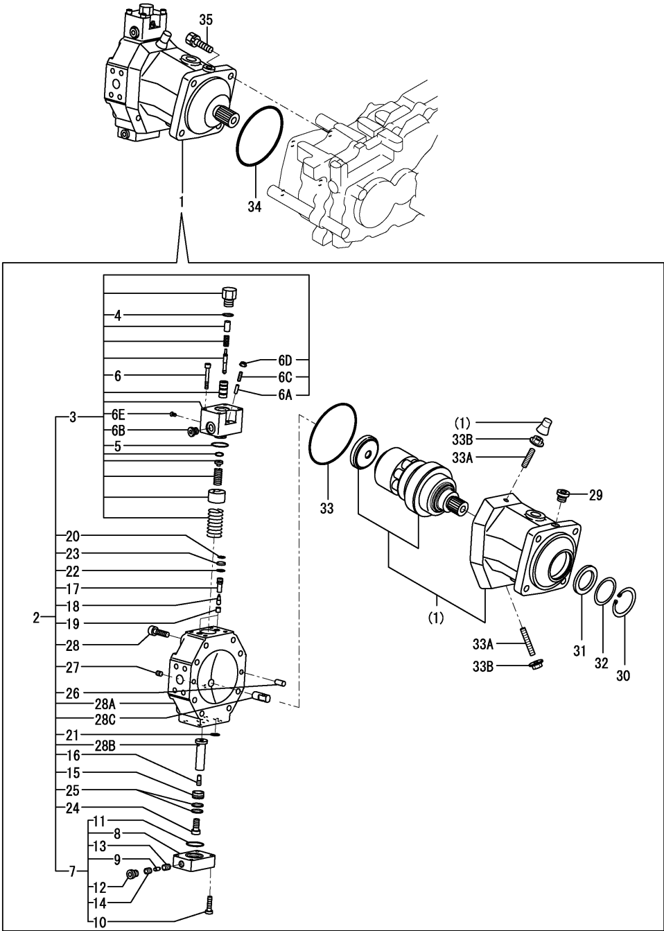
Fig.43. MOTOR
