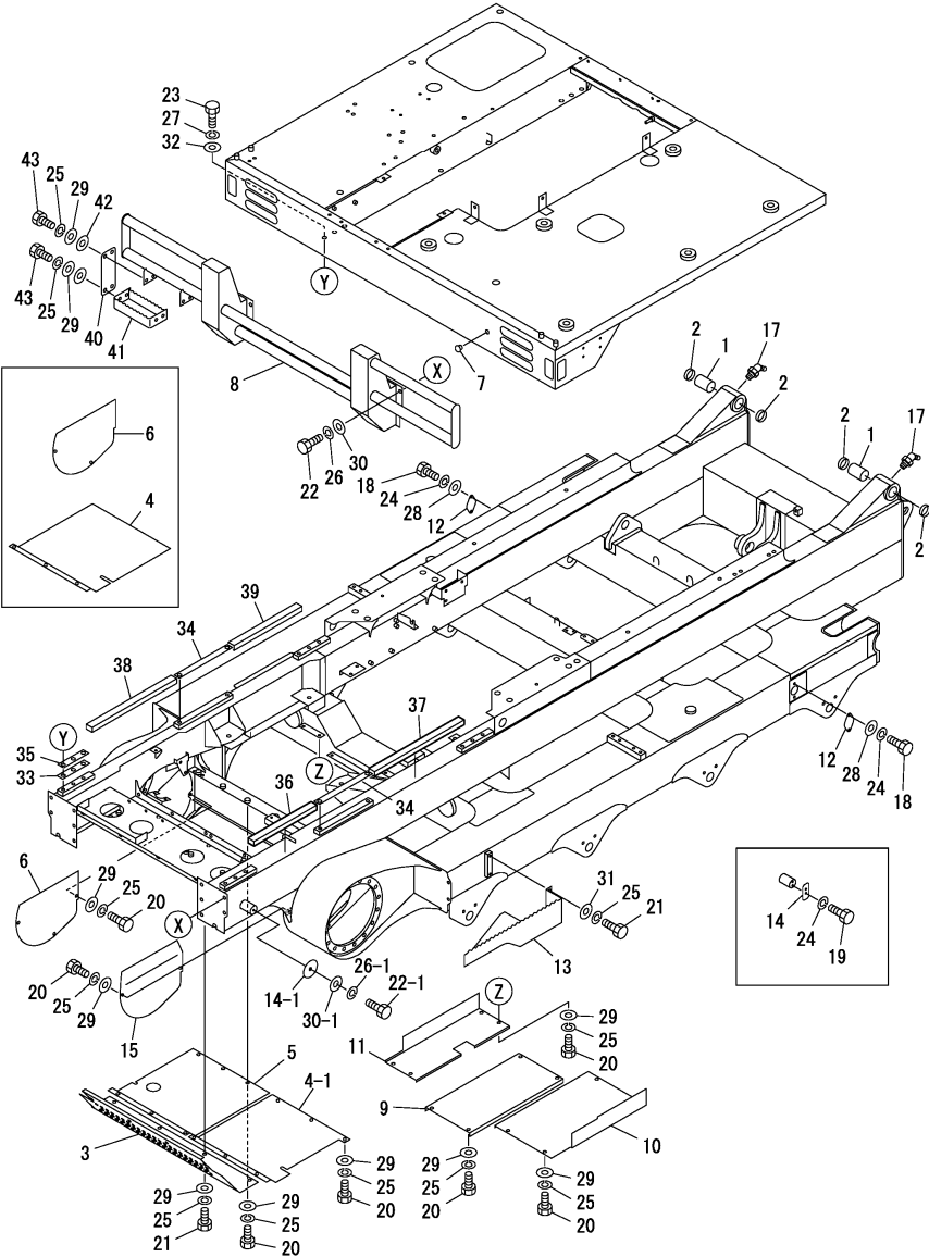
Fig.1. FRAME
