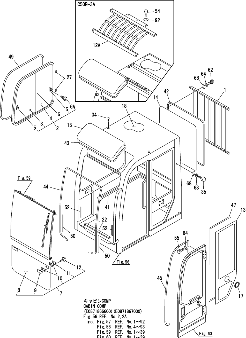
Fig.57. CABIN(2)
