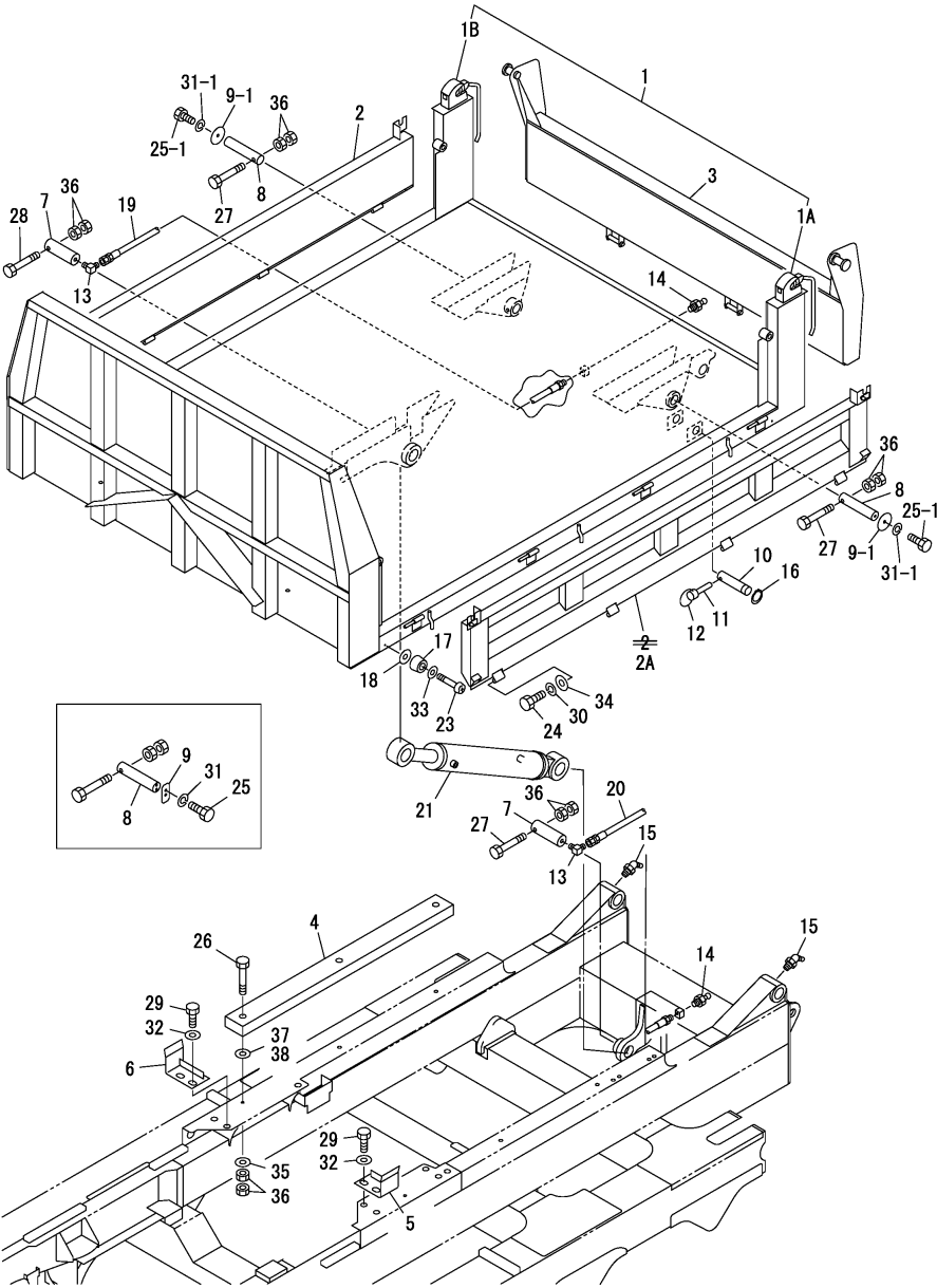
Fig.74. DUMP BODY
