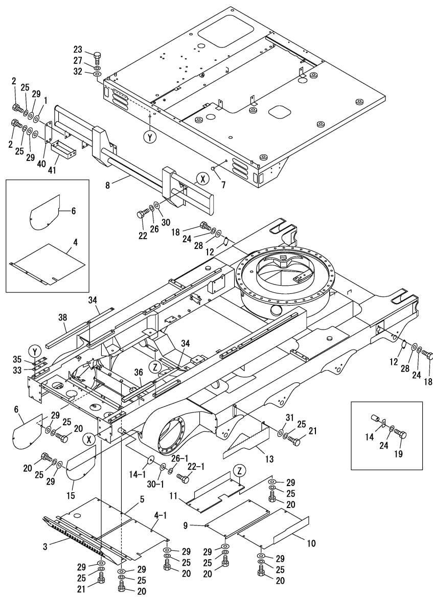
Fig.2. FRAME(TURNING)
