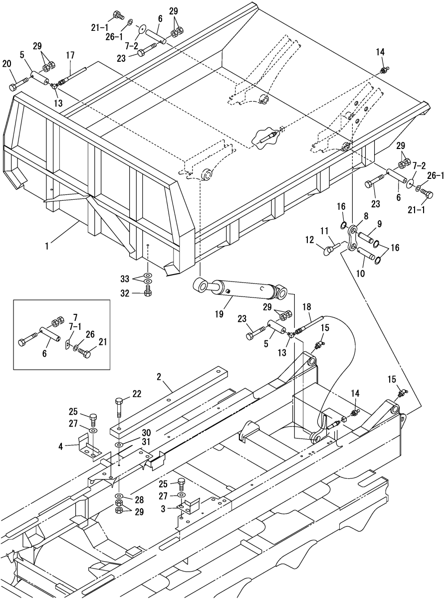
Fig.72. VESSELL
