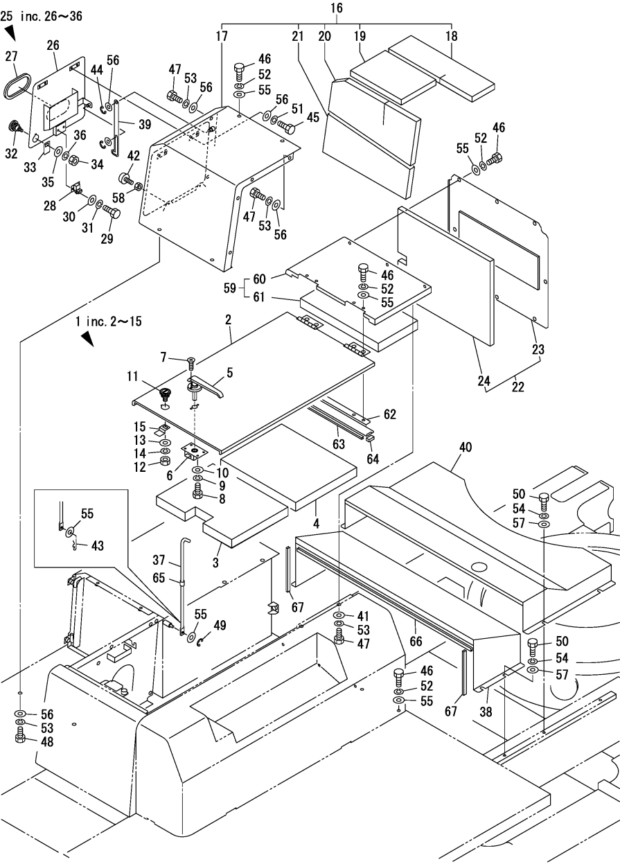
Fig.45. COVER(2)(TO M40562)
