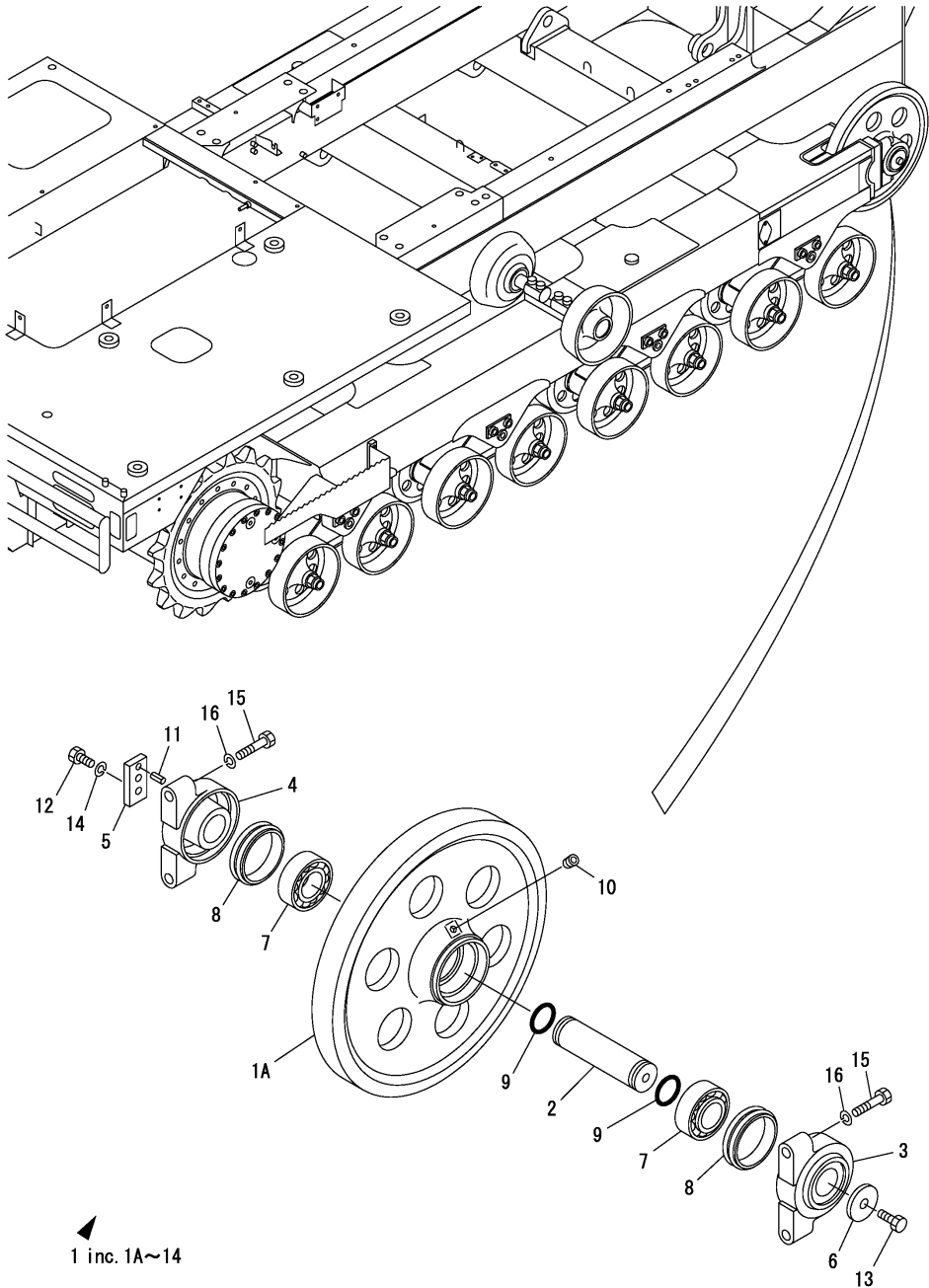
Fig.6. IDLER
