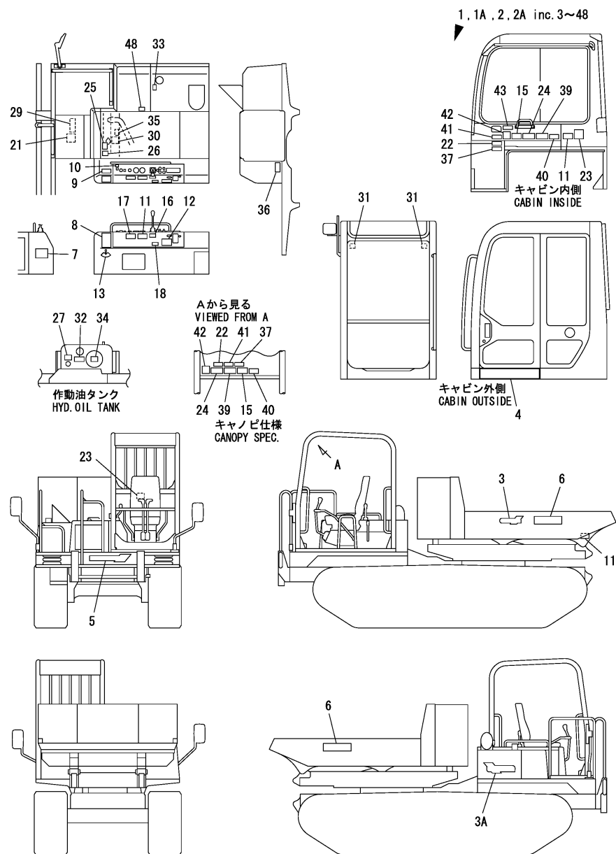
Fig.79. LABEL(TURNING)
