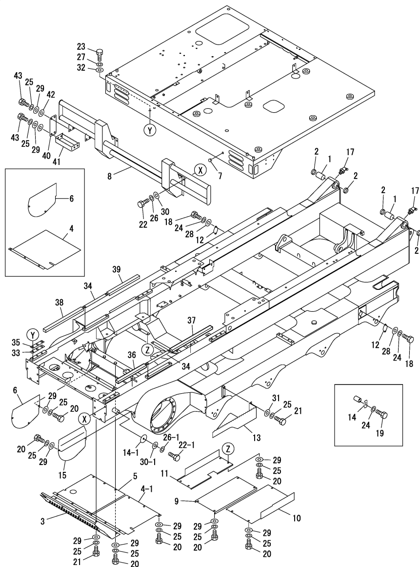
Fig.1. FRAME
