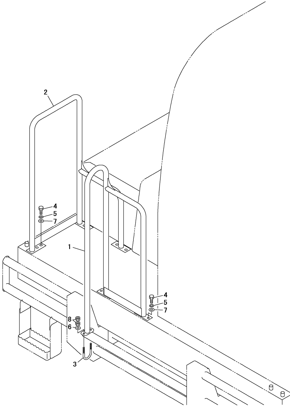
Fig.47. BALUSTRADE
