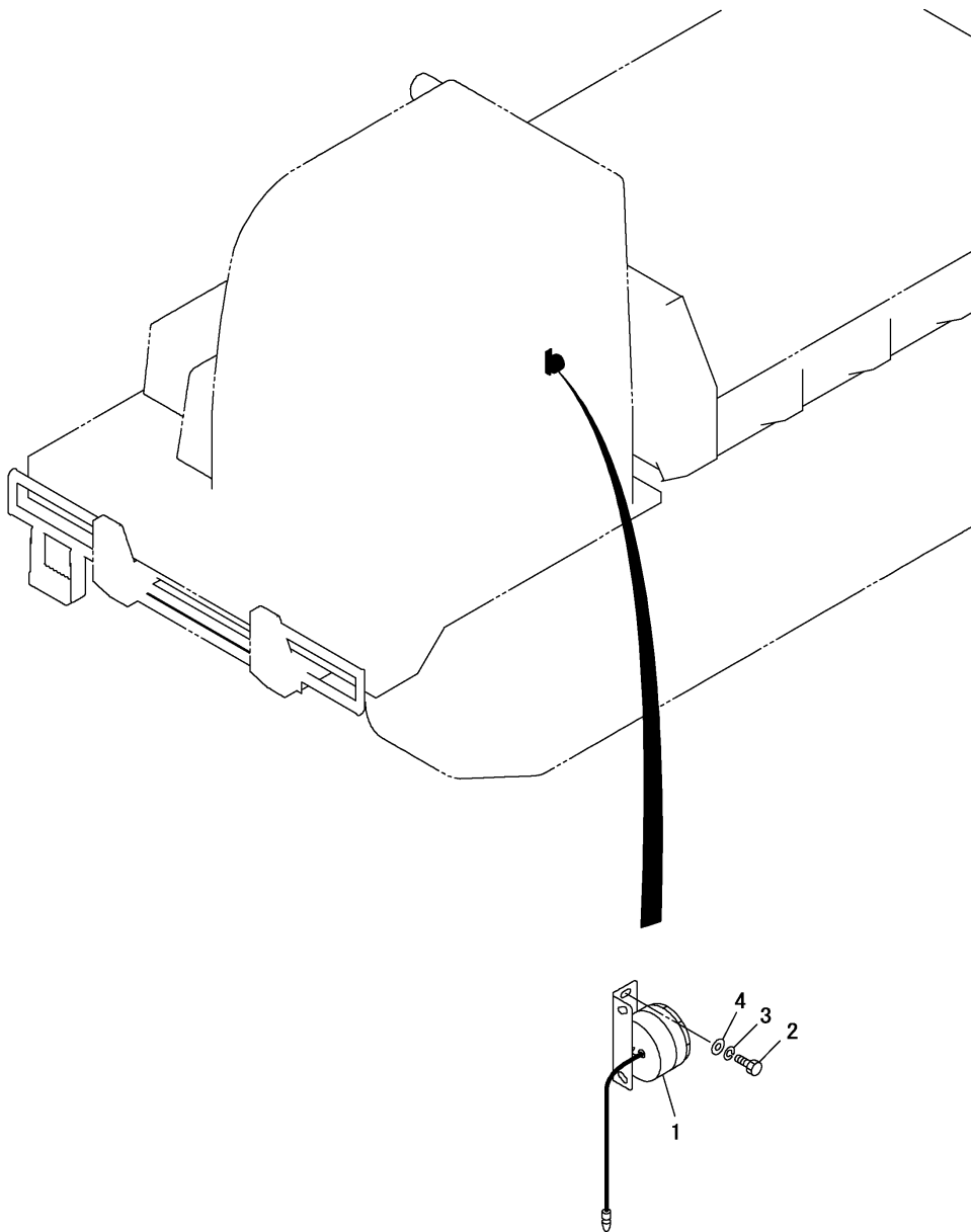
Fig.30. BACK BUZZER
