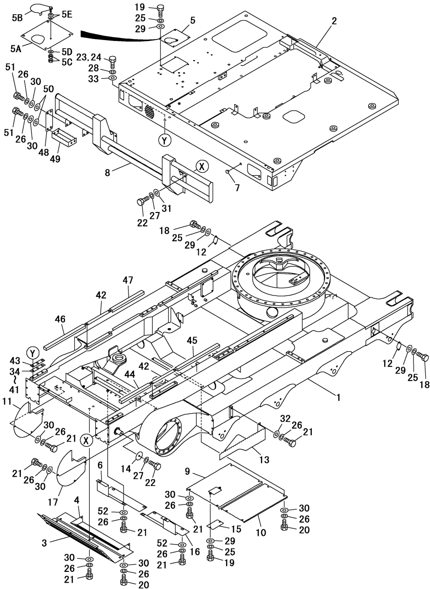
Fig.2. FRAME(TURNING)
