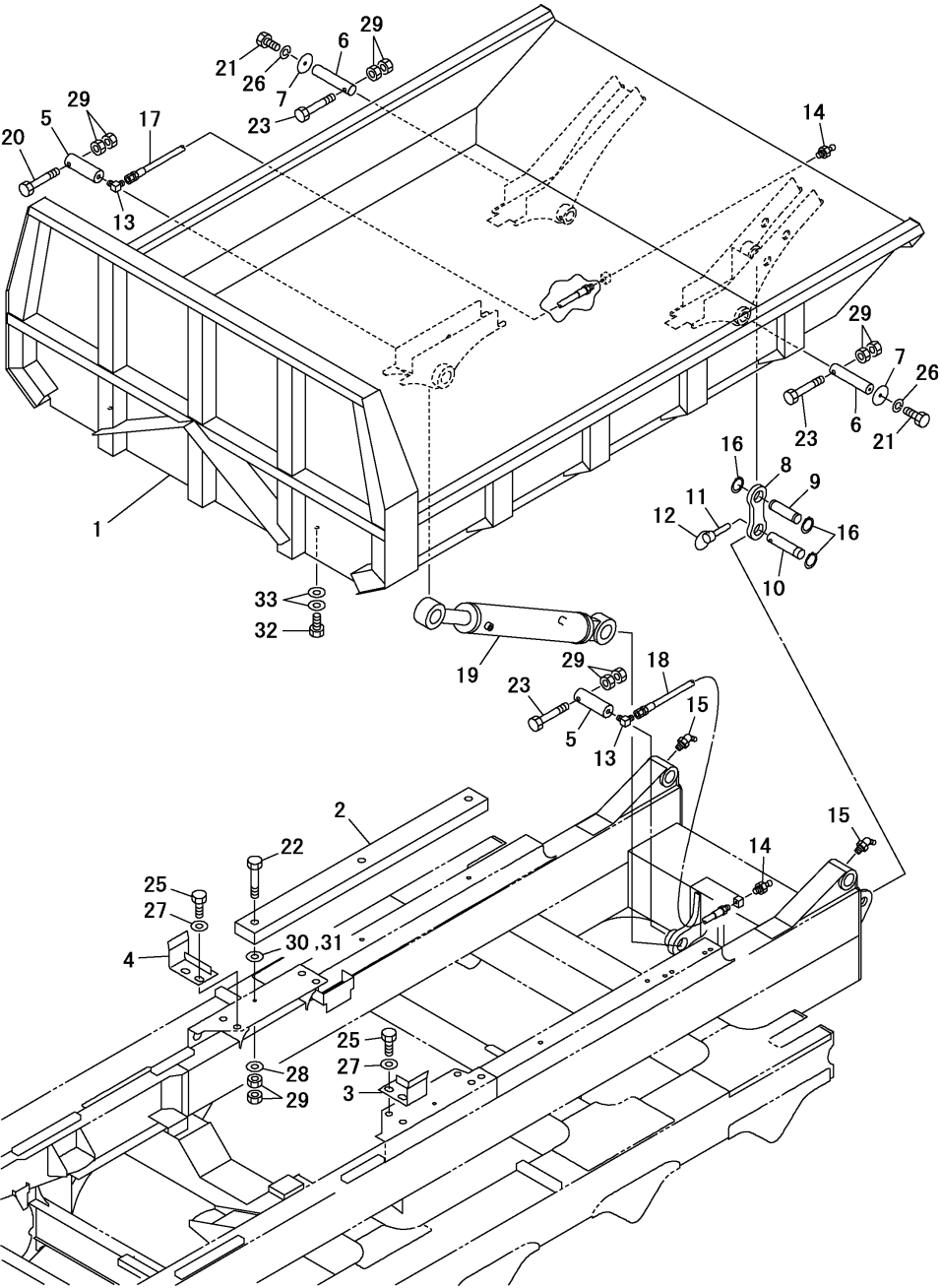
Fig.66. VESSEL
