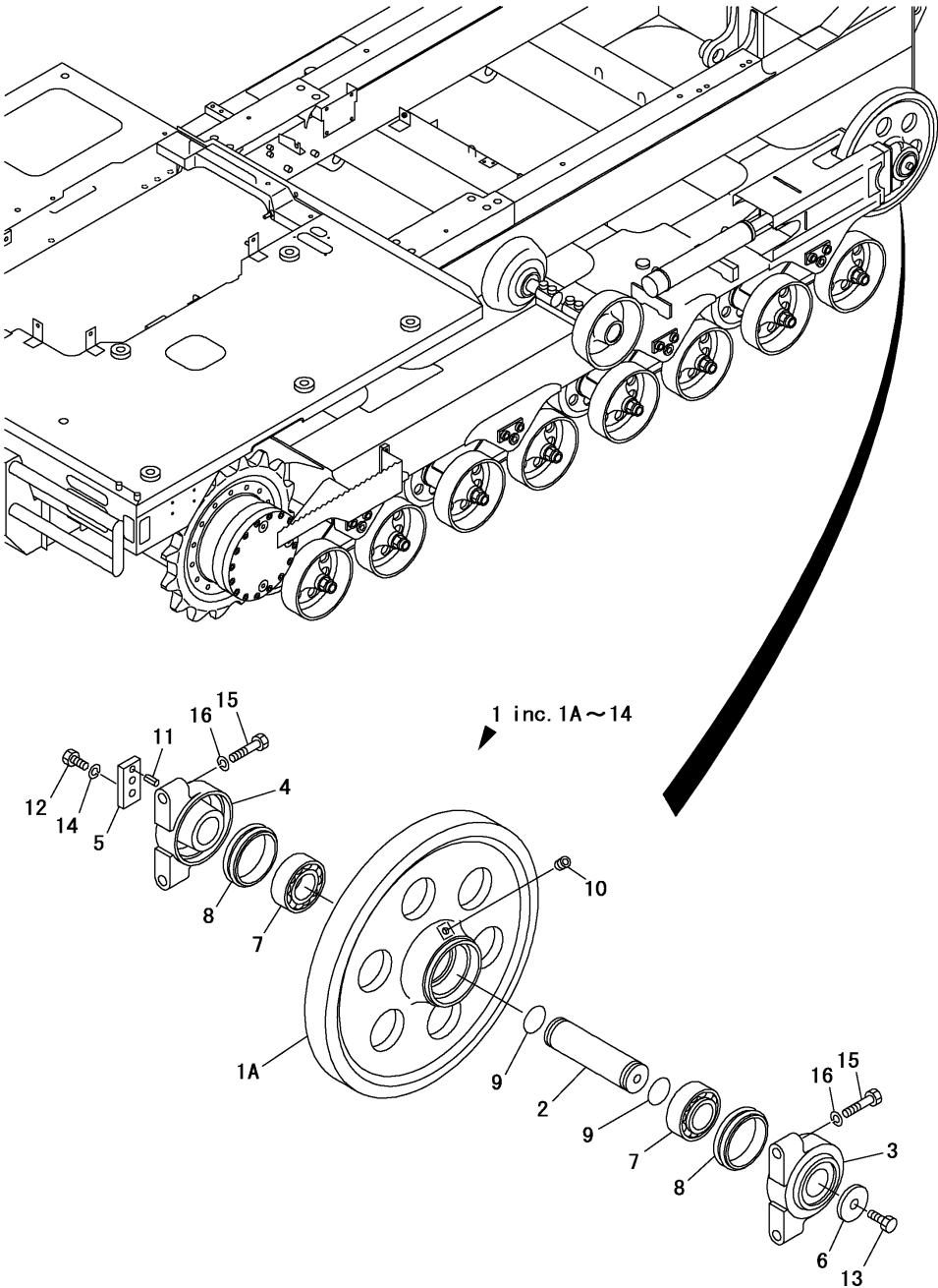
Fig.6. IDLER
