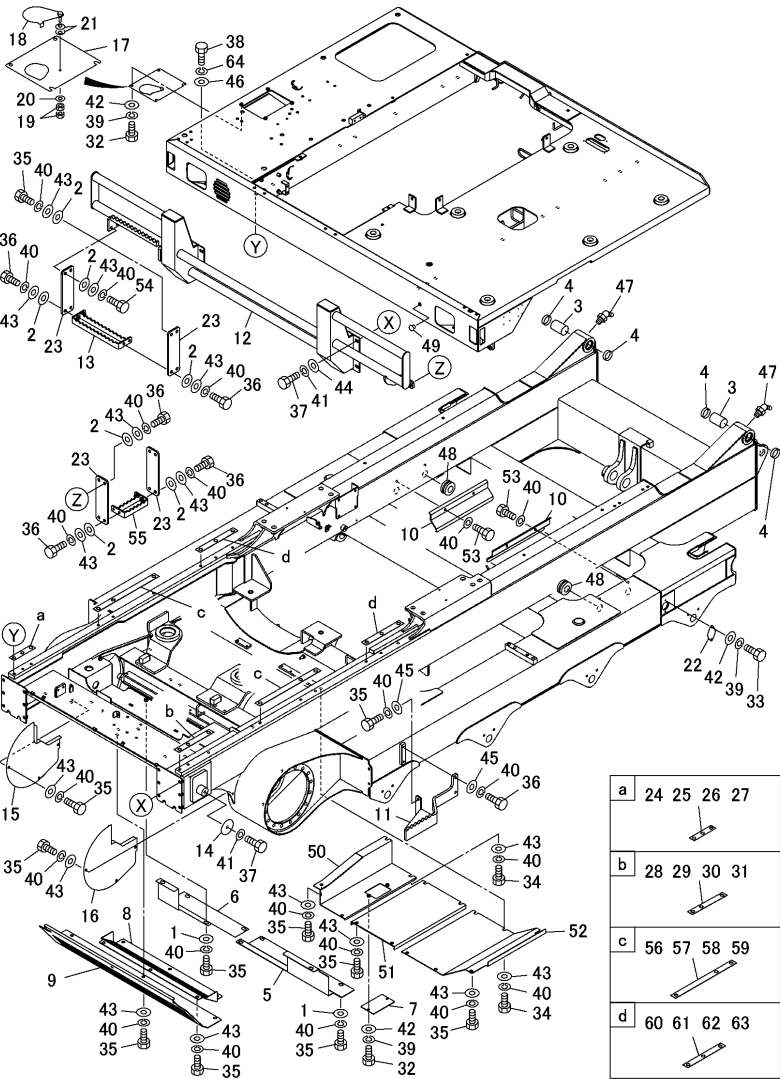
Fig.1. FRAME
