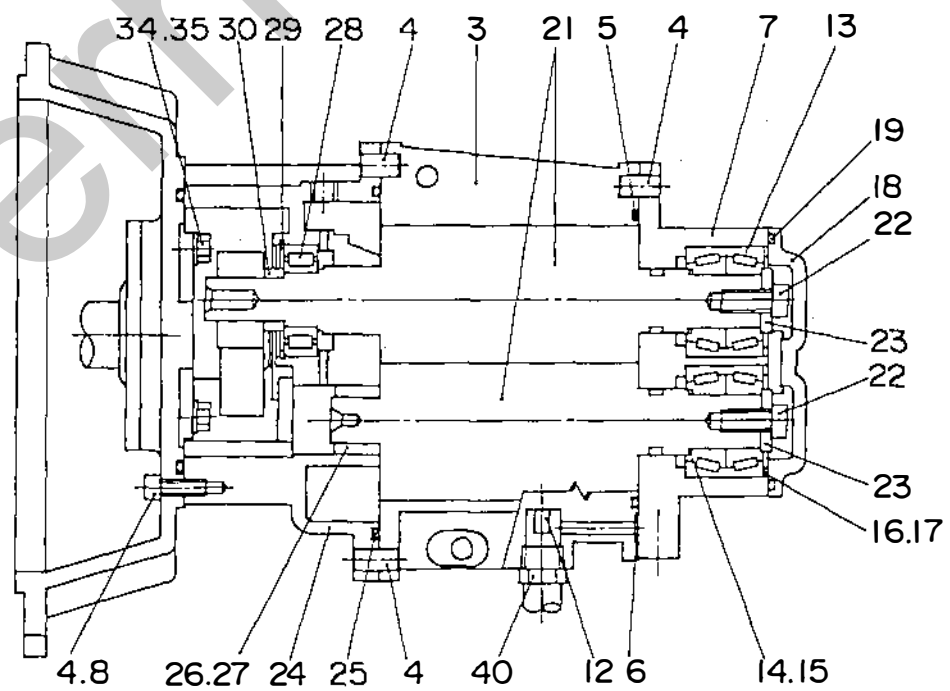
SECTION Y - Y
