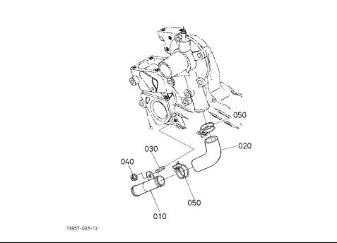
060100 ENTRADA COLECTOR
