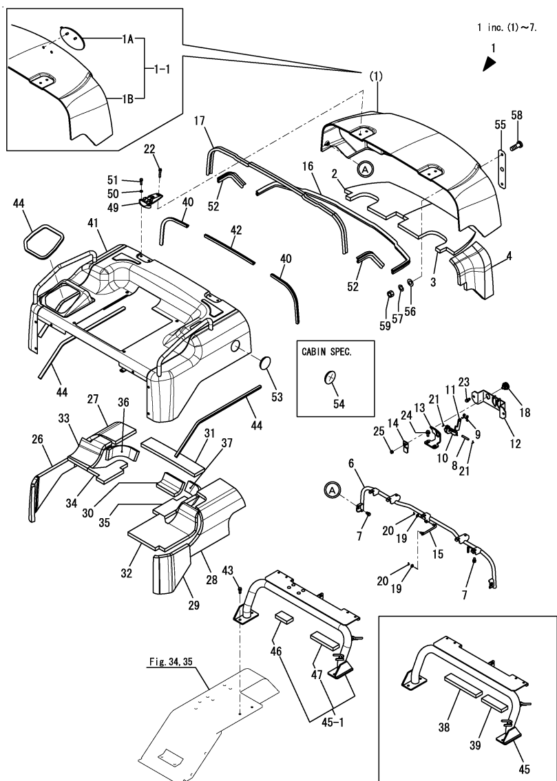
Fig.38. BONNET
