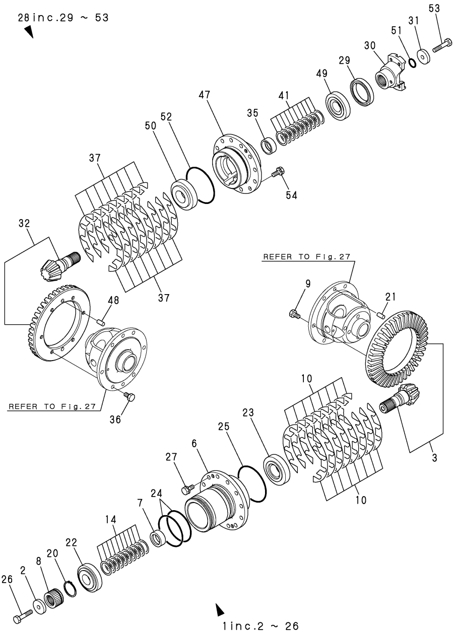
OCK20-M36003 V3/V4-5(A),V5(-A)(JP) Fig.25. SPIRAL BEVEL GEAR(2)
