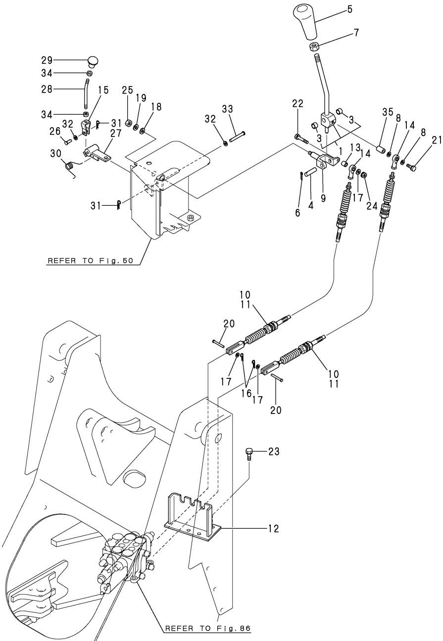
OCK20-M36003 V3/V4-5(A),V5(-A)(JP) Fig.44. HYD.OIL CONTROL LEVER(1)
