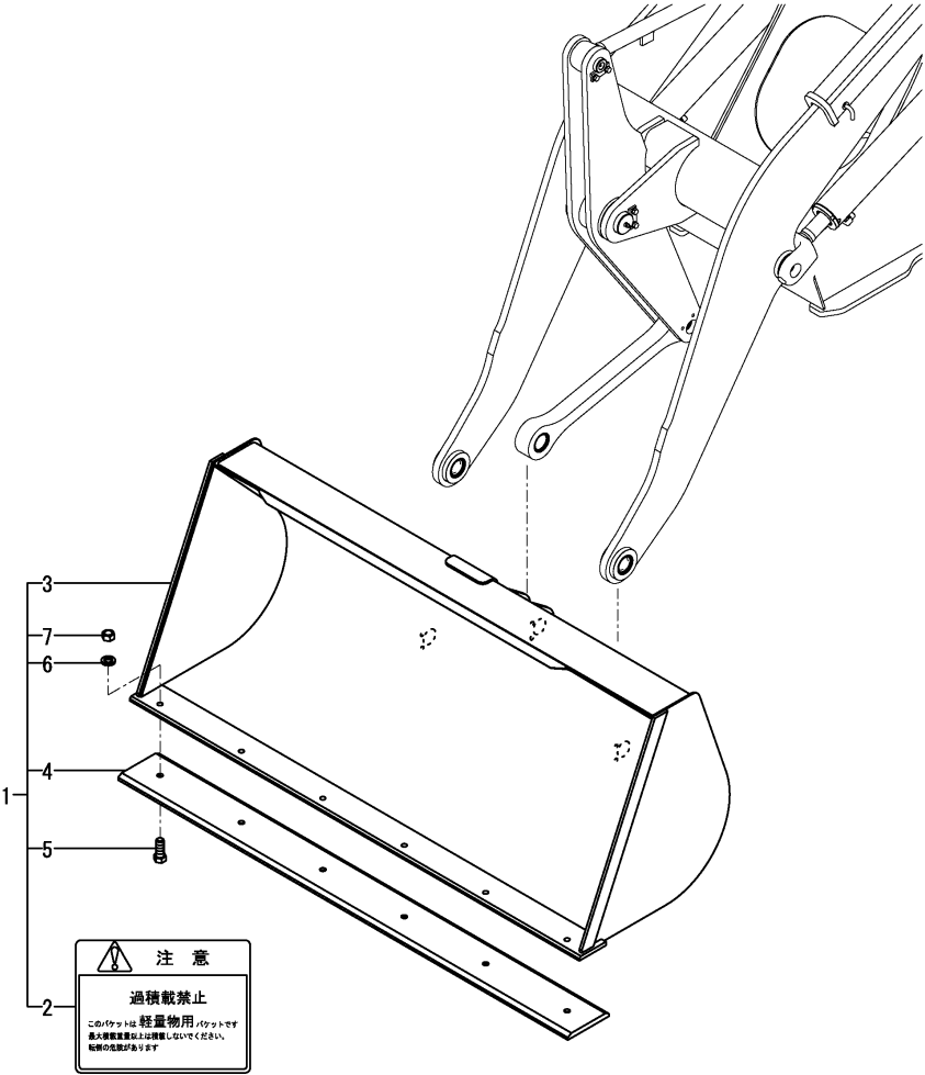
0CK20-M36003 V3/V4-5(A),V5(-A)(JP) Fig.119. BUCKET(0.8)KIT(OPTIONAL)
