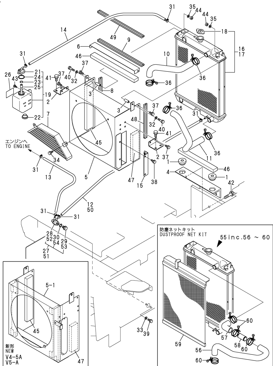
Fig.12. RADIATOR(2)
