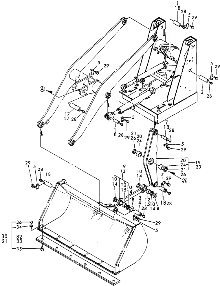
Fig.75 ローダーリンク LOADER LINK
