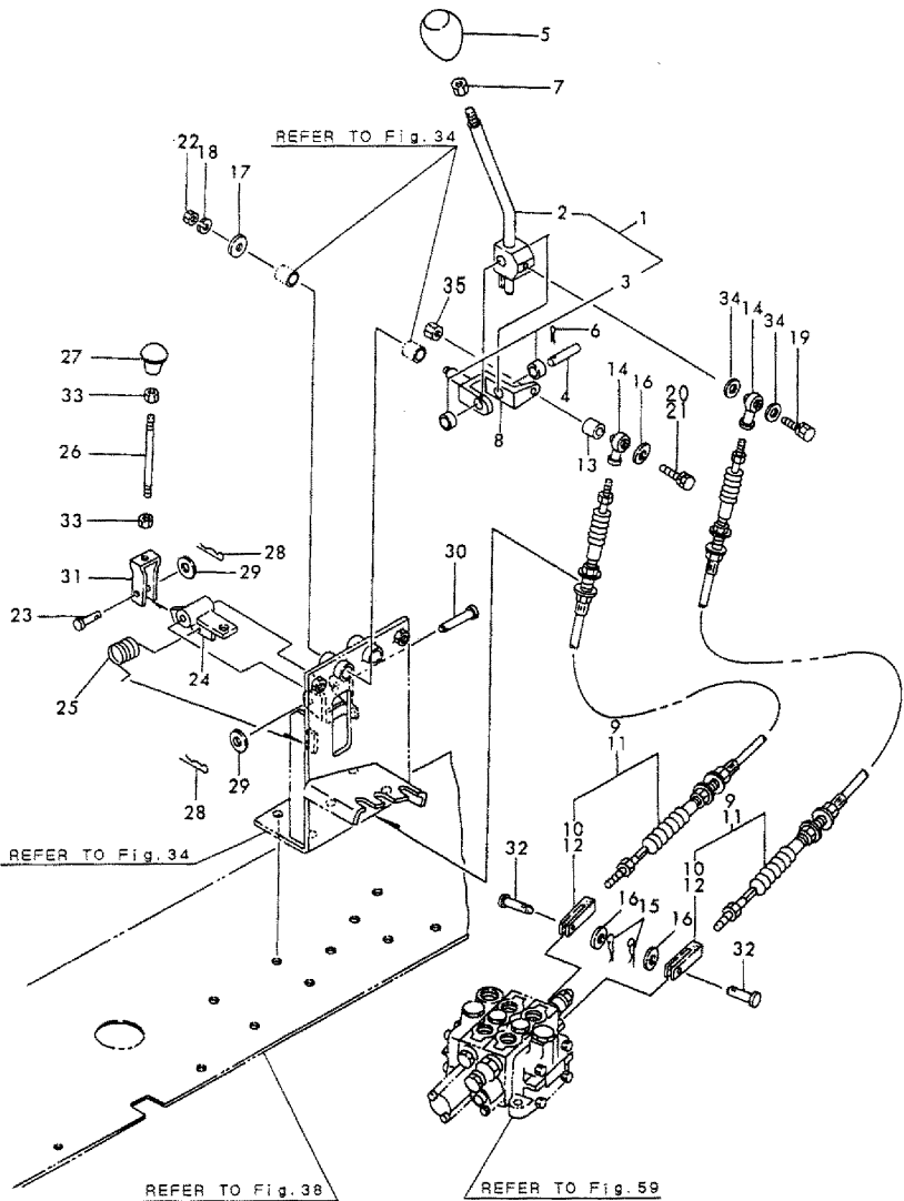
Fig.31 油圧コントロールレバー HYDRAULIC OIL CONTROL LEVER
