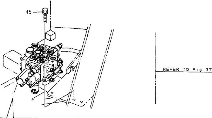
Fig.62 コントロールバルブ (オートレベラー, キャリーオーバー) CONTROL VALVE (AUTO LEVELLER, CARRY OVER)
