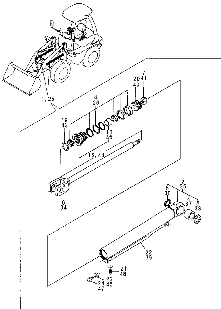
Fig. 51 リフトシリンダ LIFT CYLINDER
