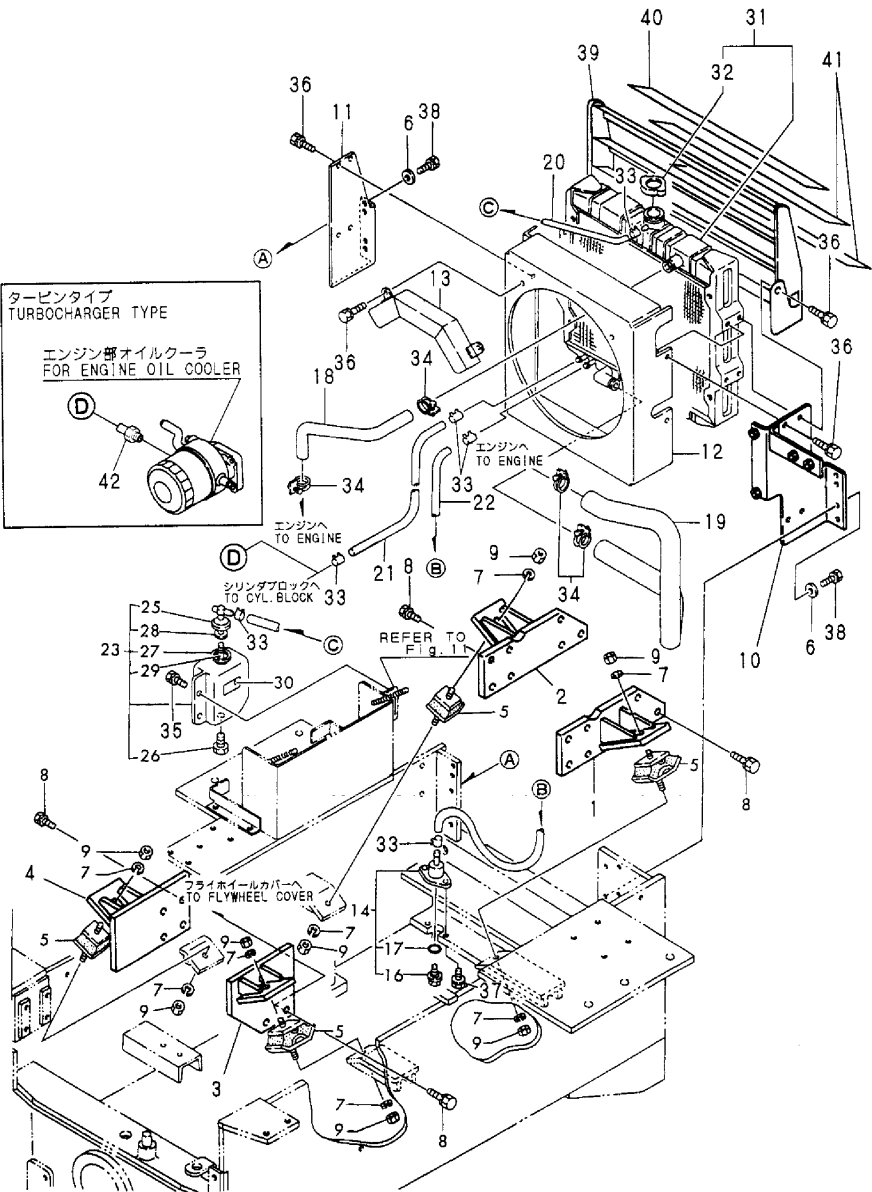
Fig.9 エンジンマウント&ラジエータ ENGINE MOUNT & RADIATOR
