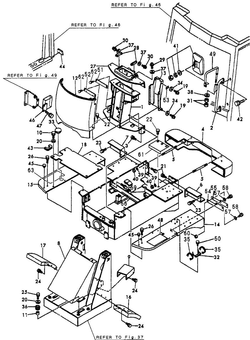
Fig.39 カバー&計器板 (キャビン) COVER & INSTRUMENT PANEL (CABIN)
