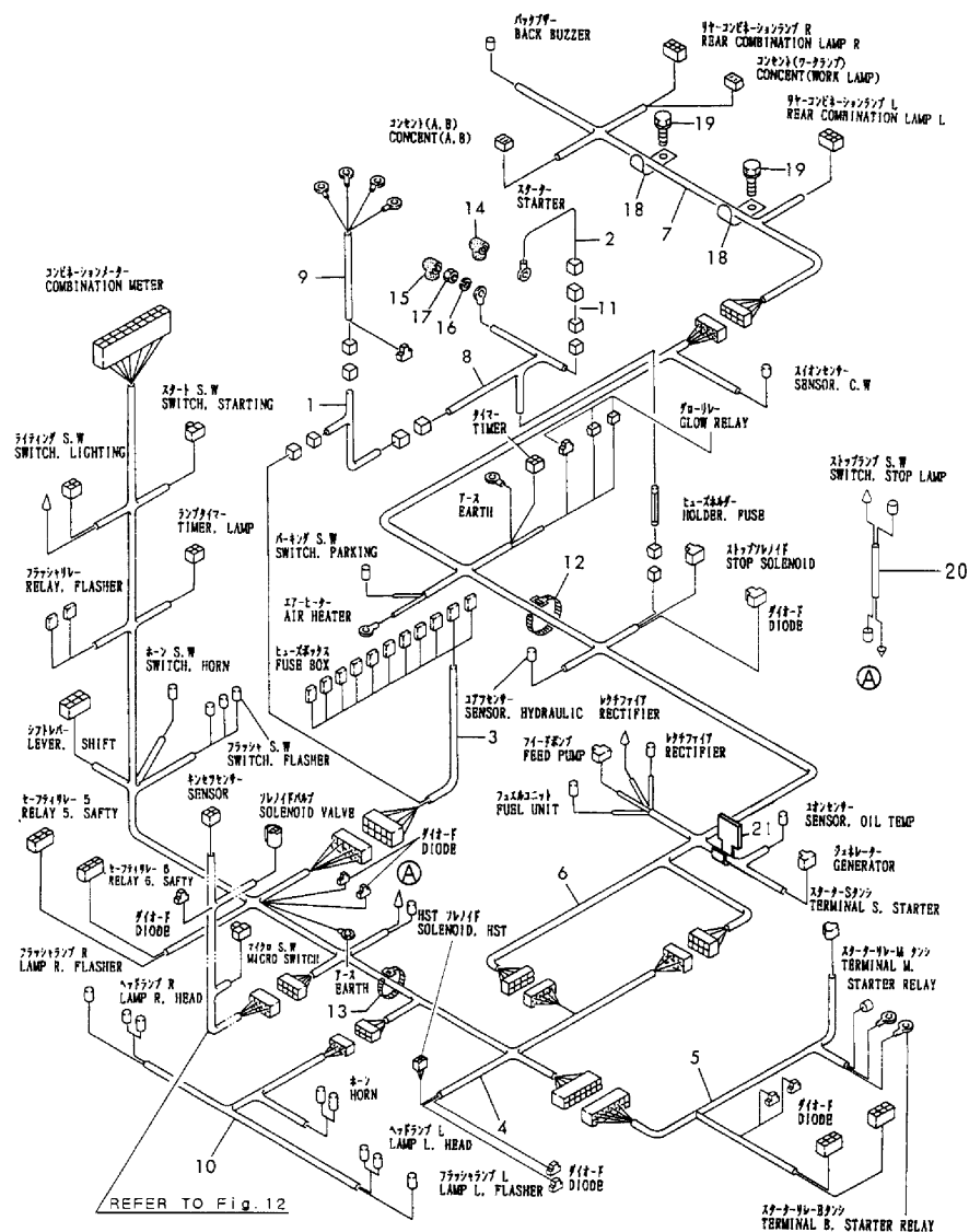
Fig. 13 ワイヤリング WIRING
