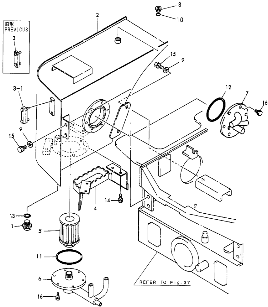
Fig.67 作動油タンク HYDRAULIC OIL TANK
