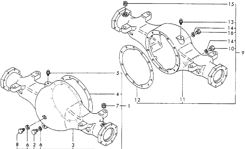
Fig.23 アクスルケース AXLE CASE
