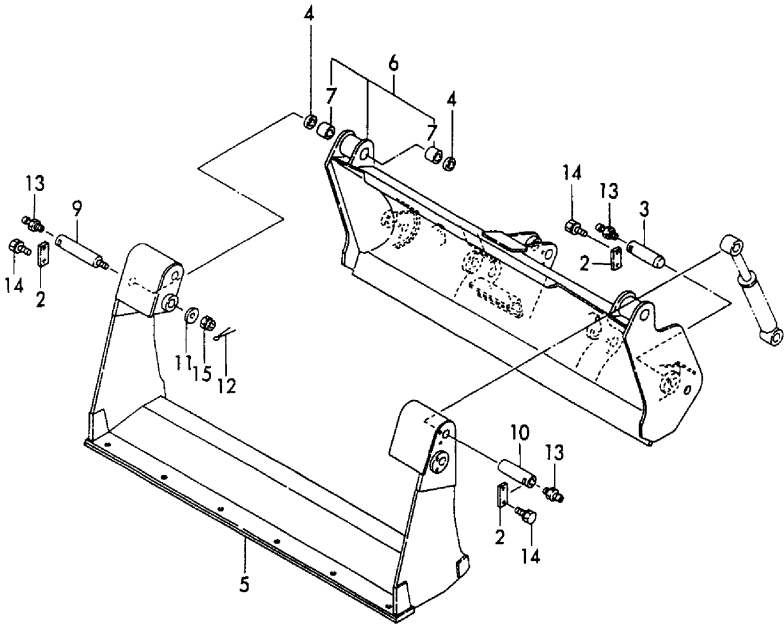
Fig.79 バケット (マルチパーパス) BUCKET (MULTIPURPOSE)
