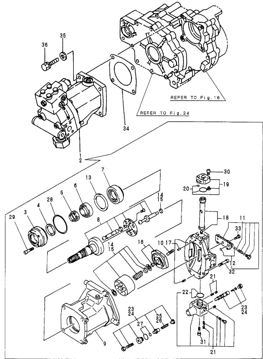
Fig.57 油圧モータ HST MOTOR
