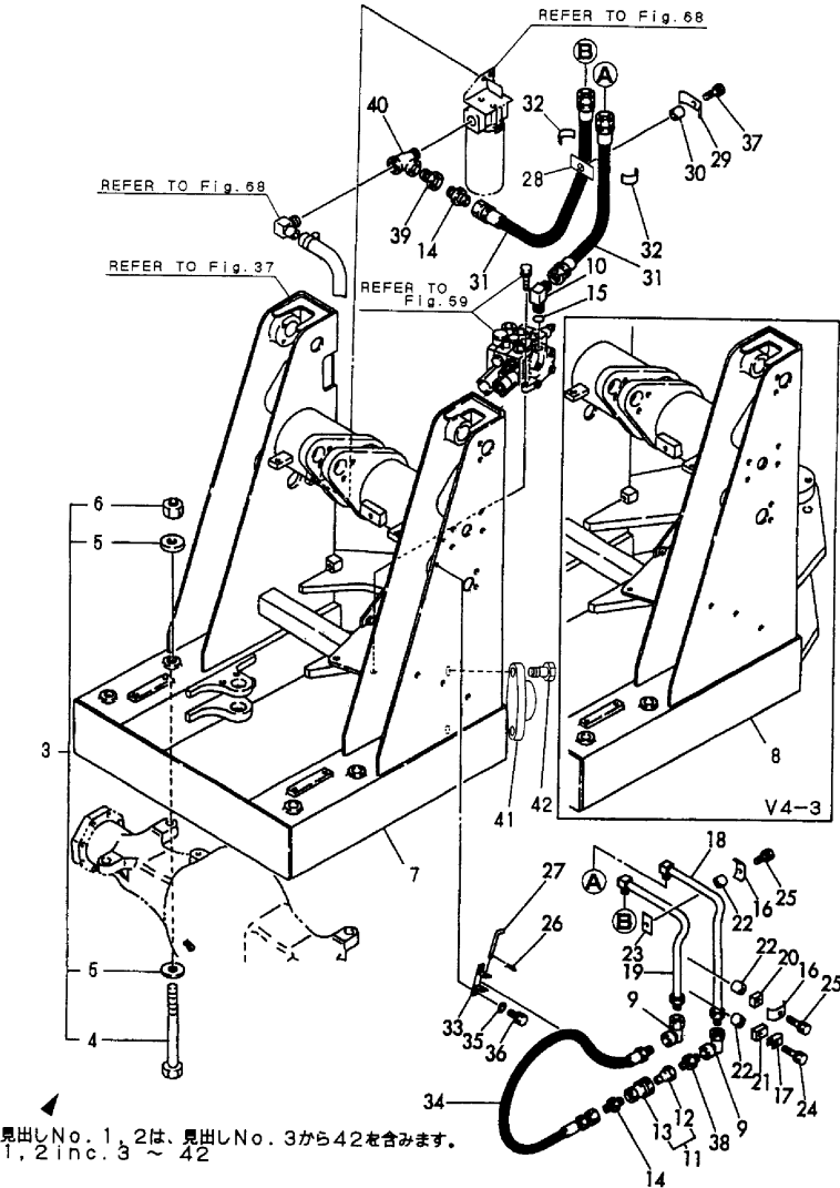
Fig.71 フロントフレーム&油圧配管 (FPTO) FRONT FRAME & HYD.OIL PIPING (FPTO)
