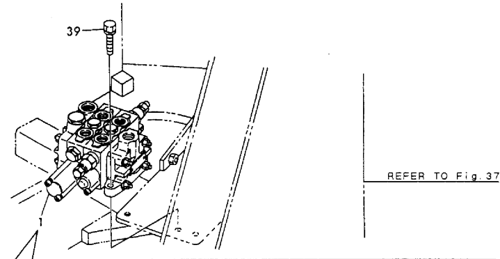
Fig. 61 コントロールバルブ (キャリーオーバー) CONTROL VALVE (CARRY OVER)
