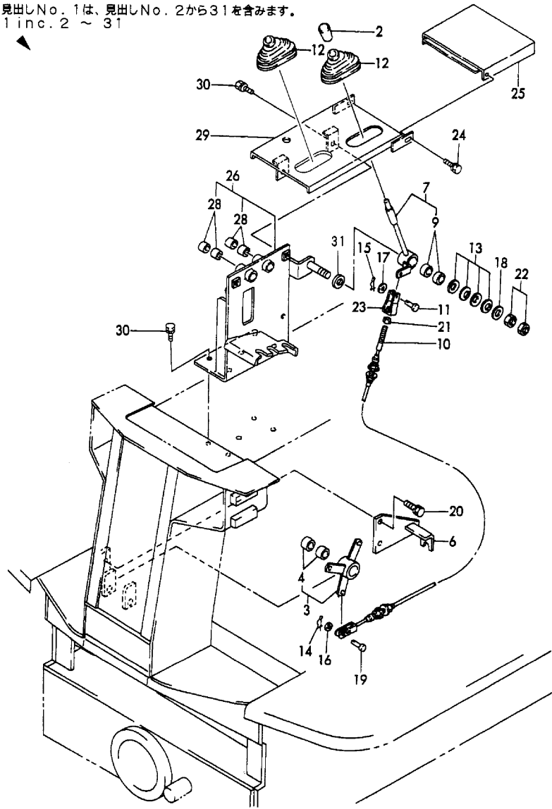
Fig.35 アクセルレバー (リヤPTO) ACCELE LEVER (REAR P. T. O.)
