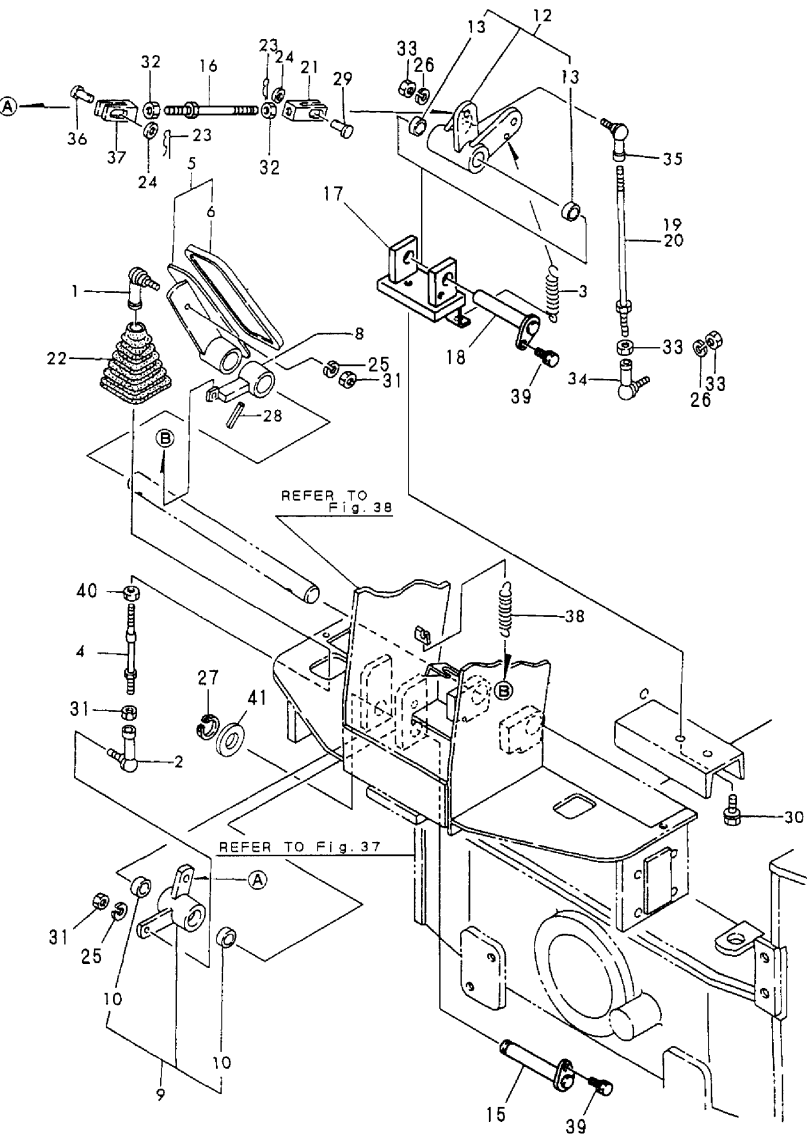
Fig.29 ブレーキペダル BRAKE PEDAL
