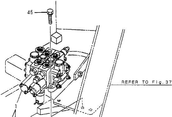
Fig.60 コントロールバルブ (オートレベラー) CONTROL VALVE (AUTO LEVELLER)
