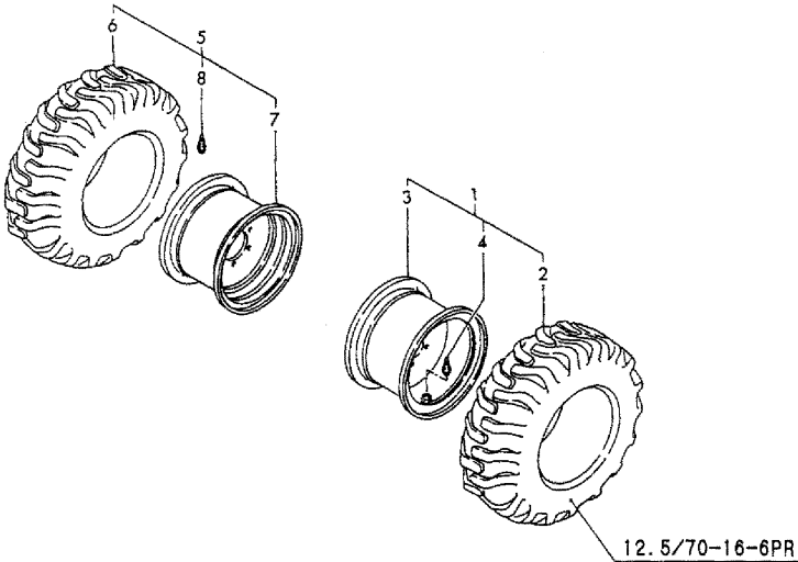
Fig.26 タイヤ&ディスク TIRE & DISK
