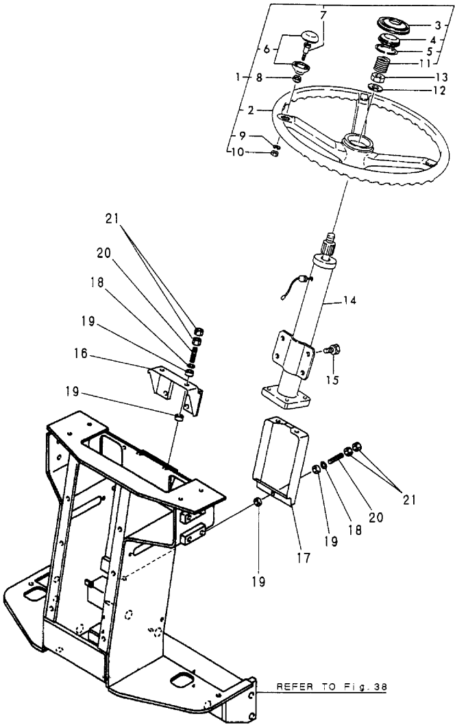
Fig.33 ステアリング&コラム STEERING WHEEL & COLUMN
