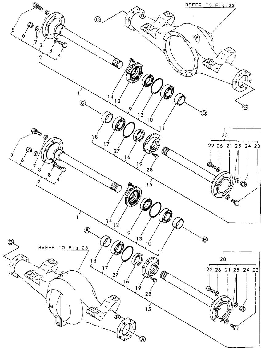
Fig.22 アクスルシャフト (V4-3) AXLE SHAFT (V4-3)
