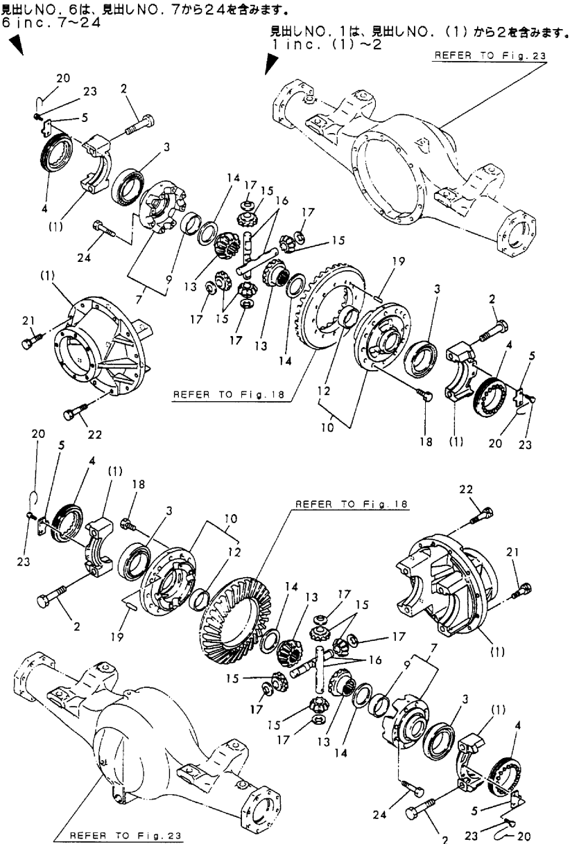
Fig.20 デファレンシャルギヤ (V4-3) DIFFERENTIAL GEAR (V4-3)
