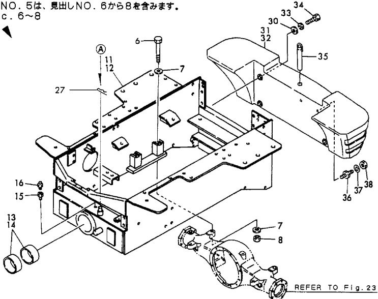
Fig.37 フレーム FRAME
