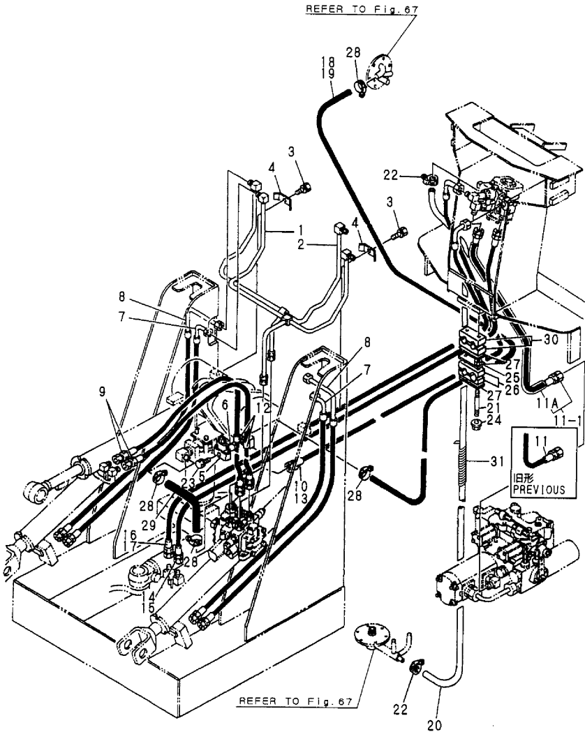
Fig. 70 油圧配管 (ローダー) HYD.OIL PIPING (LOADER)
