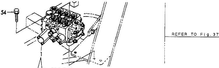
Fig.64 コントロールバルブ (3RD, キャリーオーバー) CONTROL VALVE (3RD, CARRY OVER)
