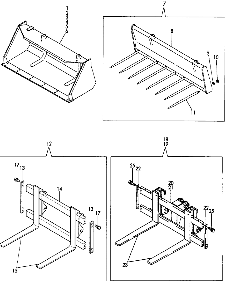
Fig.78 バケット&マニアフォーク (アタッチメント) BUCKET & MANIAFORK (ATTACHMENT)
