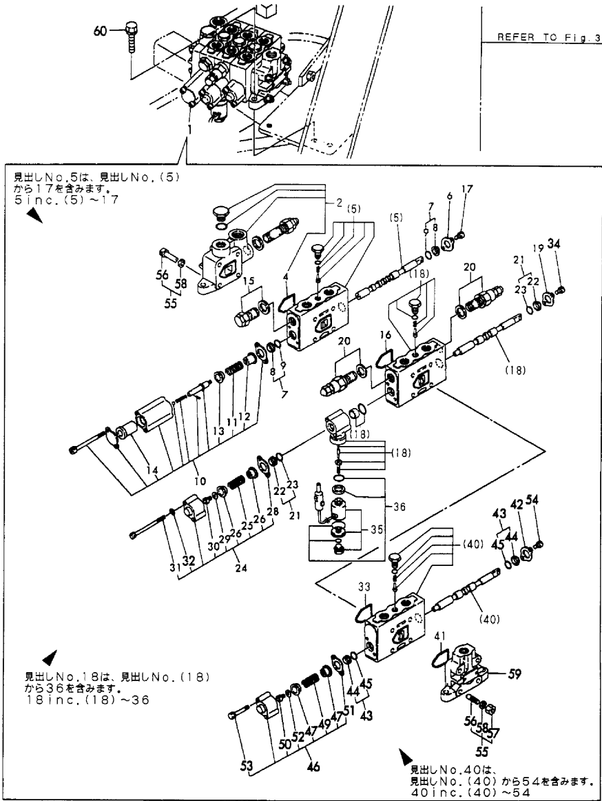
Fig.63 コントロールバルブ (3RD, オートレベラー, キャリーオーバー) CONTROL VALVE (3RD, AUTO LEVELLER, CARRY OVER)
