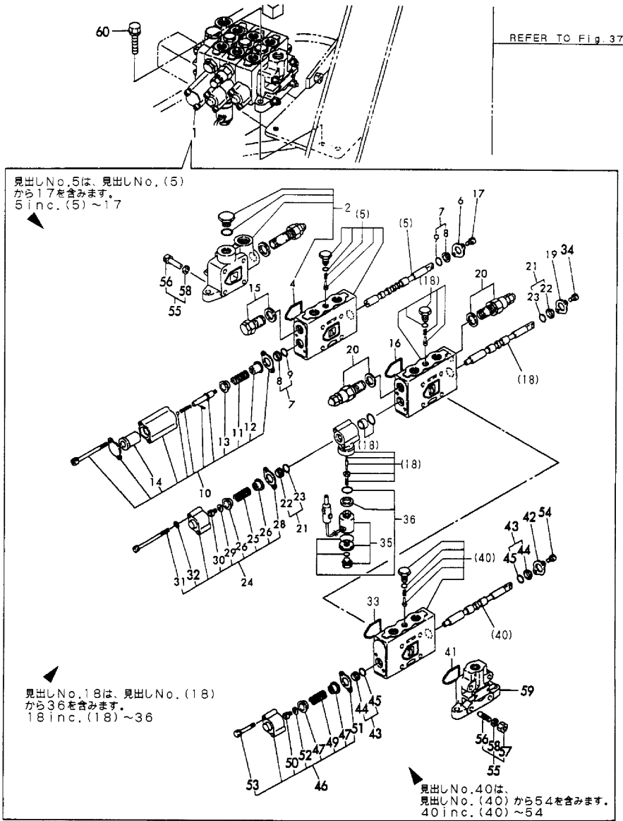
Fig.63 コントロールバルブ (3RD, オートレベラー, キャリーオーバー) CONTROL VALVE (3RD, AUTO LEVELLER, CARRY OVER)
