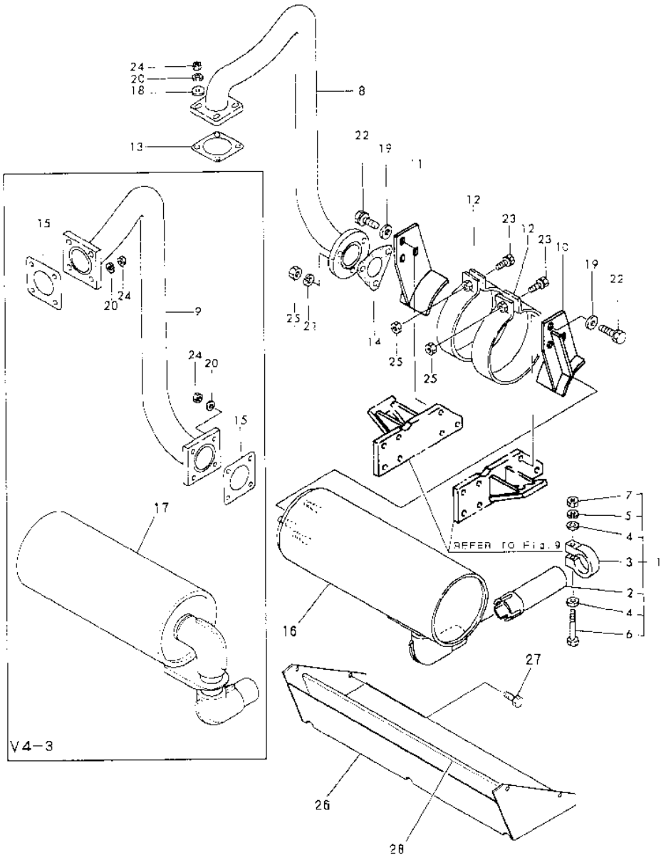
Fig.6 サイレンサ SILENCER
