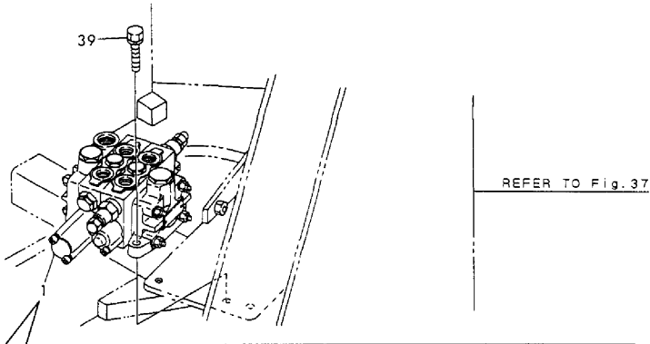
Fig.59 コントロールバルブ CONTROL VALVE
