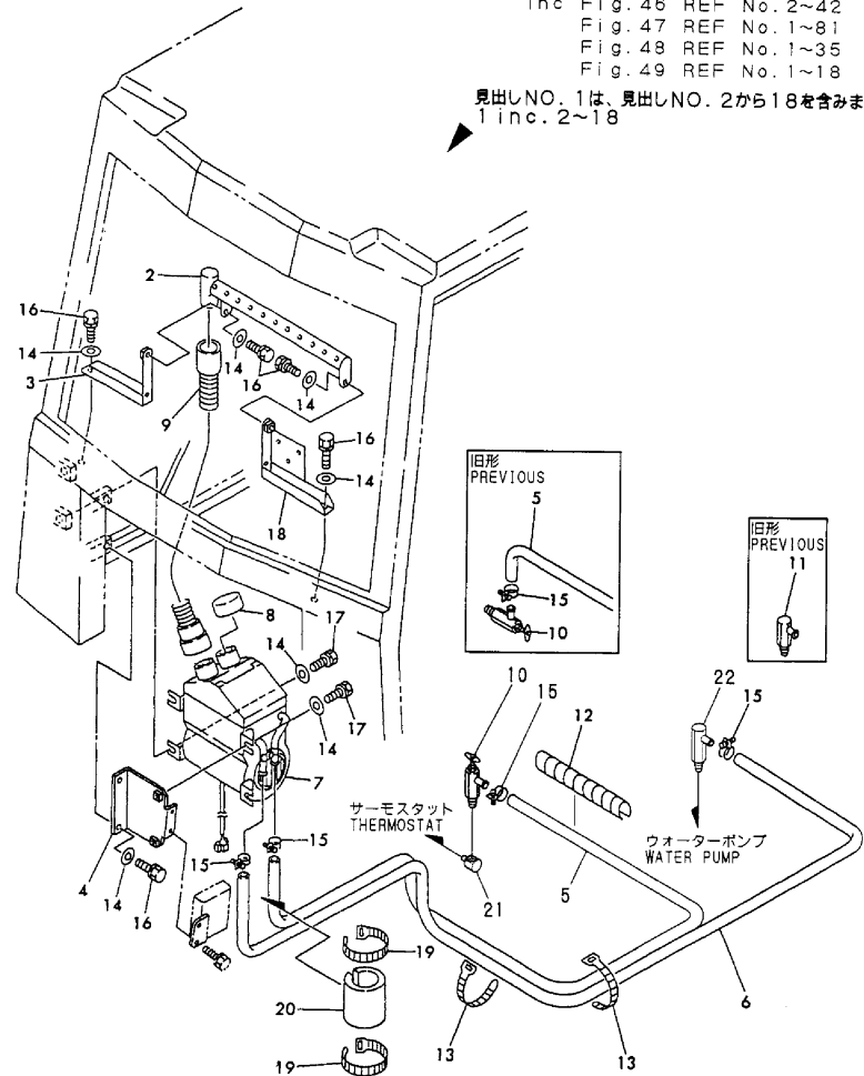
Fig.49 ヒーター&デフロスタ (キャビン) HEATER & DEFROSTER (CABIN)
