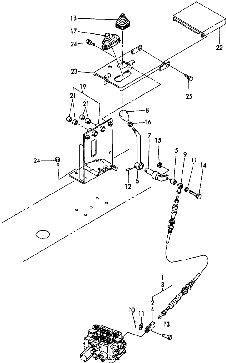
Fig.36 油圧コントロールレバー (3RD) HYDRAULIC OIL CONTROL LEVER (3RD)
