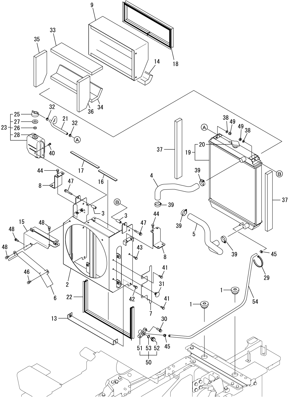
Fig.8. RADIATOR(AIR CONDITIONER SPEC.)
