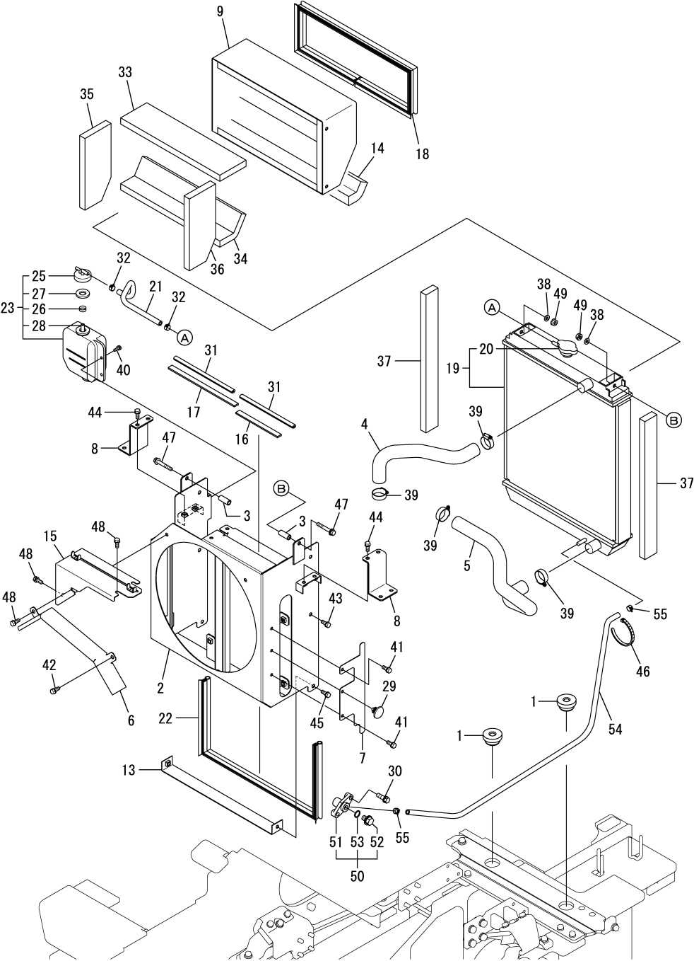
Fig.7. RADIATOR
