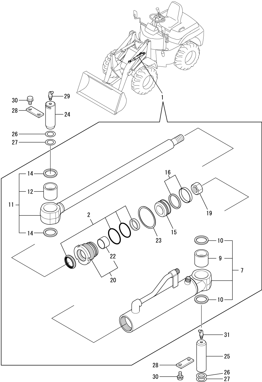
Fig.51. P.S. CYLINDER
