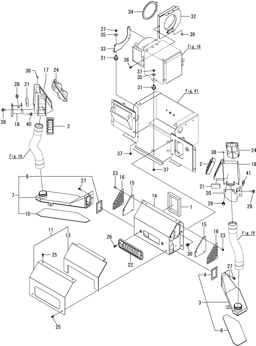
Fig.16. AIR CONDITIONER(DUCT)
