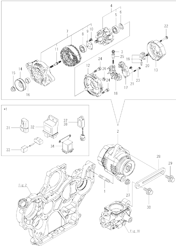
Fig.16. GENERATOR
