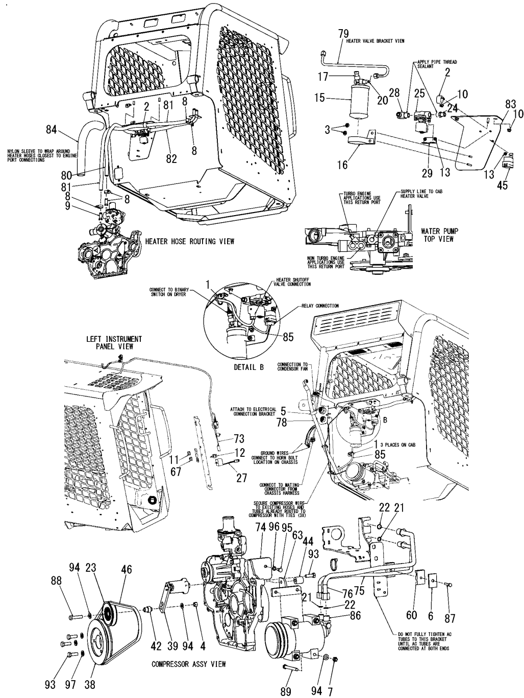
Fig.4. CHASSIS(HVAC)
