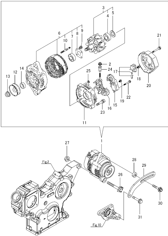
Fig.16. GENERATOR
