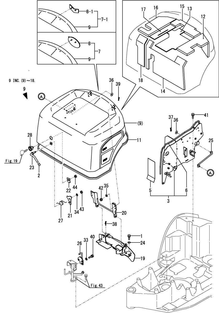
Fig.47. BONNET
