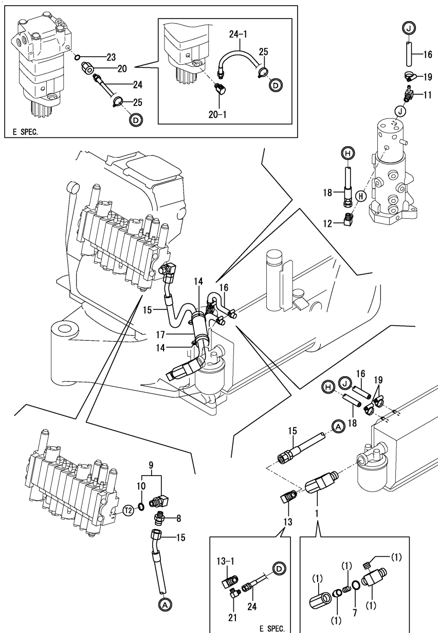
Fig.70. RETURN
