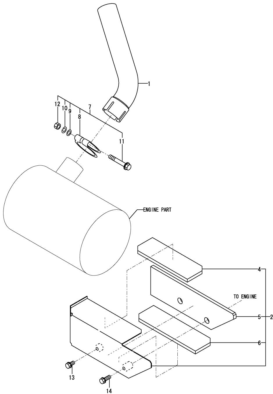
Fig.3. MUFFLER
