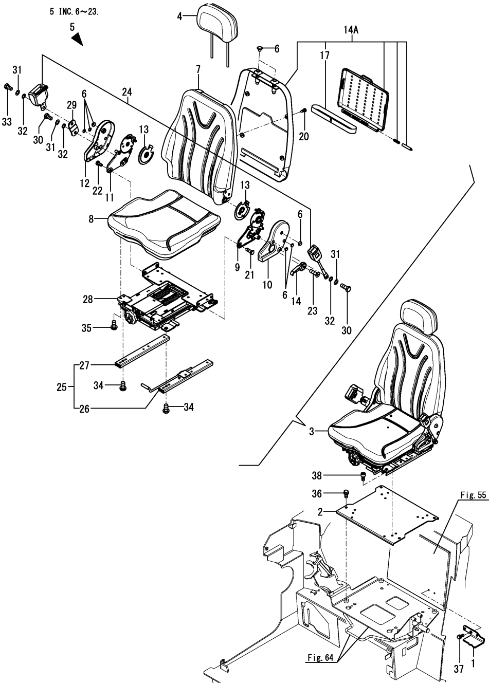
Fig.65. SEAT
