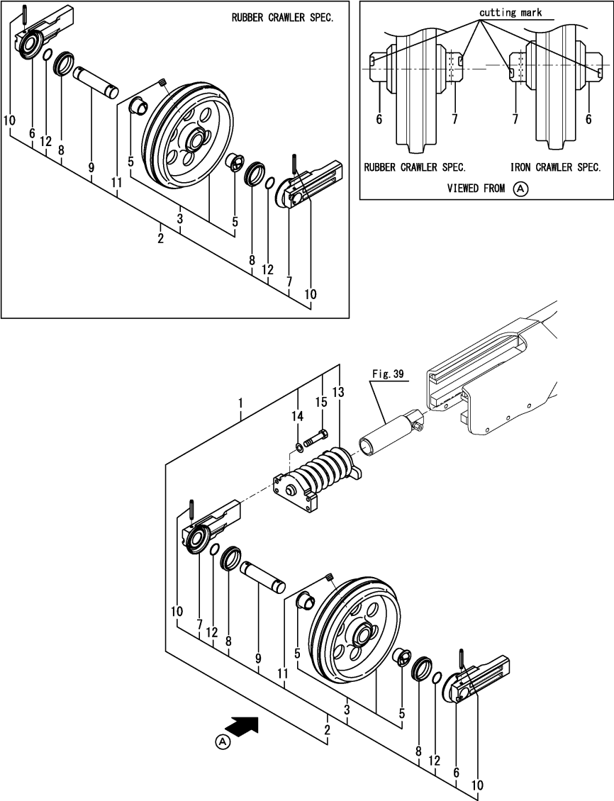
Fig.36. IDLER & ADJUST
