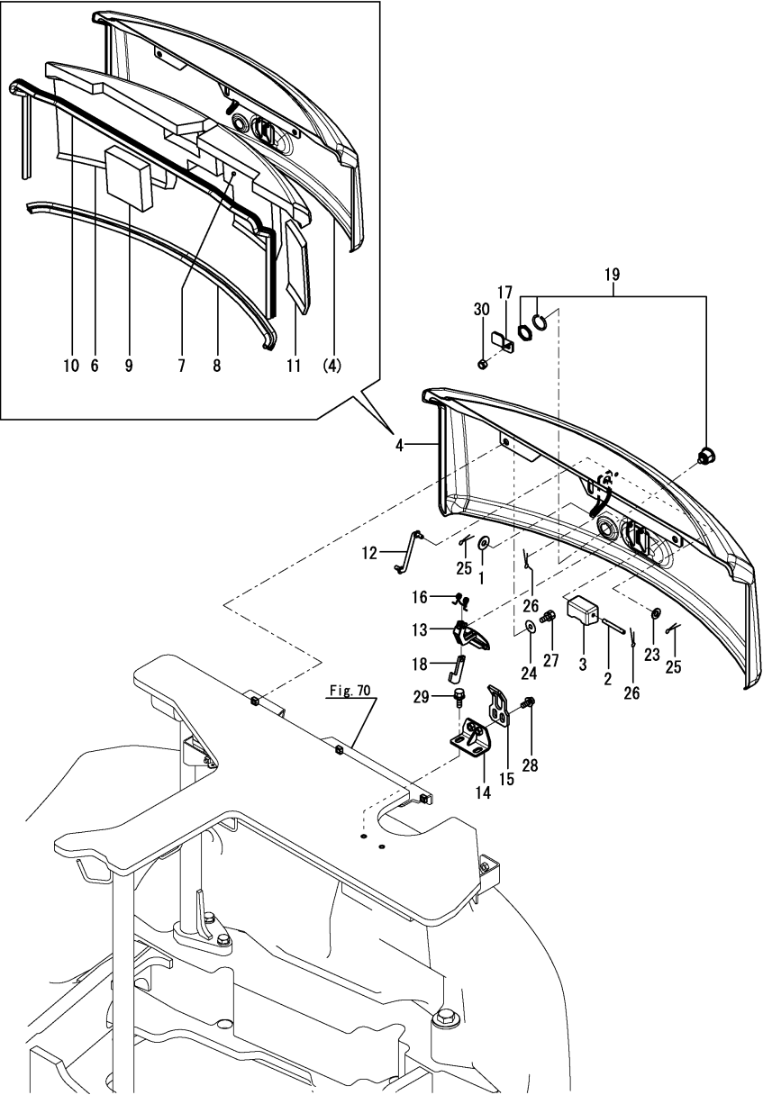
Fig.67. BONNET(REAR)
