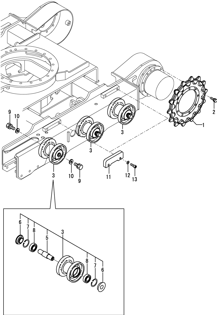
0CS10-M41801 TRAVELING Fig.16. SPROCKET & ROLLER
