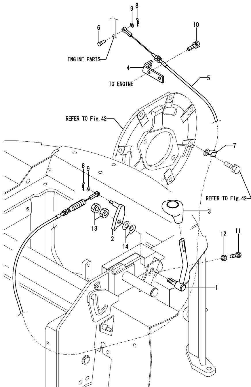
Fig.6. ACCELERATOR
