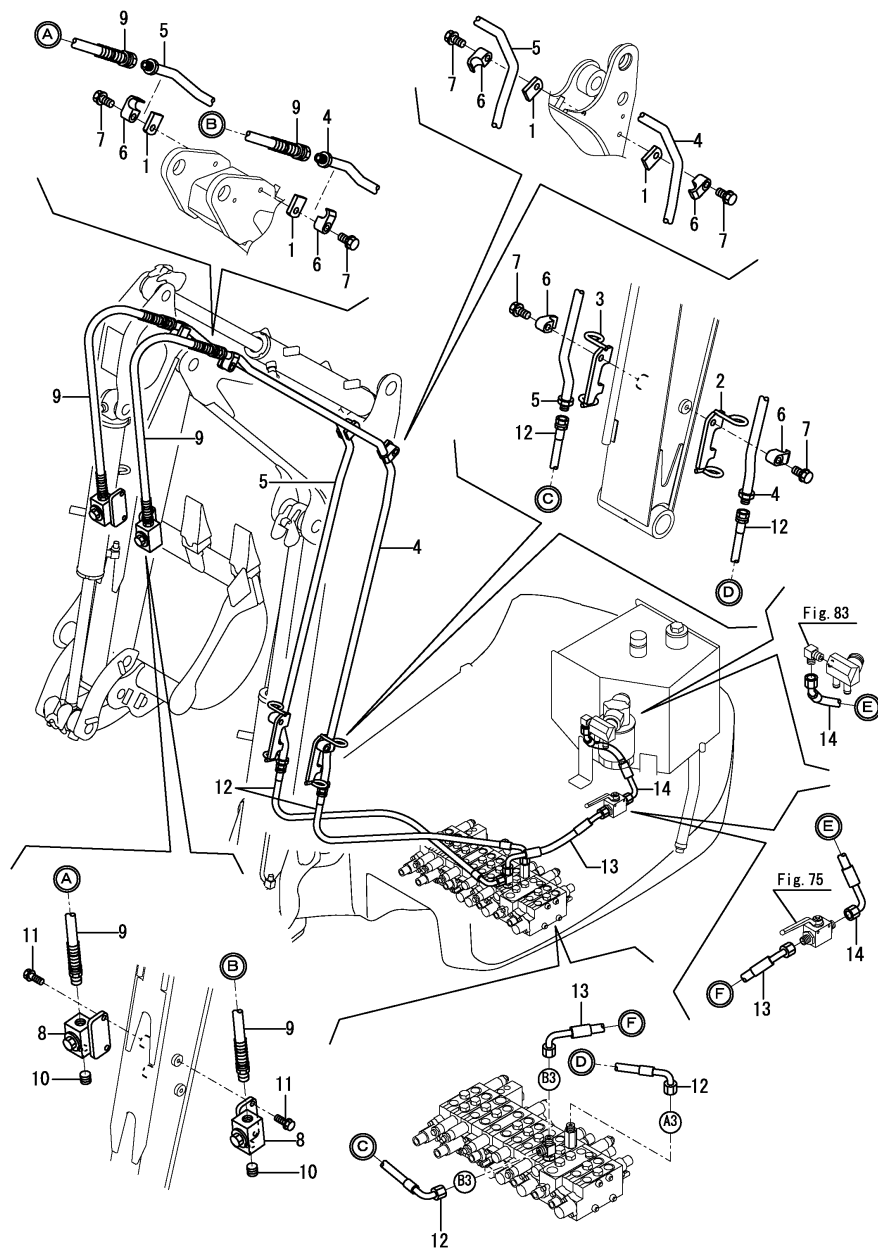
Fig.86. P.T.O.
