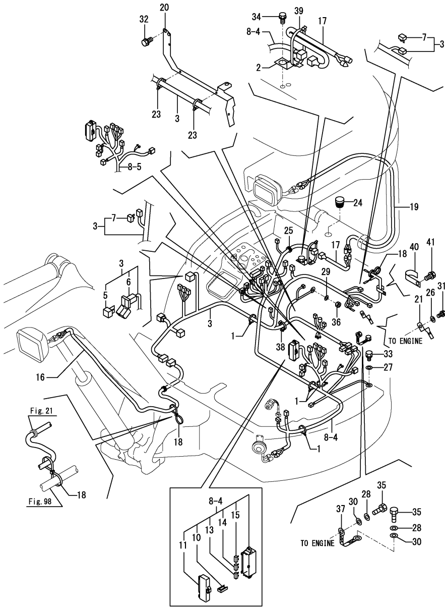
Fig.19. WIRING
