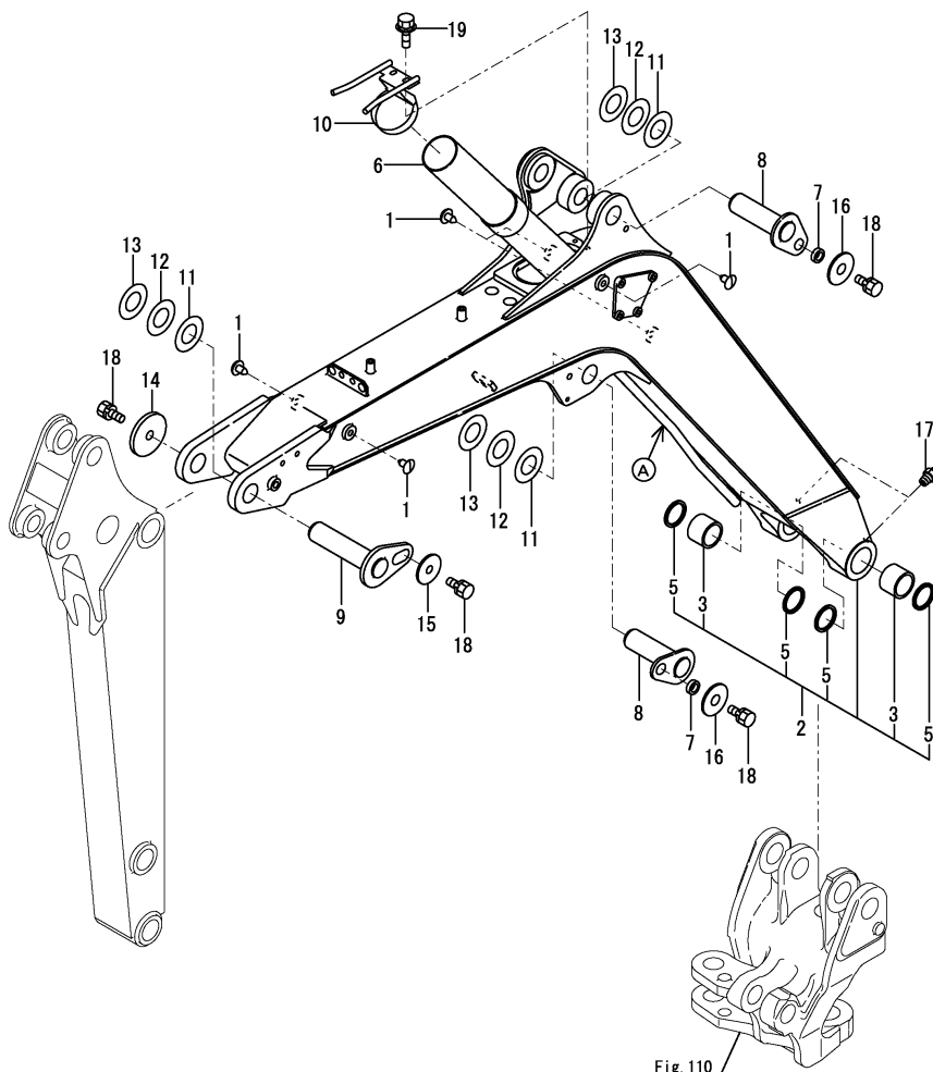
Fig. 110
