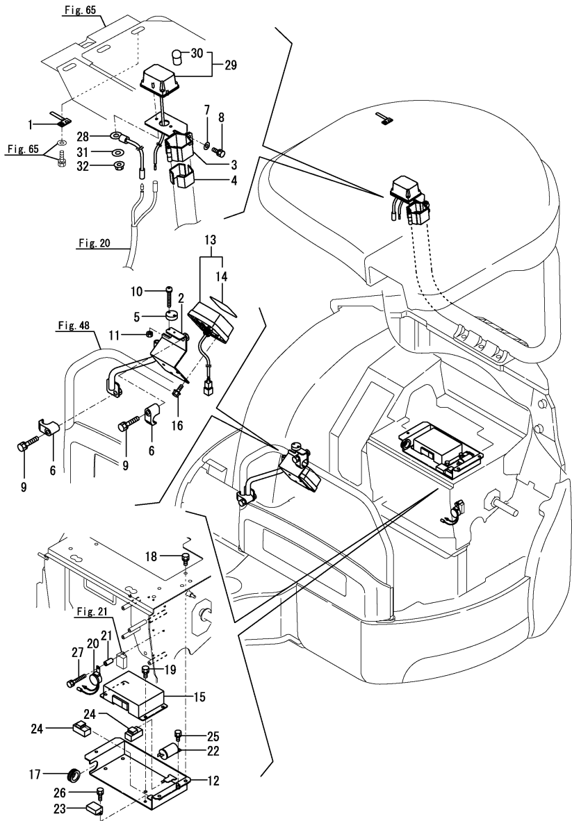
Fig.24. EQUIPMENT(CRANE)(1)
