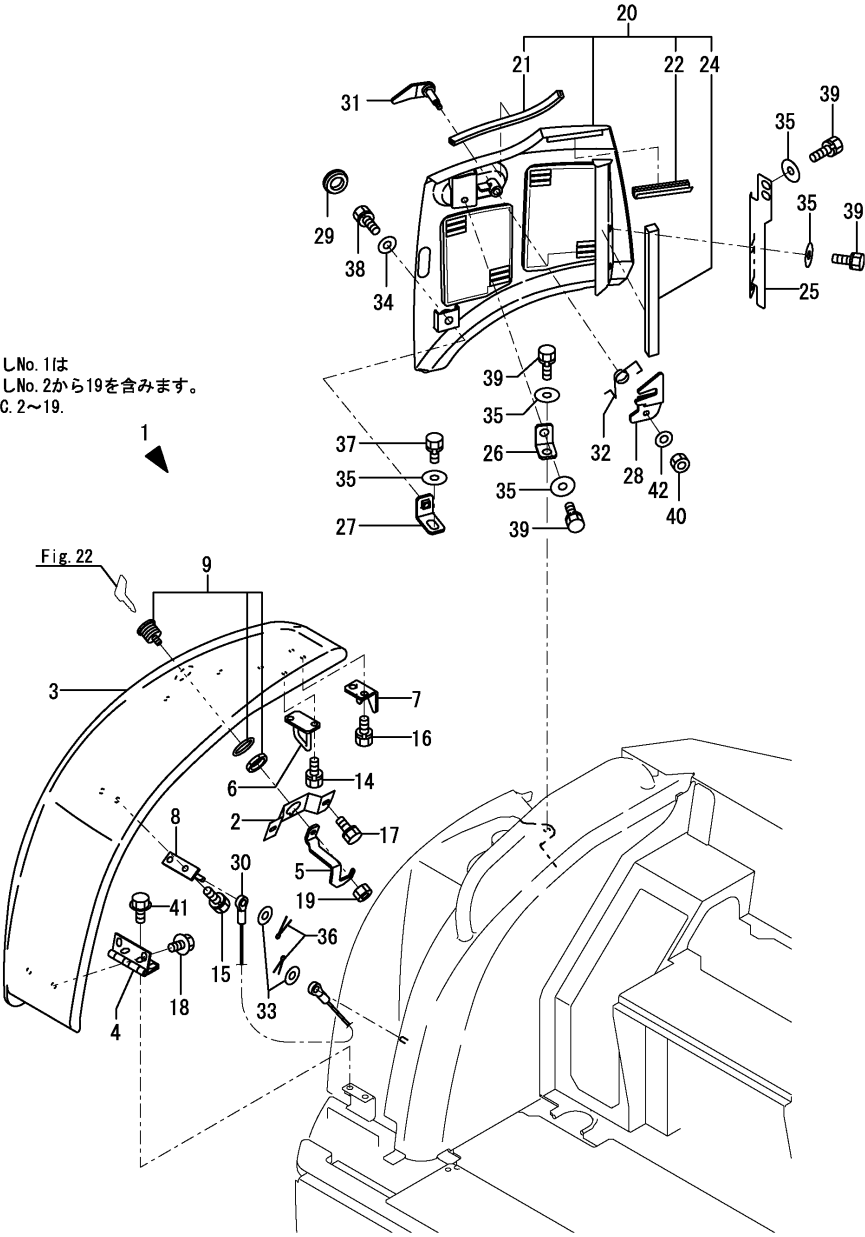
Fig.58. BONNET(2)
