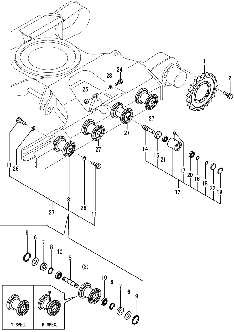
OCS10-M44901 TRAVELING Fig.23. SPROCKET & ROLLER
