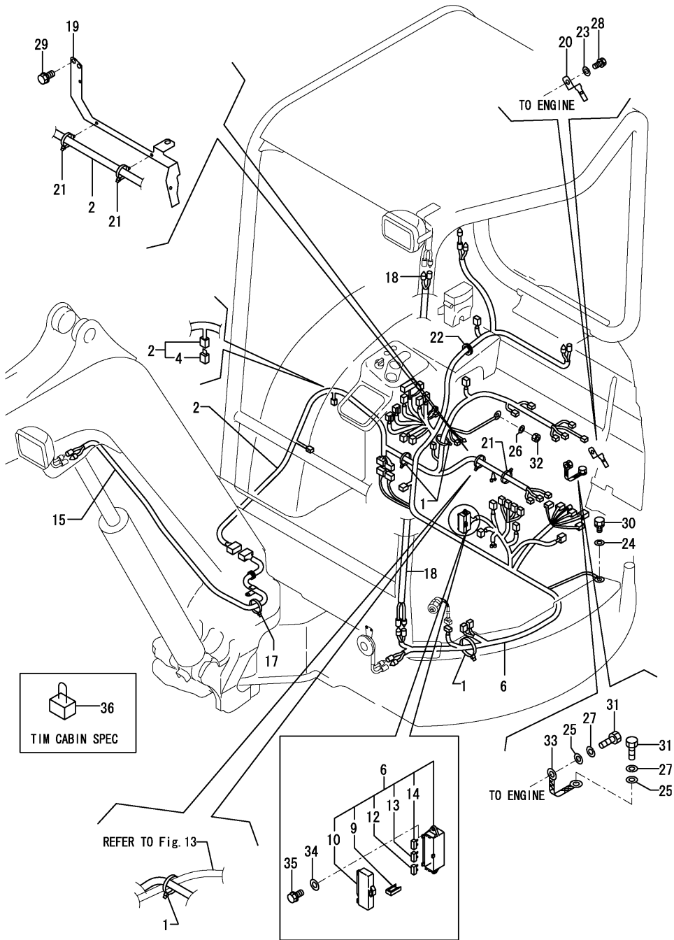
Fig.14. WIRING
