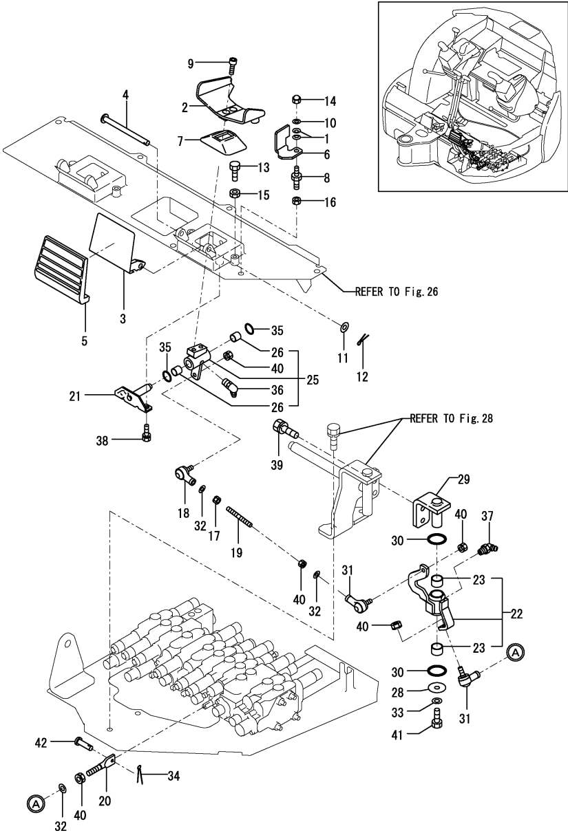
Fig.32. P.T.O. PEDAL
