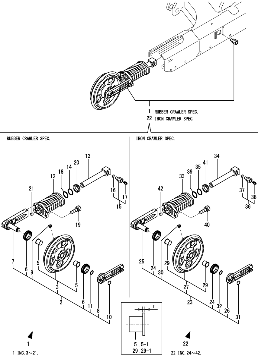
Fig.24. IDLER & ADJUST
