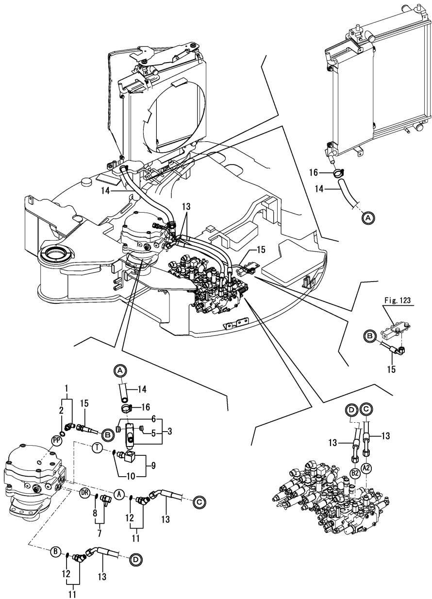
Fig.121. VÁLVULA DE CONTROLE - MOTOR DE GIRO
