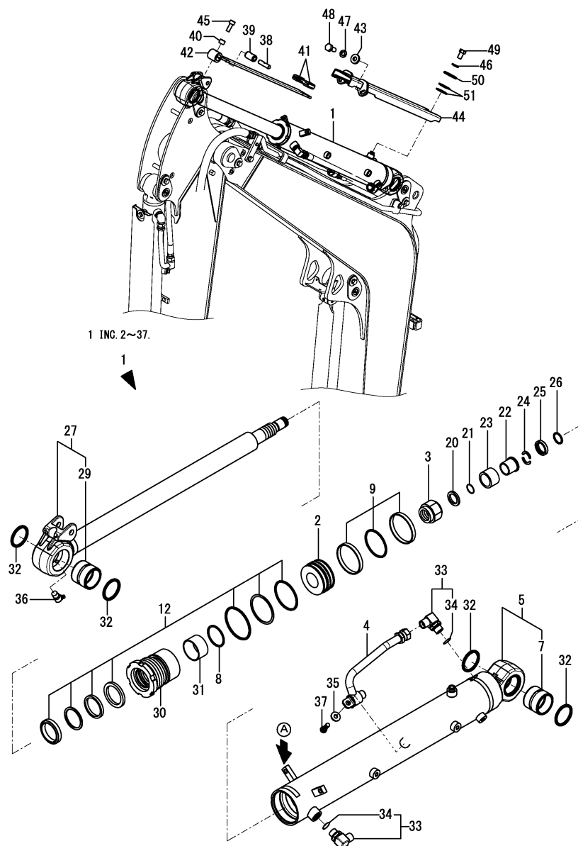
Fig.152. (100A)CILINDRO DO BRAÇO(ESPEC. K)
