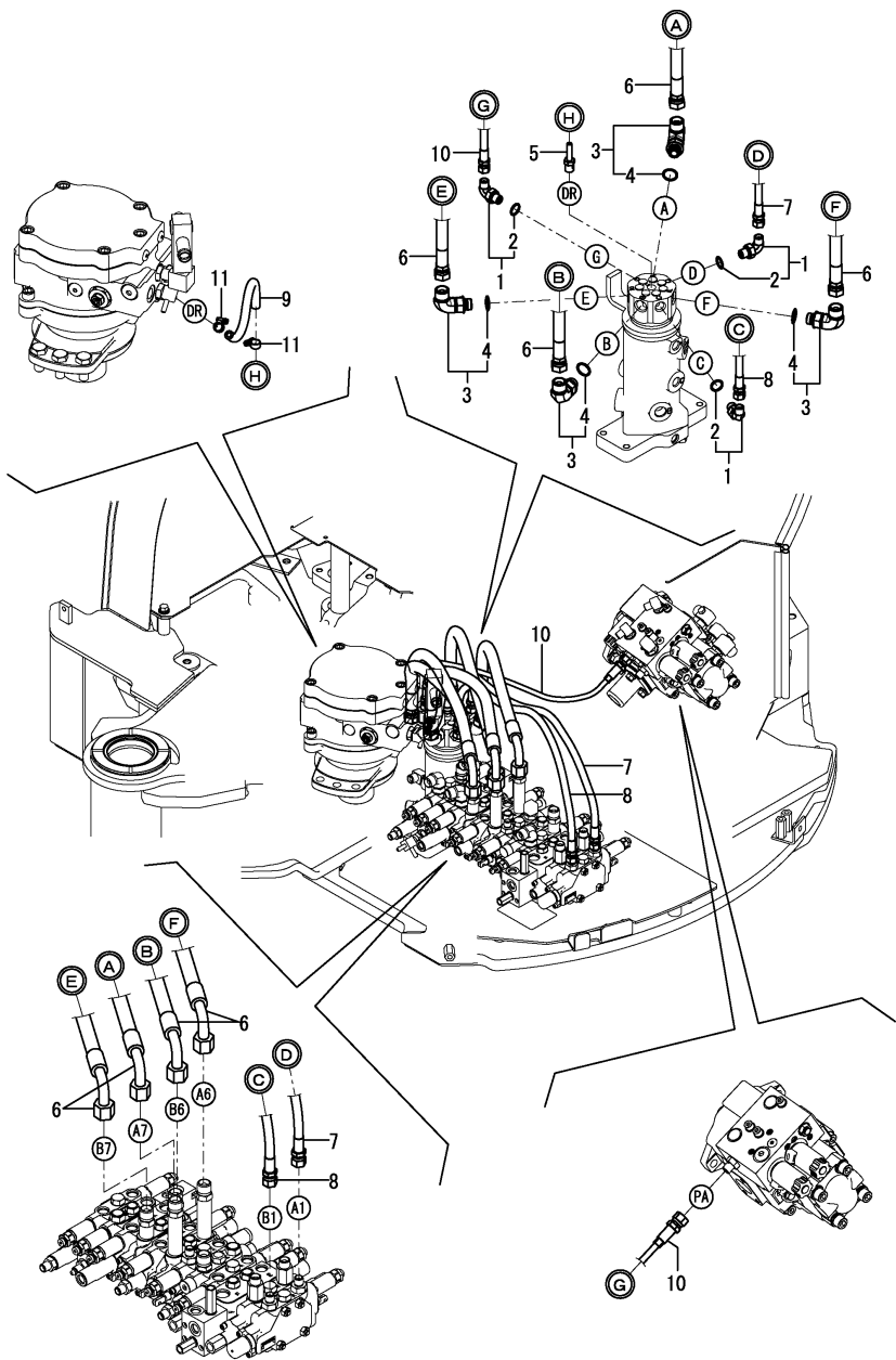
Fig.127. VÁLVULA DE CONTROLE - EIXO ROTATIVO
