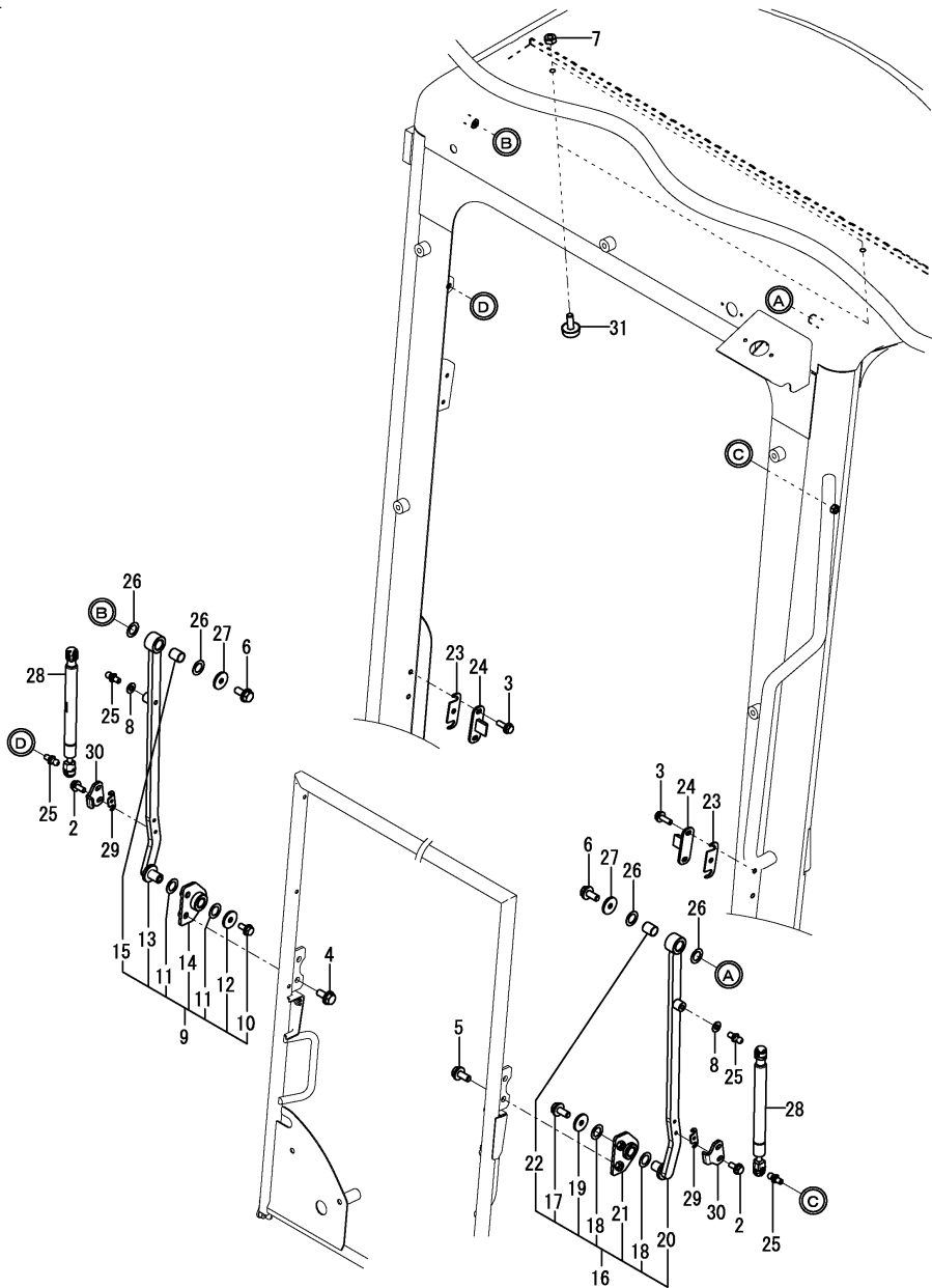
Fig.89. CABINE (JANELA DIANTEIRA)(1)
