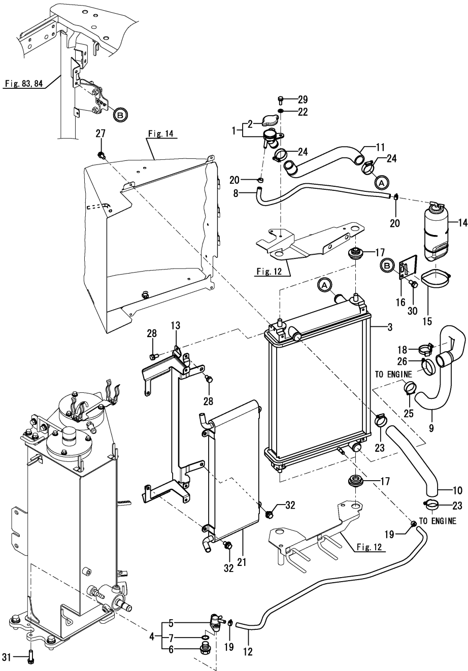
Fig.13. RADIADOR E RESFRIADOR DE ÓLEO
