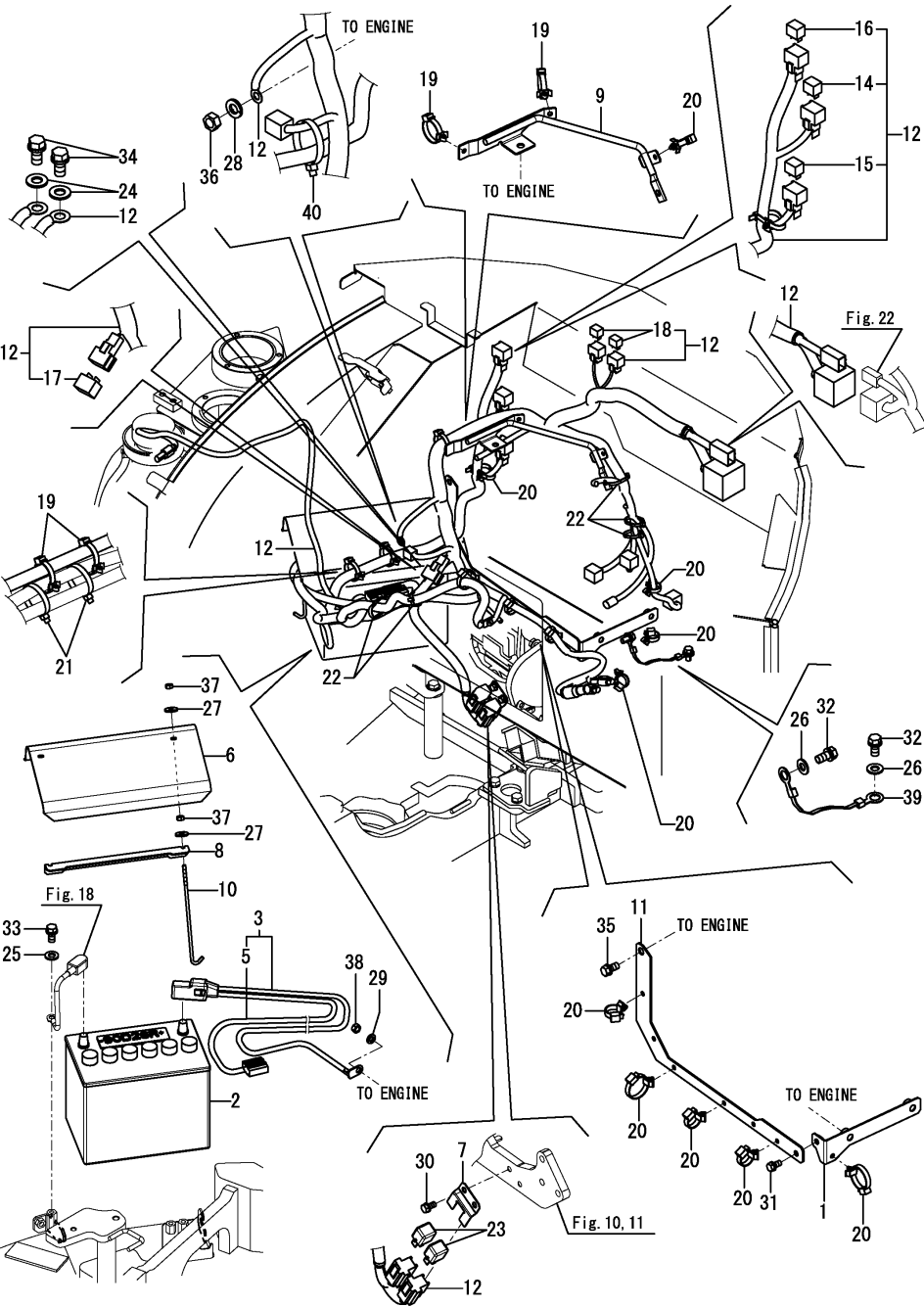
Fig.17. EM TORNO DO MOTOR
