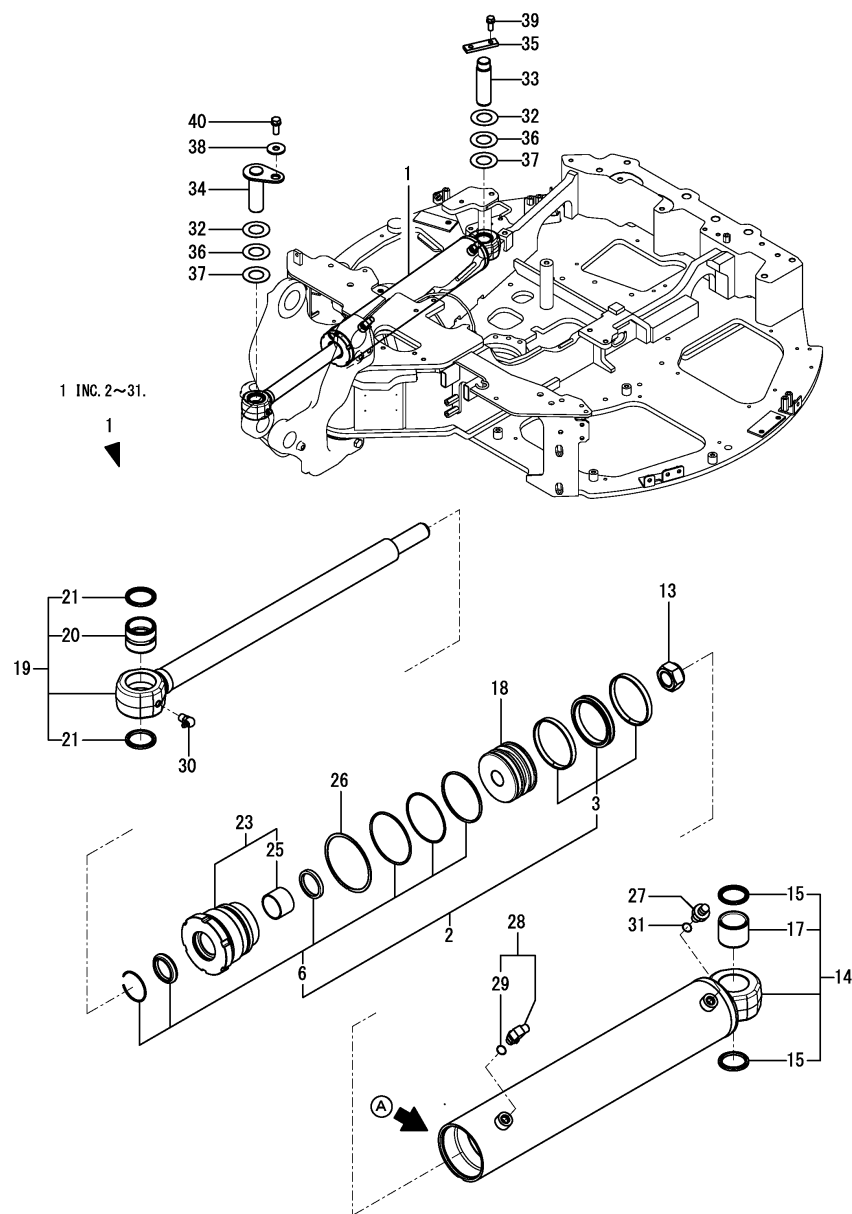
Fig.102. CILINDRO DE OSCILAÇÃO(ESPEC. Y)
