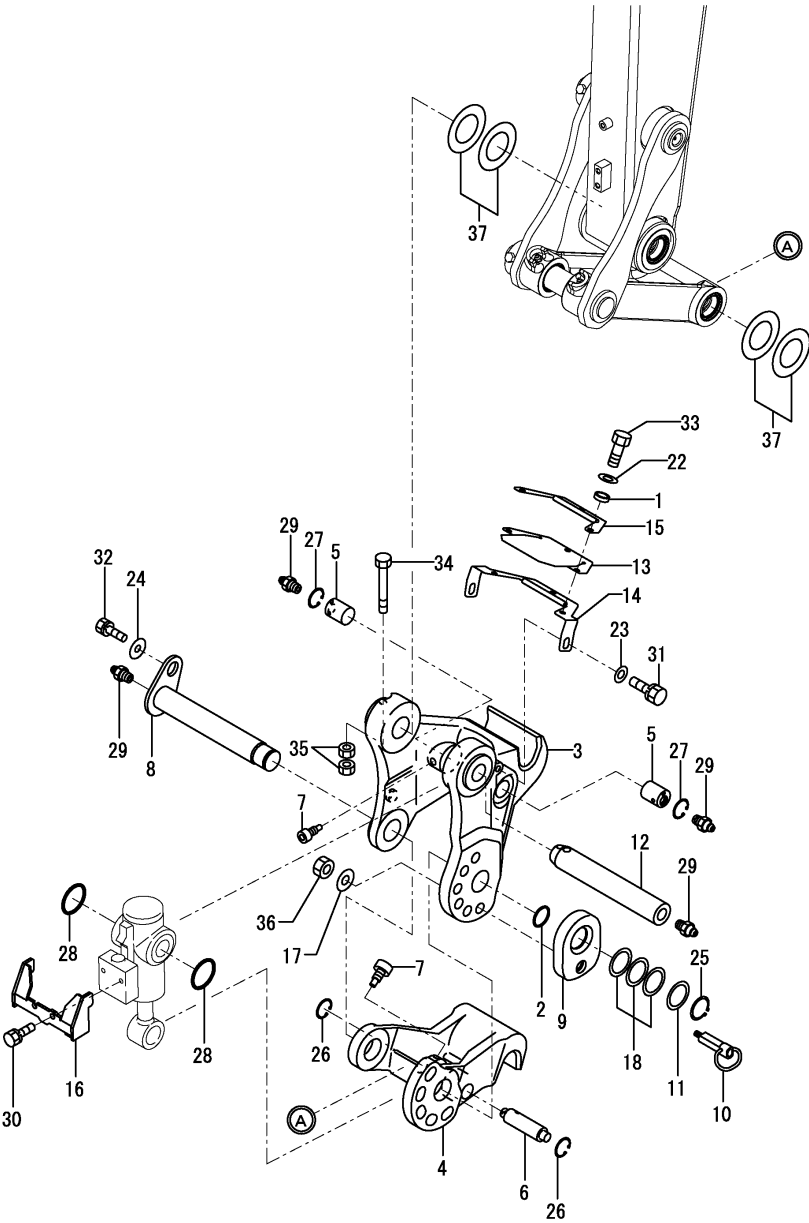
Fig.143. ENGATE RÁPIDO
