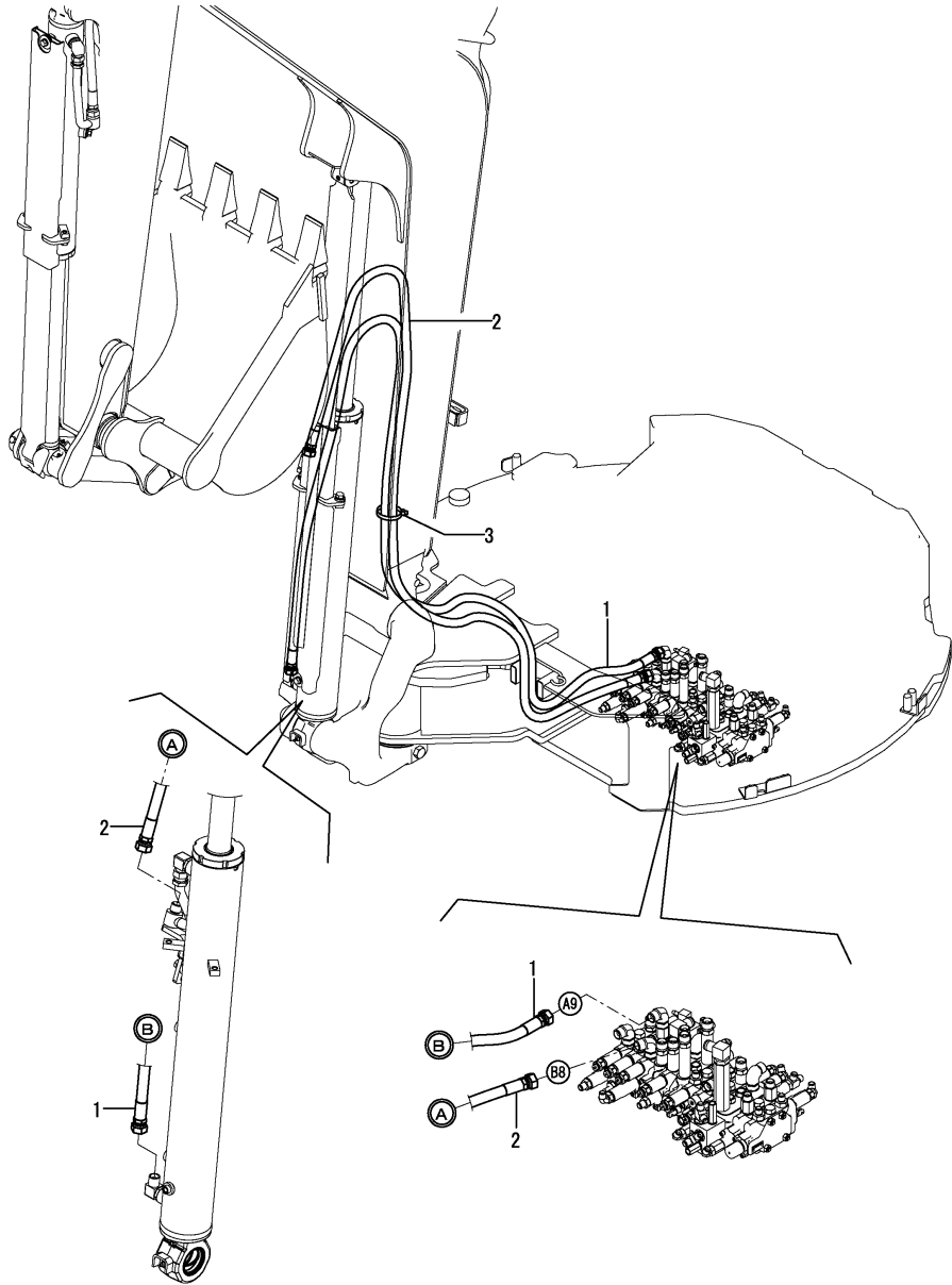
Fig.126. VÁLVULA DE CONTROLE - CILINDRO DA LANÇA
