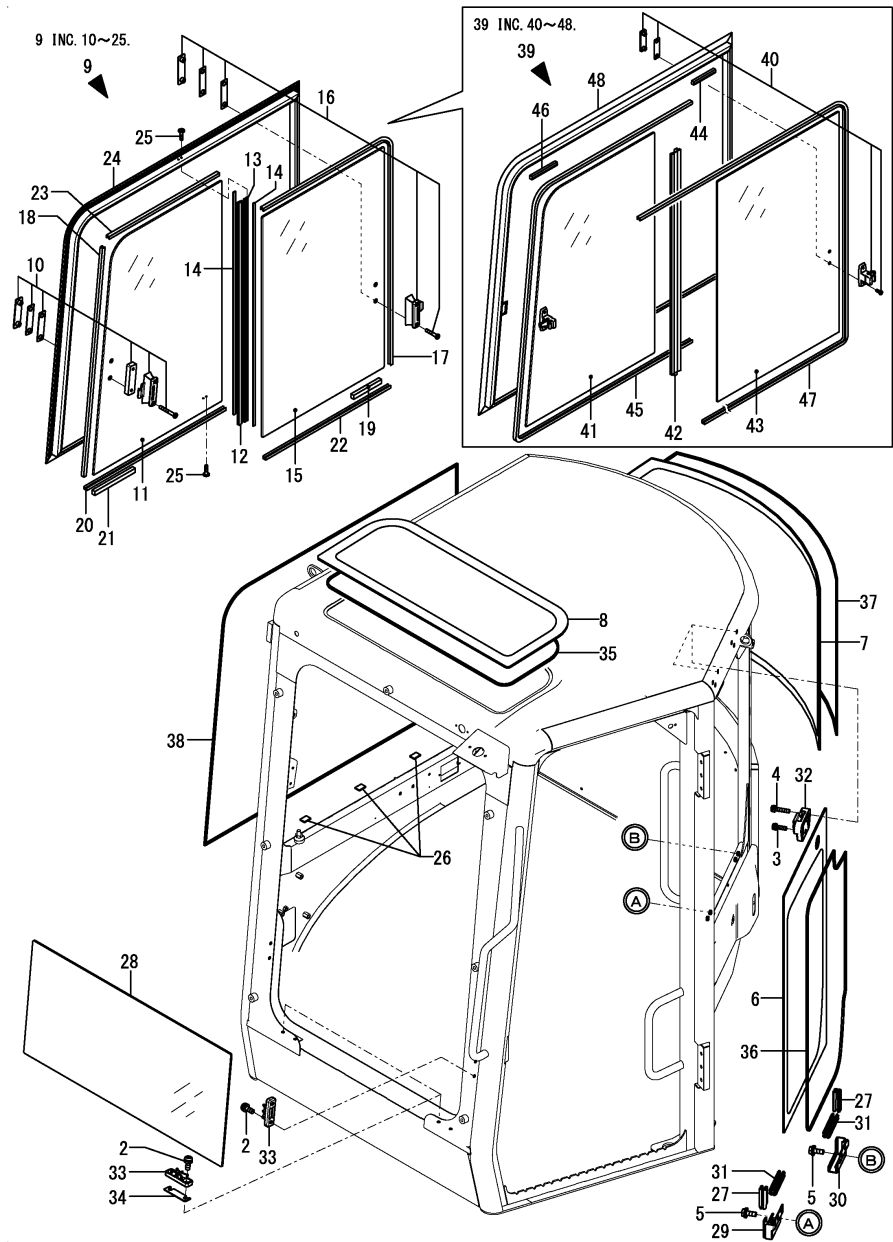
Fig.91. CABINE (VIDROS)
