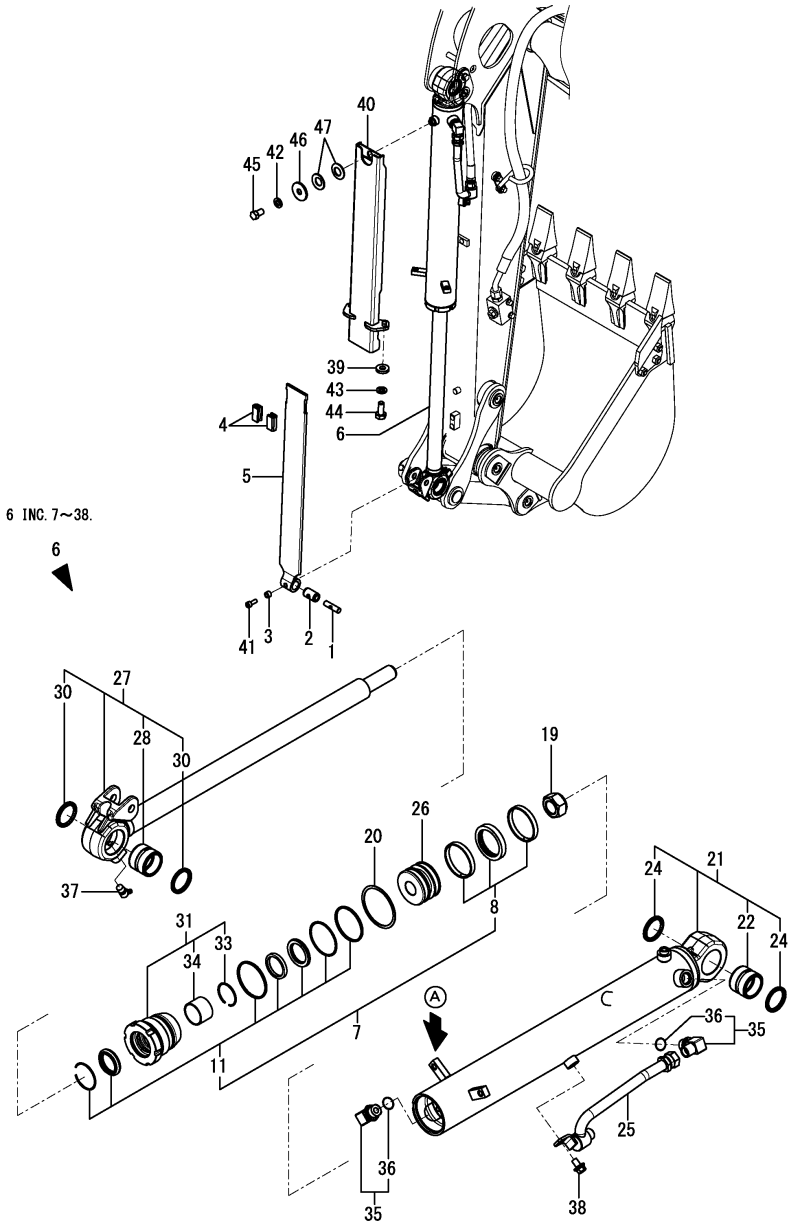
Fig.101. CILINDRO DA CAÇAMBA(ESPEC. Y)
