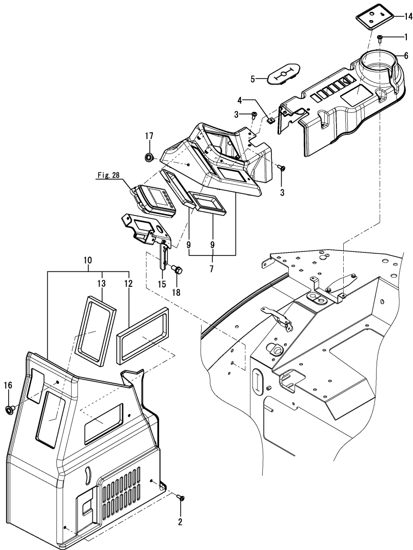
OCK50-M00170 AO REDOR DO ASSENTO Fig.69. COBERTURA (MONITOR)(CABINE)
