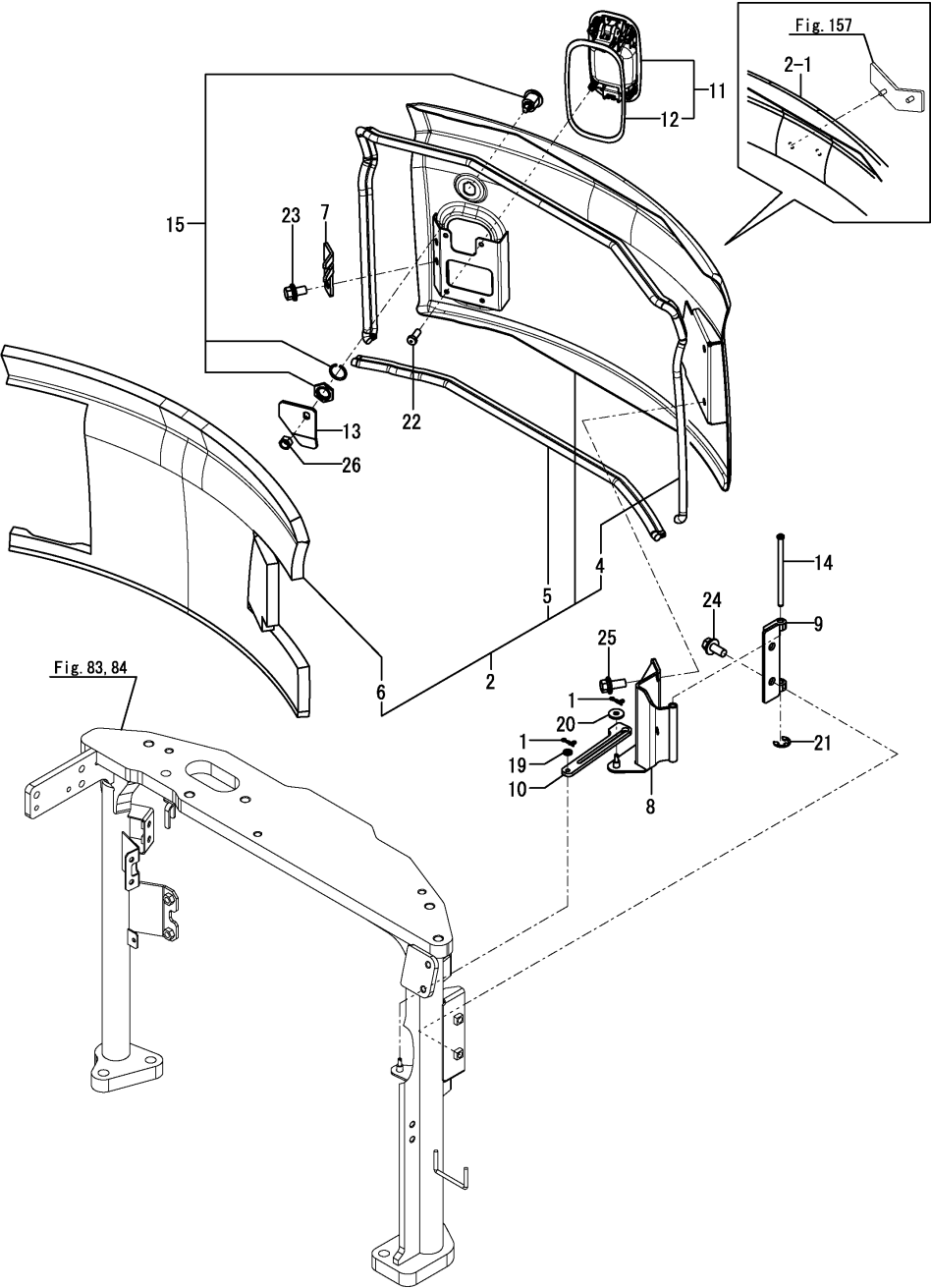
Fig.77. TAMPA TRASEIRA
