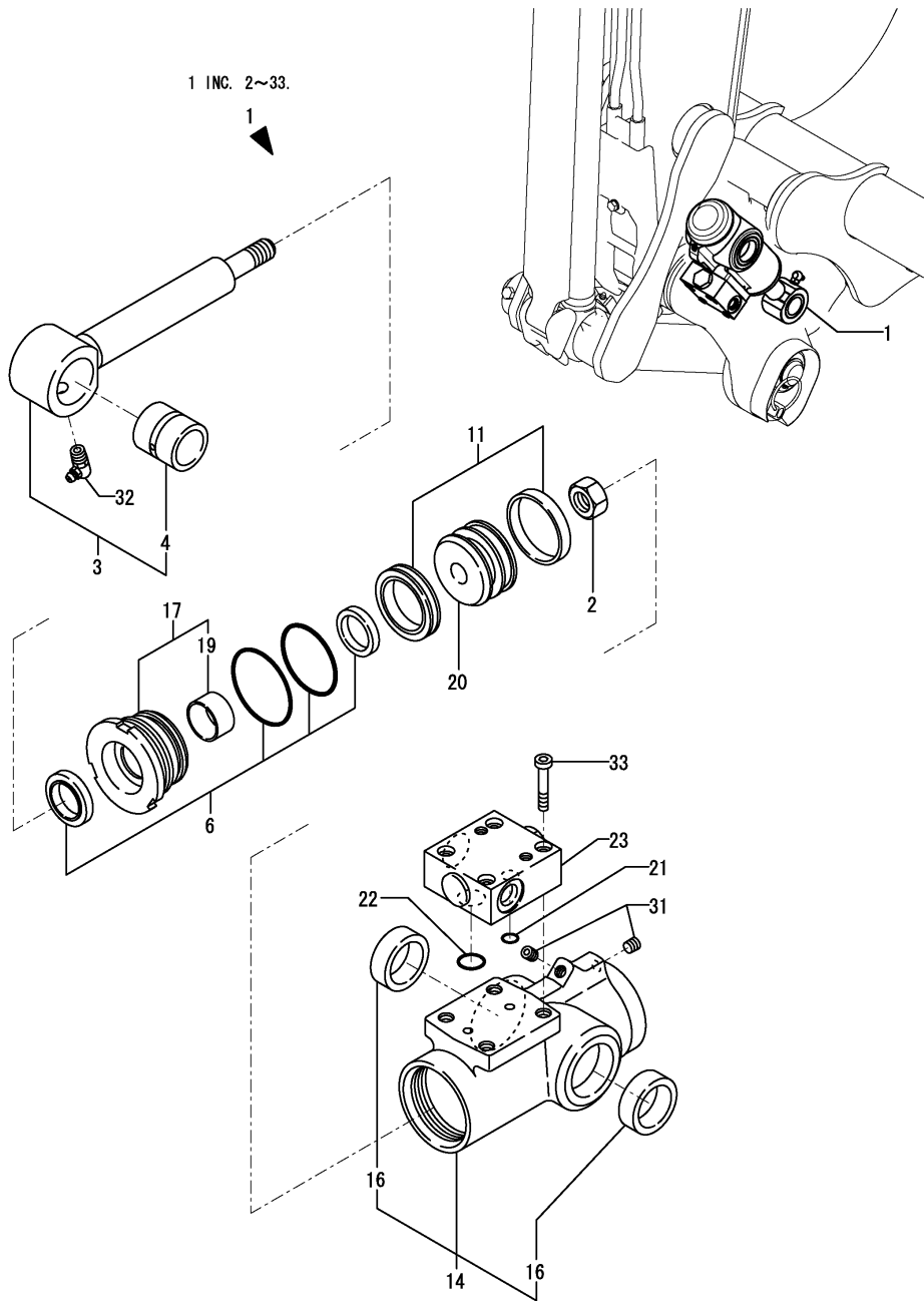
OCK50-M00170 EQUIPAMENTO HIDRÁULICO Fig.104. CILINDRO DO ENGATE RAPIDO
