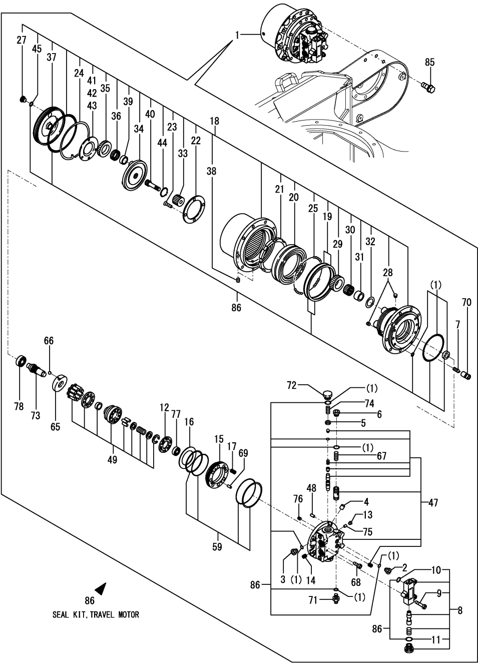
Fig.105. MOTOR DE TRAÇÃO
