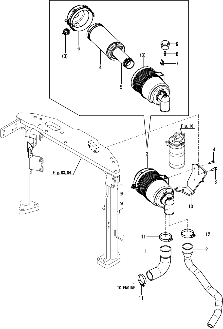
Fig.8. FILTRO DE AR
