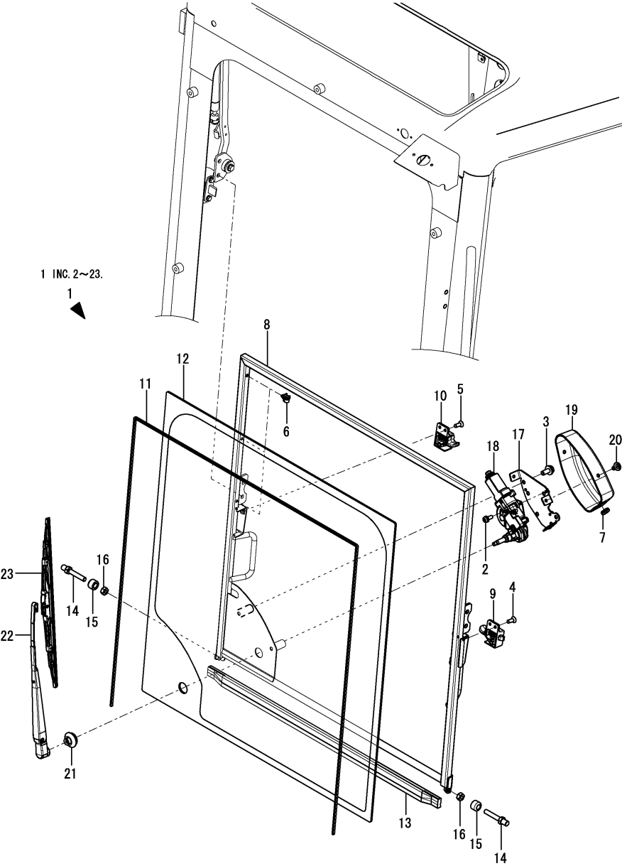
Fig.90. CABINE (JANELA DIANTEIRA)(2)
