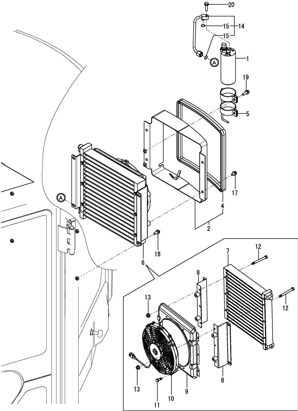
Fig.34. AR CONDICIONADO (CONDENSADOR)
