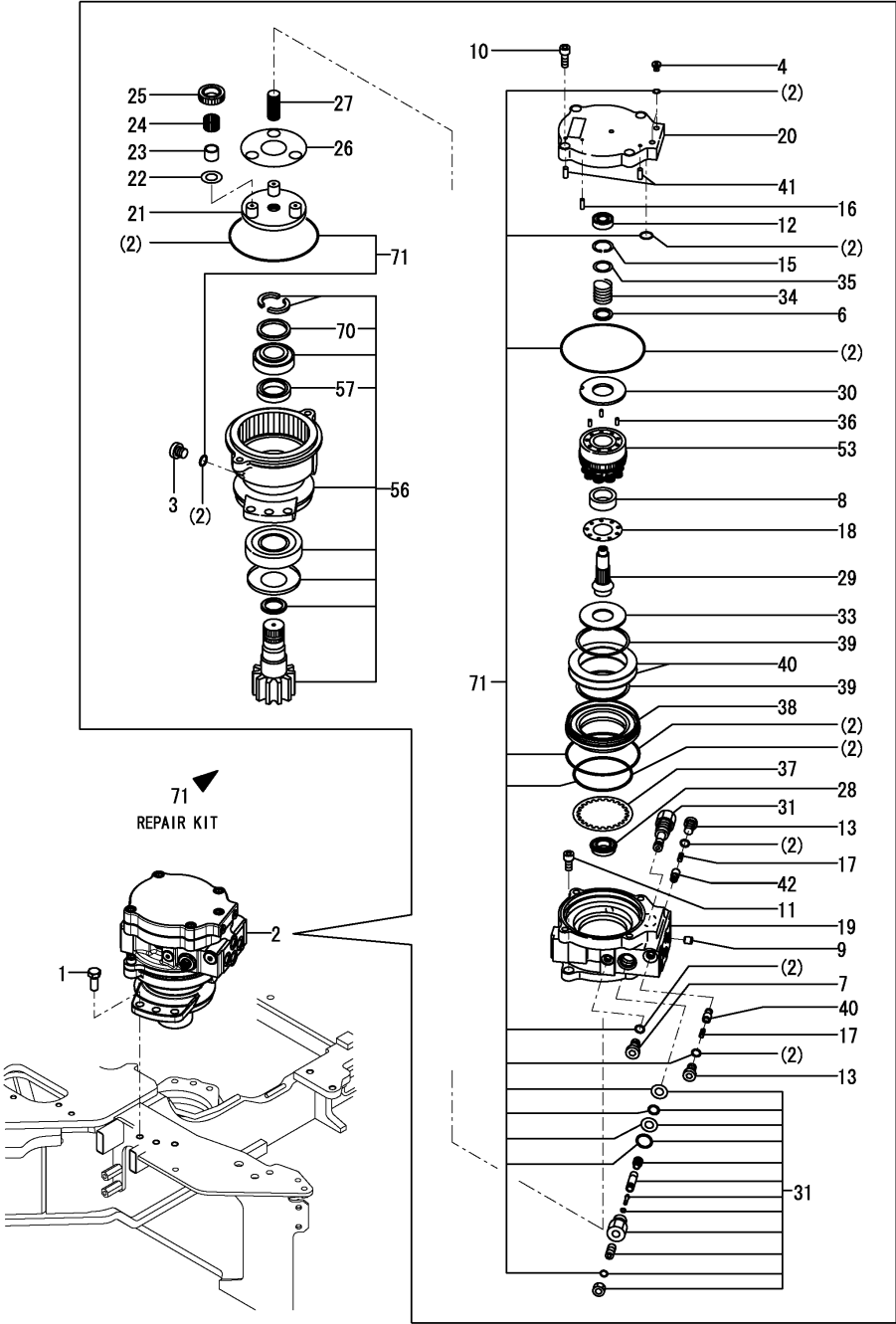
Fig.106. MOTOR DE GIRO
