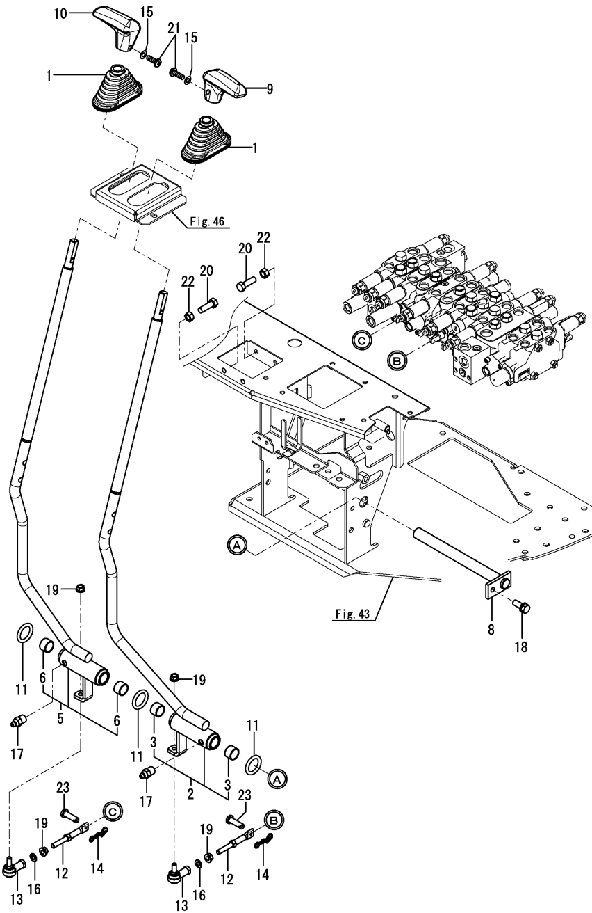
Fig.44. ALAVANCA DE ACIONAMENTO DAS ESTEIRAS
