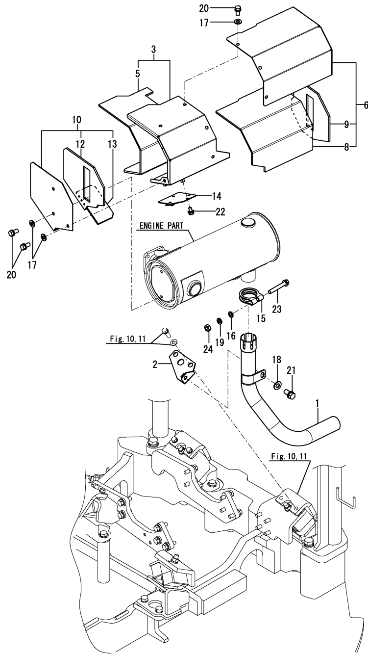
Fig.7. SILENCIOSO
