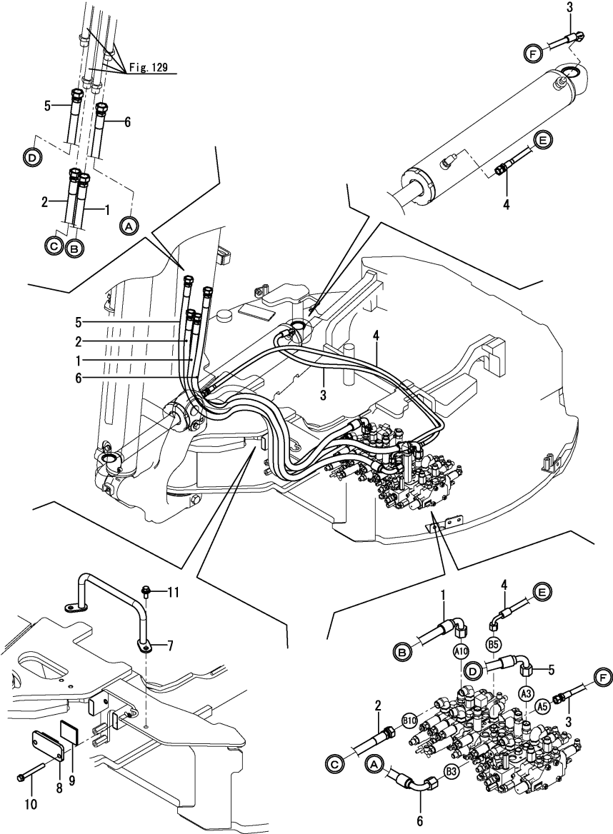
Fig.125. VÁLVULA DE CONTROLE - BULKHEAD E GIRO
