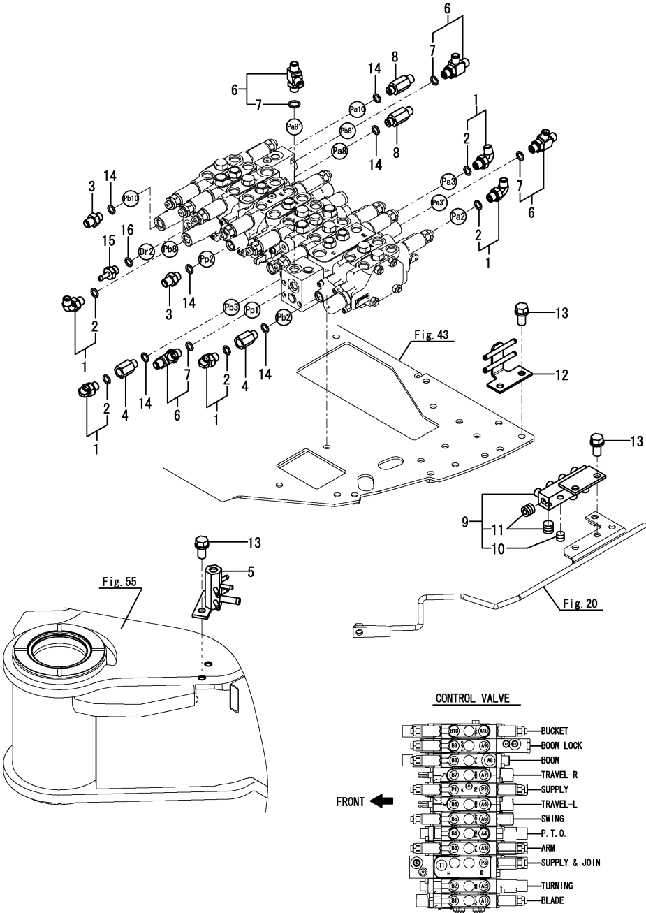
Fig.123. VÁLVULA DE CONTROLE (CONEXÃO) (2)
