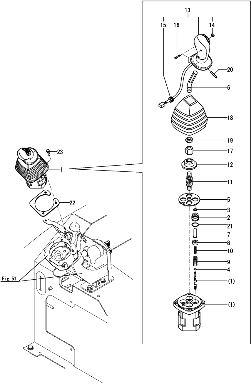
Fig.115. VÁLVULA DE CONTROLE REMOTO (DIREITA)
