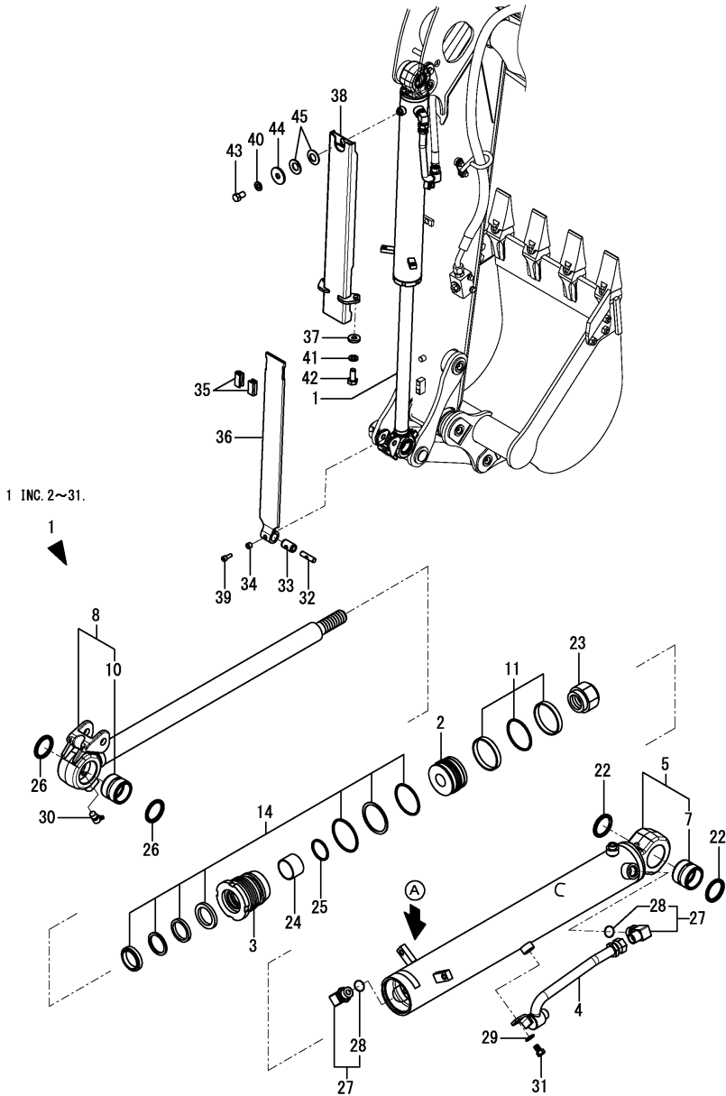
Fig.153. (101A)CILINDRO DA CAÇAMBA(ESPEC. K)
