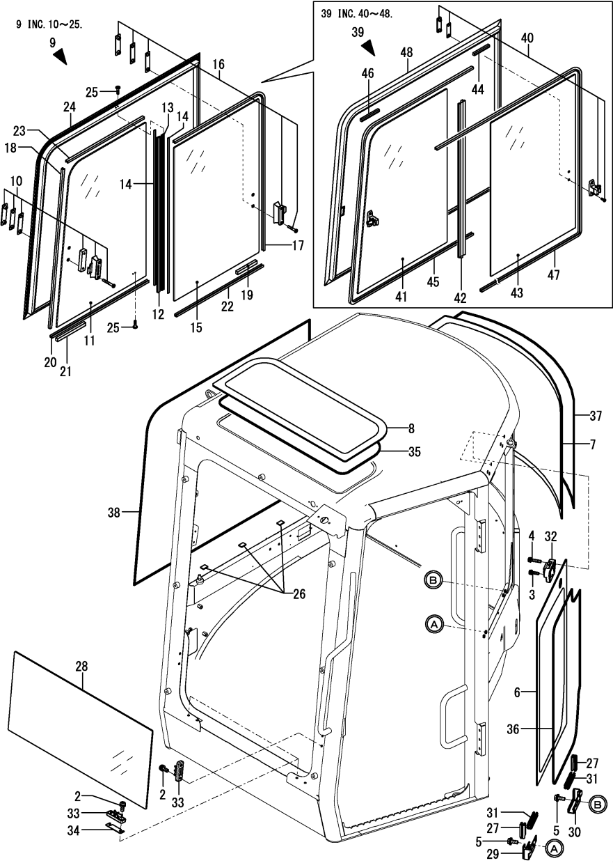
Fig.91. CABINE (VIDROS)
