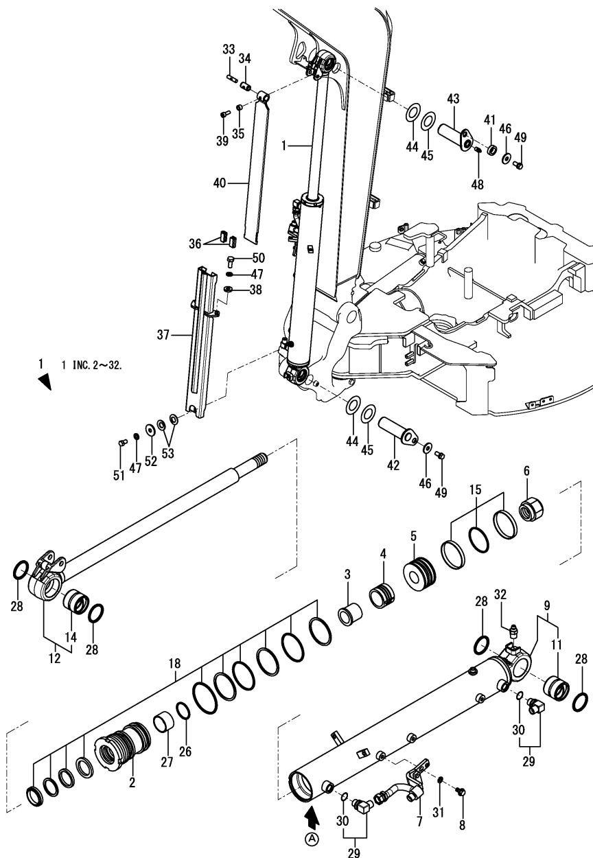
Fig.151. (99A)CILINDRO DA LANÇA(ESPEC. K)
