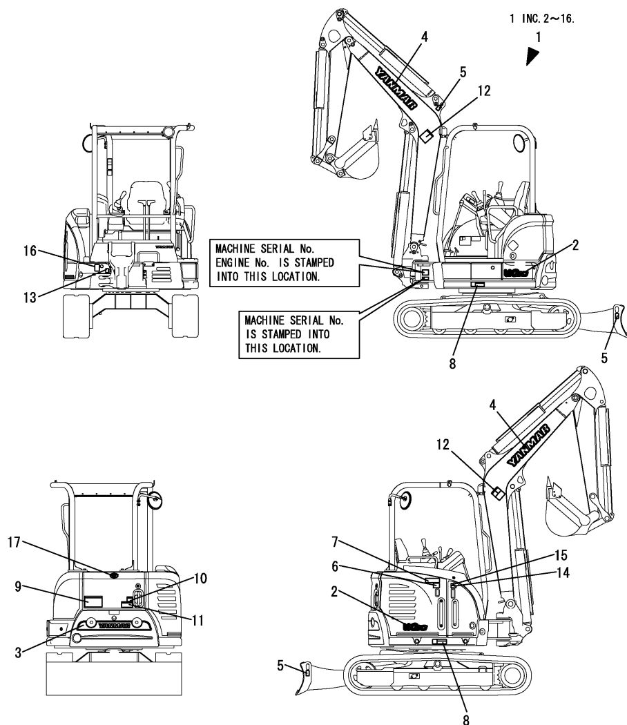
Fig.1. ETIQUETA(EXTERNA)(PARA MBF000)
