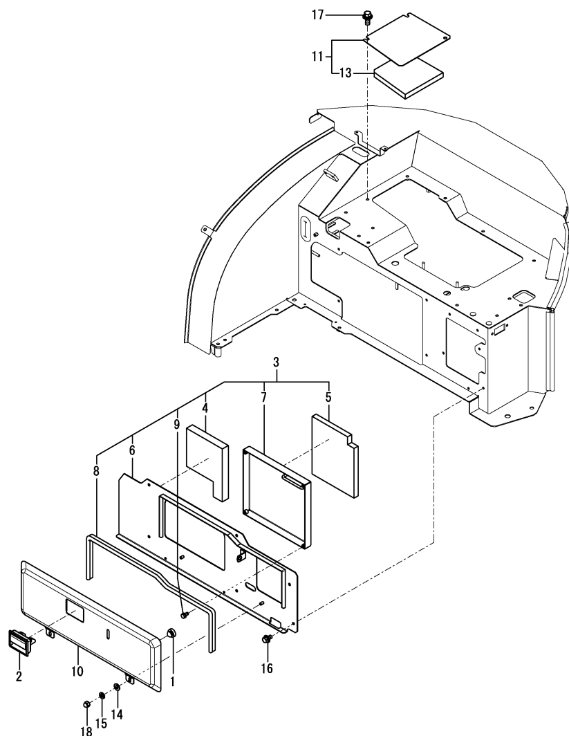
Fig.71. SUPORTE DO ASSENTO (COBERTURA)
