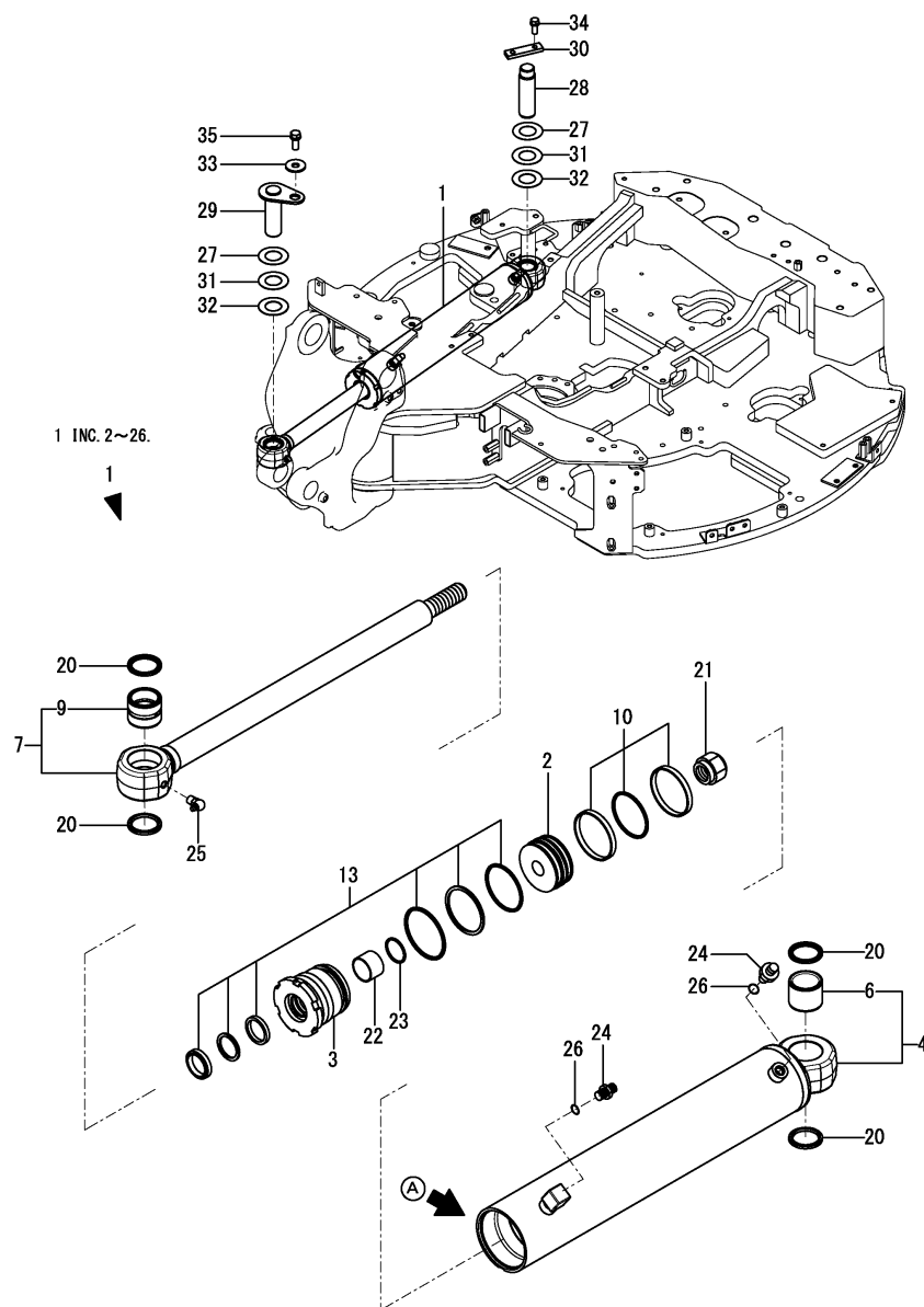
Fig.154. (102A)CILINDRO DE OSCILAÇÃO(ESPEC. K)
