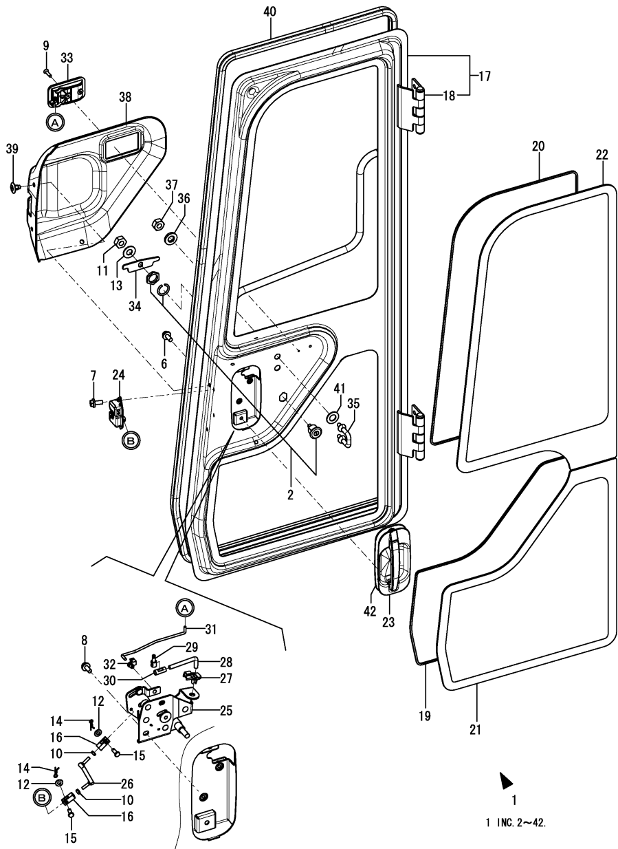
Fig.88. PORTA DA CABINE (2)
