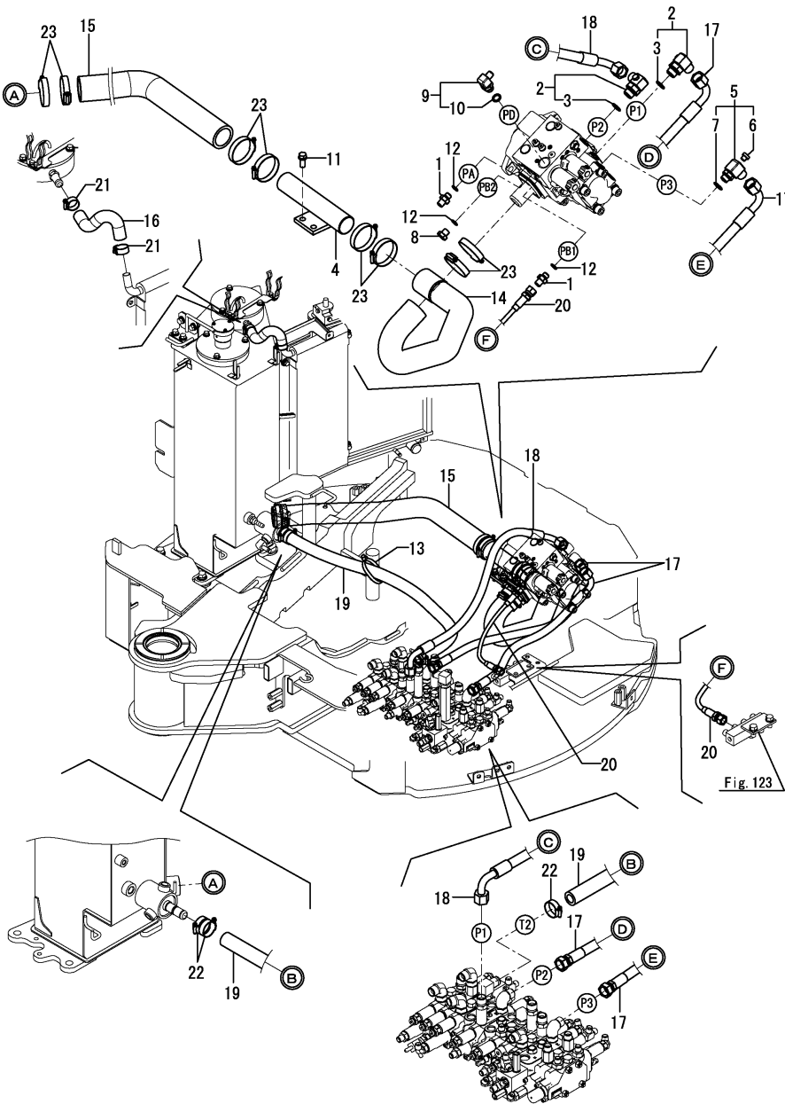
Fig.120. TANQUE - BOMBA E VÁLVULA DE CONTROLE
