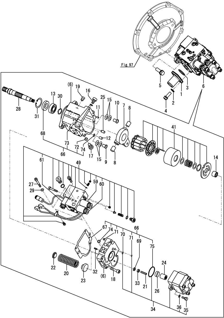
Fig.98. BOMBA HIDRAULICA
