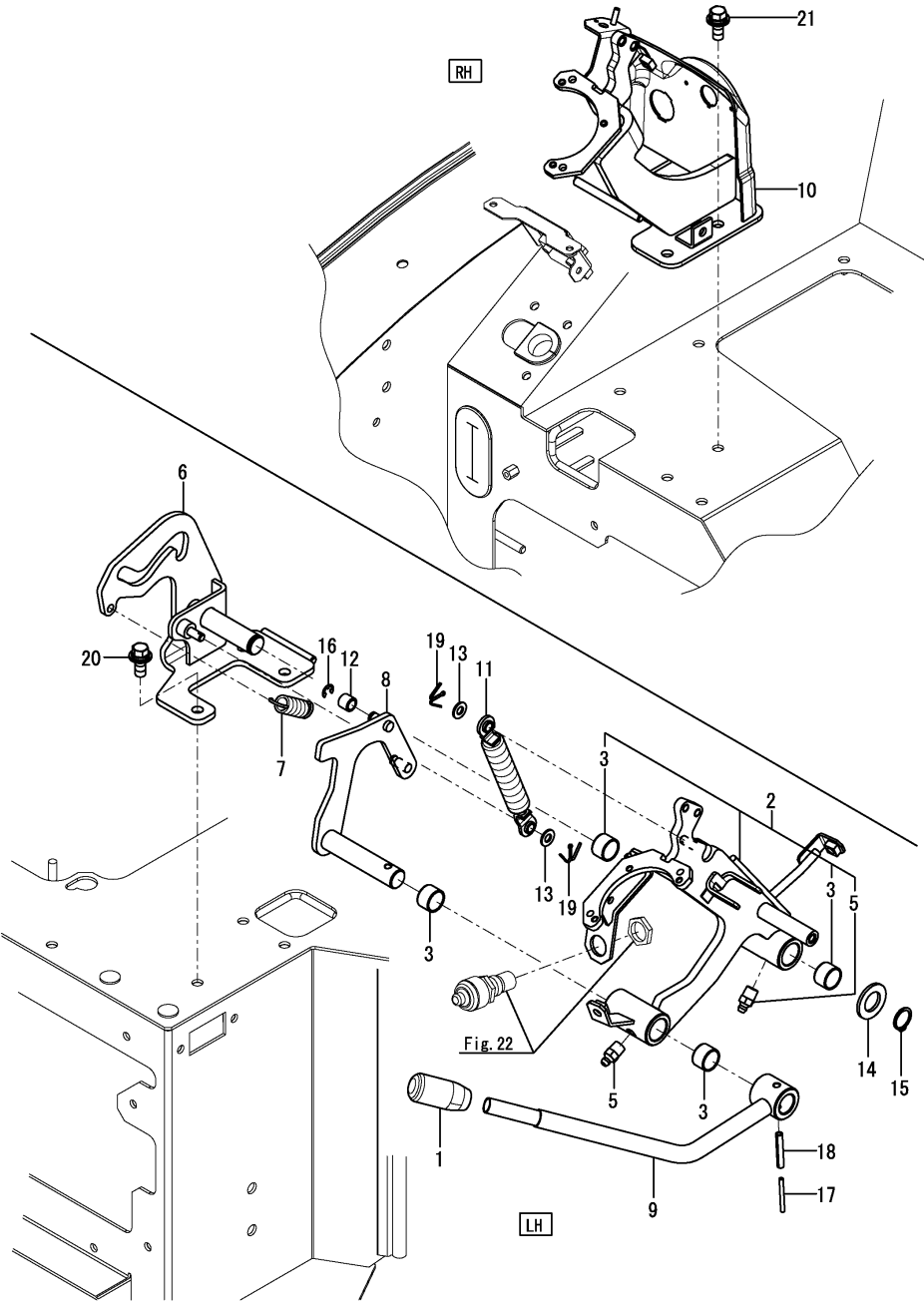
Fig.51. ALAVANCA DA BLOQUEIO E DESCANSO
