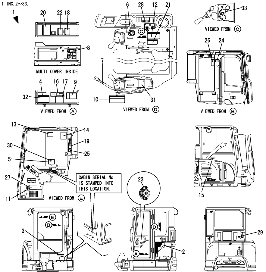
Fig.4. ETIQUETA(CABINE)(PARA MBF000)
