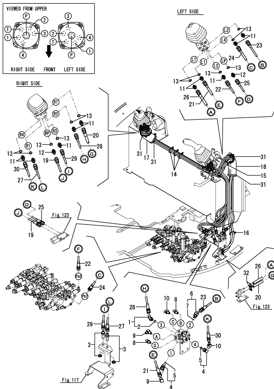
Fig.135. TUBULAÇÃO DE CONTROLE (VÁLVULA SELETORA - VÁLVULA DE CONTROLE REMOTO)
