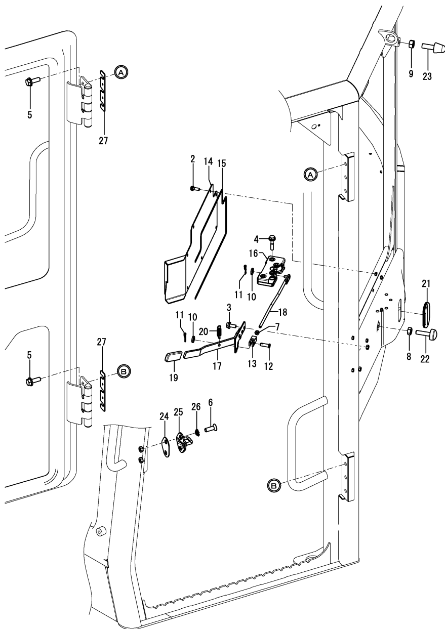
Fig.87. PORTA DA CABINE (1)
