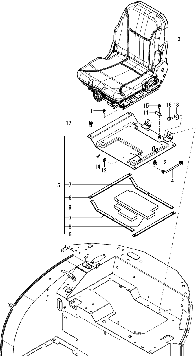
Fig.72. BANCO
