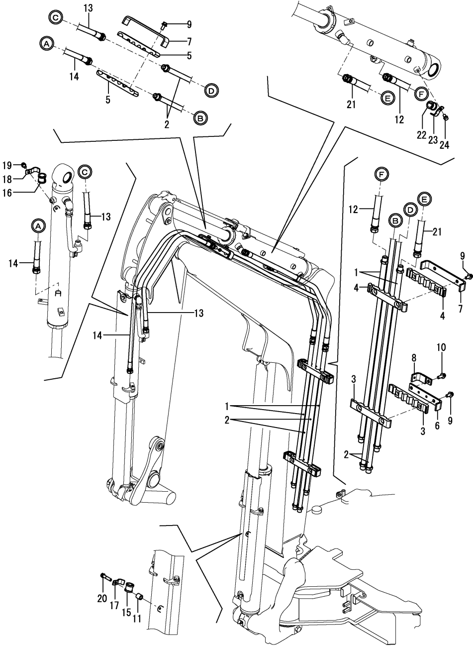
Fig.129. CILINDRO DO BRAÇO E CILINDRO DA CAÇAMBA
