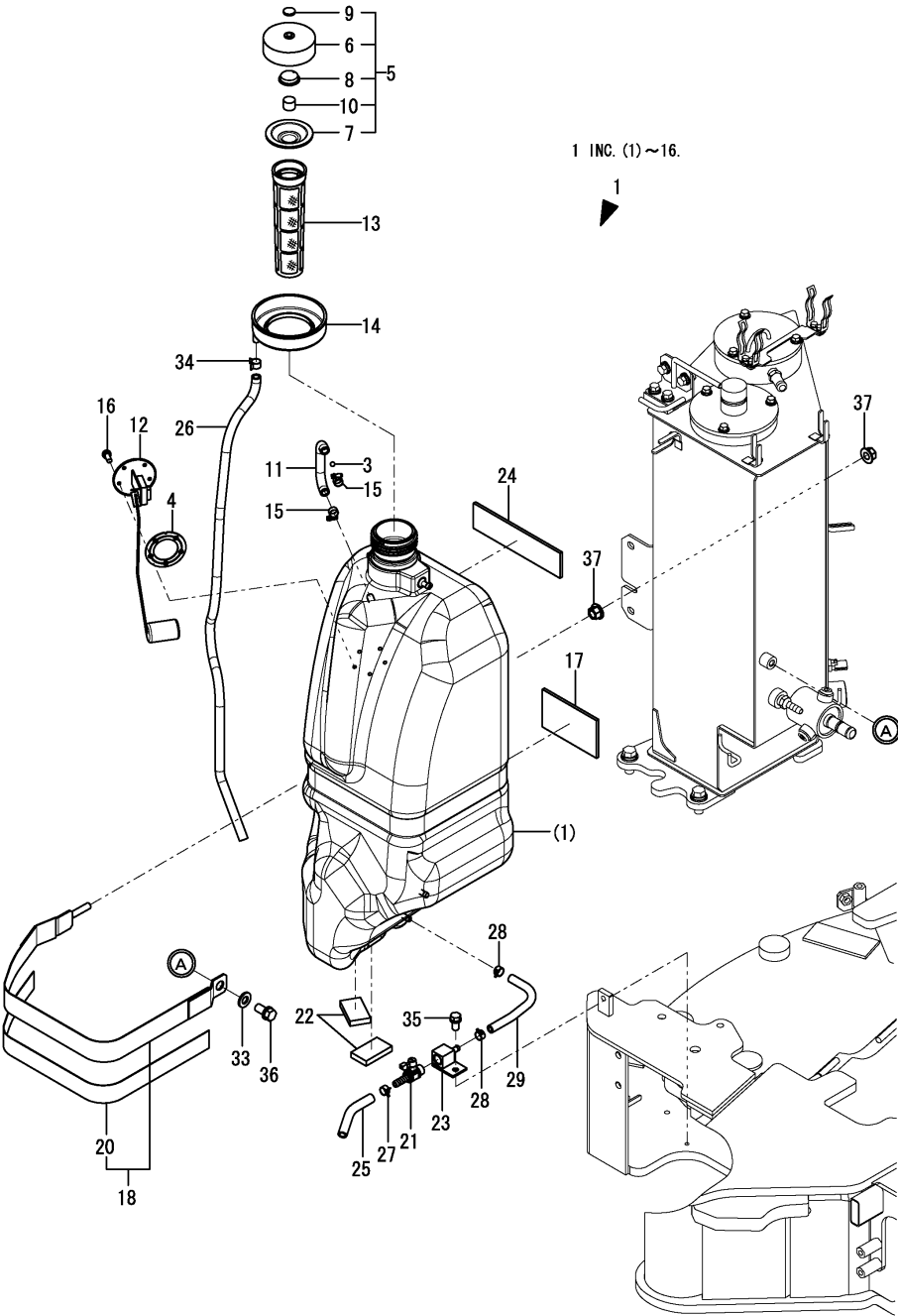
Fig.15. TANQUE DE COMBUSTÍVEL
