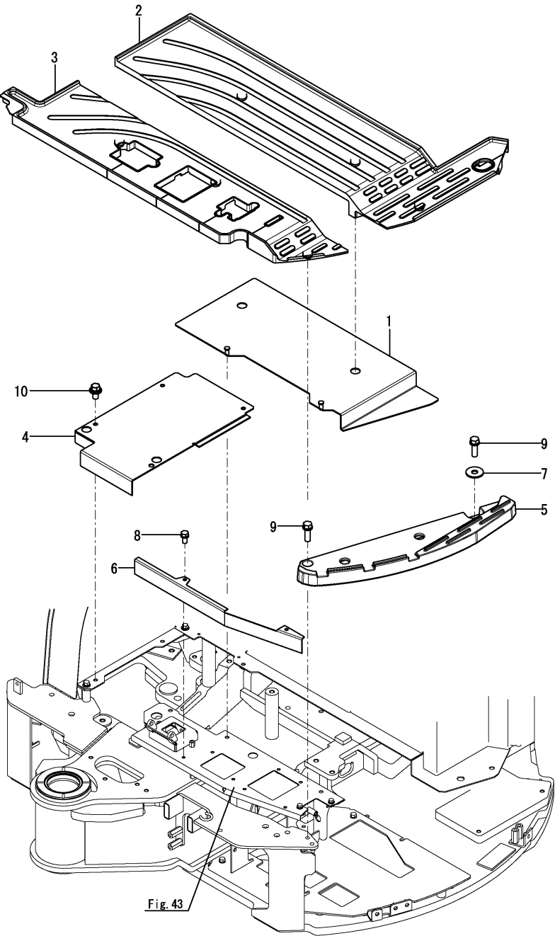
Fig.66. DEGRAU (CAPOTA)
