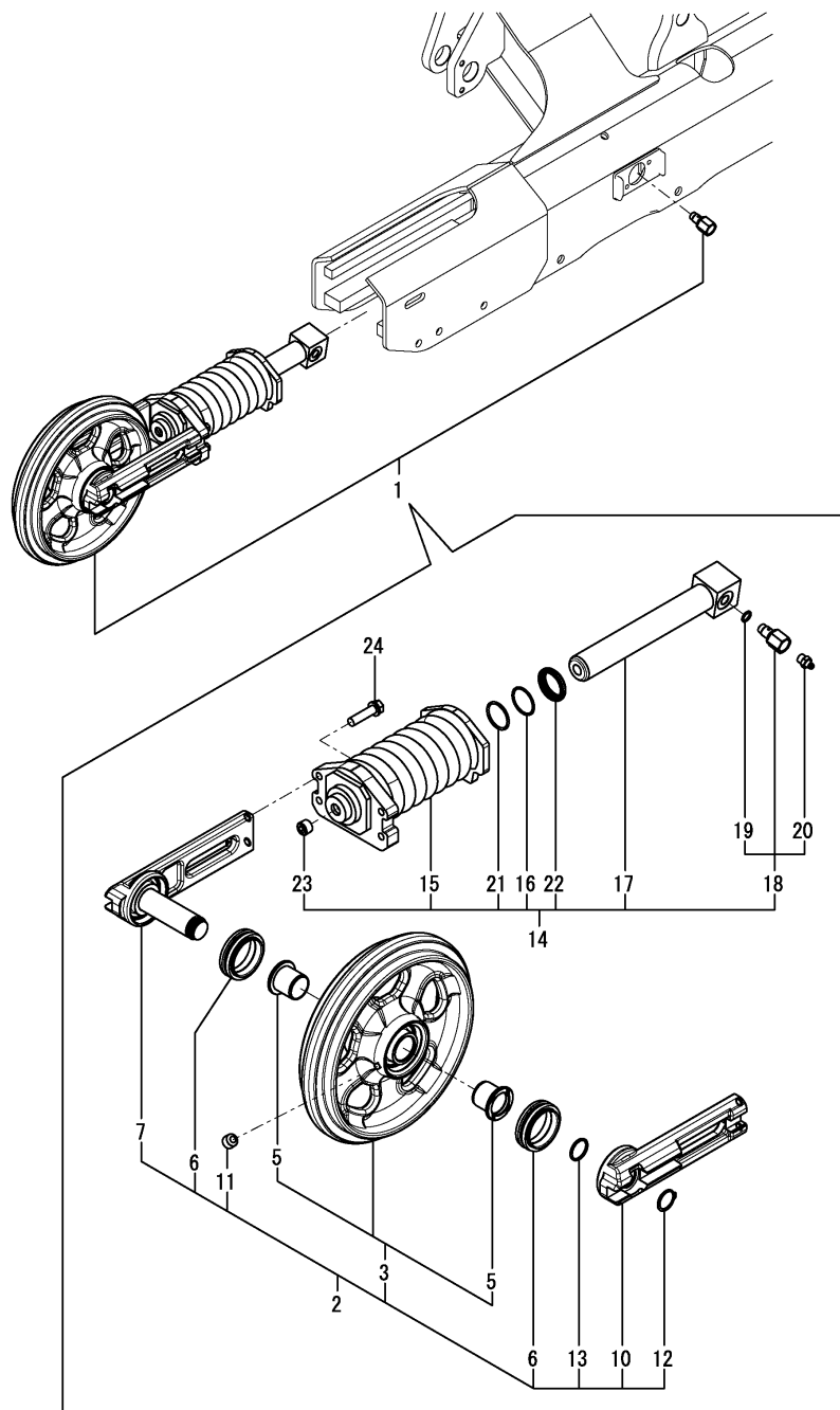
Fig.37. RODA GUIA E AJUSTE (ESPEC. ESTEIRA DE BORRACHA)
