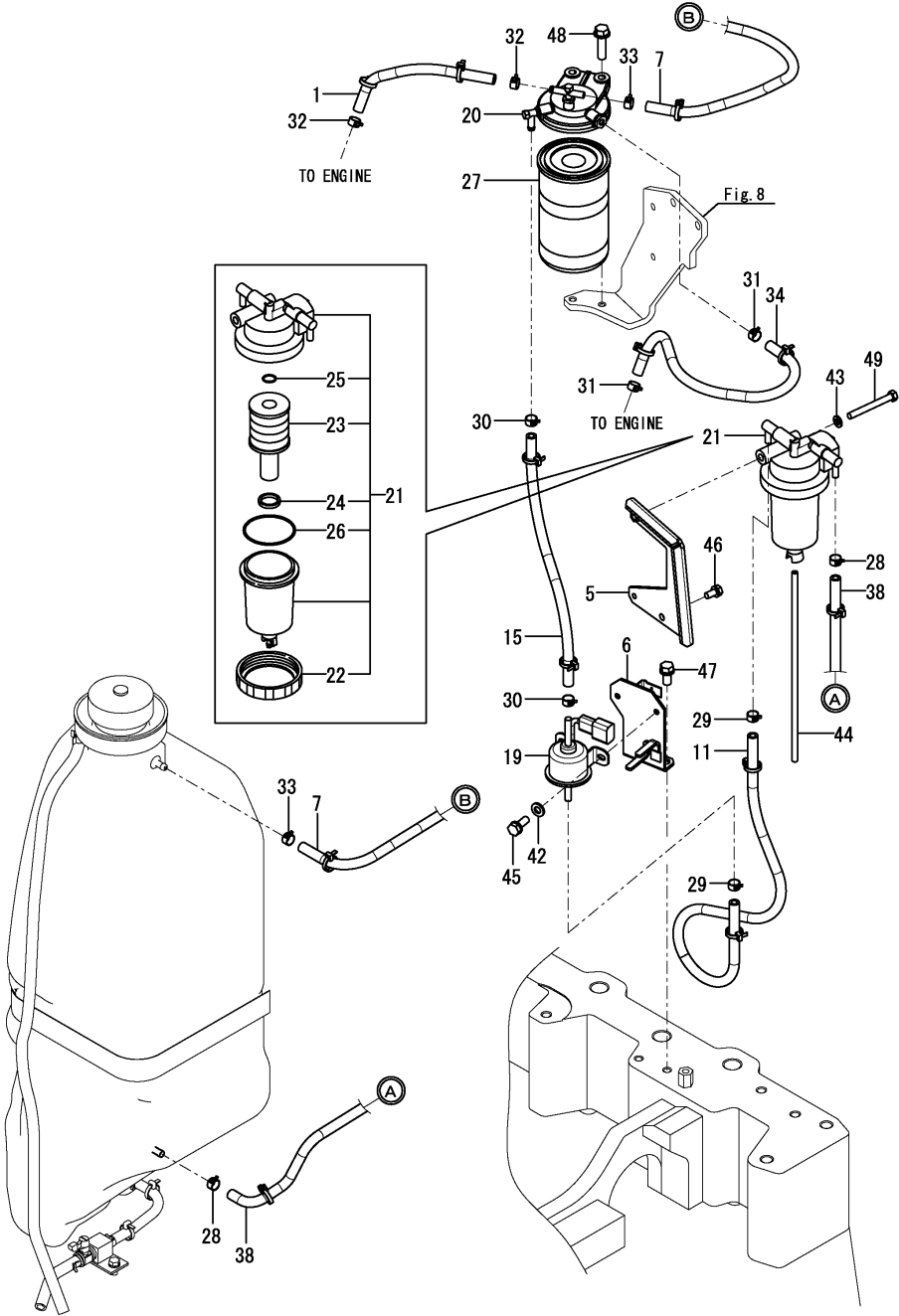
Fig.16. TUBULAÇÃO DE COMBUSTIVEL
