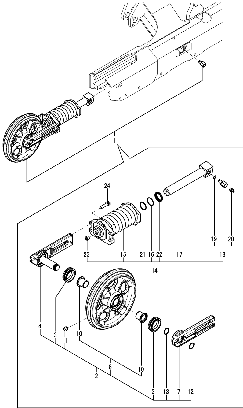
Fig.38. RODA GUIA E AJUSTE (ESPEC. ESTEIRA DE FERRO)
