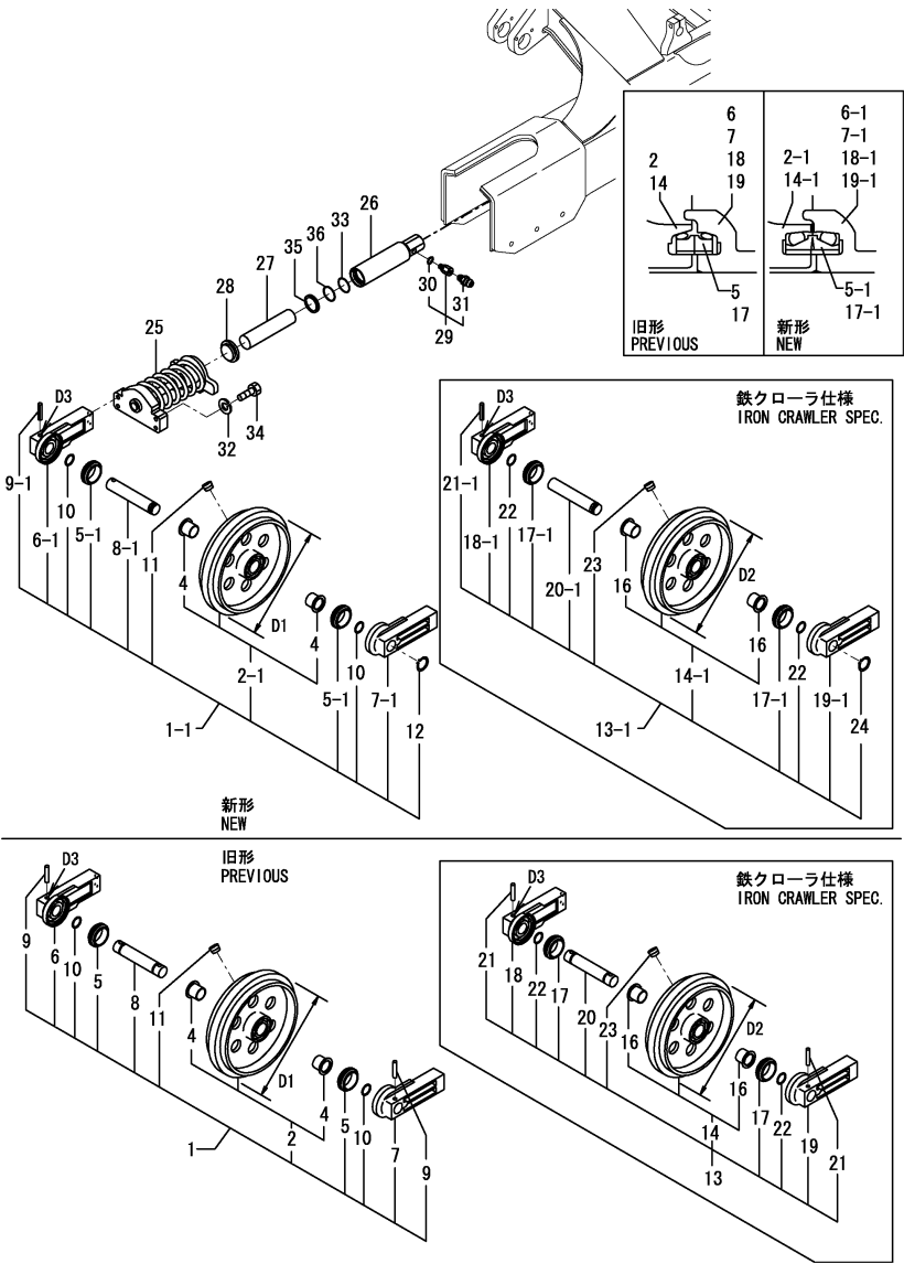
Fig.37. IDLER & ADJUST
