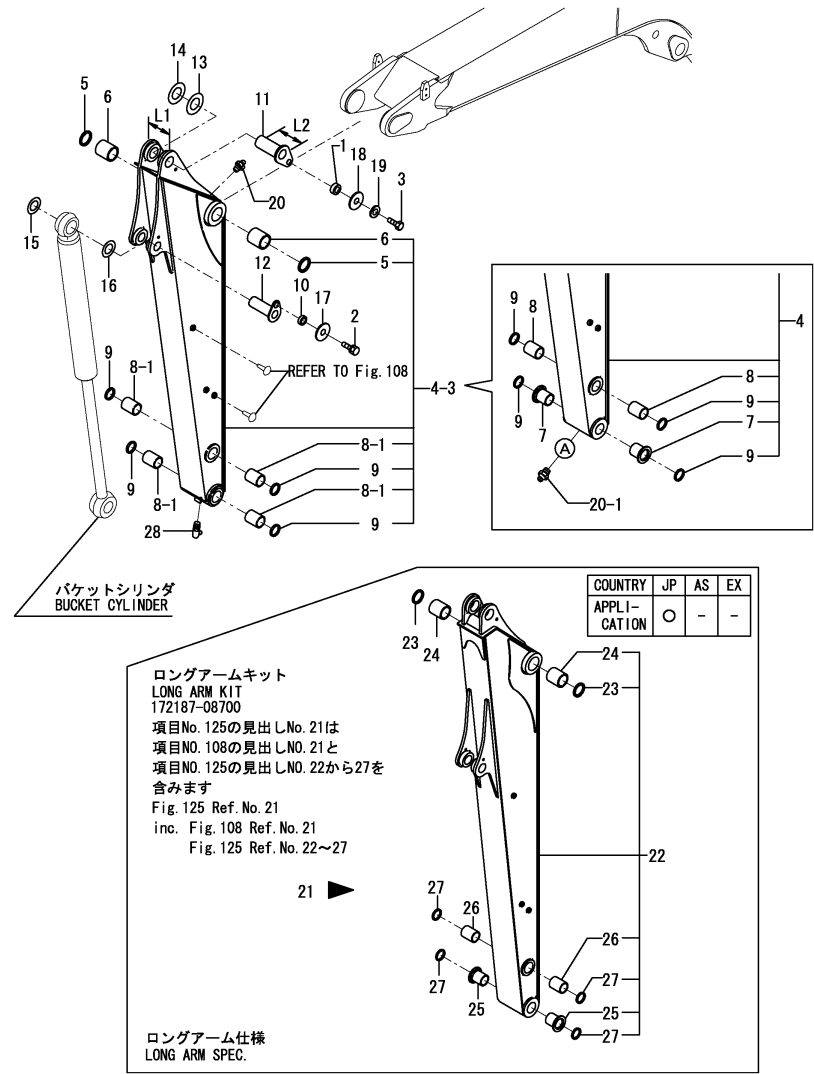
Fig.125. ARM
