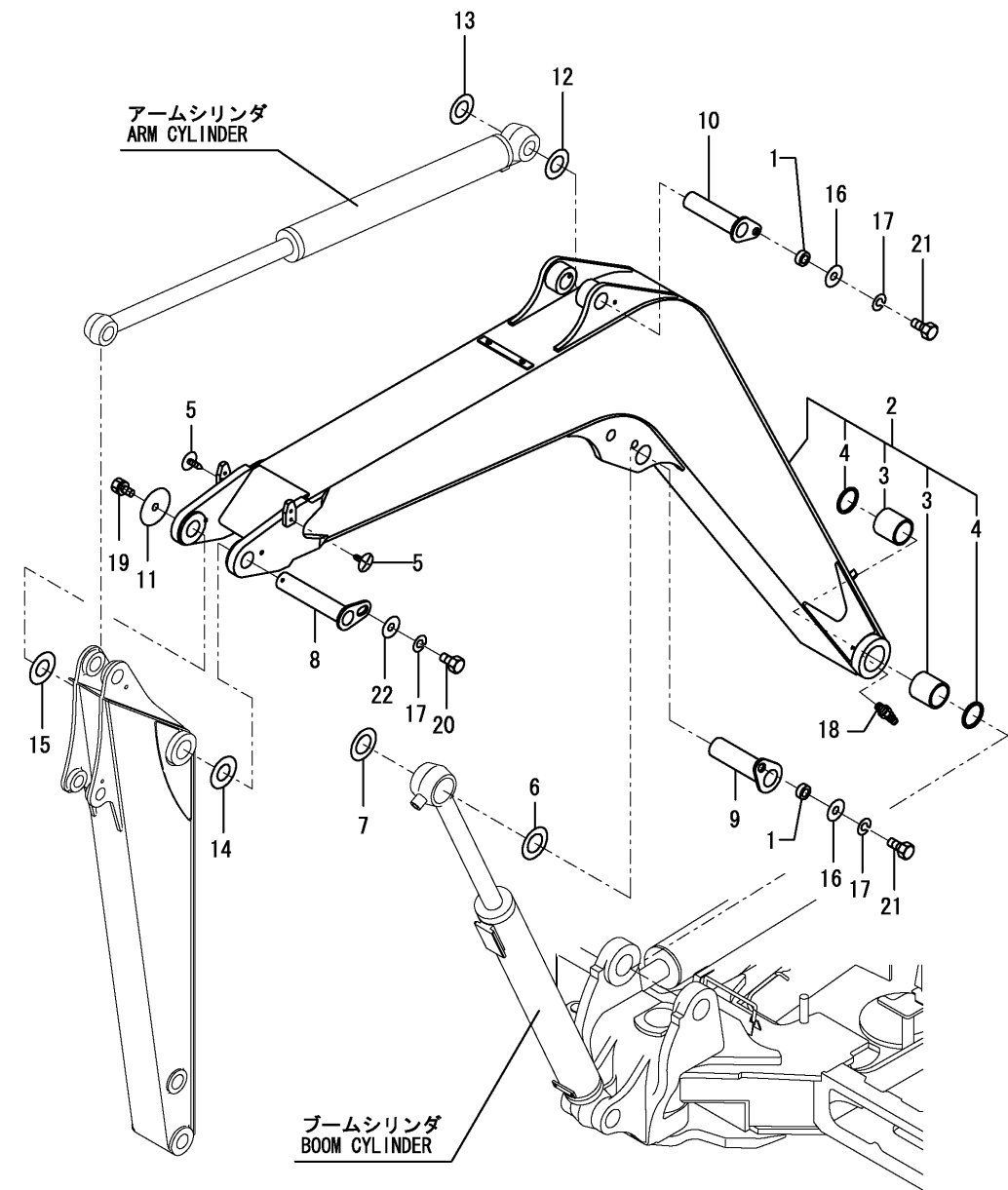
Fig.123. BOOM
