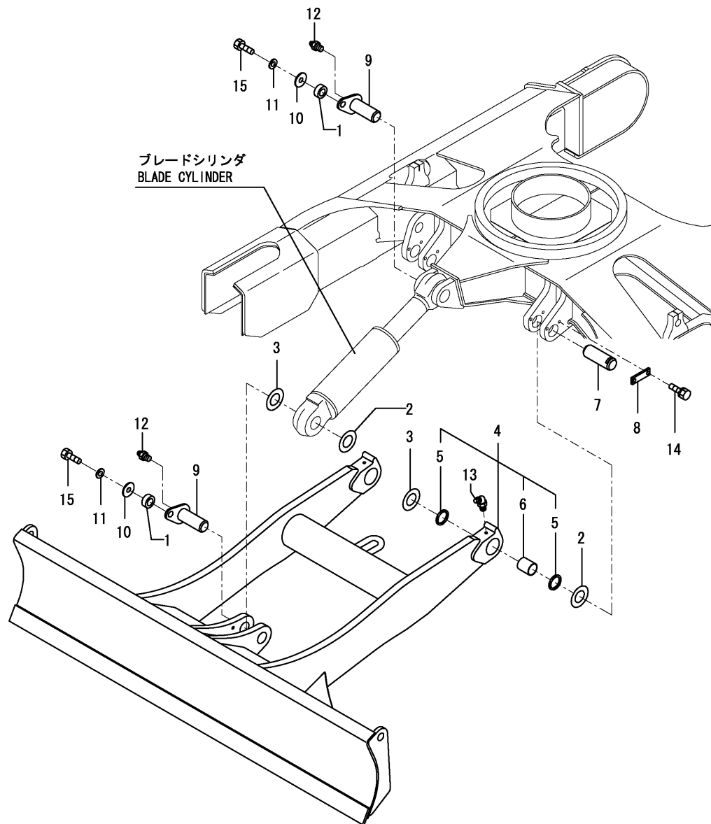
Fig.131. BLADE
