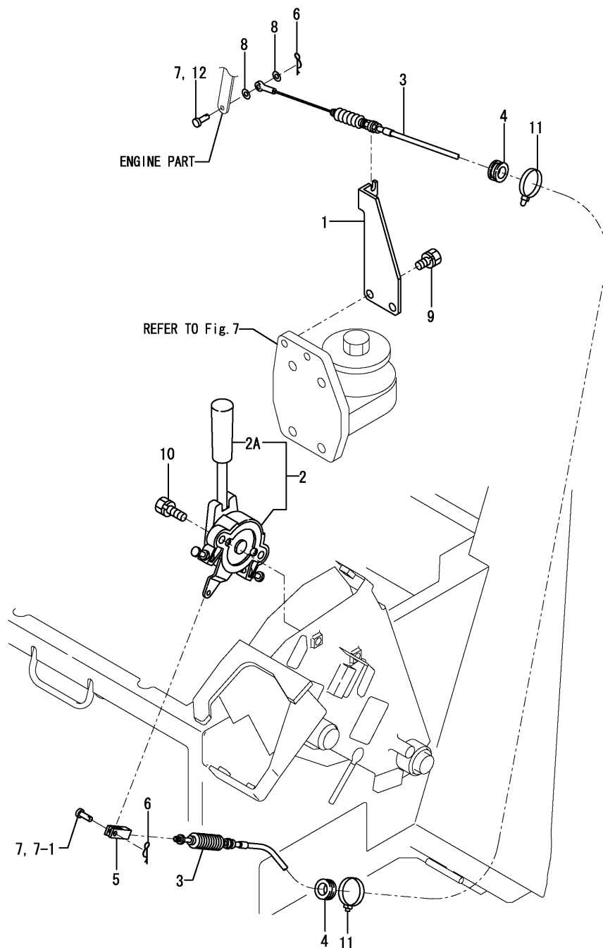
Fig.6. ACCELERATOR LEVER
