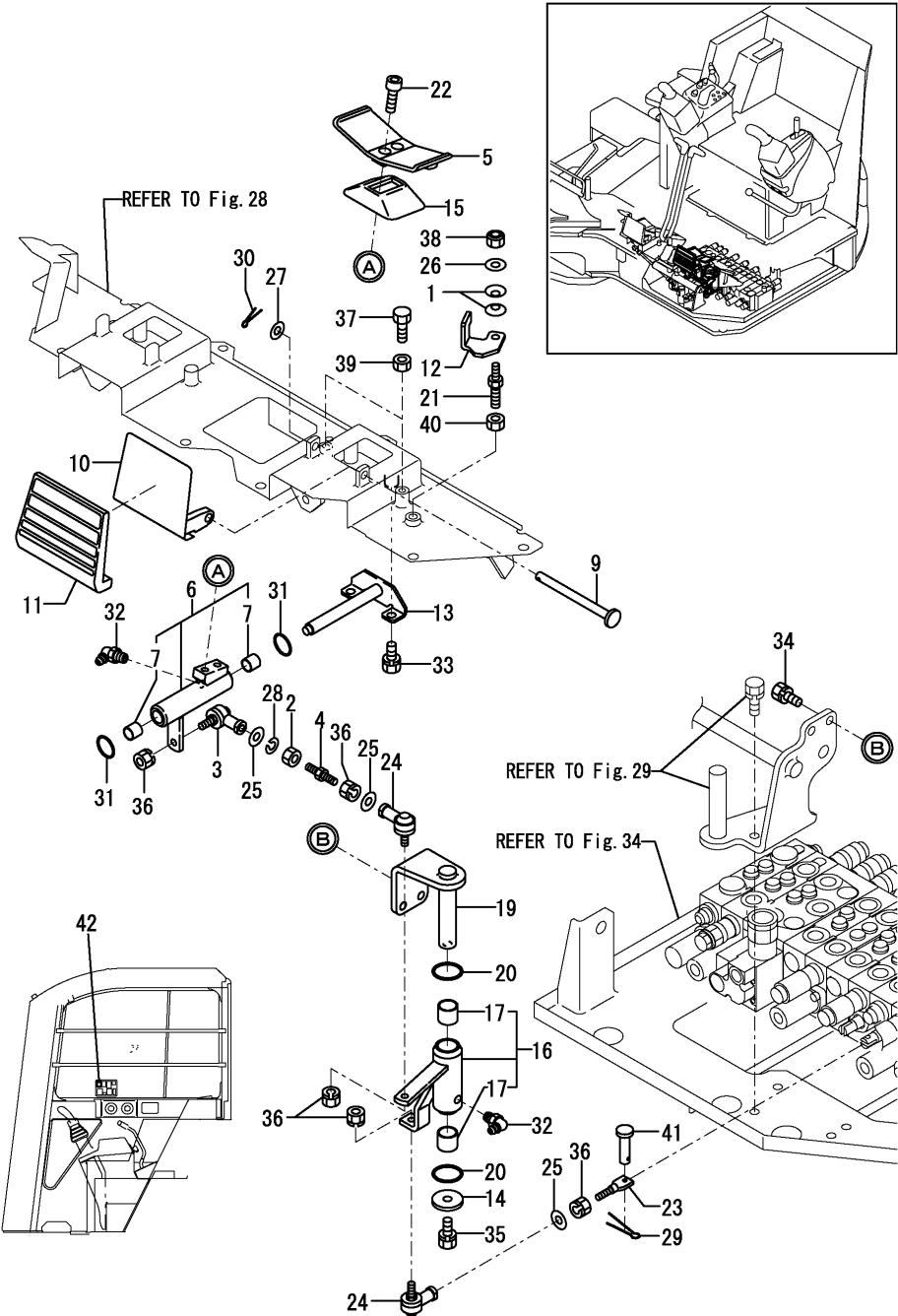
Fig.33. P.T.O.
