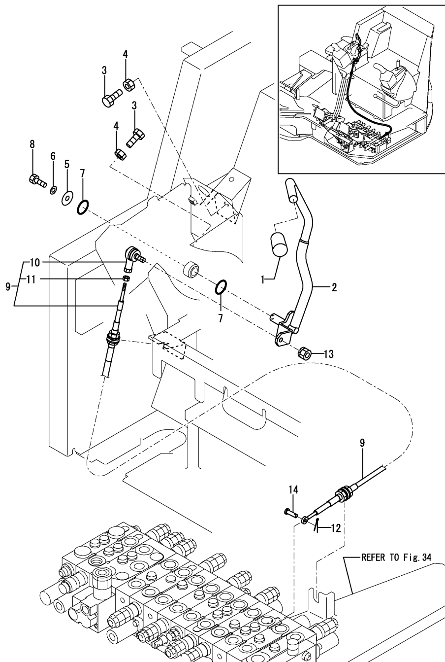
Fig.30. BLADE
