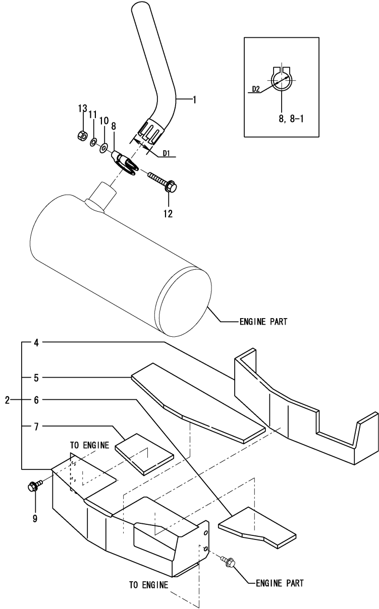
Fig.4. MUFFLER
