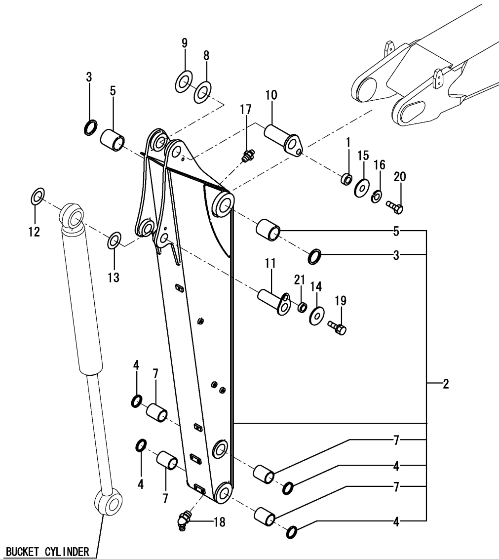
Fig.88. ARM
