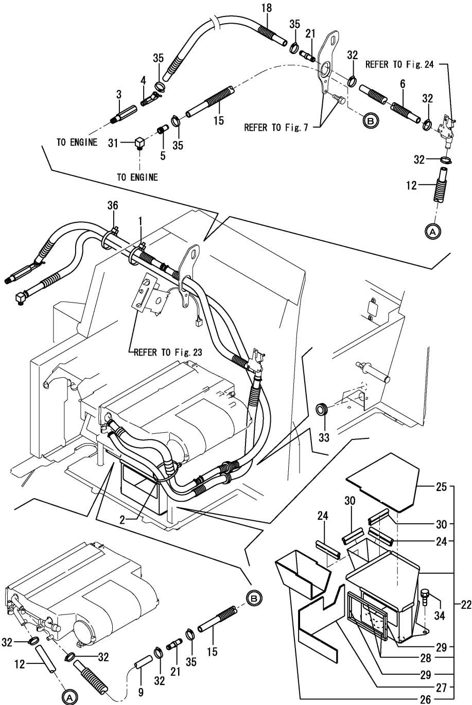
Fig.19. HEATER
