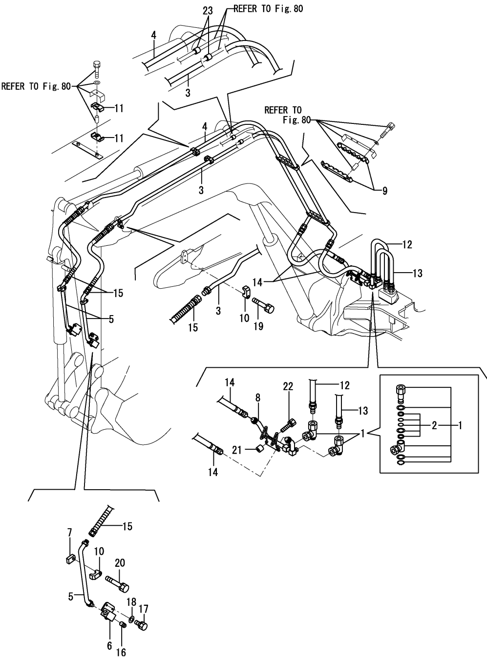
Fig.81. HYD.OIL PIPING(P.T.O. : ARM END)
