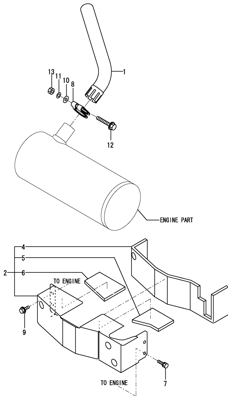
Fig.4. MUFLER
