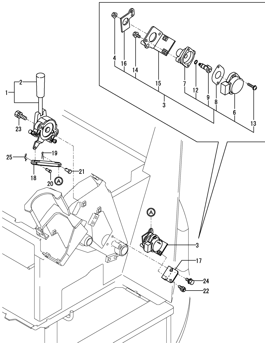
Fig.6. ACCELERATOR LEVER
