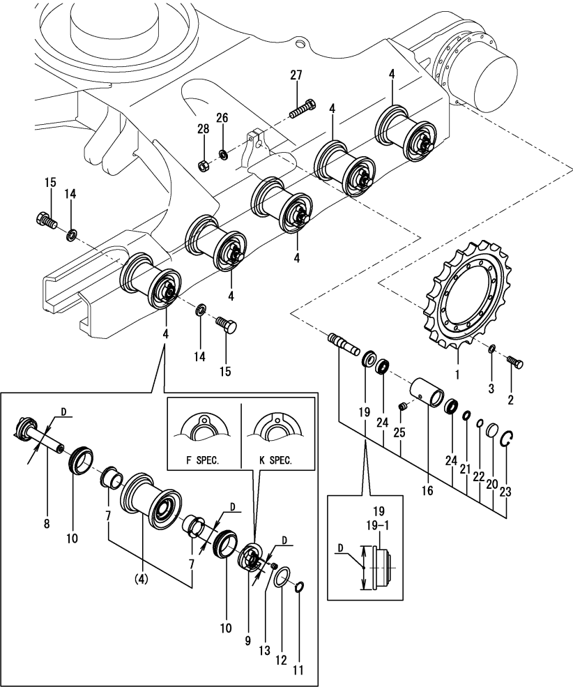
Fig.25. SPROCKET & ROLLER
