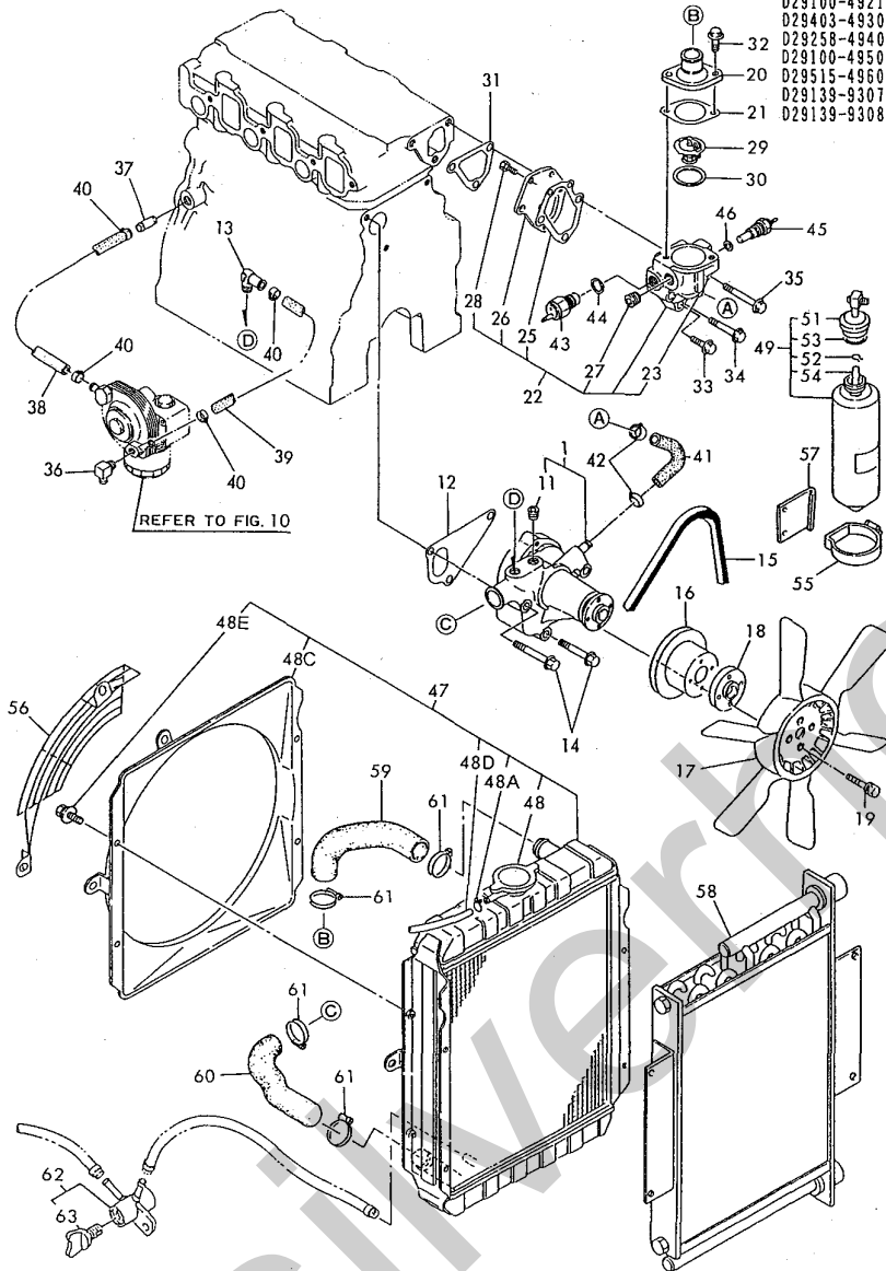
Fig. 12 CWシステム COOLING WATER SYSTEM
