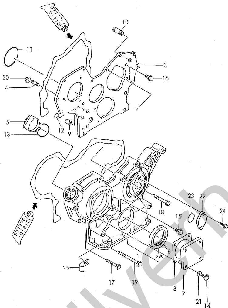
Fig. 2 ギヤケース GEAR HOUSING
