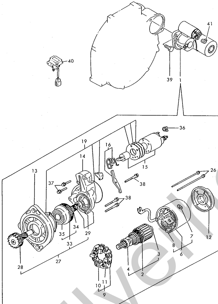
Fig. 18 スターティングモータ STARTING MOTOR
