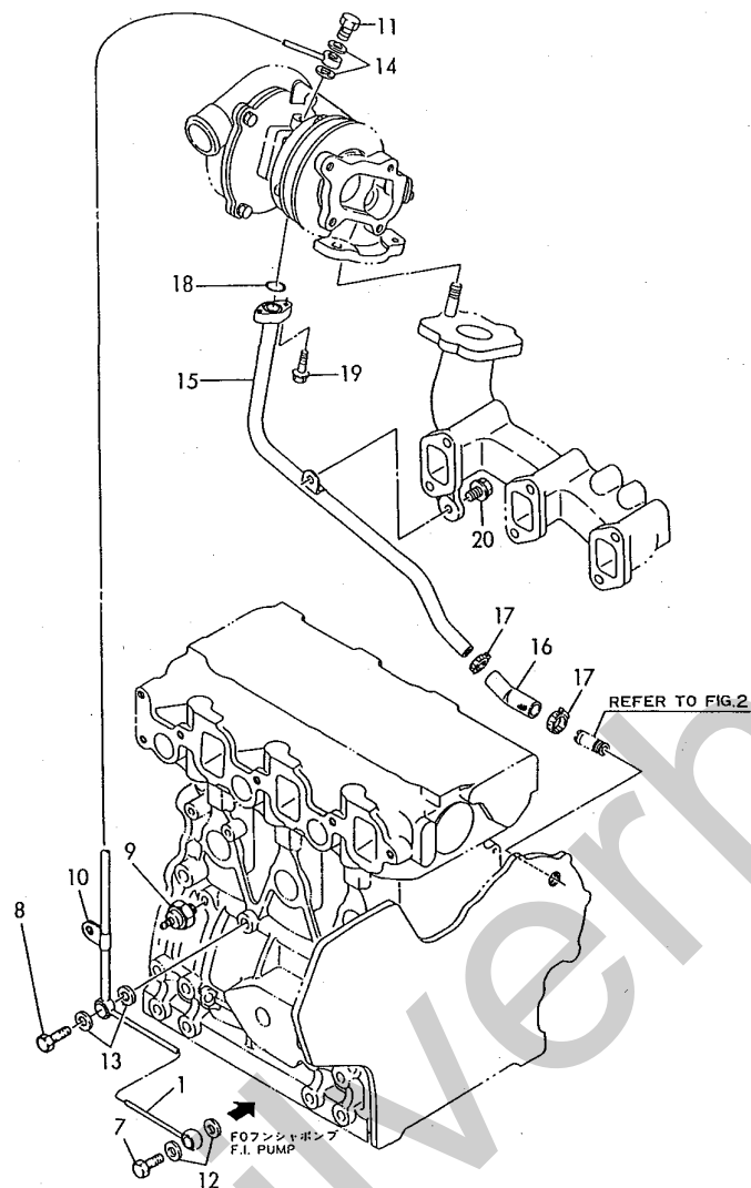
Fig. 11 LOパイプ LUB. OIL LINE
