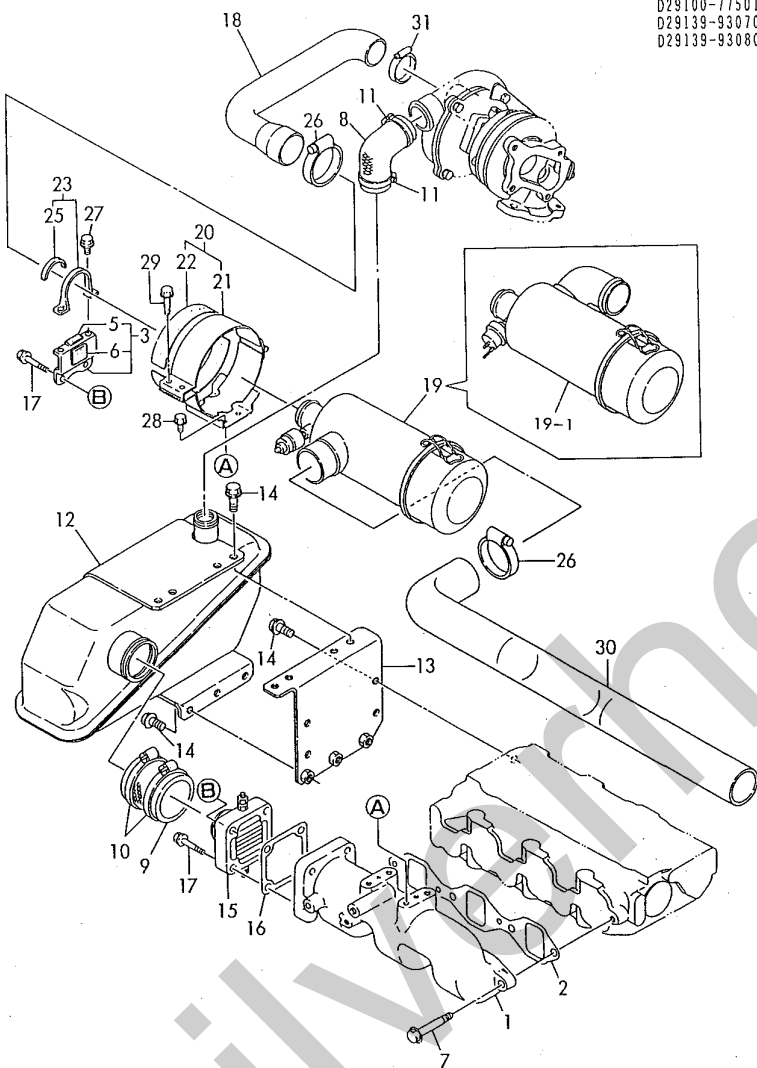
Fig. 5 キュウキマニホールド & SUCTION MANIFOLD &
