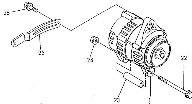
Fig. 19 ゼネレータ GENERATOR
