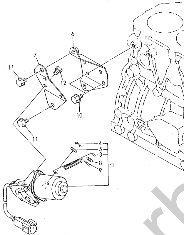
Fig. 17 キカンテイシソウチ ENGINE STOP DEVICE
