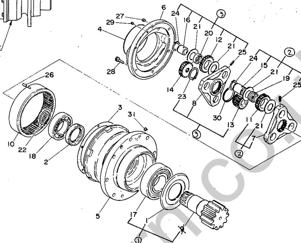
REDUCTION GEAR 減速機
