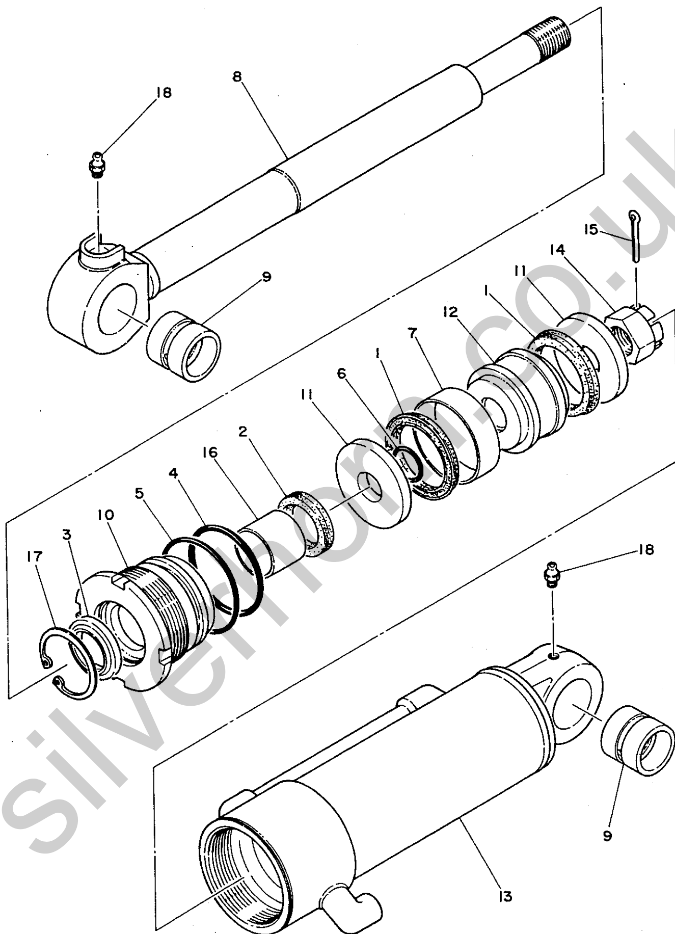
FIG. 32 BLADE CYLINDER
