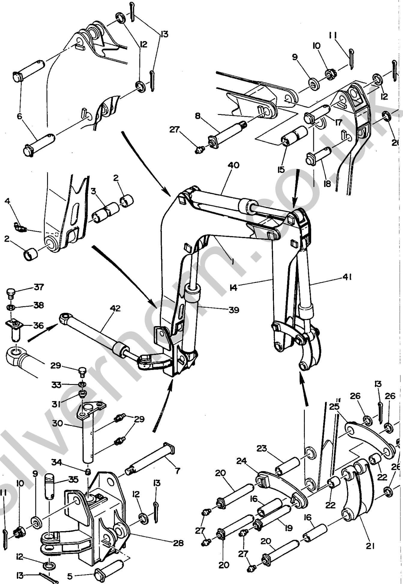
FIG. 22 HOE
