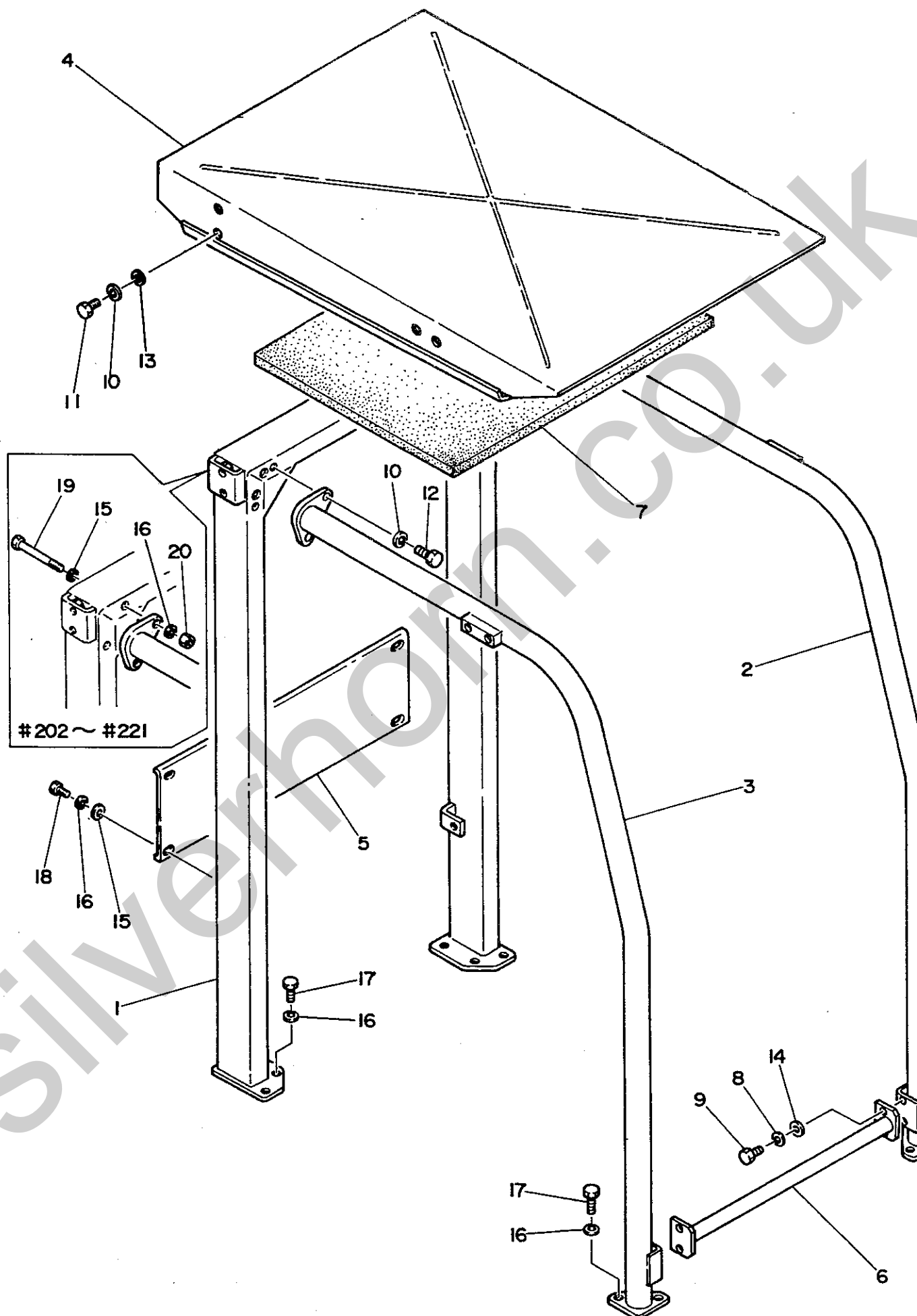
FIG. 21 CANOPY
