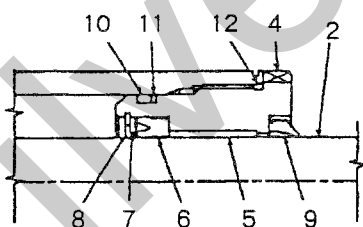
シリンダヘッド部詳細
