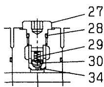
“B-B”断 面 SECTION
