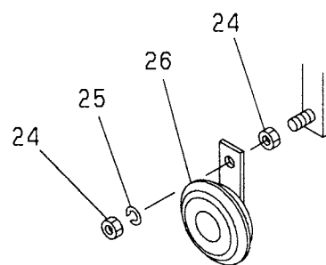
「C」詳細 DETAIL
