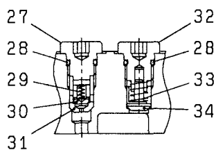
“A-A”断 面 SECTION
