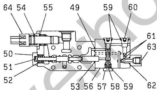
“E-E”断 面 SECTION
