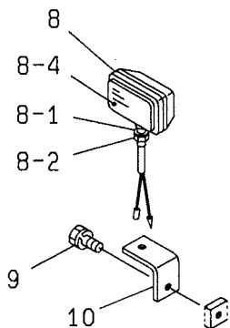
「A」詳細 DETAIL
