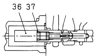
“C”断 面 SECTION
