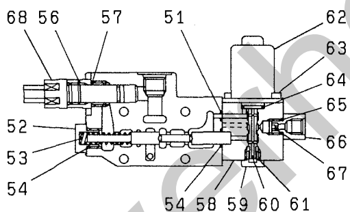
“E-E”断 面 SECTION
