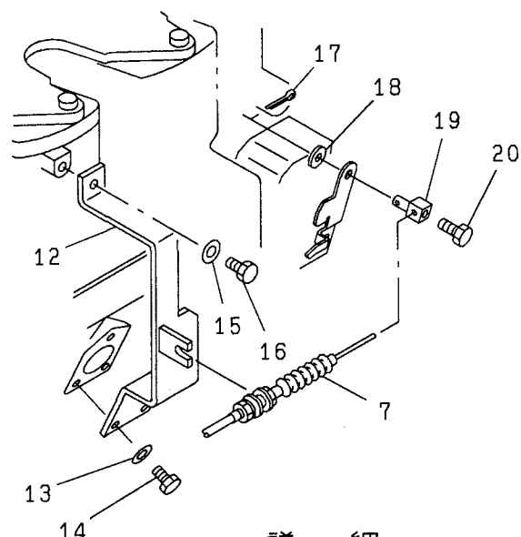
“B” 詳細 DETAIL
