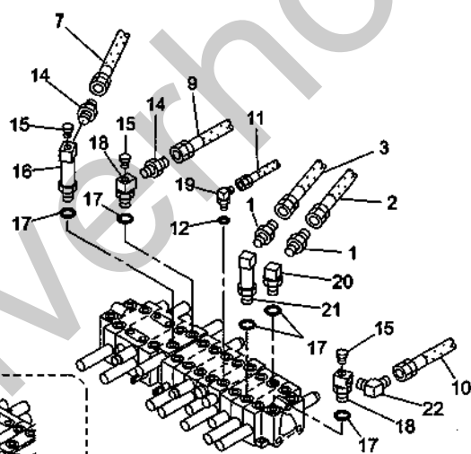
"B" 詳細 DETAIL
