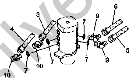
"B" 詳細 DETAIL
