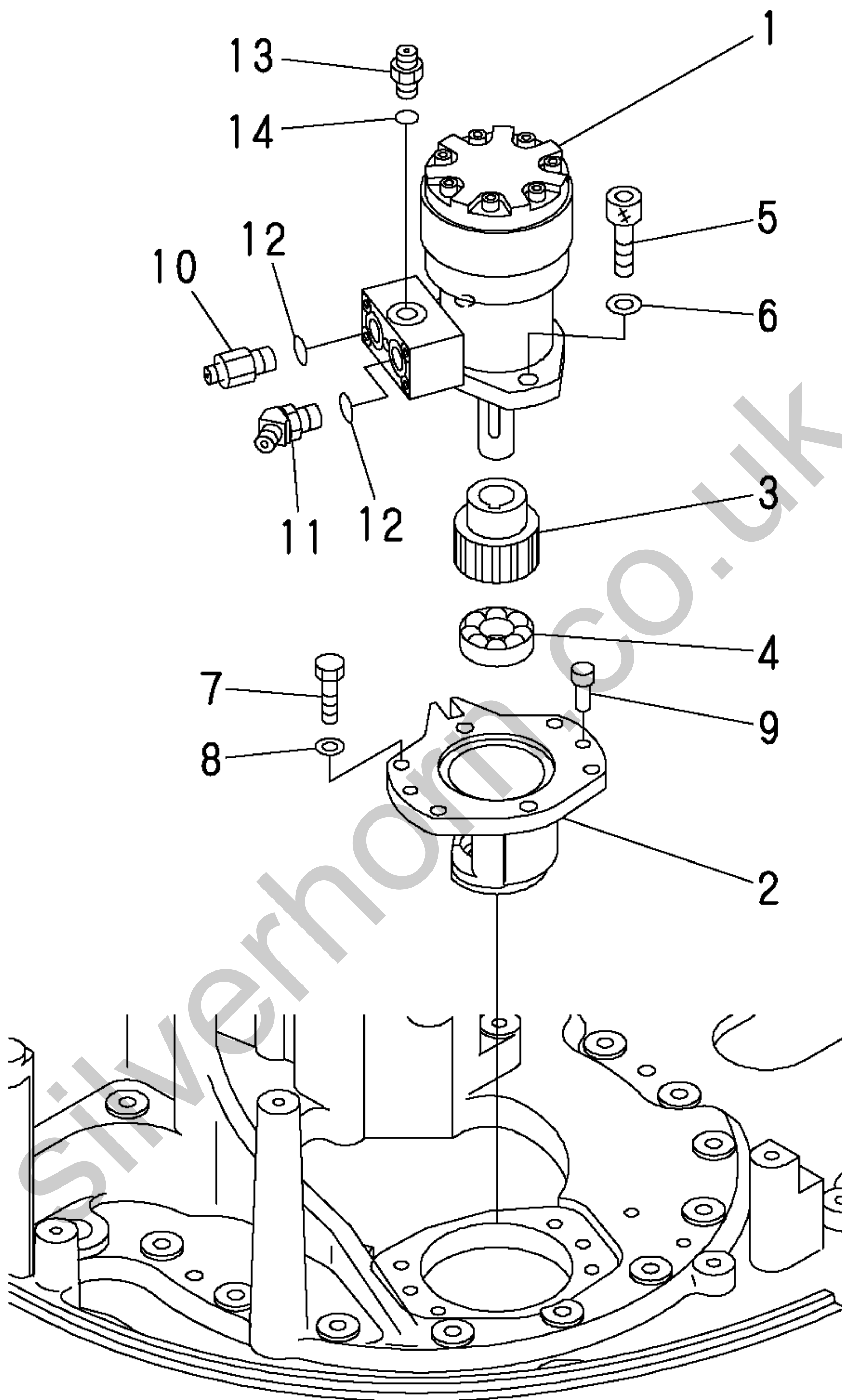
レボルピングフレーム REVOLVING FRAME
