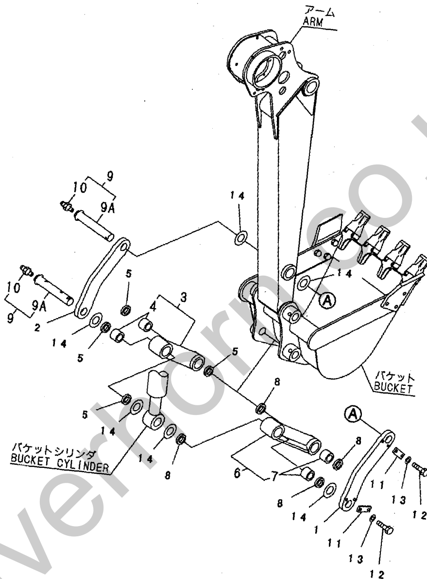
Fig. 99 バケットリンク BUCKET LINK
