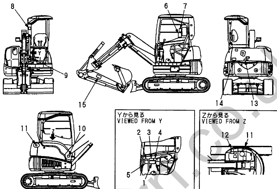
Fig. 108 安全銘板 SAFETY LABEL
