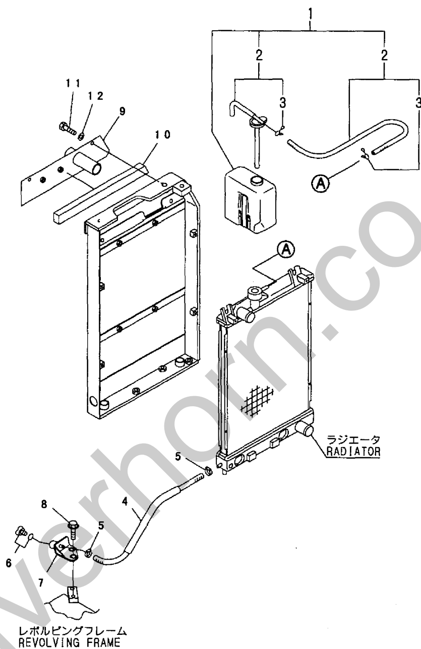
Fig. 7 サブタンク (ラジエータ) SUB TANK (RADIATOR)
