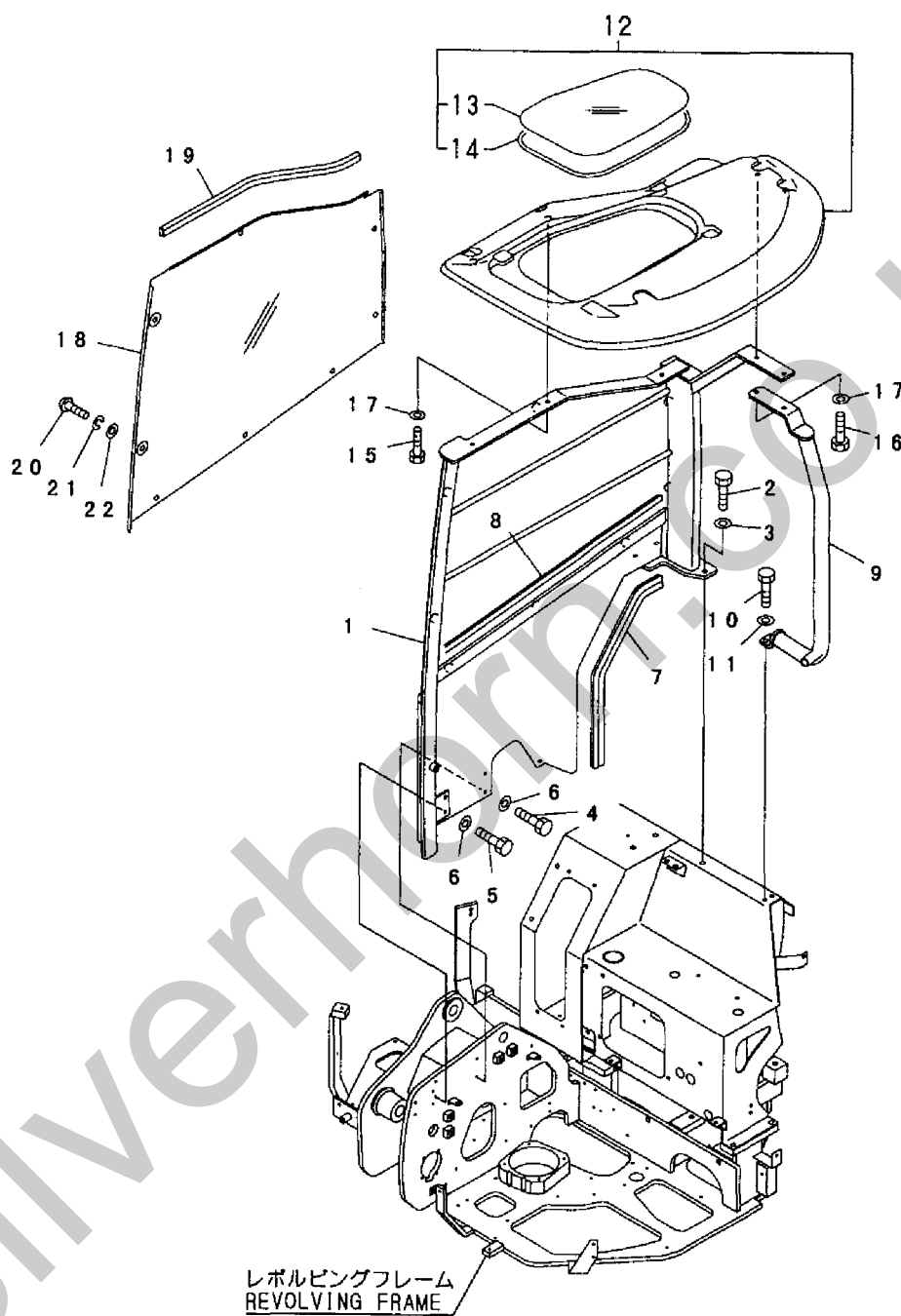
Fig. 34 キヤノピ CANOPY
