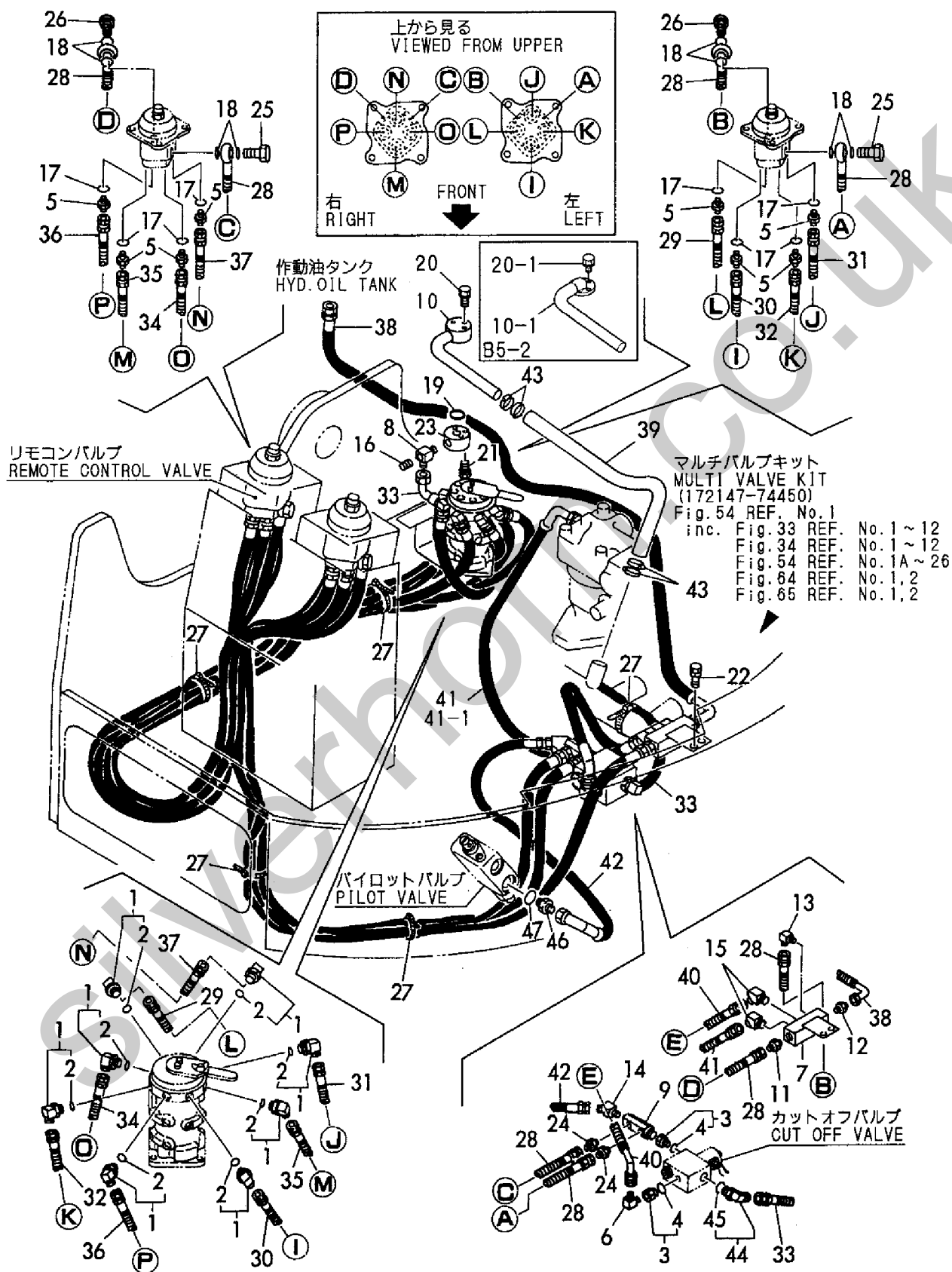
Fig. 64 コントロール配管 (リモコンバルブ~ロータリバルブ) CONTROL PIPING (REMO.-CON. VALVE ~ ROTARY VALVE)
