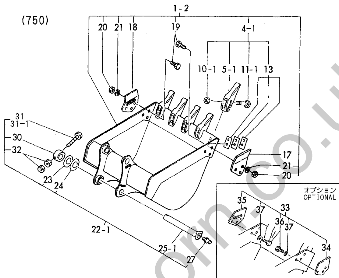
Fig. 77 バケット (700, 750) (アタッチメント) BUCKET (700, 750) (ATTACHMENT)
