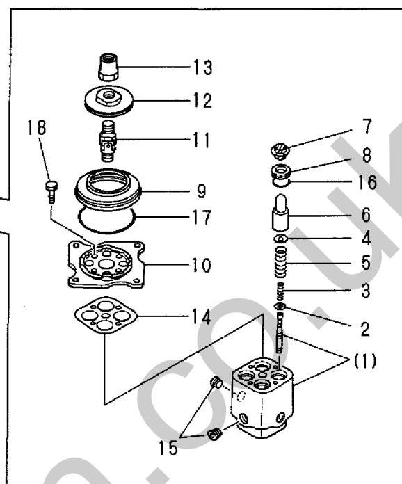
Fig. 53 リモコンバルブ&カットオフバルブ REMOTE CONTROL VALVE & CUT OFF VALVE
