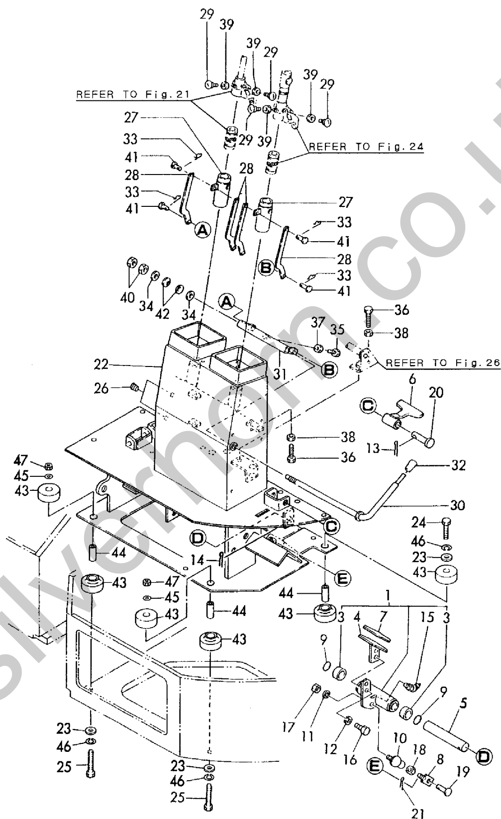
Fig. 18 操縦装置 (リンク台&レバーストッパ, マルチタイプ) CONTROL EQUIPMENT (LINK STAND & LEVER STOPPER, MULTI TYPE)
