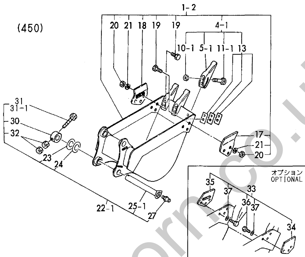
Fig. 74 バケット (400, 450) (アタッチメント) BUCKET (400, 450) (ATTACHMENT)
