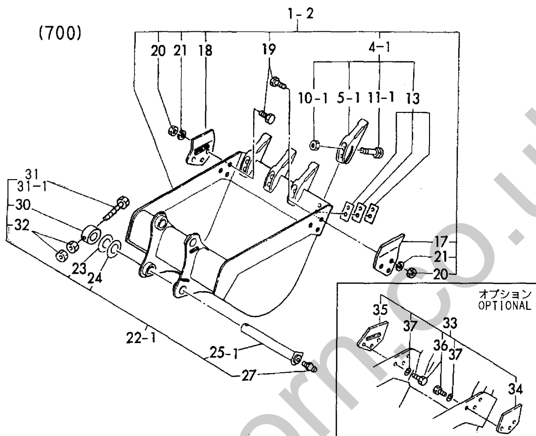
Fig. 76 バケット (650, 700) (アタッチメント) BUCKET (650, 700) (ATTACHMENT)
