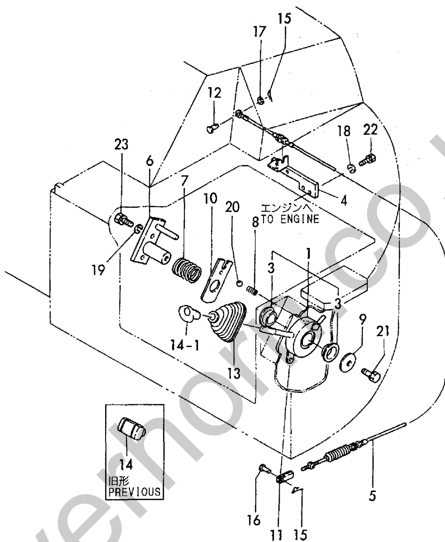
Fig. 6 アクセル ACCELERATOR
