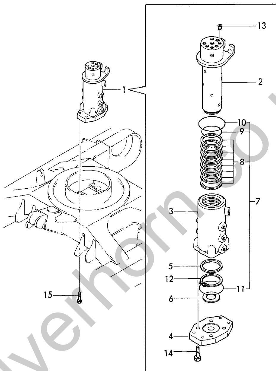
Fig. 47 スイベルジョイント SWIVEL JOINT
