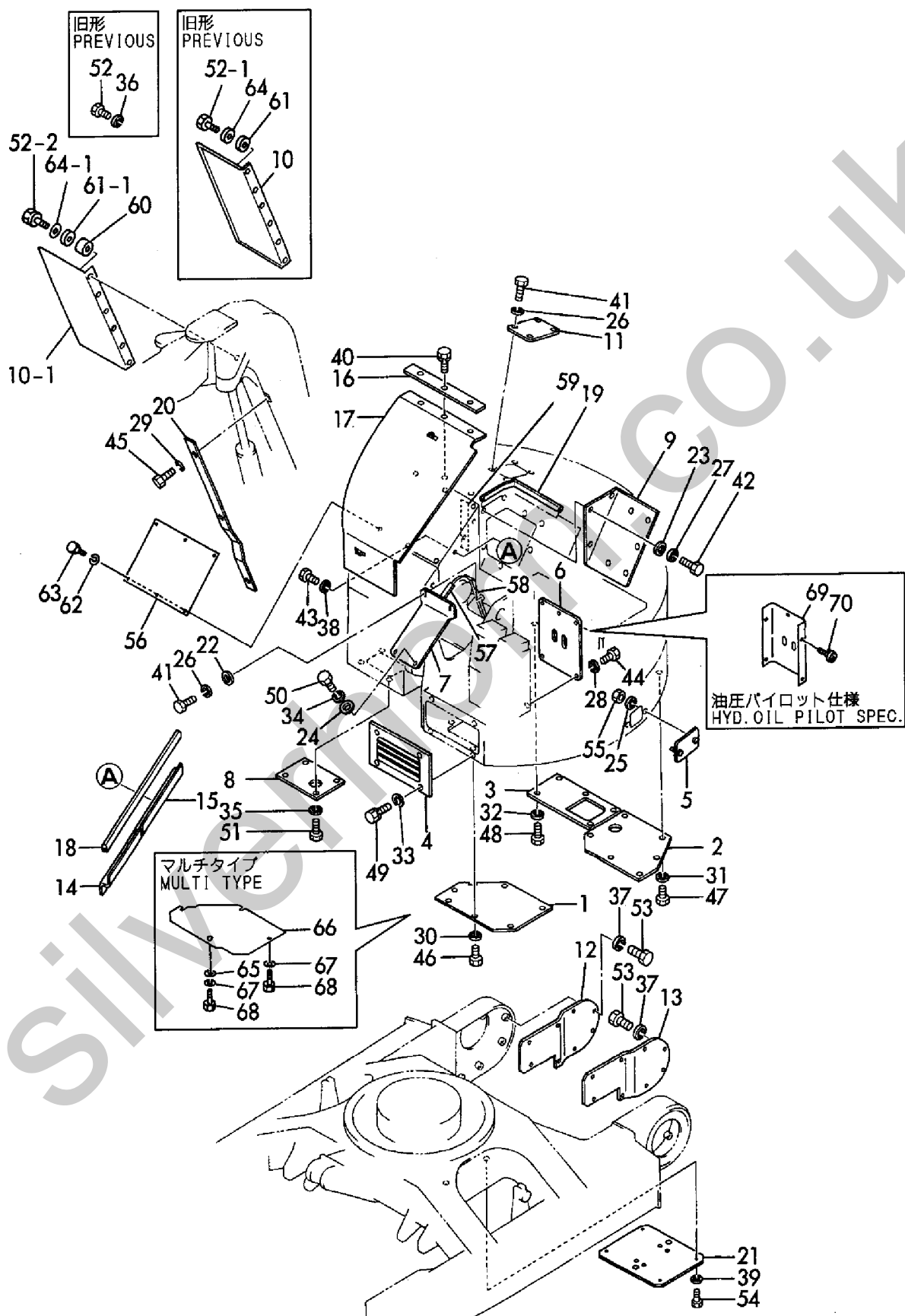
Fig. 32 フレームカバー FRAME COVER
