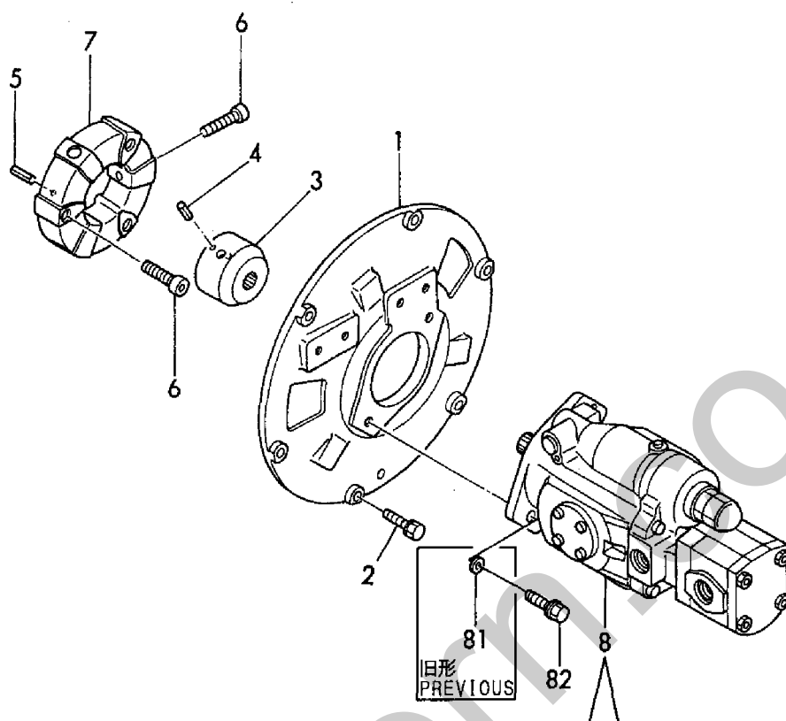
Fig. 36 油圧ポンプ&軸継手 HYD. OIL PUMP & JOINT
