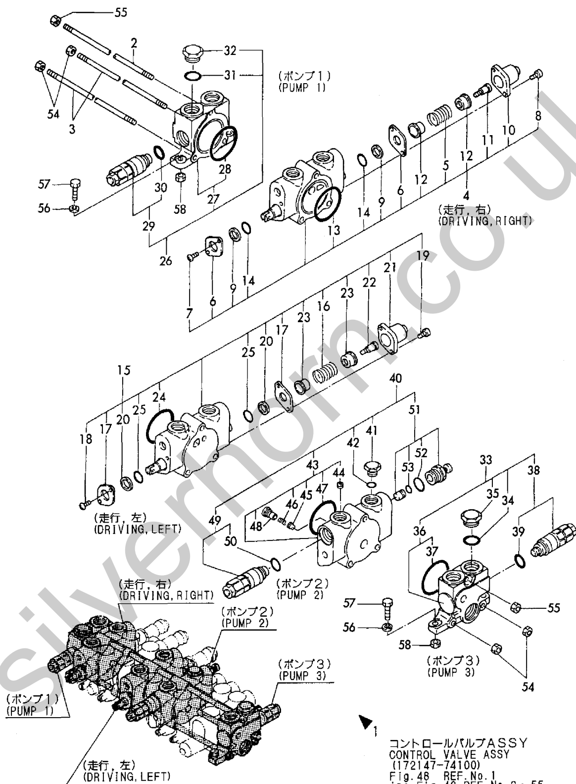
Fig. 48 コントロールバルブ (ポンプ&走行) CONTROL VALVE (PUMP & TRAVEL)
