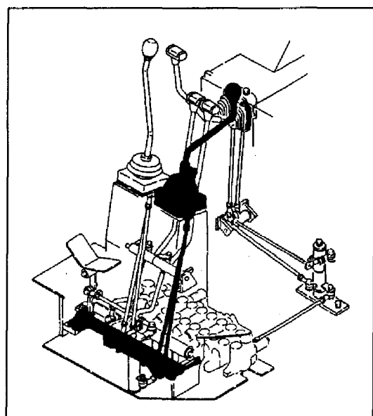
Fig. 24 操縦装置 (アーム&旋回, マルチタイプ) CONTROL EQUIPMENT (ARM & TURNING, MULTI TYPE)
