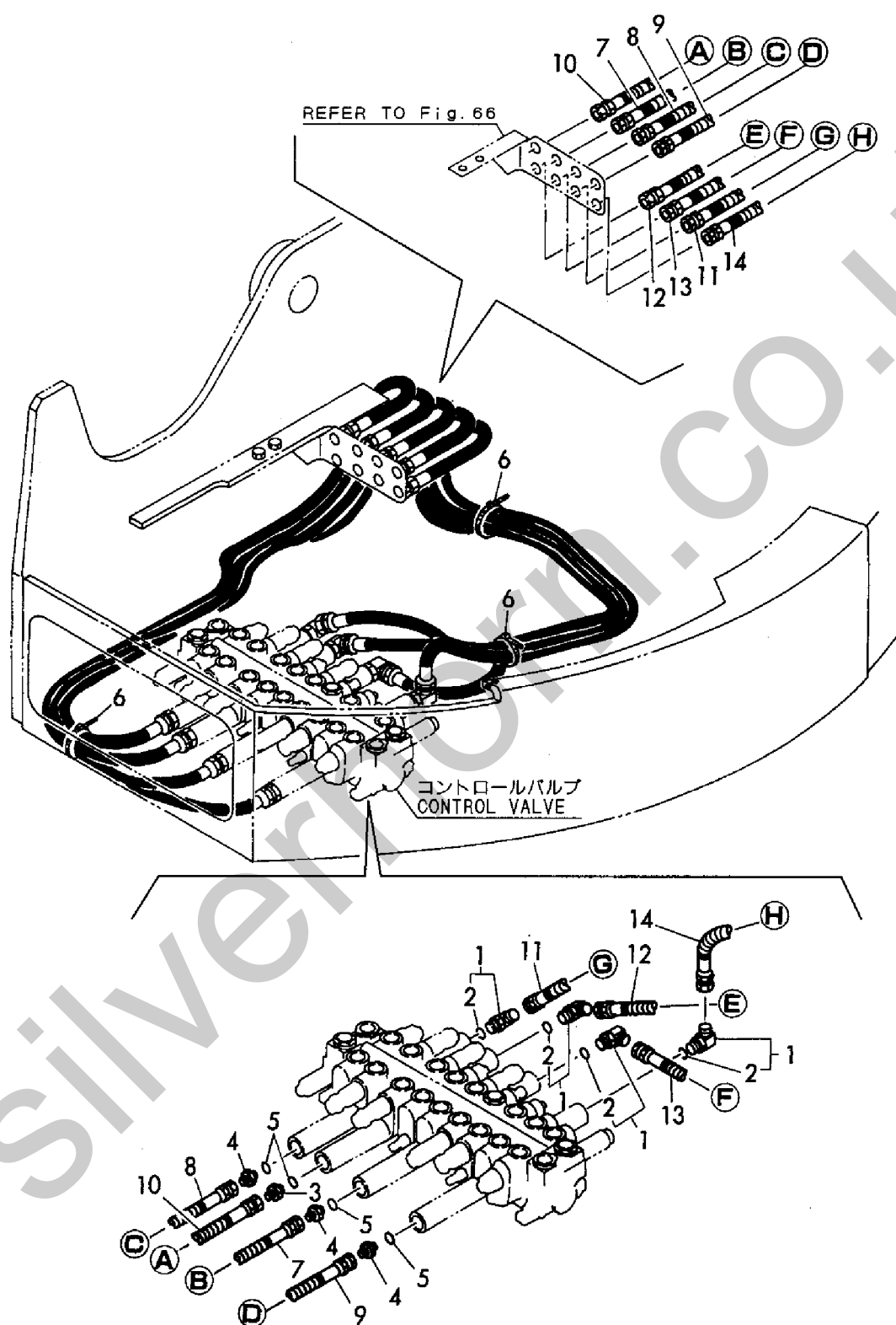
Fig. 67 コントロール配管 (隔壁~コントロールバルブ) CONTROL PIPING (PLATE ~ CONTROL VALVE)
