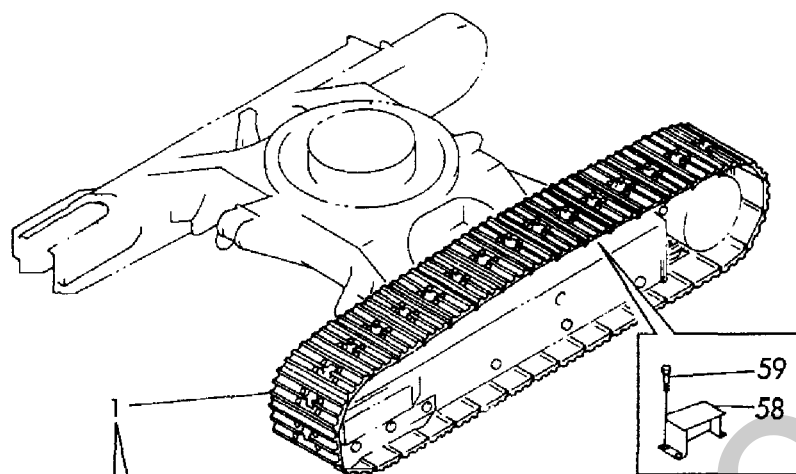
Fig. 16 クローラ (アタッチメント) CRAWLER (ATTACHMENT)
