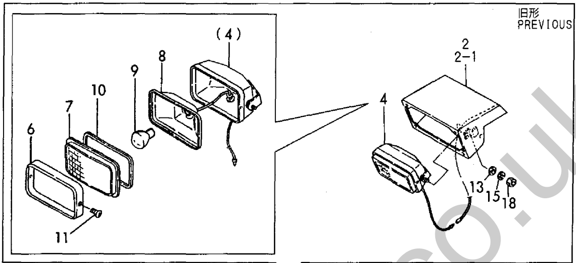
Fig. 12 ワークランプ WORK LAMP
