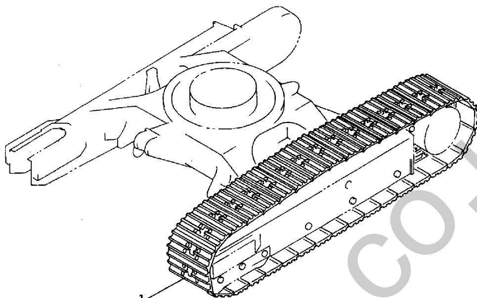
Fig. 15 クローラ (380) CRAWLER (380)
