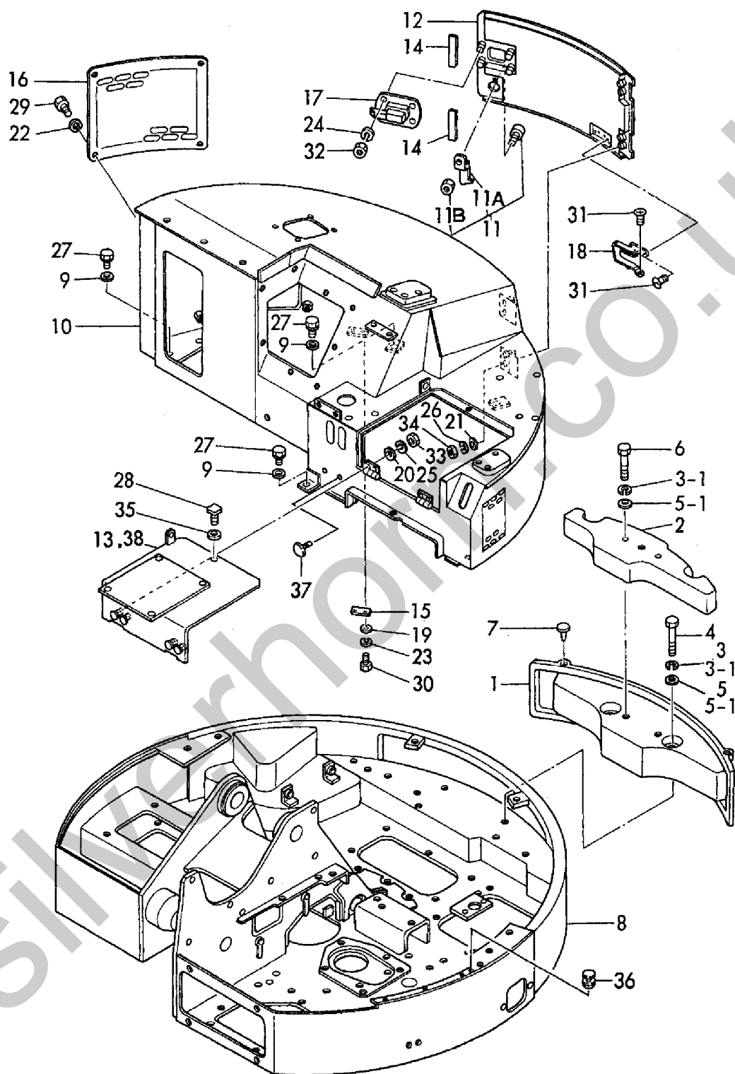
Fig. 30 旋回フレーム&ボンネット TURNING FRAME & BONNET
