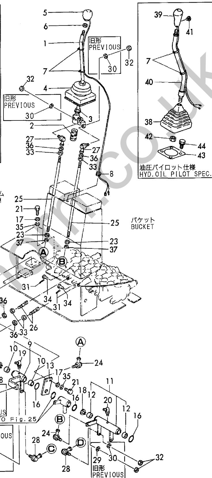
Fig. 20 操縦装置 (ブーム&バケット) CONTROL EQUIPMENT (BOOM & BUCKET)
