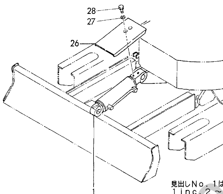
Fig. 41 ブレードシリンダ BLADE CYLINDER
