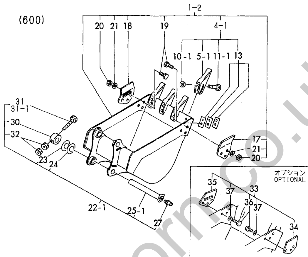
Fig. 75 バケット (550, 600) (アタッチメント) BUCKET (550, 600) (ATTACHMENT)
