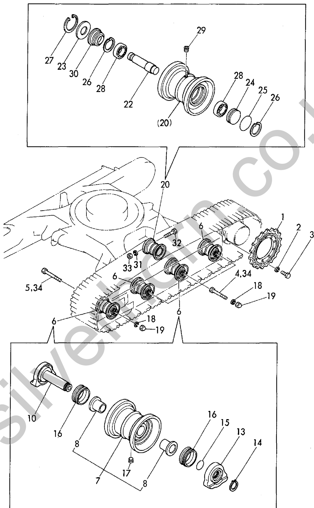
Fig. 13 ローラ&アジャスト ROLLER & ADJUST
