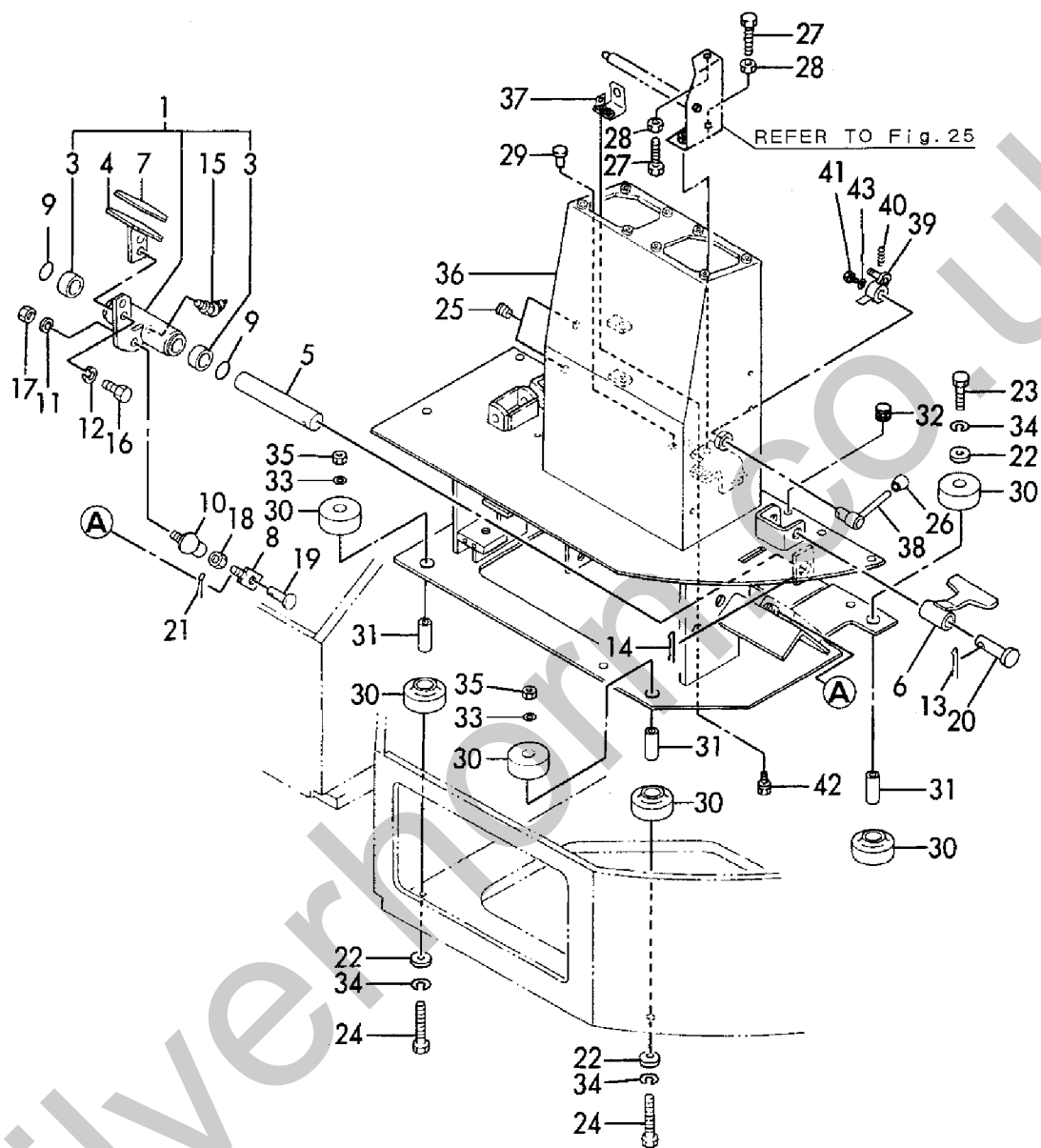
Fig. 19 操縦装置 (リンク台&レバーストップバ, 油圧パイロット) CONTROL EQUIPMENT (LINK STAND & LEVER STOPER, HYD. OIL PILOT)
