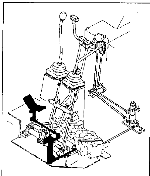
Fig. 27 操縦装置 (オフセット) CONTROL EQUIPMENT (OFFSET)
