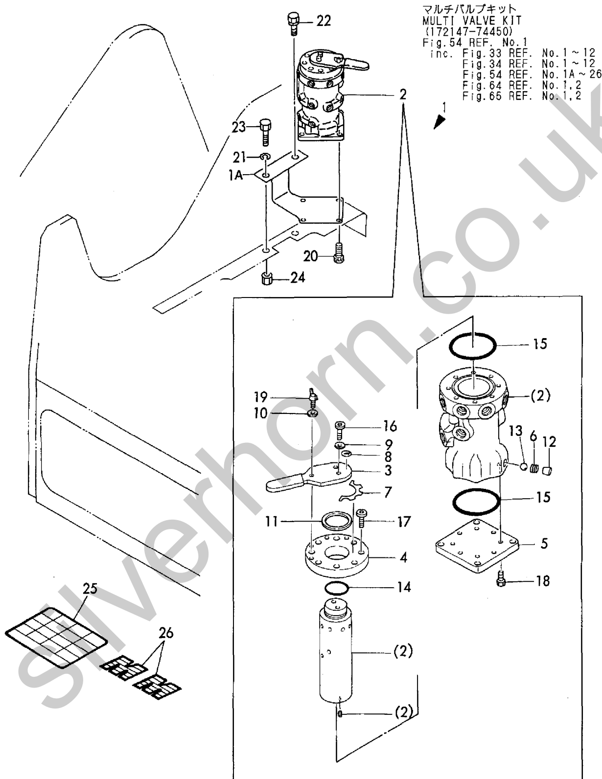
Fig. 54 ロータリバルブ (油圧マルチ) ROTARY VALVE (HYD. OIL MULTI)
