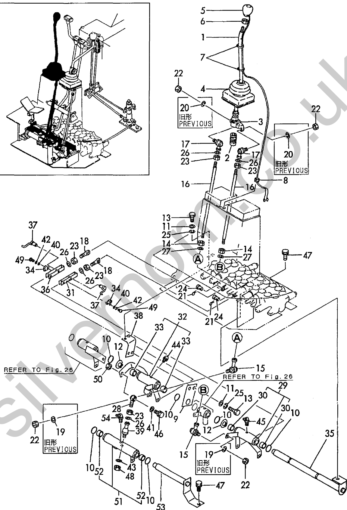
Fig. 21 操縦装置 (ブーム & バケット, マルチタイプ) CONTROL EQUIPMENT (BOOM & BUCKET, MULTI TYPE)
