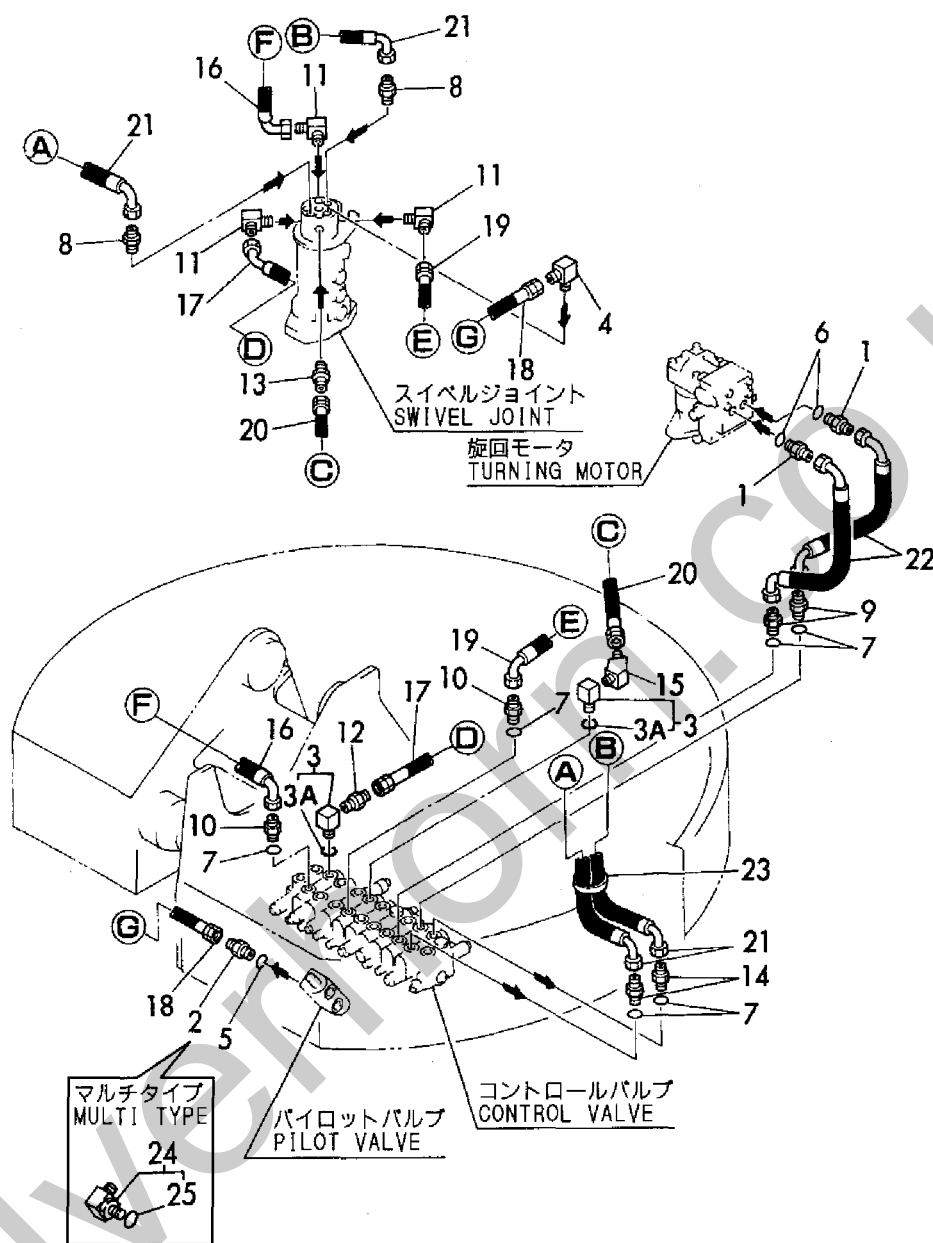
Fig. 59 油圧配管 (バルブ~スイベル~モータ) HYD. OIL PIPING (VALVE ~ SWIVEL ~ MOTOR)
