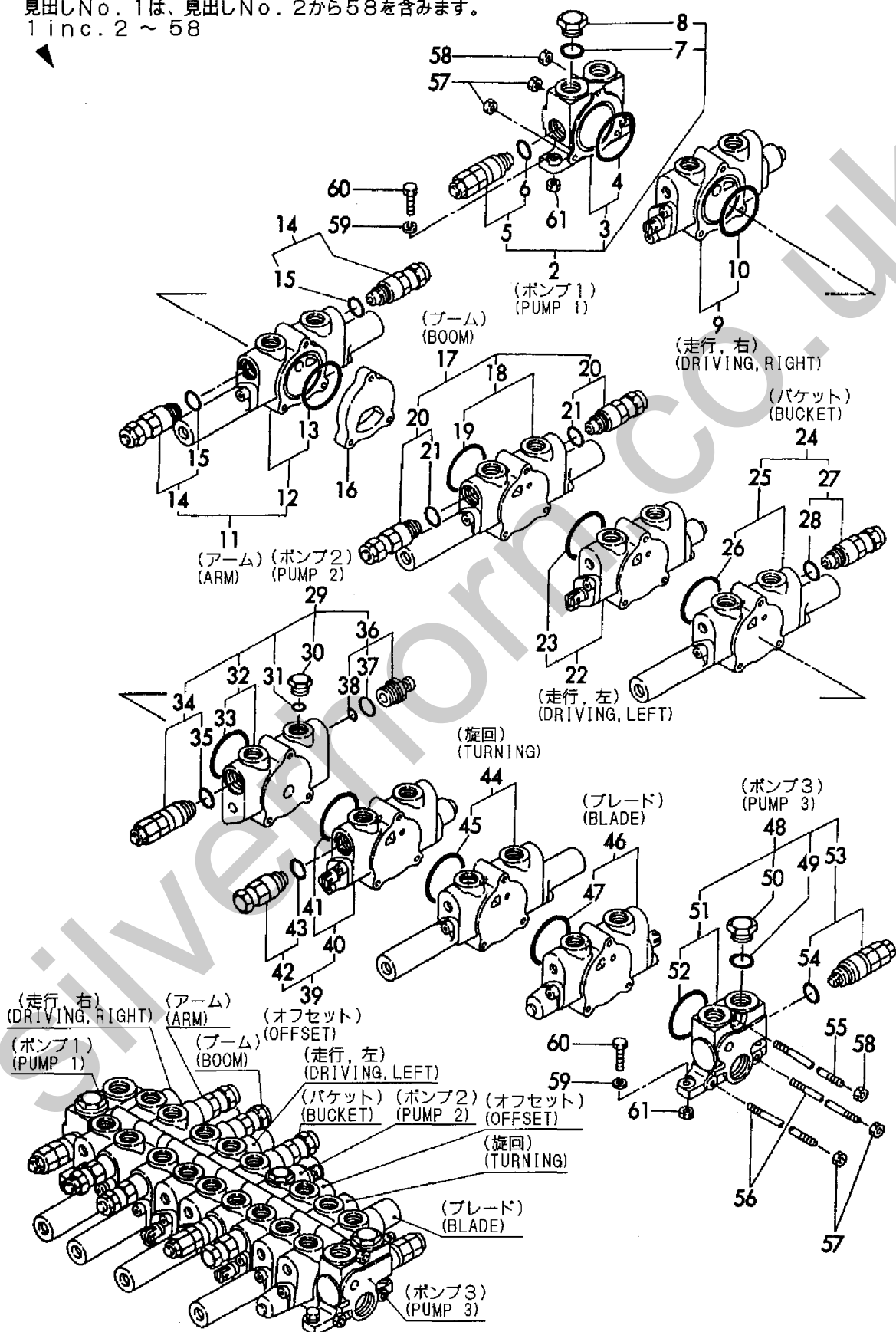
Fig. 51 コントロールバルブ (油圧パイロット) CONTROL VALVE (HYD. OIL PILOT)
