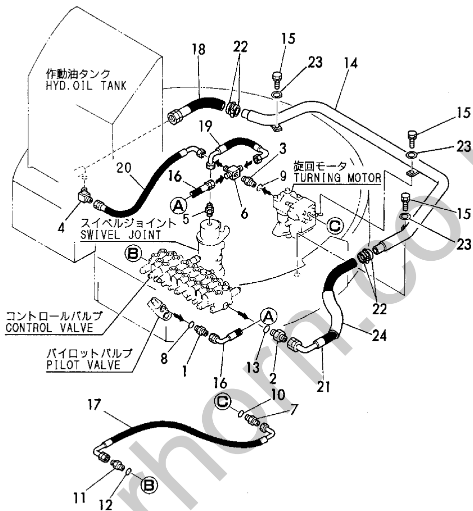
Fig. 61 油圧配管 (リターン) HYD. OIL PIPING (RETURN)
