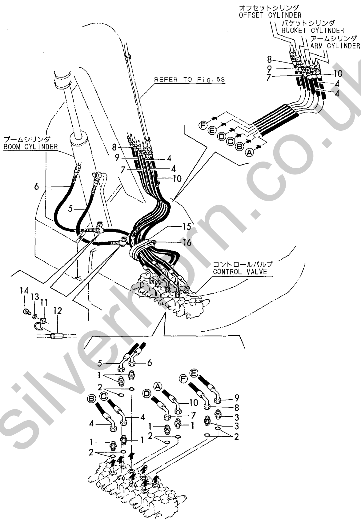
Fig. 58 油圧配管 (バルブ～ブーム) HYD. OIL PIPING (VALVE ~ BOOM)
