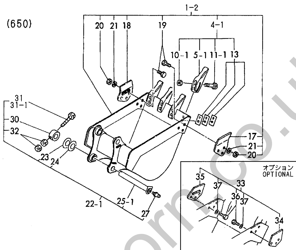
Fig. 73 バケット (600, 650) BUCKET (600, 650)
