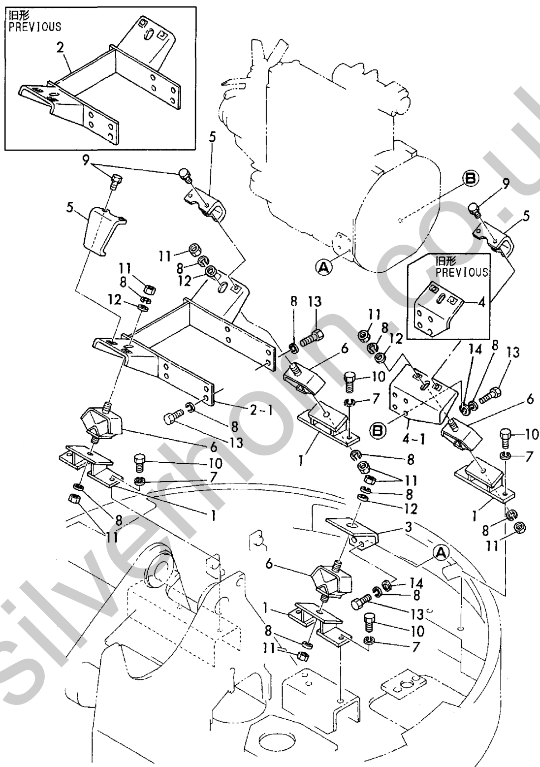
Fig. 7 エンジンマウント ENGINE MOUNT
