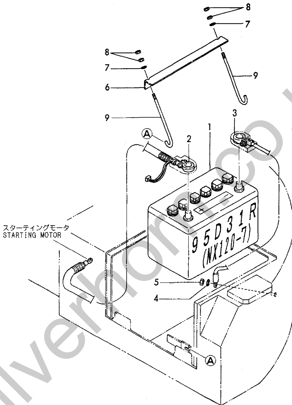
Fig. 10 バッテリ BATTERY
