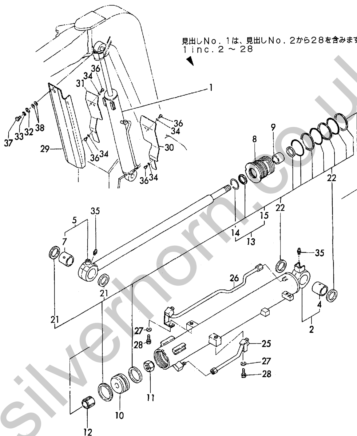
Fig. 37 ブームシリンダ BOOM CYLINDER
