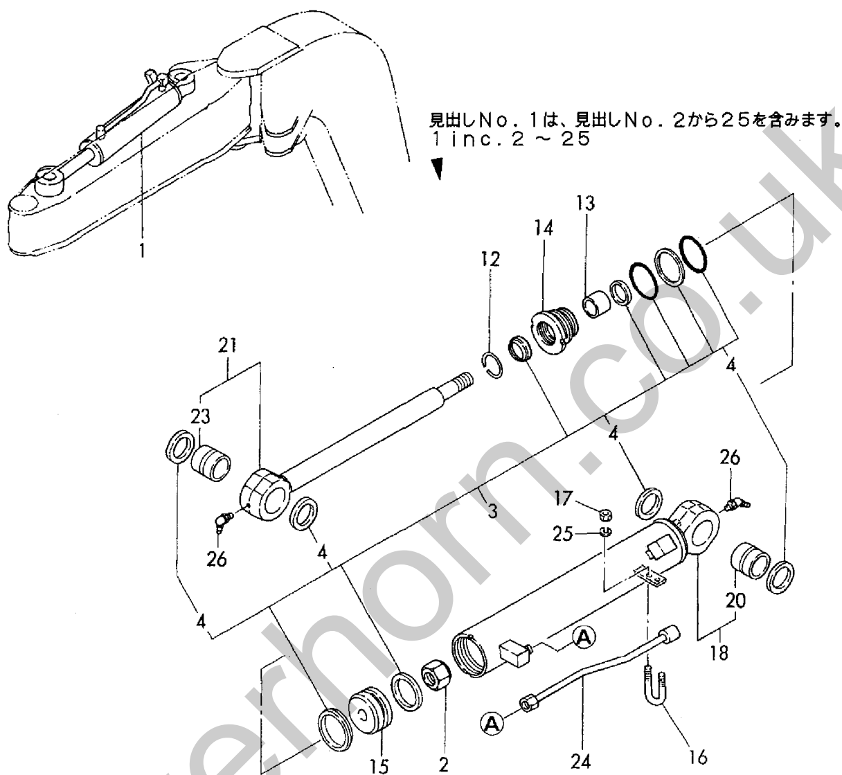
Fig. 40 オフセットシリンダ OFFSET CYLINDER
