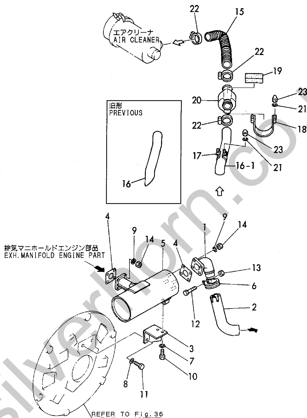
Fig. 5 サイレンサ&吸気パイプ SILENCER & SUCTION PIPE
