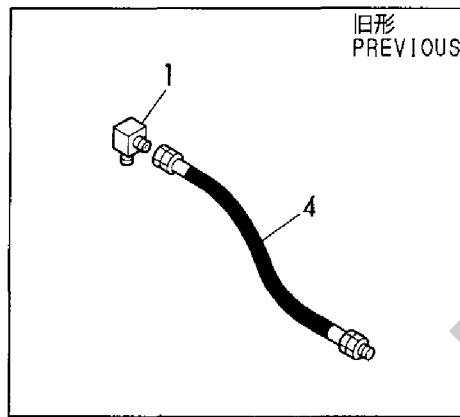
Fig. 68 グリーシング GREASING
