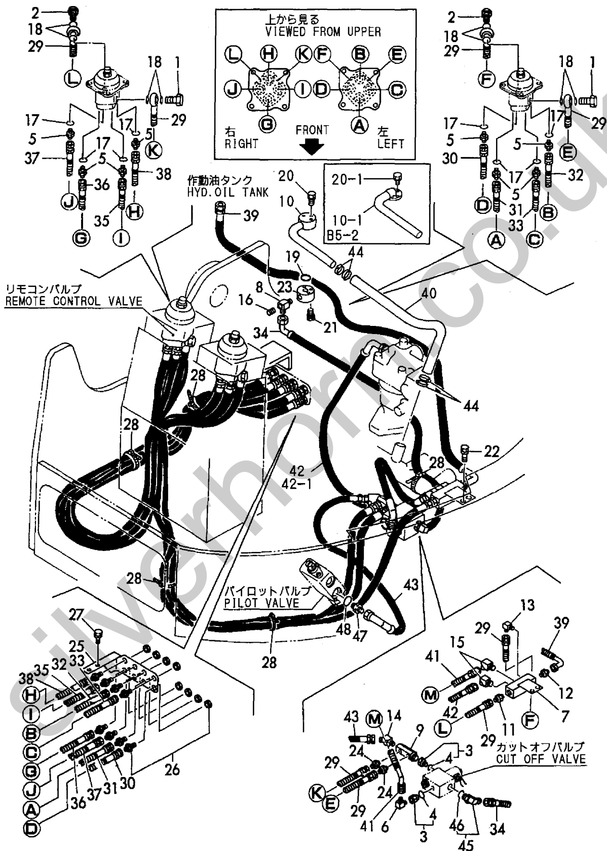
Fig. 66 コントロール配管 (リモコンバルブ~隔壁) CONTROL PIPING (REMO.-CON. VALVE ~ PLATE)
