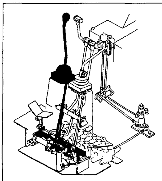
Fig. 21 操縦装置 (ブーム & バケット, マルチタイプ) CONTROL EQUIPMENT (BOOM & BUCKET, MULTI TYPE)
