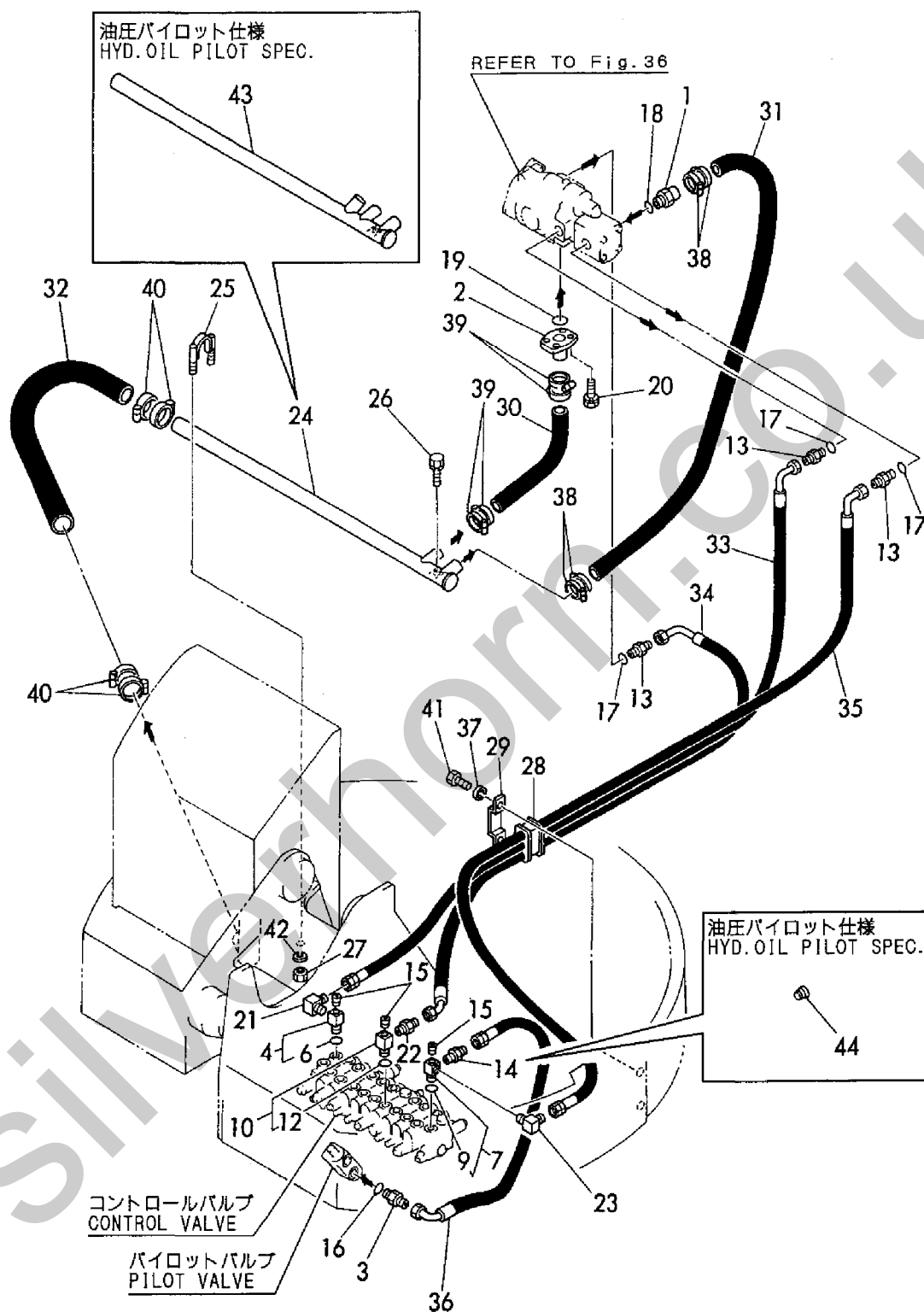
Fig. 57 油圧配管 (タンク~ポンプ~バルブ) HYD. OIL PIPING (TANK ~ PUMP ~ VALVE)
