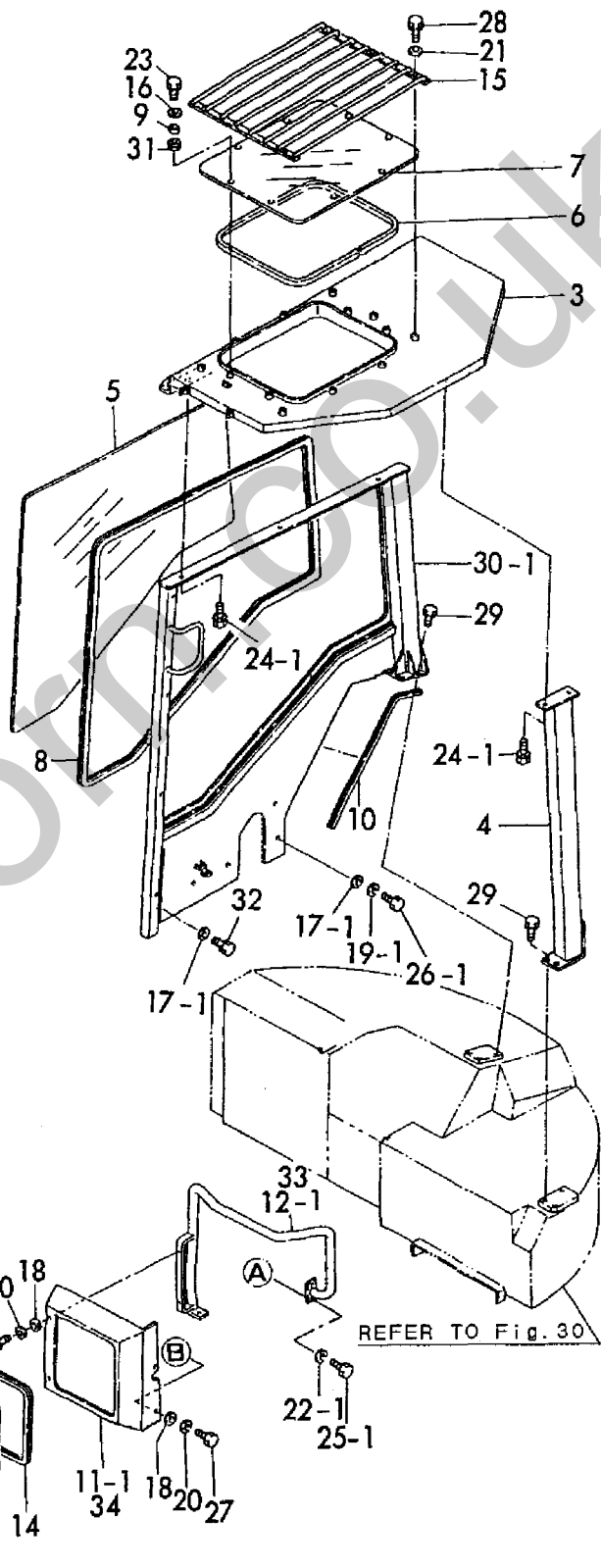
Fig. 35 キャンピ CANOPY
