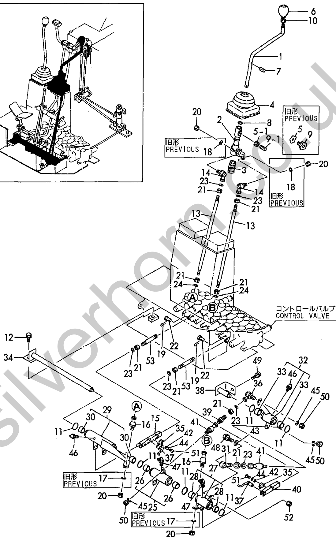
Fig. 24 操縦装置 (アーム&旋回, マルチタイプ) CONTROL EQUIPMENT (ARM & TURNING, MULTI TYPE)
