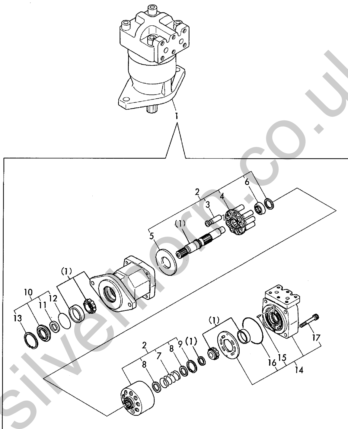
Fig. 44 旋回モーターインナーパーツ TURNING MOTOR COMPONENT PART
