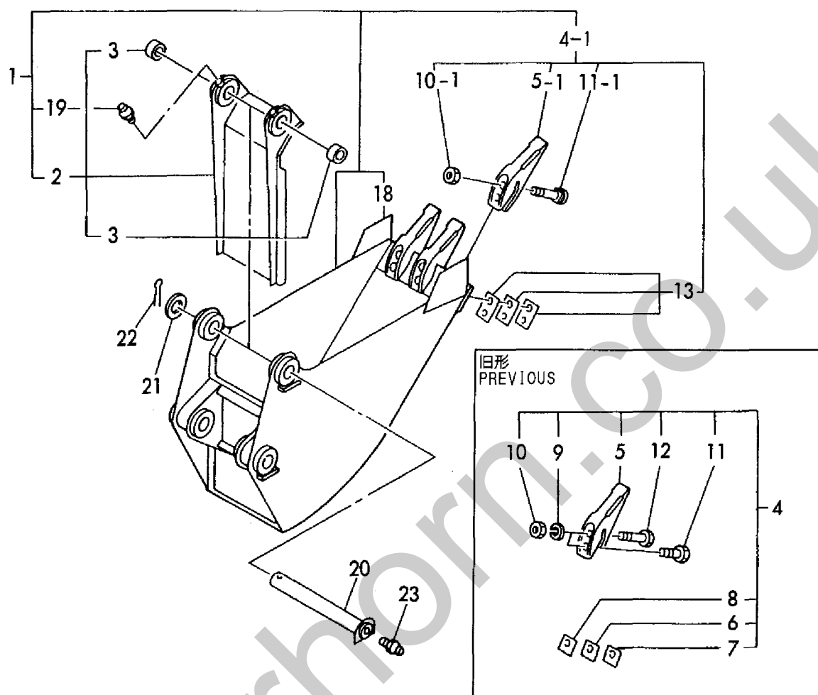
Fig. 78 バケット (330) (アタッチメント) BUCKET (330) (ATTACHMENT)
