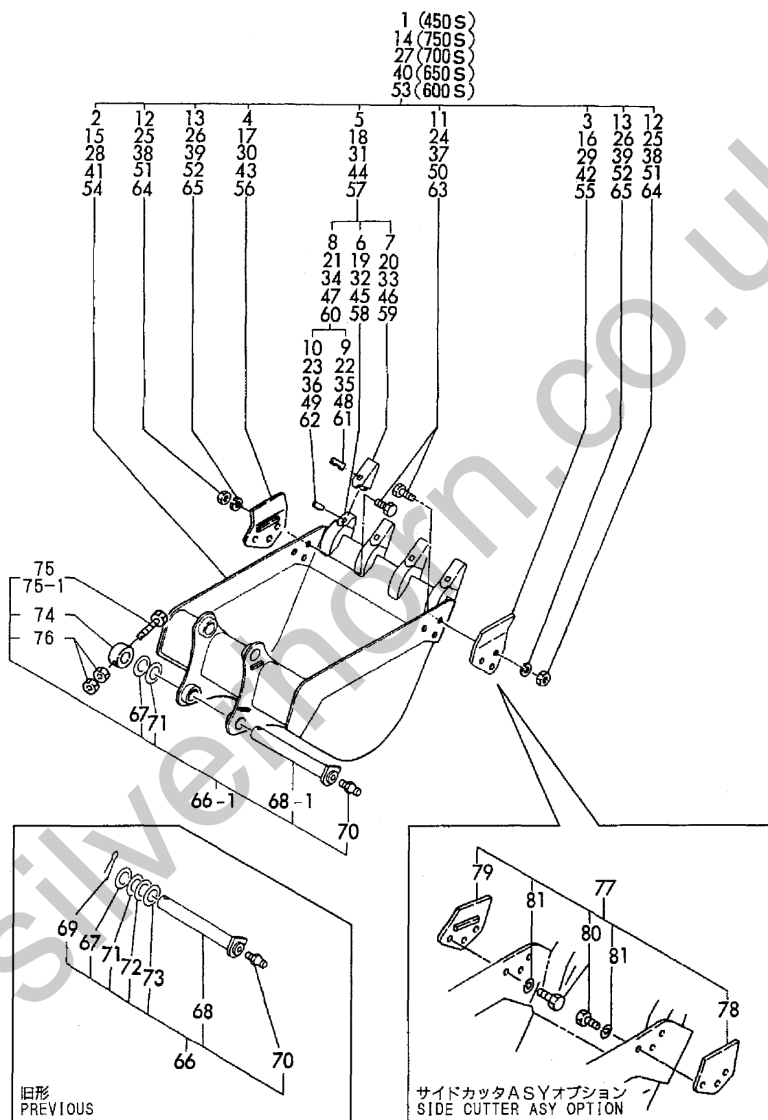
Fig. 79 バケットSタイプ (アタッチメント) BUCKET S TYPE (ATTACHMENT)
