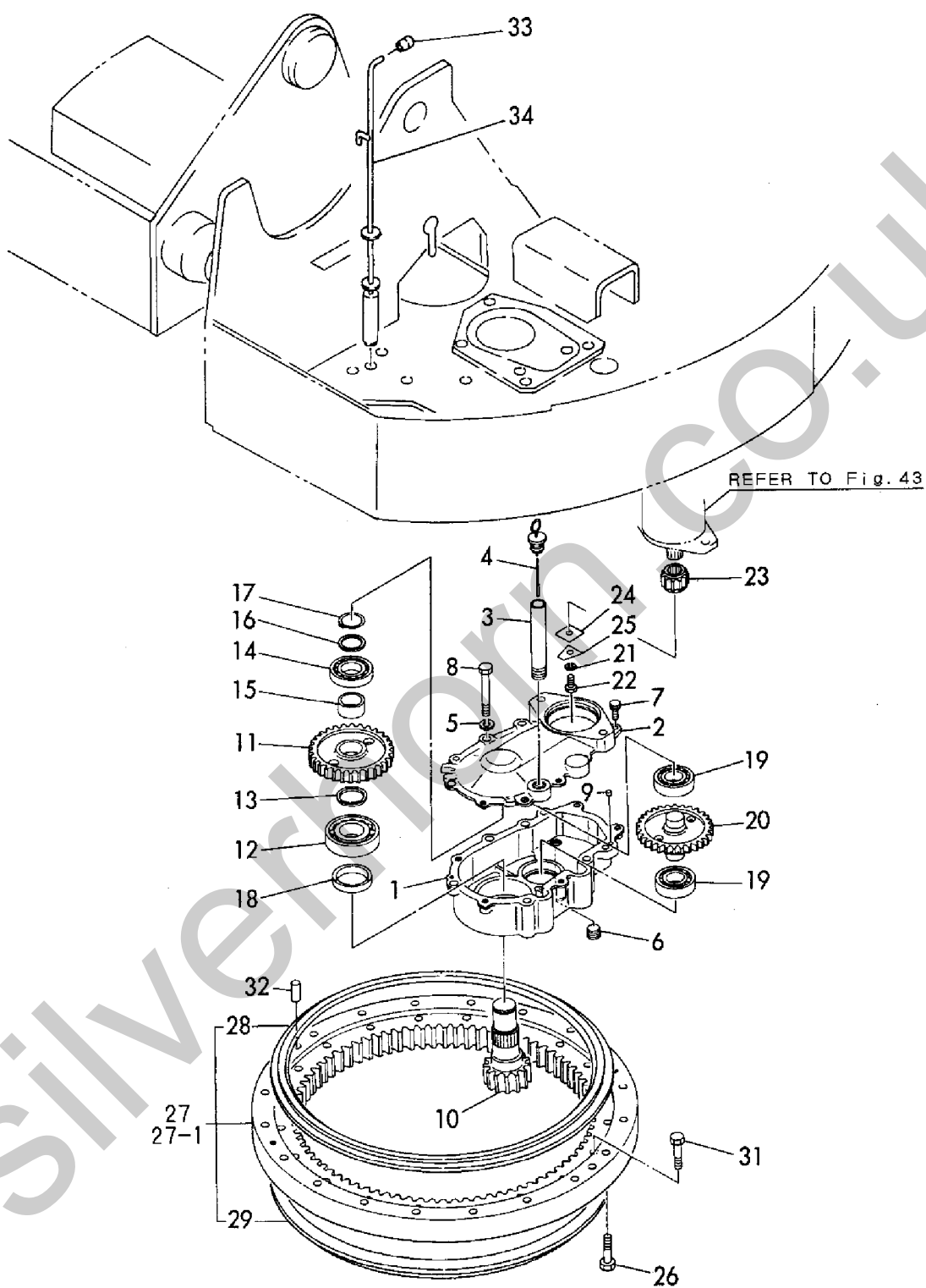
Fig. 31 旋回装置 TURNING DEVICE
