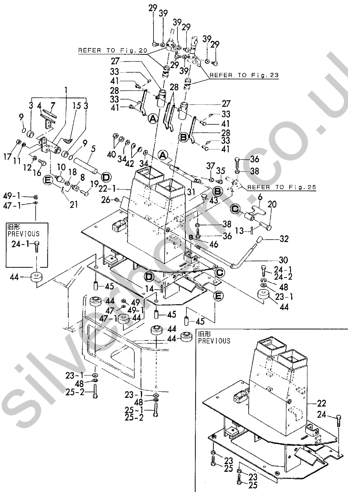
Fig. 17 操縦装置 (リンク台&レバーストッパ) CONTROL EQUIPMENT (LINK STAND & LEVER STOPER)
