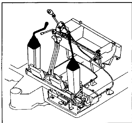
Fig. 27 操縦装置(レバー & スタンド:フロントレバー) CONTROL EQUIPMENT (LEVER & STAND: FRONT LEVER)
