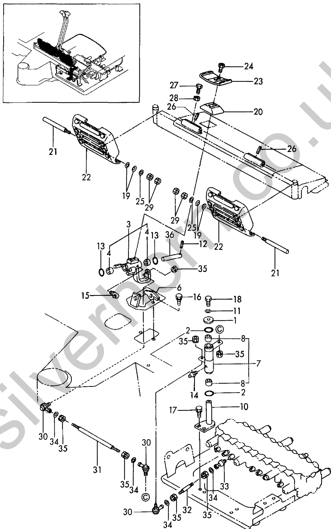
Fig. 31 操縦装置(スイング) CONTROL EQUIP. (SWING)
