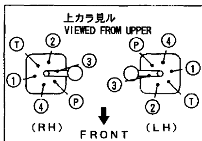
Fig. 89 コントロール配管(ポンプ～リモコンバルブ～リターン :サイドレバー-AS仕様) CONTROL PIPING(PUMP~REMO.-CON. V.~RETURN :SIDE LEVER AS SPEC.)
