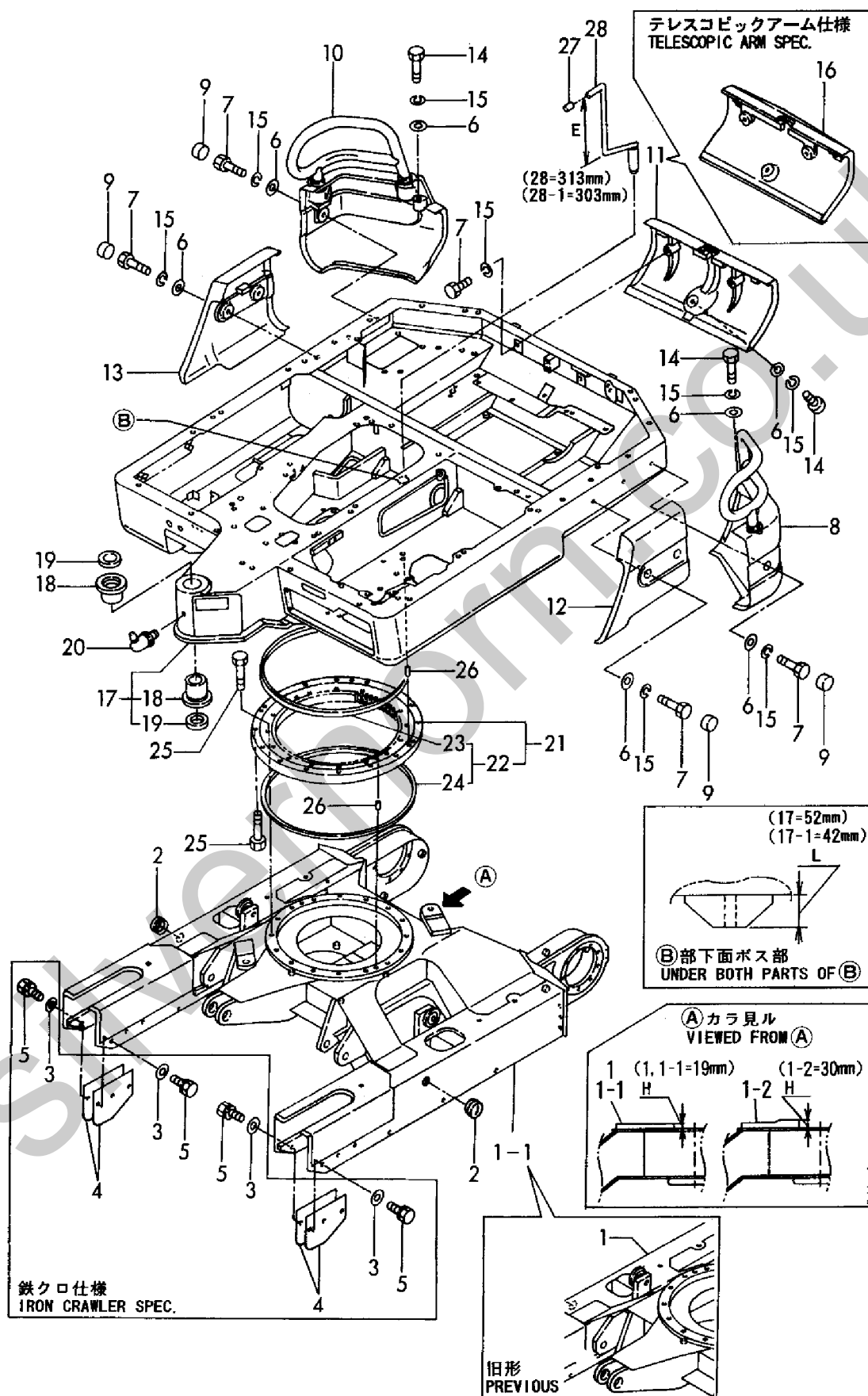
Fig. 36 フレーム & 旋回ベアリング FRAME & TURNING BEARING
