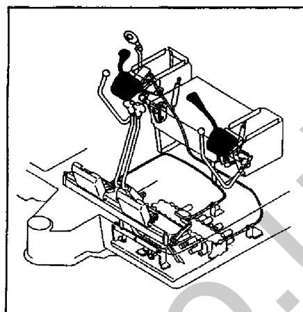
Fig. 28 操縦装置(レバー & スタンド:サイドレバー) CONTROL EQUIPMENT(LEVER & STAND:SIDE LEVER)
