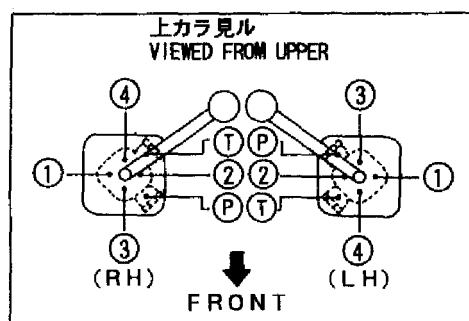
Fig. 90 コントロール配管(リモコンバルブ ~コントロールバルブ :ダイレクト, フロントレバー) CONTROL PIPING(REMO. -CON. V. ~CONTROL V. :DIRECT, FRONT LEVER)
