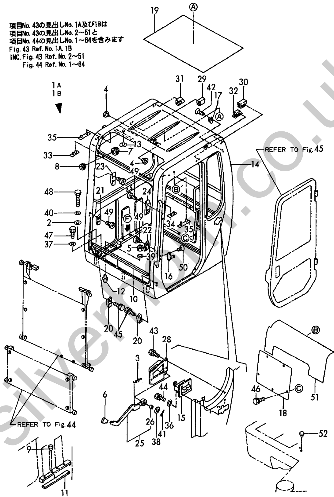
Fig. 43 キャビン(本体 & 付属) CABIN(BODY & FITTING PART)
