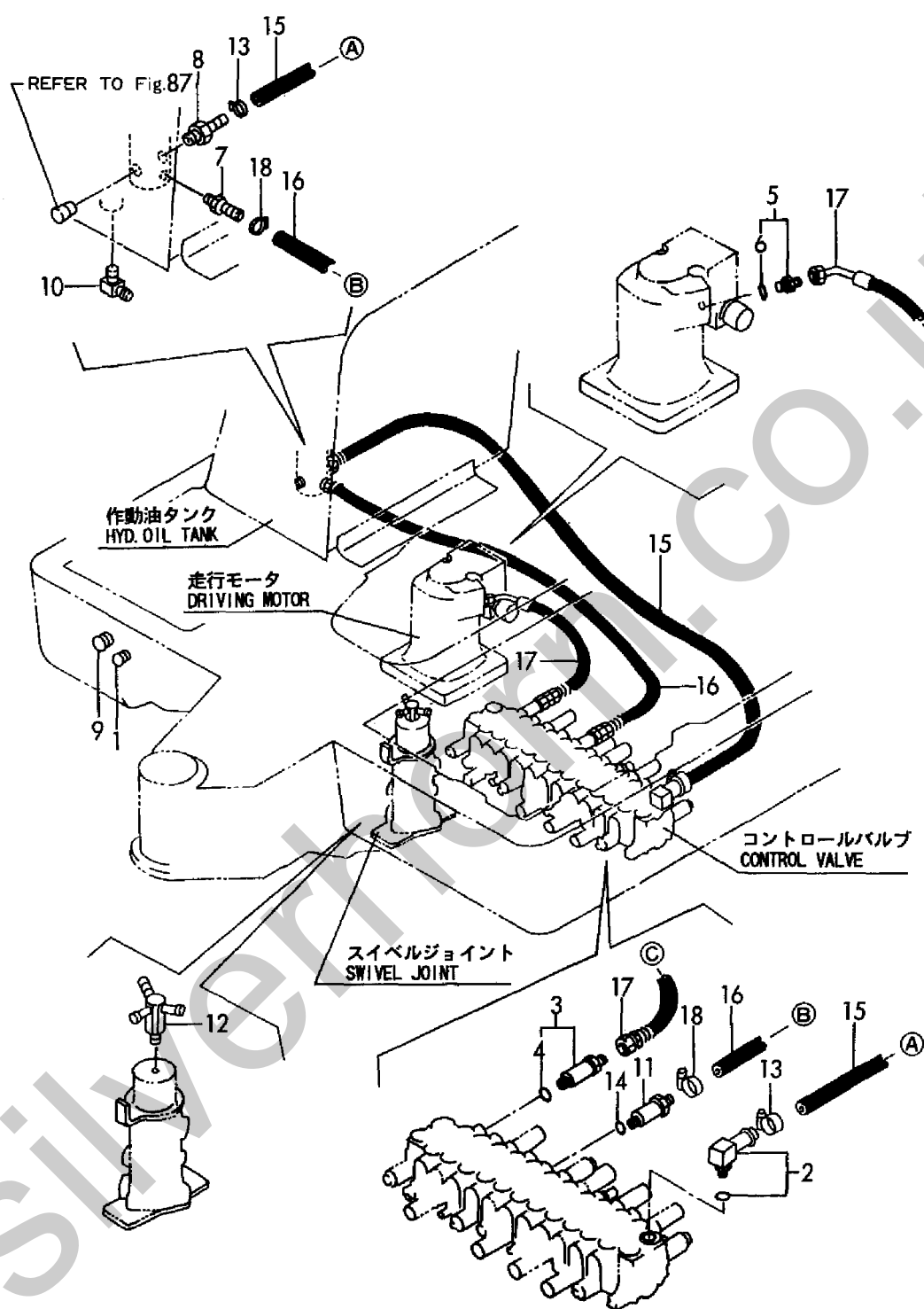
Fig. 79 油圧配管(リターン) HYD. OIL PIPING(RETURN)
