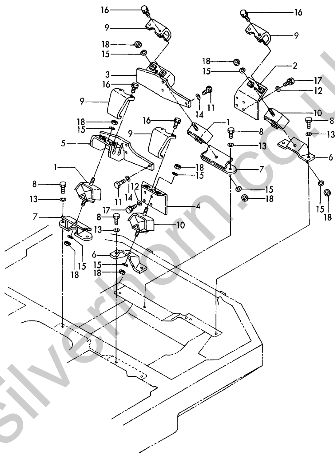
Fig. 13 エンジンマウント ENGINE MOUNT
