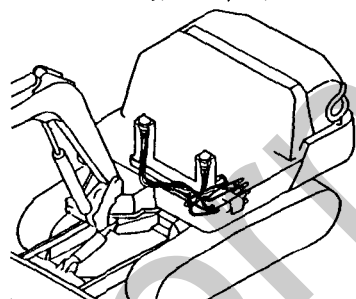
Fig. 91 コントロール配管 (リモコン・レバー～コントロール・レバー :ダイレクト, サイドレバー JP, EX仕様) CONTROL PIPING(REMO.-CON. V.～CON. V.:DIRECT, SIDE LEVER JP, EX SPEC.)
