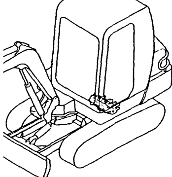
Fig. 68 コントロールバルブ (旋回 & ブレード : PTO仕様) CONTROL VALVE (TURNING & BLADE : P.T.O. SPEC.)
