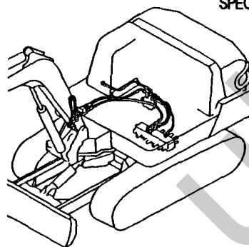
Fig. 82 油圧配管(トラックフレーム) HYD. OIL PIPING (TRACK FRAME)
