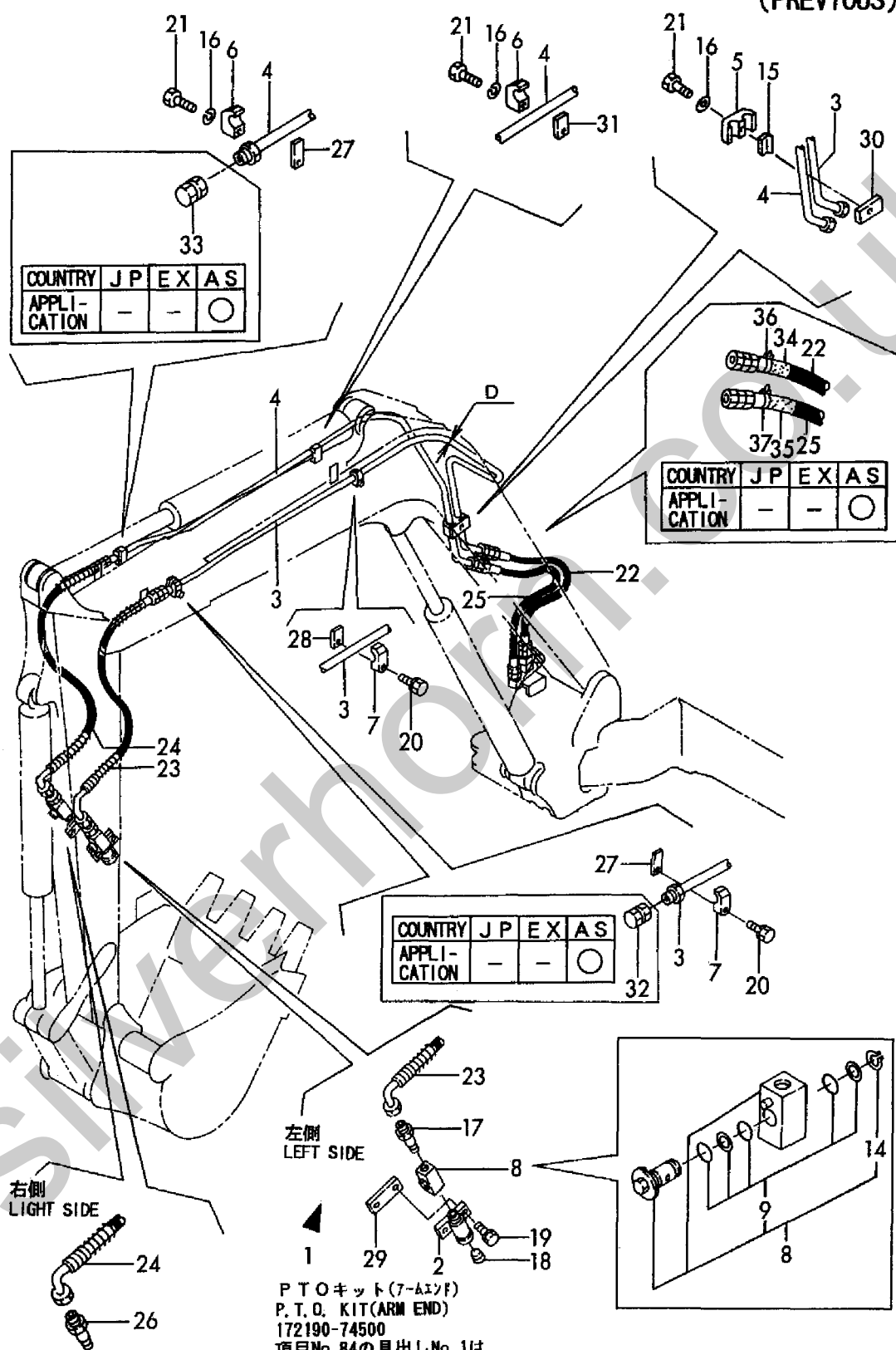
Fig. 84 油圧配管(PTO7-アームエンド仕様)(旧形) HYD. OIL PIPING(P. T. O. BOOM: ARM END SPEC.) (PREVIOUS)
