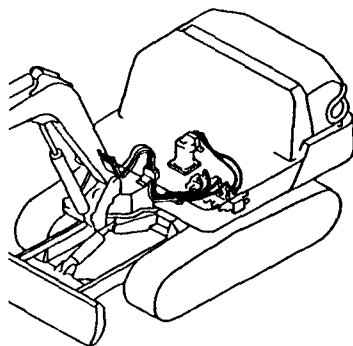
Fig. 78 油圧配管(ハルブ) ~スィベル、スイング~ HYD. OIL PIPING(VALVE ~SWIVEL, SWING)
