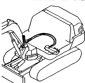
Fig. 80 油圧配管(P.T.O. フレームエンド) :単流仕様~ HYD. OIL PIPING(P. T. O. FRAME END:UNIFLOW SPEC.)
