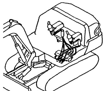
Fig. 92 コントロール配管 (リモコン・レバー～コントロール・レバー :ダイレクト, サイドレバー AS仕様) CONTROL PIPING(REMO.-CON. V.～CON. V.:DIRECT, SIDE LEVER AS SPEC.)
