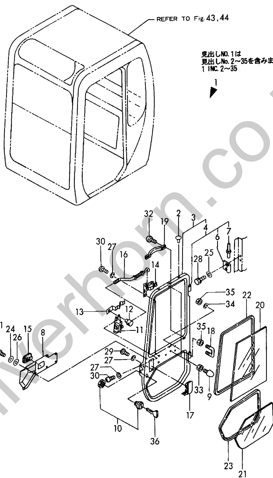
Fig. 45 キャビンドア CABIN DOOR
