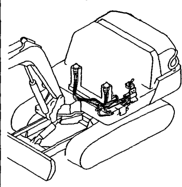
Fig. 96 コントロール配管 (2ウェイ:フロントレバー) CONTROL PIPING (2-WAY:FRONT LEVER)
