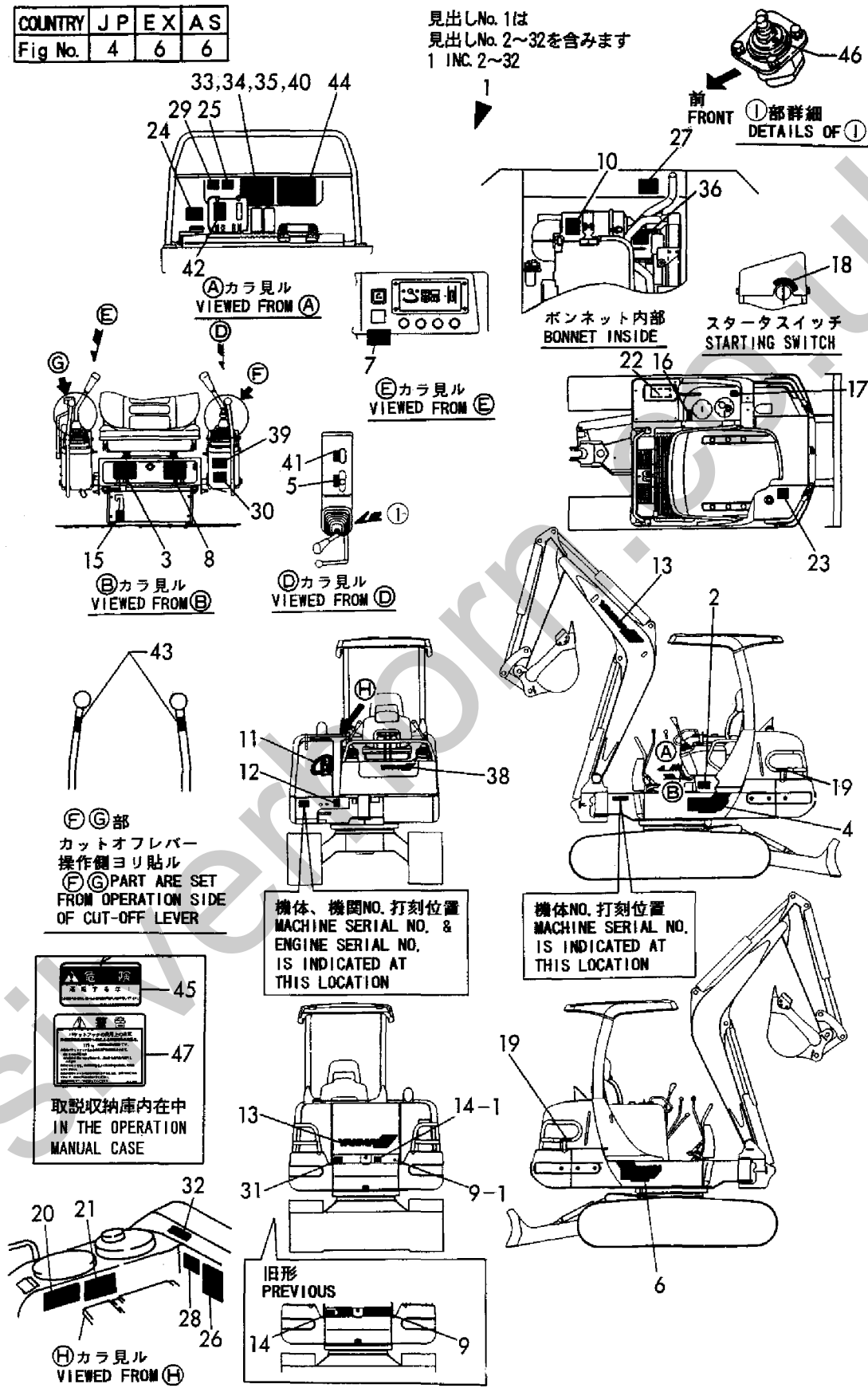
Fig. 4 銘板(キャノピー:サイドレバー) LABEL(CANOPI:SIDE LEVER)
