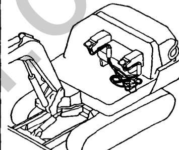
Fig. 95 コントロール配管 (マルチ・レバー～コントロール・レバー :4ウェイ) CONTROL PIPING (MULTI V.～CON. V.:4-WAY)
