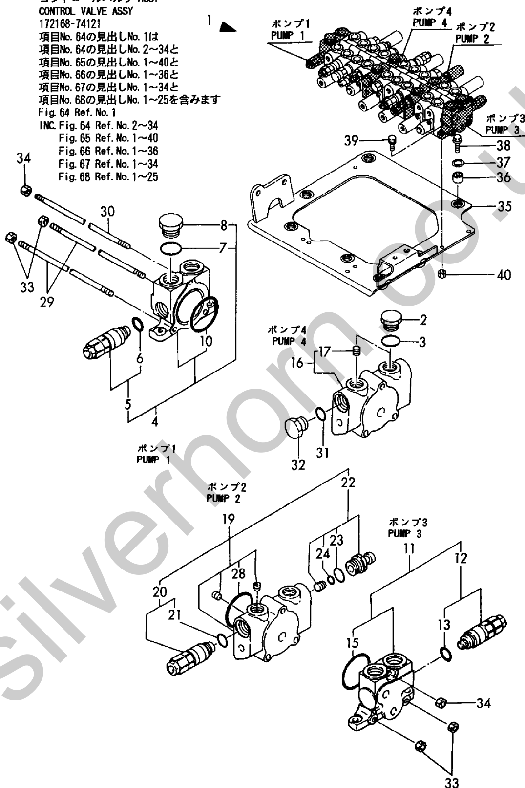
Fig. 64 64 コントロールバルブ(Pポート & バルブ台:PTO仕様) CONTROL VALVE(P PORT & VALVE STAND :P. T. O. SPEC.)
