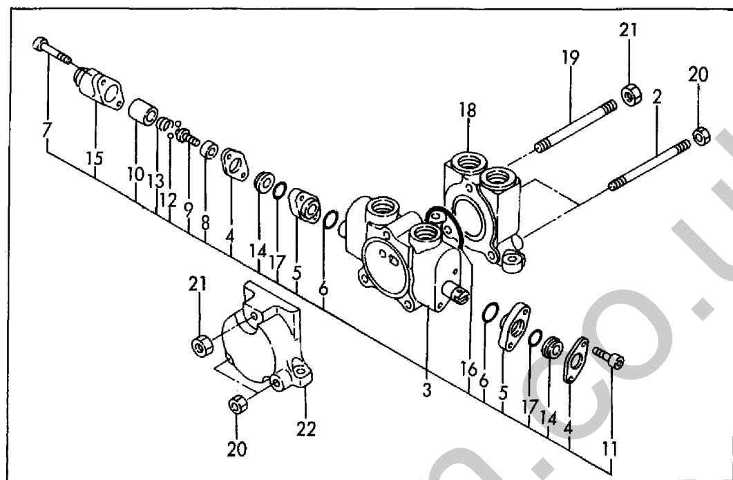
Fig. 74 P.T.O.バルブ(合流) P. T. O. VALVE(CONFLUENCE)
