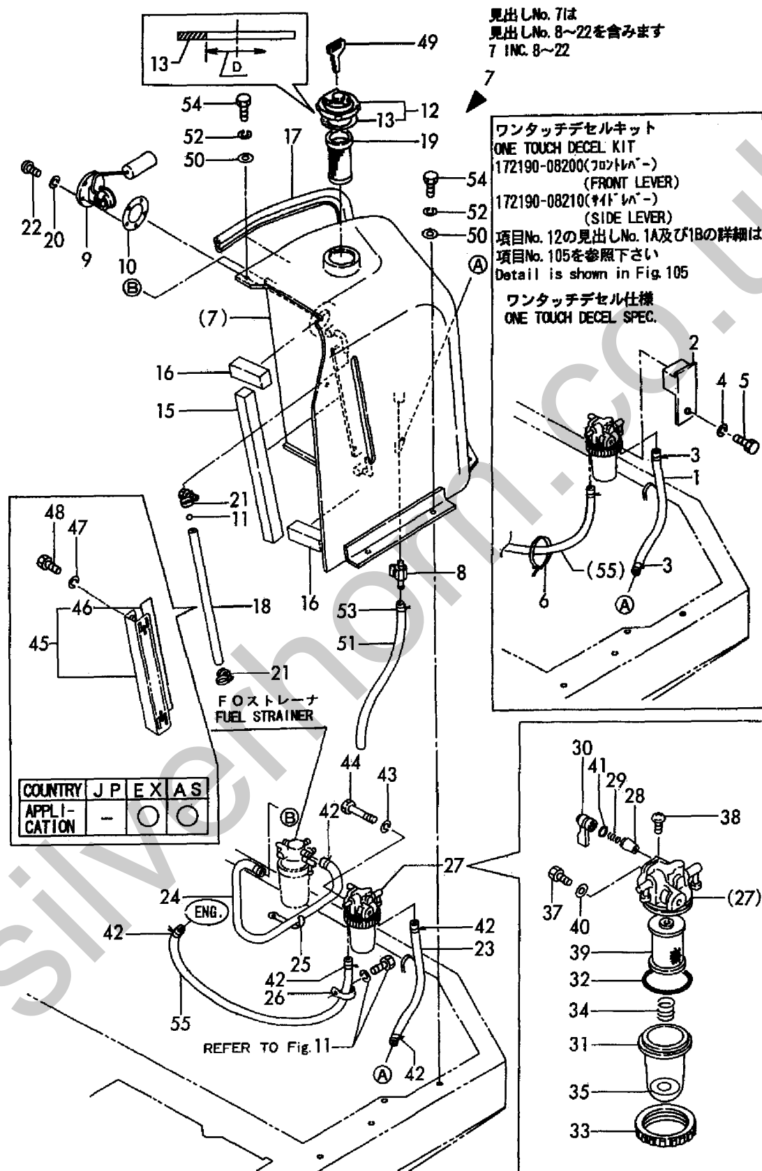
Fig. 15 FOタンク & FOパイプ FUEL TANK & FUEL LINE
