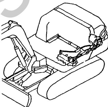
Fig. 76 油圧配管(タンク〜ポンプ) ~ハルブ~ HYD. OIL PIPING(TANK~PUMP ~VALVE)
