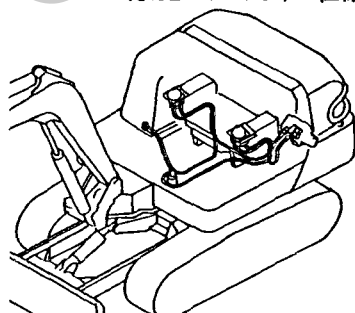
Fig. 88 コントロール配管(ポンプ～ リモコン・レバー～リターン :サイドレバー JP, EX仕様) CONTROL PIPING(PUMP～ REMO.-CON. VALVE～RETURN :SIDE LEVER JP, EX仕様)
