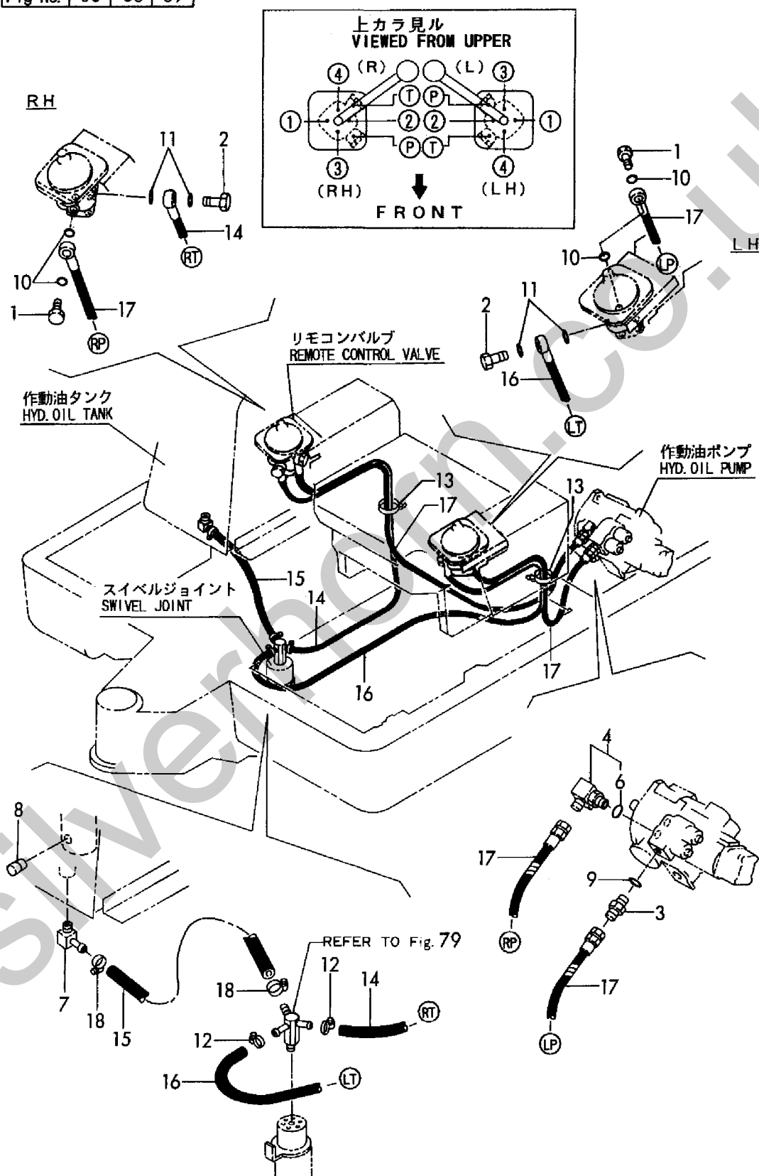
Fig. 88 コントロール配管(ポンプ～リモコンバルブ～リターン :サイドレバー JP, EX仕様) CONTROL PIPING(PUMP～REMO. -CON. V. ~RETURN :SIDE LEVER JP, EX SPEC.)
