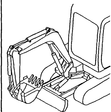
Fig. 50 アームシリンダ ARM CYLINDER
