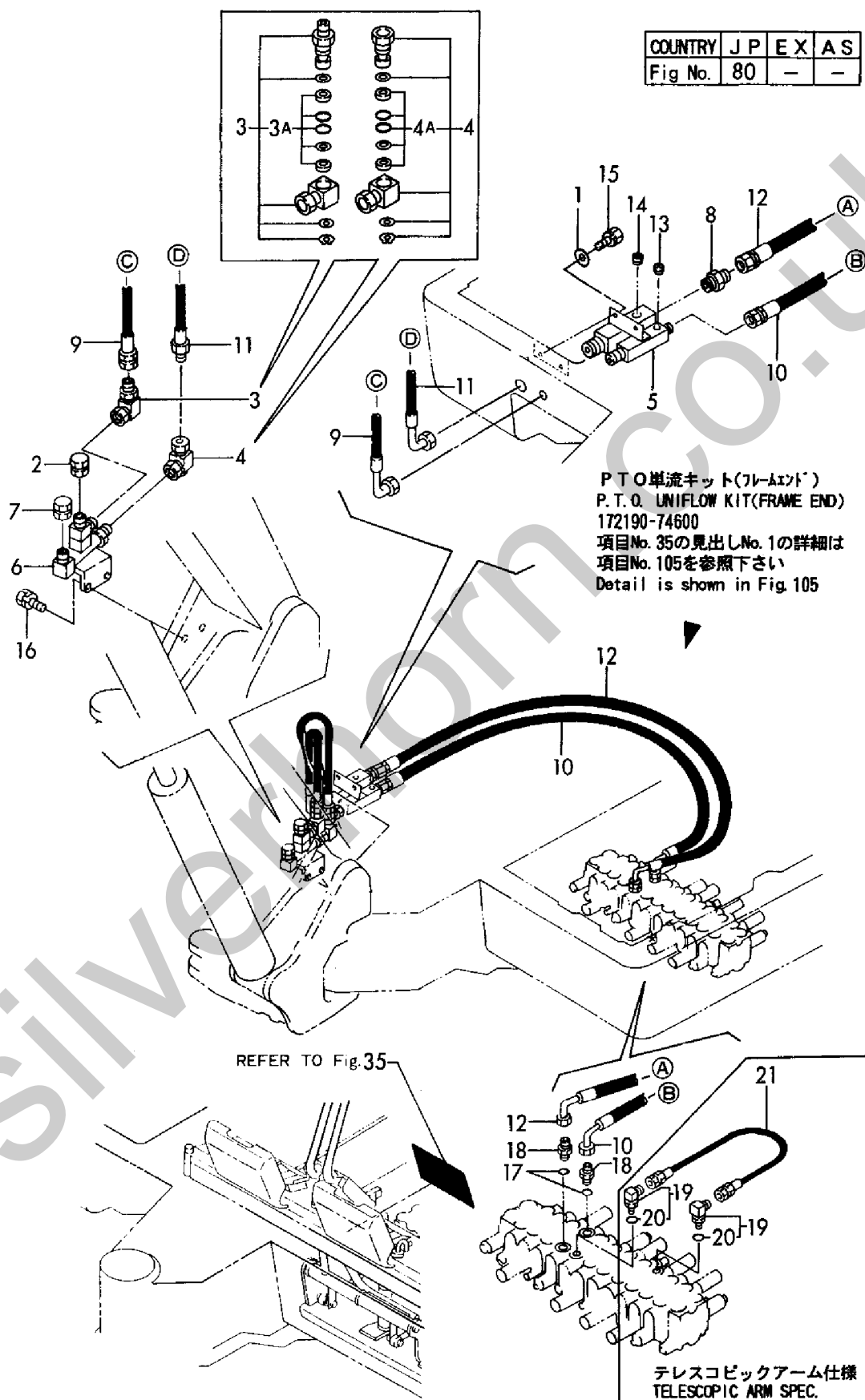
80 油圧配管(PTO, フレームエンド: 単流仕様) Fig. 80 HYD. OIL PIPING(P. T. O., FRAME END: UNIFLOW SPEC.)
