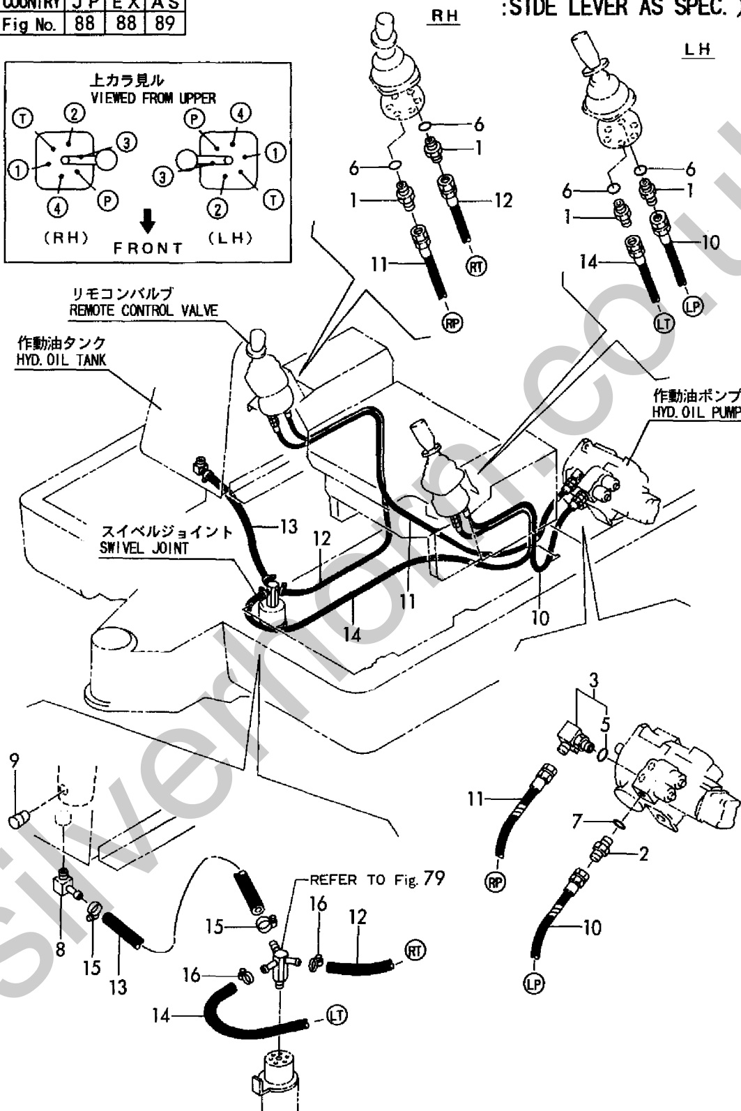
Fig. 89 コントロール配管(ポンプ～リモコンバルブ～リターン :サイドレバー-AS仕様) CONTROL PIPING(PUMP~REMO.-CON. V.~RETURN :SIDE LEVER AS SPEC.)
