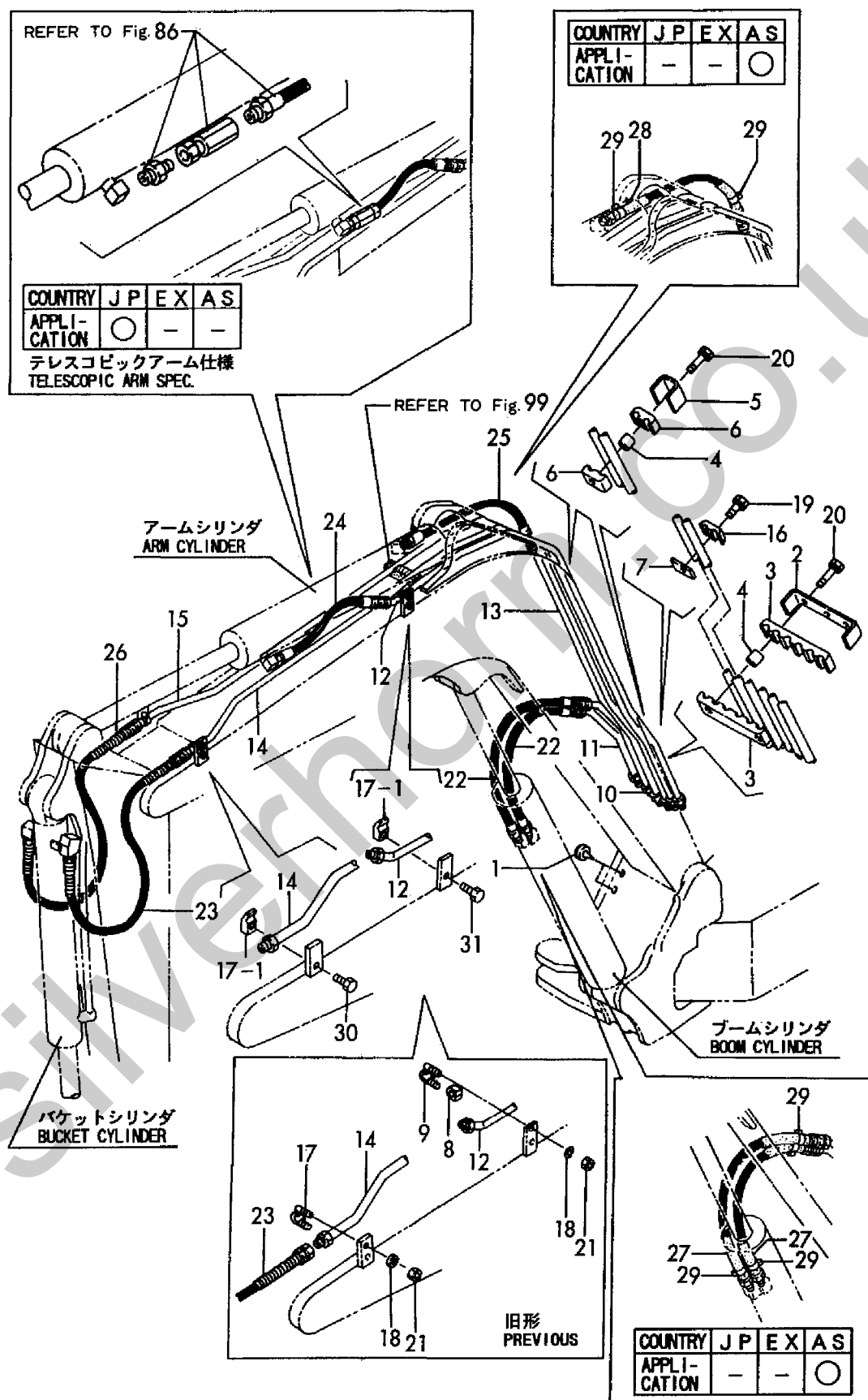
Fig. 83 油圧配管(ブーム) HYD. OIL PIPING (BOOM)
