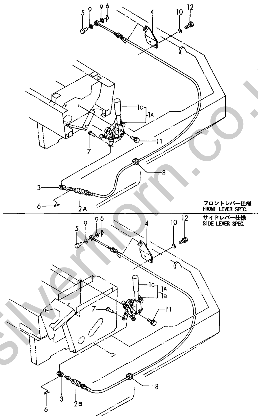
Fig. 11 アクセル(標準仕様) ACCELERATOR(STANDARD SPEC.)
