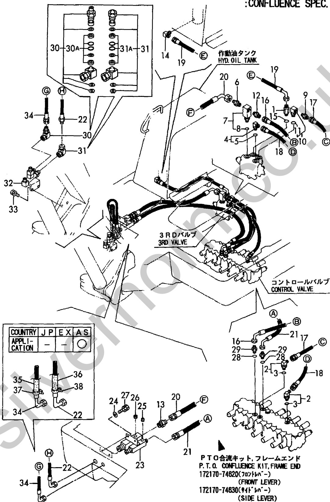
Fig. 81 油圧配管(PTO, フレームエンド : 合流仕様) HYD. OIL PIPING(P. T. O., FRAME END
