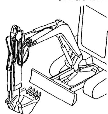
Fig. 87 コントロール配管(ポンプ～ リモコン・レバー～リターン:フロントレバー) CONTROL PIPING(PUMP～ REMO.-CON. VALVE～RETURN :FRONT LEVER)
