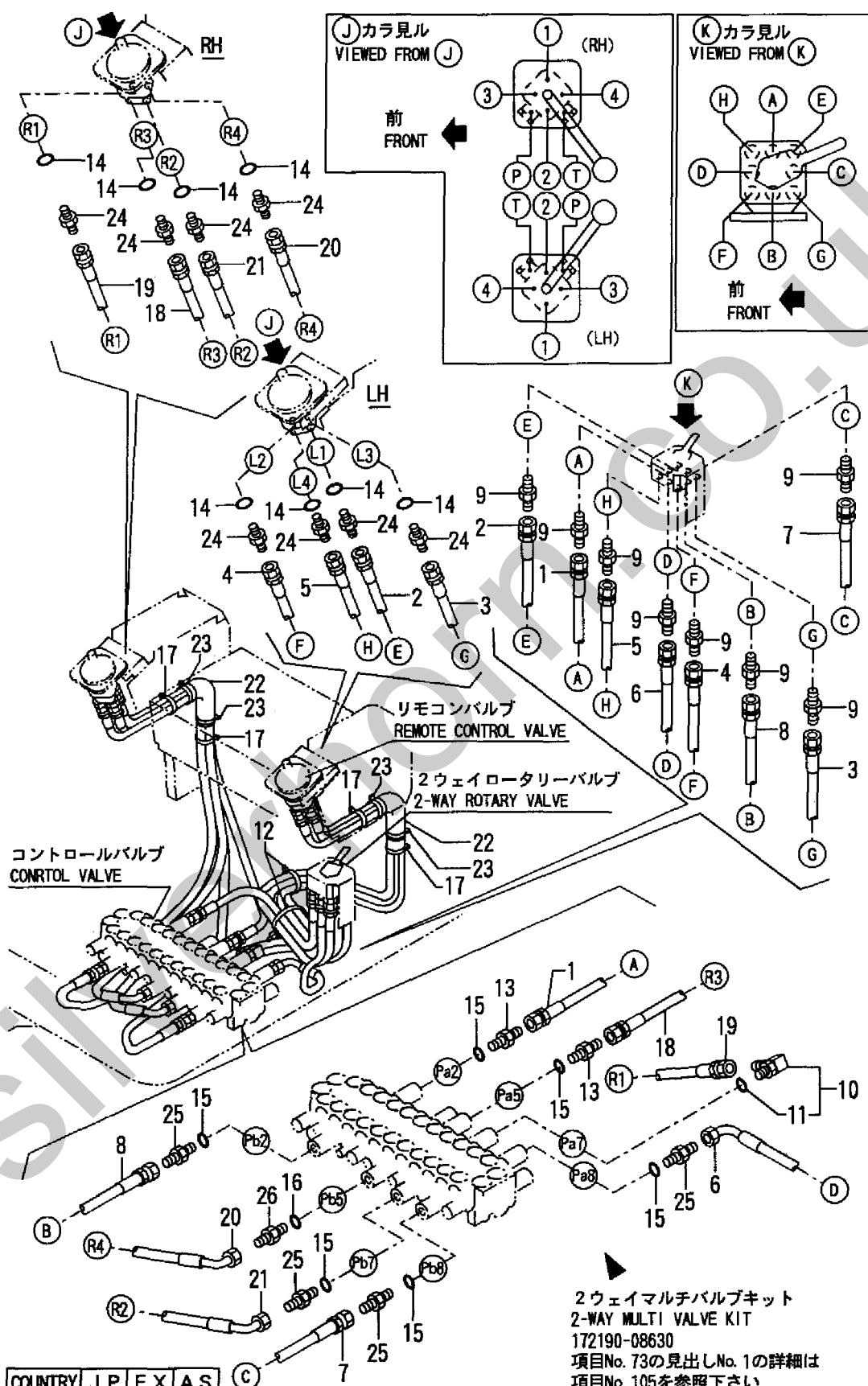
Fig. 97 コントロール配管(2ウェイ:サイドレバー) CONTROL PIPING(2-WAY:SIDE LEVER)
