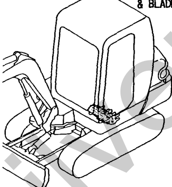
Fig. 64 コントロールバルブ (Pポート & バルブ台: PTO仕様) CONTROL VALVE (P PORT & VALVE STAND: P.T.O. SPEC.)
