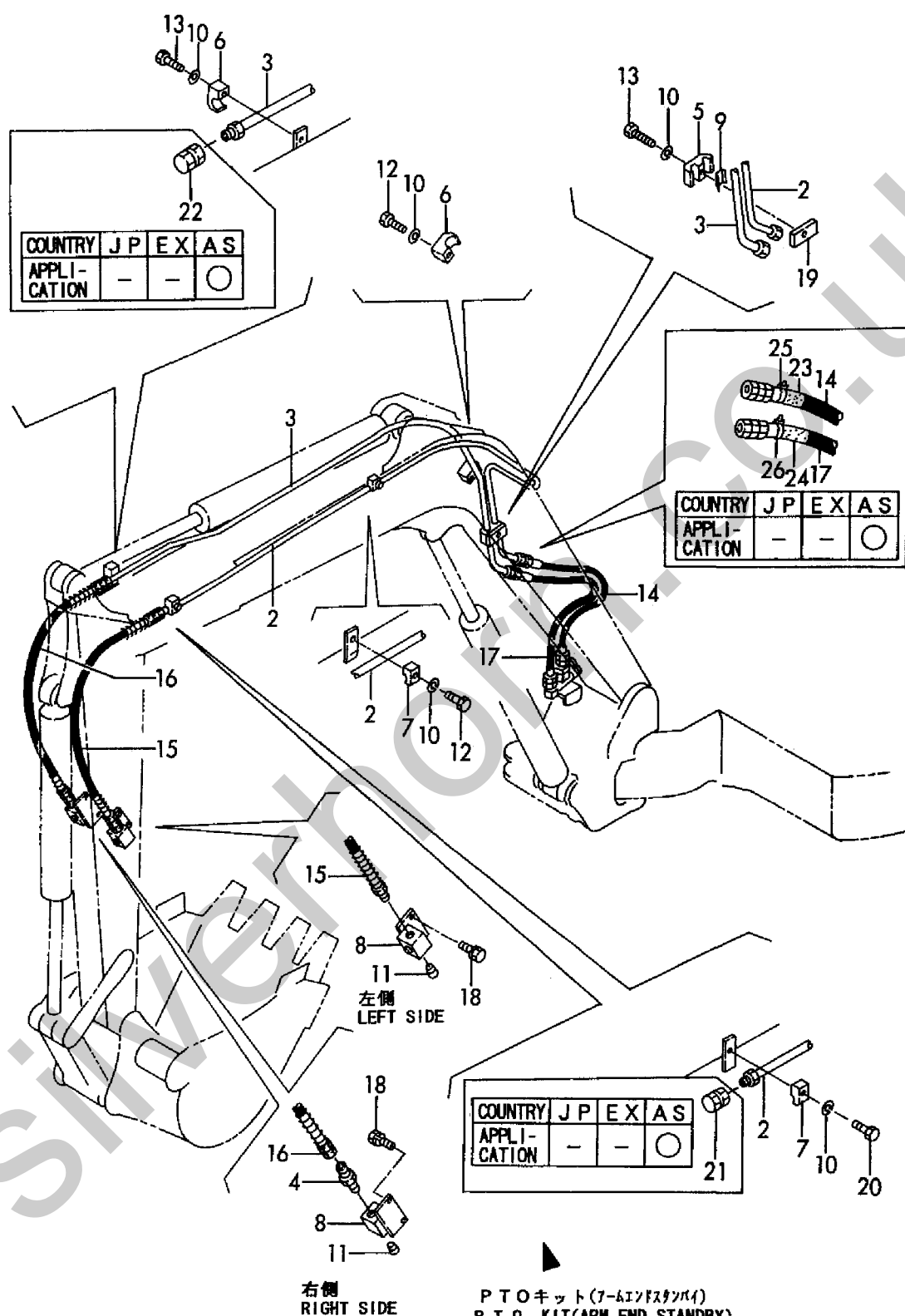
Fig. 85 油圧配管(PTO 7 -M:7-メント仕様)(新形) HYD. OIL PIPING(P. T. O. BOOM:ARM END SPEC. )(NEW)
