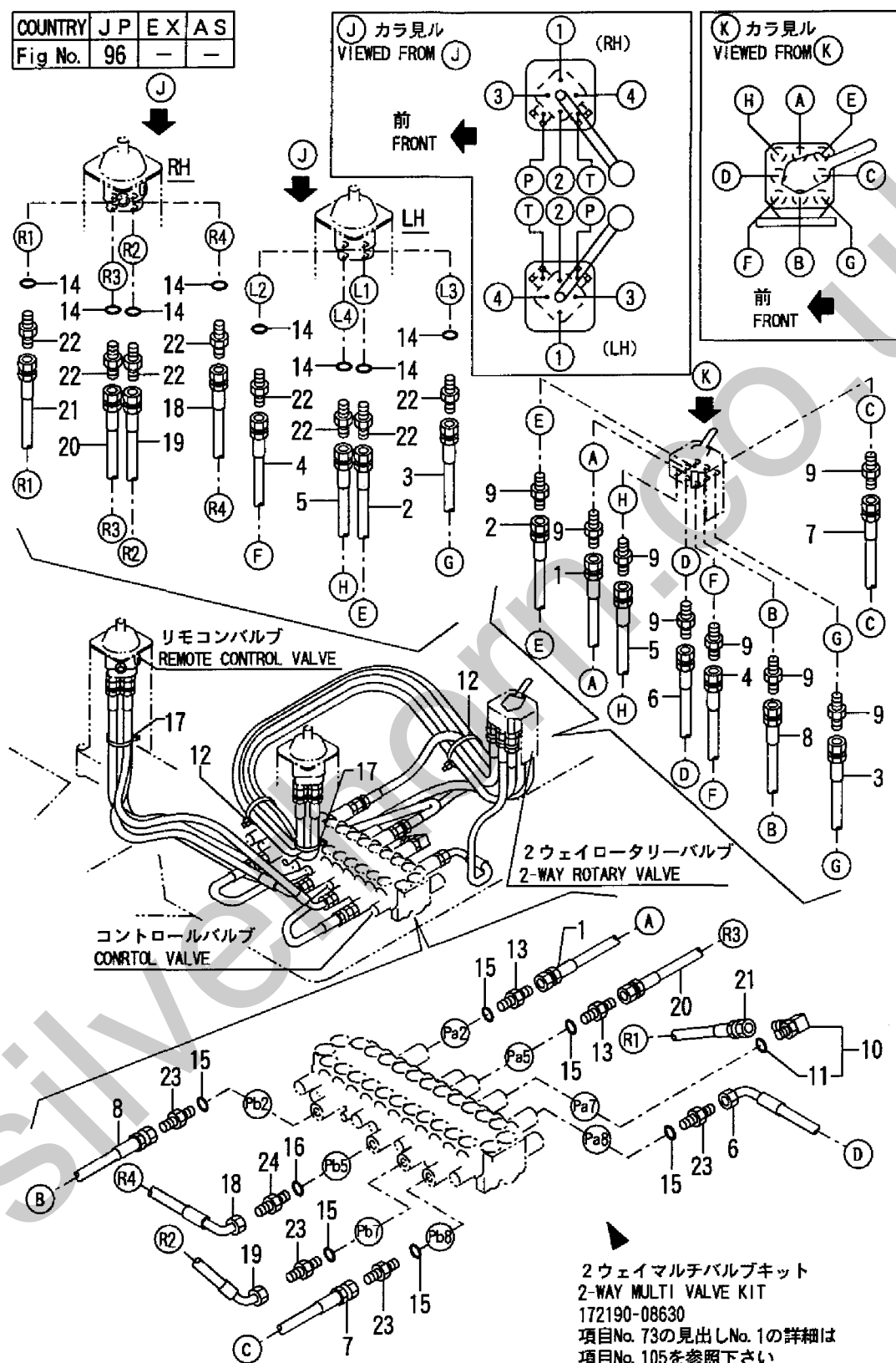
Fig. 96 コントロール配管(2ウェイ:フロントレバー) CONTROL PIPING(2-WAY:FRONT LEVER)
