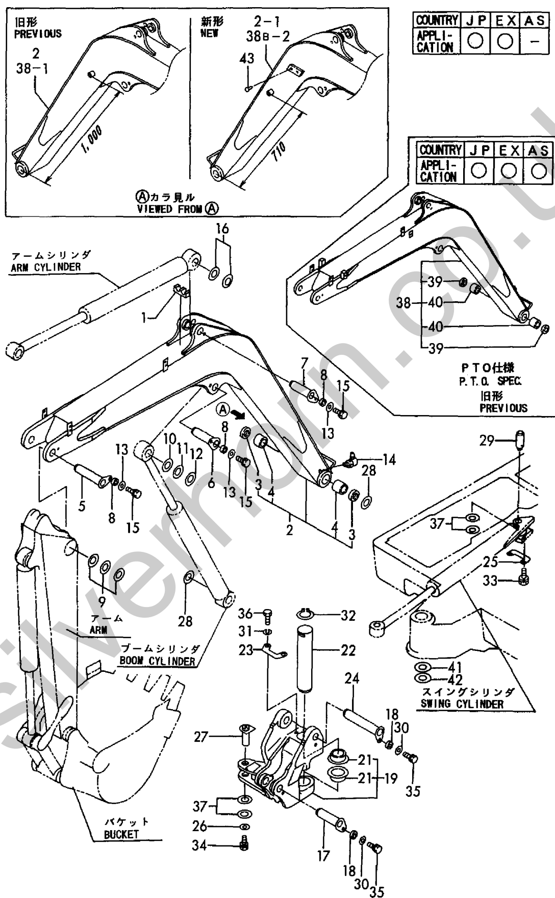
Fig. 99 99 ブーム & ブームブラケット BOOM & BOOM BRACKET
