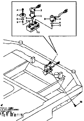
Fig. 77 PTOバルブ P.T.O. VALVE
