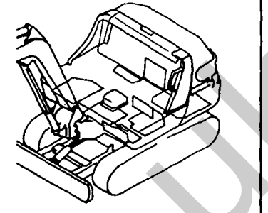
Fig. 46 シート & シートマウント (フロントレバー) SEAT & SEAT MOUNT (FRONT LEVER)
