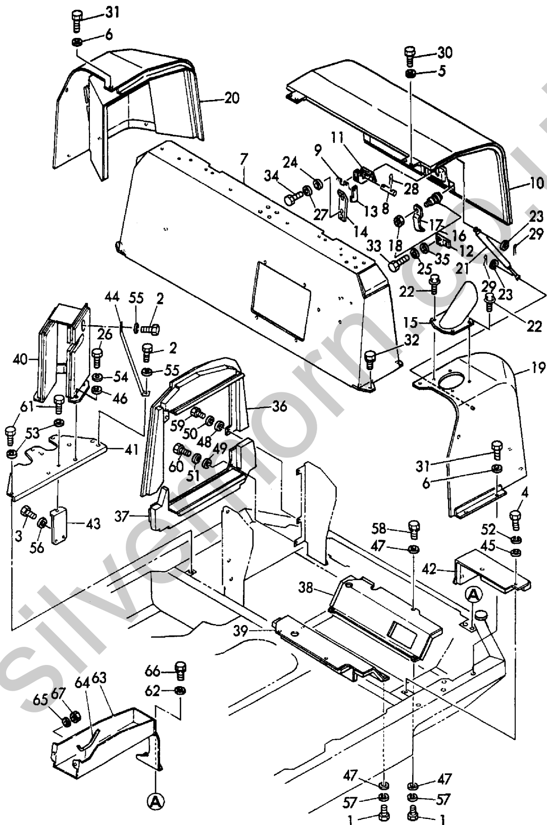
Fig. 53 ボンネット BONNET
