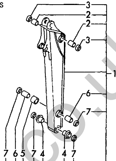
Fig. 102 アーム&バケットリンク ARM & BUCKET LINK
