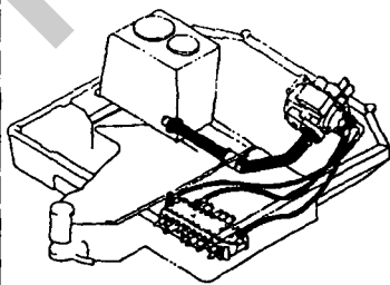
Fig. 80 油圧配管 (バルブ～ブーム) HYD. OIL PIPING (VALVE ~ BOOM)
