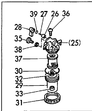
Fig. 19 燃料タンク&燃料パイプ (AS) FUEL TANK & FUEL PIPE (AS)
