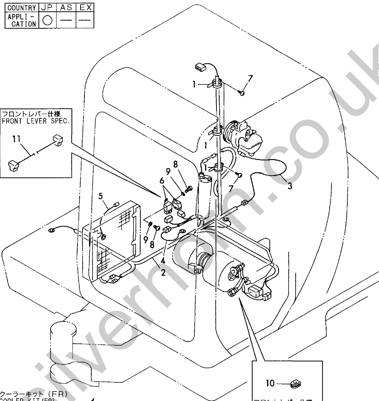
Fig. 24 電装品 (クーラ仕様) ELECTRIC PART (COOLER SPEC.)
