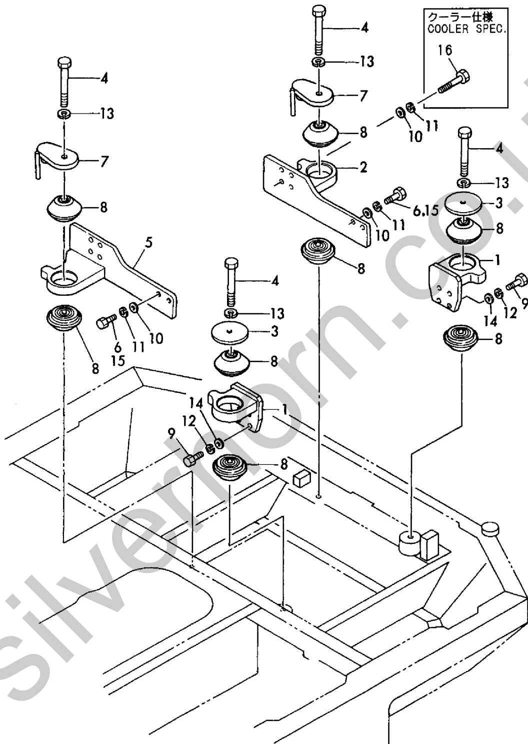
Fig. 13 エンジンマウント ENGINE MOUNT
