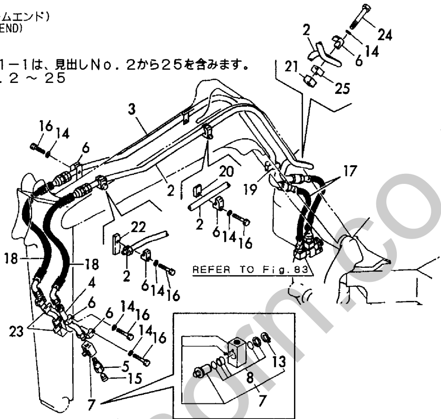
Fig. 88 油圧配管 (PTOアームエンド) HYD. OIL PIPING (P. T. O. ARM END)
