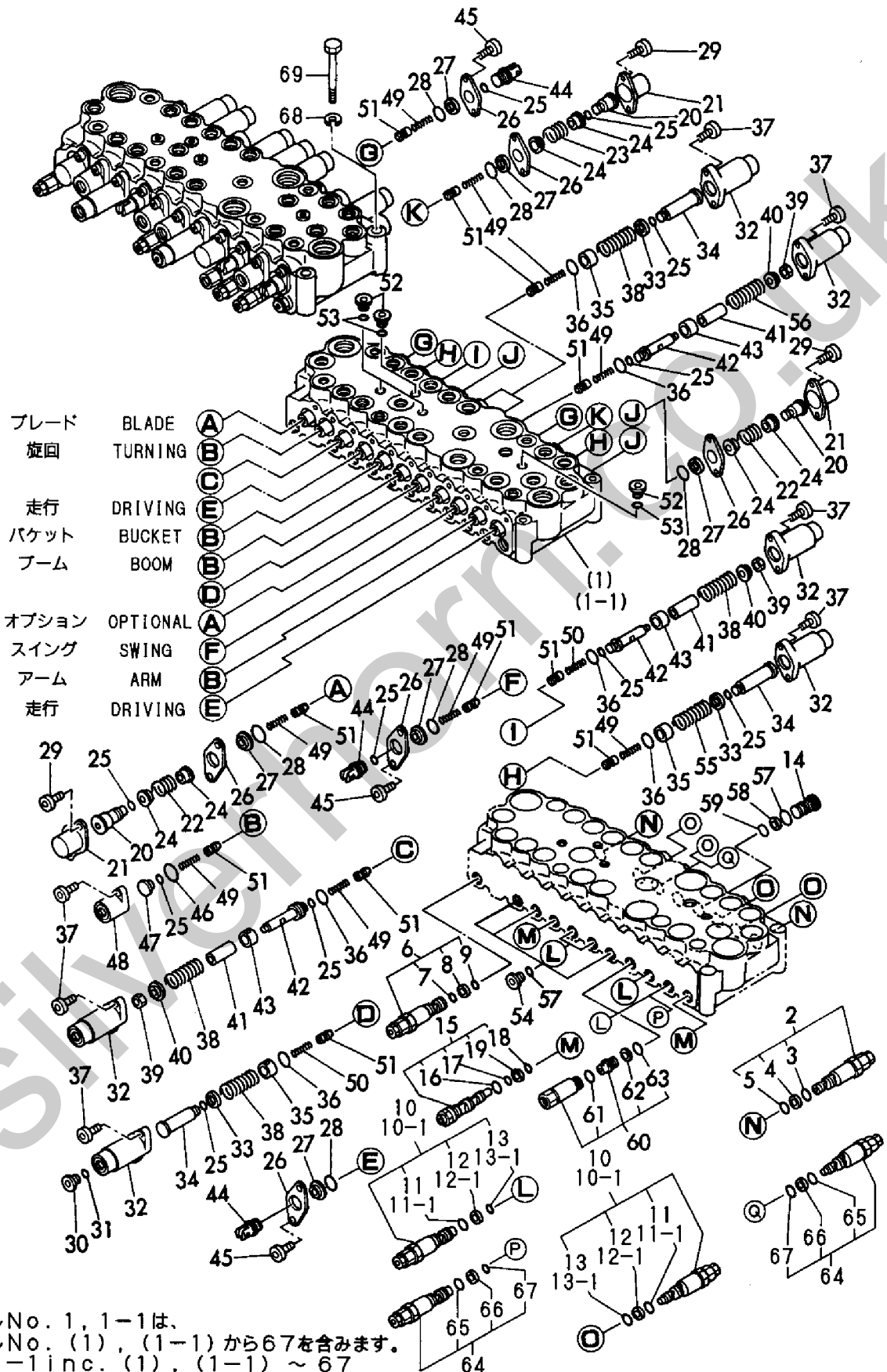
Fig. 71 コントロールバルブ (PTO) CONTROL VALVE (P. T. O.)
