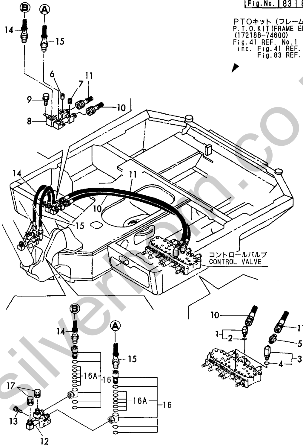
Fig. 83 油圧配管 (PTOバルブ/フレーム) HYD. OIL PIPING (P. T. O. VALVE/FRAME)
