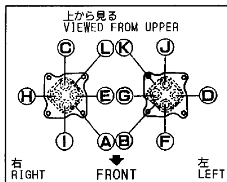
Fig. 92 コントロール配管 (フロントレバー/ダイレクト) CONTROL PIPING (FRONT LEVER/DIRECT)
