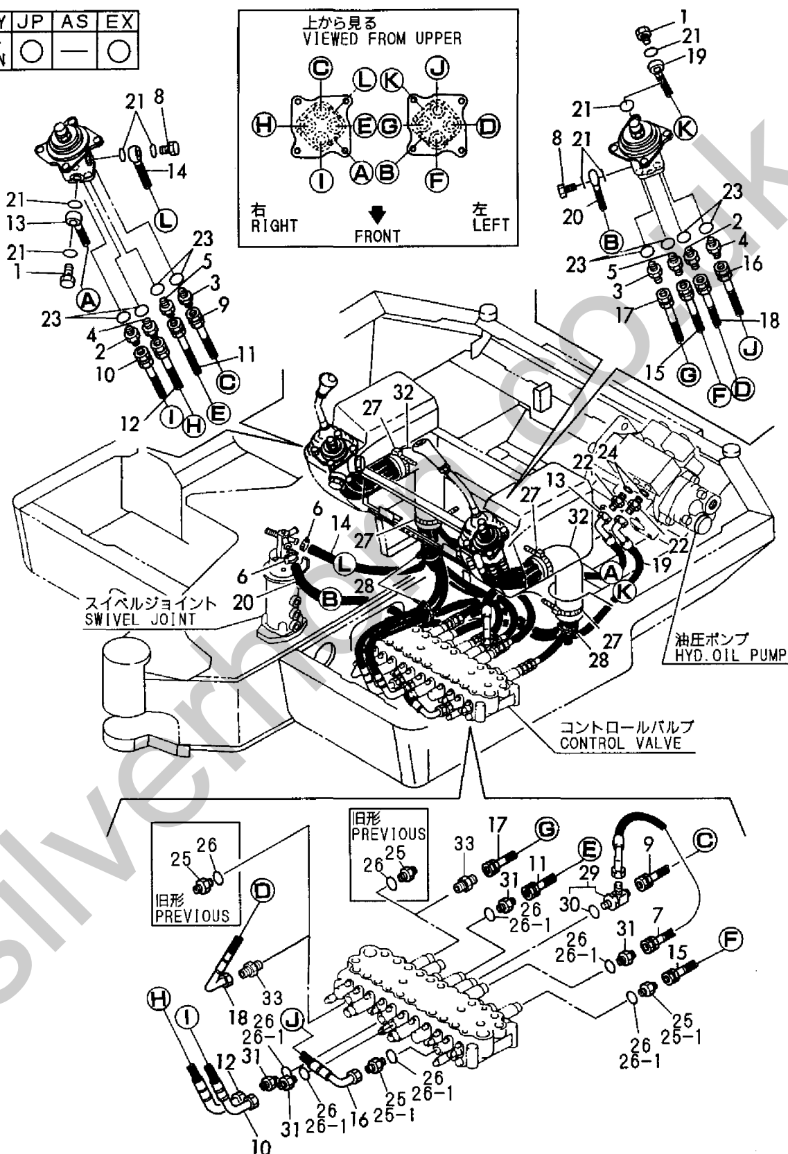
Fig. 93 コントロール配管 (サイドレバー/ダイレクト) CONTROL PIPING (SIDE LEVER/DIRECT)
