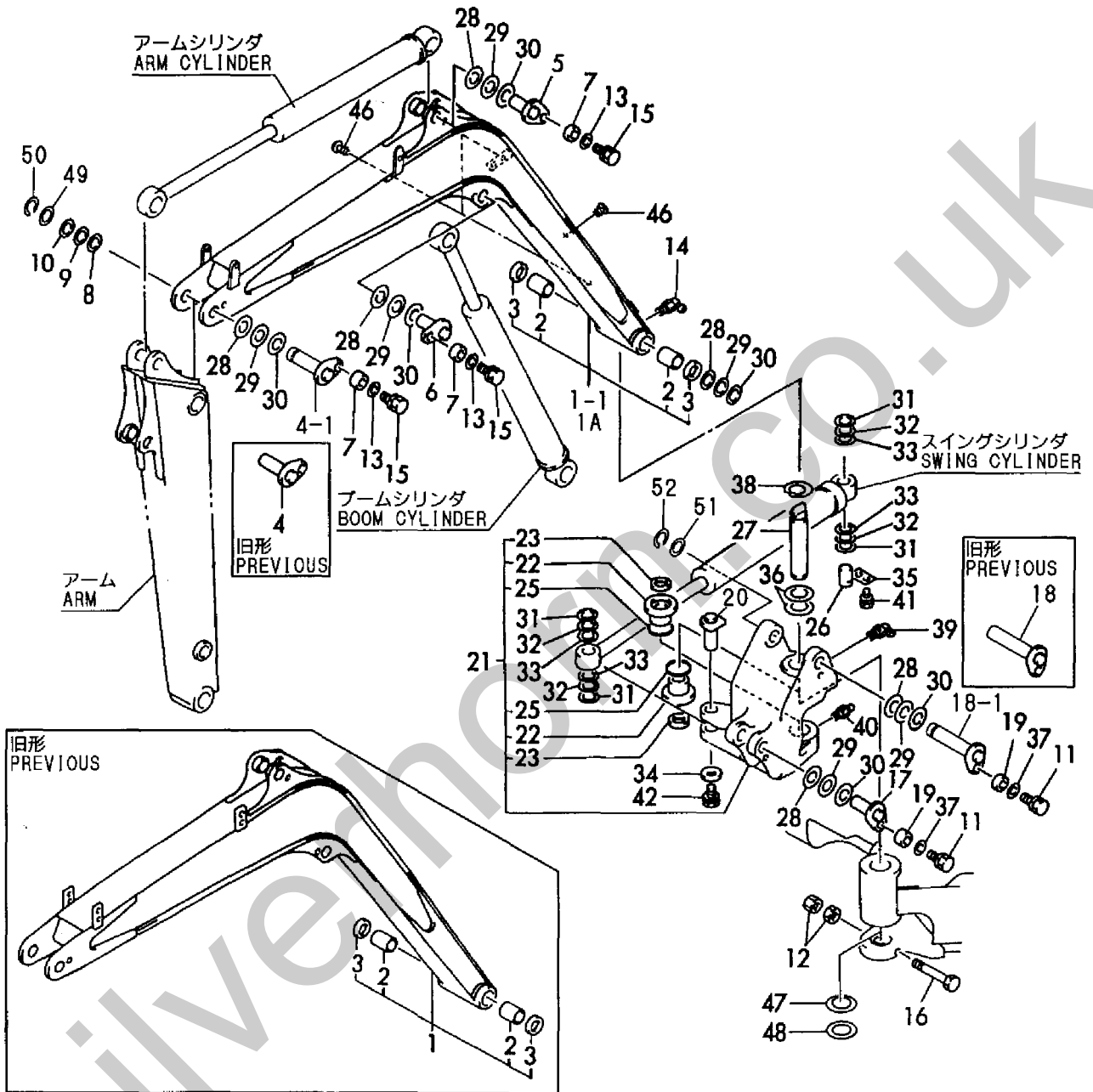
Fig. 101 ブーム&ブームブラケット BOOM & BOOM BRACKET
