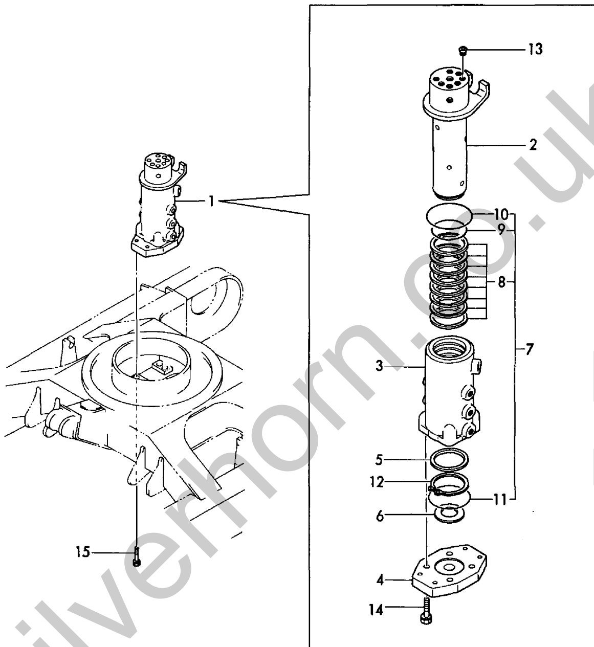
Fig. 69 スイベルジョイント SWIVEL JOINT
