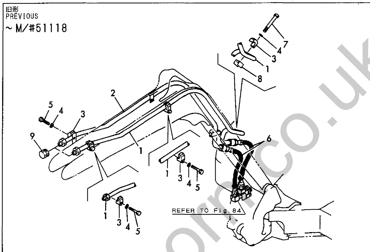
Fig. 90 油圧配管 (PTOブームエンド) (AS) (旧形) HYD. OIL PIPING (P.T.O. BOOM END) (AS) (PREVIOUS)
