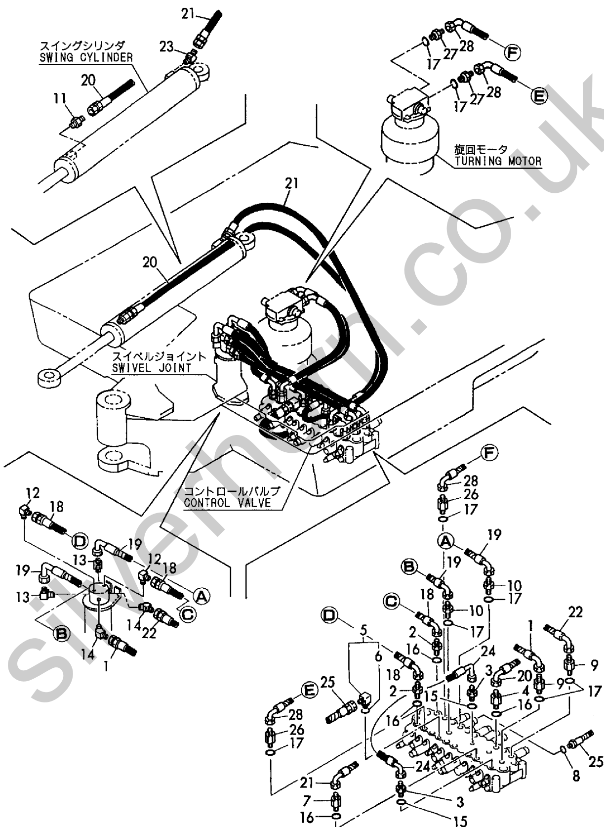
Fig. 81 油圧配管 (バルブ～スイベル～モータ) HYD. OIL PIPING (VALVE ~ SWIVEL ~ MOTOR)
