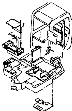
Fig. 108 クーラキット (フロントレバー) COOLER KIT (FRONT LEVER)
