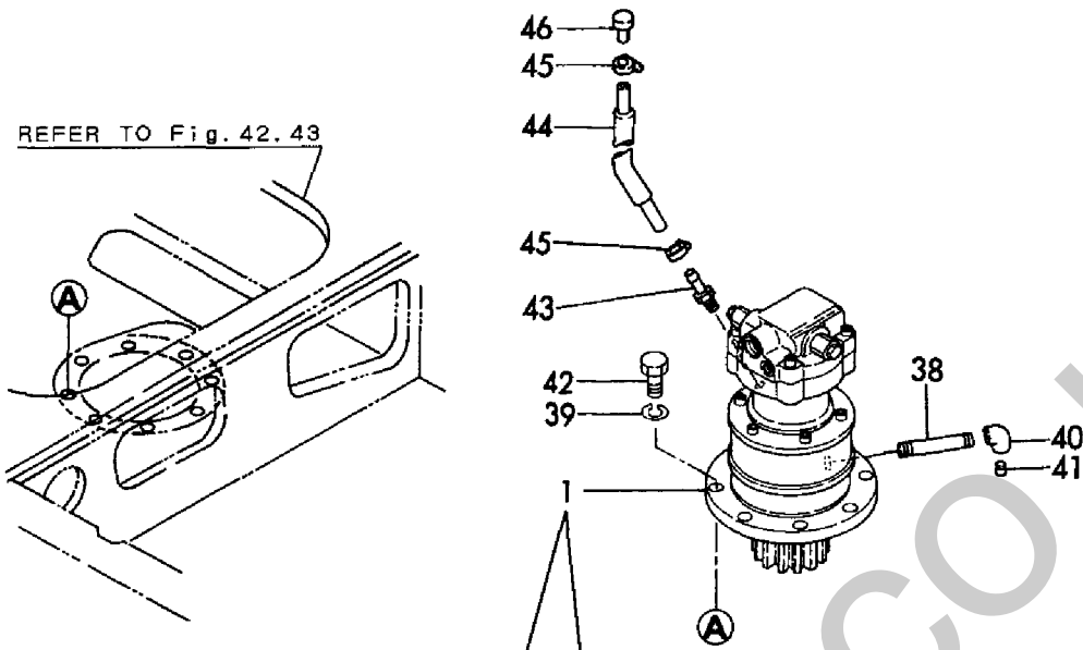
Fig. 68 旋回モータ TURNING MOTOR
