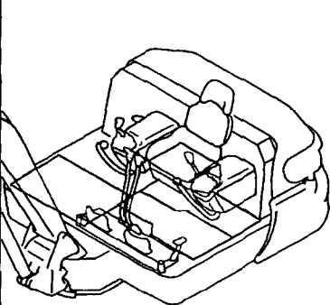
Fig. 50 シートマウント &ステップ (AS) SEAT MOUNT & STEP (AS)
