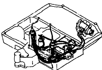
Fig. 92 コントロール配管 (フロントレバー/ダイレクト) CONTROL PIPING (FRONT LEVER/DIRECT)
