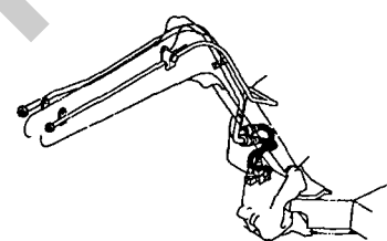
Fig. 92 コントロール配管 (フロントレバー/ダイレクト) CONTROL PIPING (FRONT LEVER/DIRECT)
