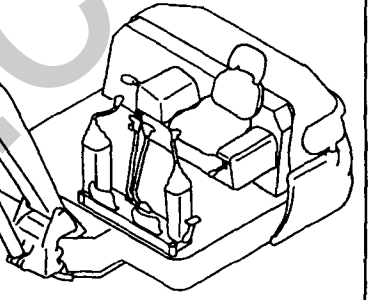
Fig. 47 シート & シートマウント (フロントレバー) (クーラ仕様) SEAT & SEAT MOUNT (FRONT LEVER) (COOLER SPEC.)
