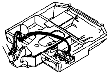
Fig. 84 油圧配管 (PTOバルブ /フレーム) (AS) HYD. OIL PIPING (P.T.O. VALVE /FRAME) (AS)
