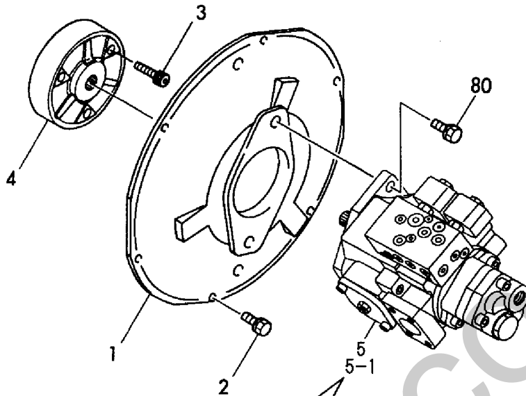
Fig. 59 油圧ポンプ&軸継手 HYD. OIL PUMP & JOINT
