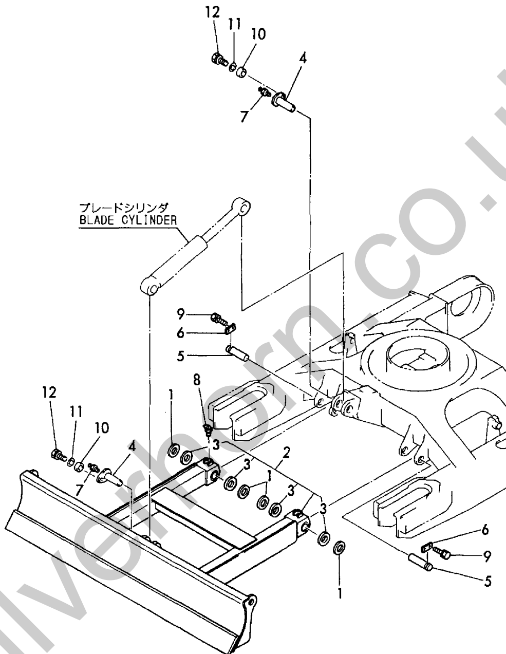
ブレード BLADE
