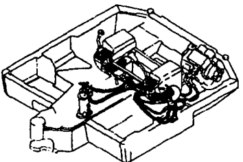
Fig. 99 コントロール配管 (マルチチェンジバルブ ~コントロールバルブ) CONTROL PIPING (MULTI CHANGE VALVE ~ CONTROL VALVE)
