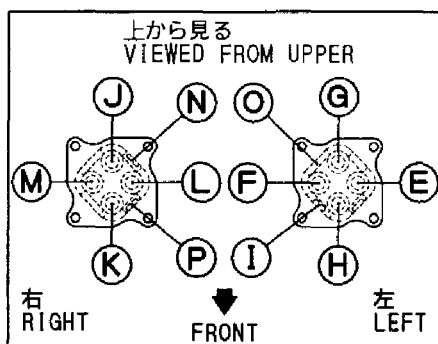
Fig. 96 コントロール配管 (サイドレバー/2ウェイマルチチェンジ) CONTROL PIPING (SIDE LEVER/2WAY MULTI CHANGE)
