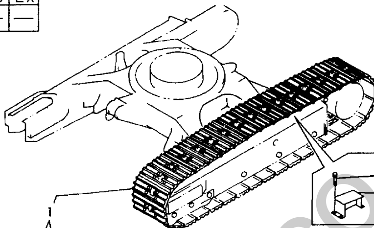
Fig. 107 クローラ (アタッチメント) CRAWLER (ATTACHMENT)
