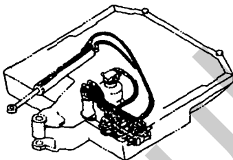
Fig. 82 油圧配管 (リターン) HYD. OIL PIPING (RETURN)
