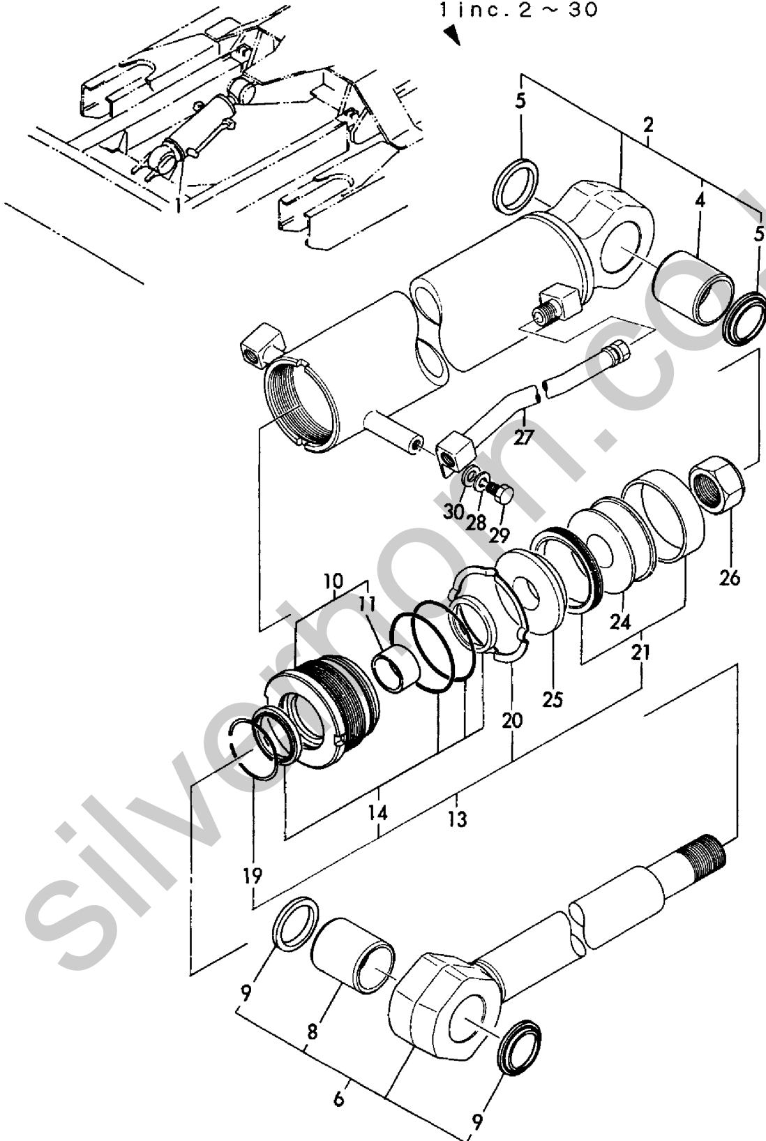
Fig. 66 ブレードシリンダ BLADE CYLINDER
