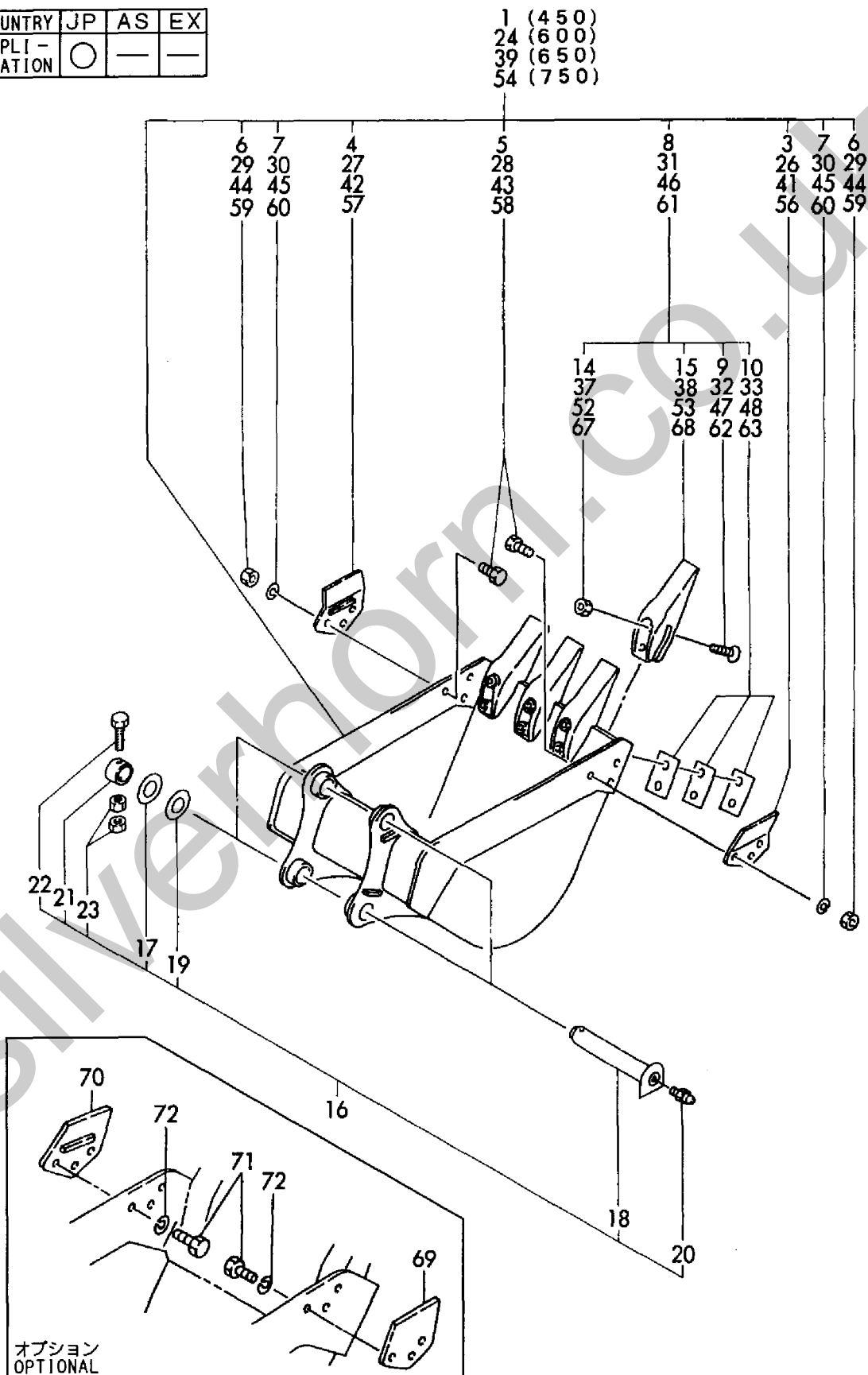
Fig. 104 バケット (アタッチメント) BUCKET (ATTACHMENT)
