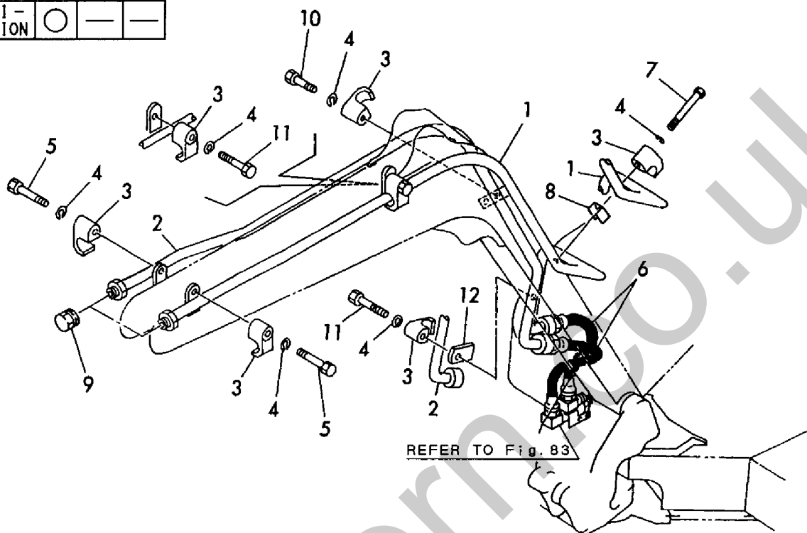
Fig. 89 油圧配管 (PTOブームエンド) (JP) HYD. OIL PIPING (P.T.O. BOOM END) (JP)
