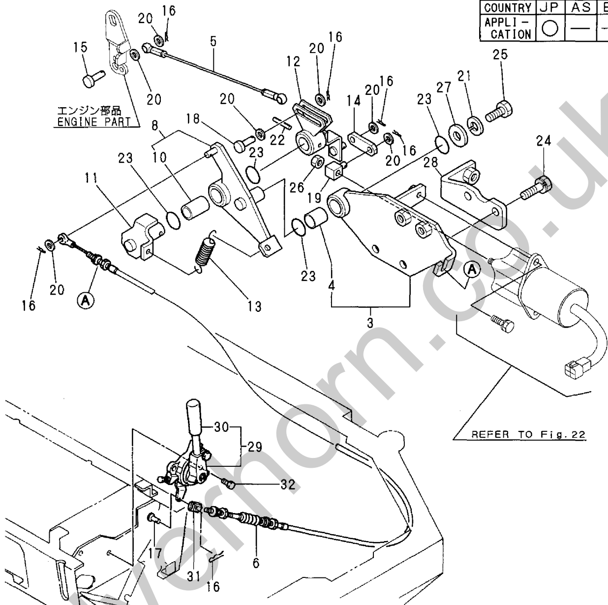
Fig. 12 アクセル (ワンタッチデセル) ACCELERATOR (ONE TOUCH DECEL)
