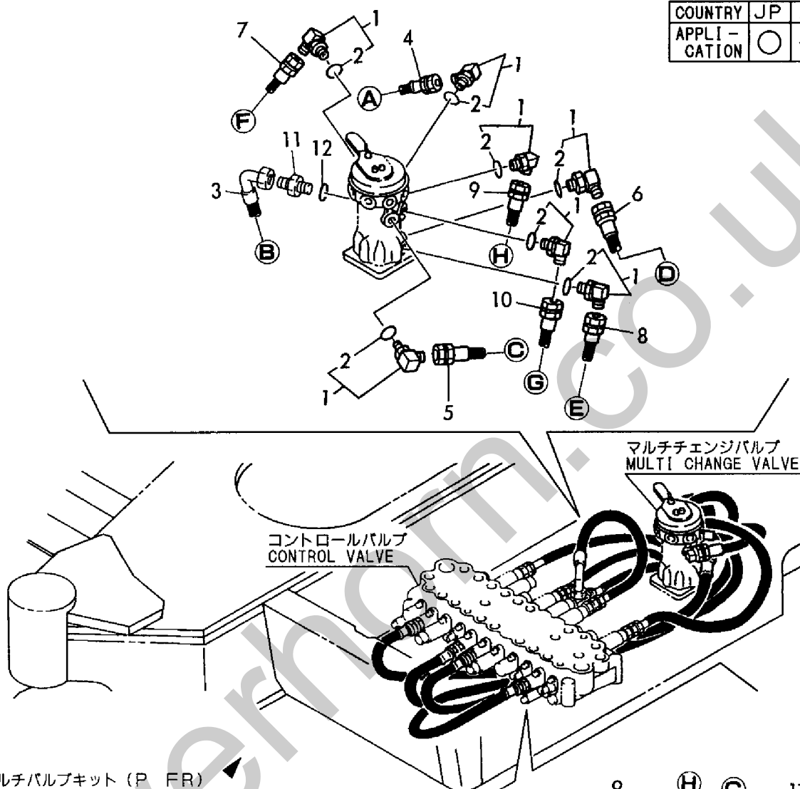
Fig. 99 コントロール配管 (マルチチェンジバルブ~コントロールバルブ) CONTROL PIPING (MULTI CHANGE VALVE ~ CONTROL VALVE)
