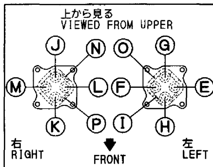
Fig. 97 コントロール配管 (フロントマルチ/リモコンバルブ~チェンジバルブ) CONTROL PIPING (FRONT MULTI/REMO-CON VALVE ~ CHANGE VALVE)
