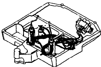
Fig. 97 コントロール配管 (フロントマルチ /リモコンバルブ ~チェンジバルブ) CONTROL PIPING (FRONT MULTI /REMO-CON VALVE ~ CHANGE VALVE)
