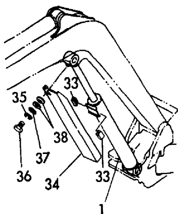
Fig. 60 ブームシリンダ (キャビン) BOOM CYLINDER (CABIN)
