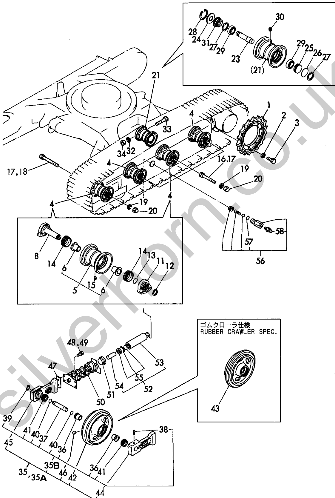
Fig. 28 ローラ&アジャスト ROLLER & ADJUST
