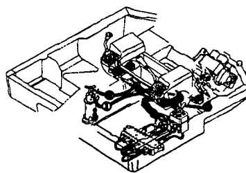
Fig. 96 コントロール配管 (サイドレバー /2ウェイマルチチェンジ) CONTROL PIPING (SIDE LEVER /2WAY MULTI CHANGE)
