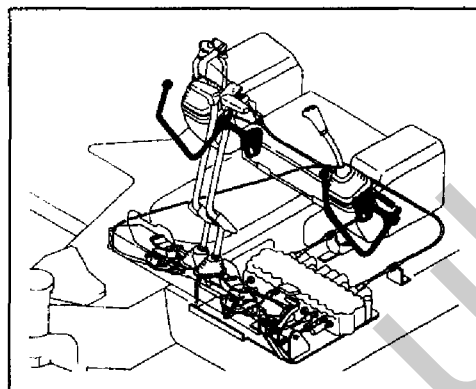
Fig. 38 操縦装置 (カットオフレバー/サイドレバー) CONTROL EQUIPMENT (CUT OFF LEVER/SIDE LEVER)
