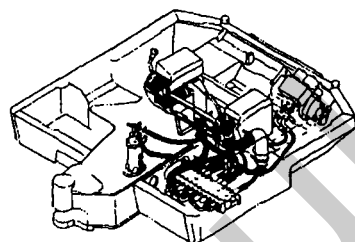
Fig. 94 コントロール配管 (ダイレクト) (AS) CONTROL PIPING (DIRECT) (AS)
