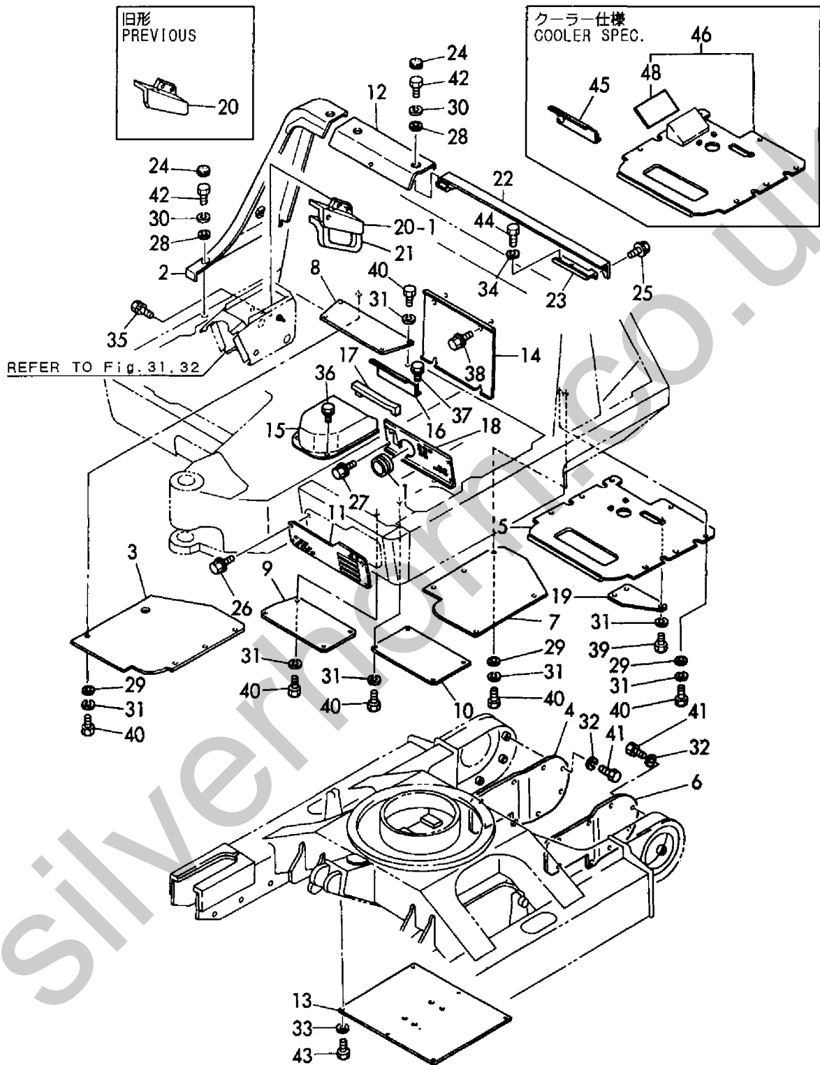
Fig. 44 フレームカバー (キャビン) FRAME COVER (CABIN)
