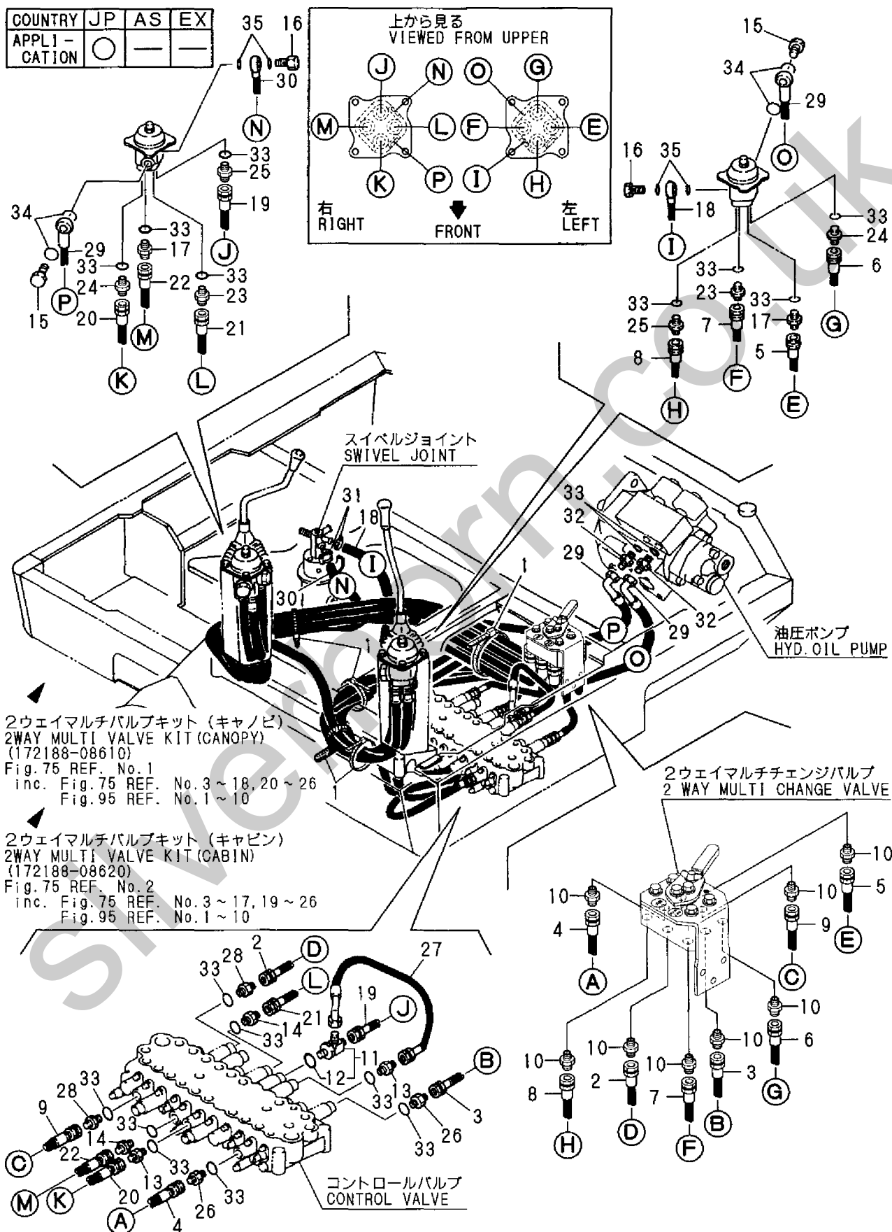
Fig. 95 コントロール配管 (フロントレバー/2ウェイマルチチェンジ) CONTROL PIPING (FRONT LEVER/2WAY MULTI CHANGE)
