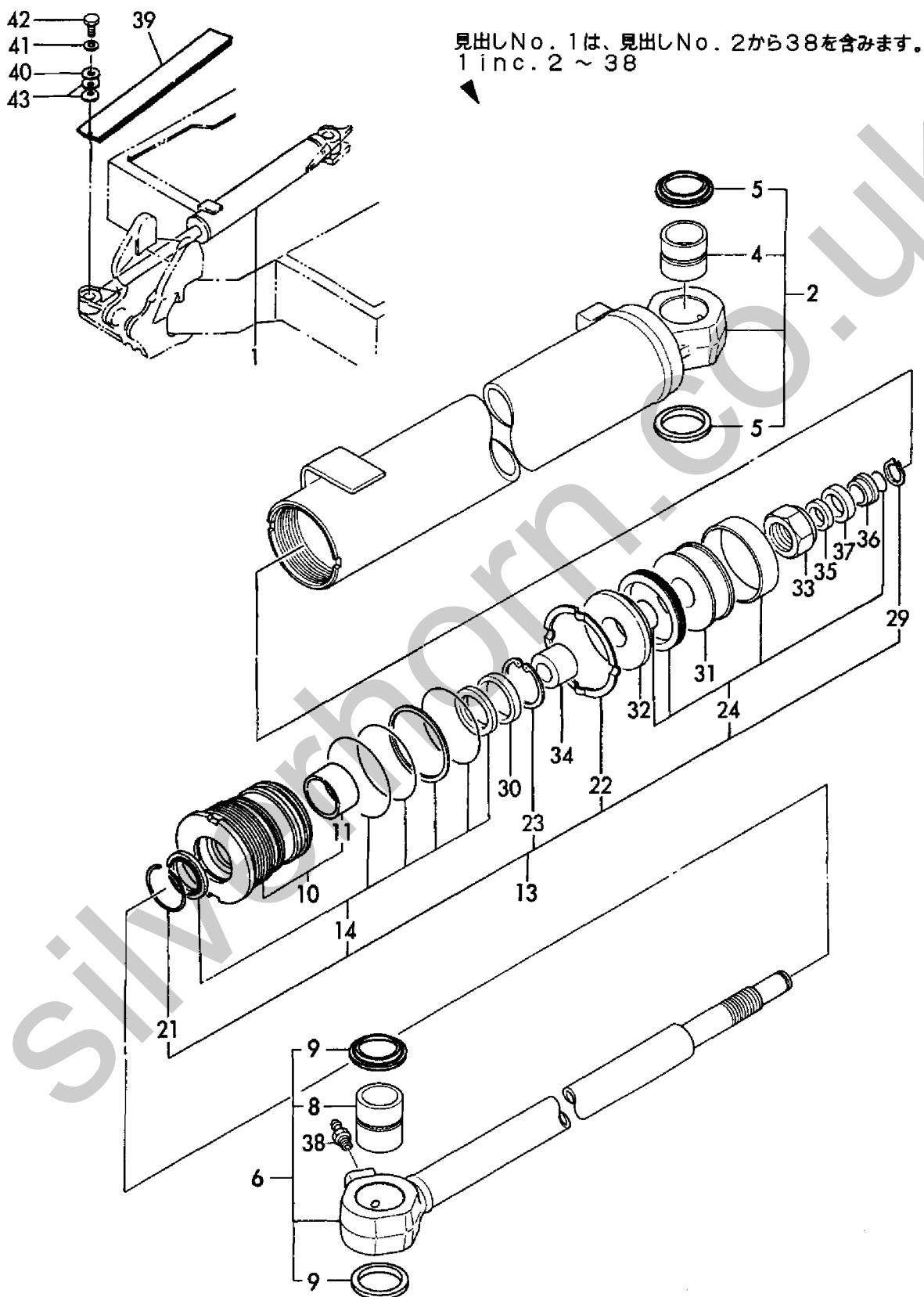
Fig. 65 スイグシリンダ (キャノピ) SWING CYLINDER (CANOPY)
