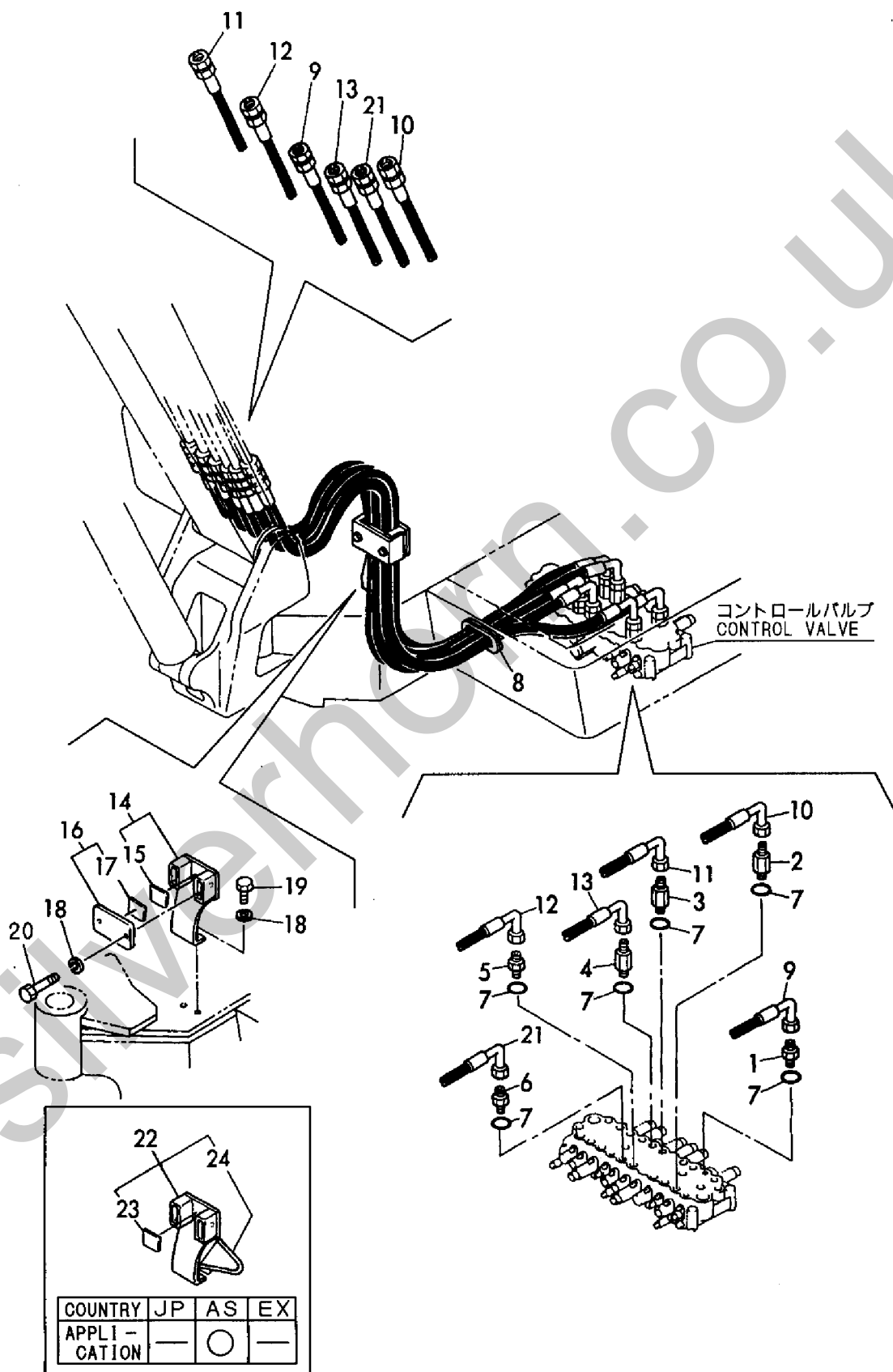
Fig. 80 油圧配管 (バルブ～ブーム) HYD. OIL PIPING (VALVE ~ BOOM)
