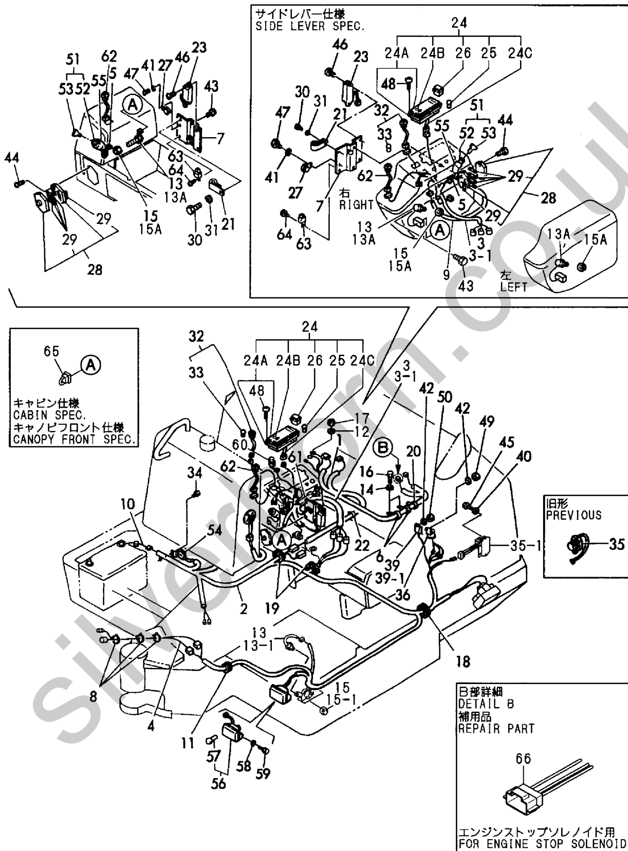
Fig. 21 電装品 (キャビン, キャノピ) ELECTRIC PART (CABIN, CANOPY)
