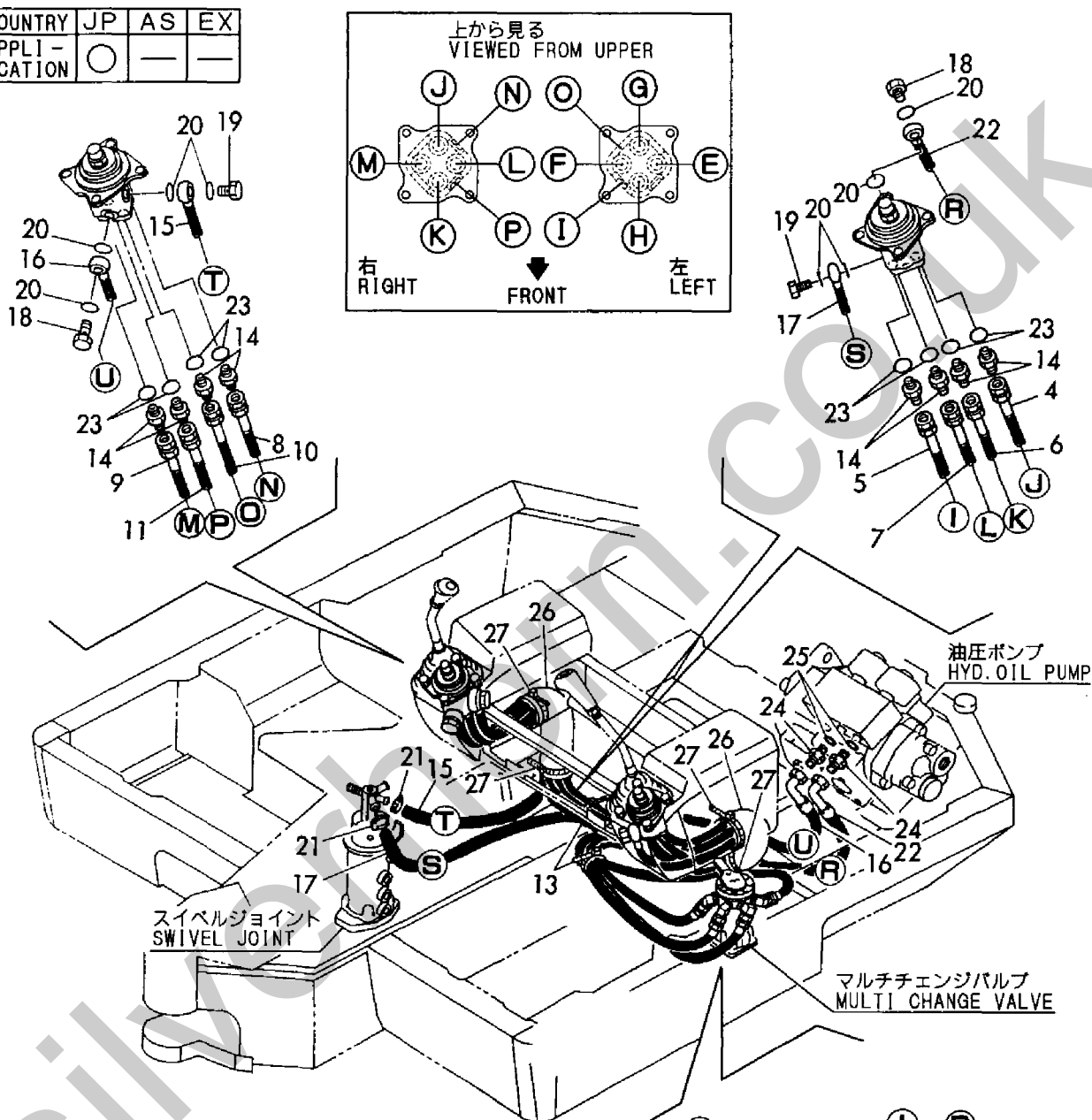
Fig. 98 コントロール配管 (サイドマルチ/リモコンバルブ~チェンジバルブ) CONTROL PIPING (SIDE MULTI/REMO-CON VALVE ~ CHANGE VALVE)
