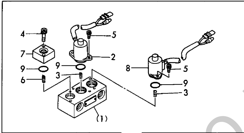
Fig. 77 PTOバルブ P.T.O. VALVE
