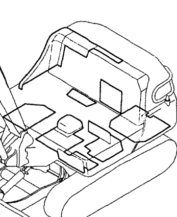
Fig. 42 フレームカバー (キャノピー) FRAME COVER (CANOPY)
