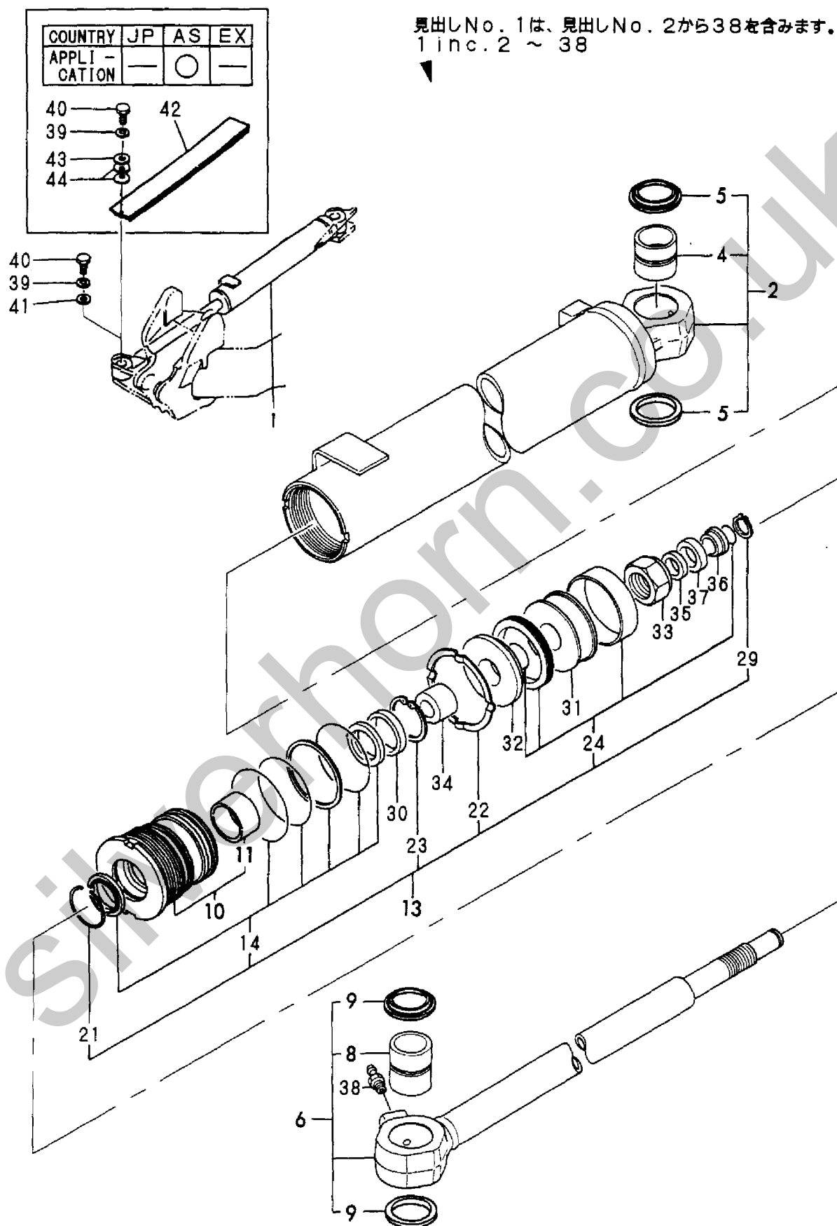
Fig. 60 スイグシリンダ (キャビン) SWING CYLINDER (CABIN)
