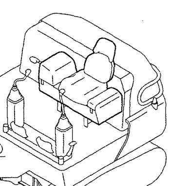
Fig. 44 シート & シートマウント (フロントレバー) (クーラ仕様) SEAT & SEAT MOUNT (FRONT LEVER) (COOLER SPEC.)
