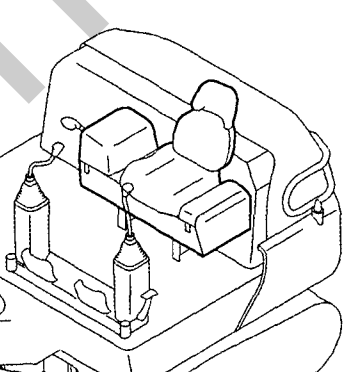
Fig. 44 シート & シートマウント (フロントレバー) (クーラ仕様) SEAT & SEAT MOUNT (FRONT LEVER) (COOLER SPEC.)
