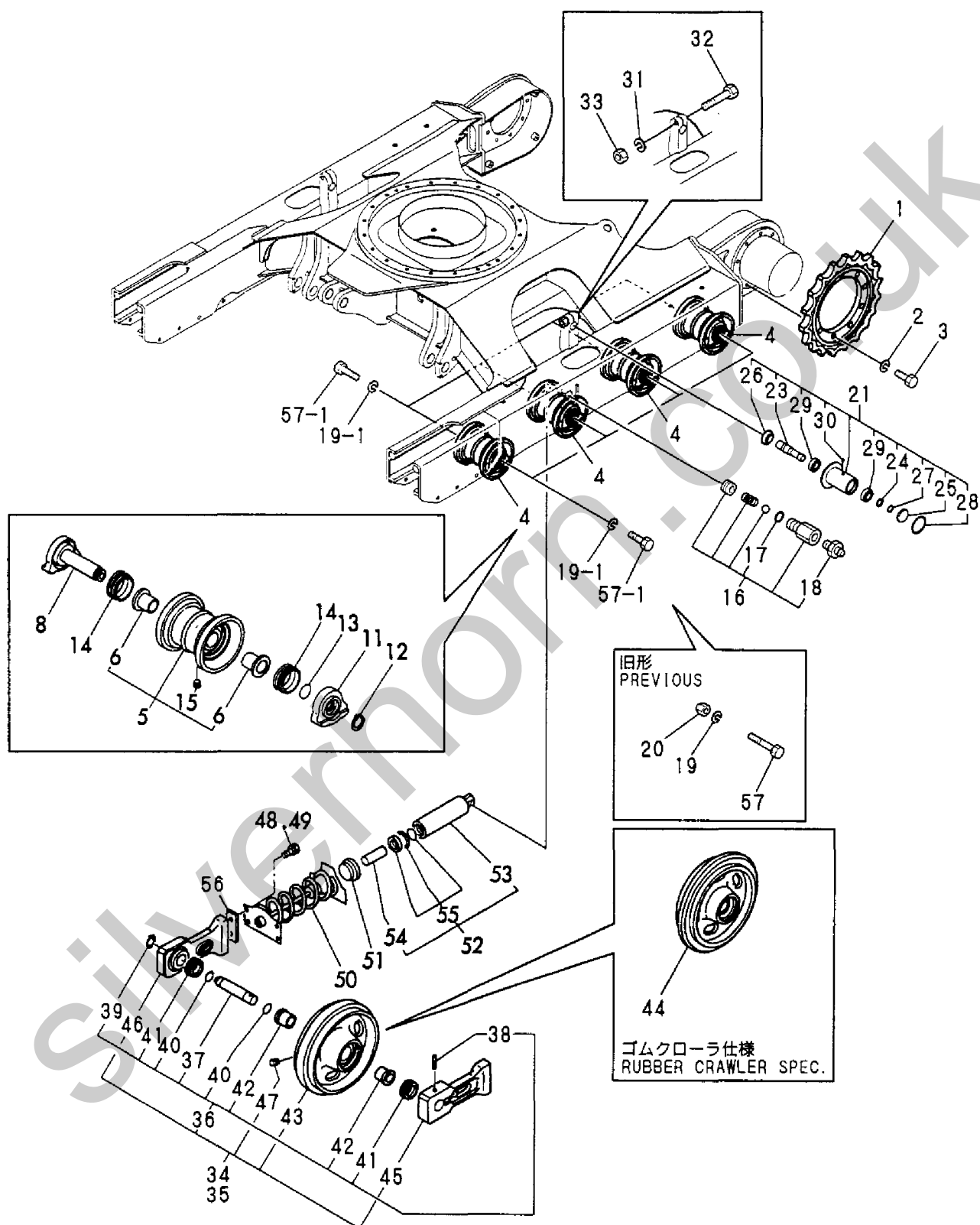
Fig. 27 ローラ&アジャスト ROLLER & ADJUST
