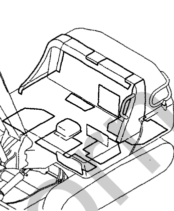
Fig. 43 シート & シートマウント (フロントレバー) SEAT & SEAT MOUNT (FRONT LEVER)
