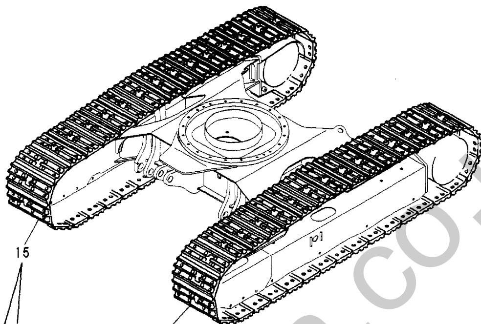
Fig. 28 クローラ CRAWLER
