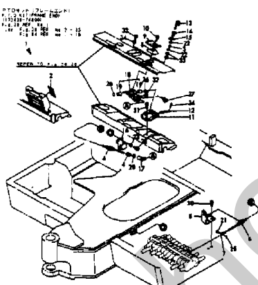
Fig. 84 油圧配管 (PTOフレームエンド) HYD. OIL PIPING (P.T.O. FRAME END)
