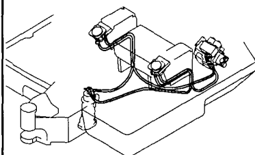
Fig. 88 コントロール配管 (ポンプ～リモコンバルブ ～リターン/サイドレバー) CONTROL PIPING (PUMP ~ REMO. -CON. V. ~ RETURN/SIDE LEVER)
