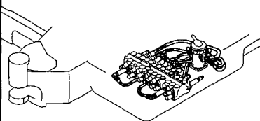
Fig. 95 コントロール配管 (マルチバルブ ～コントロールバルブ /4ウェイマルチ) CONTROL PIPING (MULTI V. ~ CONTROL V. /4-WAY MULTI)
