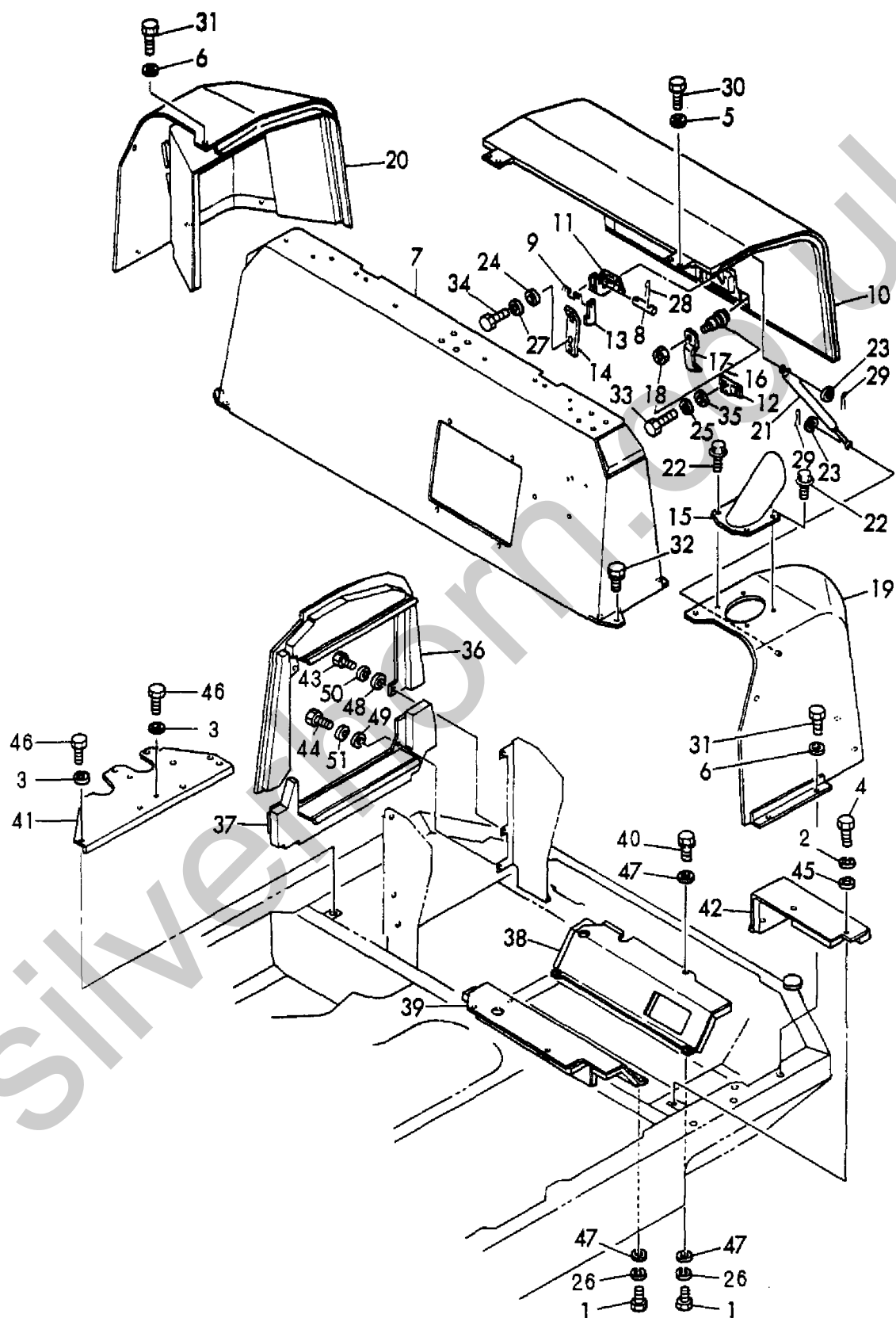
Fig. 50 ボンネット BONNET
