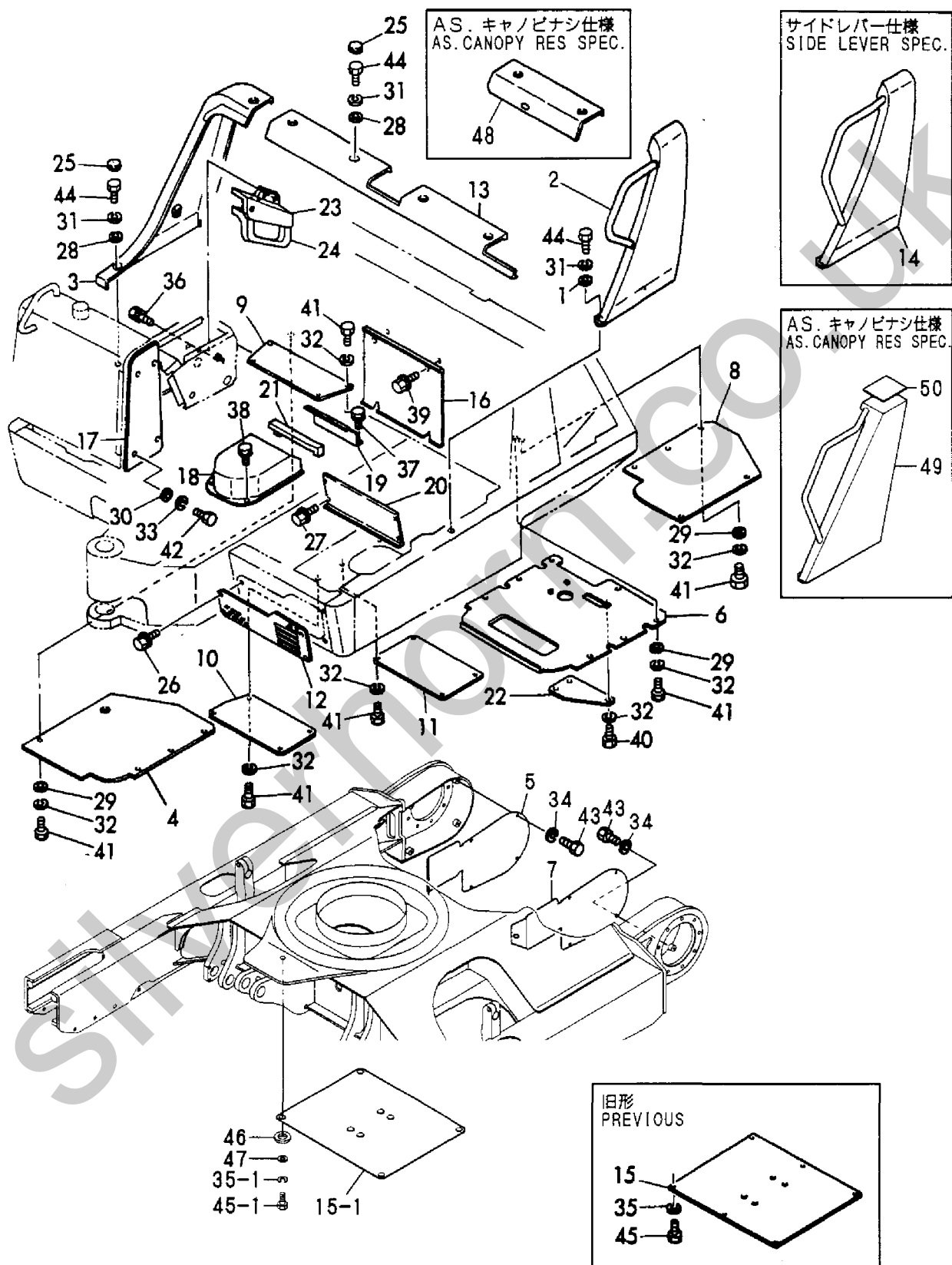
Fig. 42 フレームカバー (キャノピ) FRAME COVER (CANOPY)
