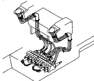
Fig. 92 コントロール配管 (リモコンバルブ ～コントロールバルブ/ダイレクト) (AS) CONTROL PIPING (REMO. -CON. V. ~ CONTROL V. /DIRECT) (AS)
