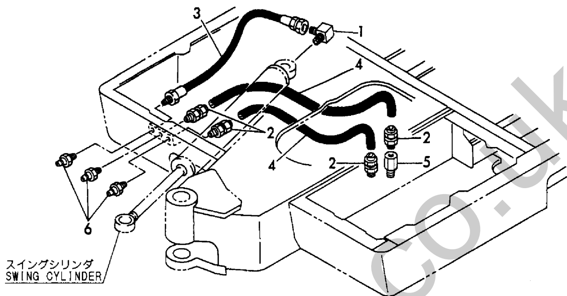
Fig. 98 遠隔グリーシング GREASING
