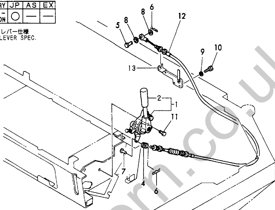
Fig. 10 アクセル ACCELERATOR
