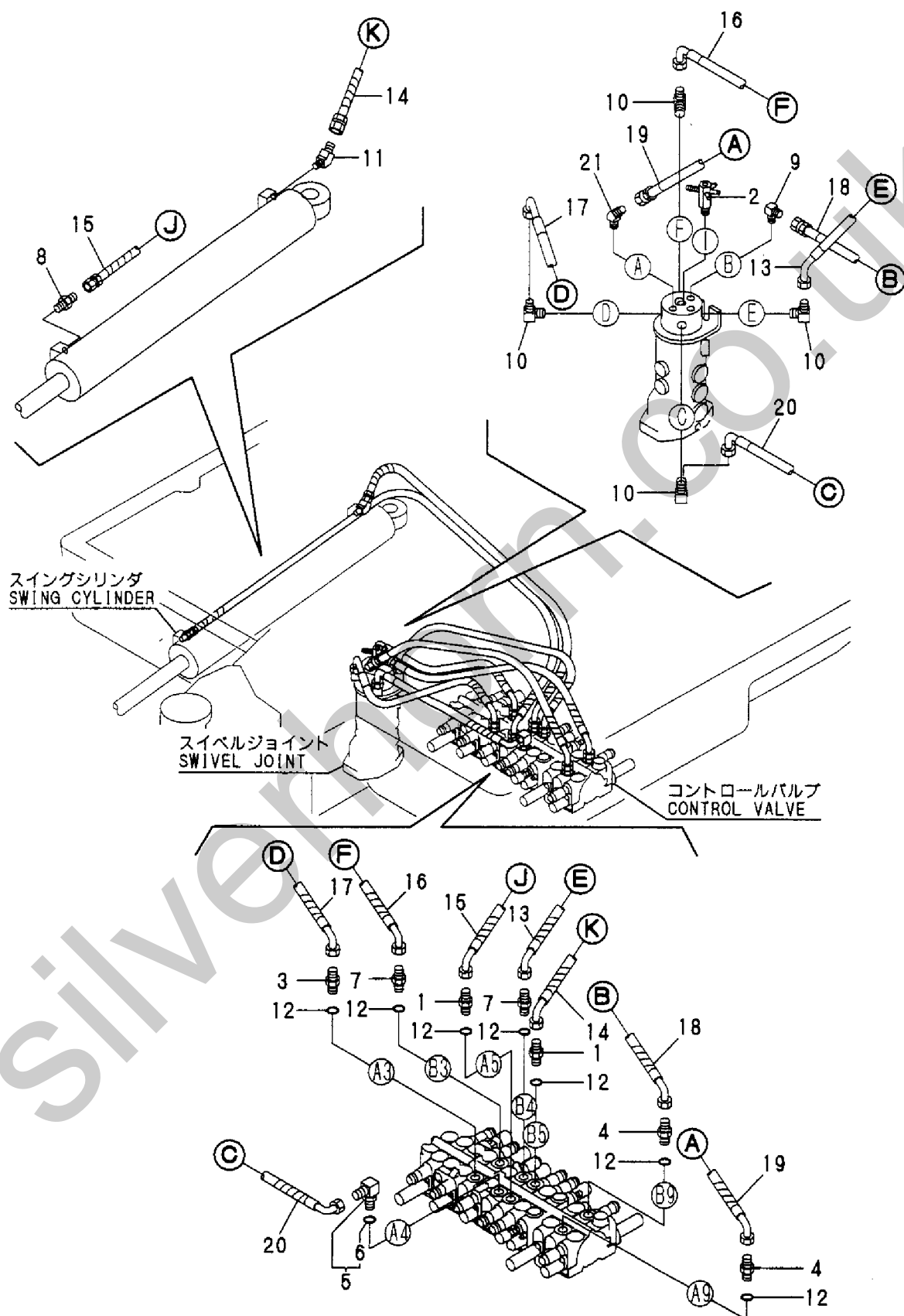
Fig. 79 油圧配管 (バルブ~スイベル、スイング) HYD. OIL PIPING (VALVE~SWIVEL, SWING)
