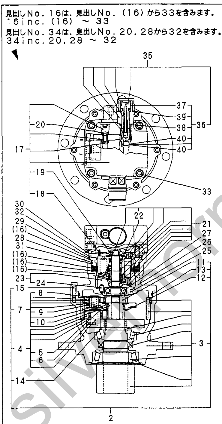
Fig. 64 旋回モータ TURNING MOTOR
