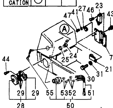
ワンタッチデセルキット (フロント) ONE TOUCH DECEL KIT (FRONT) (172188-08200) Fig. 11 REF No. 1 inc. Fig. 11 REF No. 3 ~ 28 Fig. 13 REF No. 52 ~ 55 Fig. 18 REF No. 59 ~ 81, 84 Fig. 29 REF No. 28 ~ 33
