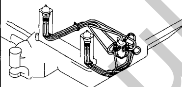
Fig. 94 コントロール配管 (リモコンバルブ ～マルチバルブ /4ウェイ, サイドレバー) CONTROL PIPING (REMO. -CON. V. ~ MULTI V. /4-WAY, SIDE LEVER)
