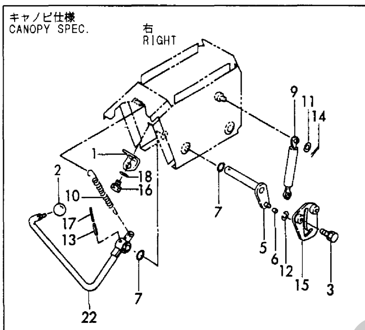
Fig. 38 操縦装置 (カットオフレバー) (AS) CONTROL EQUIP. (CUT OFF LEVER) (AS)
