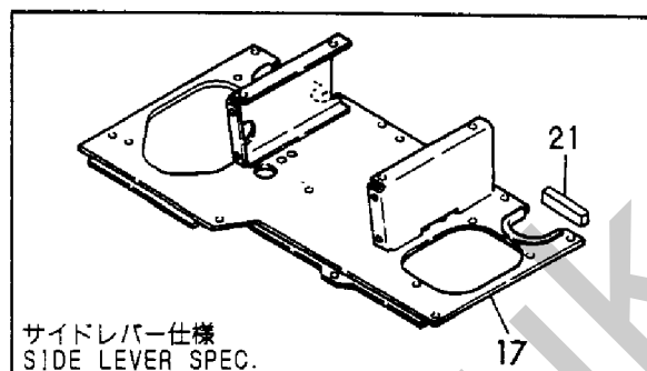
Fig. 48 ステップ STEP
