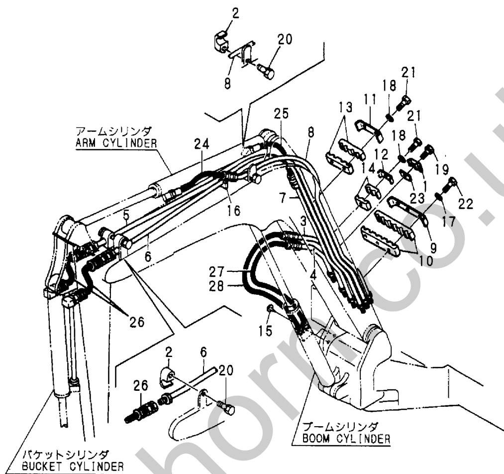
Fig. 83 油圧配管 (ブーム) HYD. OIL PIPING (BOOM)
