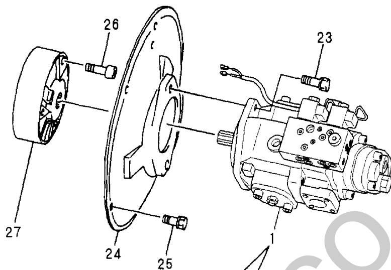
Fig. 55 油圧ポンプ&軸継手 HYD. OIL PUMP & JOINT
