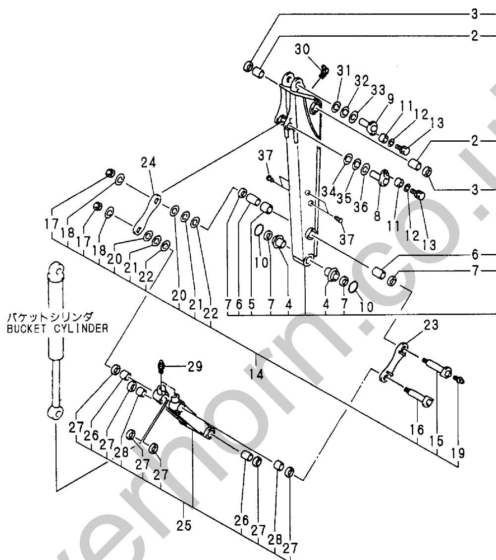
Fig. 100 アーム&バケットリンク ARM & BUCKET LINK
