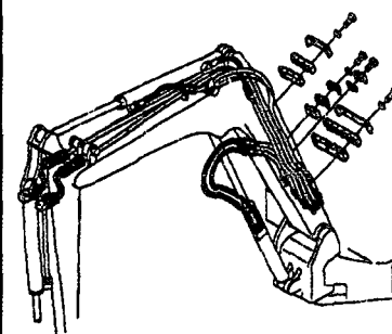
Fig. 84 油圧配管 (PTOフレームエンド) HYD. OIL PIPING (P.T.O. FRAME END)
