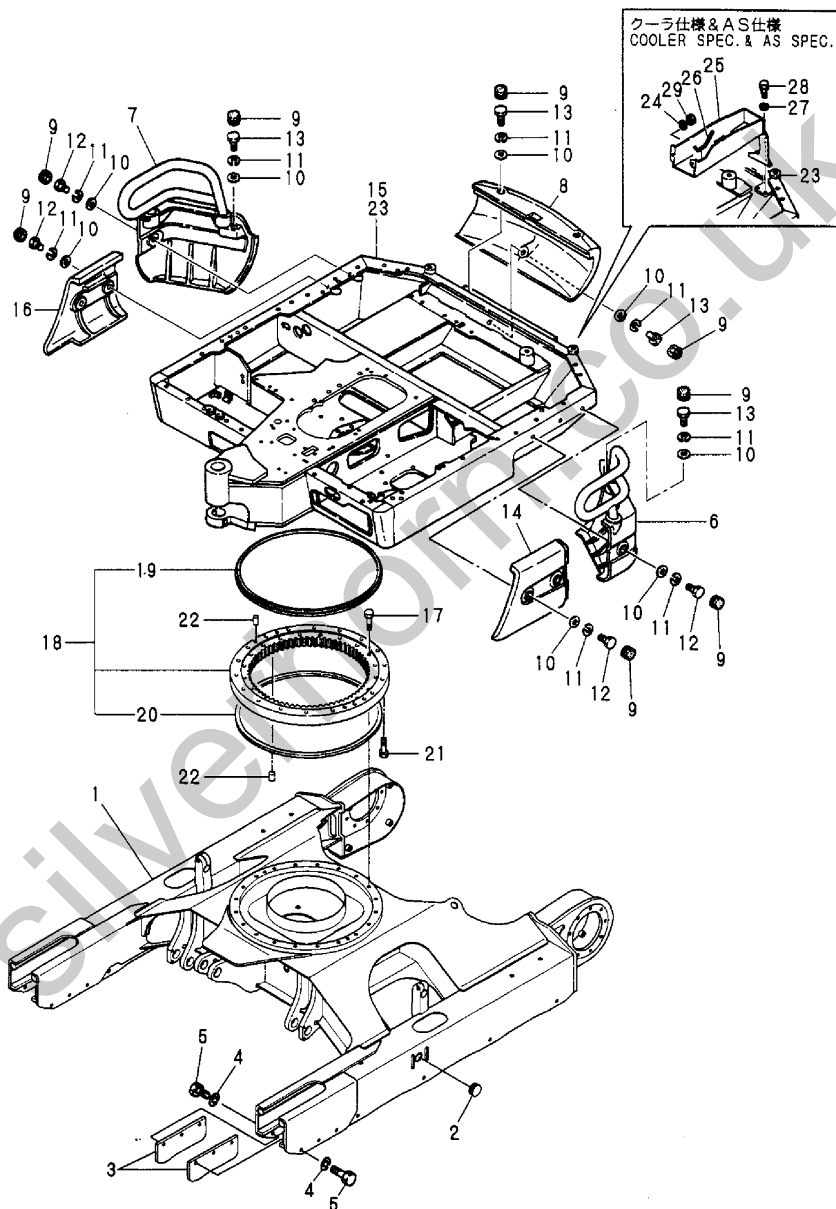
Fig. 40 フレーム&旋回ベアリング FRAME & TURNING BEARING
