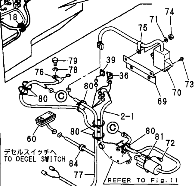
キャビン仕様 CABIN SPEC. キャノピフロント仕様 CANOPY FRONT SPEC.
