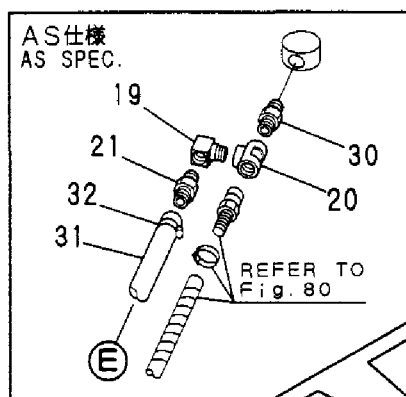
Fig. 84 油圧配管 (PTOフレームエンド) HYD. OIL PIPING (P. T. O. FRAME END)
