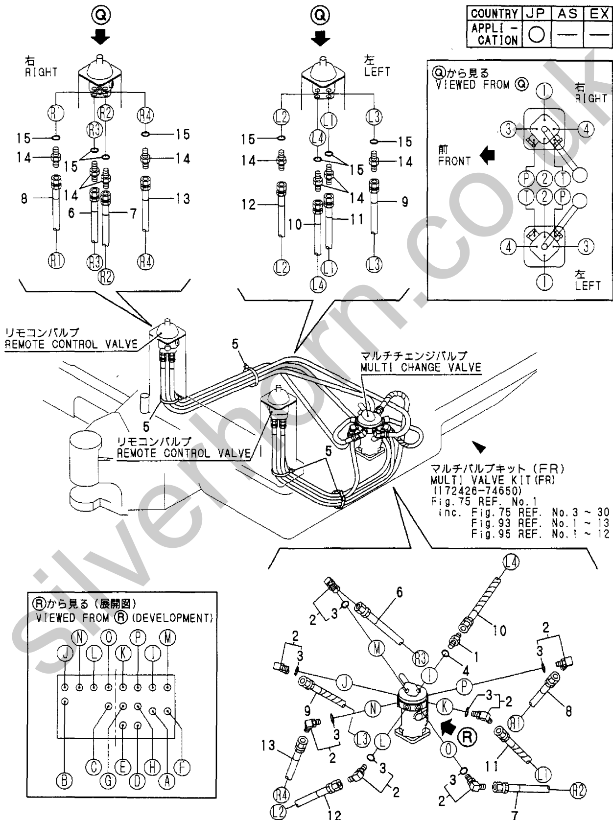
Fig. 93 コントロール配管 (リモコンバルブ~マルチバルブノ4ウェイ, フロントレバー) CONTROL PIPING (REMO.-CON. V. ~ MULTI V./4-WAY, FRONT LEVER)
