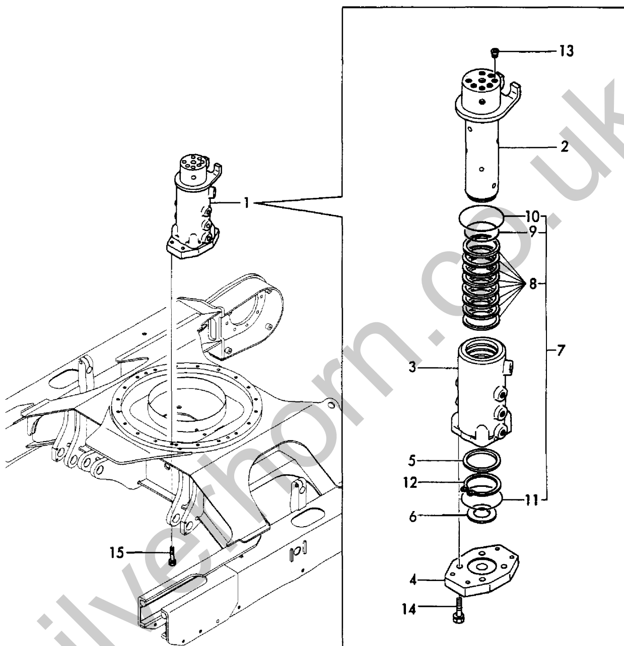
Fig. 65 スイベルジョイント SWIVEL JOINT
