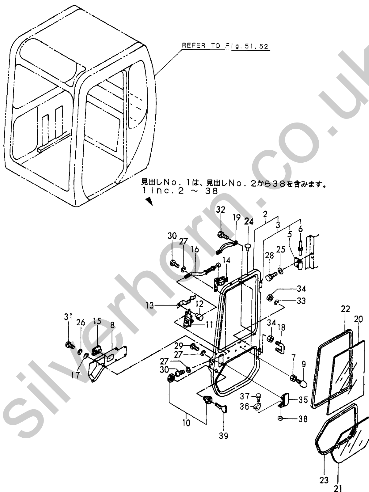
Fig. 53 キャビンドア CABIN DOOR
