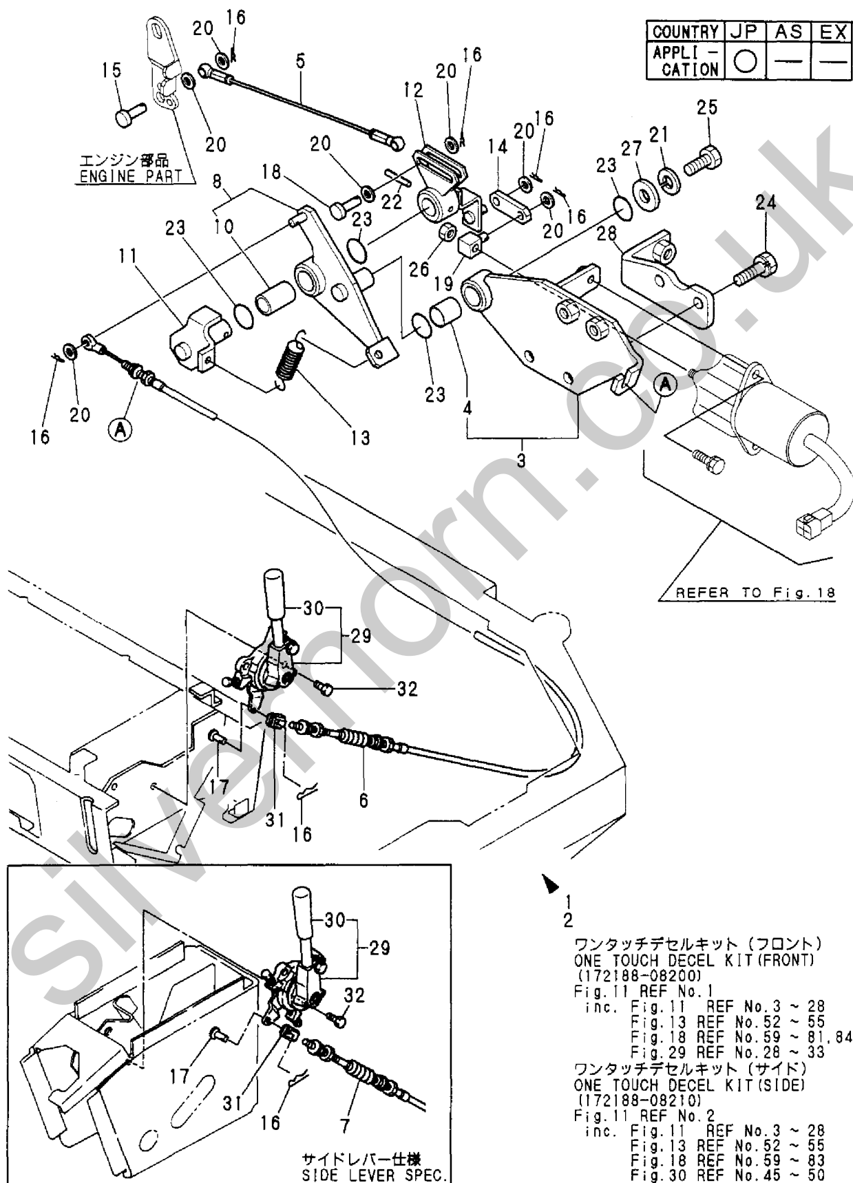
Fig. 11 アクセル (ワンタッチデセル) ACCELERATOR (ONE TOUCH DECEL)
