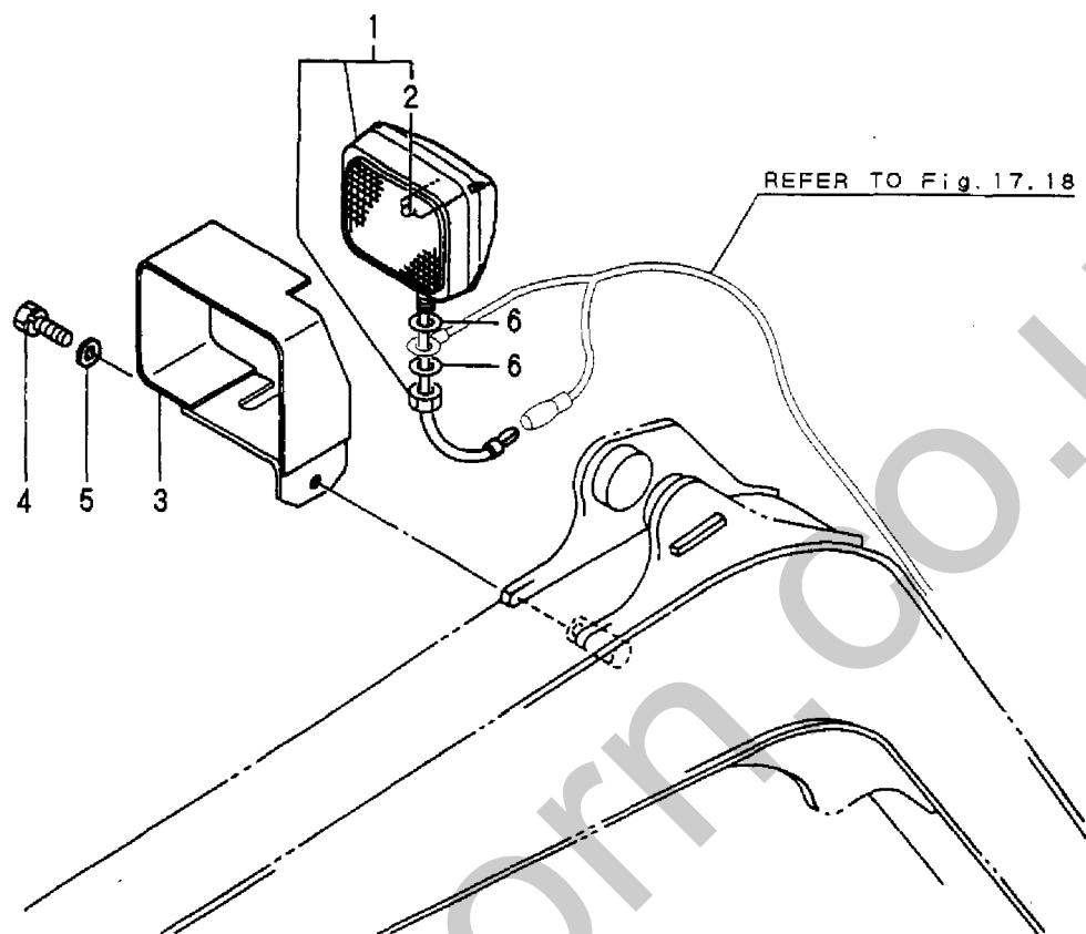
Fig. 21 ワークランプ WORK LAMP
