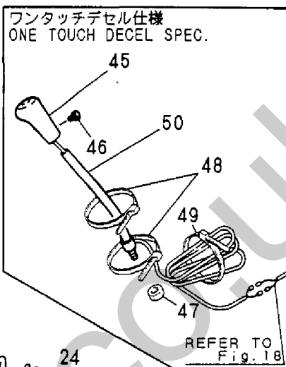
Fig. 30 操縦装置 (リンク台&作業レバー/サイドレバー) CONTROL EQUIP. (LINK STAND & OPERATION LEVER /SIDE LEVER)
