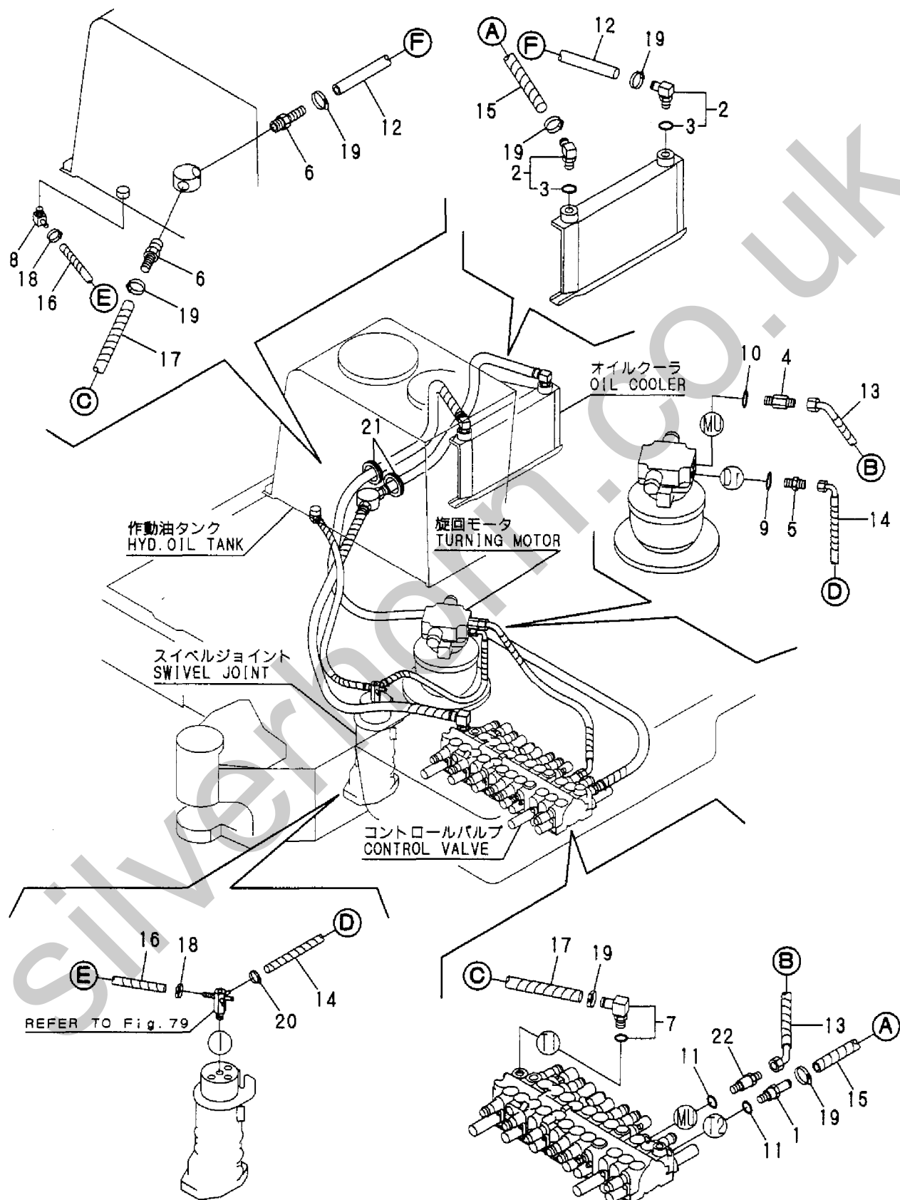
Fig. 80 油圧配管 (リターン: 1) HYD. OIL PIPING (RETURN: 1)
