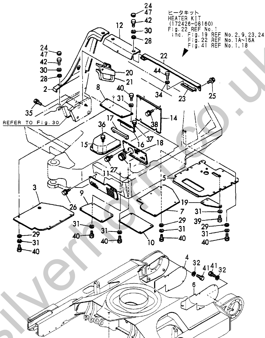
Fig. 41 フレームカバー (キャビン) FRAME COVER (CABIN)
