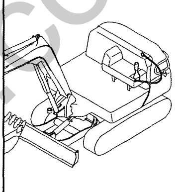
Fig. 11 アクセル (ワンタッチデセル) ACCELERATOR (ONE TOUCH DECEL)
