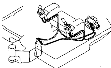
Fig. 89 コントロール配管 (ポンプ～リモコン バルブ～リターン) (AS) CONTROL PIPING (PUMP ~ REMO. -CON. V. ~ RETURN) (AS)
