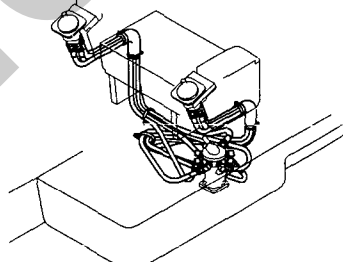
Fig. 95 コントロール配管 (マルチバルブ ～コントロールバルブ /4ウェイマルチ) CONTROL PIPING (MULTI V. ~ CONTROL V. /4-WAY MULTI)
