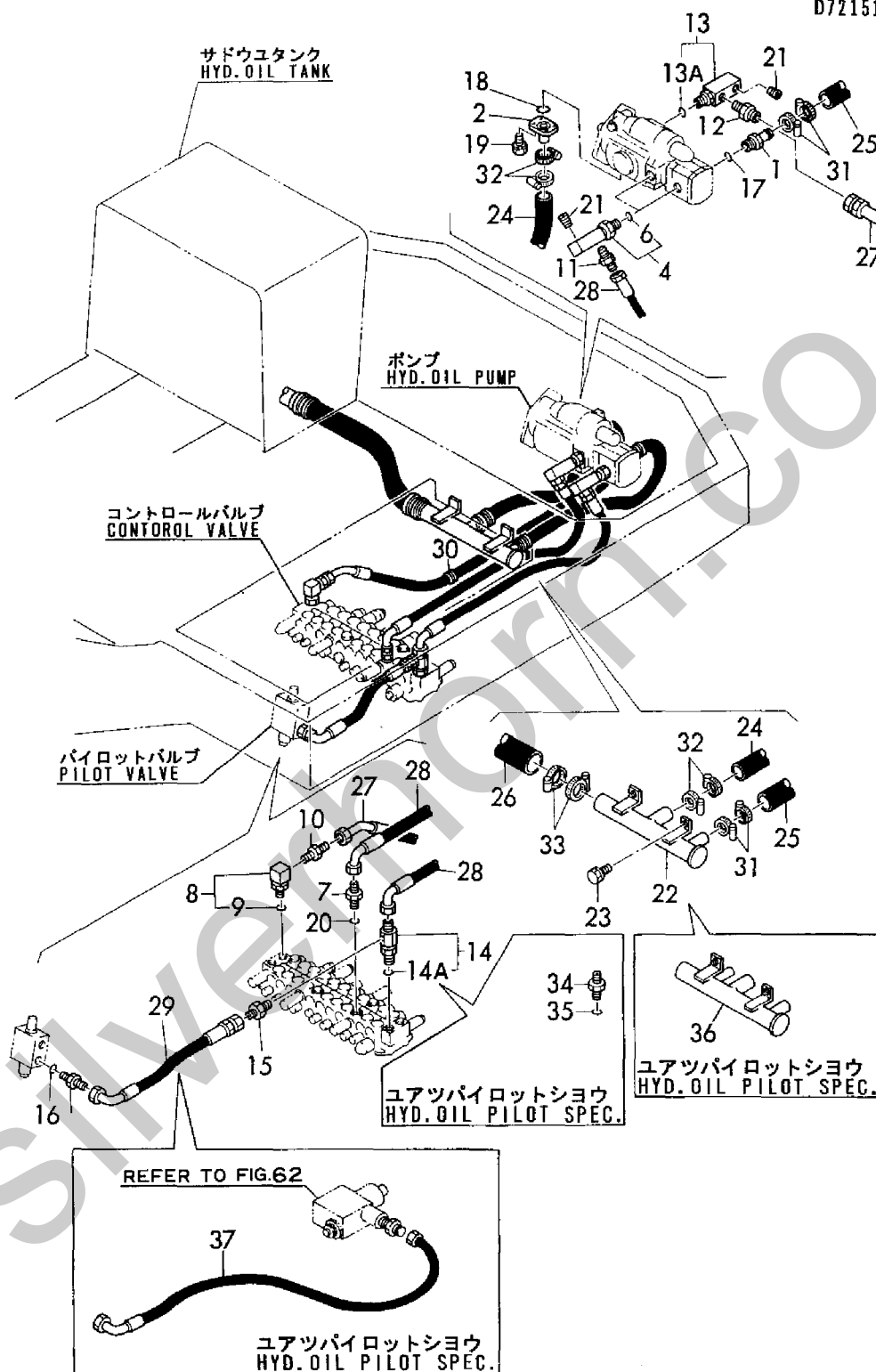
Fig. 67 ユアツハイカン(タンク-ポンプ-バルブ) HYD. OIL PIPING (TANK-PUMP-VALVE)
