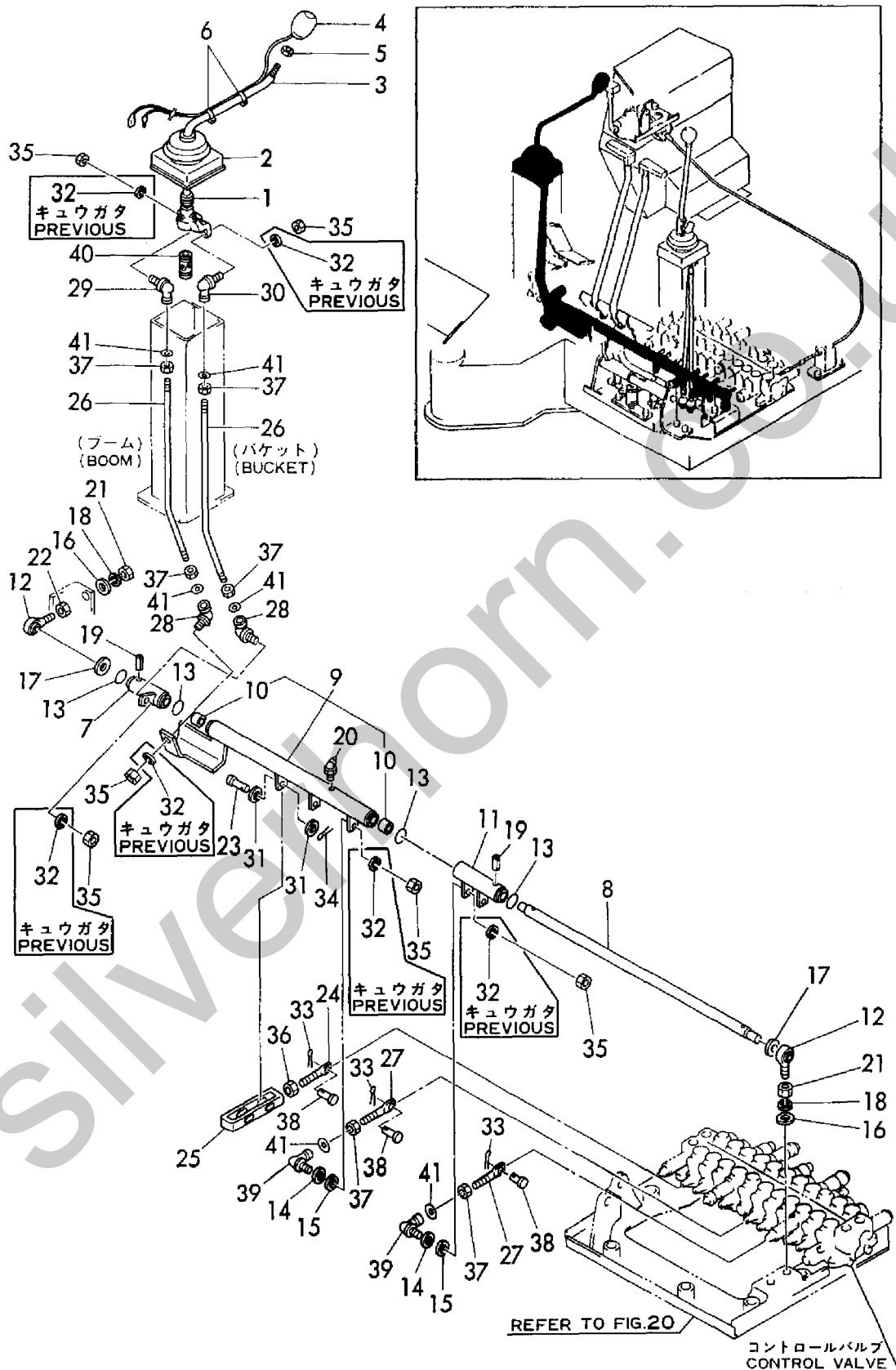
Fig. 22 ソウジュウソウチ(ブーム&バケット) CONTROL EQUIPMENT (BOOM & BUCKET)
