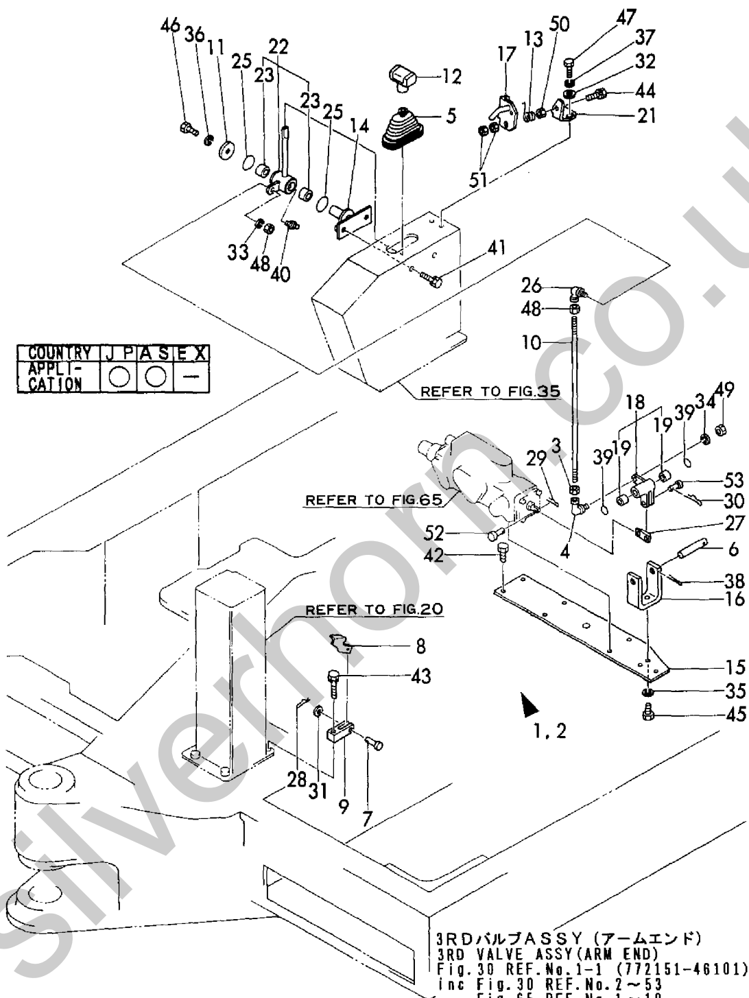
Fig. 30 ソウジュウソウチ(3RDバルブ) CONTROL EQUIPMENT (3RD VALVE)
