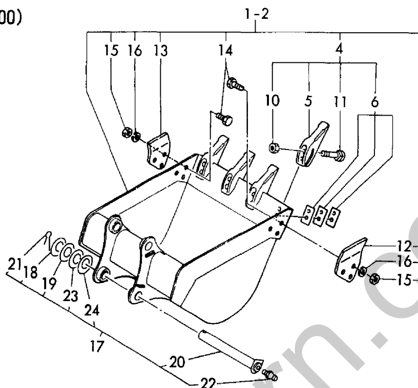
Fig. 84 バケット(650, 700) BUCKET (650, 700)
