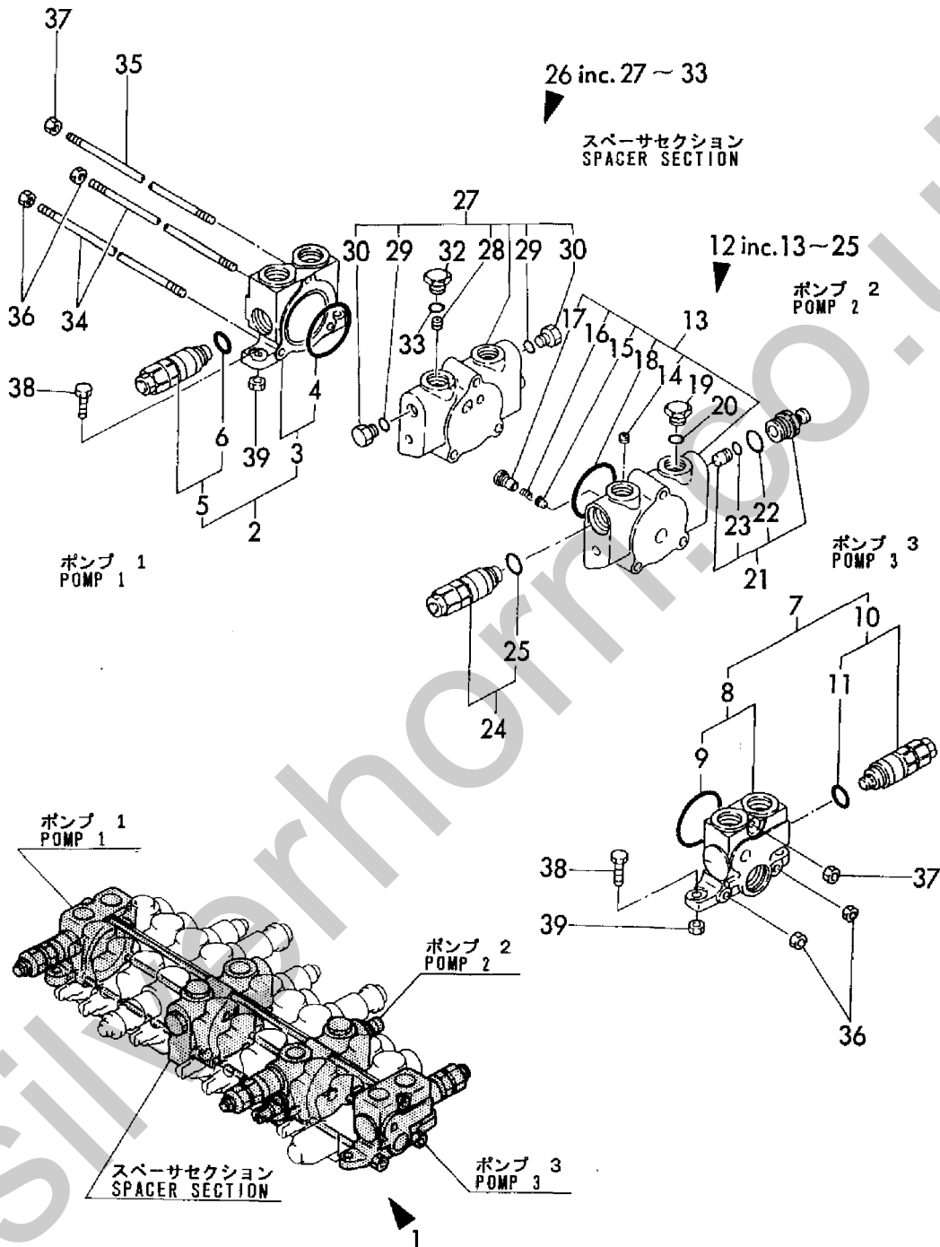
Fig. 51 コントロールバルブ(Pポート) CONTROL VALVE (P PORT)
