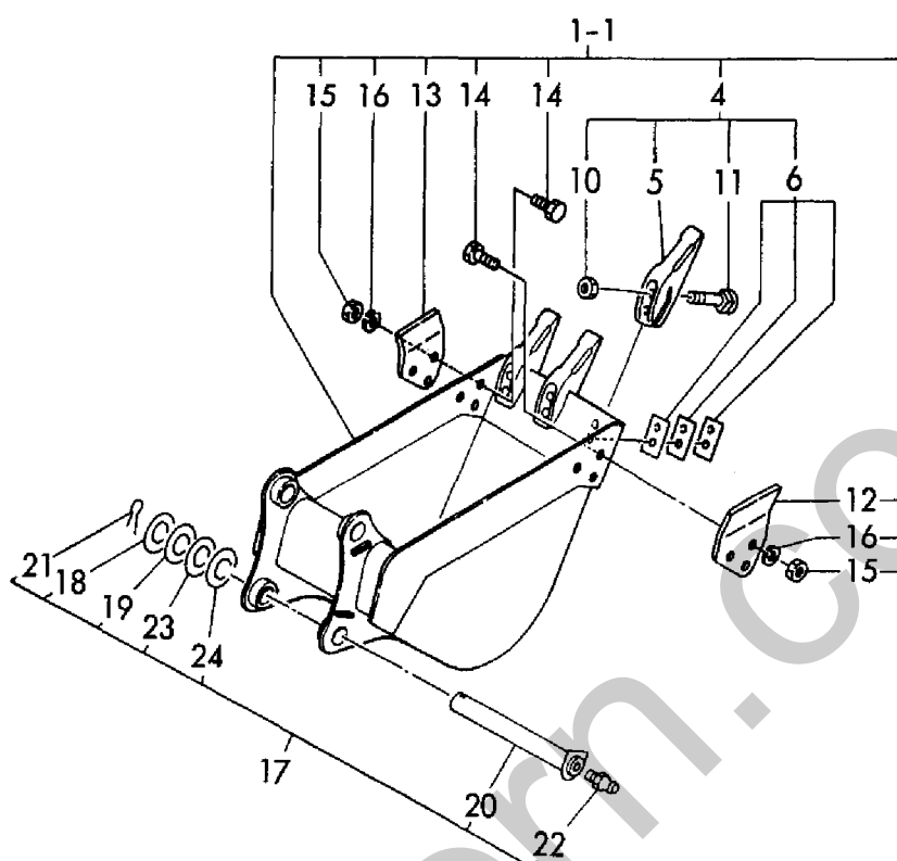
Fig. 85 バケット(400,450)(アタッチメント) BUCKET (400,450)(ATTACHMENT)
