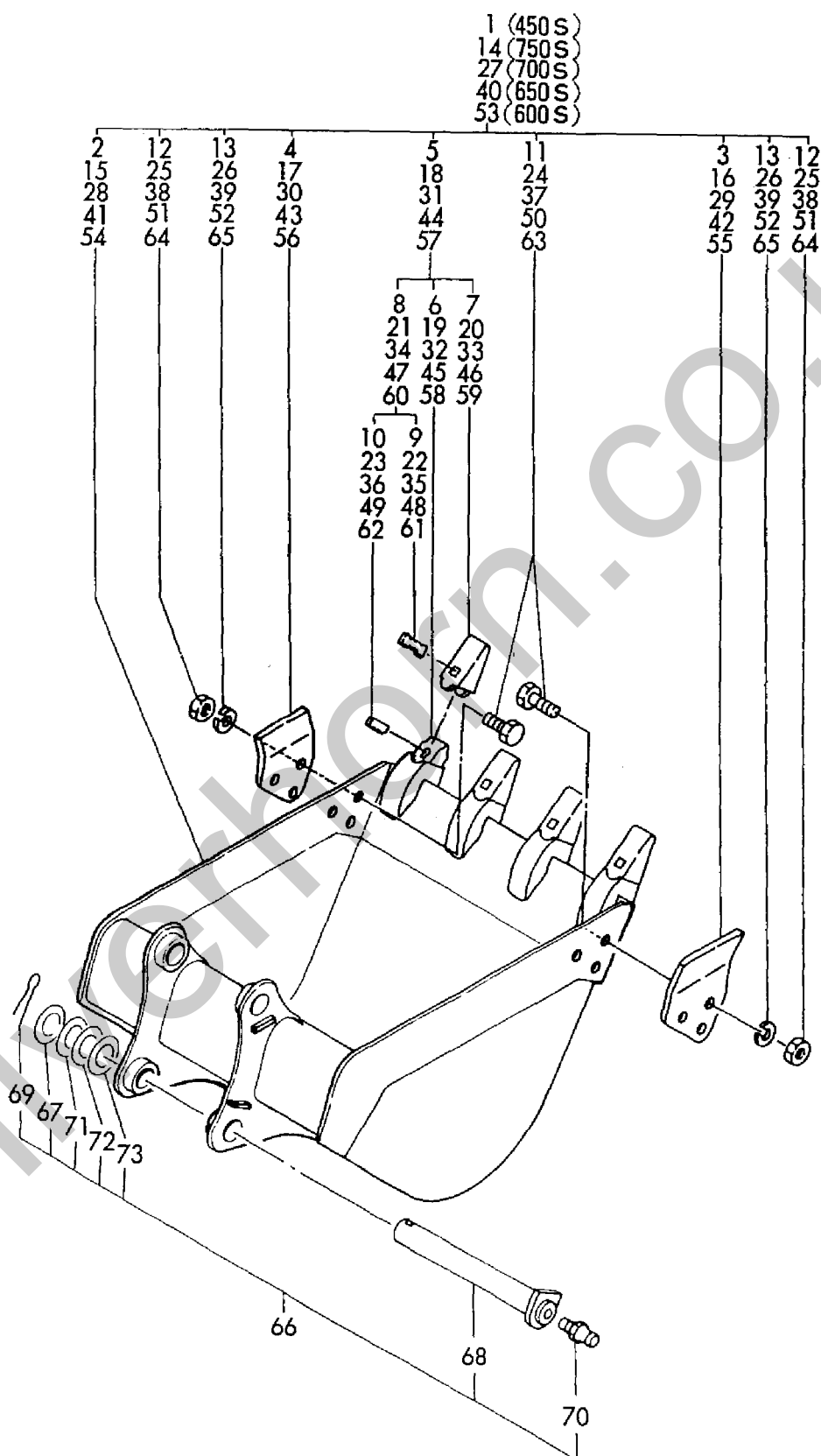
Fig. 90 バケット(Sタイプ)(アタッチメント) BUCKET(S TYPE)(ATTACHMENT)
