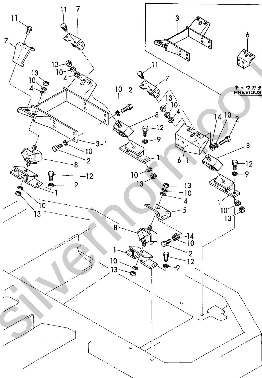
Fig. 8 エンジンマウント ENGINE MOUNT
