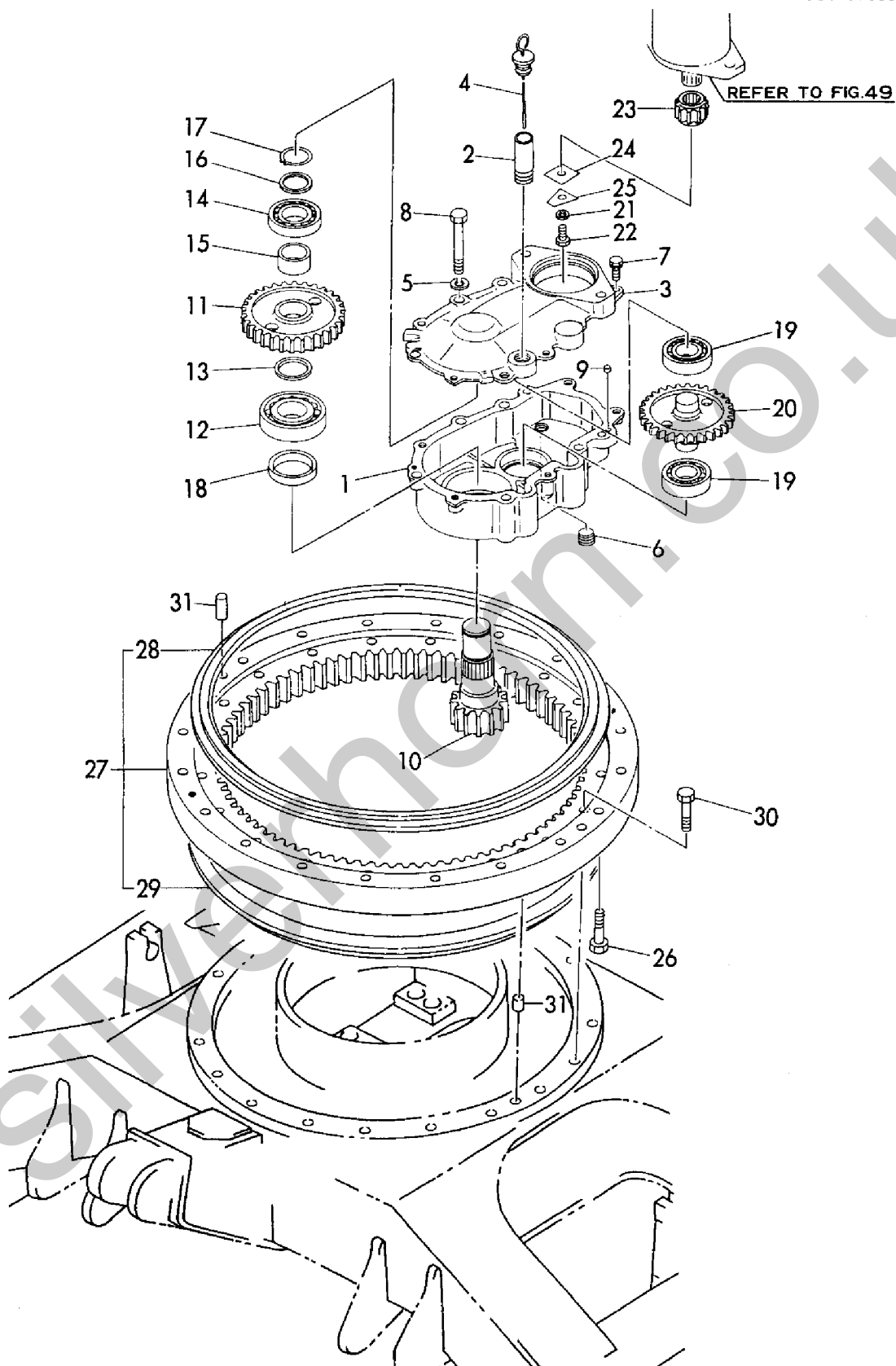
Fig. 34 センカイクドウソウチ SWING DRIVING GEARS
