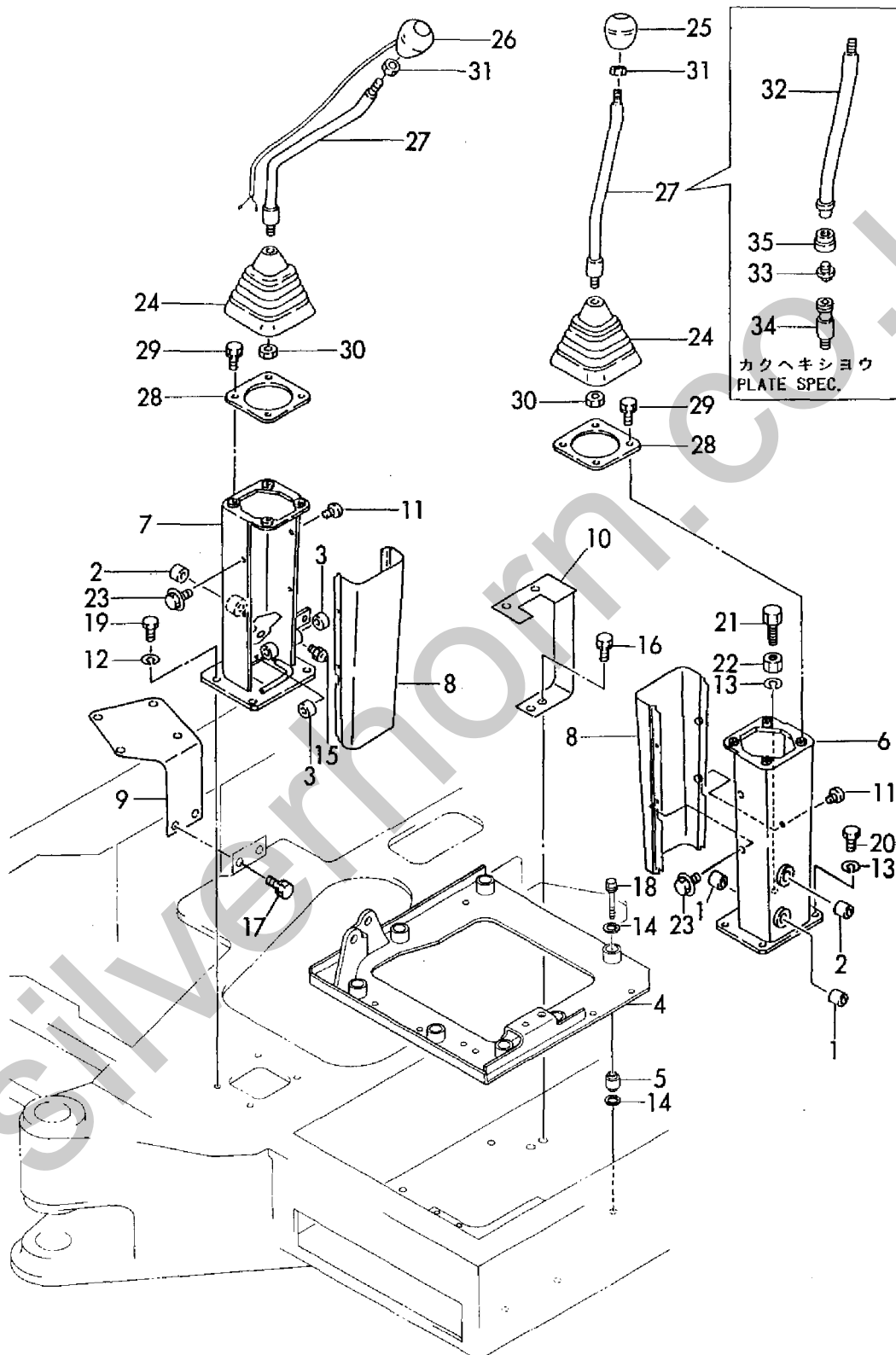
Fig. 21 ソウジュウソウチ (レバースタンド CONTROL EQUIPMENT (LEVER STAND & リンクダイ (ユアツパイロット) & LINK STAND) (HYD. OIL PILOT)
