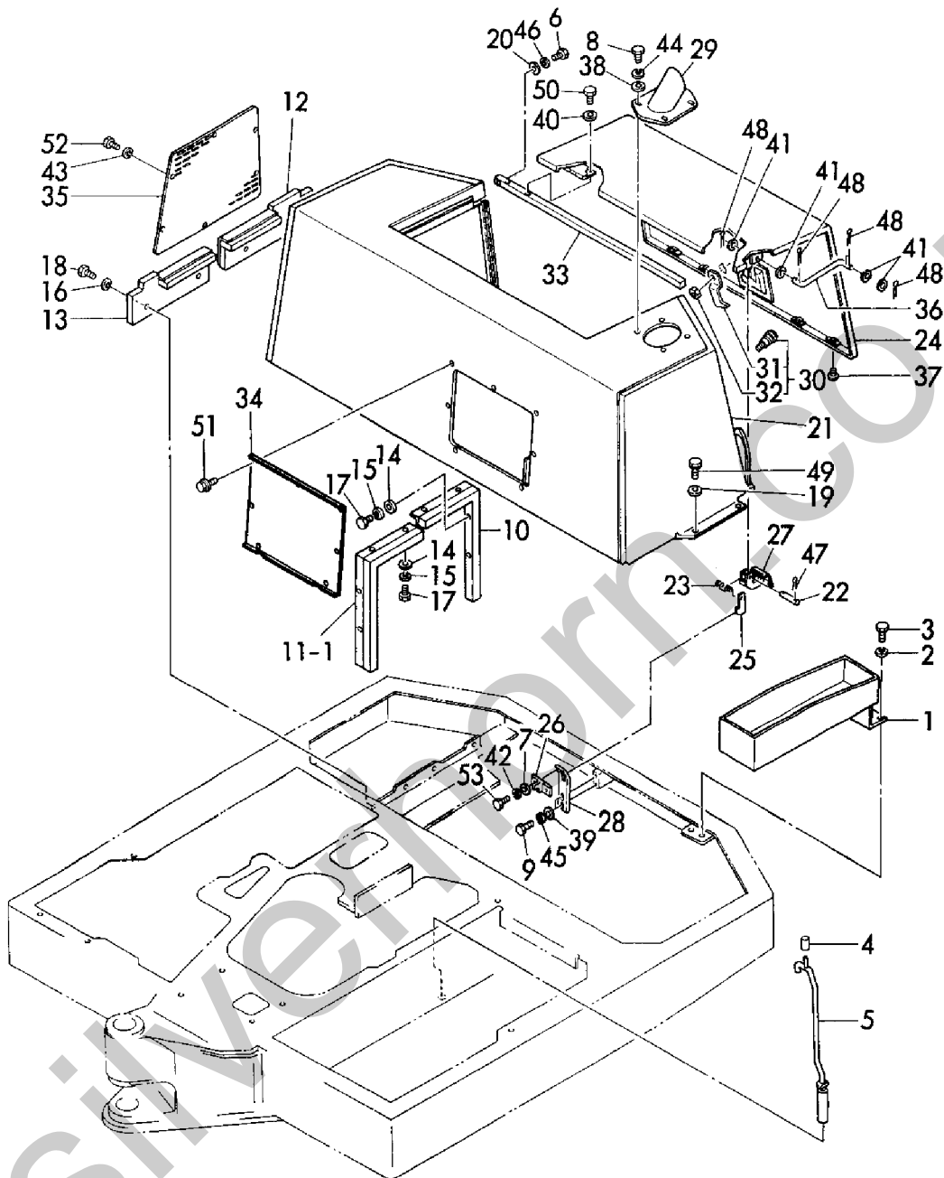
Fig. 37 ボンネット BONNET
