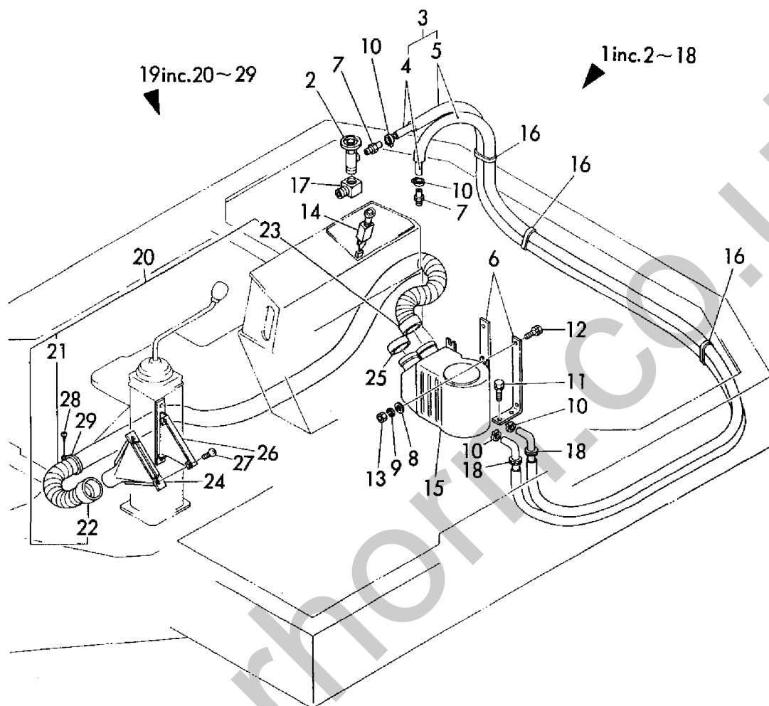
Fig. 15 ヒータ&デフロスタ HEATER & DEFROSTER
