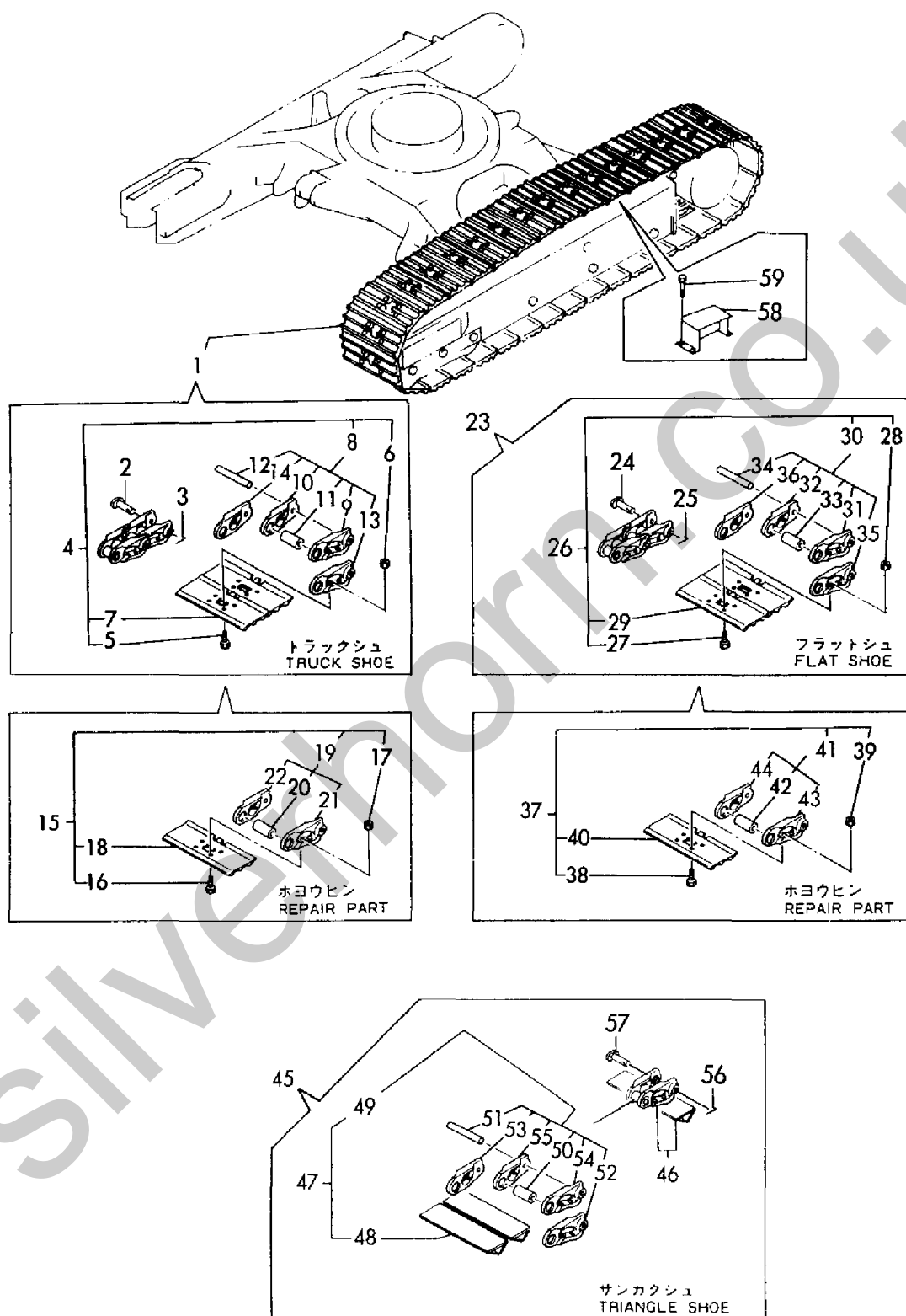
Fig. 92 クローラ(アタッチメント) CRAWLER (ATTACHMENT)
