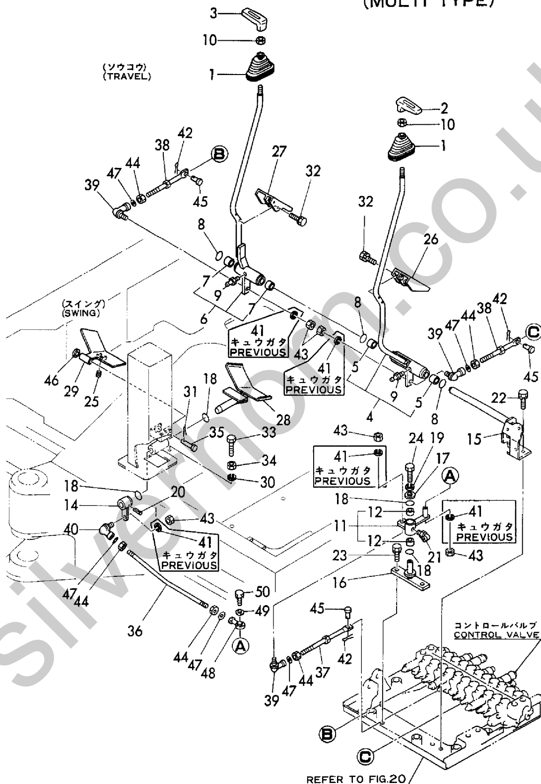
Fig. 28 ソウジュウソウチ(ソウコウ&スイング) CONTROL EQUIPMENT (TRAVEL & SWING) (マルチタイプ) (MULTI TYPE)
