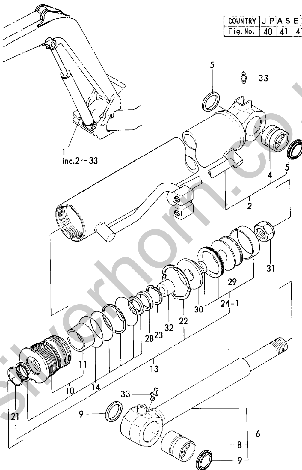
Fig. 40 ブームシリンダ(キャビン) BOOM CYLINDER(CABIN)
