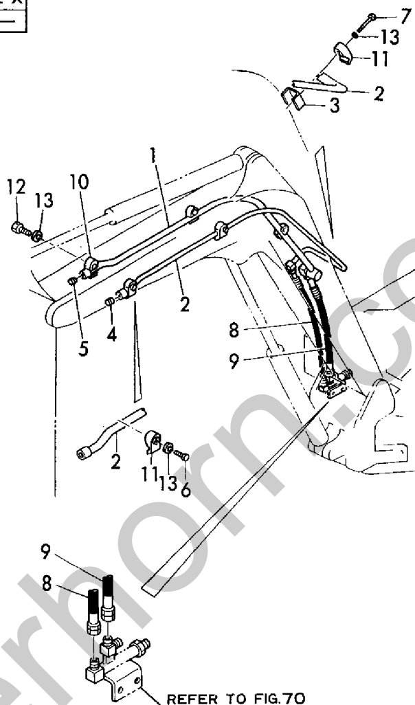
Fig. 74 ユアツハイカン(3RDバルブ, ブームエンド) HYD. OIL PIPING (3RD VALVE, BOOM END)
