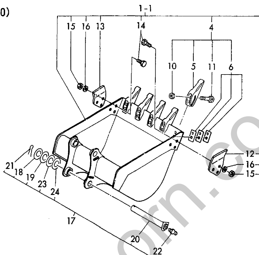
Fig. 88 バケット(700,750)(アタッチメント) BUCKET (700,750) (ATTACHMENT)
