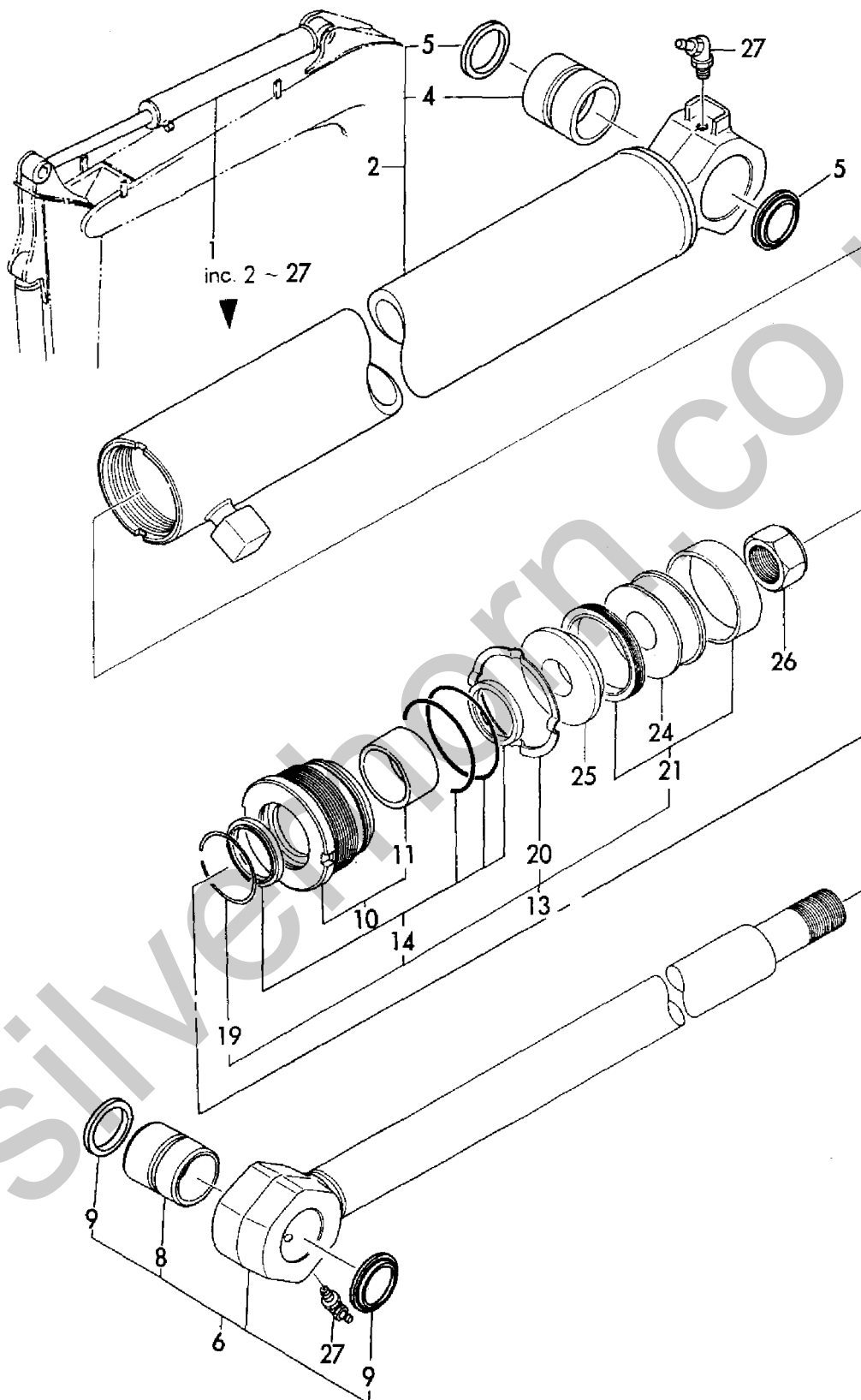
Fig. 43 アームシリンダ ARM CYLINDER
