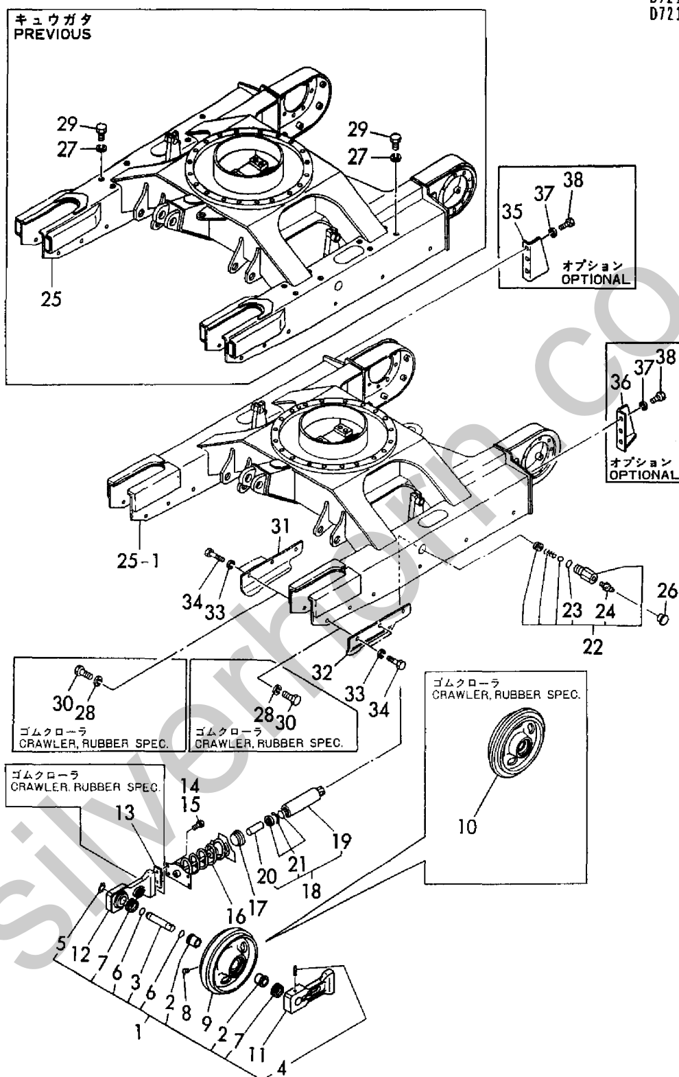
Fig. 18 トラックフレーム&アイドラ TRACK FRAME & IDLER
