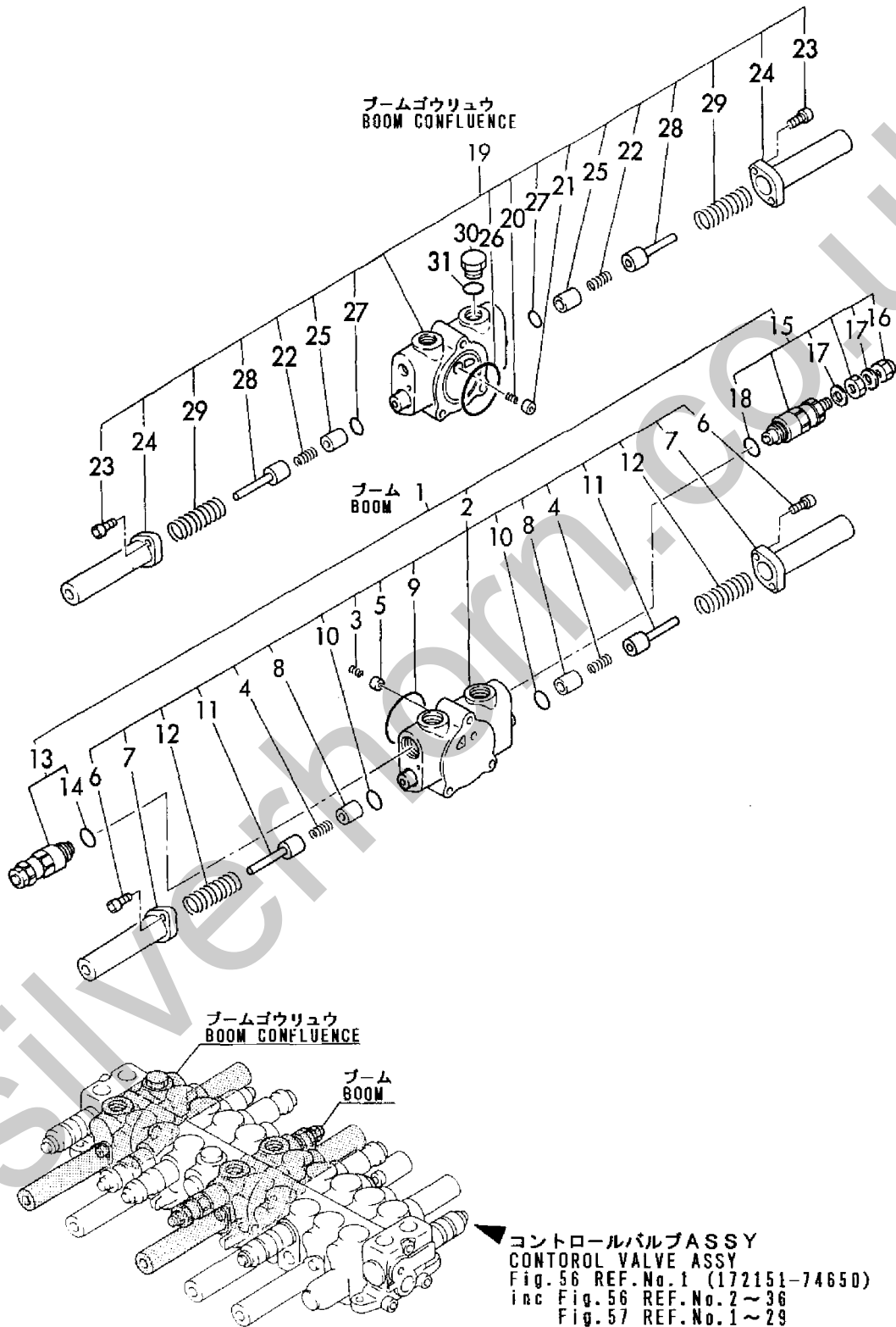
Fig. 57 コントロールバルブ(ブーム)(ユアツパイロット) CONTROL VALVE(BOOM)(HYD. OIL PILOT)
