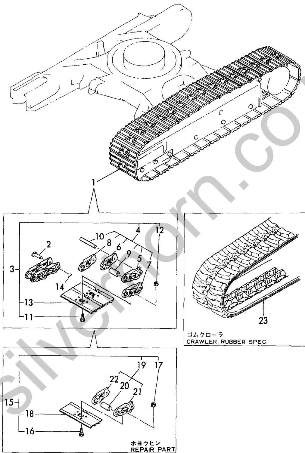
Fig. 19 クローラ(380) CRAWLER (380)
