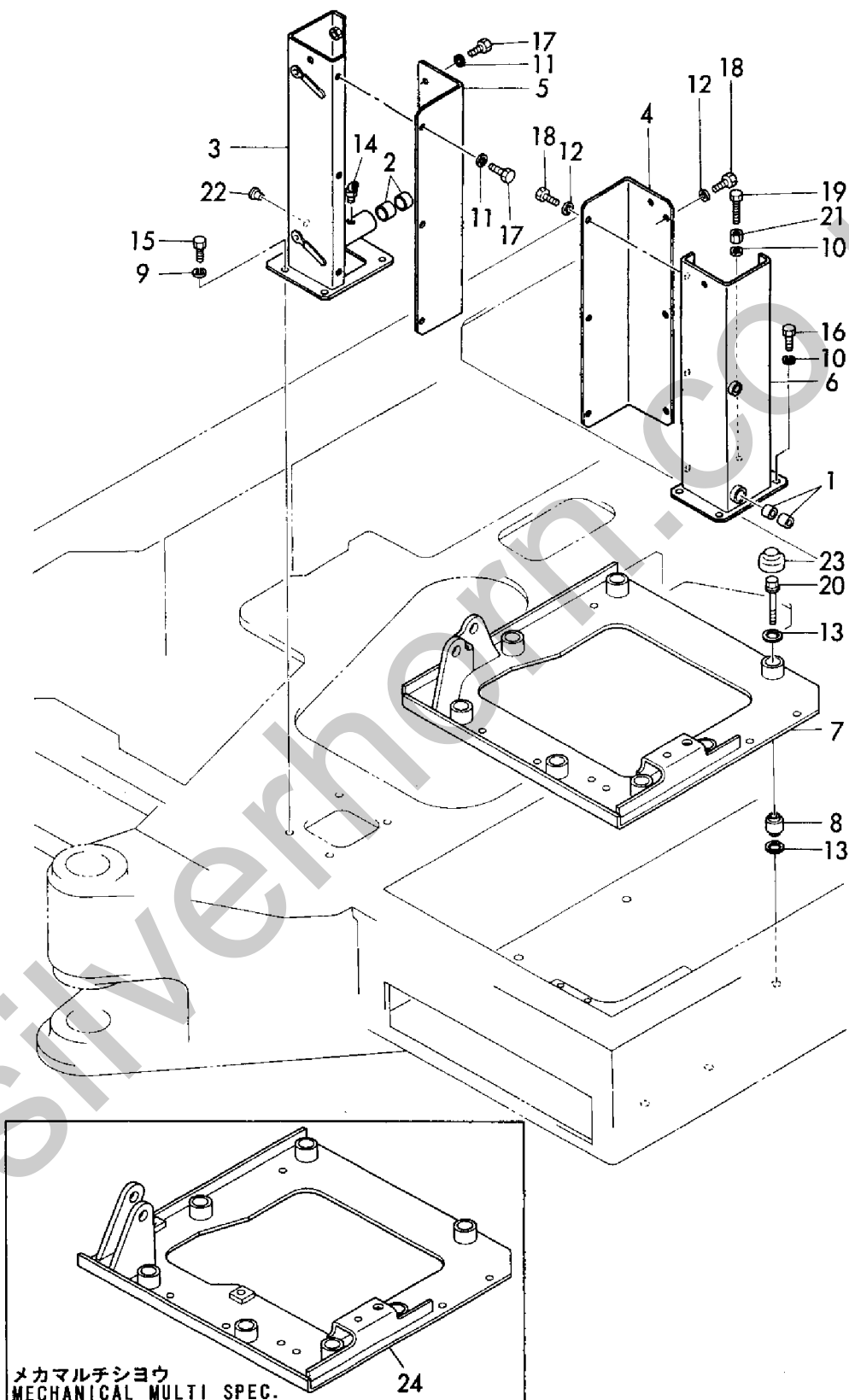
Fig. 20 ソウジュウソウチ (レバースタンド&リンクダイ) CONTROL EQUIPMENT (LEVER STAND & LINK STAND)
