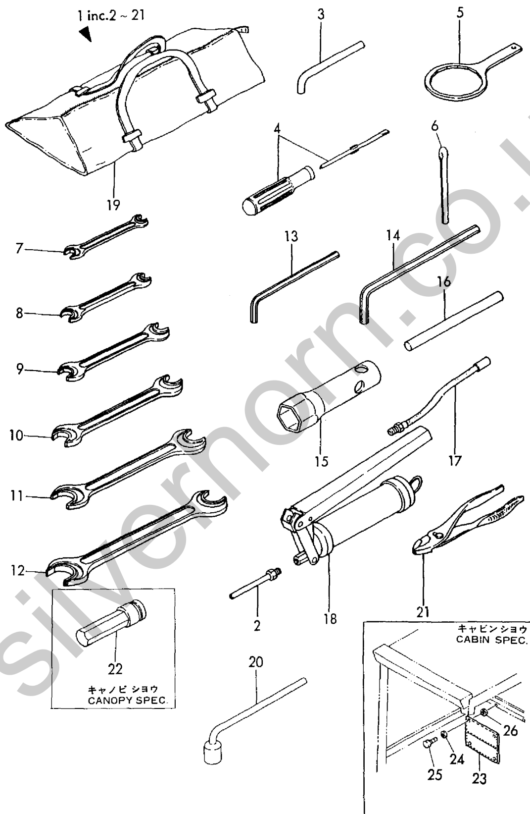
Fig. 5 コウグ TOOL
