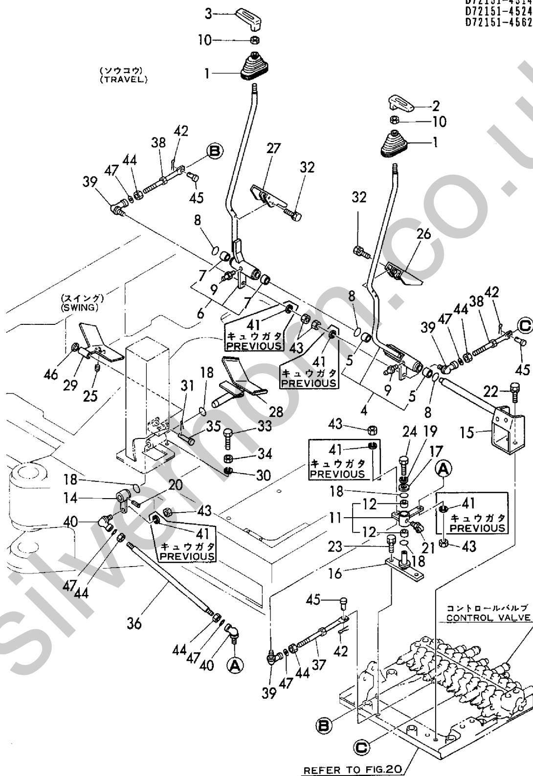
Fig. 27 ソウジュウソウチ(ソウコウ&スイング) CONTROL EQUIPMENT (TRAVEL & SWING)
