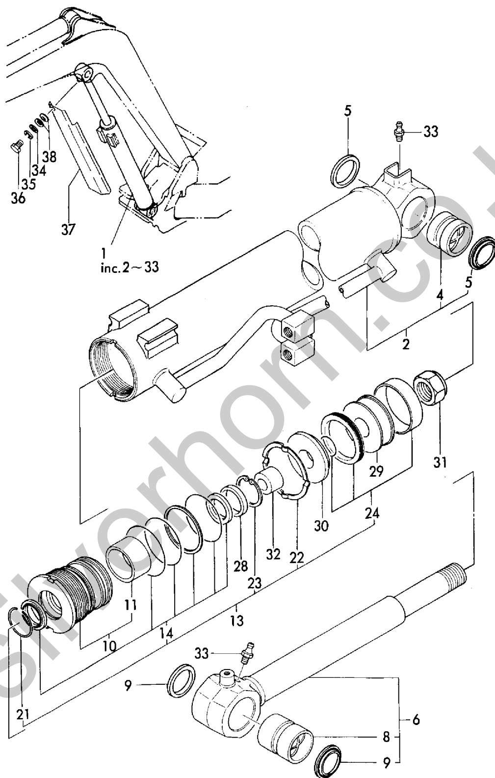
Fig. 42 ブームシリンダ(キャノピ) BOOM CYLINDER(CANOPY)
