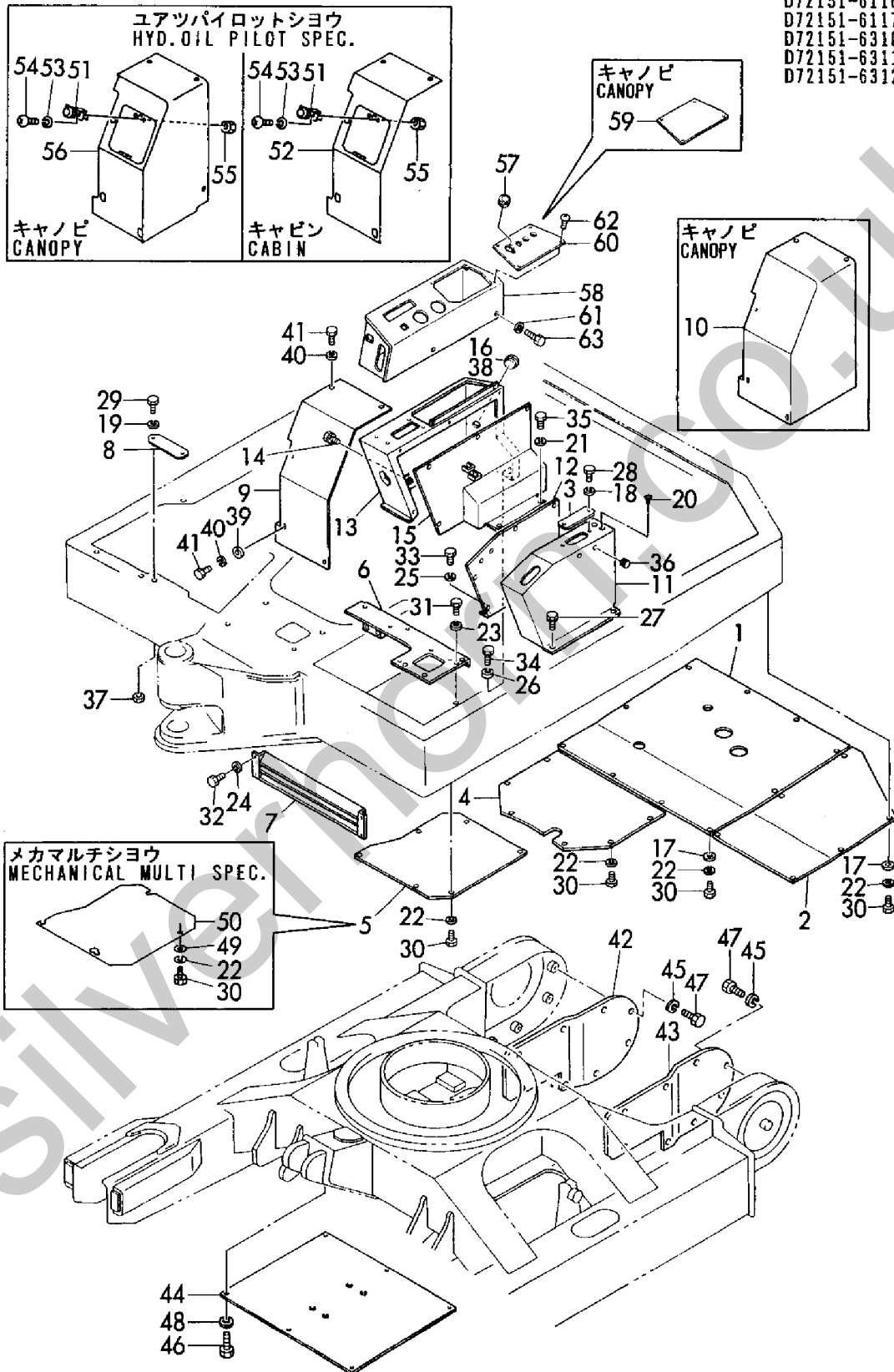
Fig. 35 フレームカバー FRAME COVER
