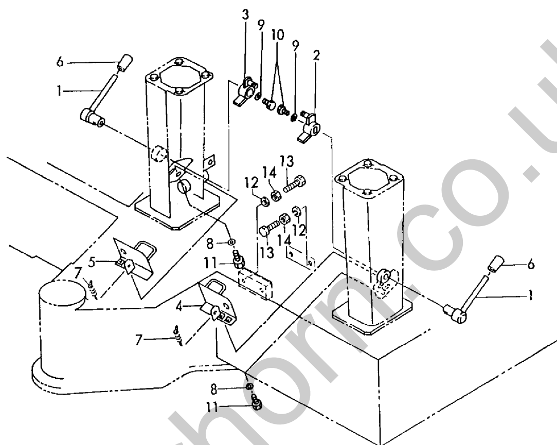
Fig. 32 サギョウレバーストッパ(ユアツコントロール) OPERATION LEVER STOPPER (HYD. OIL CONTROL)
