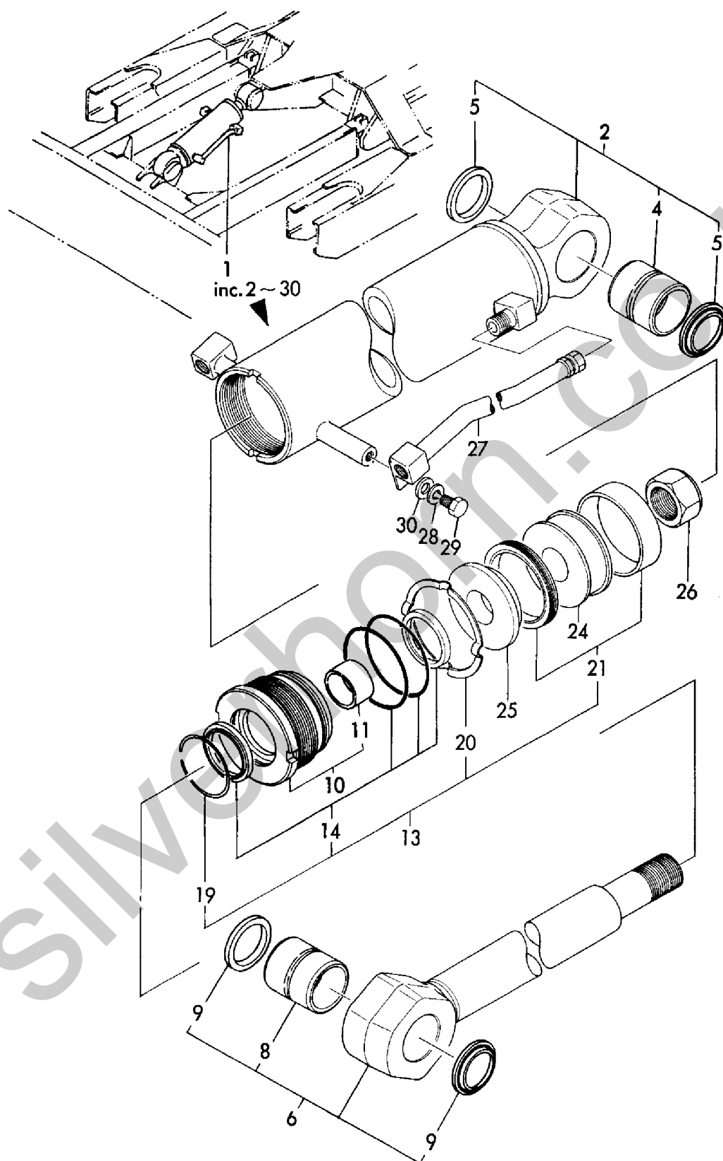
Fig. 46 ブレードシリンダ BLADE CYLINDER
