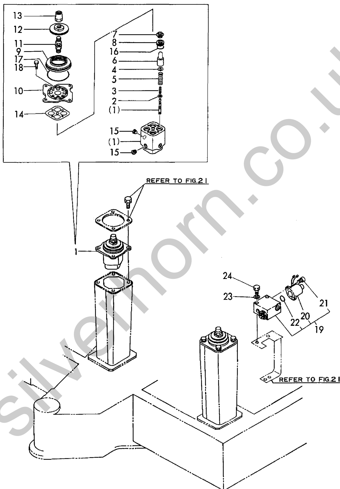
Fig. 62 リモコンバルブ&カutoffバルブ REMOTE CONTROL VALVE & CUT OFF VALVE
