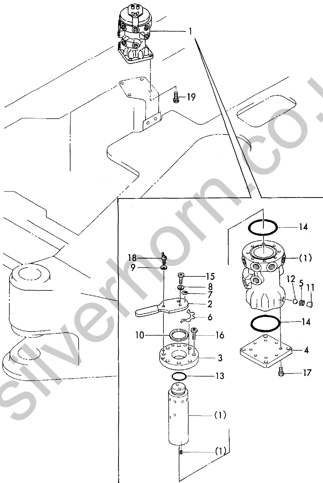
Fig. 63 ロータリバルブ(ユアツマルチ) ROTARY VALVE (HYD. OIL MULTI)
