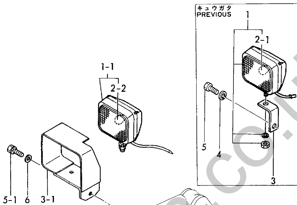
Fig. 14 ワークランプ WORK LAMP
