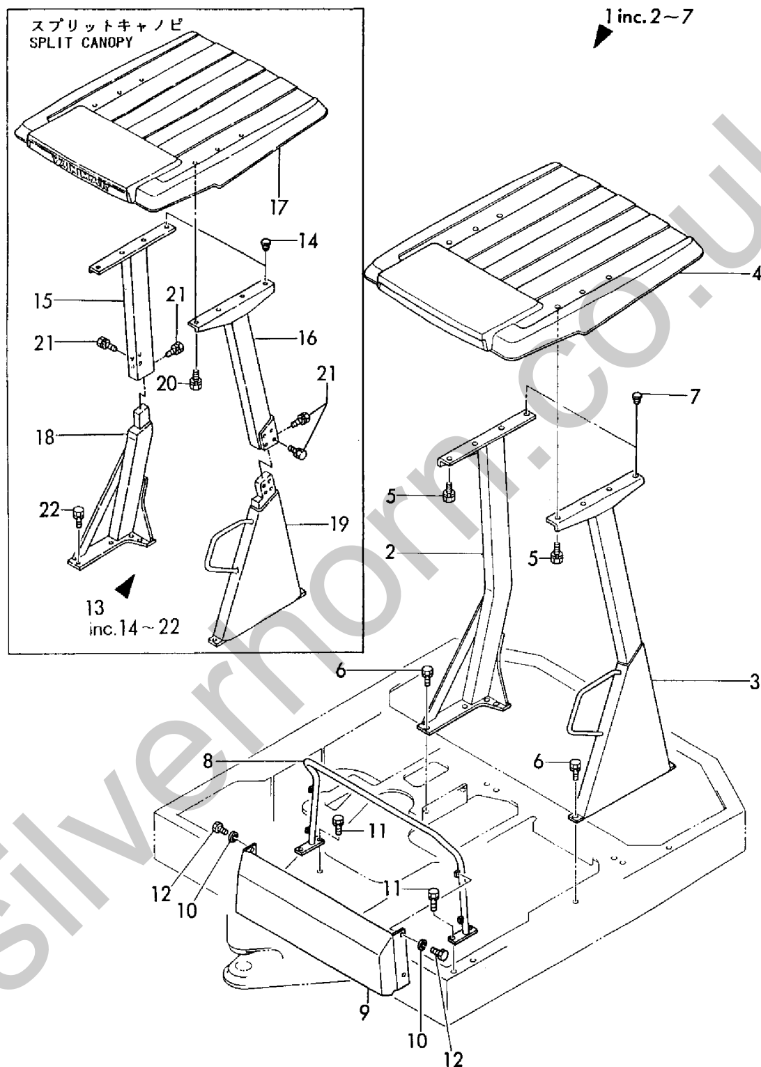
Fig. 39 キャノピ CANOPY
