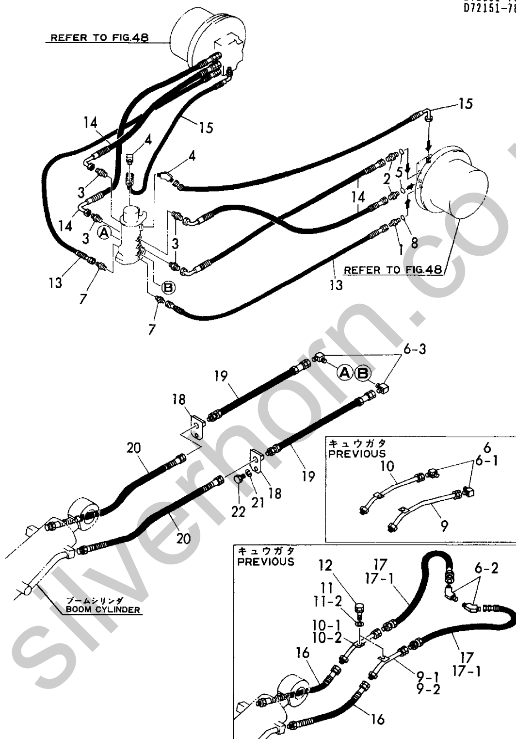
Fig. 72 ユアツハイカン(ソウコウ) HYD. OIL PIPING (TRAVEL)
