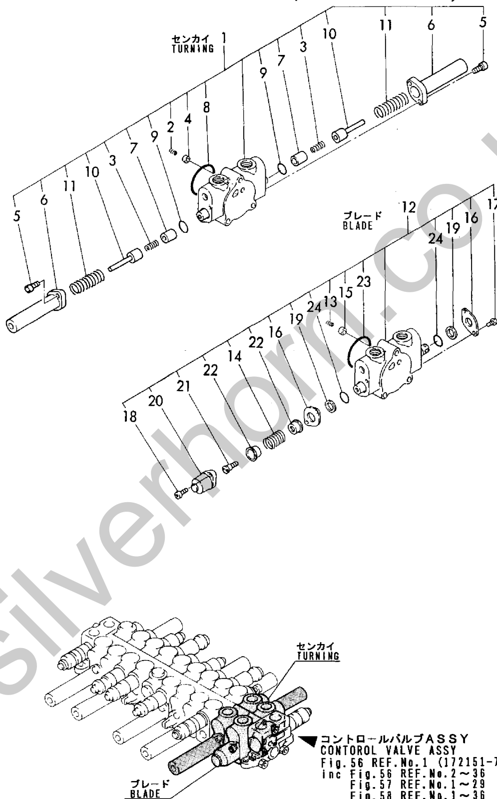
Fig. 60 コントロールバルブ(ブレード & センカイ) CONTROL VALVE (BLADE & TURNING) (ユアツパイロット) (HYD. OIL PILOT)
