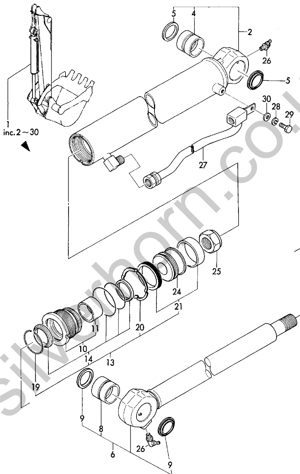
Fig. 44 バケットシリンダ BUCKET CYLINDER
