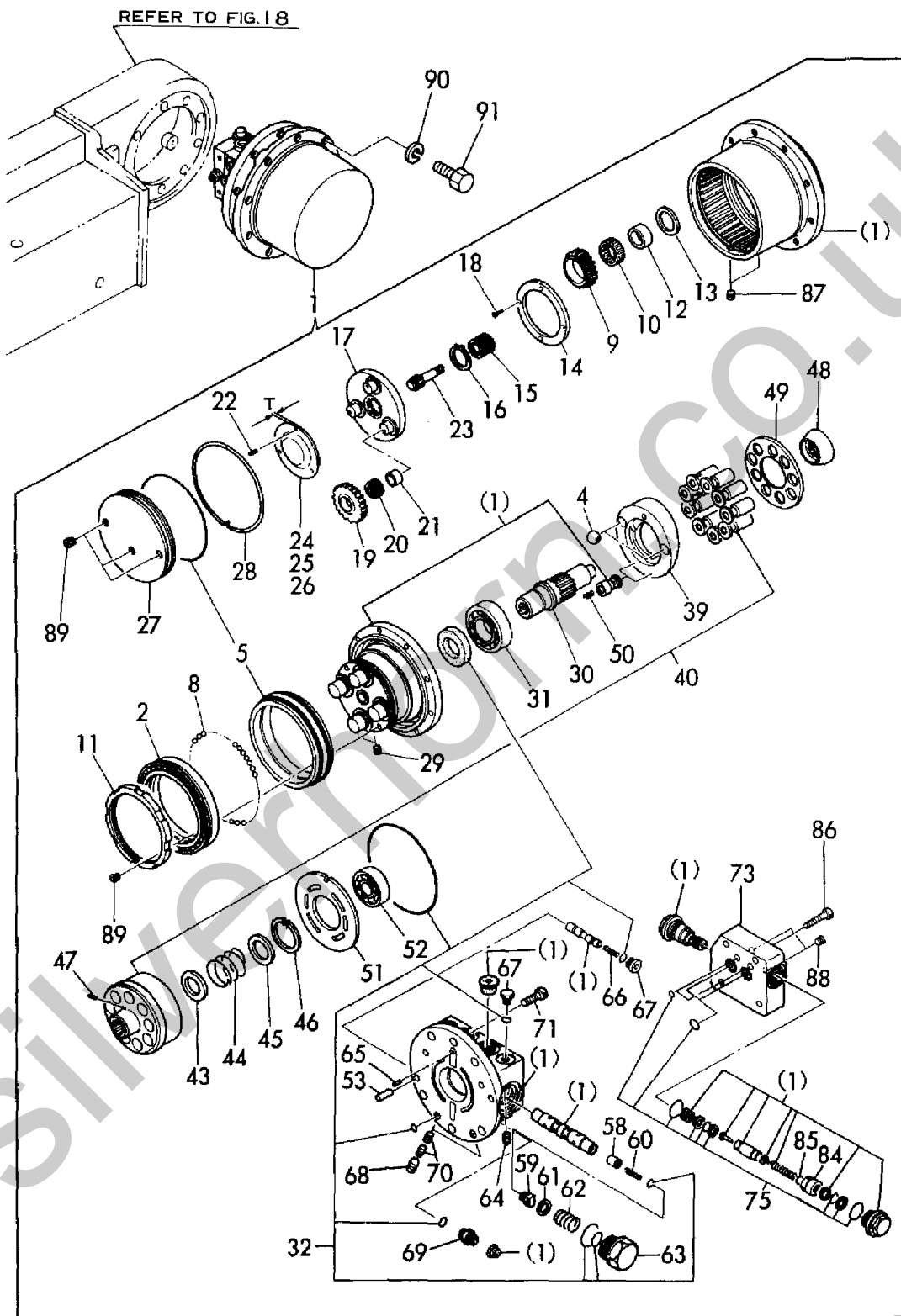
Fig. 48 ソウコウモータ TRAVEL MOTOR
