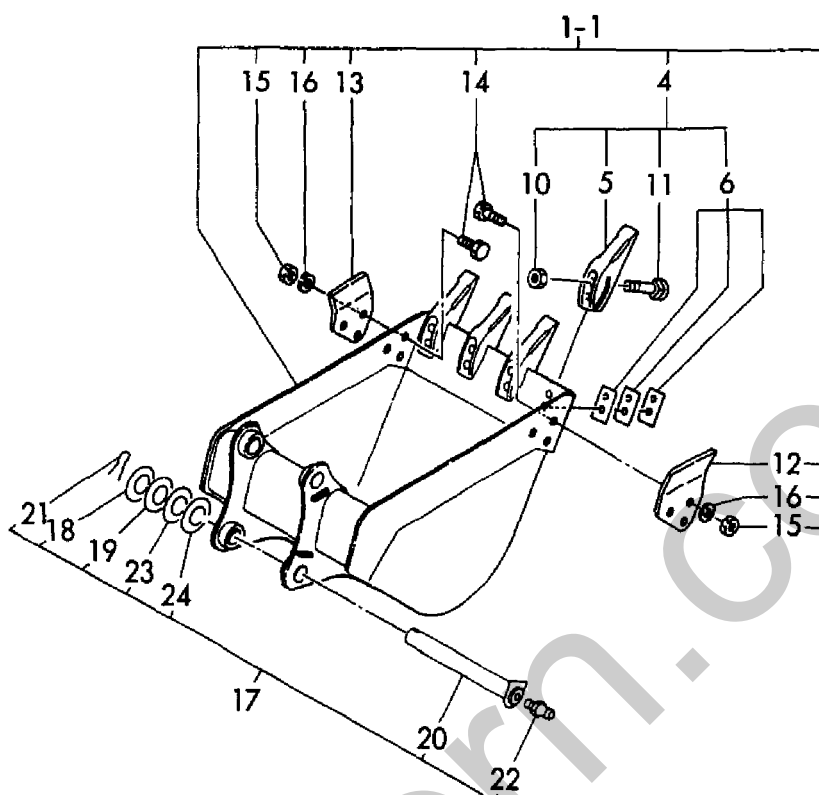
Fig. 87 バケット (600, 650) (アタッチメント) BUCKET (600, 650) (ATTACHMENT)
