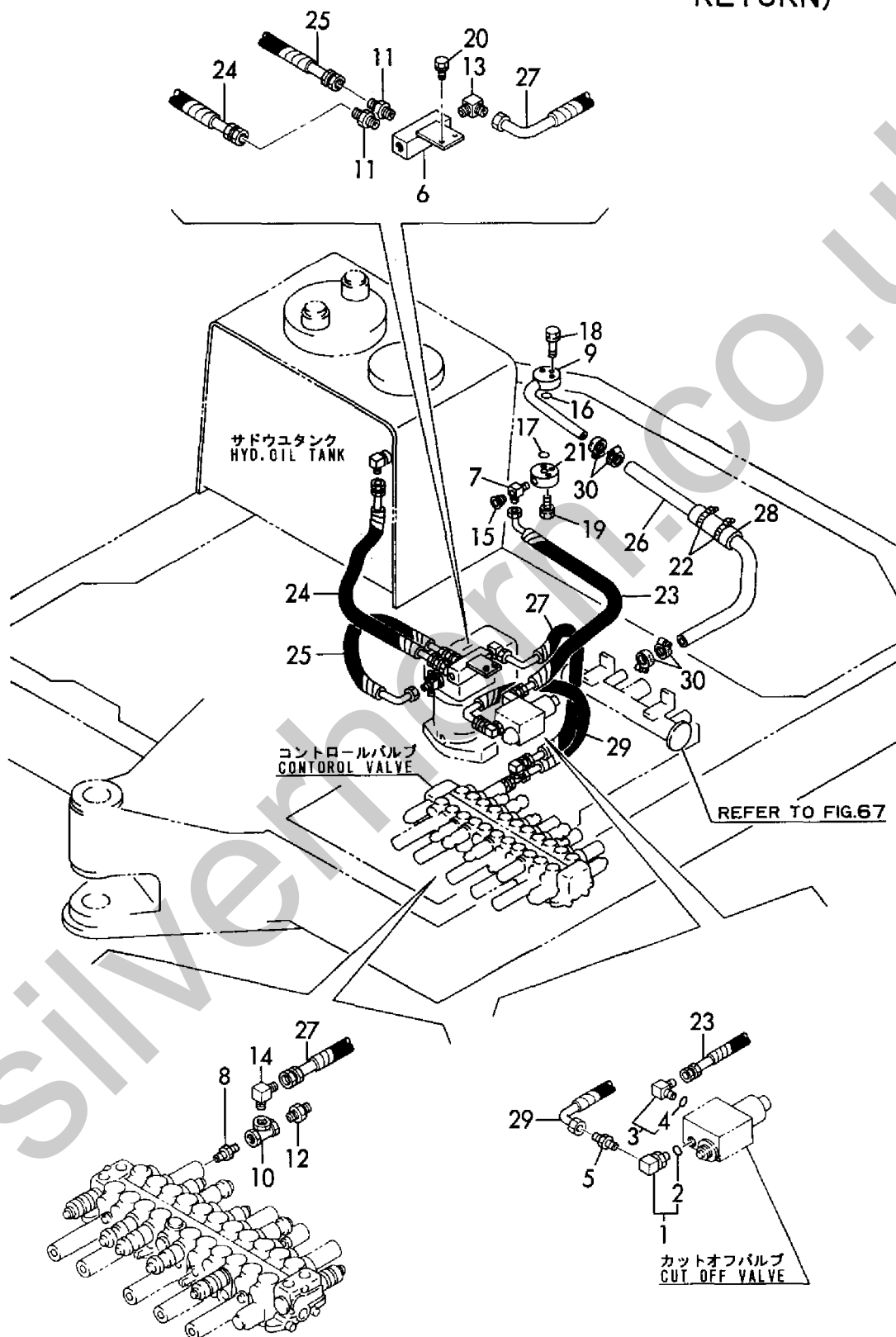
Fig. 76 コントロールパイカン(ポンプ-カットオフバルブ-リターン) CONTROL PIPING (PUMP-CUT OFF VALVE-RETURN)
