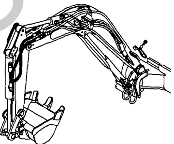
Fig. 40 油圧配管 (ブーム) HYD. OIL PIPING (BOOM)
