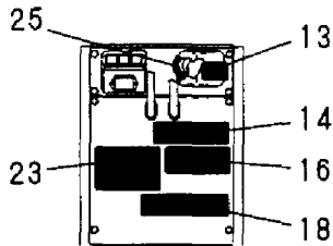
Bから見る VIEWED FROM B
