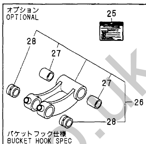
Fig. 44 アーム&バケットリンク ARM & BUCKET LINK
