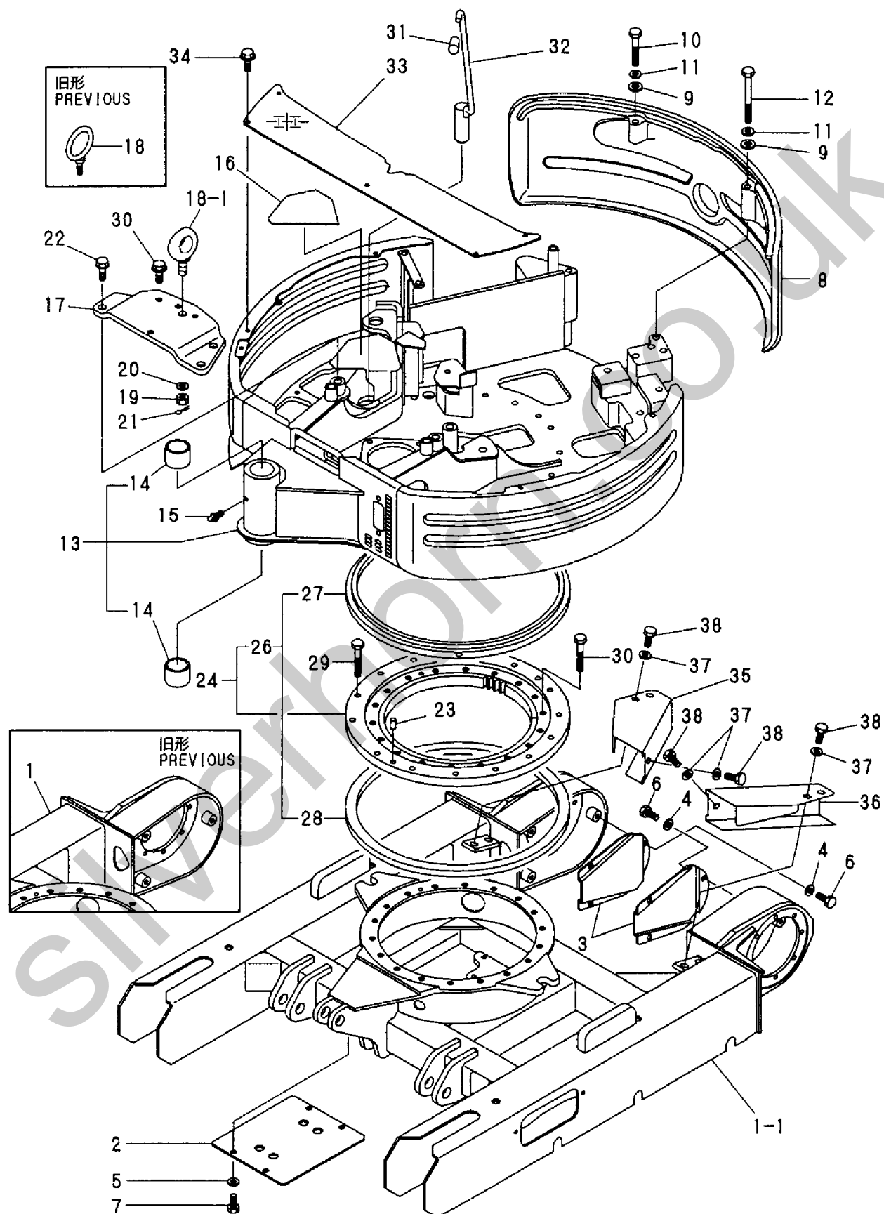
Fig. 20 フレーム&旋回ベアリング FRAME & TURNING BEARING
