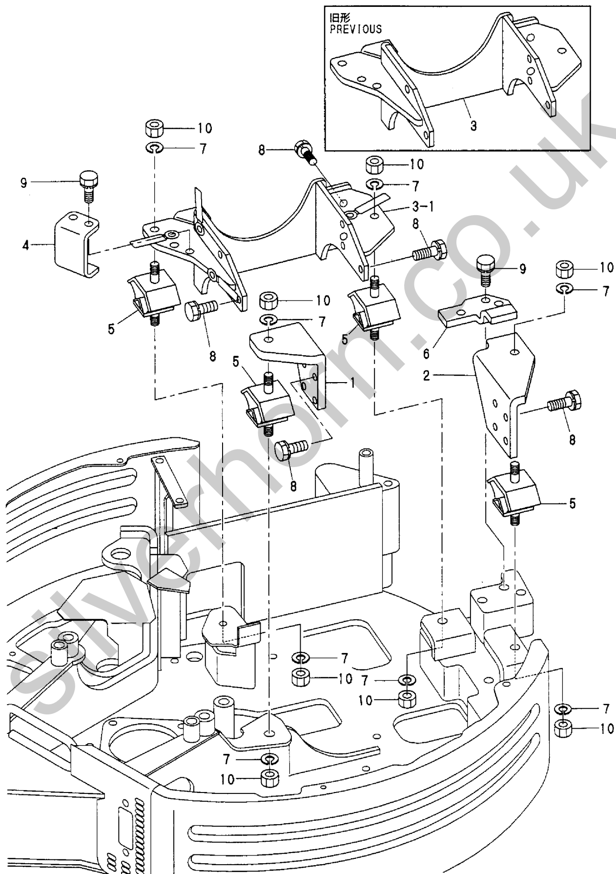
Fig. 7 エンジンマウント ENGINE MOUNT
