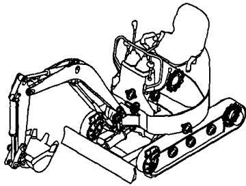
Fig. 14 操縦装置 (リンク台&レバーストップ) CONTROL EQUIPMENT (LINK STAND & LEVER STOPPER)
