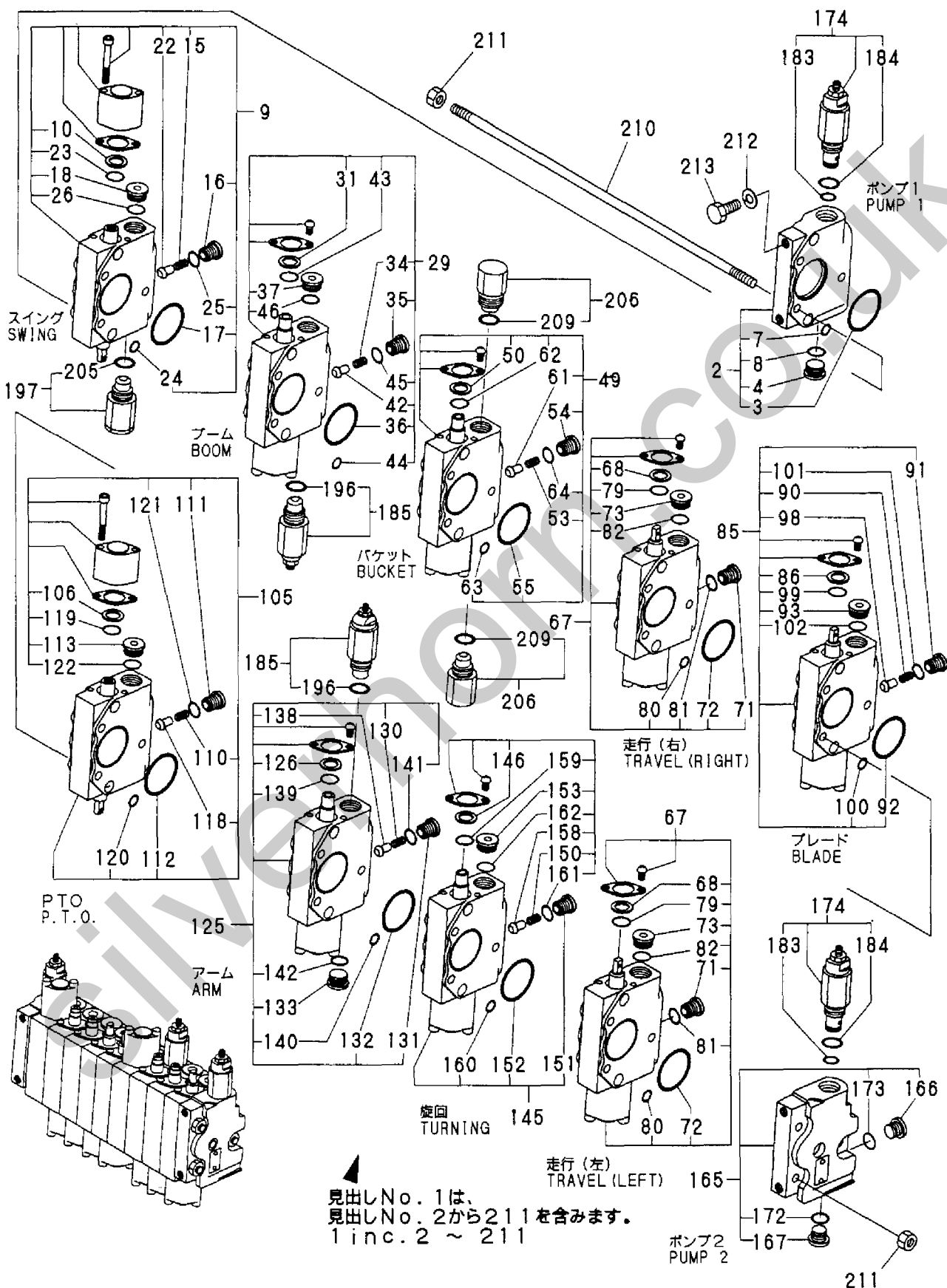
Fig. 31 コントロールバルブ CONTROL VALVE
