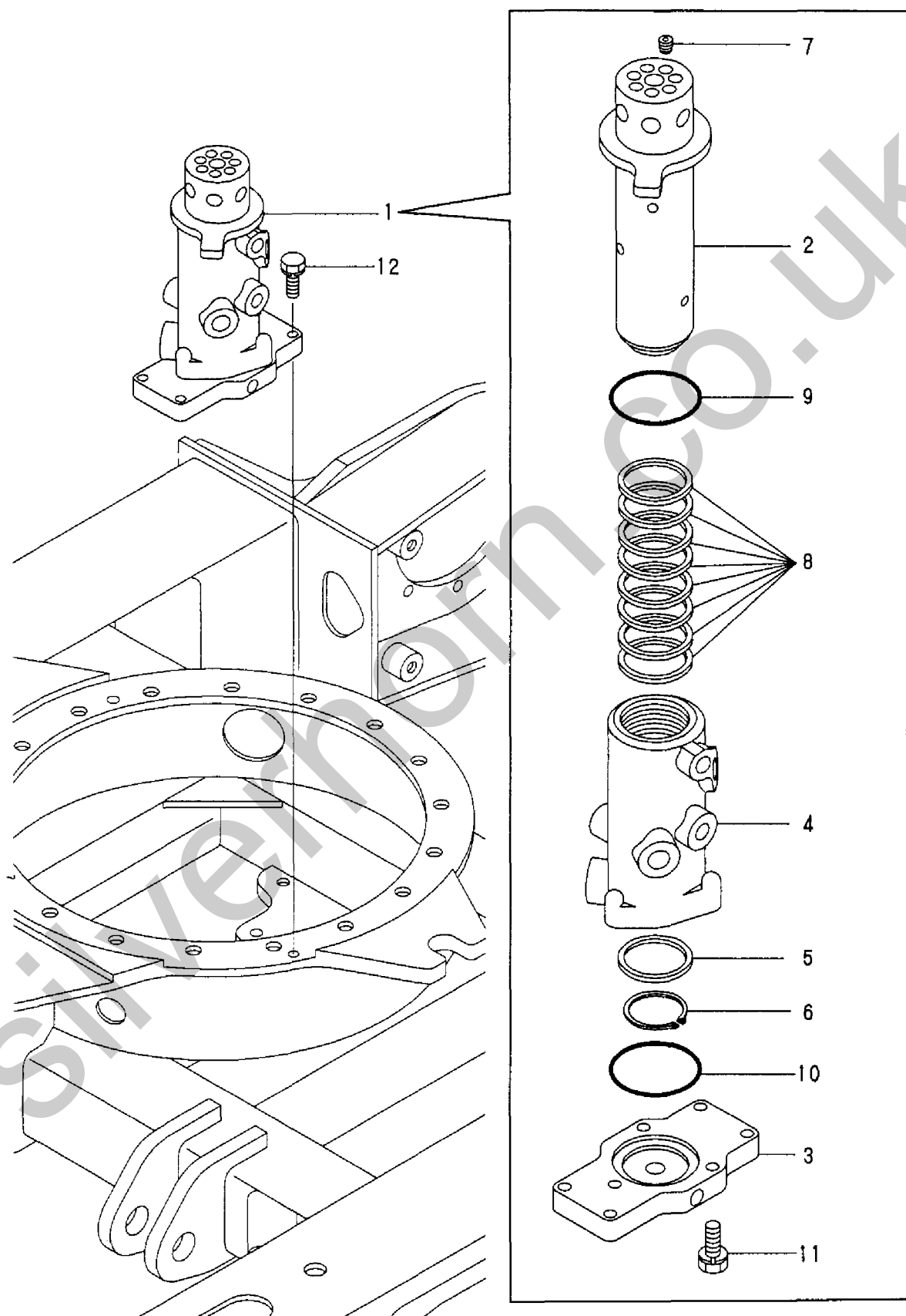
Fig. 30 スイベルジョイント SWIVEL JOINT
