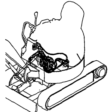
Fig. 36 油圧配管 (バルブ ~スイベル〜スイング) HYD. OIL PIPING (VALVE~SWIVEL~SWING)
