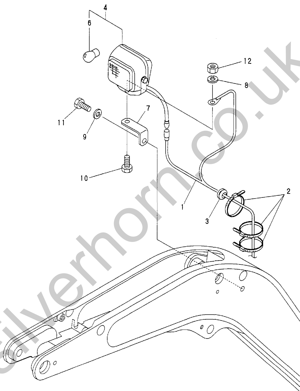
Fig. 12 ワークランプ WORK LAMP
