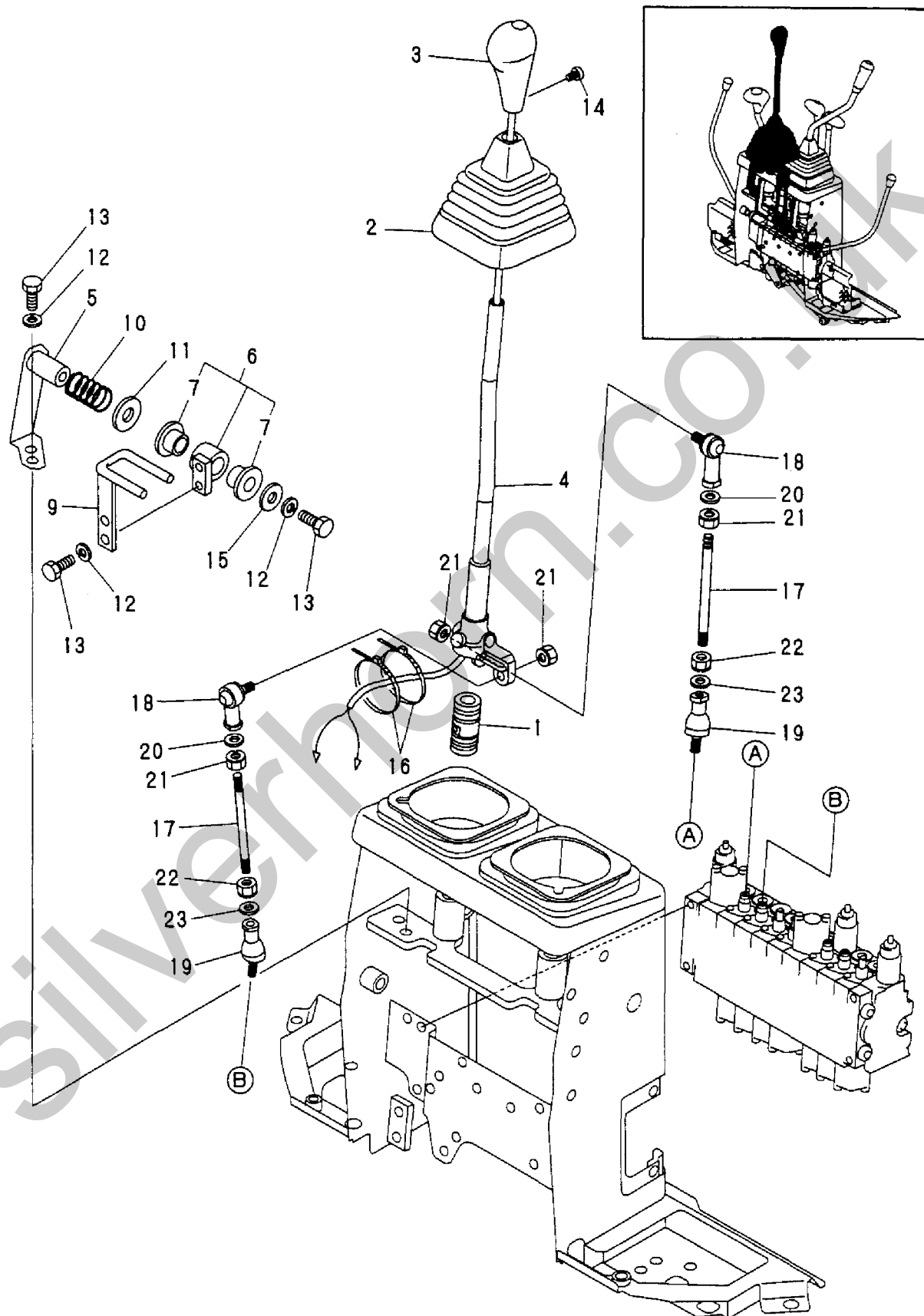
Fig. 15 操縦装置 (ブーム & バケット) CONTROL EQUIPMENT (BOOM & BUCKET)
