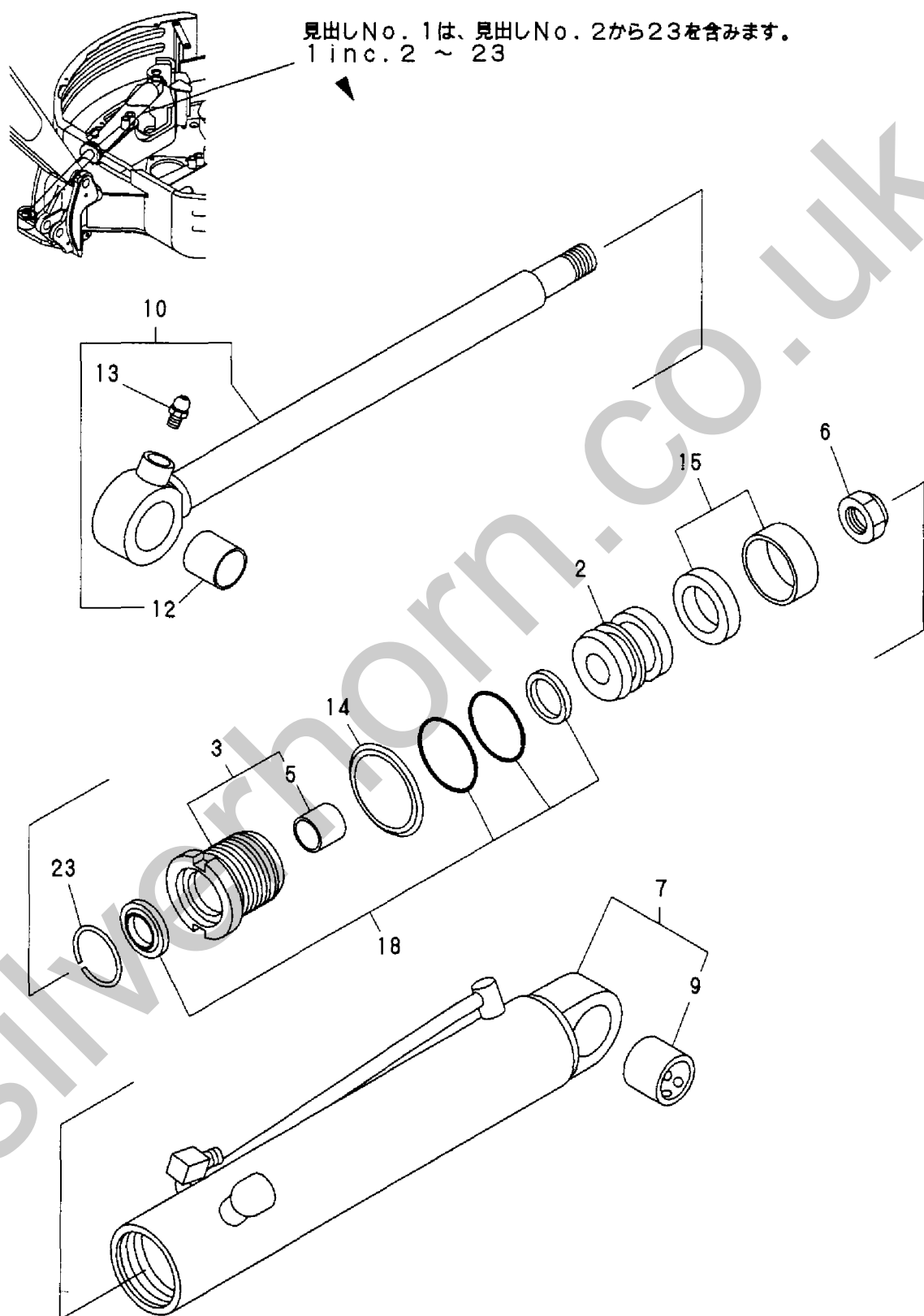
Fig. 26 スイングシリンダ SWING CYLINDER
