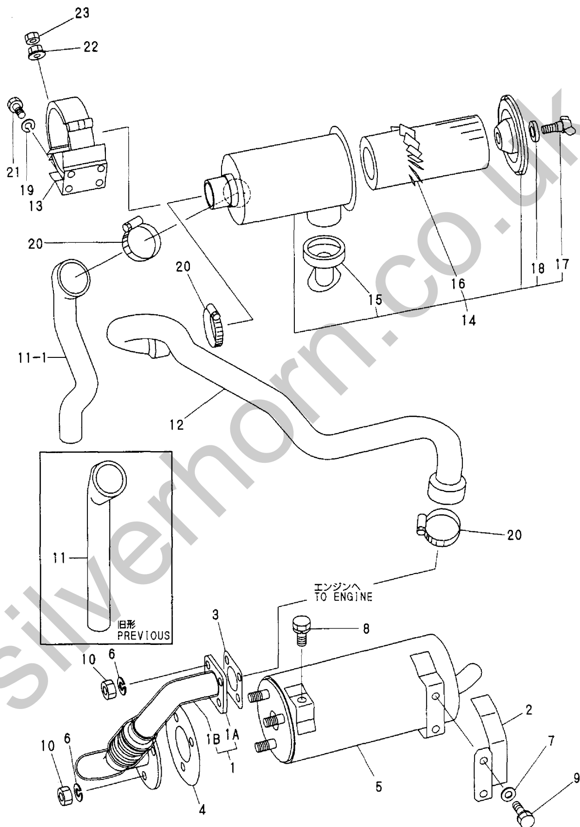
Fig. 5 サイレンサ&エアクリーナ SILENCER & AIR CLEANER
