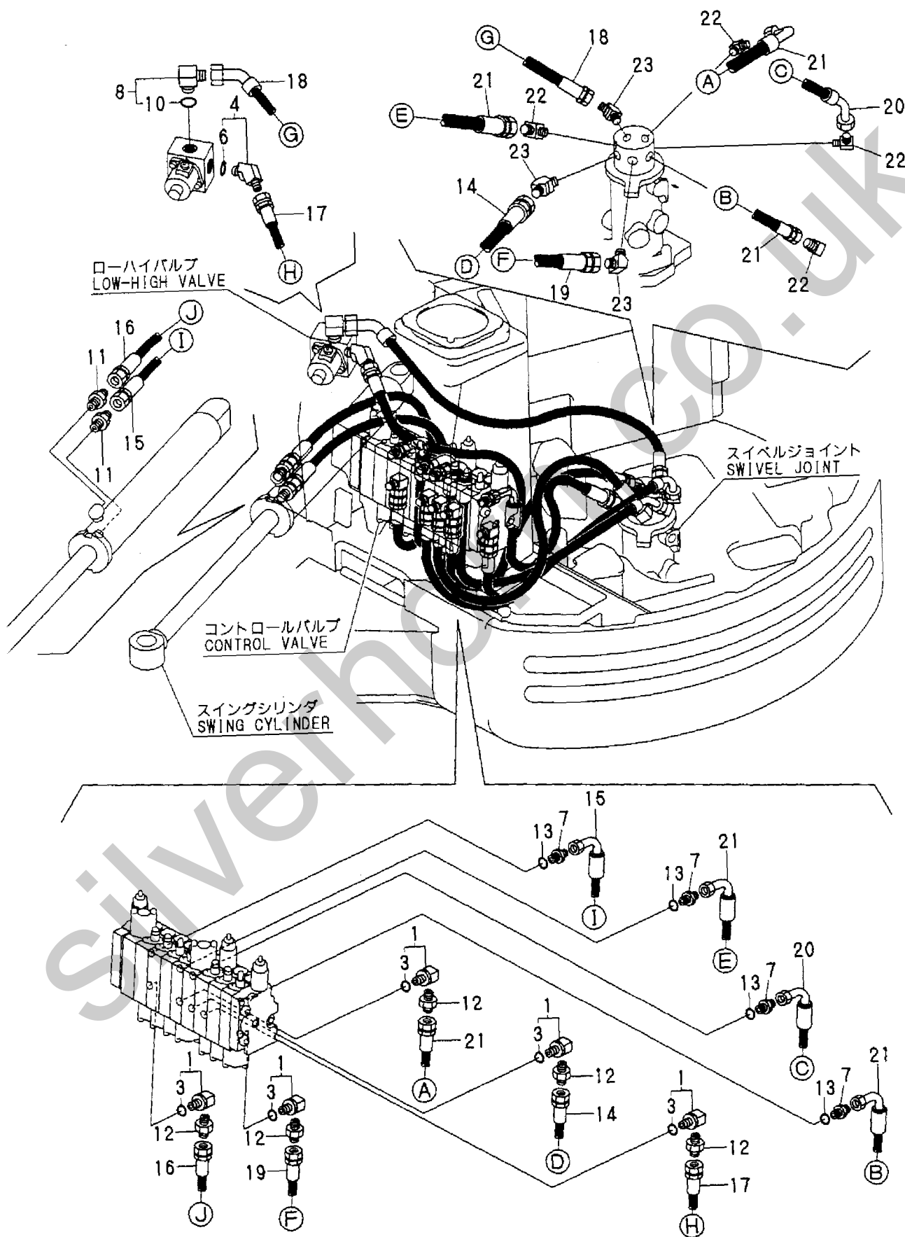
Fig. 36 油圧配管 (バルブ~スイベル~スイング) HYD. OIL PIPING (VALVE~SWIVEL~SWING)
