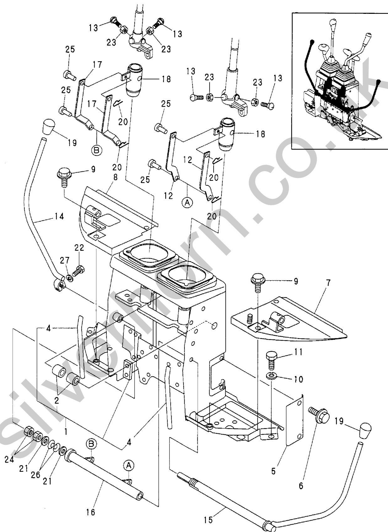
Fig. 14 操縦装置 (リンク台&レバーストップパ) CONTROL EQUIPMENT (LINK STAND & LEVER STOPPER)
