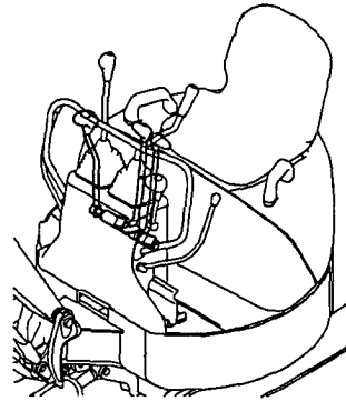
Fig. 18 操縦装置 (スイング) CONTROL EQUIPMENT (SWING)
