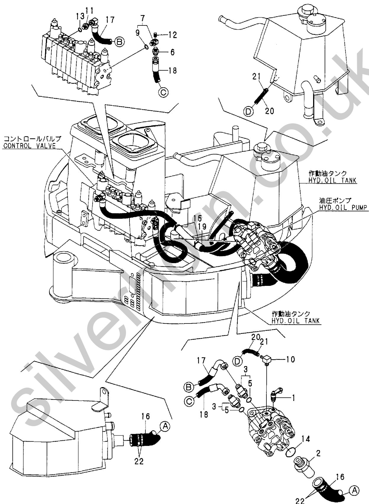
Fig. 34 油圧配管 (タンク~ポンプ~バルブ) HYD. OIL PIPING (TANK~PUMP~VALVE)
