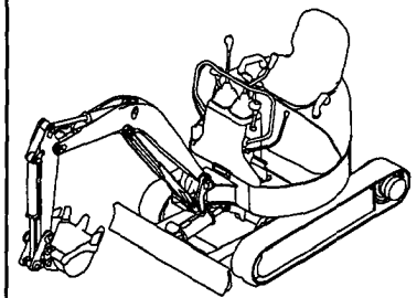
Fig. 24 アームシリンダ ARM CYLINDER
