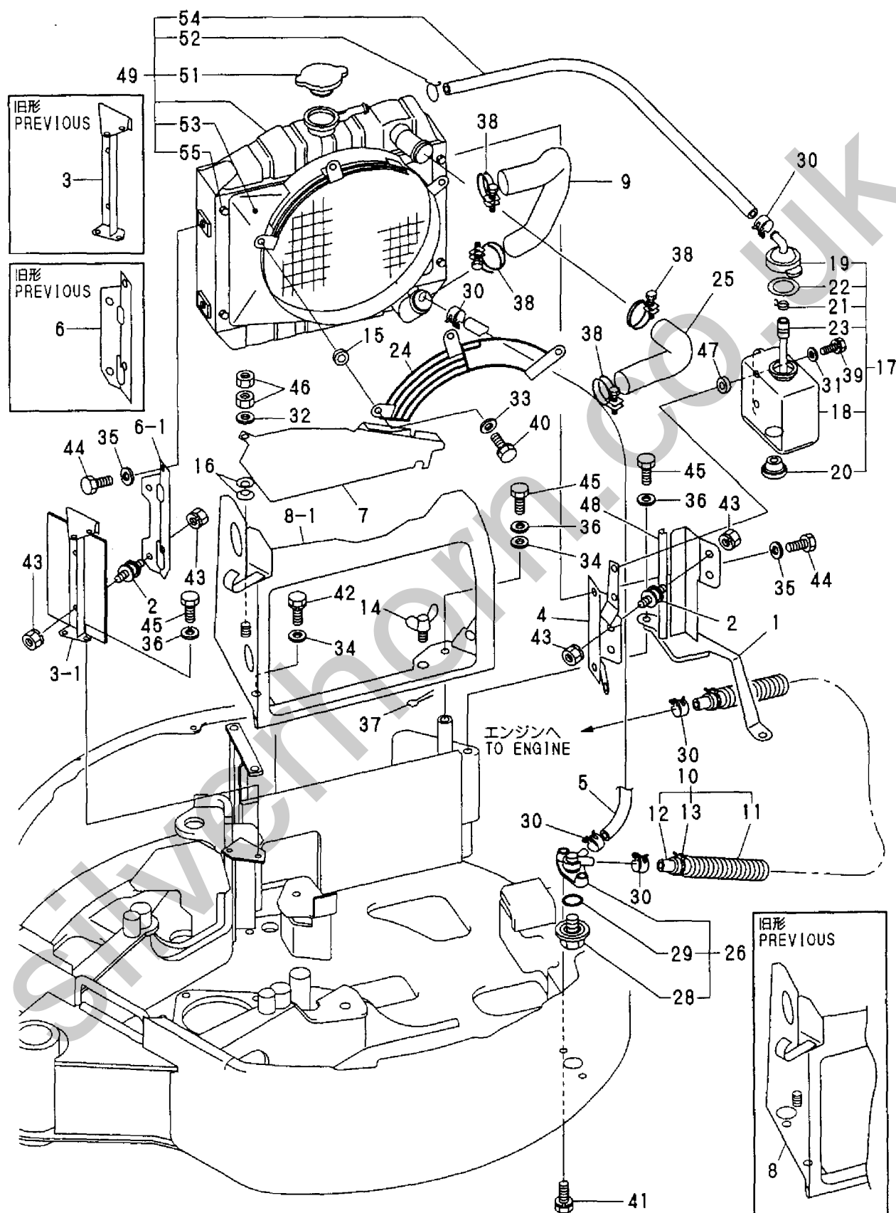
Fig. 8 ラジエータ&マウント RADIATOR & MOUNT
