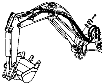
Fig. 41 油圧配管 (PTOアームエンド) HYD. OIL PIPING (P. T. O. ARM END)
