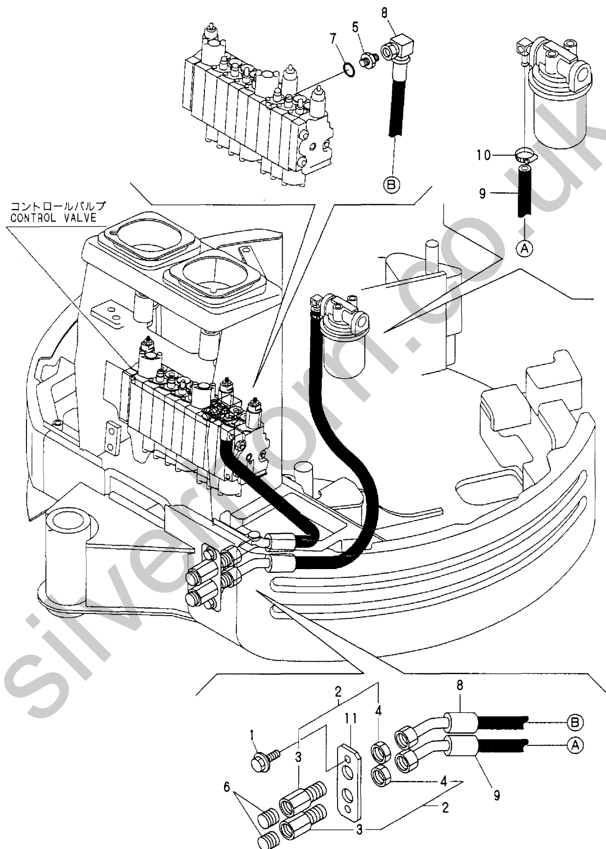
Fig. 38 油圧配管 (PTOバルブ~フレームエンド) HYD. OIL PIPING (P. T. O. VALVE~FRAME END)
