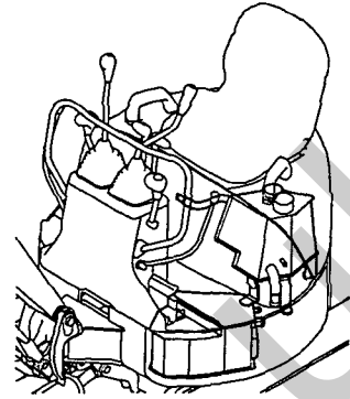
Fig. 34 油圧配管 (タンク〜ポンプ ~バルブ) HYD. OIL PIPING (TANK~PUMP~VALVE)
