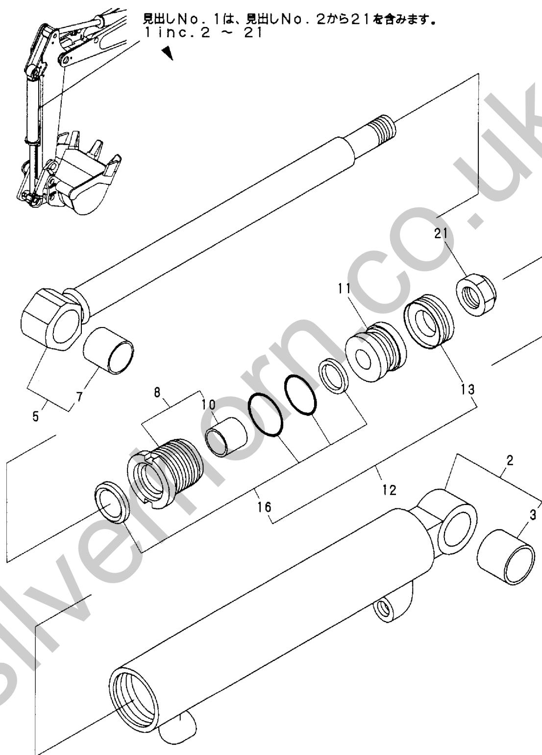
Fig. 25 バケットシリンダ BUCKET CYLINDER
