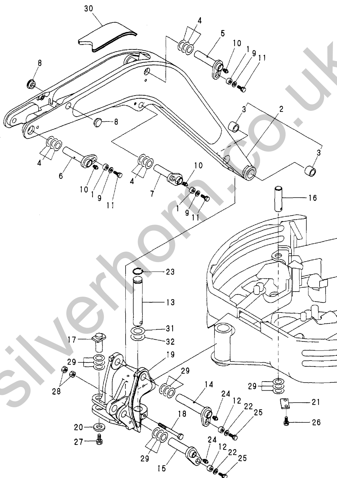
Fig. 43 ブーム&ブームブラケット BOOM & BOOM BRACKET
