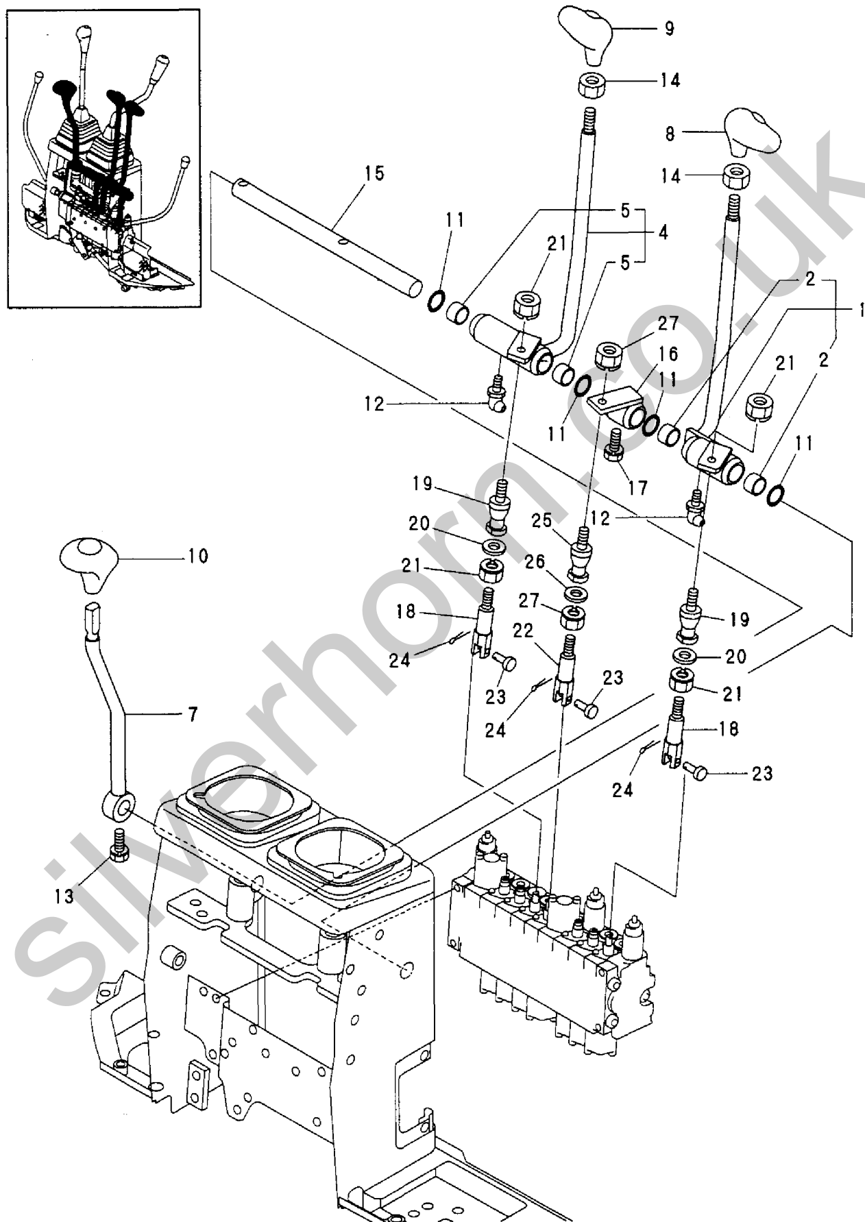
Fig. 17 操縦装置 (走行&ブレード) CONTROL EQUIPMENT (DRIVE & BLADE)
