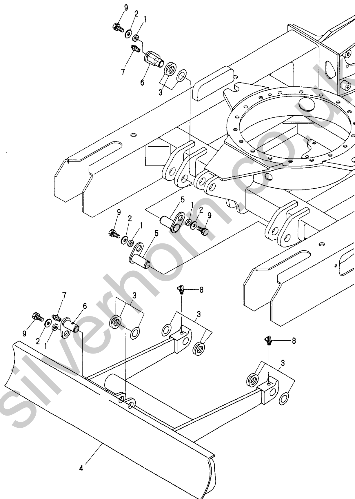
Fig. 47 ブレード BLADE
