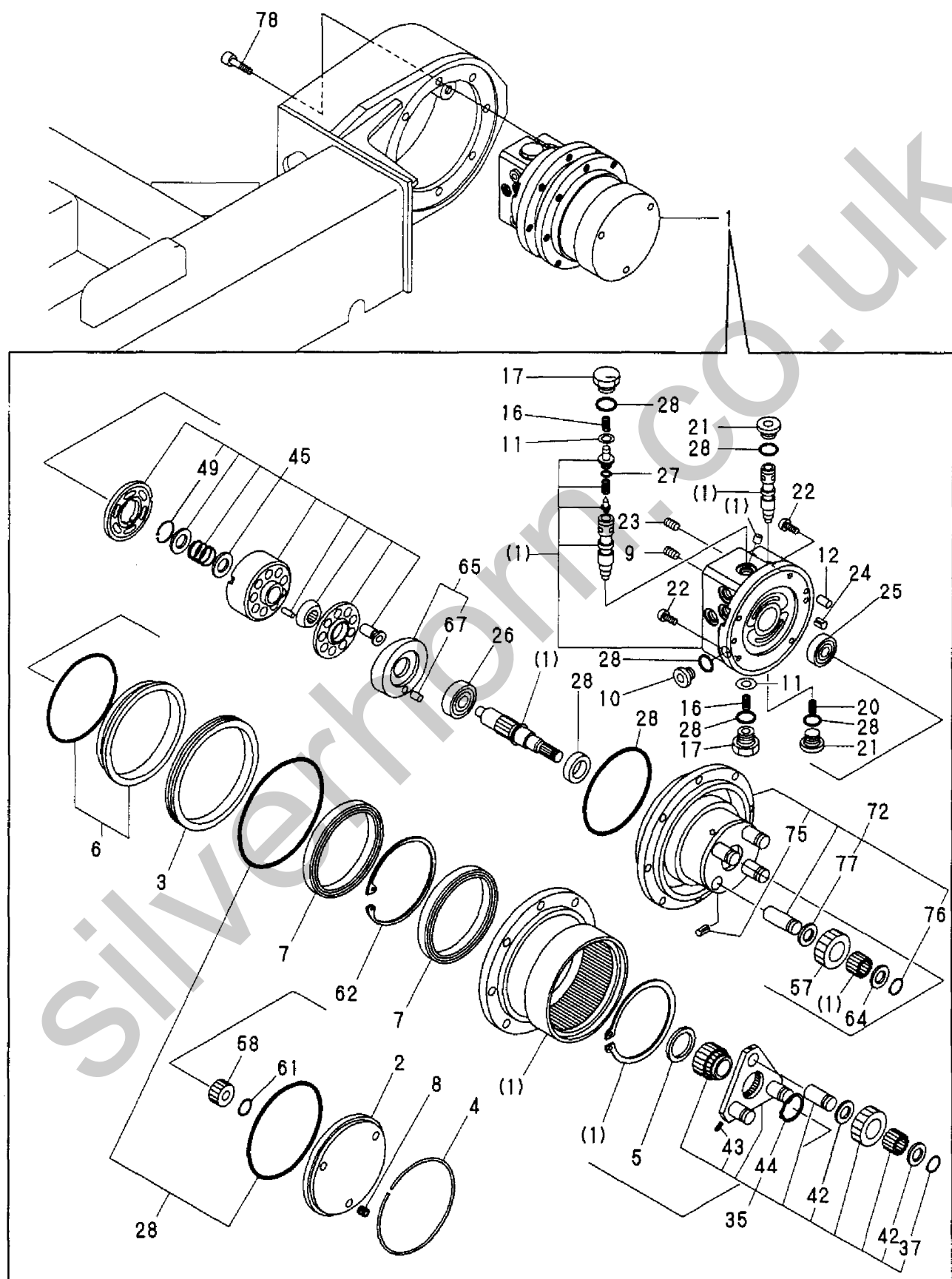
Fig. 28 走行モータ TRAVEL MOTOR
