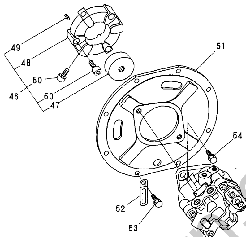
Fig. 22 ポンプ&軸継手 HYD. OIL PUMP & JOINT
