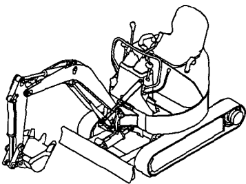
Fig. 27 ブレードシリンダ BLADE CYLINDER
