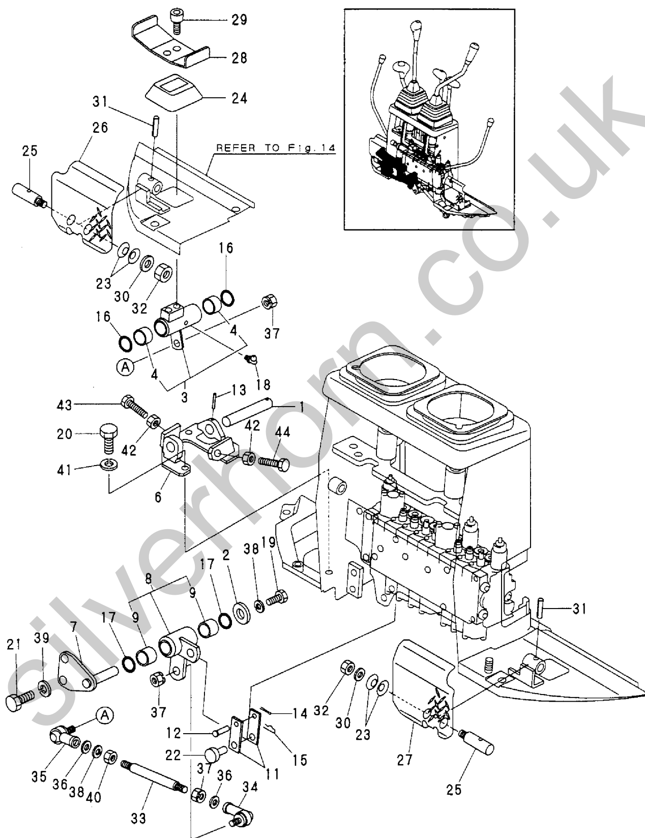
Fig. 18 操縦装置 (スイング) CONTROL EQUIPMENT (SWING)
