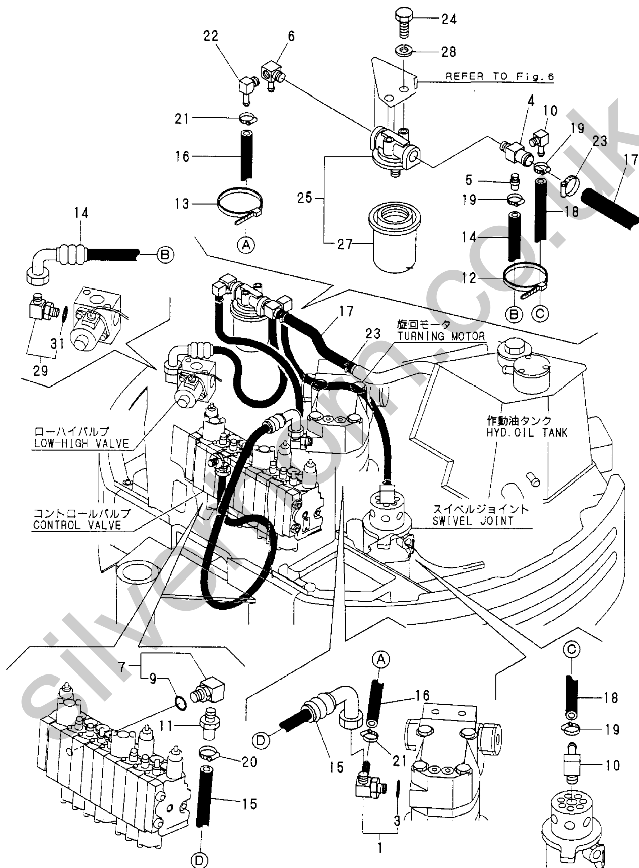
Fig. 37 油圧配管 (リターン) HYD. OIL PIPING (RETURN)
