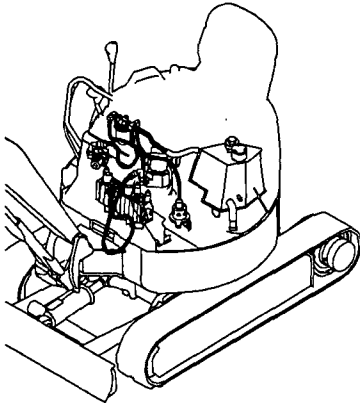
Fig. 38 油圧配管 (PTOバルブ ~フレームエンド) HYD. OIL PIPING (P. T. O. VALVE~FRAME END)
