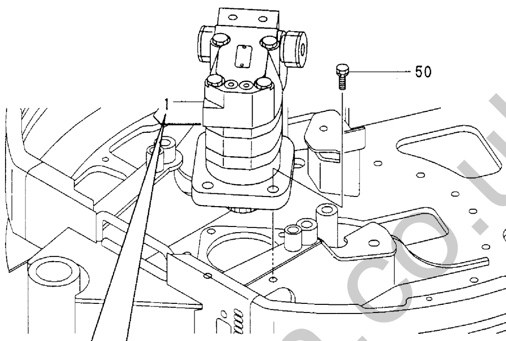
Fig. 29 旋回モータ TURNING MOTOR
