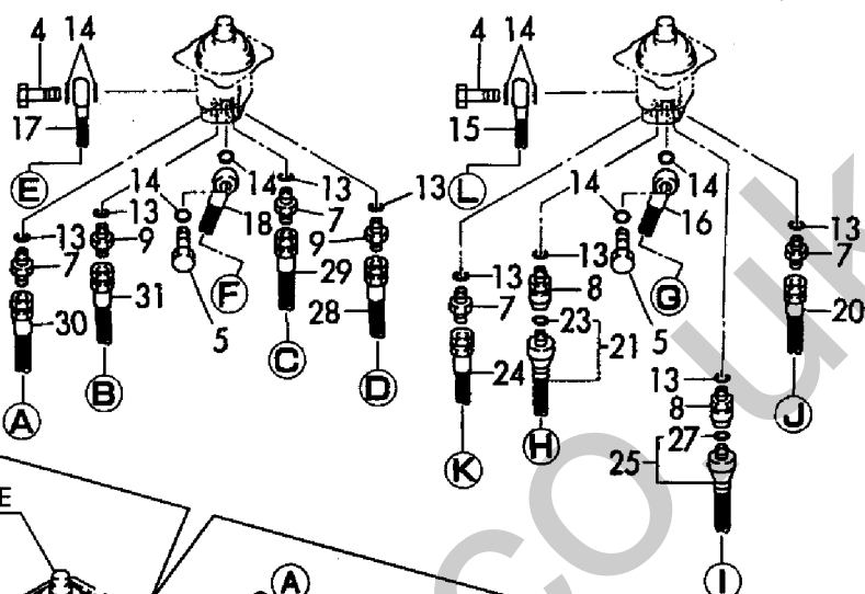
Fig. 53 コントロール配管 (ダイレクト, パターンB) CONTROL PIPING (DIRECT, PATTERN B)
