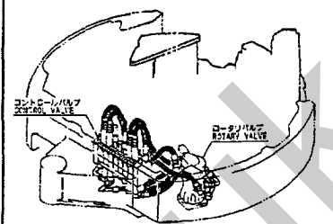
Fig. 57 コントロール配管 (ロータリバルブ~コントロールバルブ) CONTROL PIPING (ROTARY VALVE~CONTROL VALVE)
