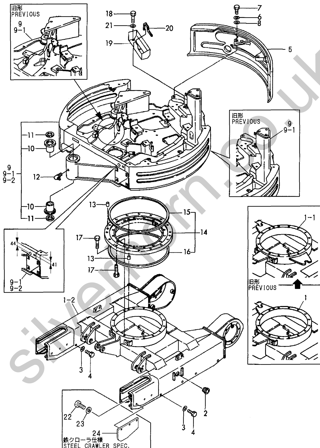
Fig. 21 フレーム&旋回ベアリング FRAME & TURNING BEARING
