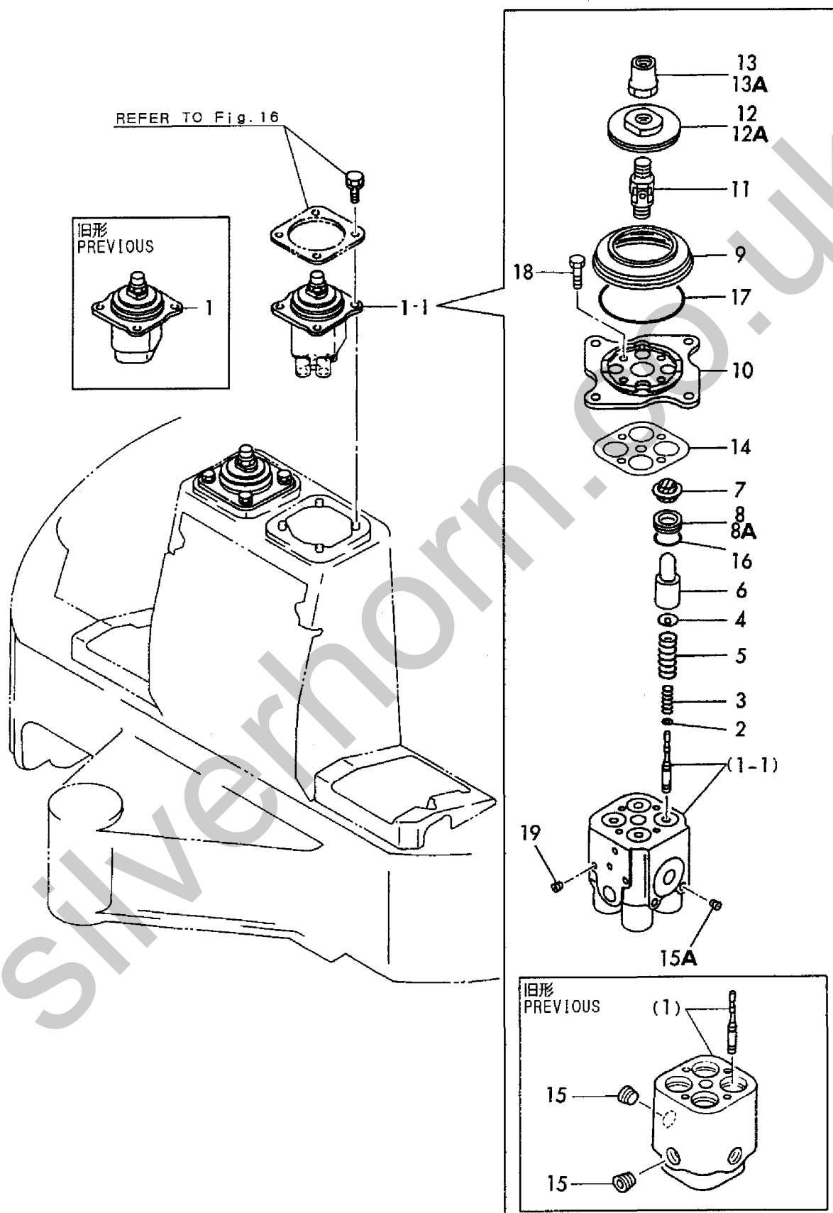
リモコンバルブ REMOTE CONTROL VALVE Fig. 38
