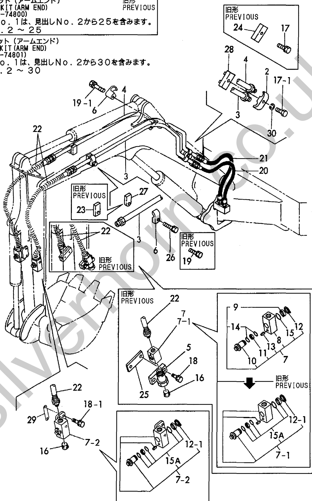
Fig. 51 油圧配管 (PTOアームエンド) HYD. OIL PIPING (P. T. O. ARM END)
