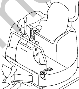
Fig. 20 操縦装置 (PTOコントロール) CONTROL EQUIPMENT (P. T. O. CONTROL)
