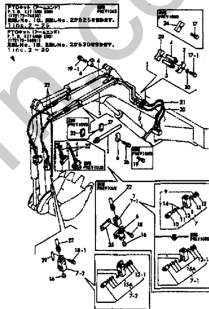
Fig. 51 油圧配管 (PTOアームエンド) HYD. OIL PIPING (P.T.O. ARM END)
