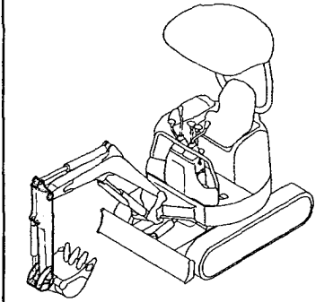
Fig. 60 アーム&バケットリンク ARM & BUCKET LINK
