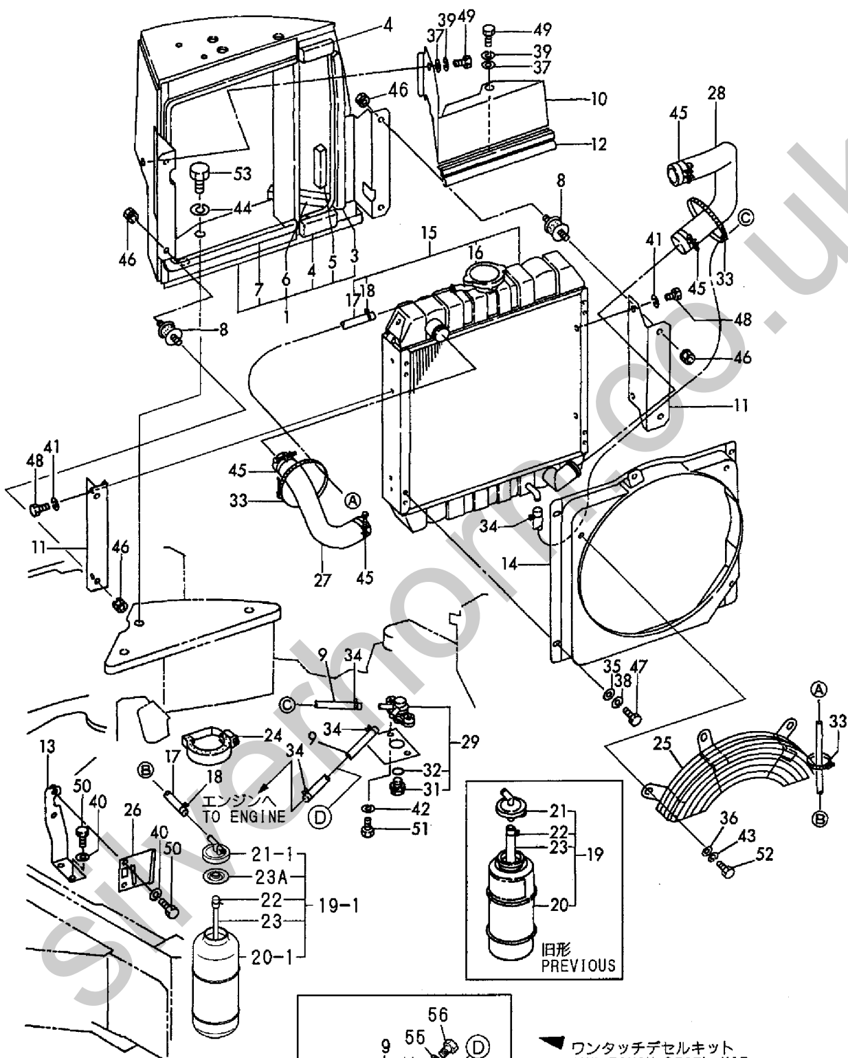
Fig. 7 ラジエータ&マウント RADIATOR & MOUNT
