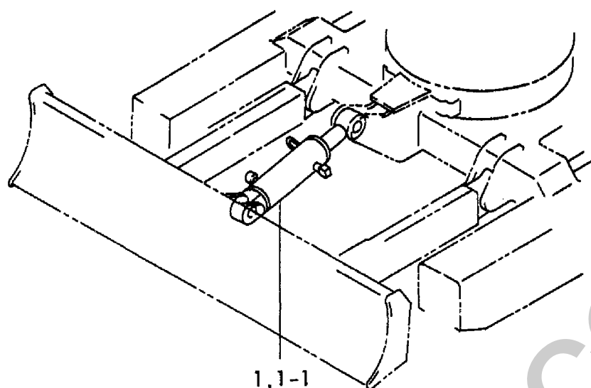
Fig. 32 ブレードシリンダ BLADE CYLINDER
