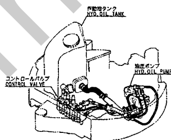
Fig. 43 油圧配管 (タンク〜ポンプ〜バルブ) HYD. OIL PIPING (TANK~PUMP~VALVE) ~M/#03463, 03466
