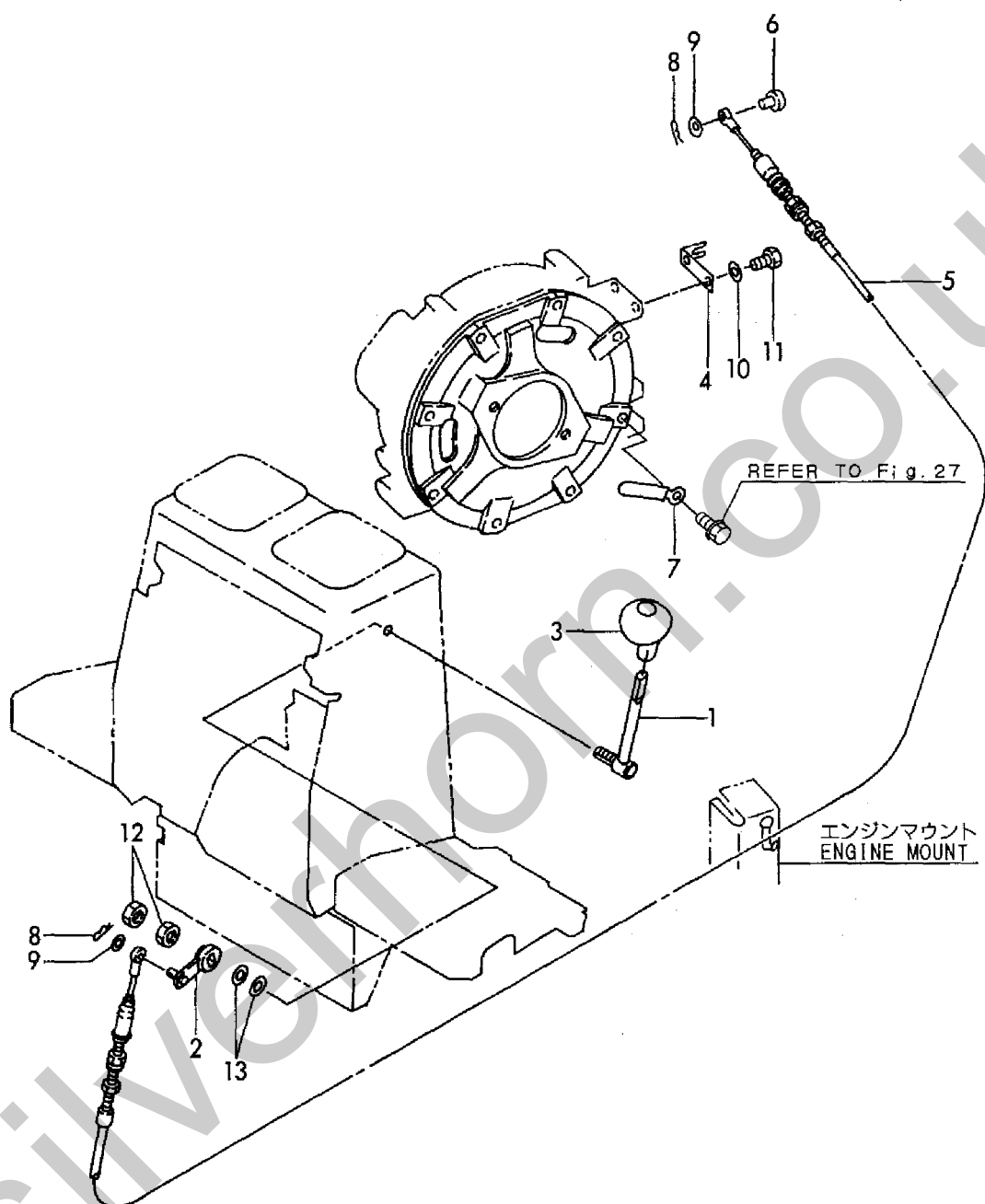
Fig. 4 アクセル ACCELERATOR
