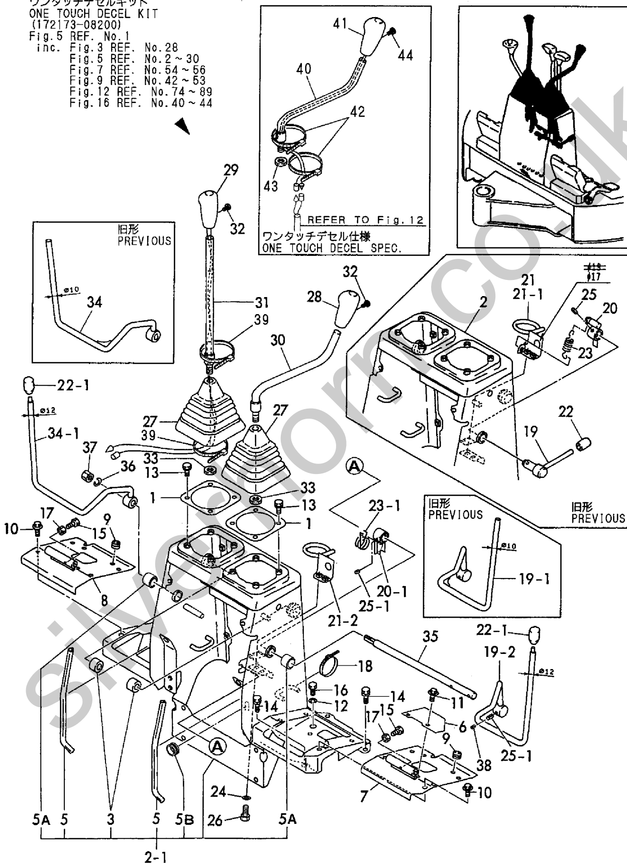
Fig. 16 操縦装置 (レバー&スタンド) CONTROL EQUIPMENT (LEVER & STAND)
