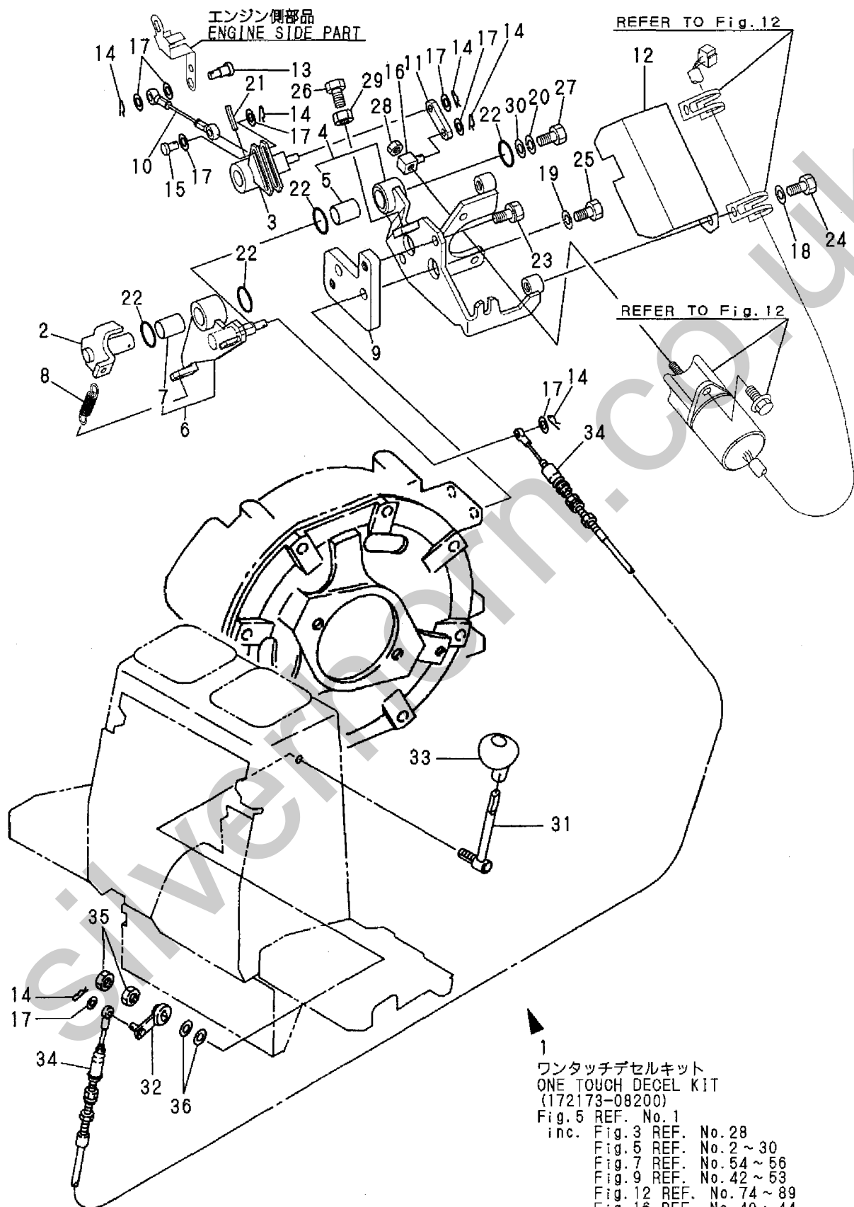
Fig. 5 アクセル (ワンタッチデセル) ACCELERATOR (ONE TOUCH DECEL)
