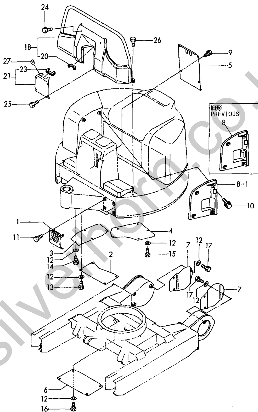
Fig. 22 フレームカバー FRAME COVER
