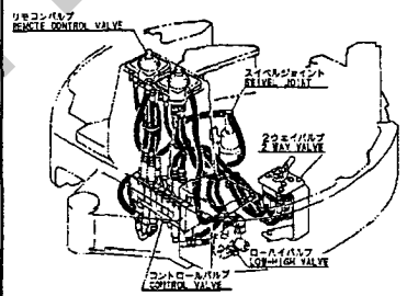
Fig. 55 コントロール配管 (2ウェイマルチチェンジ) CONTROL PIPING (2WAY MULTI CHANGE)
