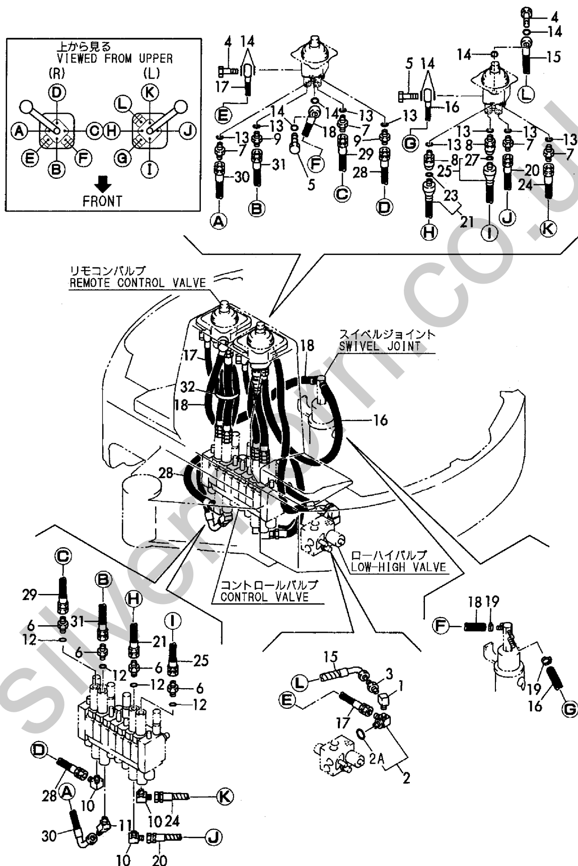
Fig. 52 コントロール配管 (ダイレクト) CONTROL PIPING (DIRECT)
