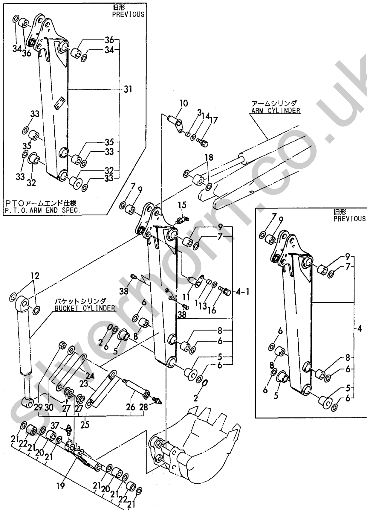
Fig. 60 アーム&バケットリンク ARM & BUCKET LINK
