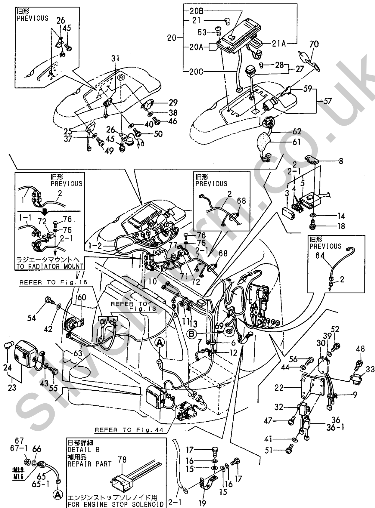
Fig. 11 電装品 ELECTRIC PART
