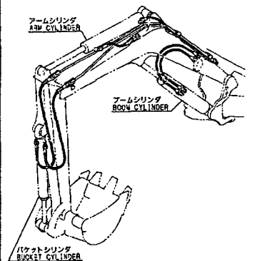
Fig. 51 油圧配管 (PTOアームエンド) HYD. OIL PIPING (P. T. O. ARM END)
