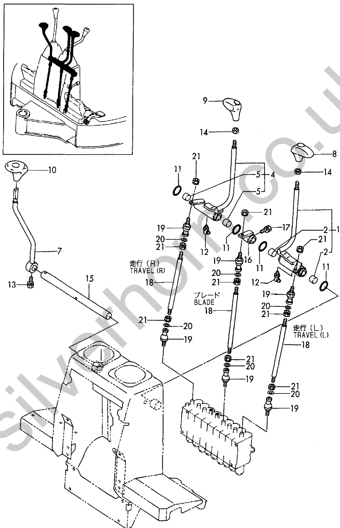
Fig. 17 操縦装置 (走行 & ブレード) CONTROL EQUIPMENT (TRAVEL & BLADE)
