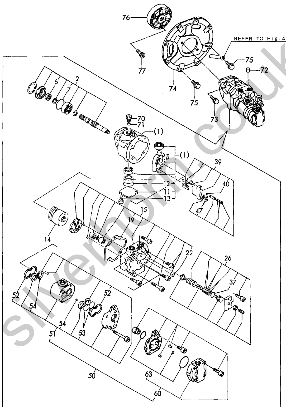
Fig. 27 油圧ポンプ&軸継手 HYD. OIL PUMP & JOINT
