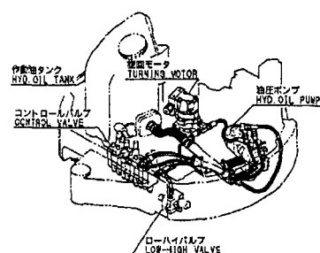
Fig. 44 油圧配管 (タンク〜ポンプ〜バルブ) HYD. OIL PIPING (TANK~PUMP~VALVE) M/#03464~
