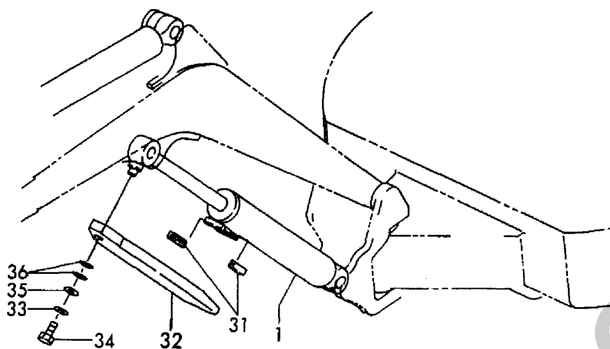
Fig. 28 ブームシリンダ BOOM CYLINDER
