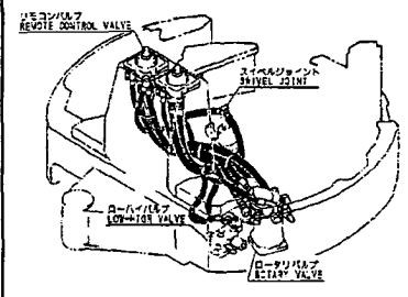
Fig. 56 コントロール配管 (リモコンバルブ ~ロータリバルブ) CONTROL PIPING (REMOCON VALVE~ROTARY VALVE)
