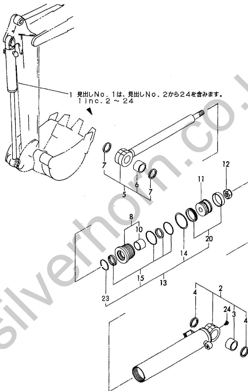
Fig. 30 バケットシリンダ BUCKET CYLINDER
