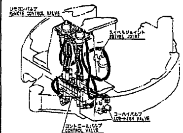
Fig. 53 コントロール配管 (ダイレクト パターンB) CONTROL PIPING (DIRECT PATTERN B)
