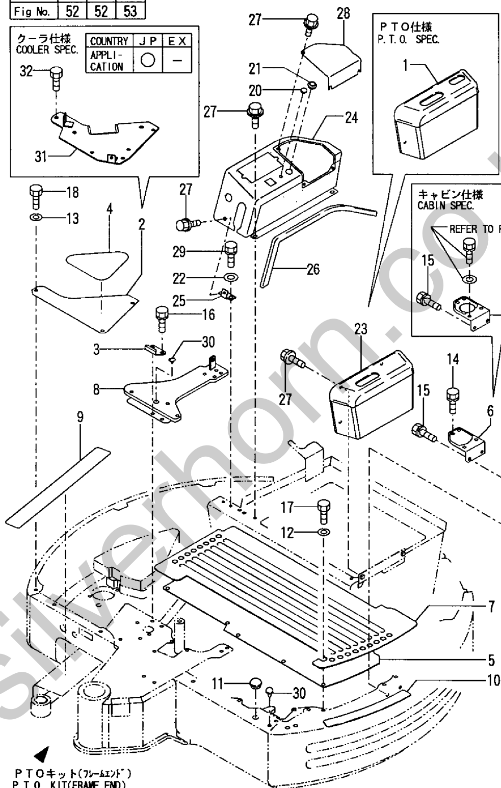
Fig. 52 ステップ & インパネ(JP, EX) STEP & INSTRUMENT PANEL(JP, EX)
