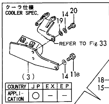
Fig. 18 エンジンマウント ENGINE MOUNT
