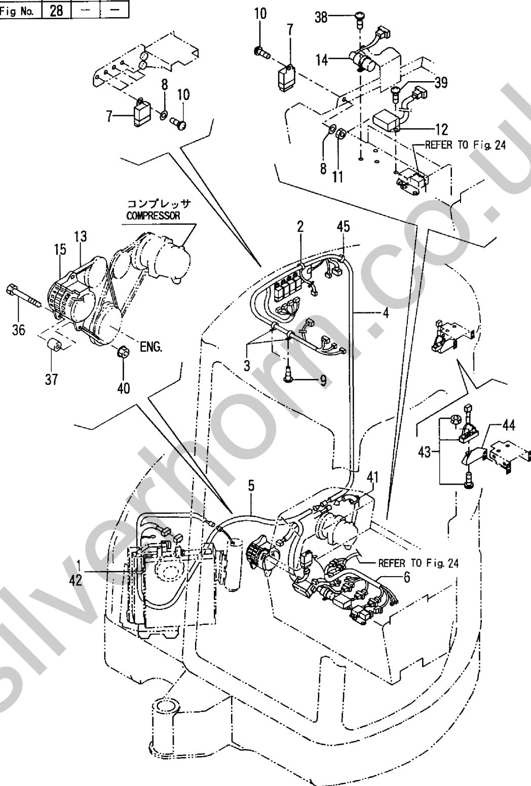
Fig. 28 電装品(クーラ仕様) ELECTRIC PART(COOLER SPEC.)
