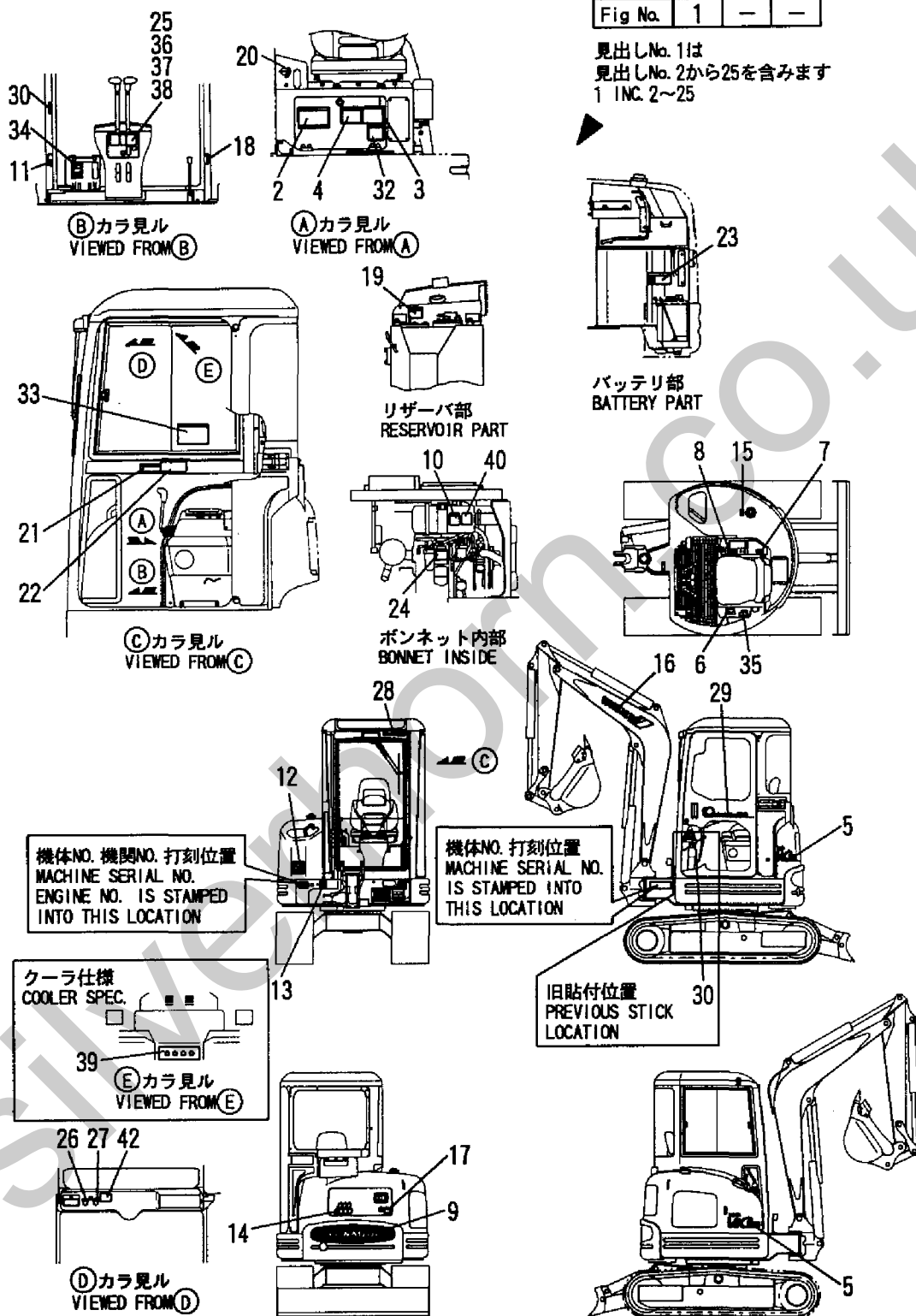
Fig. 1 銘板(キャビン:JP)(旧形) LABEL(CABIN:JP)(PREVIOUS)
