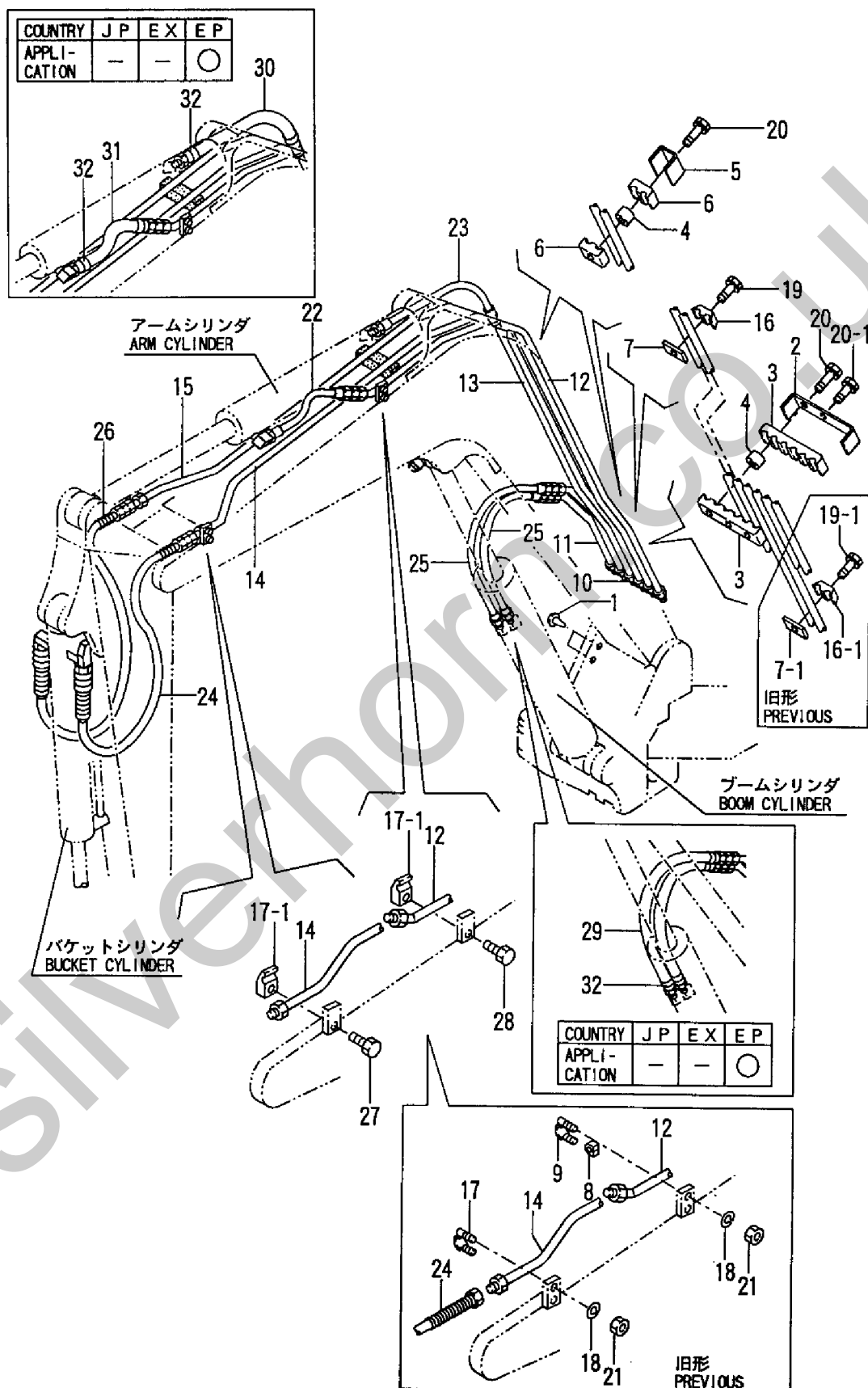
Fig. 95 油圧配管(ブーム) HYD. OIL PIPING (BOOM)
