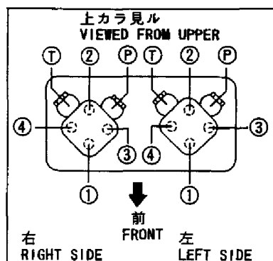
Fig. 105 コントロール配管 (リモコンバルブ ~ 2ウェイチェンジバルブ ~ コントロールバルブ) CONTROL PIPING (REMOTE CONTROL VALVE ~ 2-WAY CHANGE VALVE ~ CONTROL VALVE)
