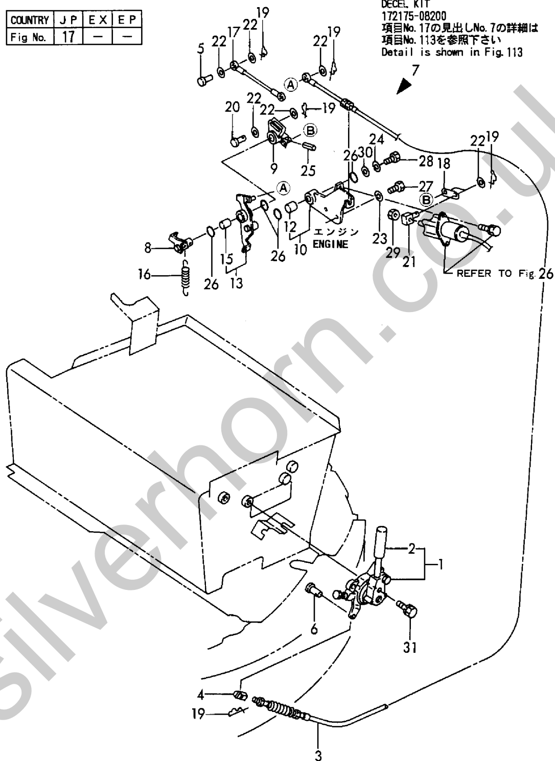
Fig. 17 アクセル(ワンタッチデセル仕様) ACCELERATOR(ONE TOUCH DECEL SPEC.)
