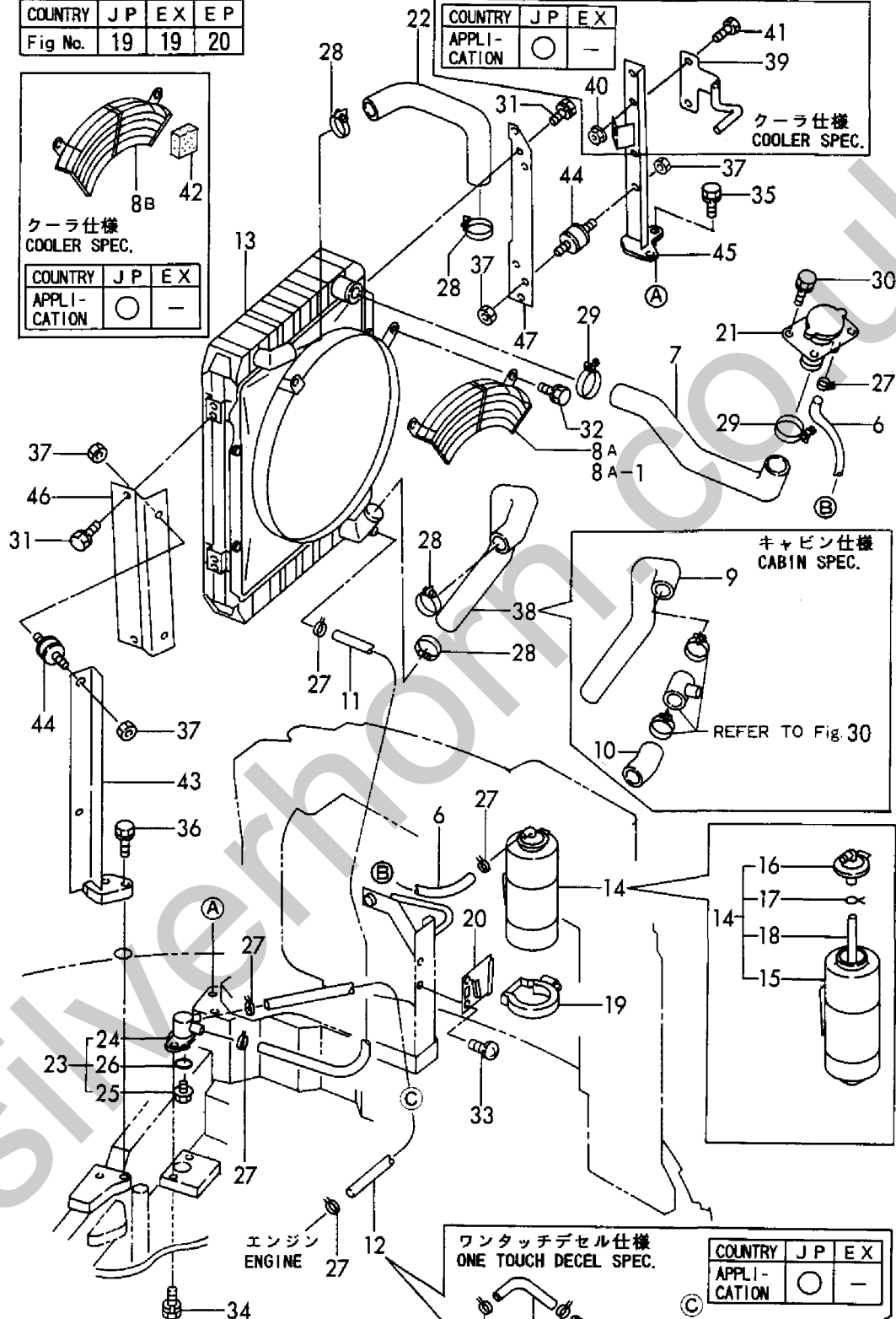
Fig. 19 ラジエータ & マウント(JP, EX) RADIATOR & MOUNT(JP, EX)
