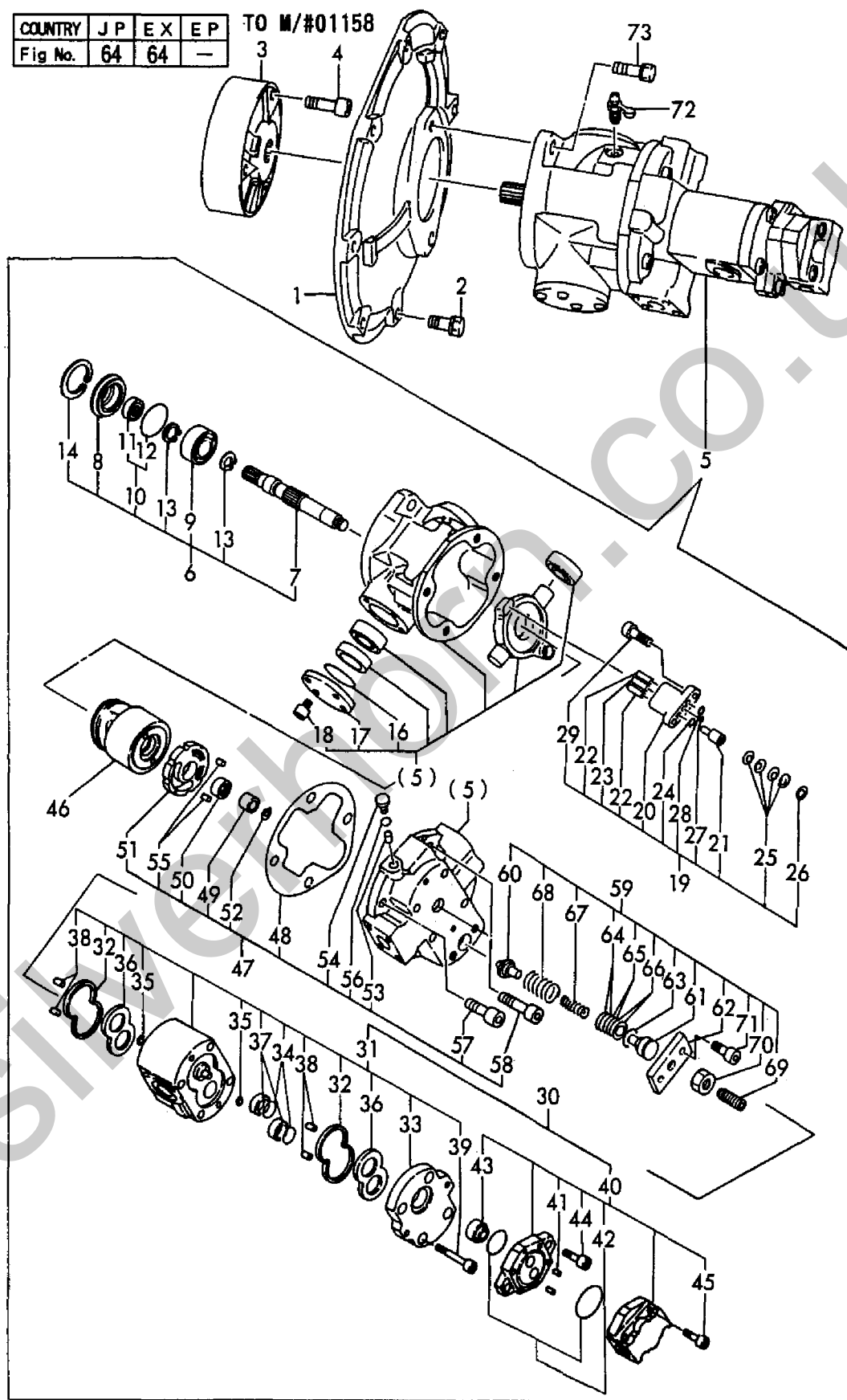
Fig. 64 油圧ポンプ & 軸継手(旧形) HYD. OIL PUMP & JOINT(PREVIOUS)
