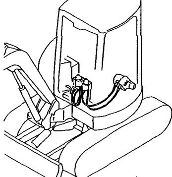
Fig.102 コントロール配管 (ダイレクト仕様) CONTROL PIPING (DIRECT SPEC.)
