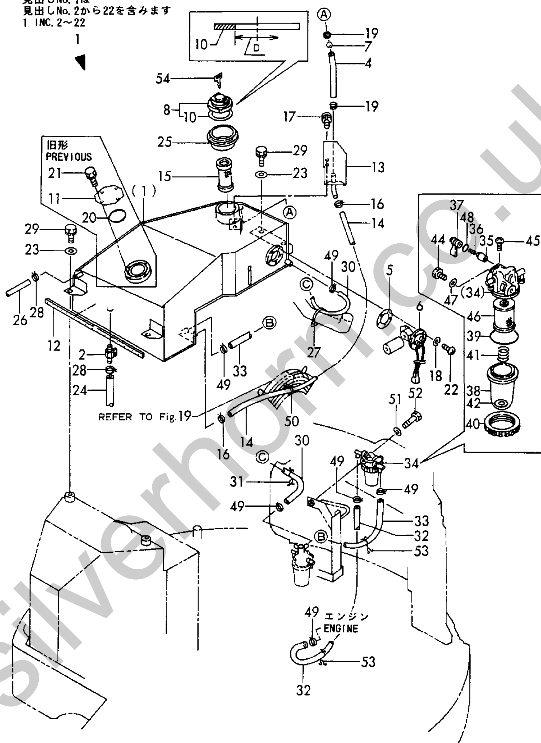
Fig. 21 燃料タンク & 燃料パイプ FUEL TANK & FUEL LINE
