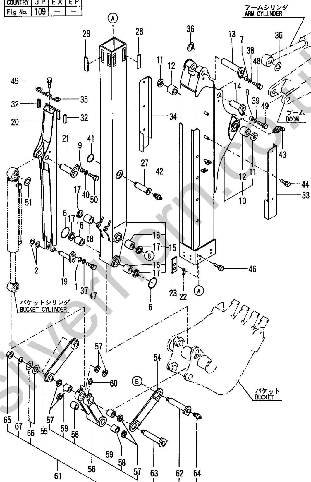
Fig. 109 テレスコピックアーム & バケットリンク TELESCOPIC ARM & BUCKET LINK
