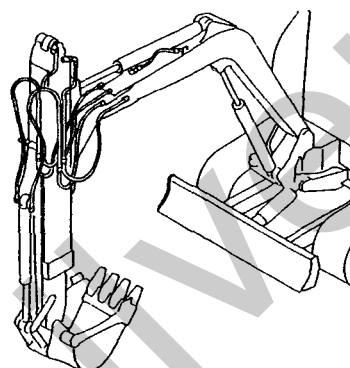
Fig.100 コントロール配管(ポンプ ～バルブ～リターン)(旧形) CONTROL PIPING(PUMP VALVE～RETURN)(PREVIOUS)
