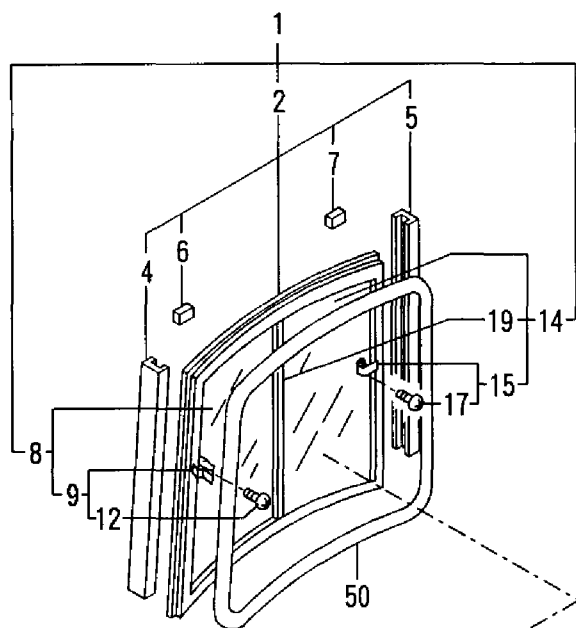
Fig. 59 キャビン(2)(サッシ) CABIN(2)(SASH)
