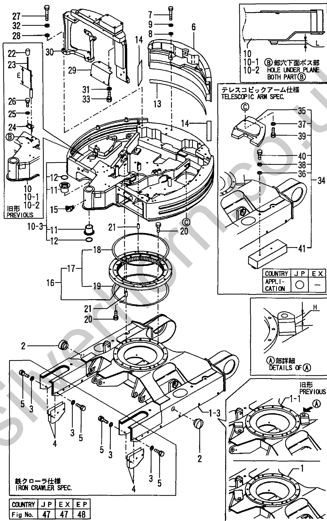
Fig. 47 フレーム & 旋回ベアリング(JP, EX) FRAME & TURNING BEARING(JP, EX)
