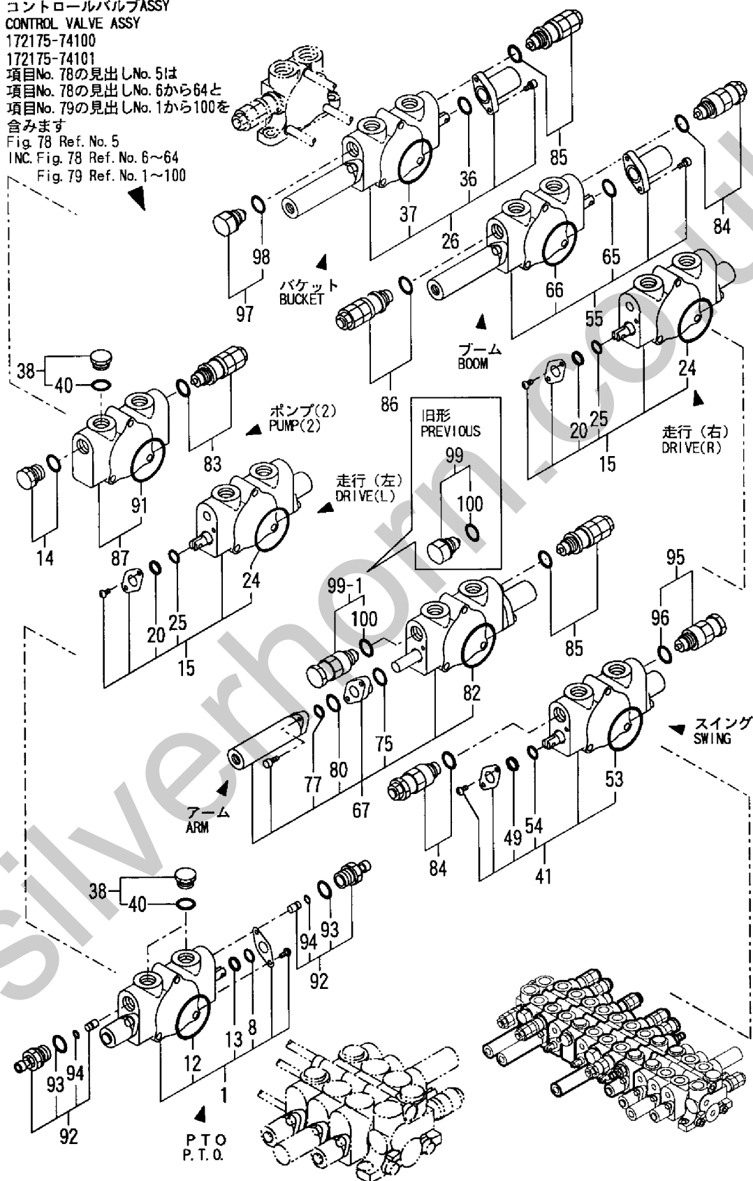
Fig. 79 コントロールバルブ(2/2) CONTROL VALVE(2/2)
