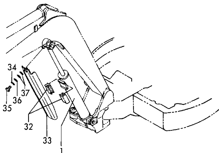
Fig. 66 ブームシリンダ(キャビン) BOOM CYLINDER(CABIN)
