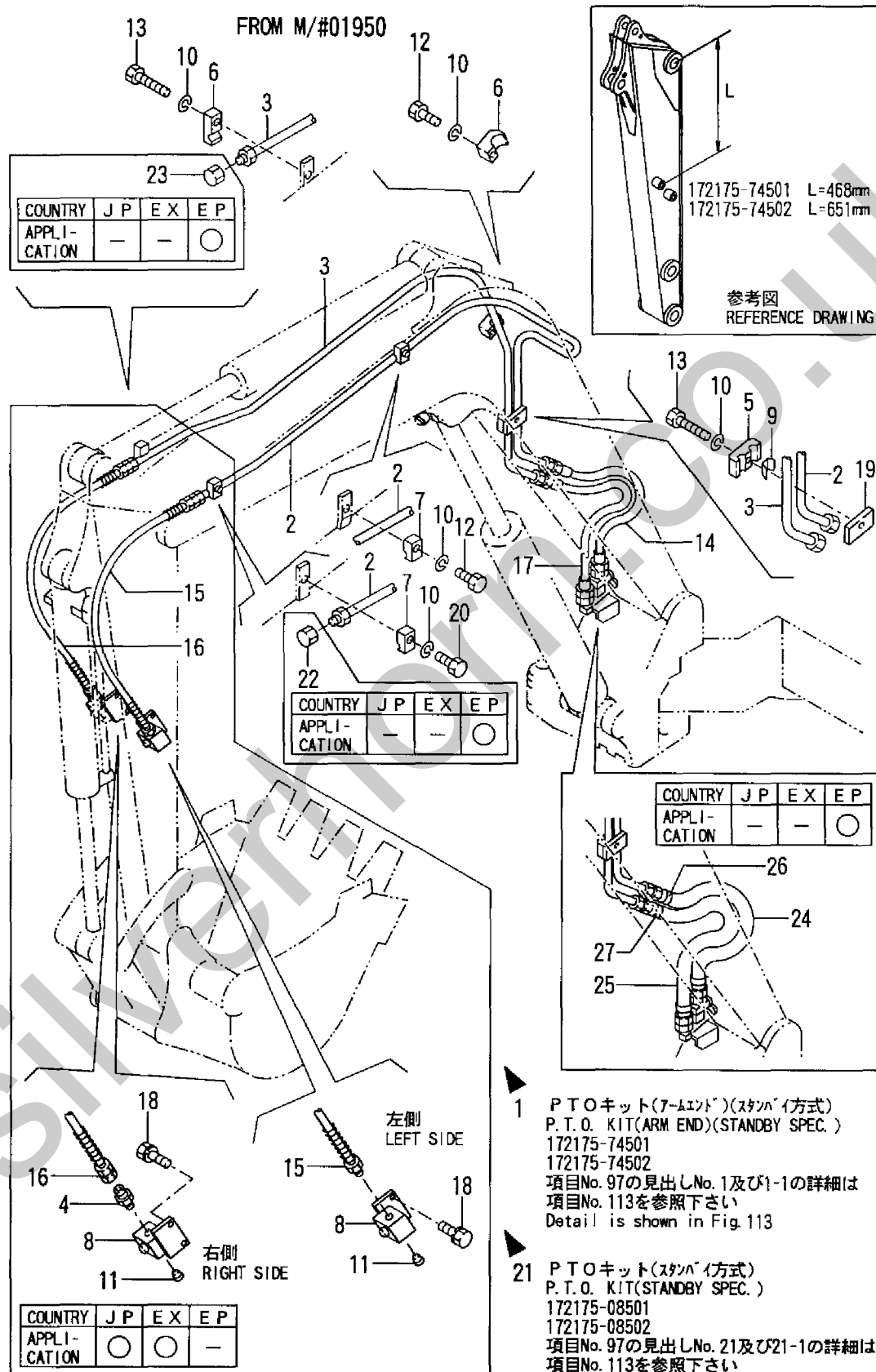
Fig. 97 油圧配管(PTO7-エンド)(新形) HYD. OIL PIPING(P. T. O. ARM END)(NEW)
