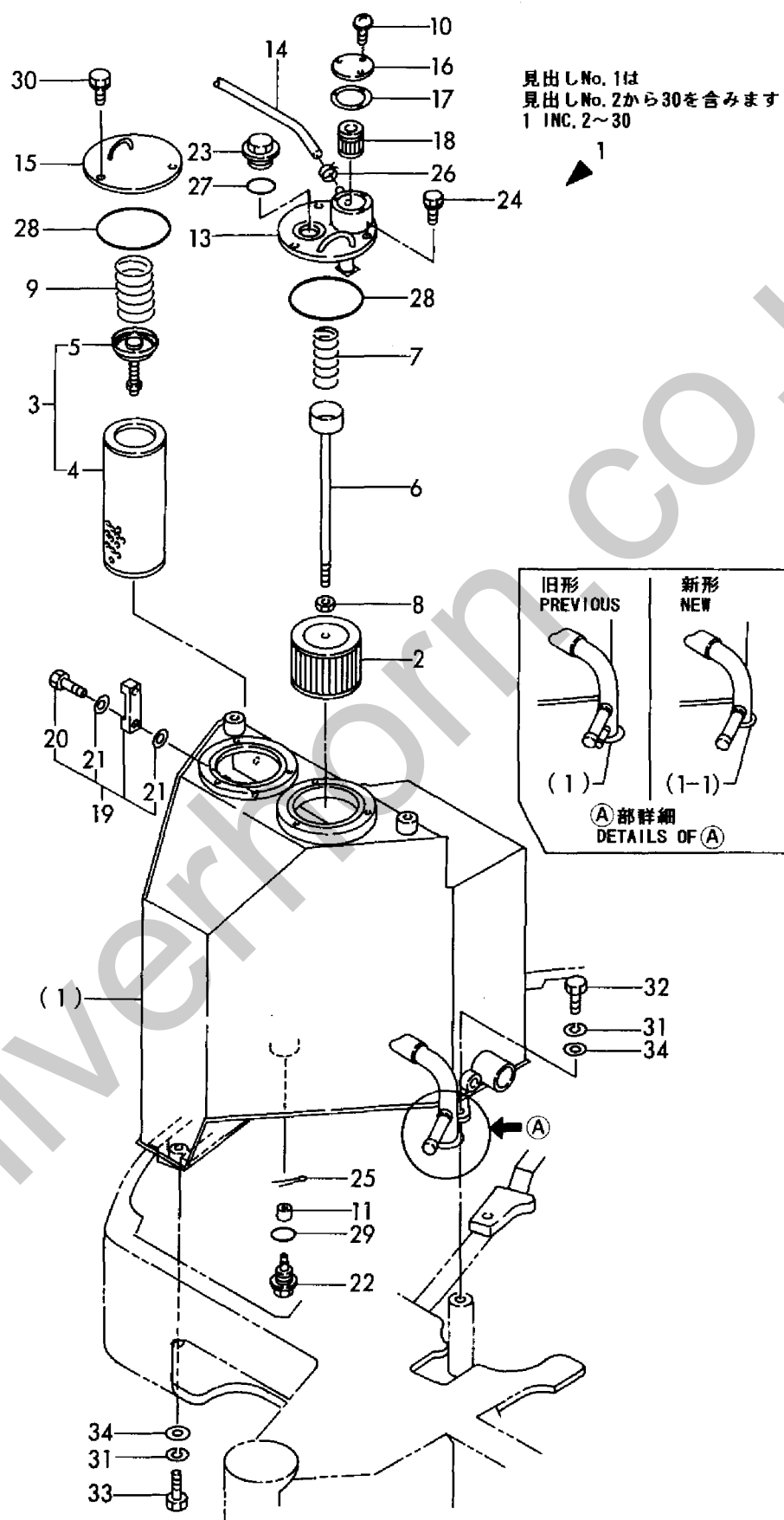
Fig. 84 作動油タンク HYD. OIL TANK
