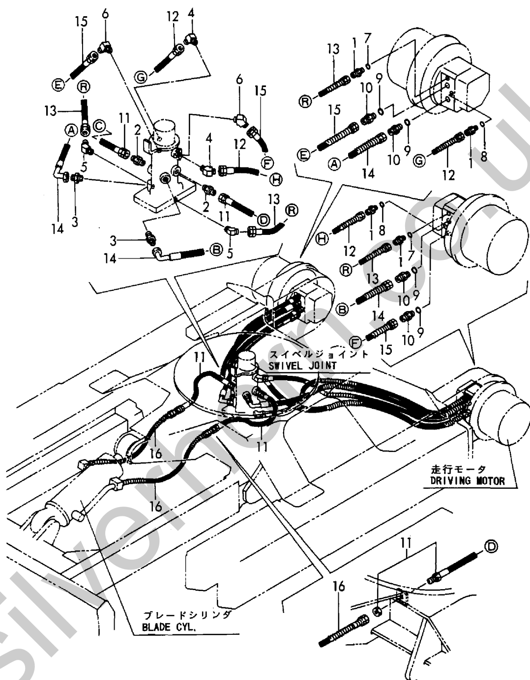
Fig. 94 油圧配管(トラックフレーム) HYD. OIL PIPING (TRACK FRAME)
