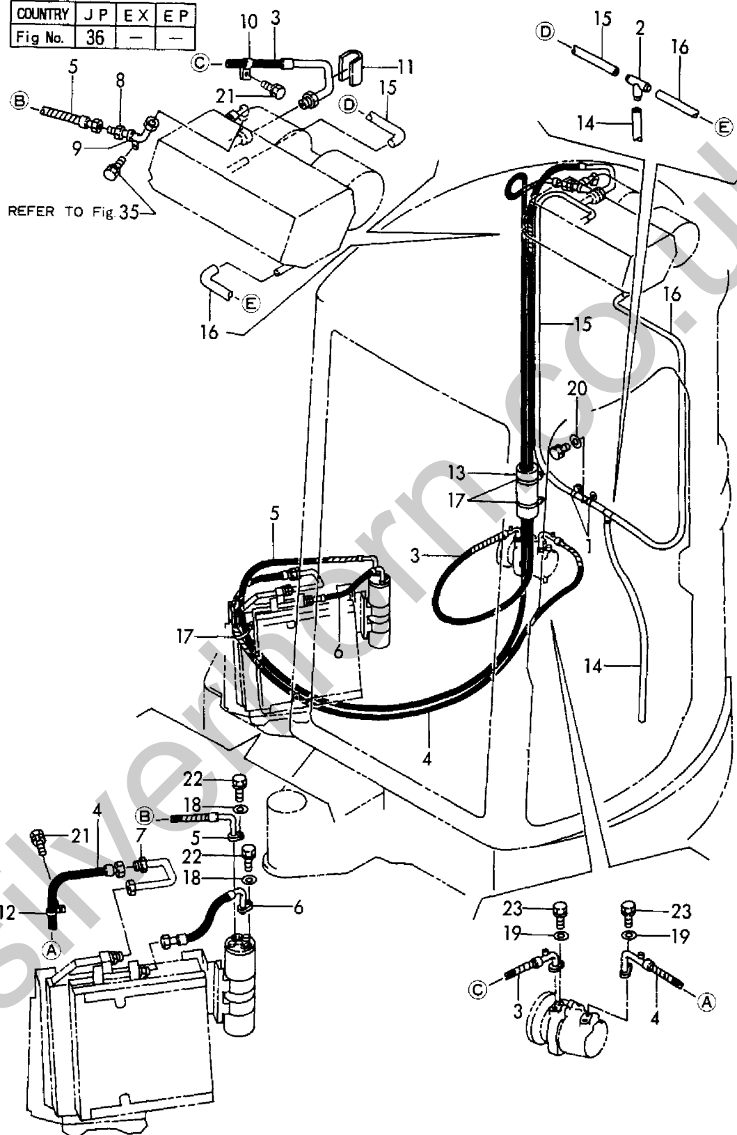
Fig. 36 クーラ(配管) COOLER(HYD. OIL PIPING)
