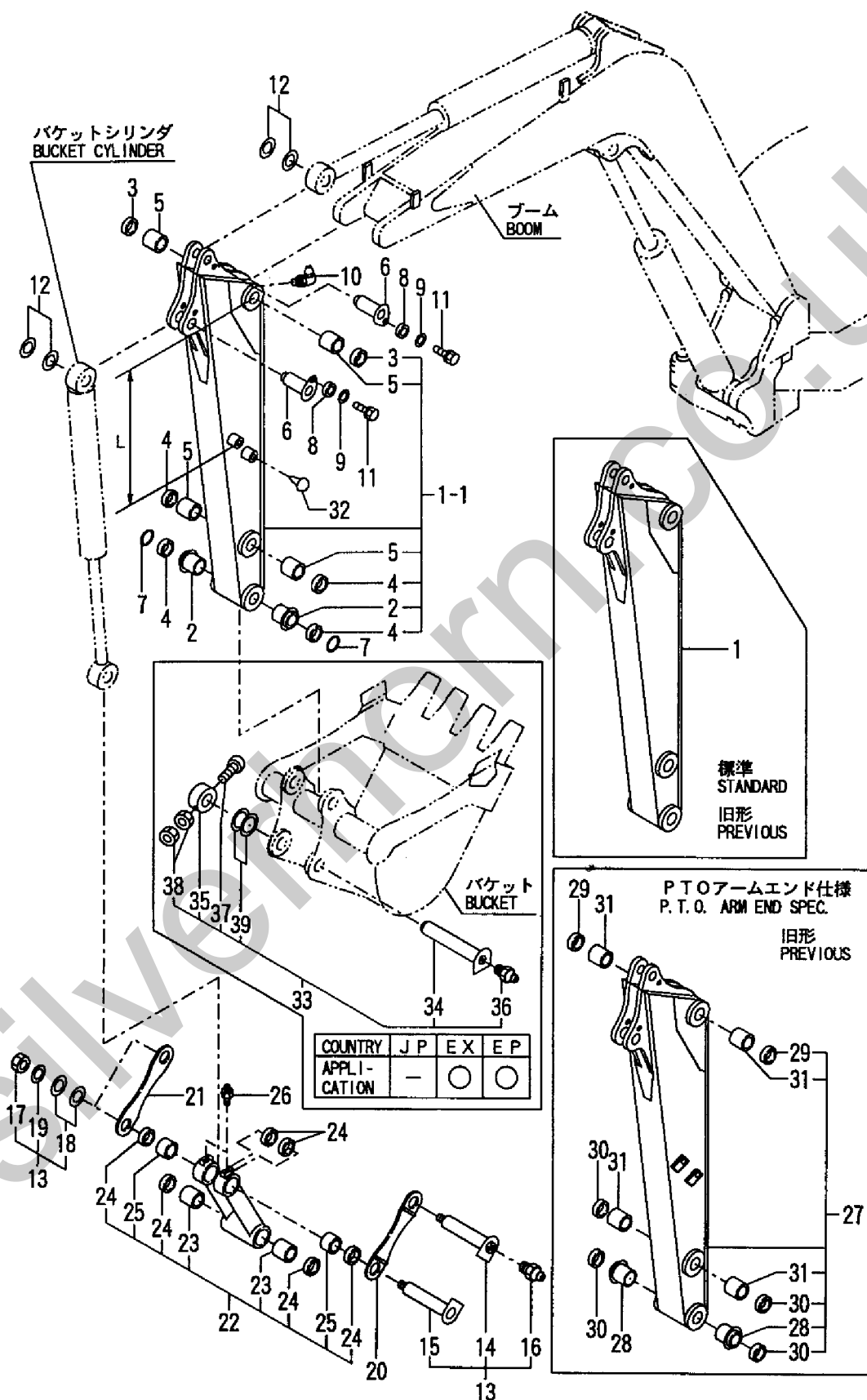
Fig. 108 アーム & バケットリンク ARM & BUCKET LINK
