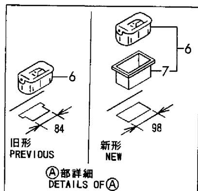
Fig. 27 電装品(キャビン専用) ELECTRIC PART(CABIN)
