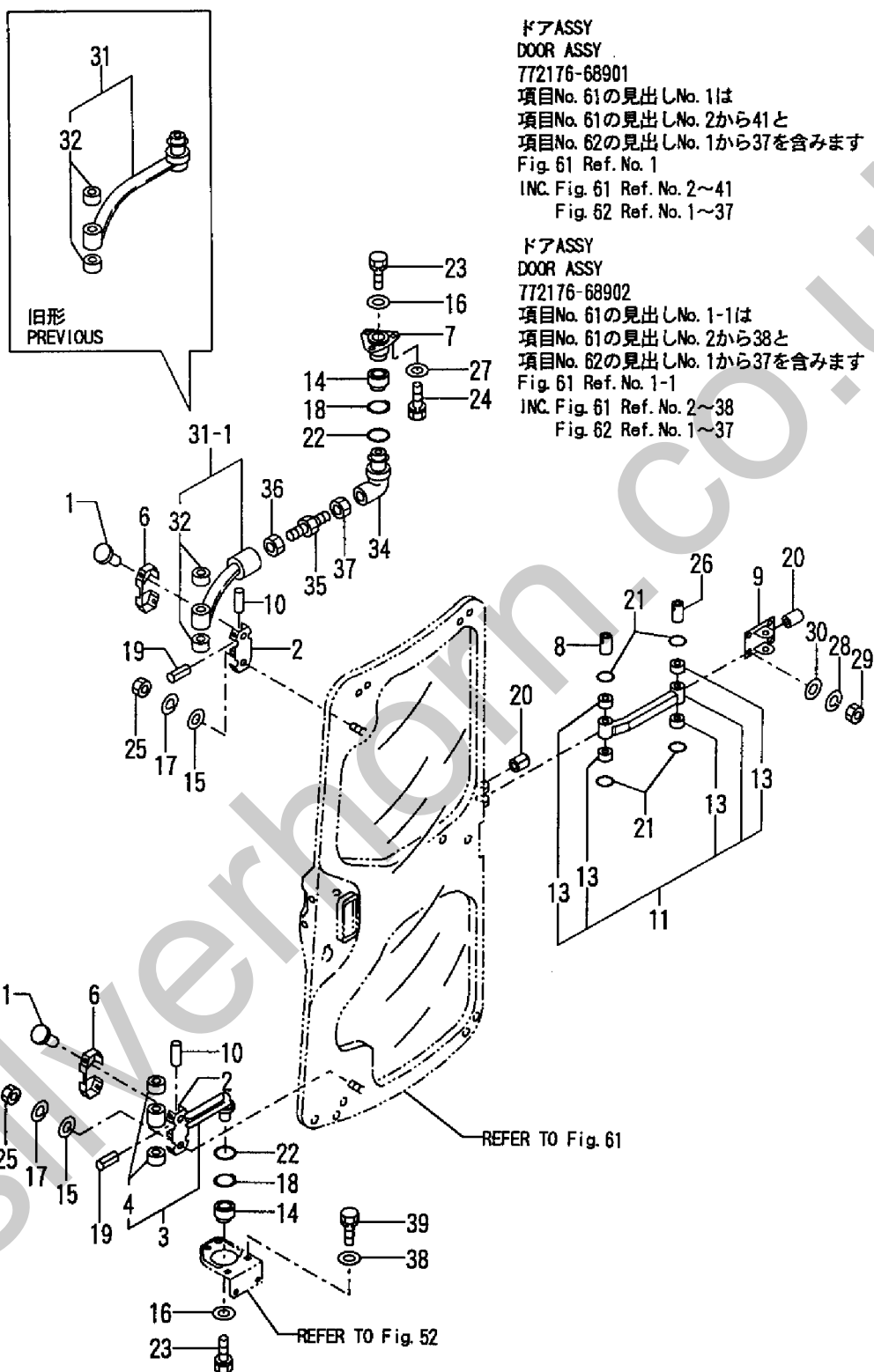
Fig. 62 キャビンドア(2)(付属品) CABIN DOOR(2)(FITTING PART)
