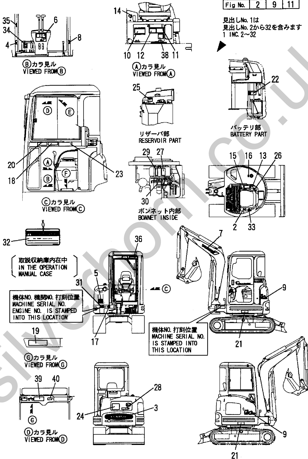
Fig. 9 銘板(キャビン:EX) LABEL (CABIN:EX)
