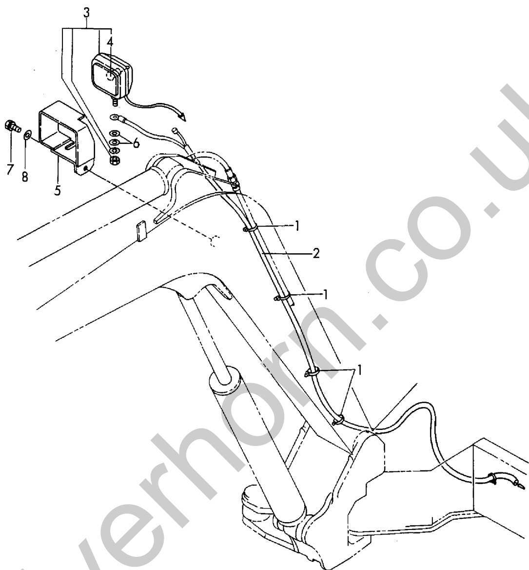
Fig. 29 ワークランプ WORK LAMP
