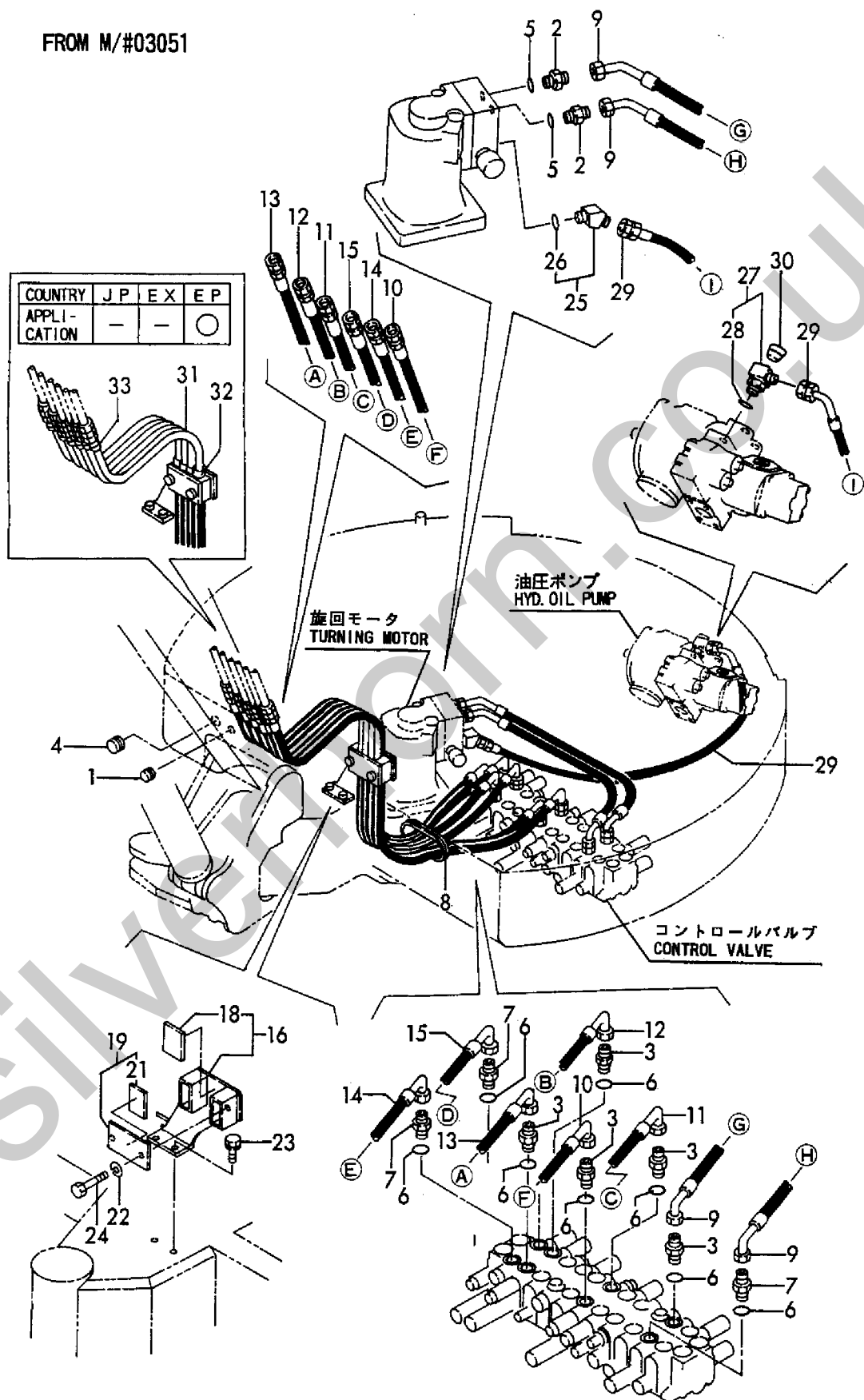
Fig. 88 油圧配管(ポンプ、バルブ〜モータ、ブーム) HYD. OIL PIPING(PUMP, VALVE~MOTOR, BOOM)
