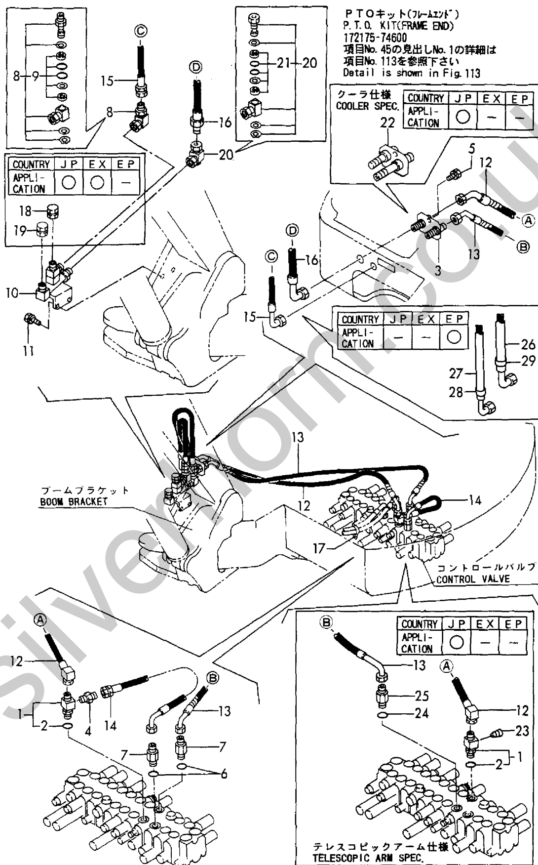
Fig. 93 油圧配管(PTOフレームエンド) HYD. OIL PIPING(P. T. O. FRAME END)
