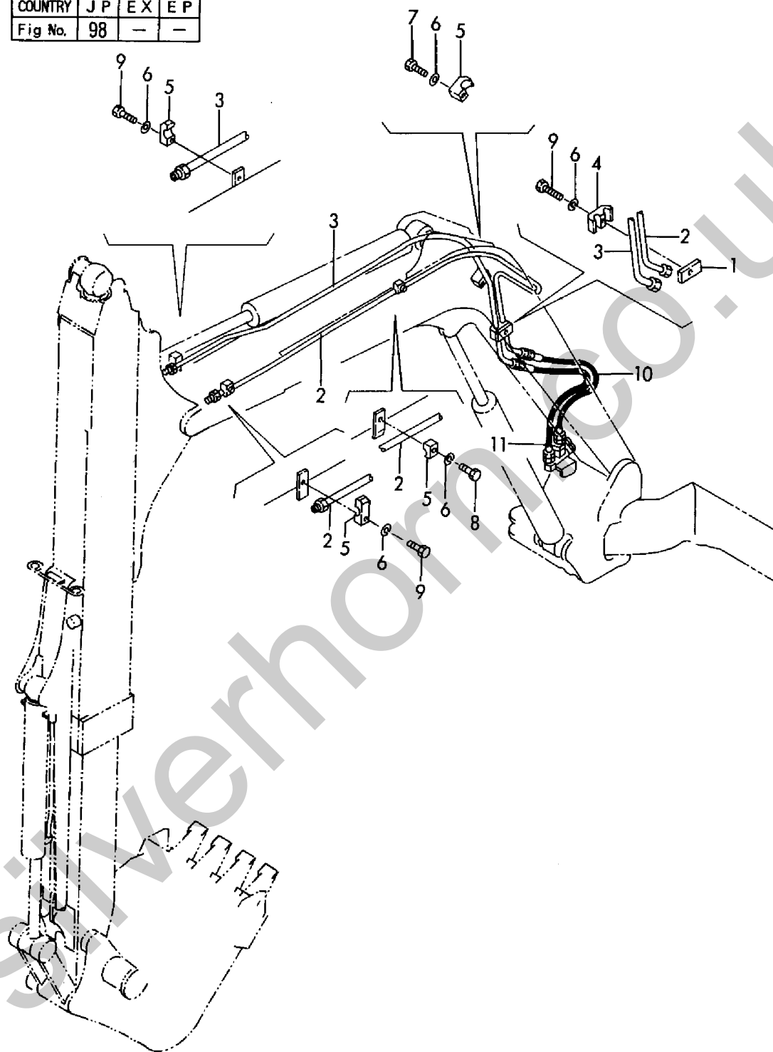
Fig. 98 油圧配管(テレスコピックアーム:ブーム) HYD. OIL PIPING (TELESCOPIC ARM: BOOM)
