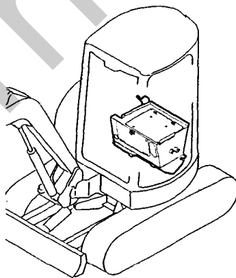
Fig. 56 ボンネット BONNET
