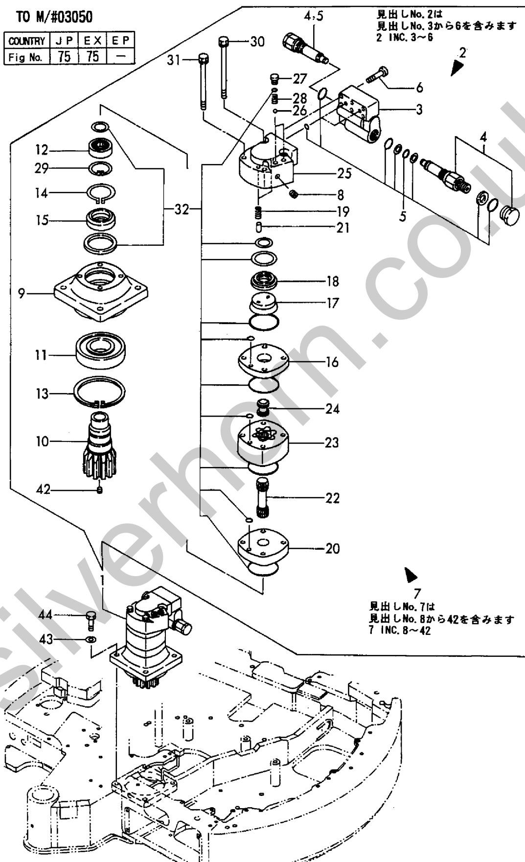
Fig. 75 旋回モータ(旧形) TURNING MOTOR(PREVIOUS)
