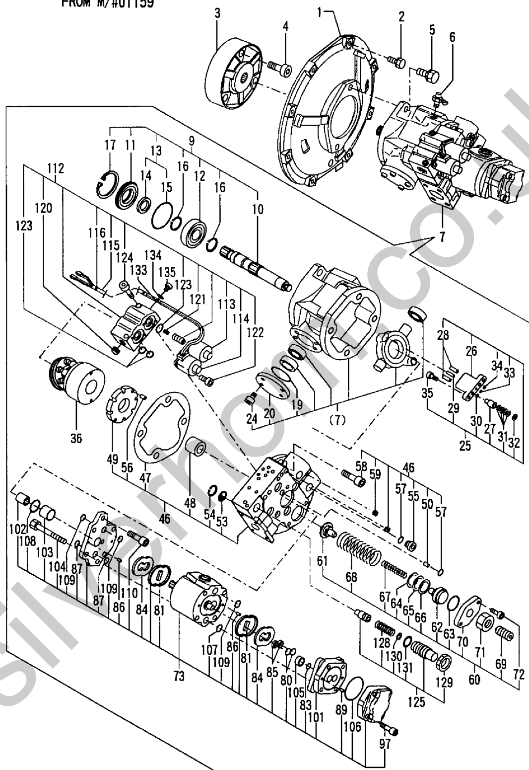
Fig. 65 油圧ポンプ & 軸継手(新形) HYD. OIL PUMP & JOINT(NEW)
