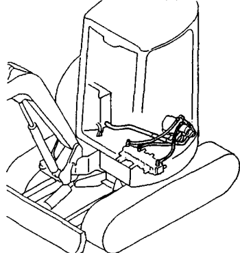
Fig. 86 油圧配管(タンク～ポンプ ～バルブ)(新形) HYD. OIL PIPING(TANK～PUMP ～VALVE)(NEW)
