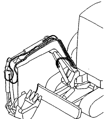
Fig. 96 油圧配管(PTOフレームエンド) HYD. OIL PIPING (P. T. O. ARM END)(PREVIOUS)
