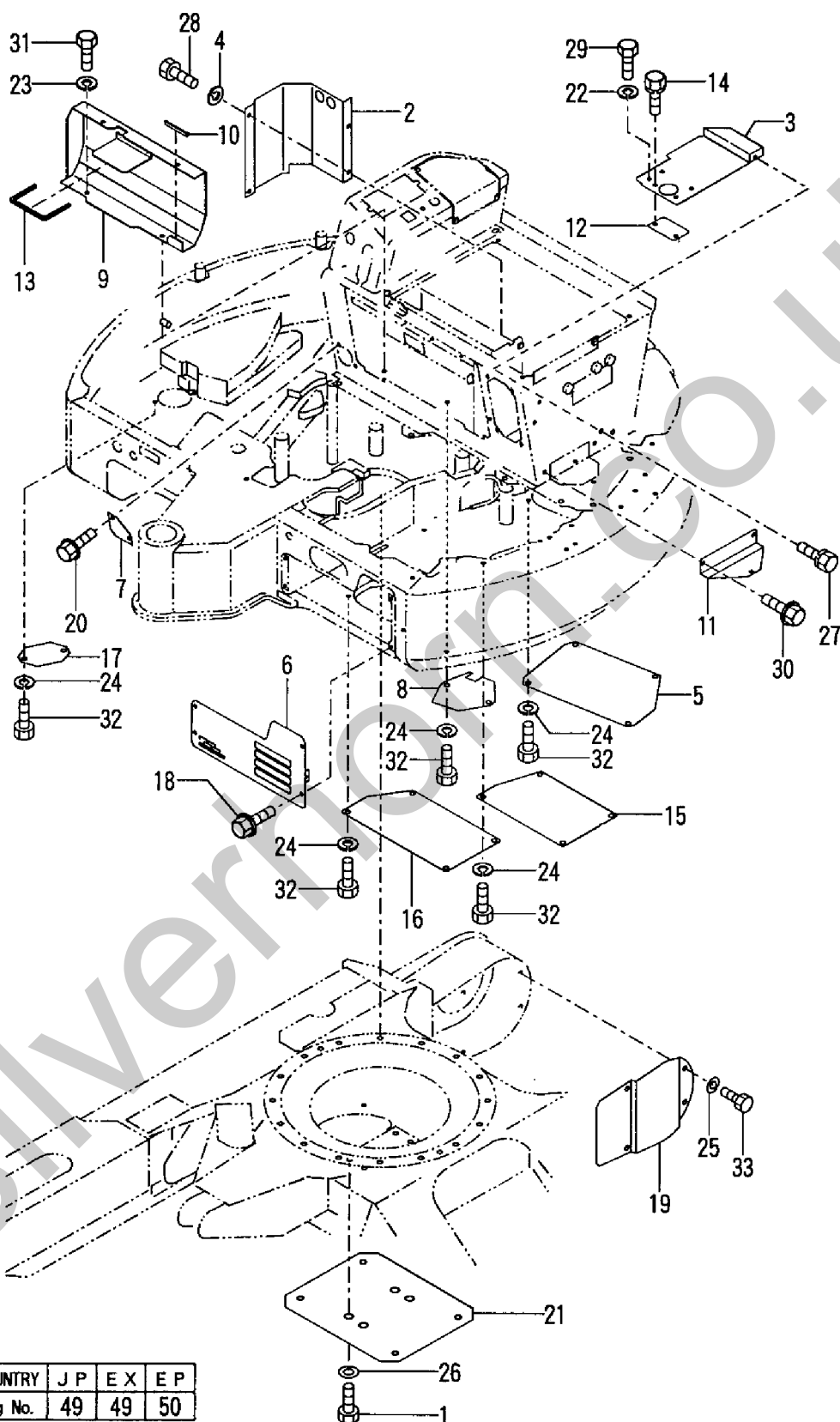
Fig. 50 フレームカバー(キャビン仕様)(EP) FRAME COVER(CABIN SPEC.)(EP)
