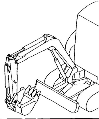
Fig.108 アーム & バケットリンク ARM & BUCKET LINK
