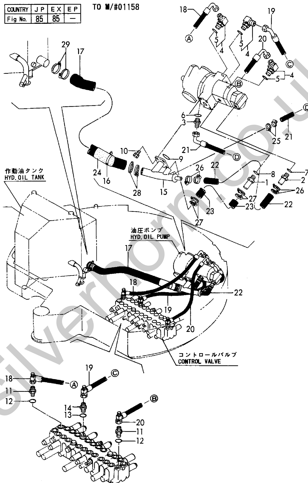
Fig. 85 油圧配管(タンク〜ポンプ〜バルブ)(旧形) HYD. OIL PIPING(TANK~PUMP~VALVE)(PREVIOUS)
