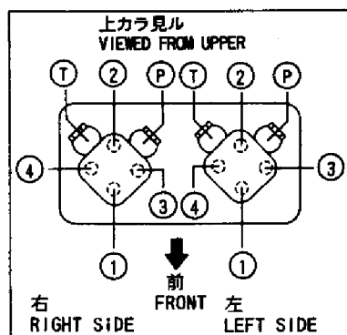
Fig. 101 コントロール配管(ポンプ～バルブ～リターン)(新形) CONTROL PIPING(PUMP～VALVE～RETURN)(NEW)
