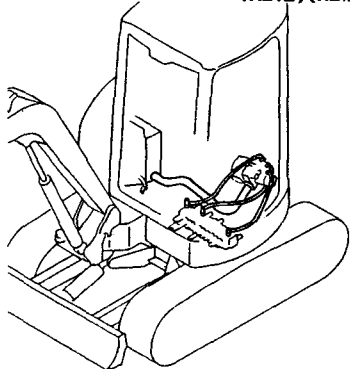
Fig. 87 油圧配管(バルブ～モータ, ブーム) HYD. OIL PIPING(VAIVE ～MOTOR, BOOM)
