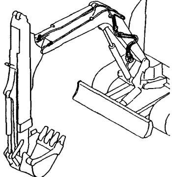
Fig.99 油圧配管(テレスコピックアーム:アーム) HYD. OIL PIPING (TELESCOPIC ARM:ARM)
