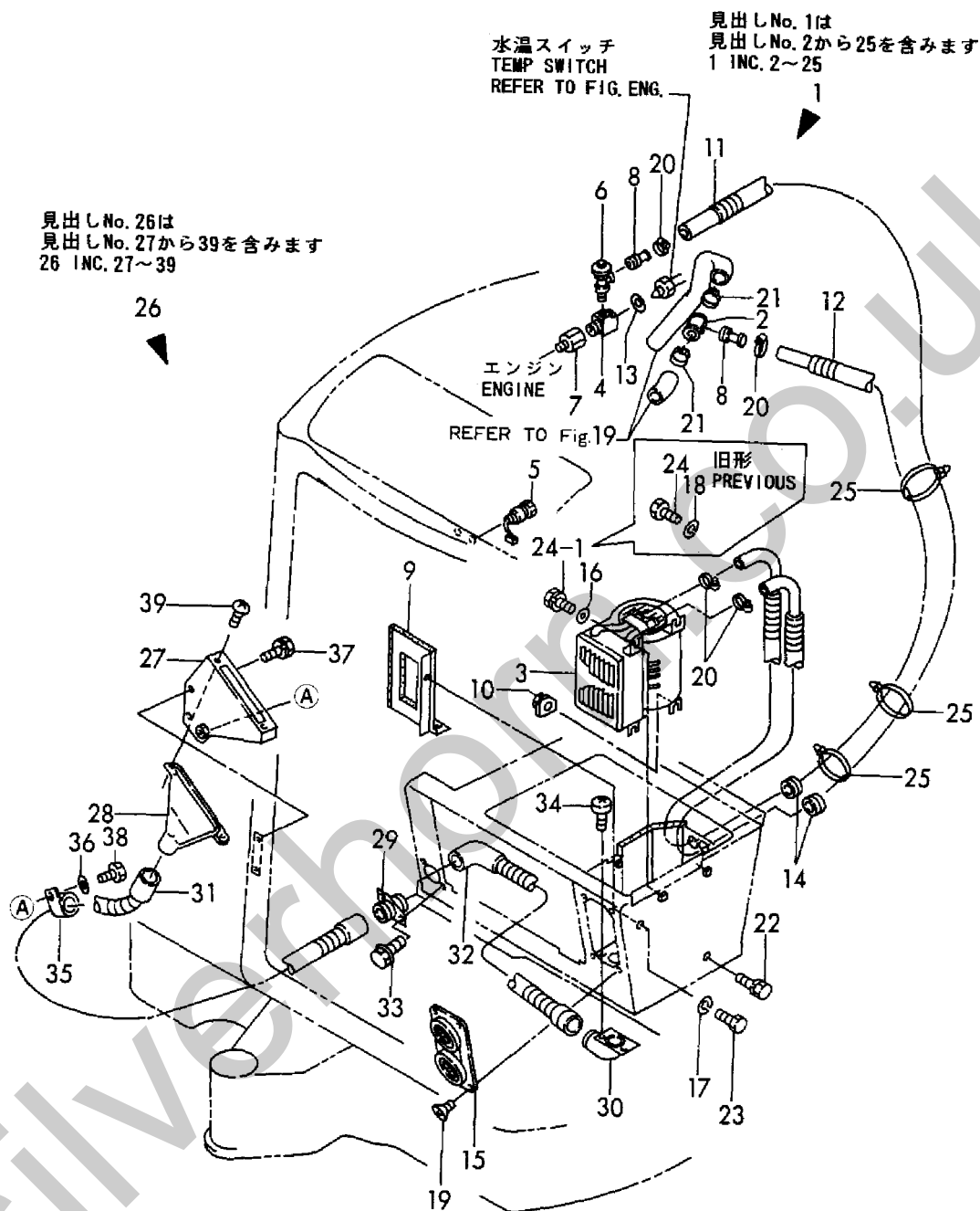
Fig. 30 ヒータ & デフロスタ HEATER & DEFROSTER
