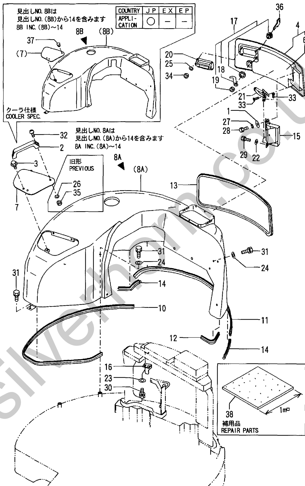
Fig. 56 ボンネット BONNET
