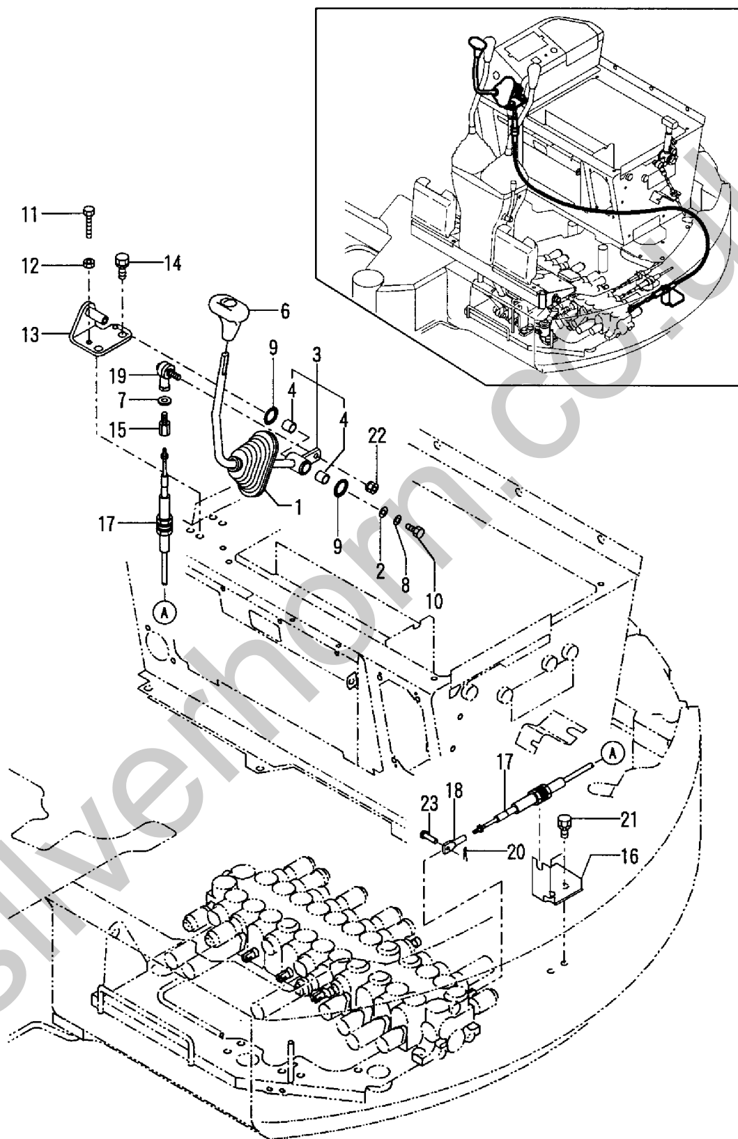
Fig. 44 操縦装置(ブレード) CONTROL EQUIPMENT (BLADE)
