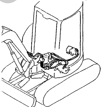
Fig. 88 油圧配管(ポンプ, バルブ ～モータ, ブーム) HYD. OIL PIPING(PUMP, VAIVE ～MOTOR, BOOM)
