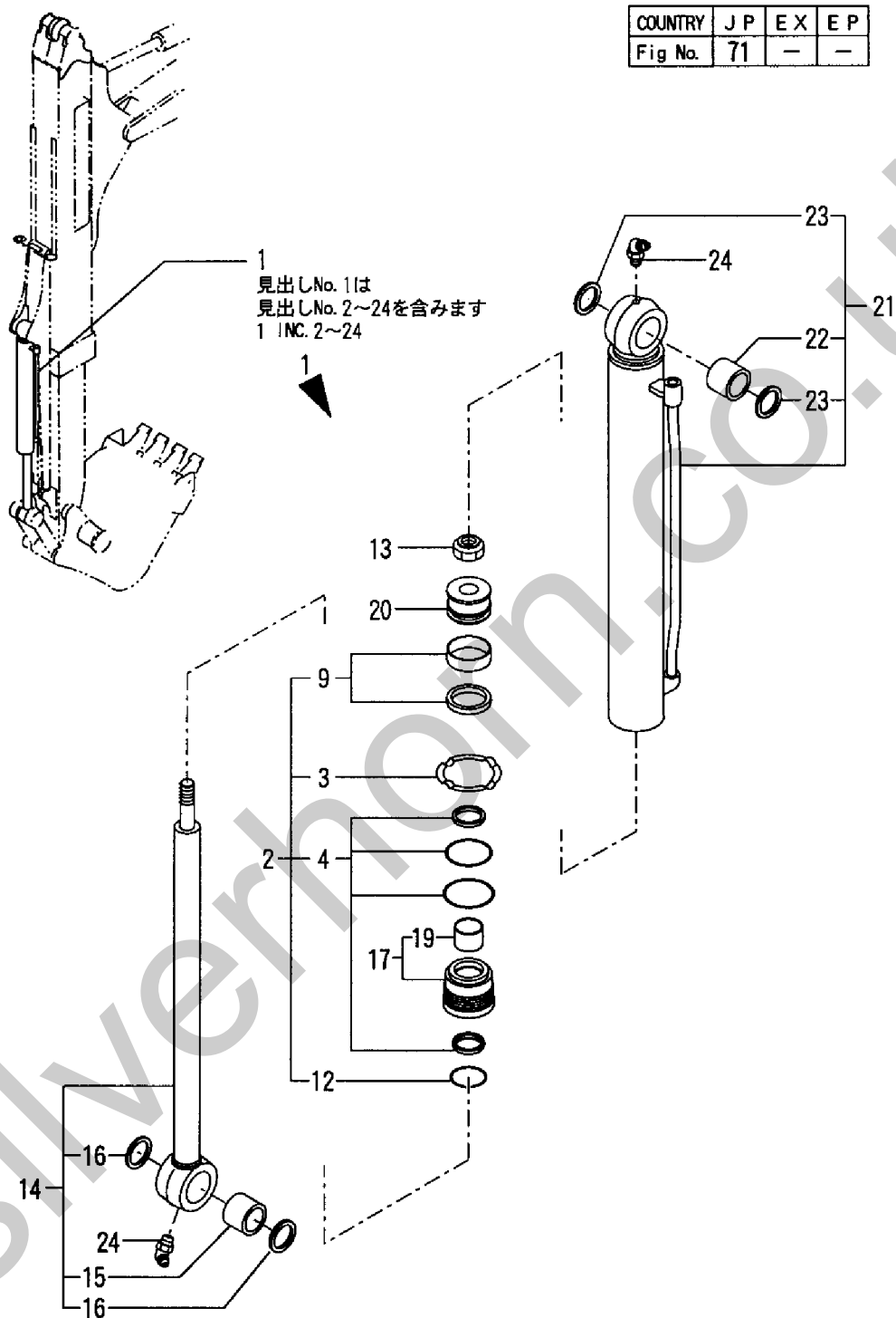
Fig. 71 バケットシリンダ(テレスコピックアーム仕様) BUCKET CYLINDER (TELESCOPIC ARM SPEC.)
