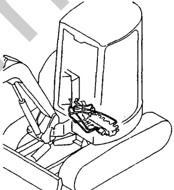
Fig. 92 油圧配管(リターン)(新形) HYD. OIL PIPING(RETURN) (NEW)
