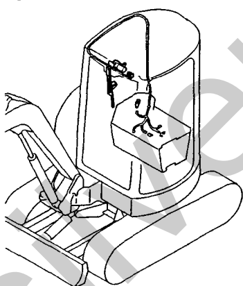
Fig.28 電装品(クーラ仕様) ELECTRIC PART(COOLER SPEC.)
