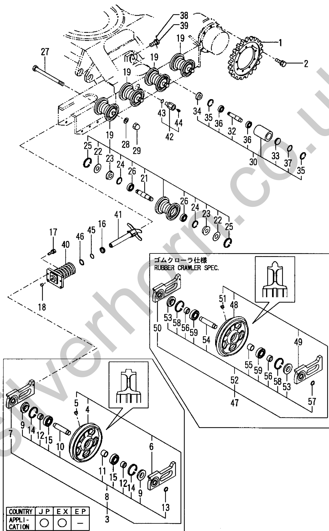
Fig. 37 ローラ & アジャスト ROLLER & ADJUST
