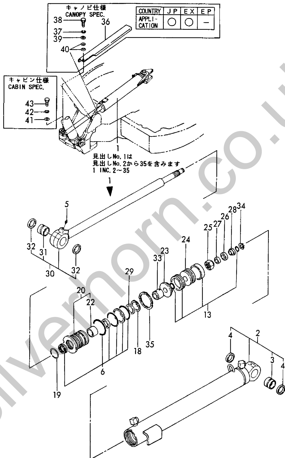
Fig. 72 スイングシリンダ SWING CYLINDER
