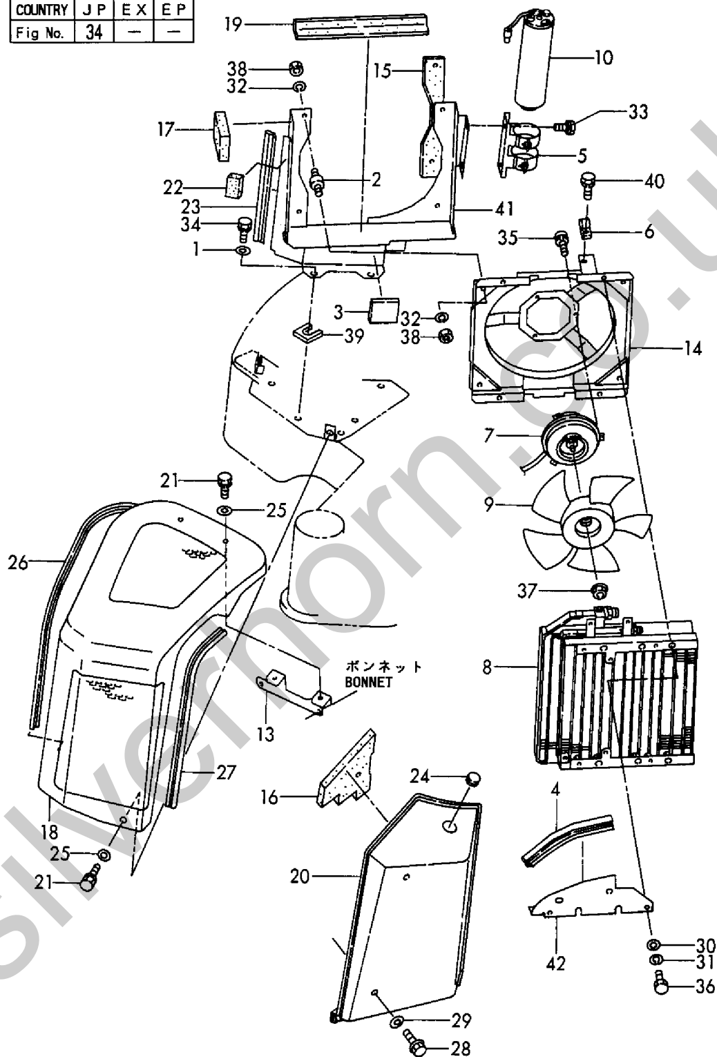
Fig. 34 クーラ(コンデンサ関連) COOLER(CONDENSER RELATED)
