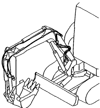
Fig.98 油圧配管 (テレスコピックアーム:ブーム) HYD. OIL PIPING (TELESCOPIC ARM:BOOM)
