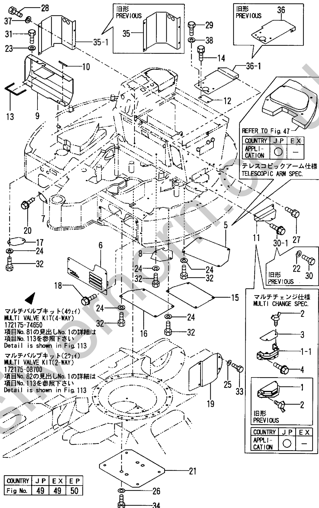
Fig. 49 フレームカバー(キャビン仕様)(JP, EX) FRAME COVER(CABIN SPEC.)(JP, EX)
