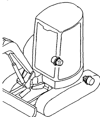
Fig. 75 旋回モータ(旧形) TURNING MOTOR(PREVIOUS)
