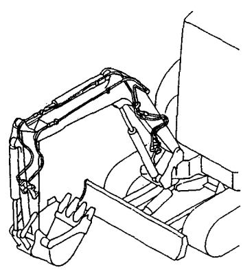
Fig. 96 油圧配管(PTOフレームエンド) HYD. OIL PIPING (P. T. O. ARM END)(PREVIOUS)
