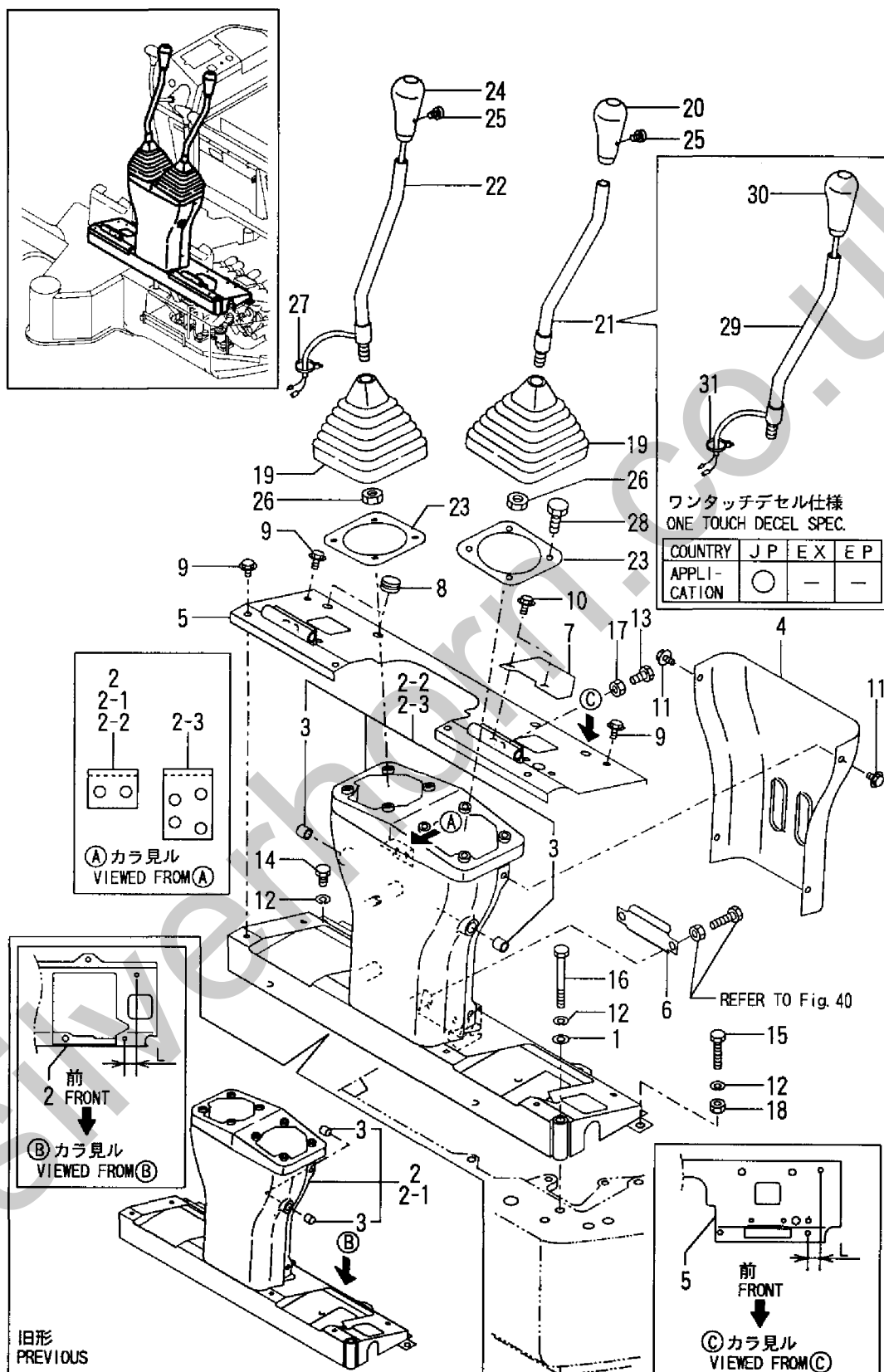
Fig. 39 操縦装置(作業レバー & スタンド) CONTROL EQUIPMENT(OPERATION LEVER & STAND)
