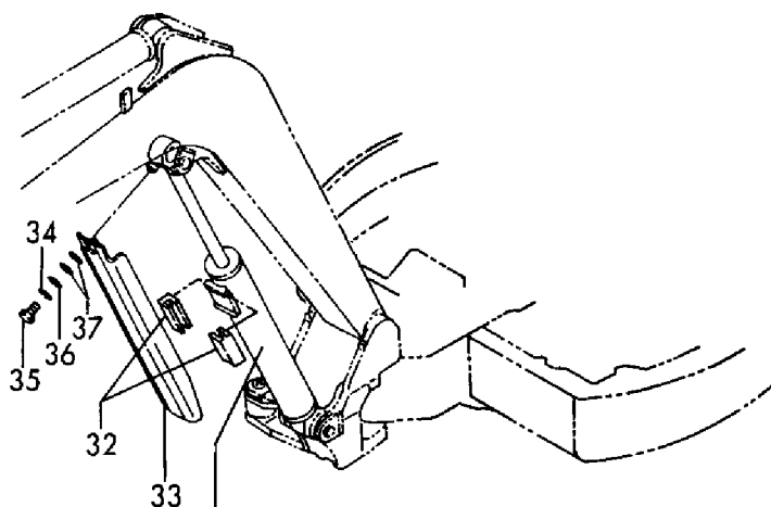
Fig. 67 ブームシリンダ(キャピ°) BOOM CYLINDER(CANOPY)
