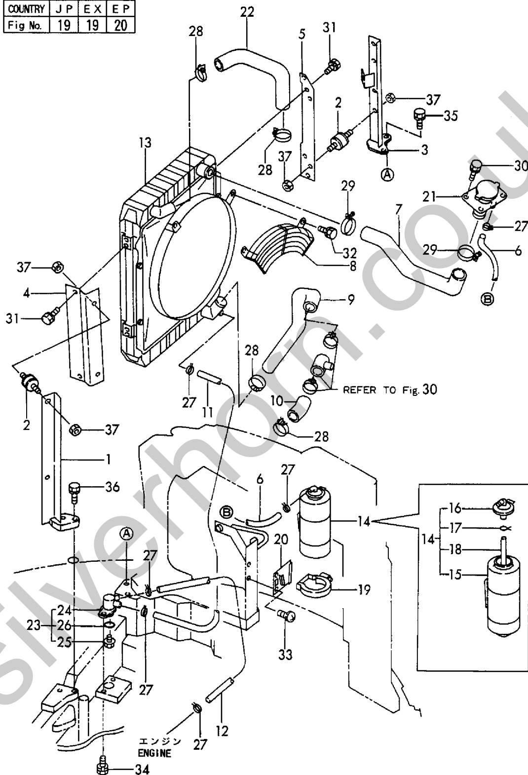
Fig. 20 ラジエータ & マウント(EP) RADIATOR & MOUNT(EP)
