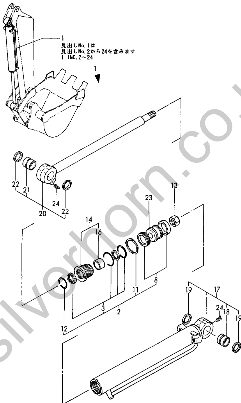
Fig. 70 バケットシリンダ(標準仕様) BUCKET CYLINDER(STANDARD SPEC.)
