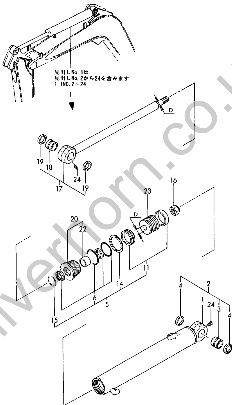
Fig. 68 アームシリンダ ARM CYLINDER
