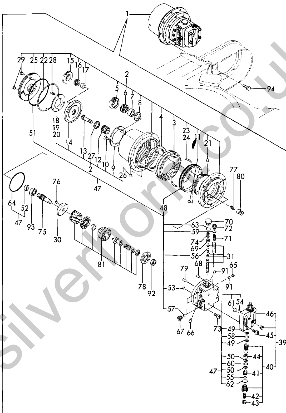
Fig. 74 走行モータ DRIVING MOTOR
