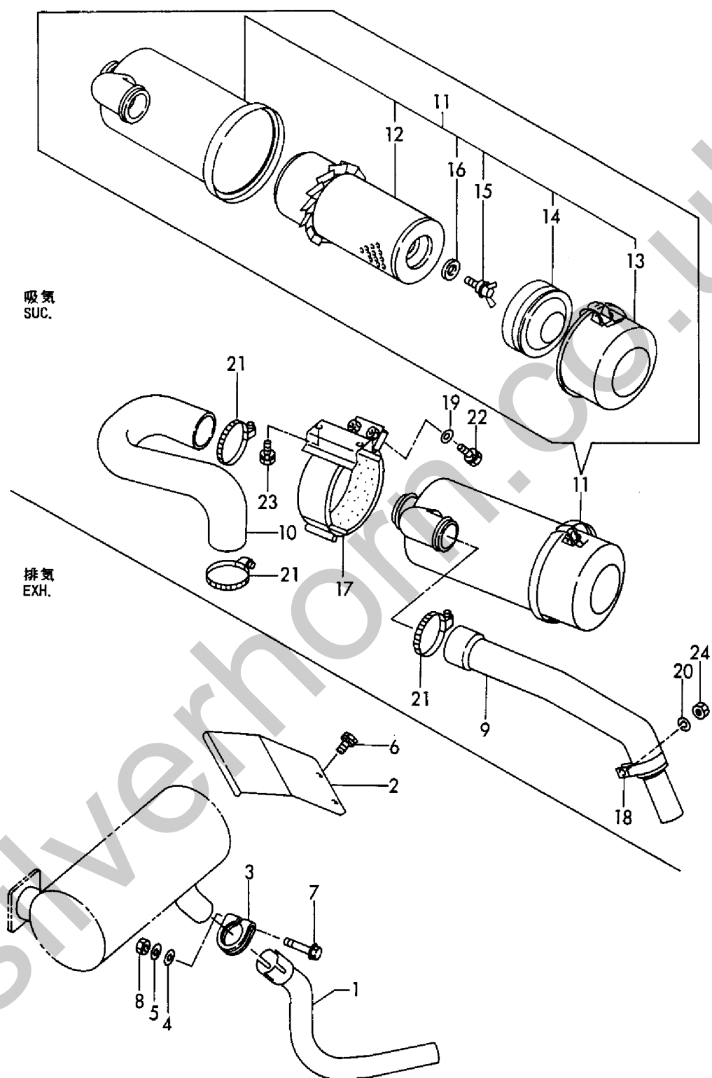
Fig. 15 吸気管 & 排気管 SUC. PIPE & EXH. PIPE
