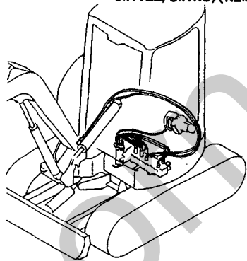
Fig. 91 油圧配管(リターン)(旧形) HYD. OIL PIPING(RETURN) (PREVIOUS)
