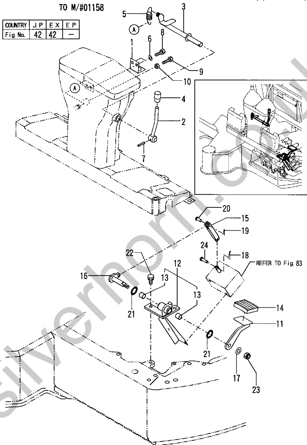
Fig. 42 操縦装置(カットオフレバー & ローハイペダル)(旧形) CONTROL EQUIPMENT(CUT-OFF LEVER & LOW-HIGH PEDAL)(PREVIOUS)
