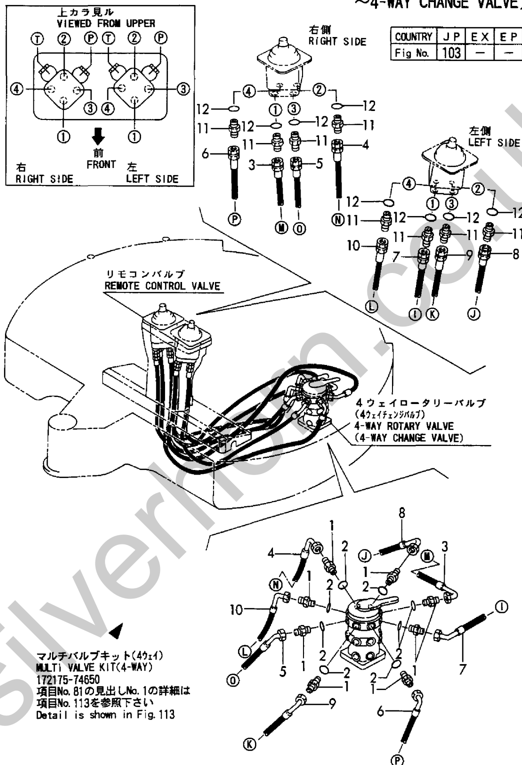
Fig. 103 コントロール配管(リモコンバルブ ~4ウェイチェンジバルブ) CONTROL PIPING(REMOTE CONTROL VALVE ~4-WAY CHANGE VALVE)
