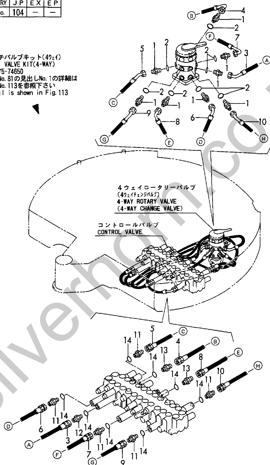
Fig. 104 コントロール配管(4ウェイチェンジバルブ ~コントロールバルブ) CONTROL PIPING(4-WAY CHANGE VALVE ~CONTROL VALVE)
