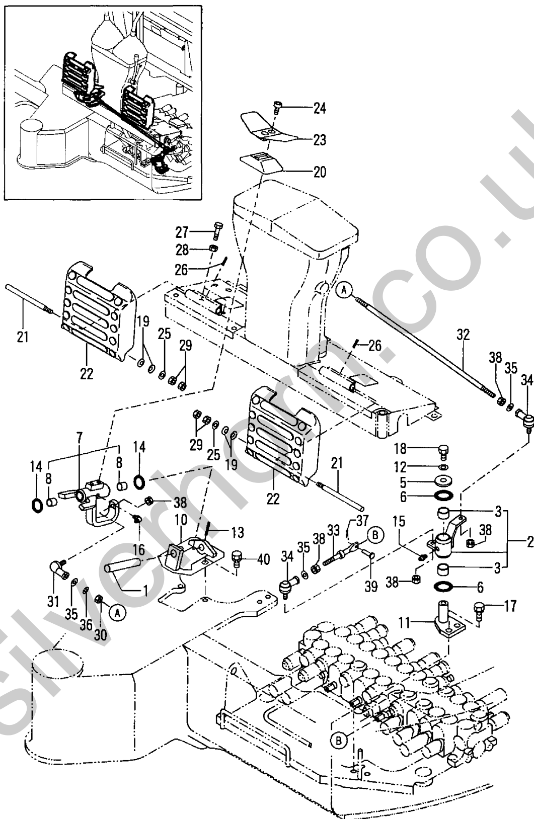
Fig. 41 操縦装置(スイング) CONTROL EQUIPMENT(SWING)
