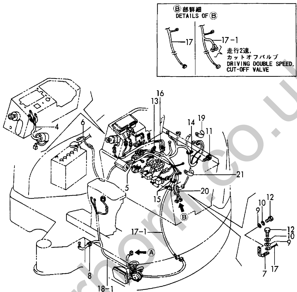
Fig. 23 電装品(ワイリング) ELECTRIC PART(WIRING)
