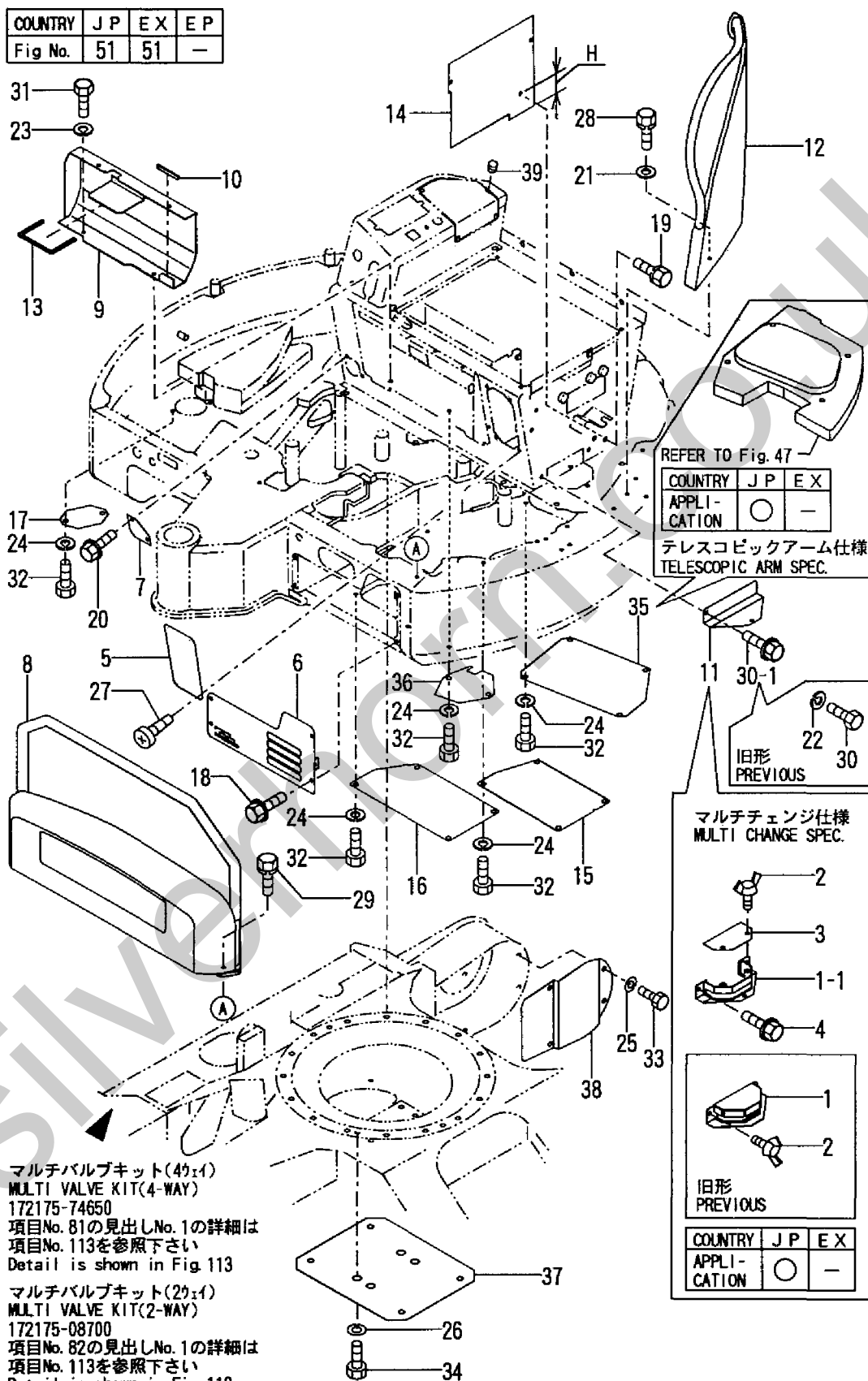
Fig. 51 フレームカバー(キャノピー仕様) FRAME COVER(CANOPY SPEC.)
