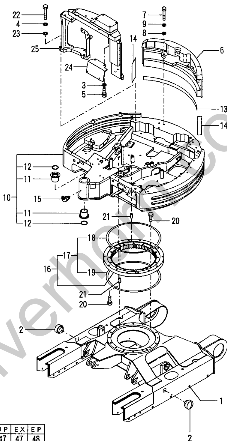
Fig. 48 フレーム & 旋回ベアリング(EP) FRAME & TURNING BEARING(EP)
