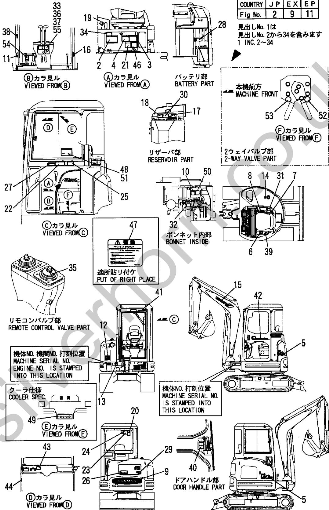
Fig. 2 銘板(キabin:JP)(新形:PL仕様) LABEL(CABIN:JP)(NEW:PL SPEC.)
