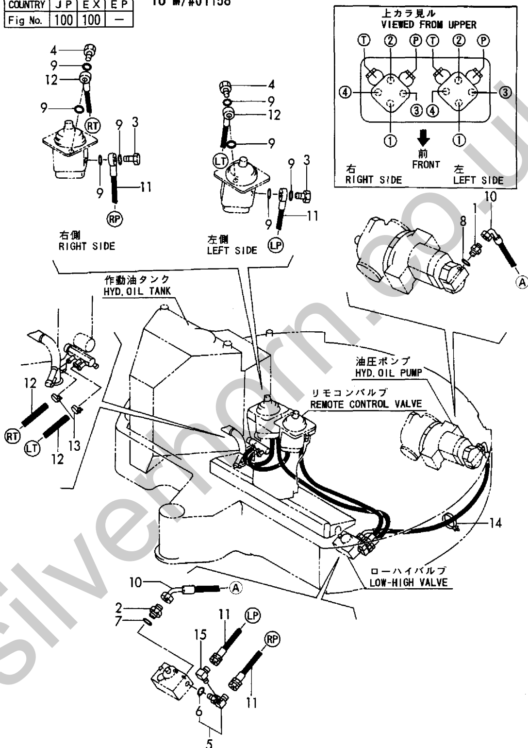
Fig. 100 コントロール配管(ポンプ～バルブ～リターン)(旧形) CONTROL PIPING(PUMP～VALVE～RETURN) (PREVIOUS)
