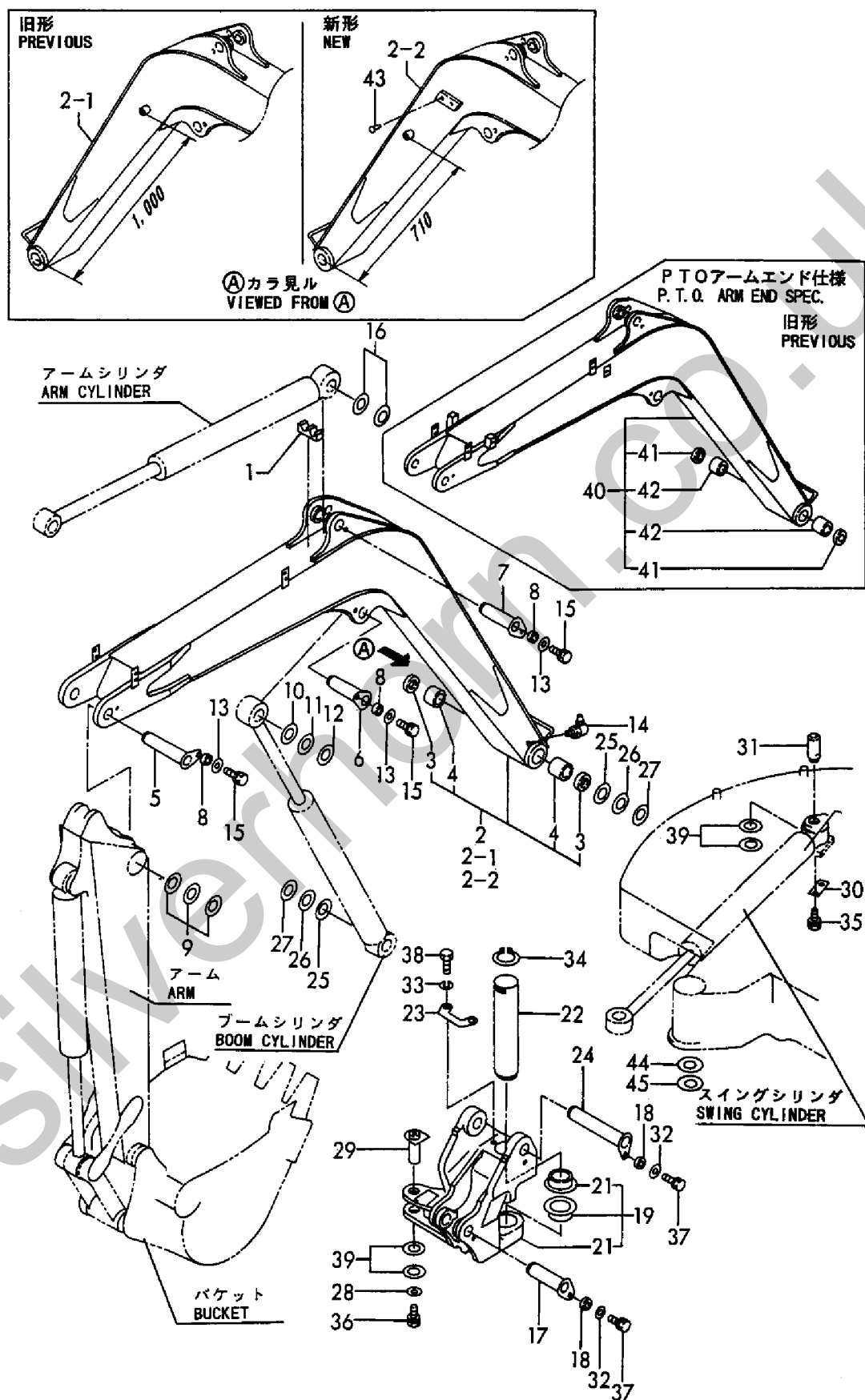
Fig. 107 ブーム & ブームブラケット BOOM & BOOM BRACKET
