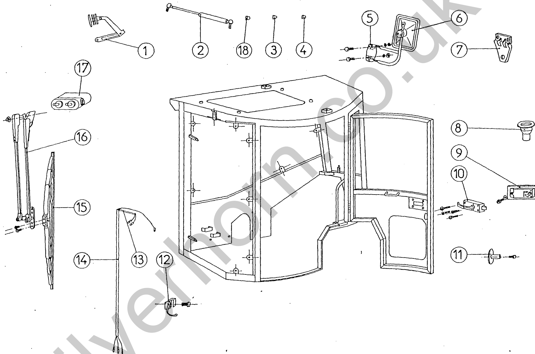
YANMAR Cabine YB5 Nomenclature Divers
