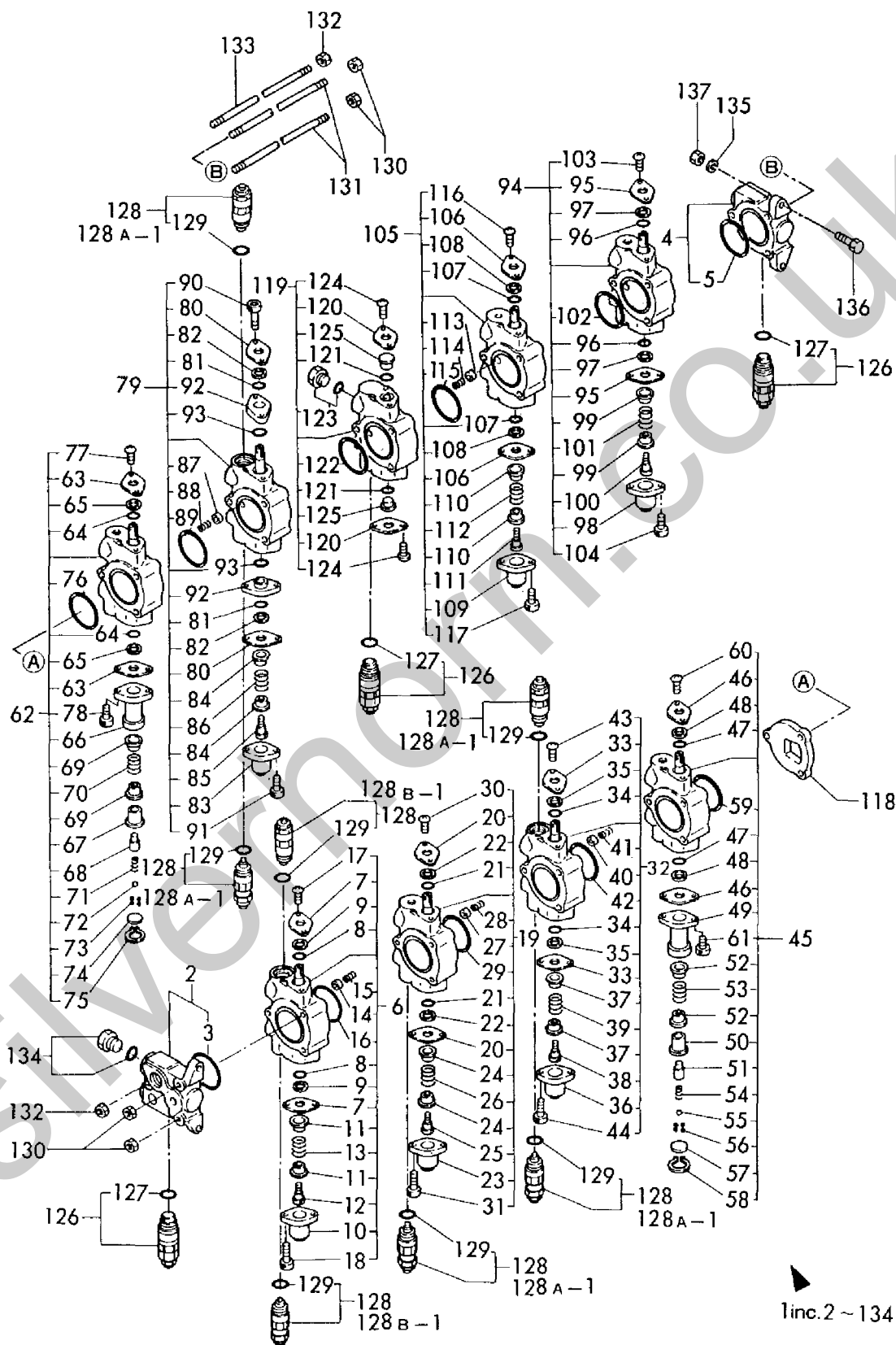
Fig. 82 コントロールバルブ(ブレード) CONTROL VALVE (BLADE) SPEC. CODE D72312-74100
