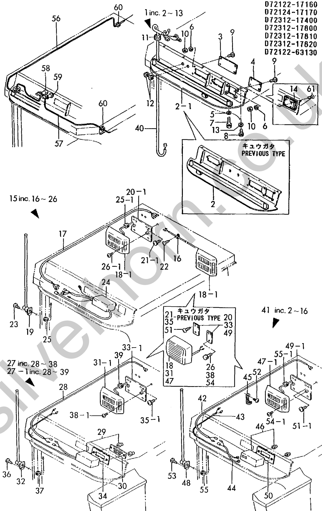
Fig. 24 オーバヘッドパネル & ラジオ(オプション) OVERHEAD PANEL & RADIO(OPTIONAL)
