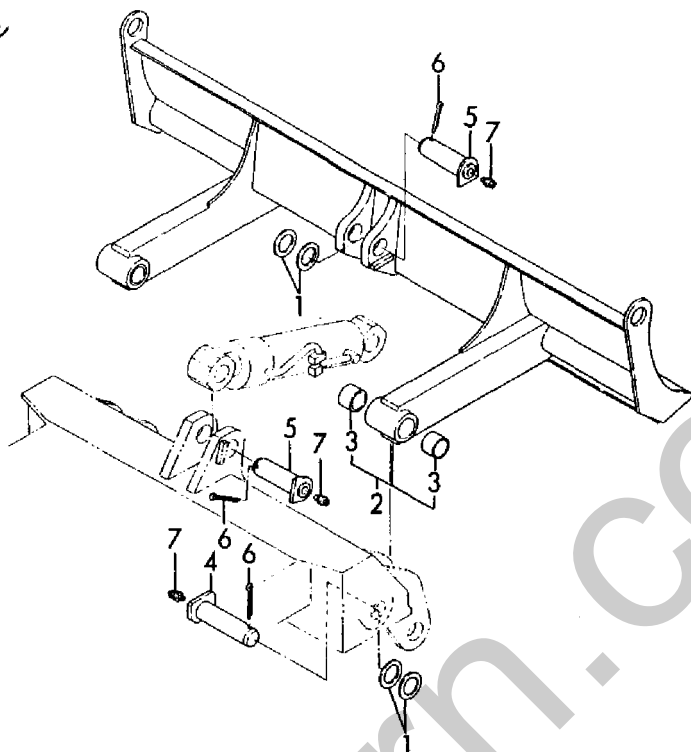
Fig. 104 ブレード BLADE
