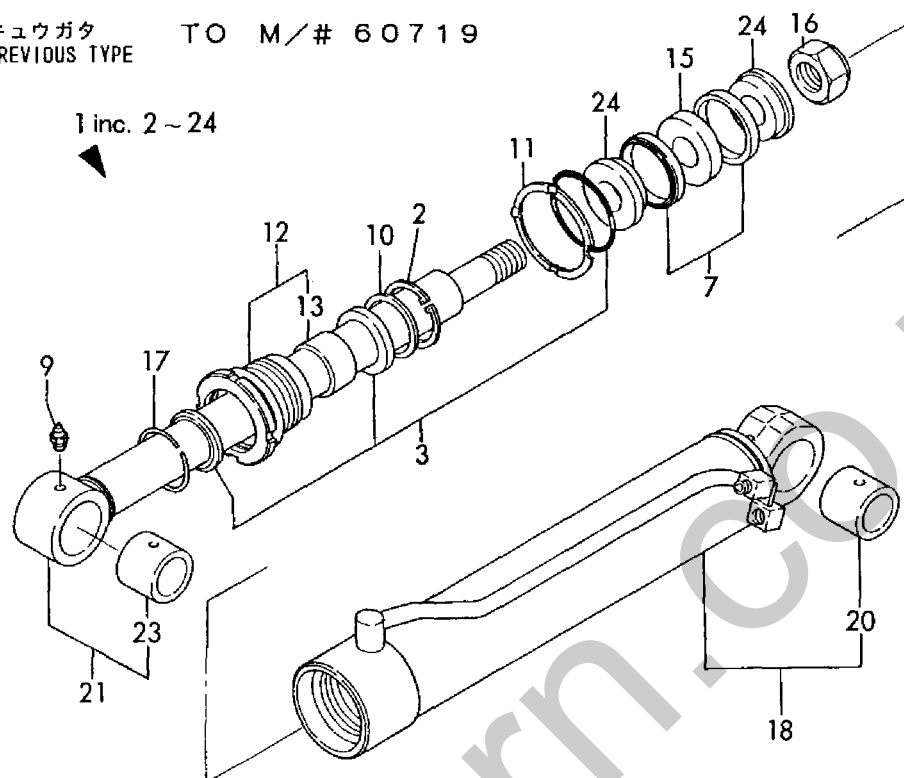
Fig. 71 スイングシリンダ SWING CYLINDER
