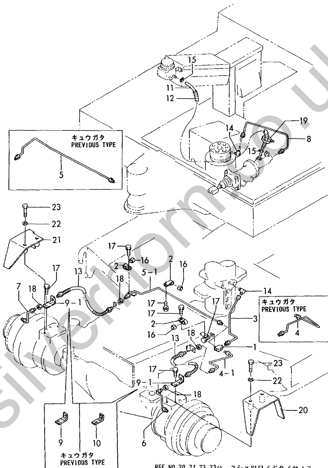
Fig. 98 ユアツハイカン(ブレーキ) HYD. OIL PIPING (BRAKE)
