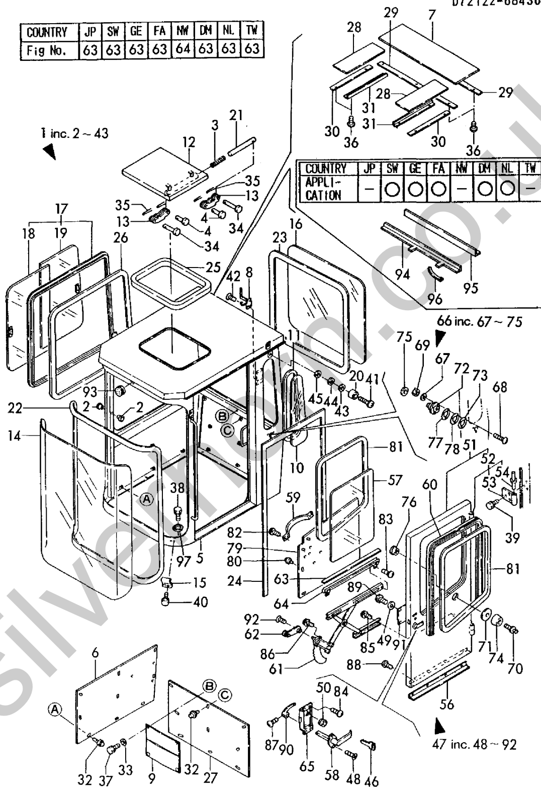
Fig. 63 キャビン CABIN
