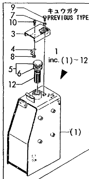
Fig. 14 F.O.タンク & F.O.パイプ FUEL TANK & FUEL LINE
