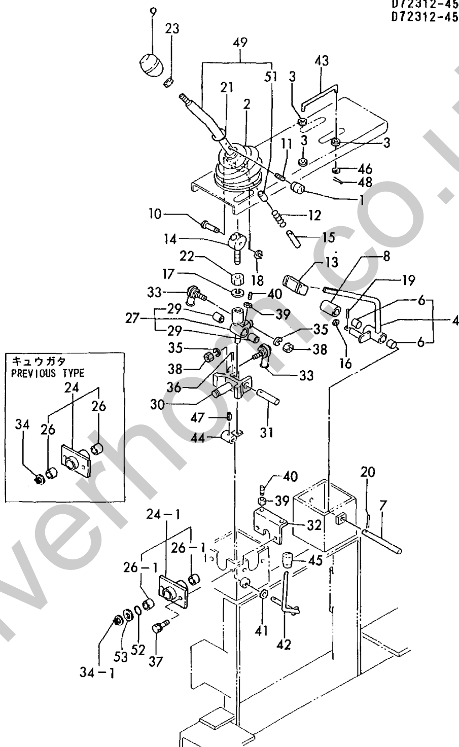
Fig. 41 ソウジュウソウチ(レバー L サイド)(ブレード) CONTROL EQUIPMENT (LEVER L SIDE) (BLADE)
