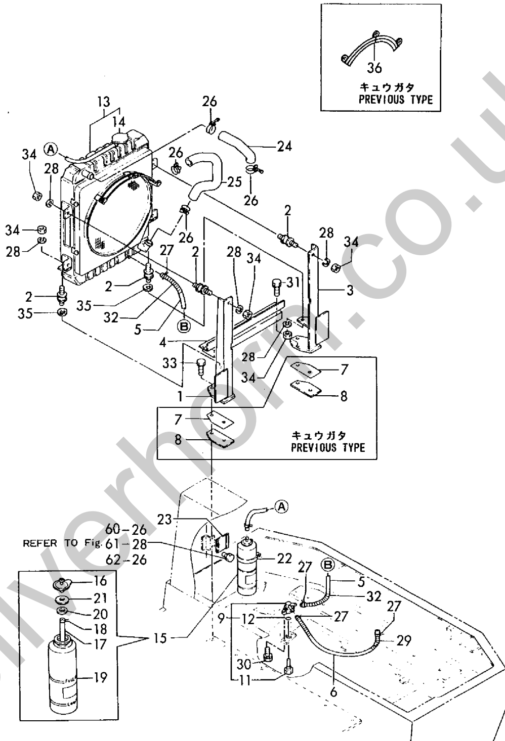
Fig. 13 ラジエータマウント RADIATOR MOUNT
