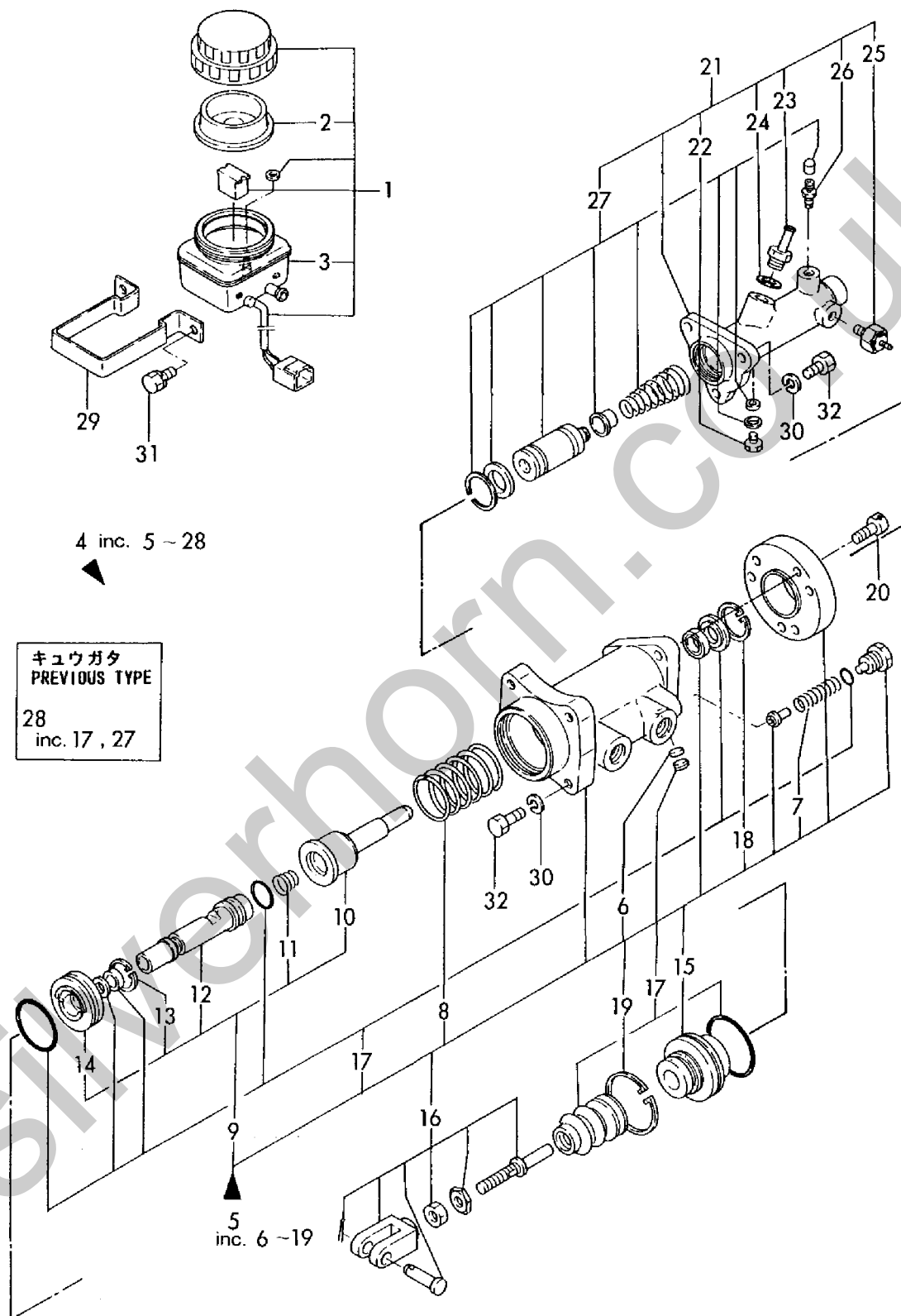
Fig. 100 ユアツキキブレーキ BRAKE HYD. UNIT
