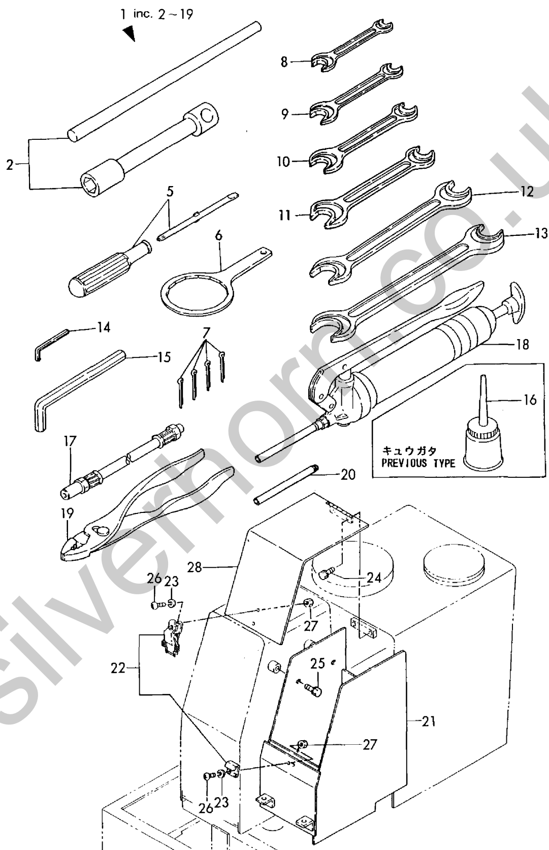
Fig. 9 コウグ & コウグバコ TOOL & TOOL BOX
