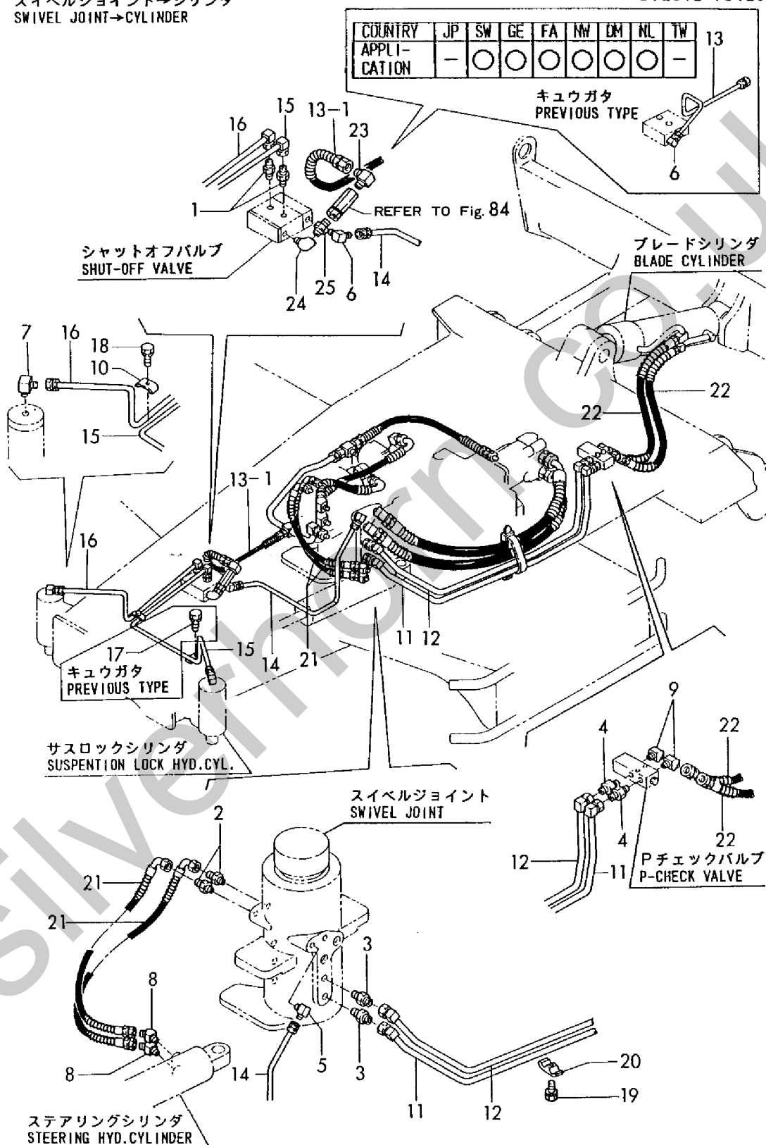
Fig. 96 ユアツハイカン(シャーシ 2)(ブレード) HYD.OIL PIPING (CHASSIS 2) (BLADE)
