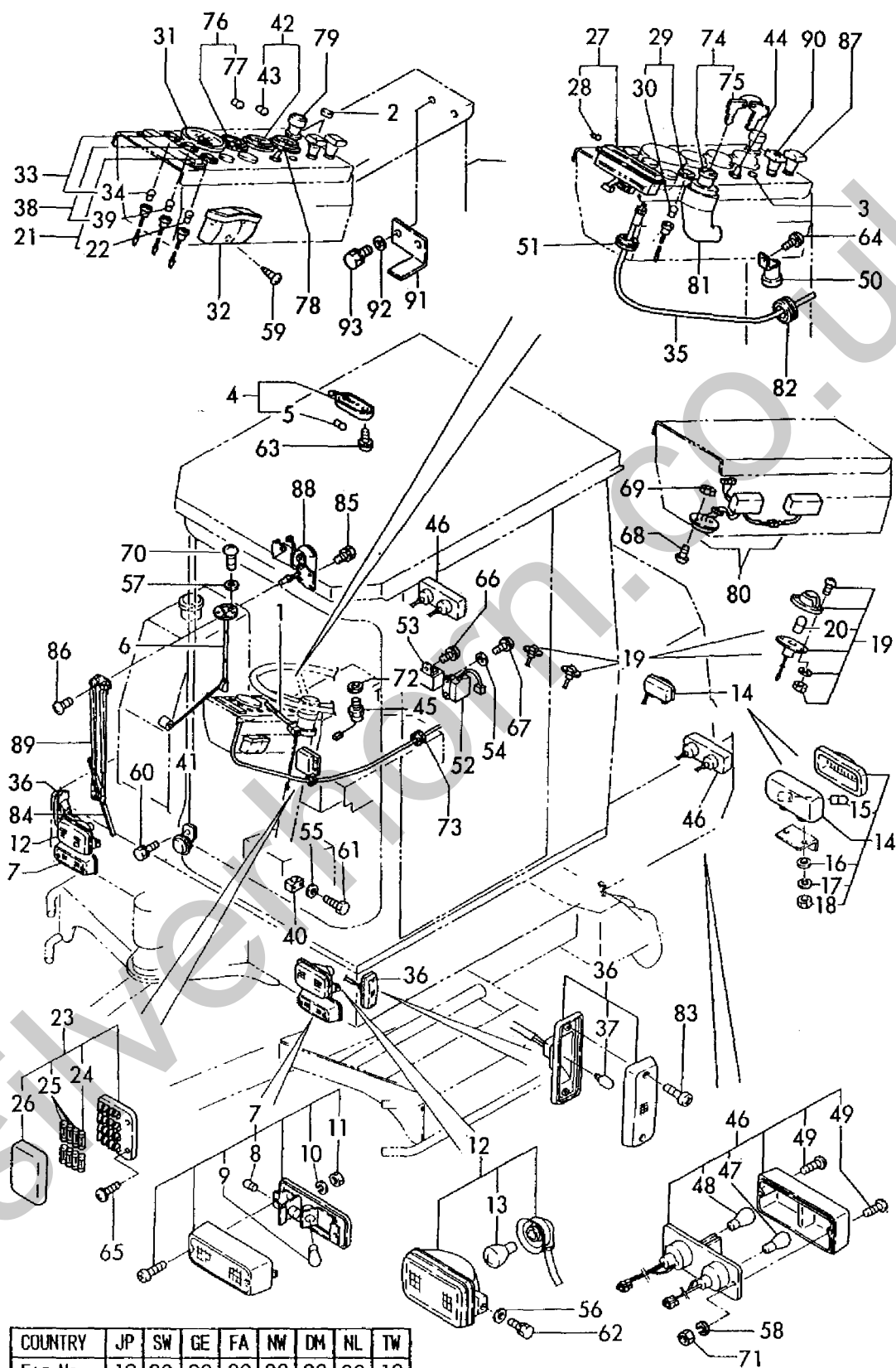
Fig. 19 デンキキキ(キャビン) ELECTRIC PARTS (CABIN)
