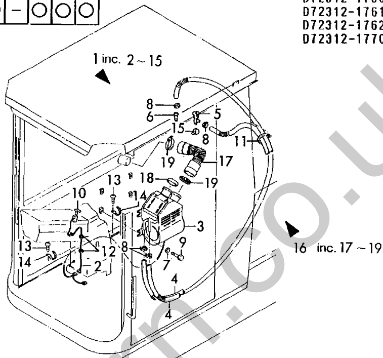
Fig. 23 ヒータ (33RD) & デフロスタ HEATER (33RD) & DEFROSTER
