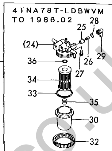
Fig. 14 F.O.タンク & F.O.パイプ FUEL TANK & FUEL LINE
