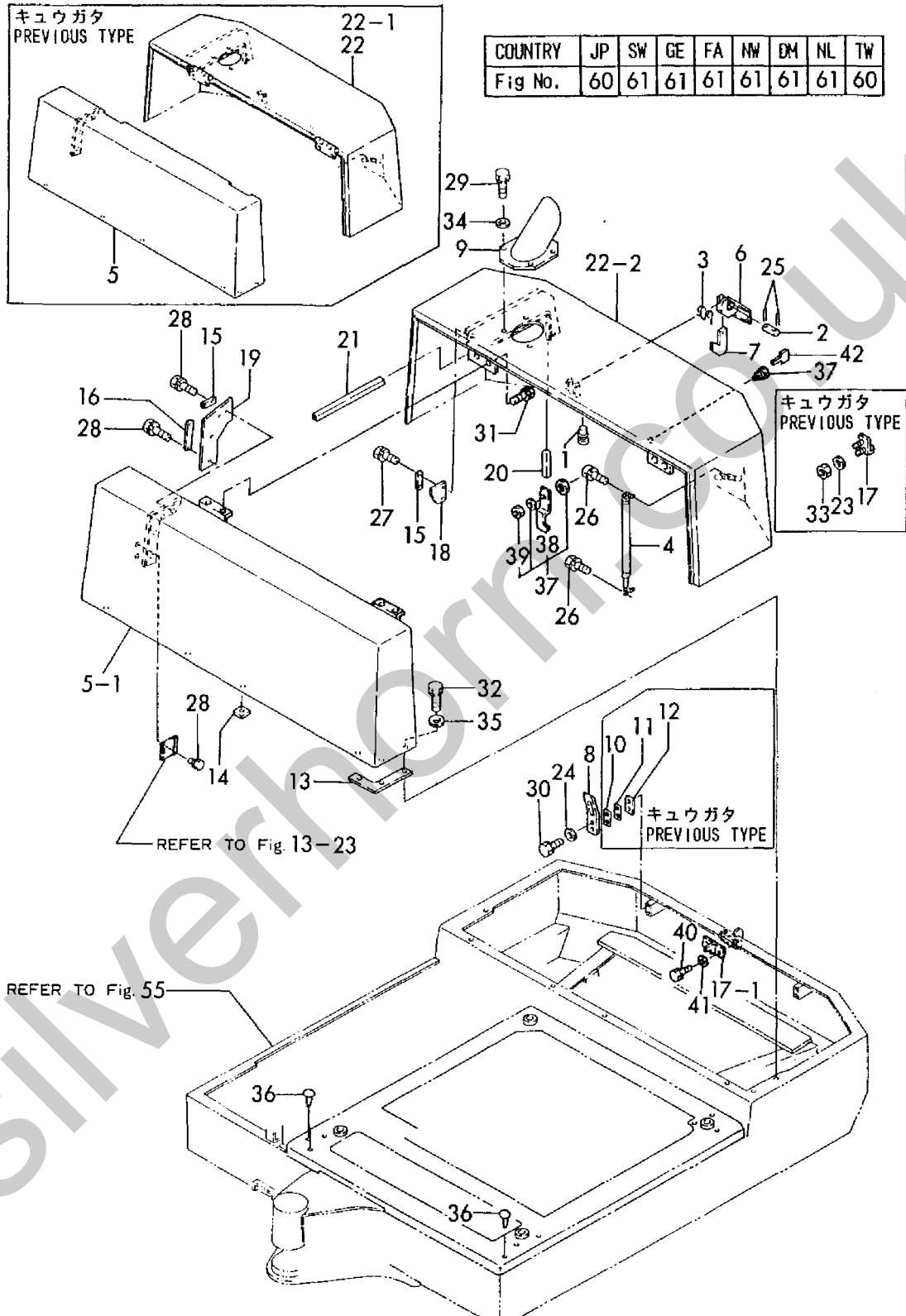
Fig. 61 ボンネット(キャビン) BONNET (CABIN)
