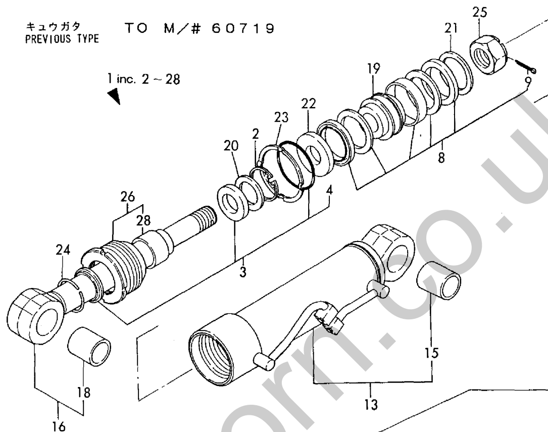
Fig. 73 ブレードシリンダ BLADE CYLINDER
