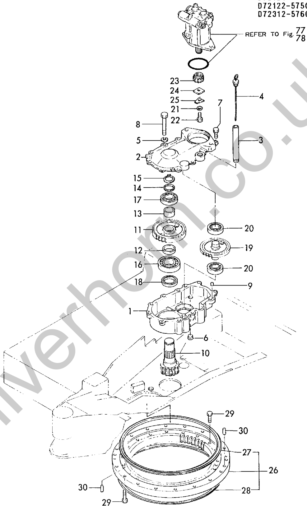
Fig. 56 センカイクドウソウチ TURNING DRIVING EQUIPMENT
