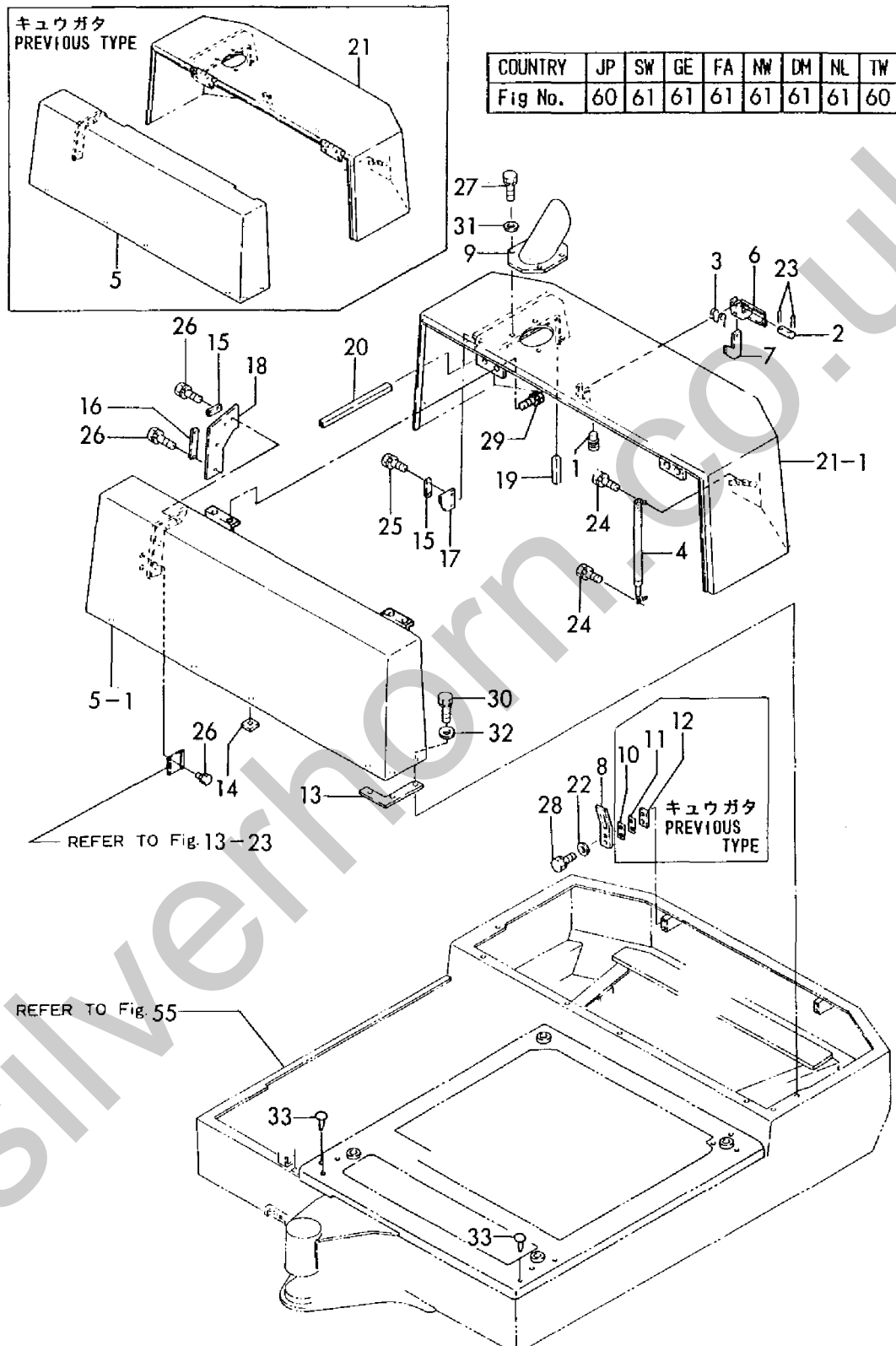
Fig. 60 ボンネット(キャビン) BONNET (CABIN)
