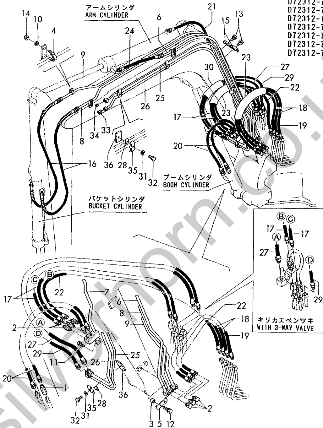
Fig. 87 ユアツハイカン(ブーム) HYD. OIL PIPING (BOOM)
