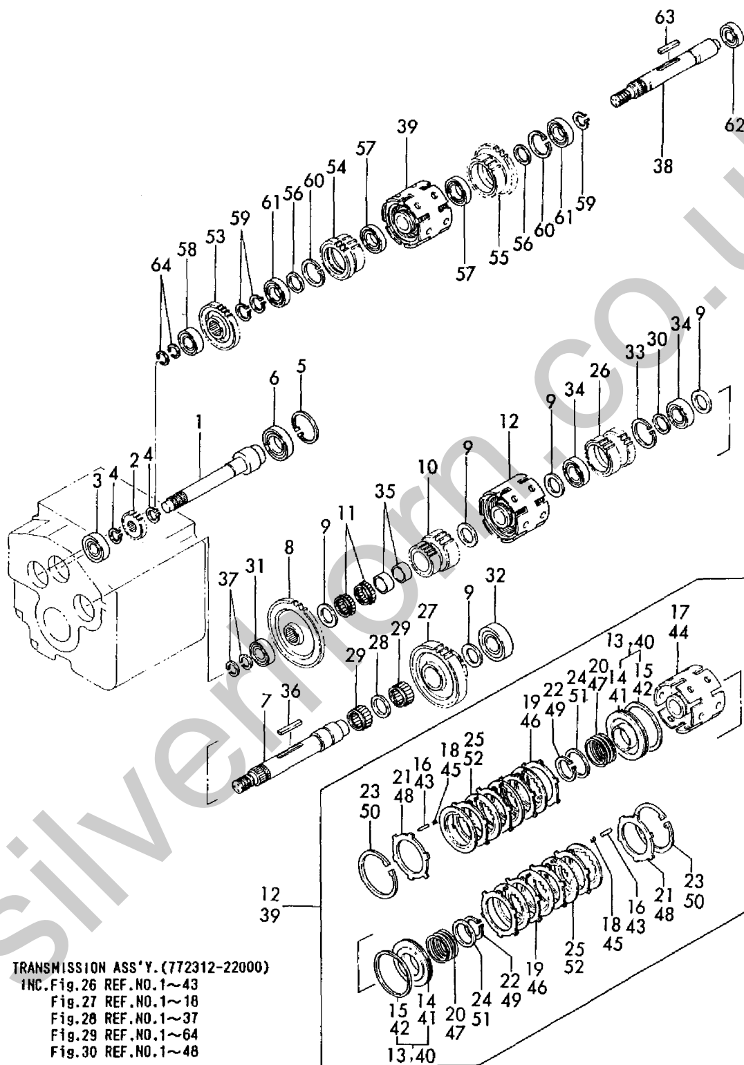
Fig. 29 ミッション1ジク & 2ジク TRANSMISSION 1ST & 2ND SHAFT
