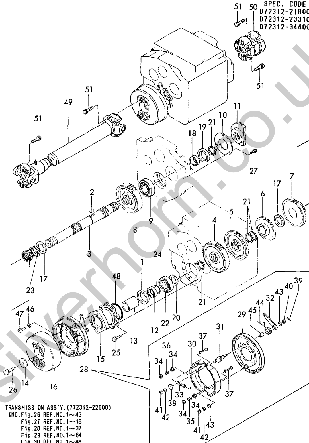
Fig. 30 3 ジク, センタブレーキ & ドライブシャフト 3RD SHAFT, CENTER BRAKE
