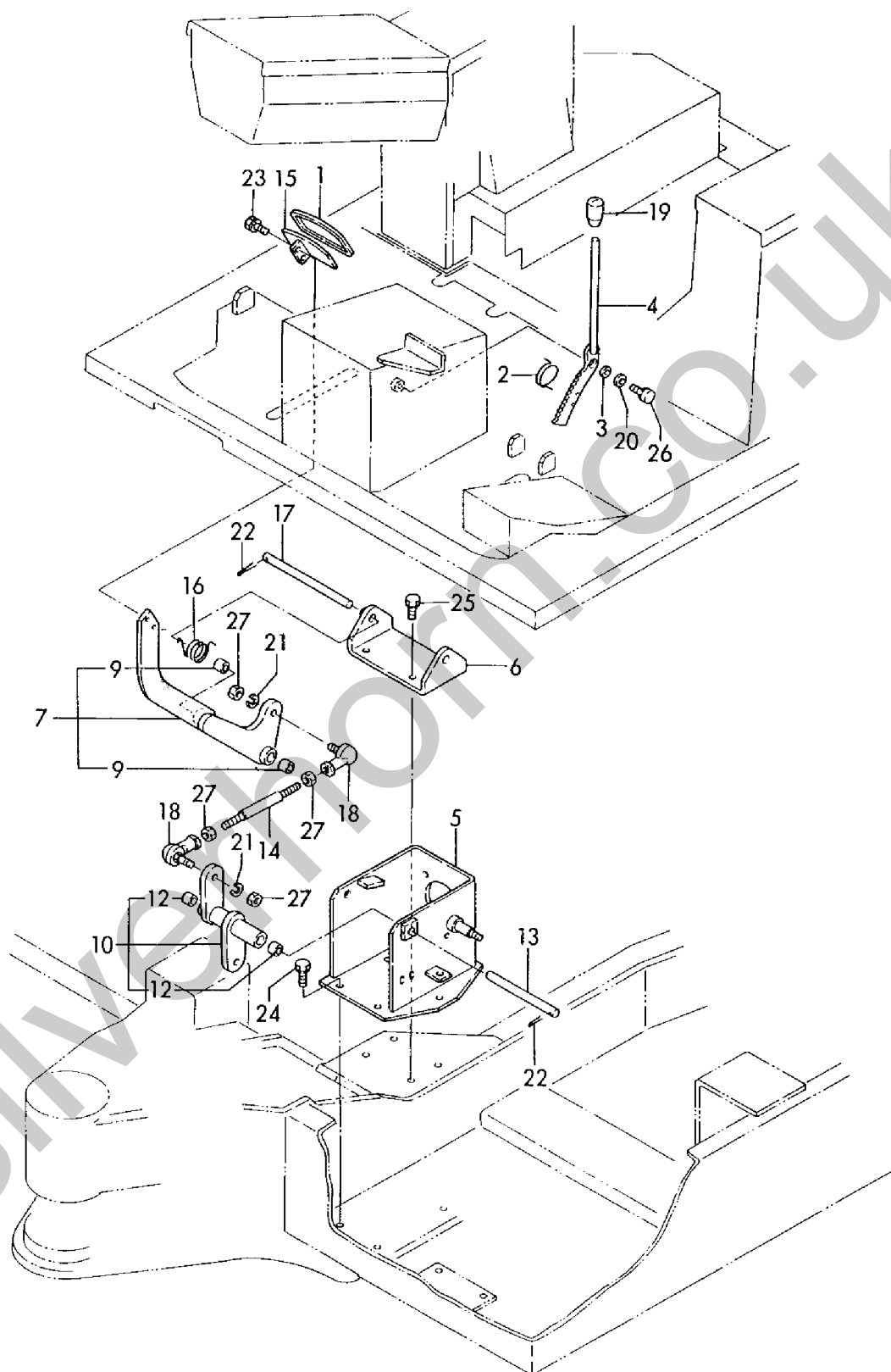
Fig. 47 ペダル・リンケージ(ブレーキ) PEDAL & LINKAGE (BRAKE)
