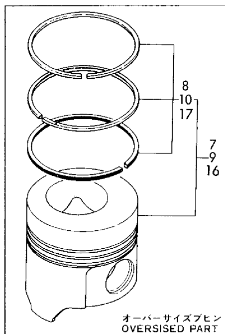
Fig. 12 ピストン&コネクティングロッド PISTON & CONNECTING ROD
