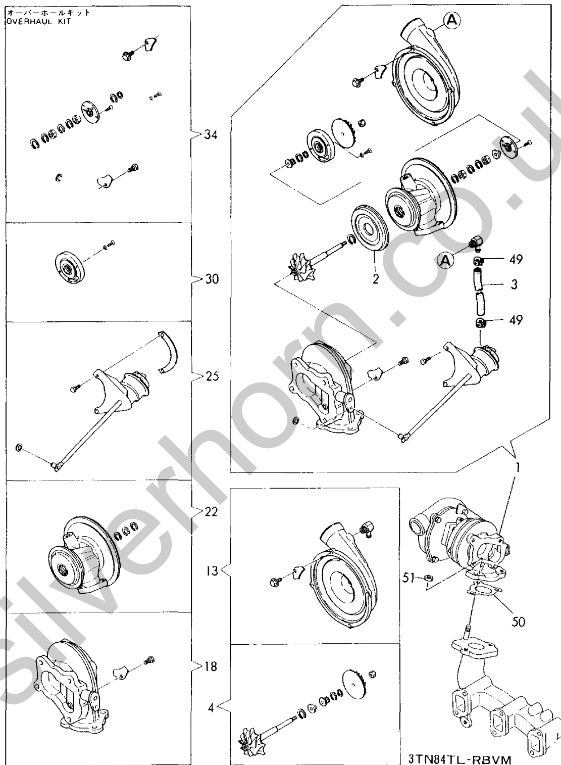
Fig. 10 タービン(インナーパーツ) TURBOCHARGER (COMPONENT PARTS)
