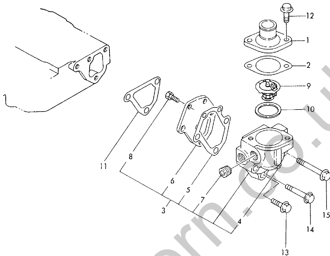
Fig. 17 サーモスタット THERMOSTAT
