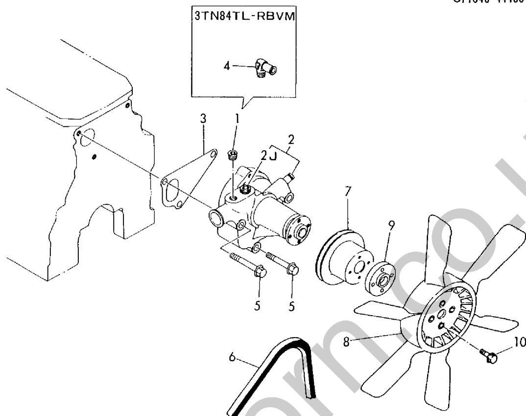
Fig. 16 CWシステム COOLING WATER SYSTEM
