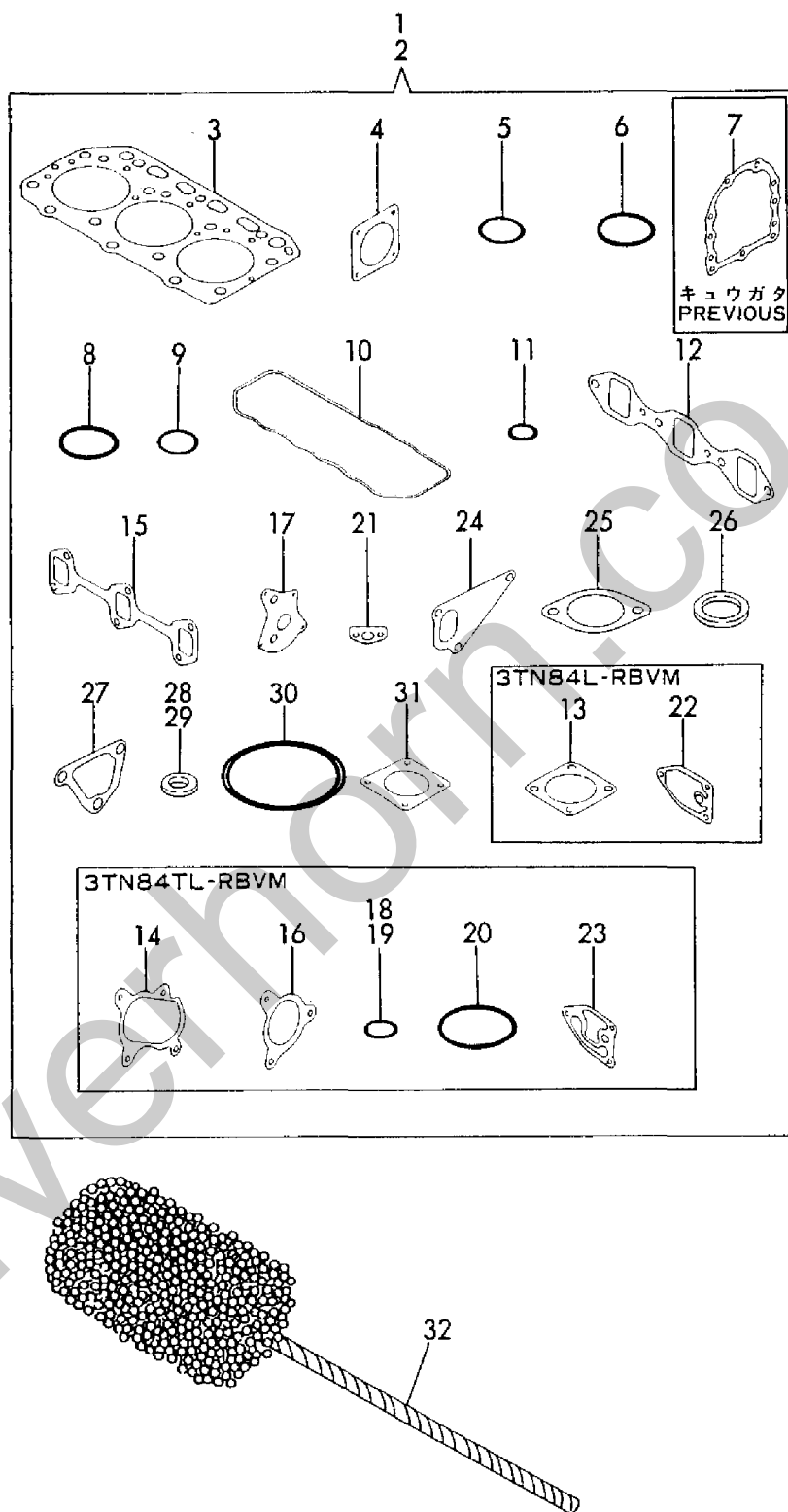
Fig. 28 パッキンセット&トクシュコウグ(オプション) GASKET SET & SPECIAL TOOL (OPTIONAL)
