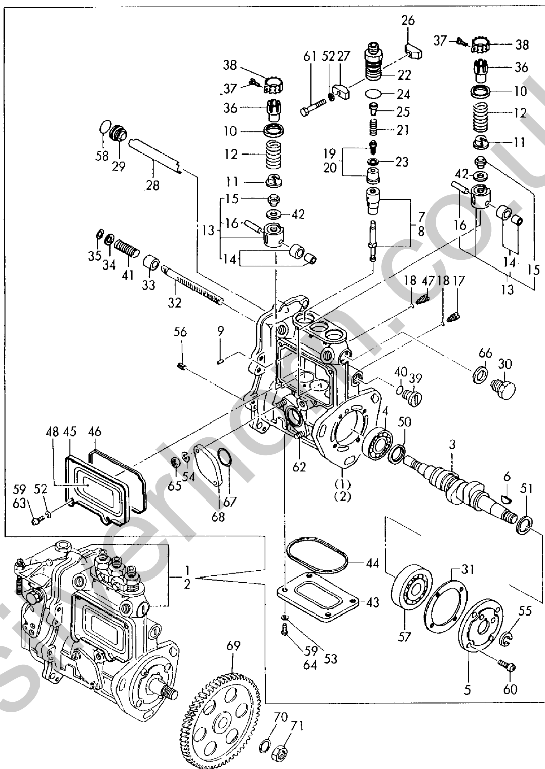
Fig. 19 FOフンシャポンプ FUEL INJECTION PUMP
