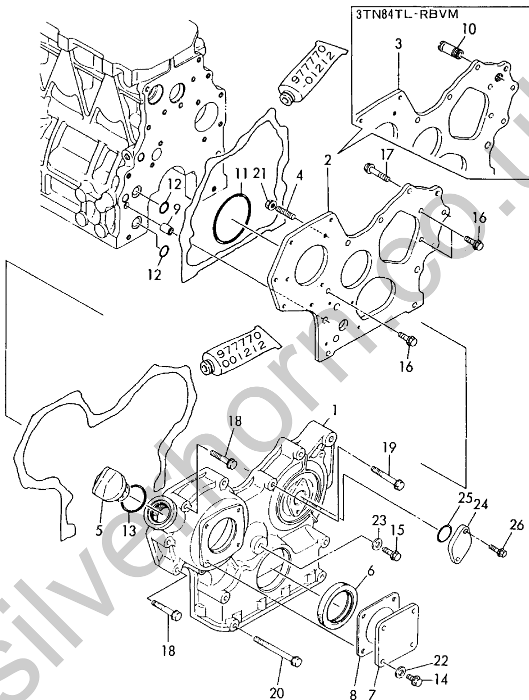
Fig. 2 ギヤケース GEAR HOUSING
