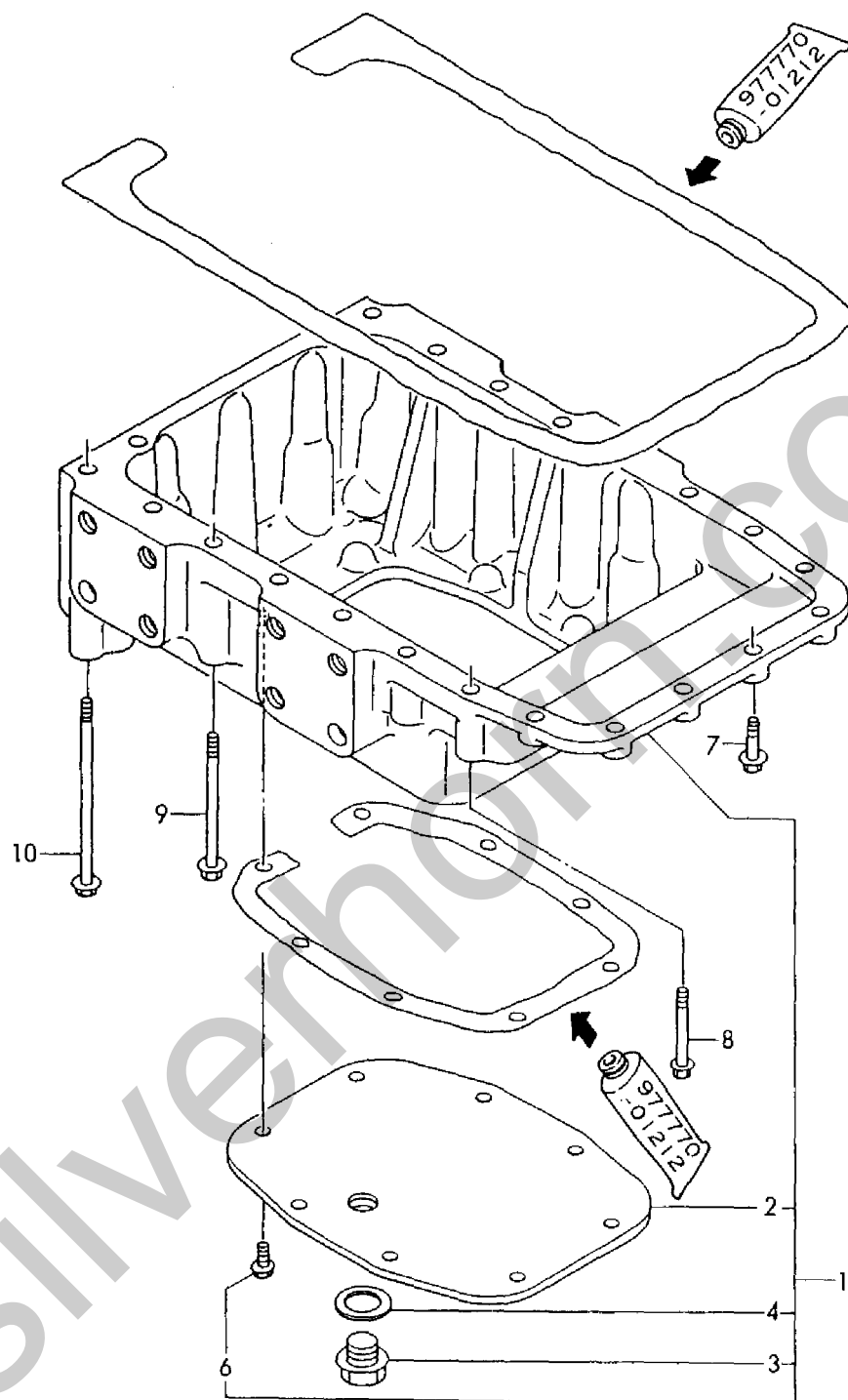
Fig. 4 オイルパン LUB. OIL SUMP
