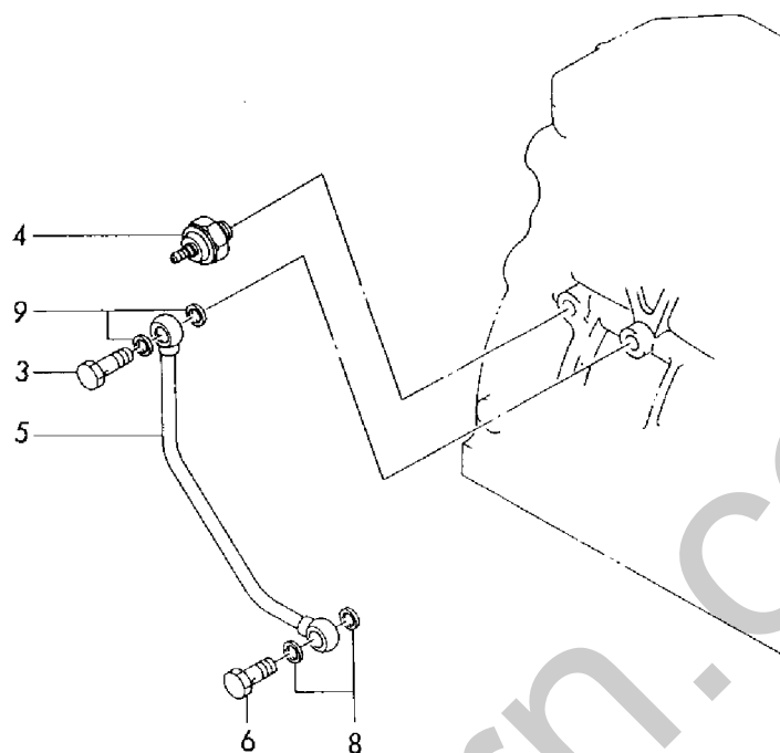
Fig. 14 LOパイプ LUB. OIL LINE
