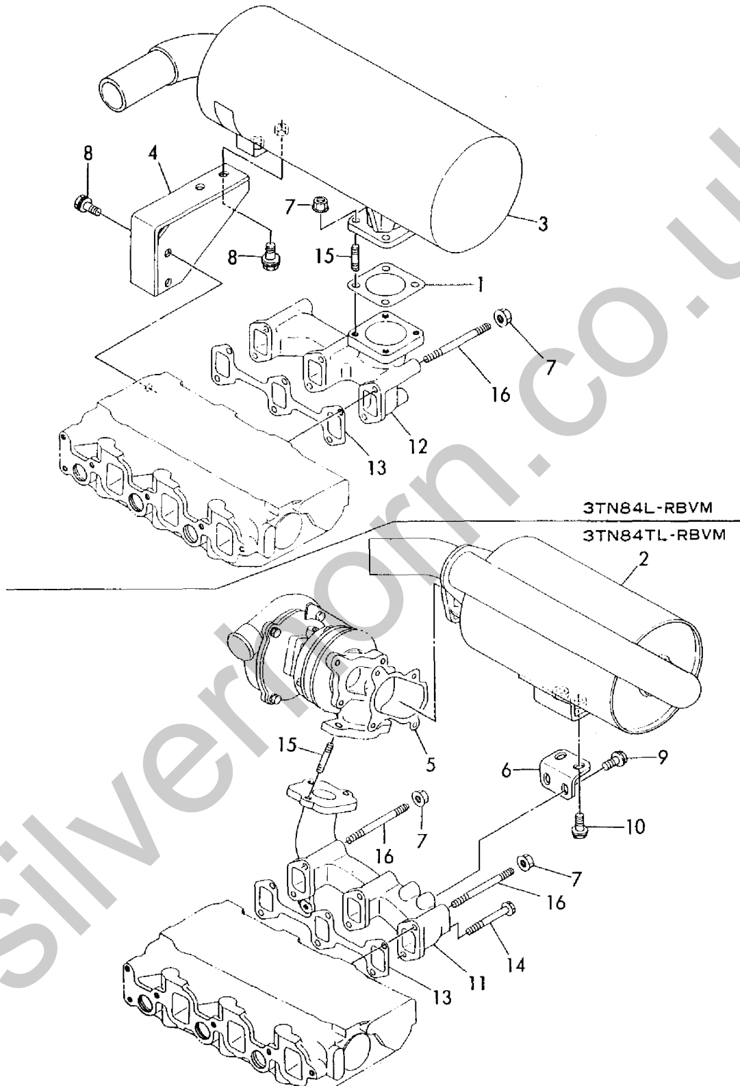
Fig. 8 ハイキマニホールド&サイレンサ EXH. MANIFOLD & SILENCER
