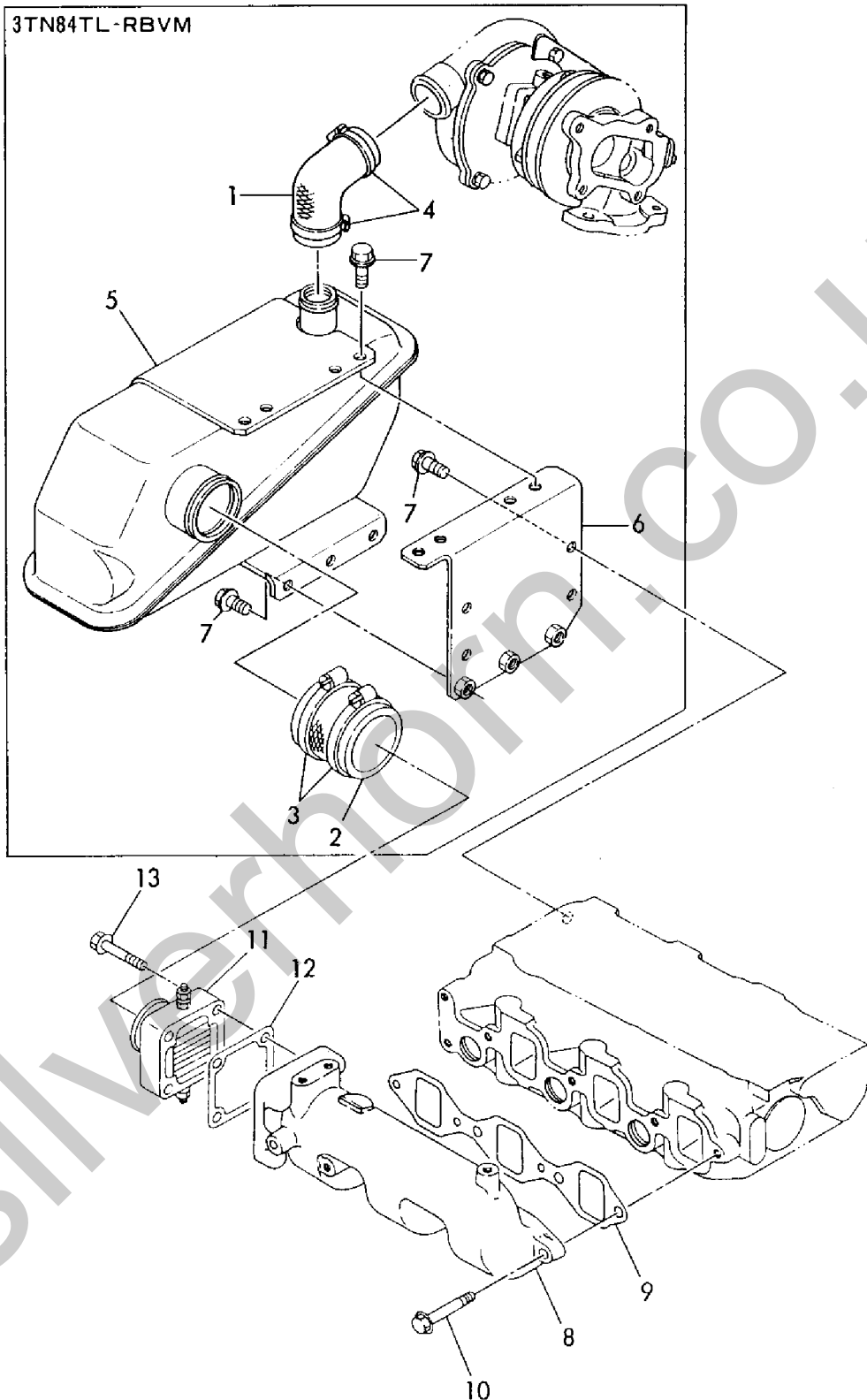
Fig. 7 キュウキマニホールド SUCTION MANIFOLD
