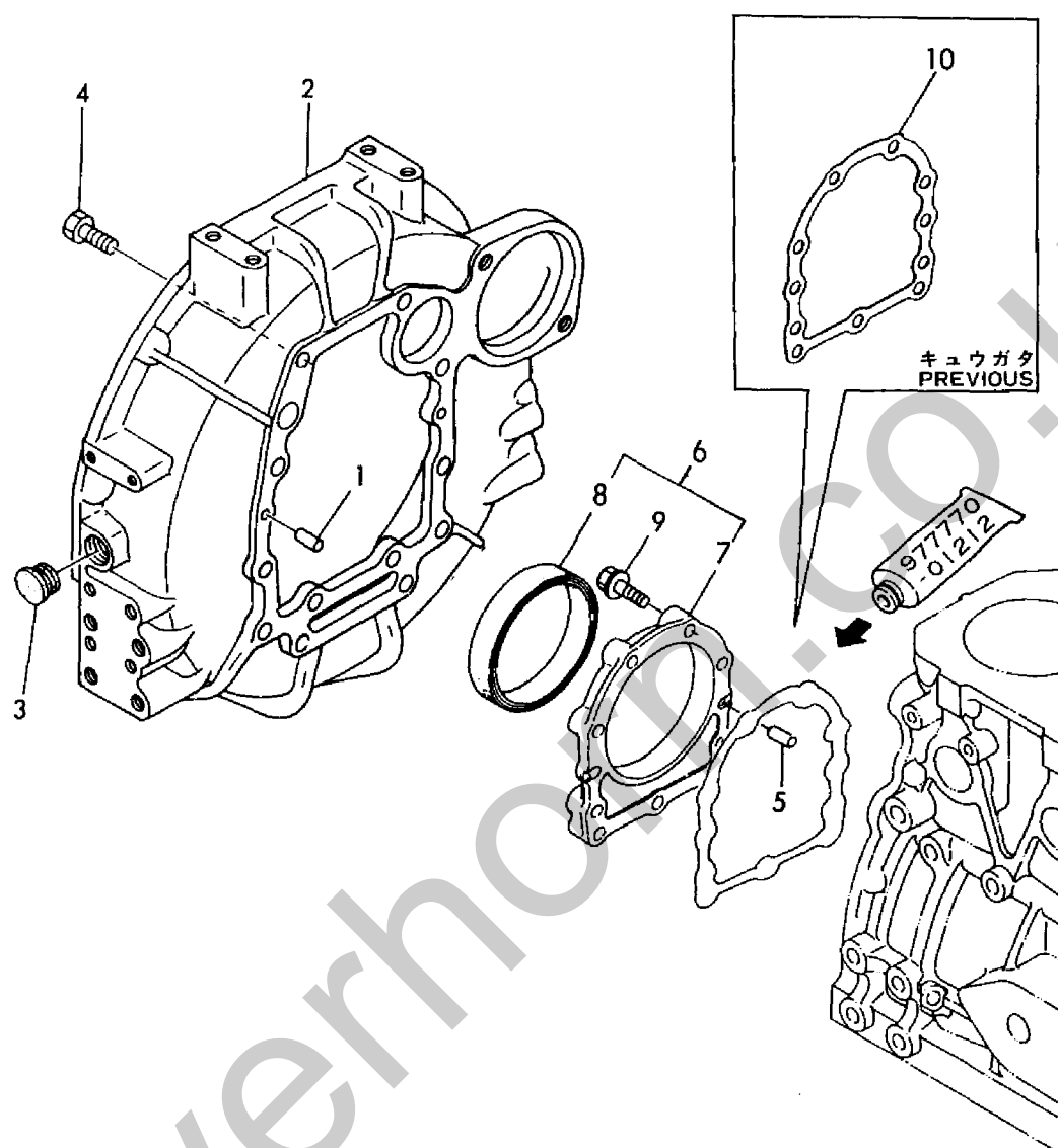
Fig. 3 フライホイールハウジング FLYWHEEL HOUSING
