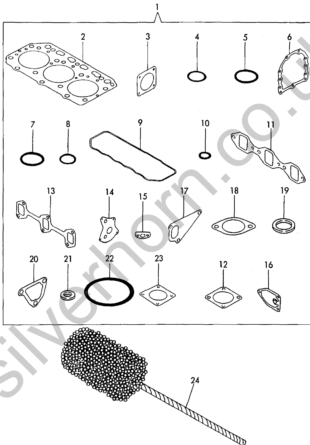
Fig. 23 パッキンセット & トクシュコウゲ (オプション) GASKET SET & SPECIAL TOOL (OPTIONAL)
