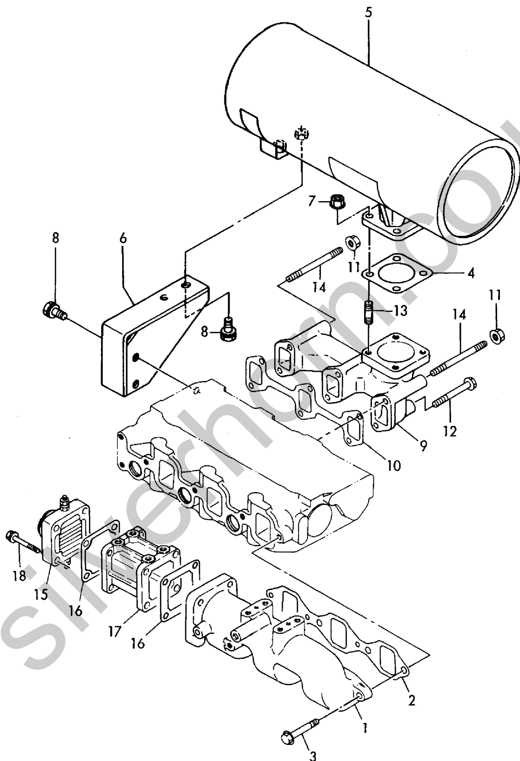
Fig. 7 キュウハイキマニホールド SUCTION & EXHAUST MANIFOLD
