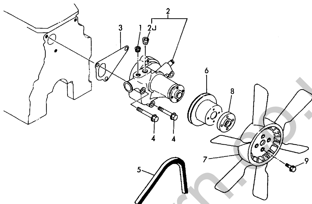
Fig. 13 CWシステム COOLING WATER SYSTEM
