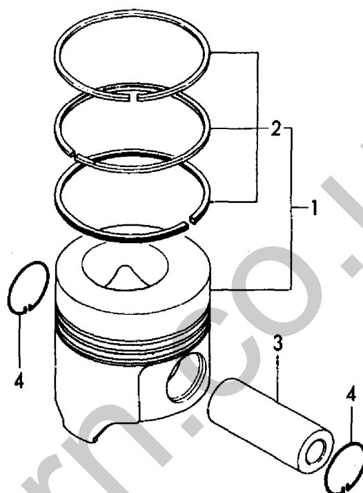
Fig. 10 ピストン&コネクティングロッド PISTON & CONNECTING ROD
