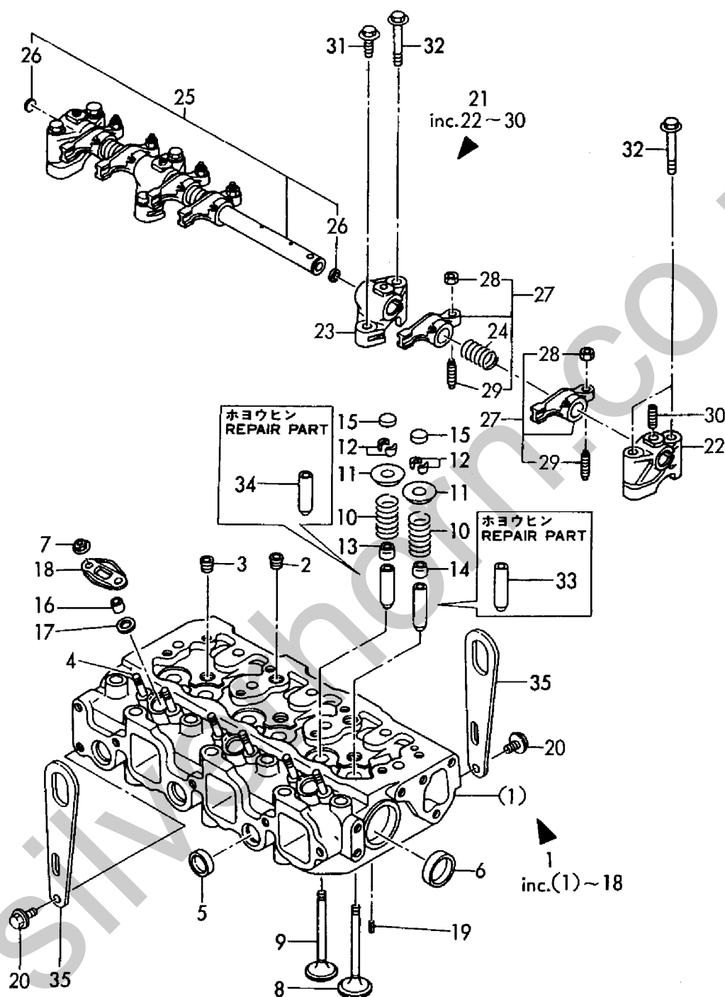
Fig. 6 シリンダヘッド CYLINDER HEAD
