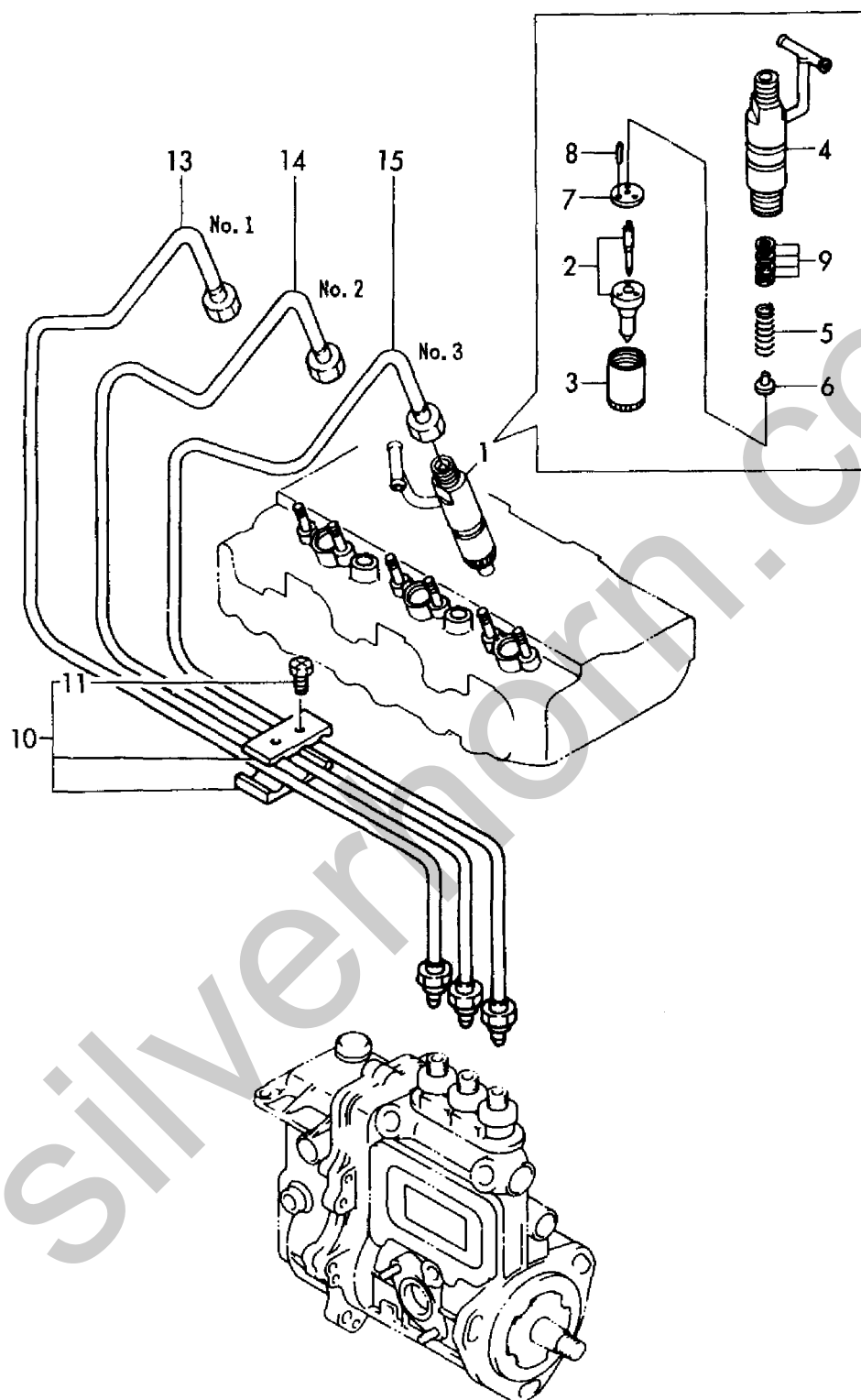
Fig. 17 FOフンシャパイプ FUEL INJECTION LINE
