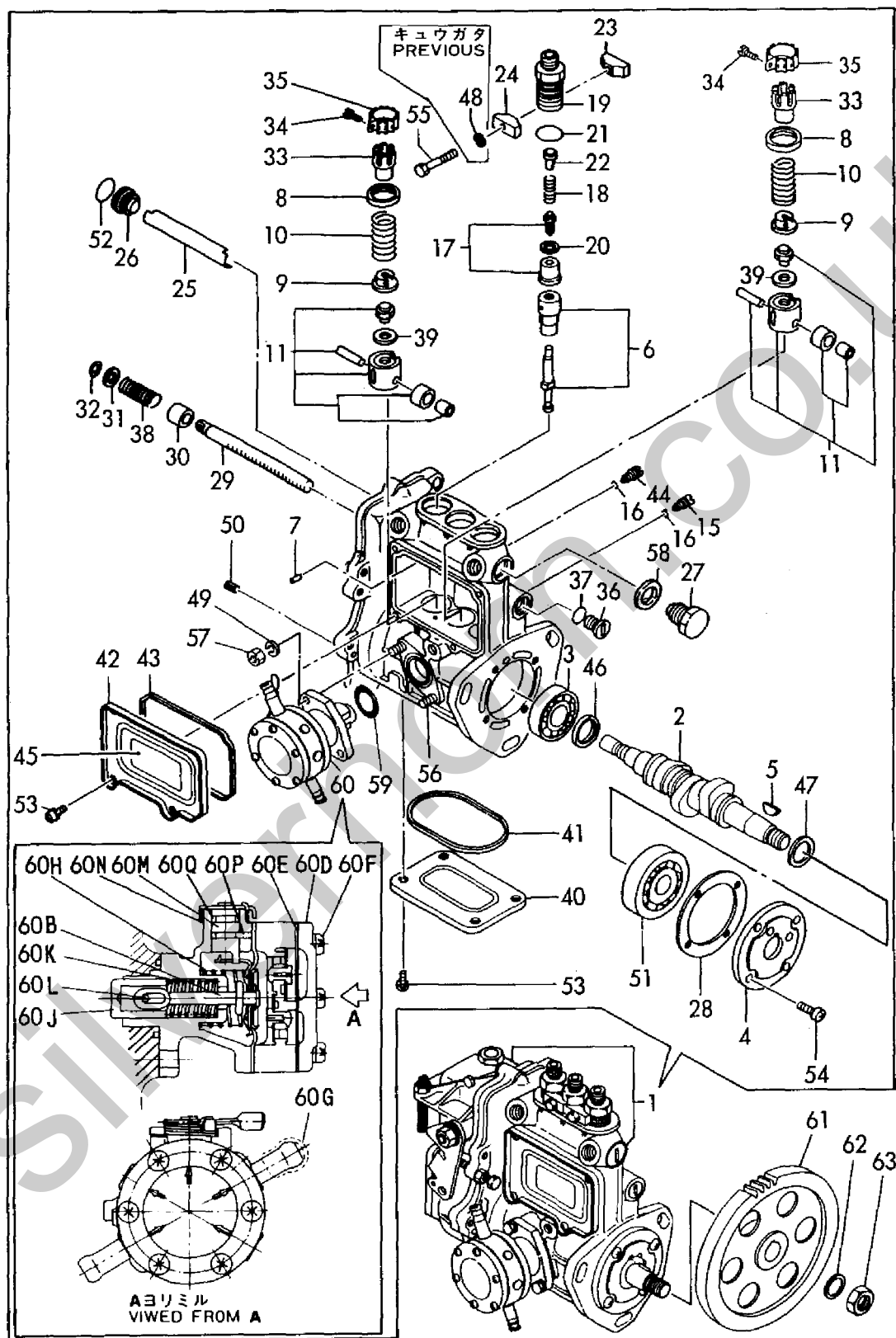
Fig. 16 FOファンシャポンプ FUEL INJECTION PUMP
