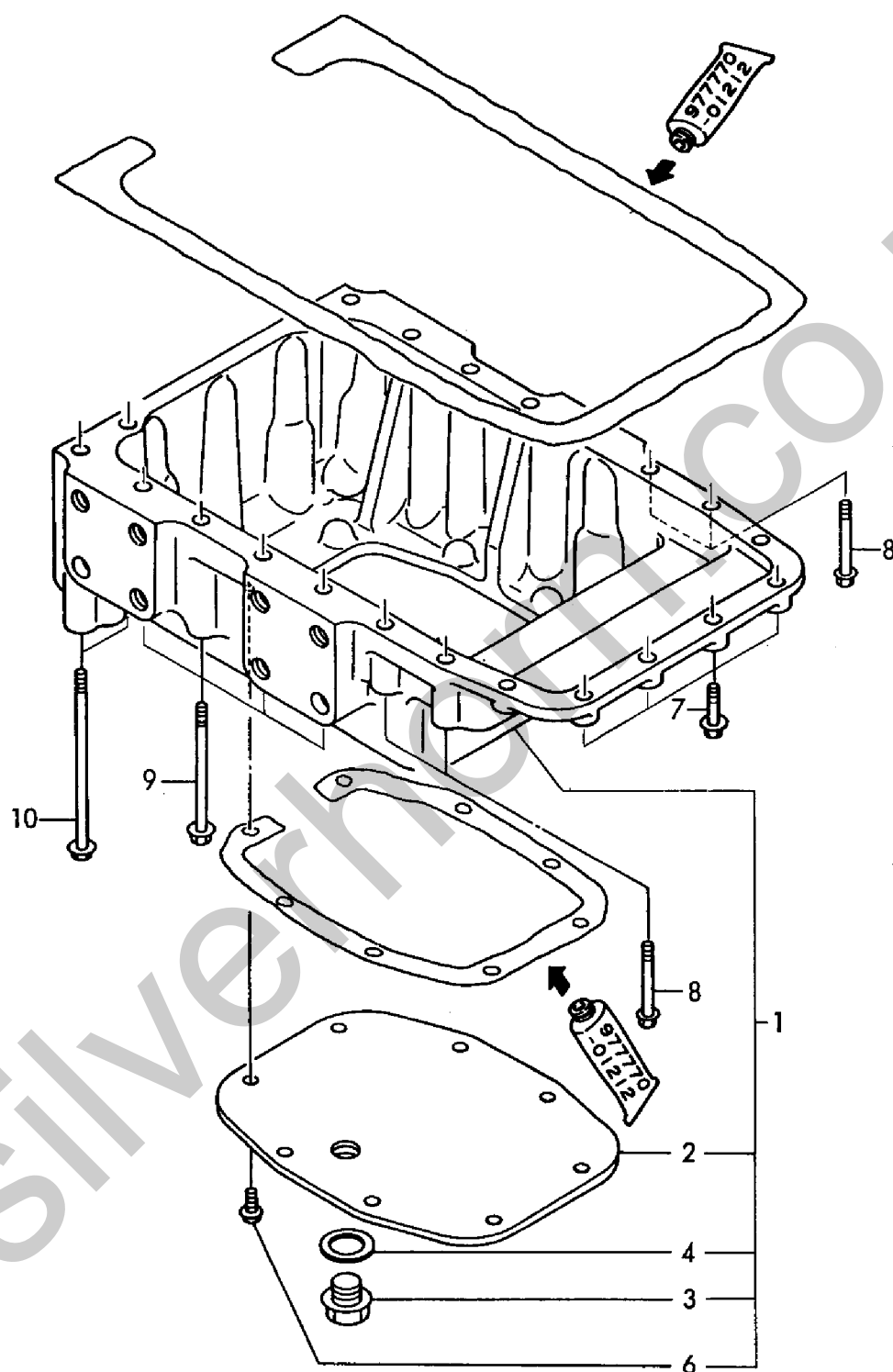
Fig. 4 オイルパン LUB. OIL SUMP
