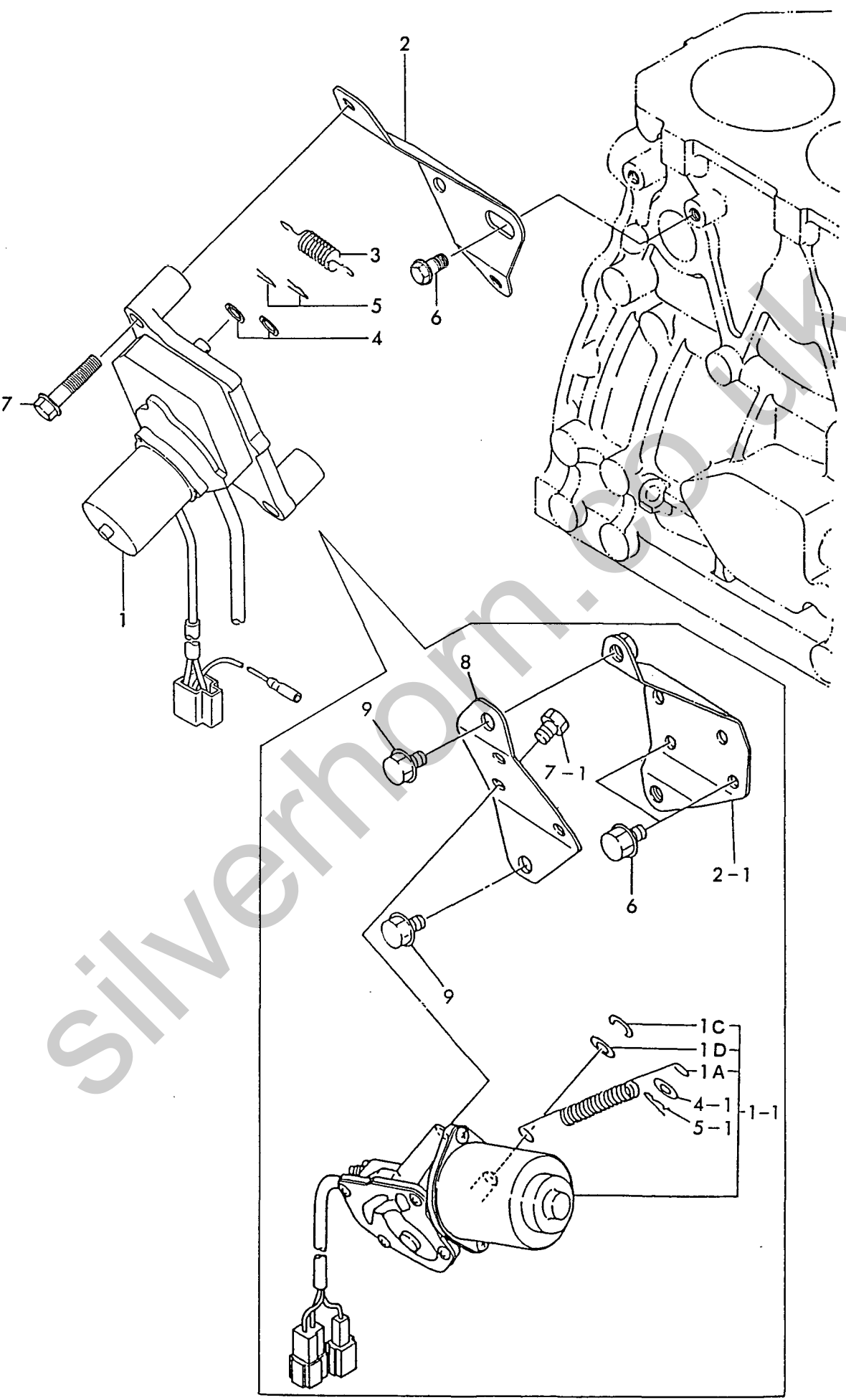
Fig. 18 キカンテイシソウチ ENGINE STOP DEVICE
