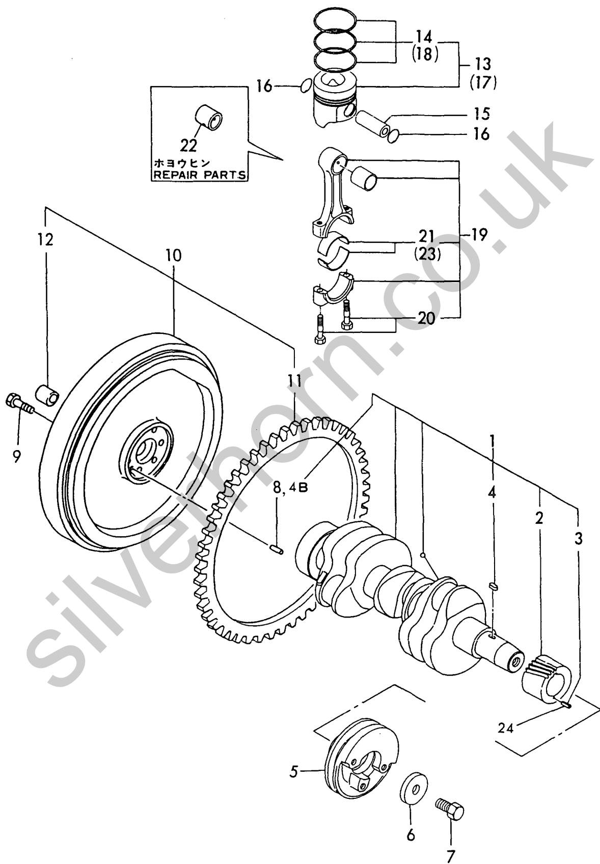
Fig. 9 クランクシャフト & ピストン CRANKSHAFT & PISTON
