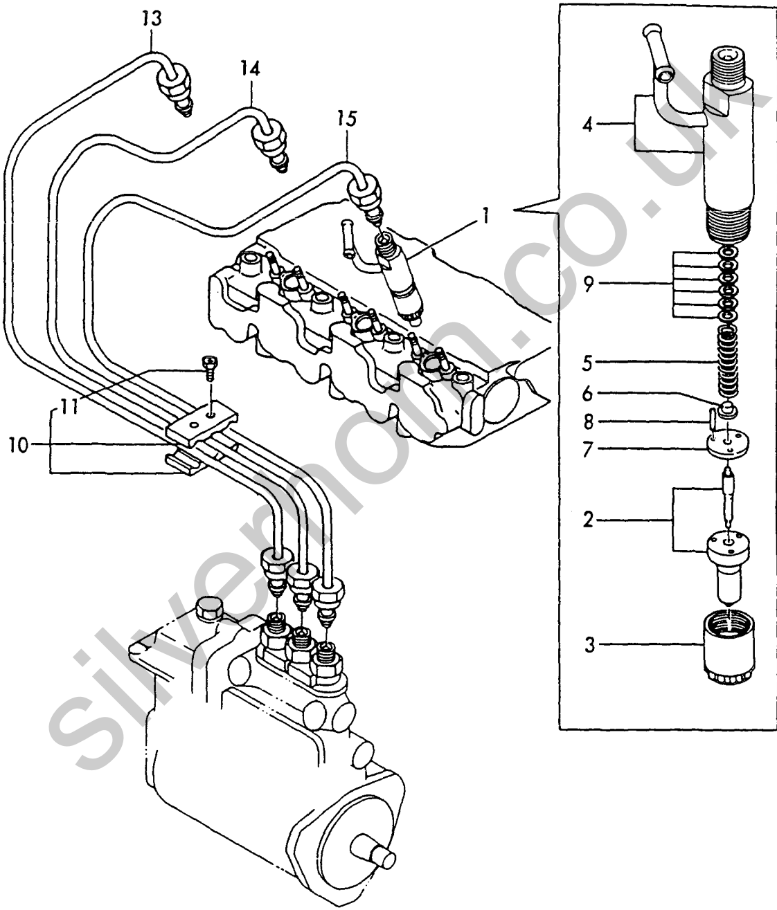
Fig. 15 FOフンシャパイプ FUEL INJECTION LINE
