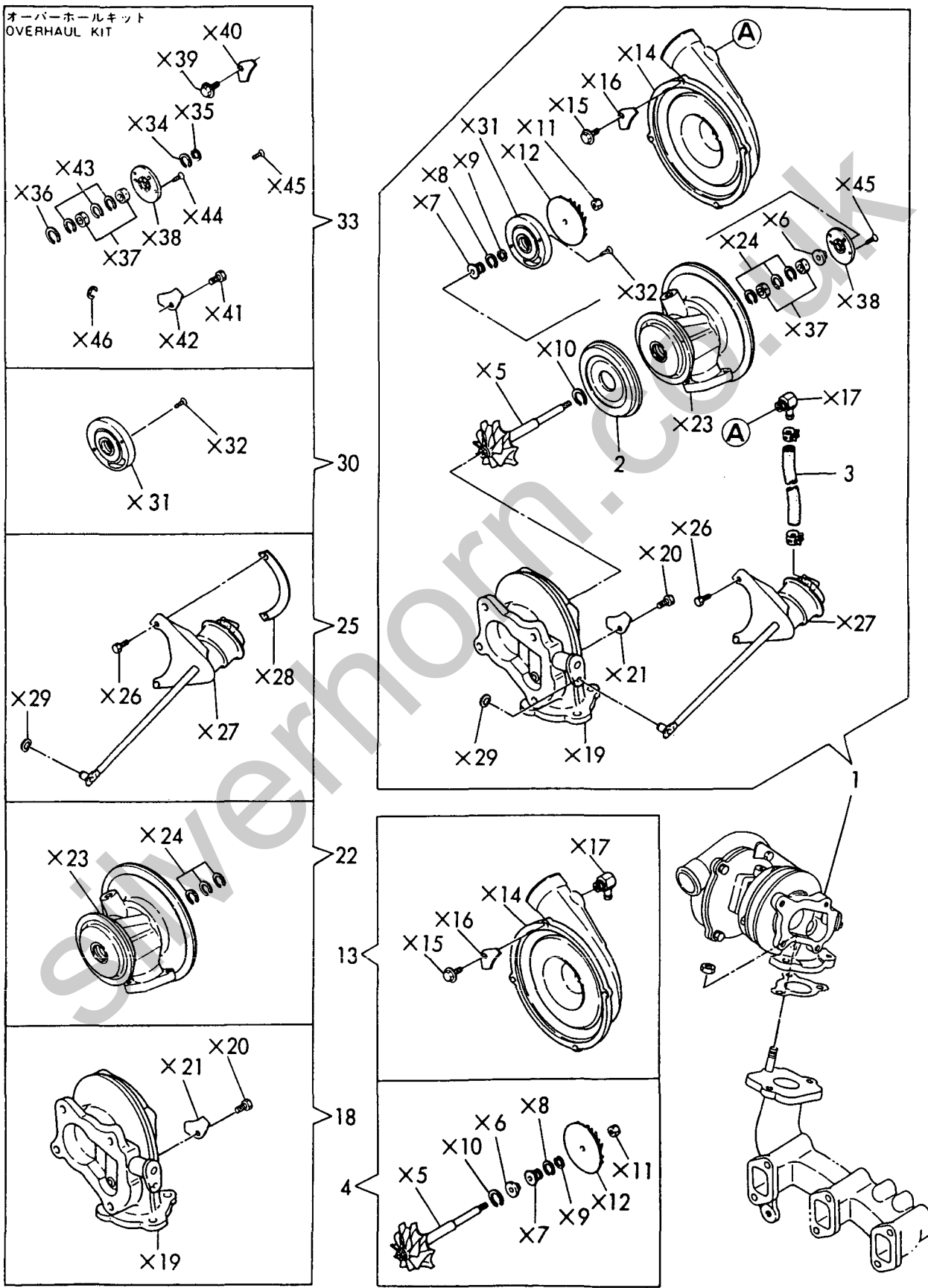
8 タービン(インナーパーツ) Fig. 8 TURBOCHARGER (COMPONENT PARTS)
