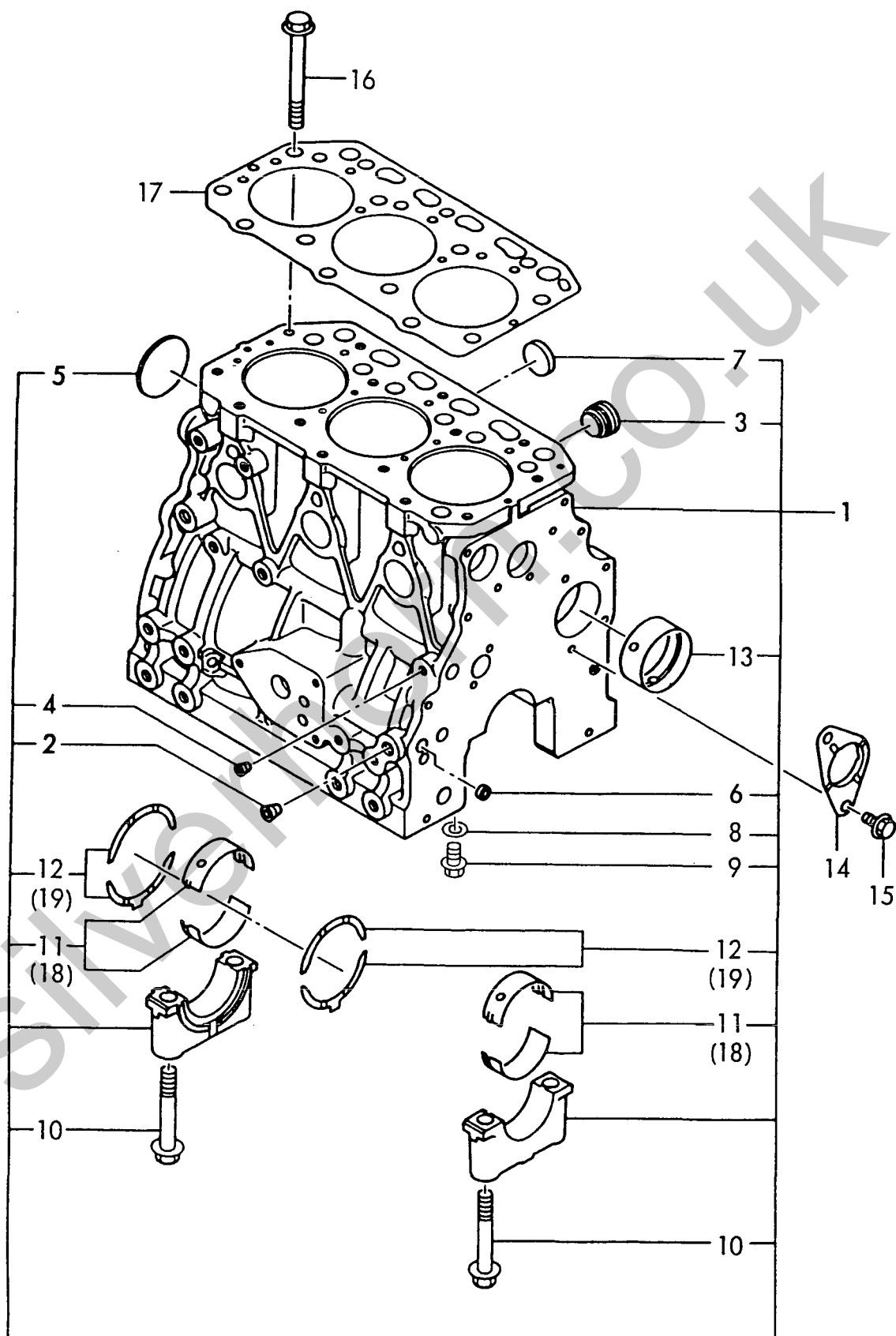
Fig. 1 シリンダブロック CYLINDER BLOCK
