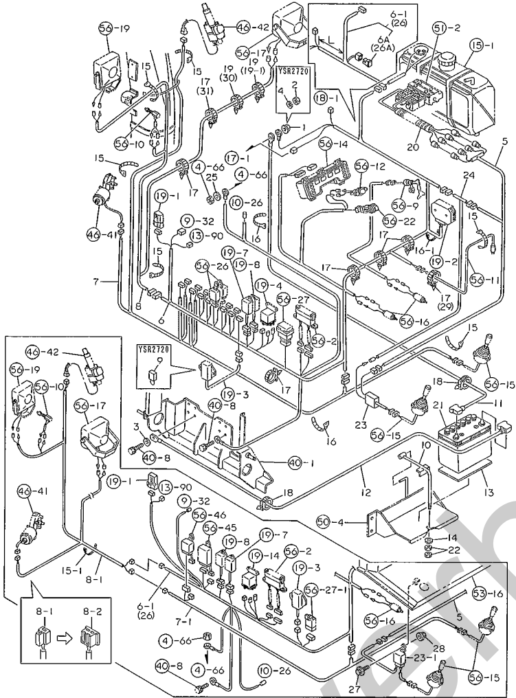
Fig.57. ELECTRICAL PARTS
