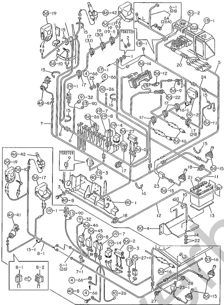
Fig.57. ELECTRICAL PARTS
