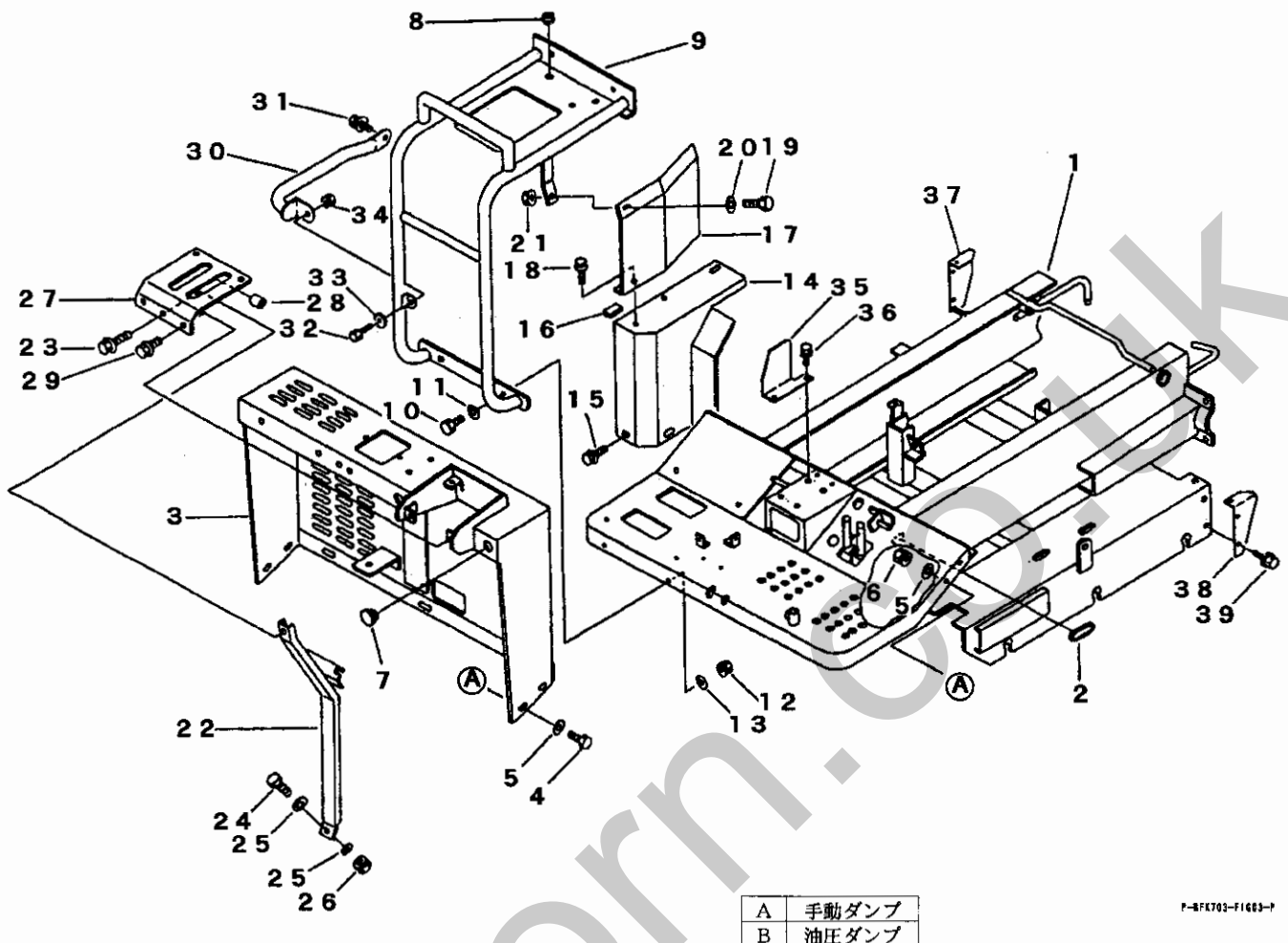
FIG 3 フレーム FRAME (ガソリン)
