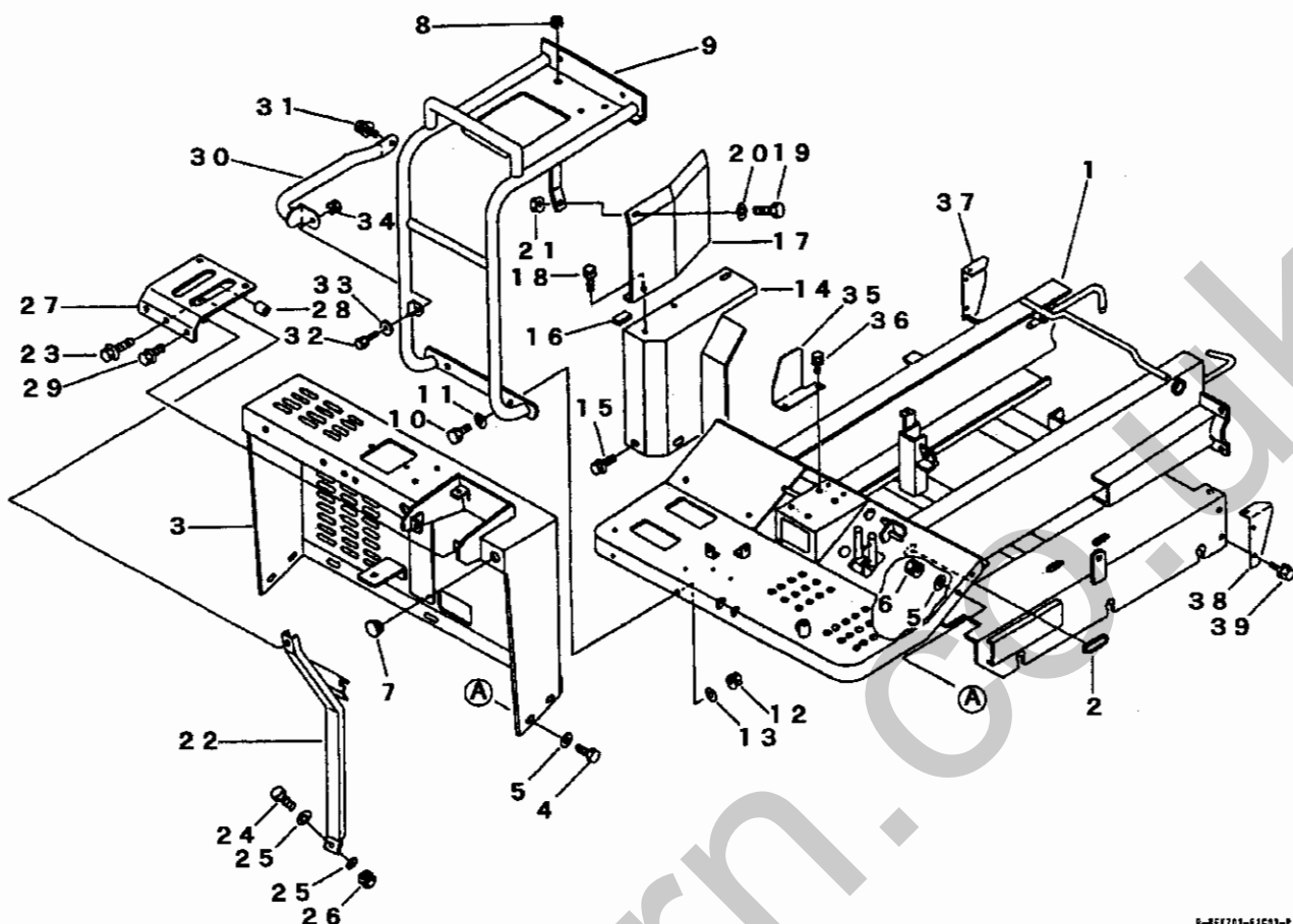
FIG 3 フレーム FRAME (ガソリン)
