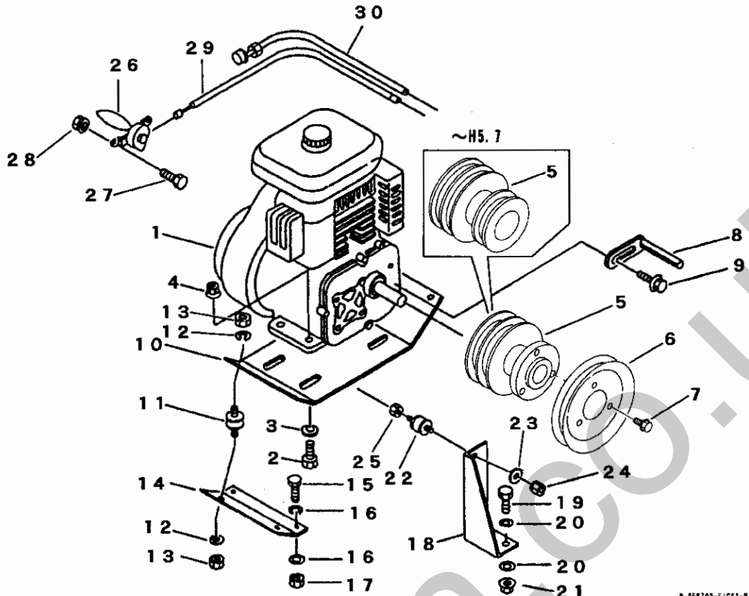
FIG 1 エンジン ENGINE (ガソリン)
