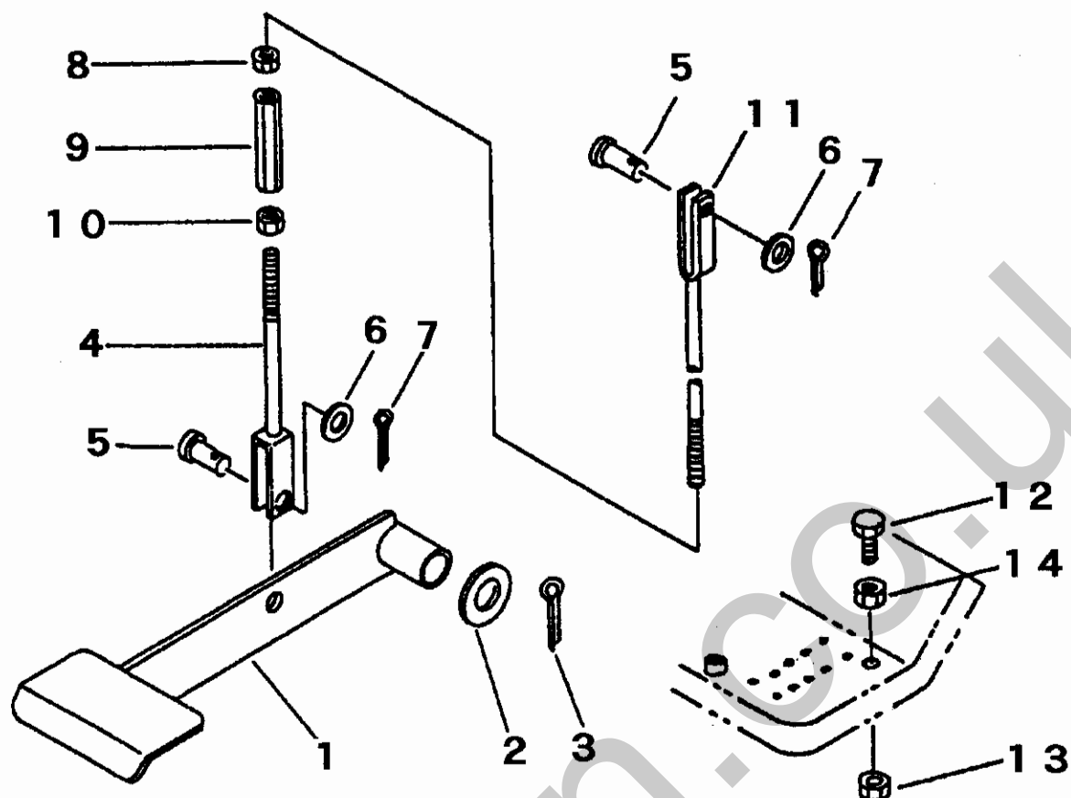
FIG 14 アンゼンソウチ DEADMAN'S CONTOROL BREAK
