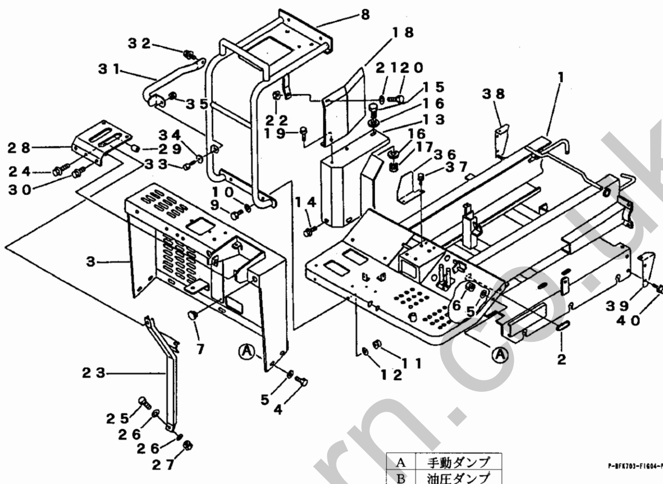
FIG 4 フレーム FRAME (ディーゼル)
