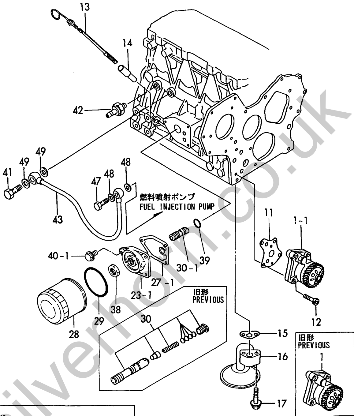
Fig. 9 潤滑油システム LUB. OIL SYSTEM
