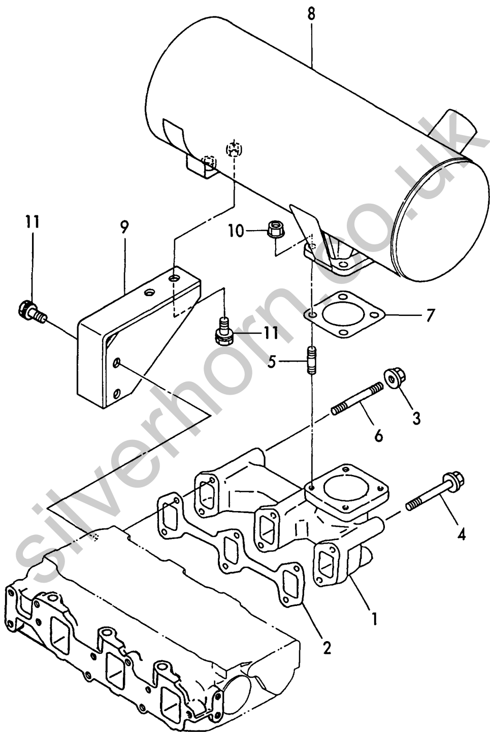
Fig. 6 排気マニホールド&サイレンサ EXHAUST MANIFOLD & SILENCER
