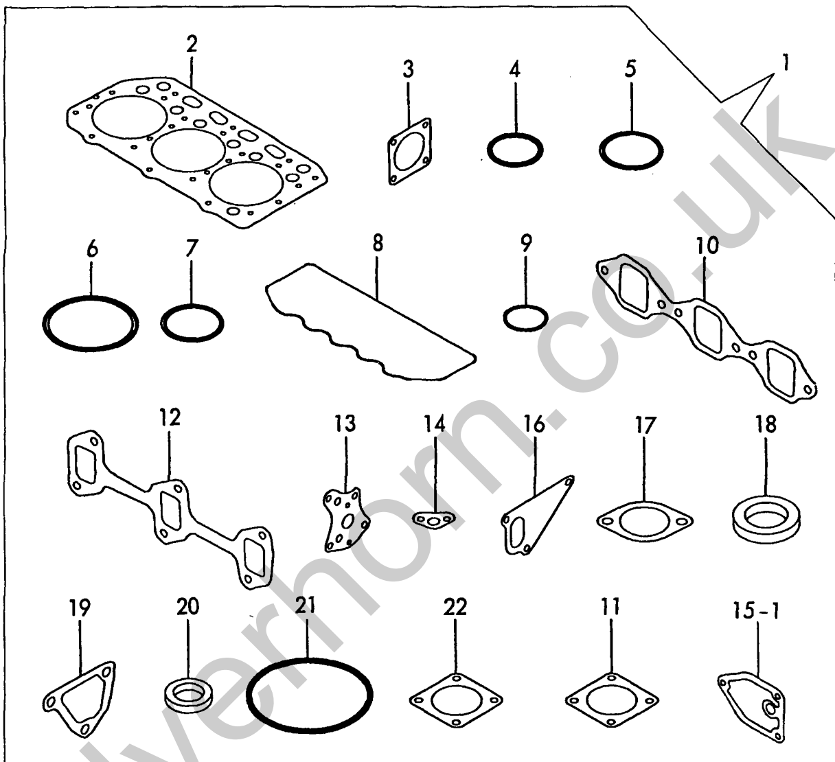
Fig. 18 パッキンセット(オプション)&工具 GASKET SET(OPTIONAL)& TOOL
