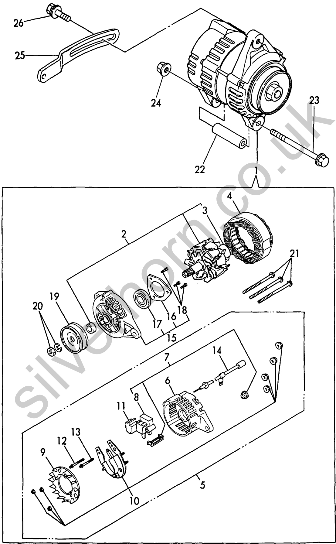
Fig. 17 ジェネレータ GENERATOR
