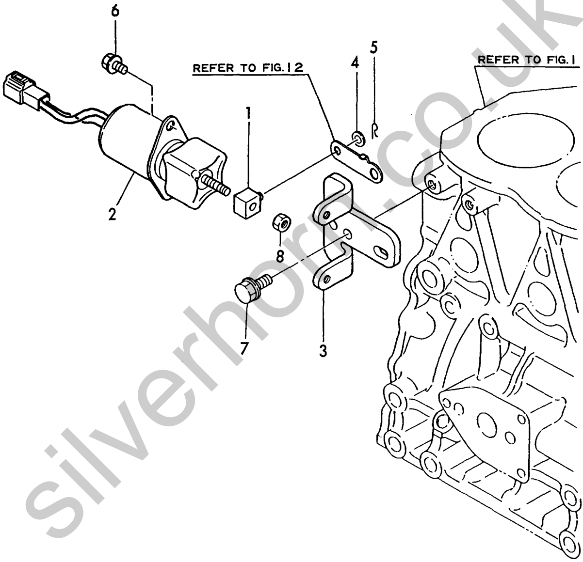
Fig. 15 機関停止装置 ENGINE STOP DEVICE
