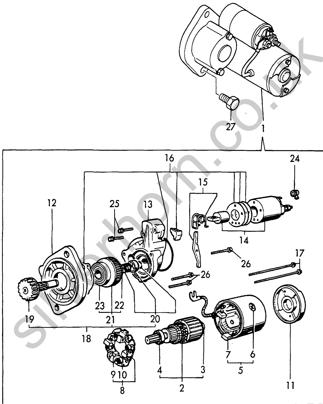
Fig. 16 スターティングモータ STARTING MOTOR
