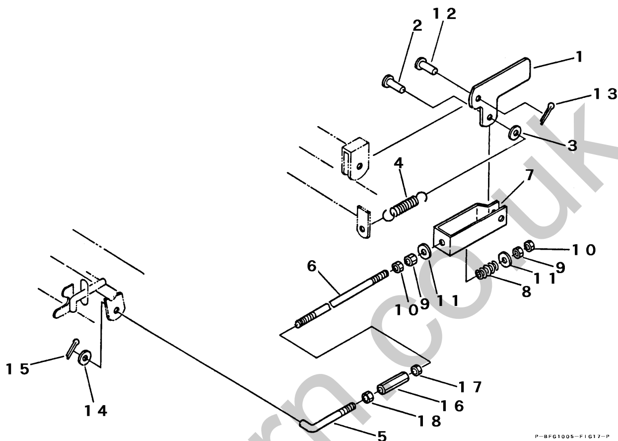
FIG 17 ゲートロック (一方ダンプ) GATE LOCK (1-WAY DUMPING)
