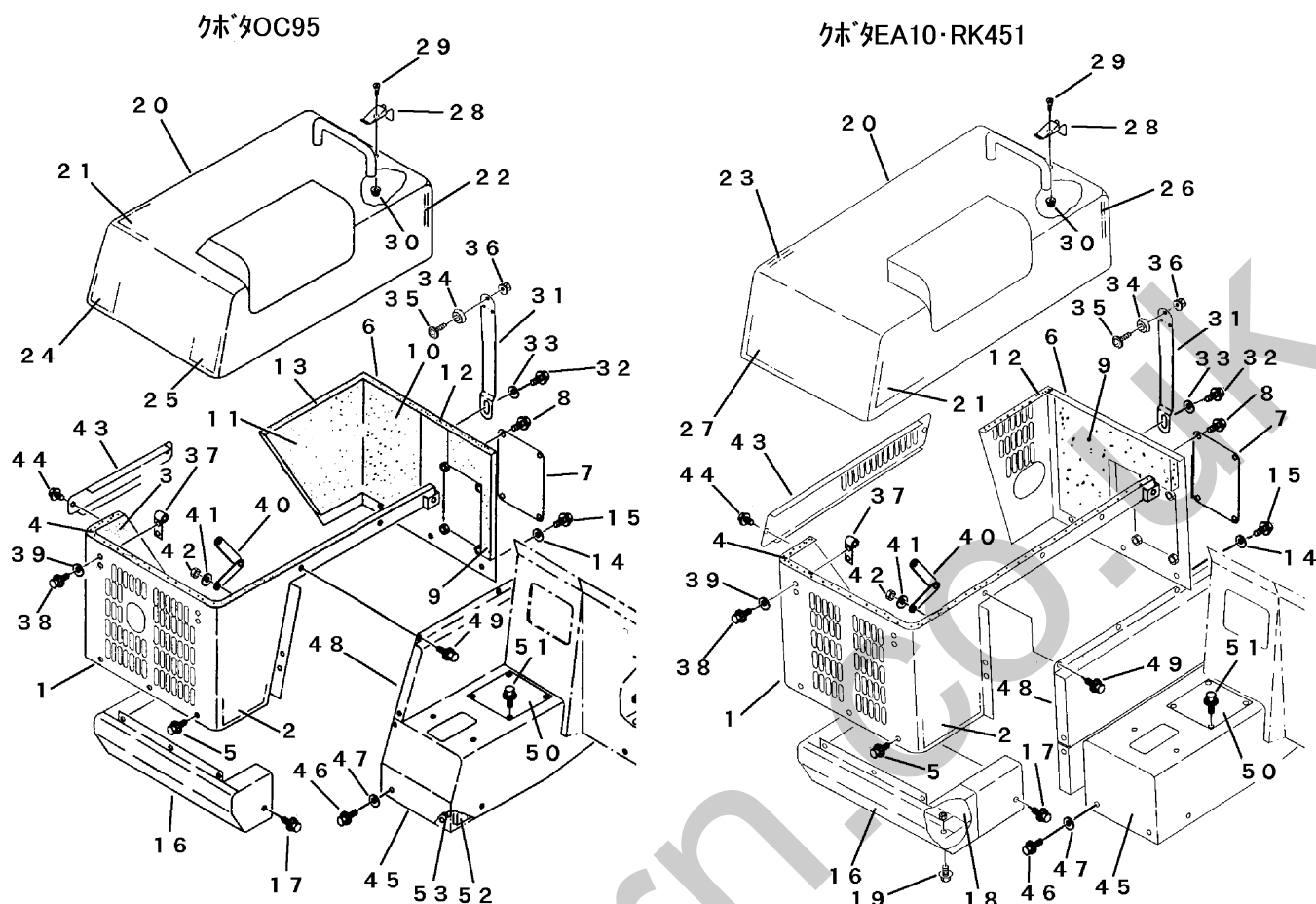
FIG 8 エンジンカバー COVER
