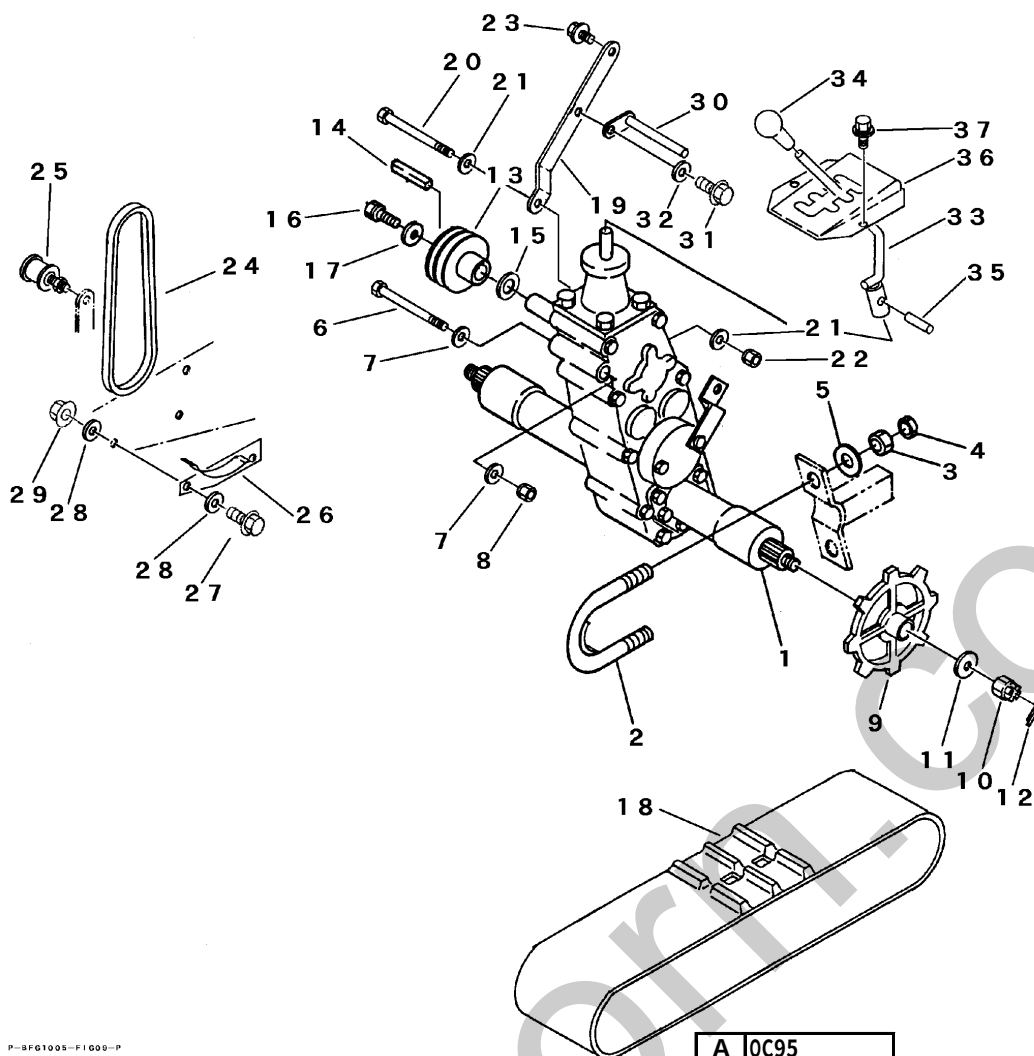
FIG 9 ミッション TRANSMISSION
