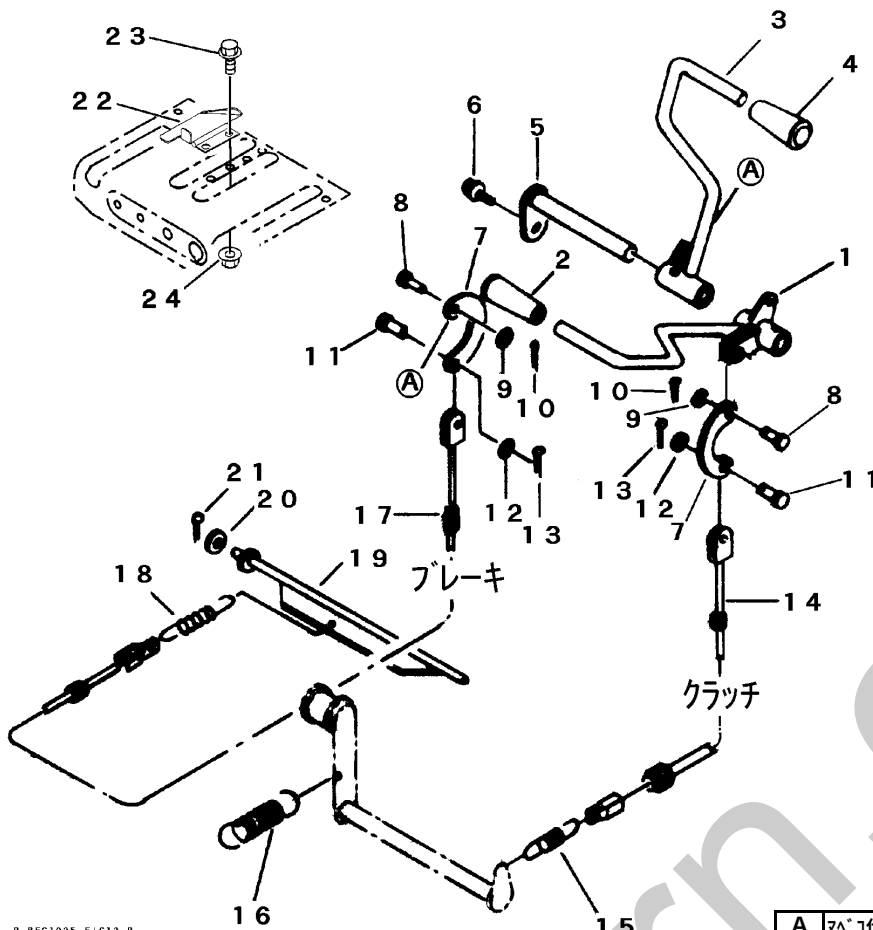
FIG 12 クラッチ & ブレーキ CLUTCH & BRAKE LEVER
