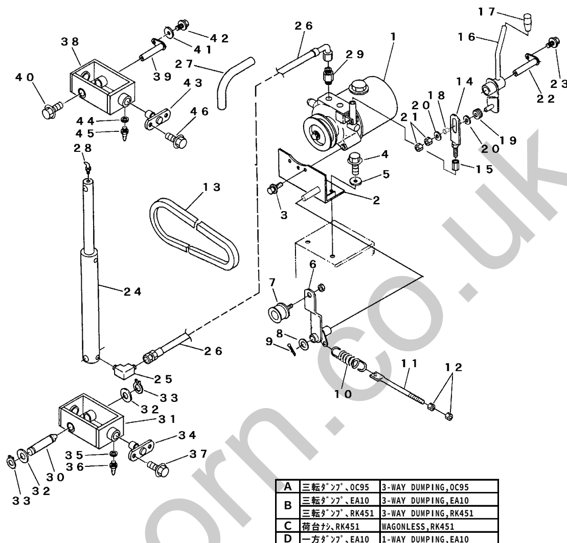
FIG 18 ユアツソウチ HYDRAULIC EQUIPMENT
