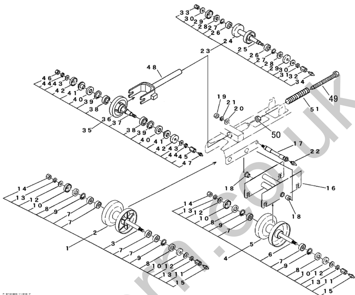
FIG 10 テンリン &amp; ユウドウリン ROLLER &amp; IDLER
