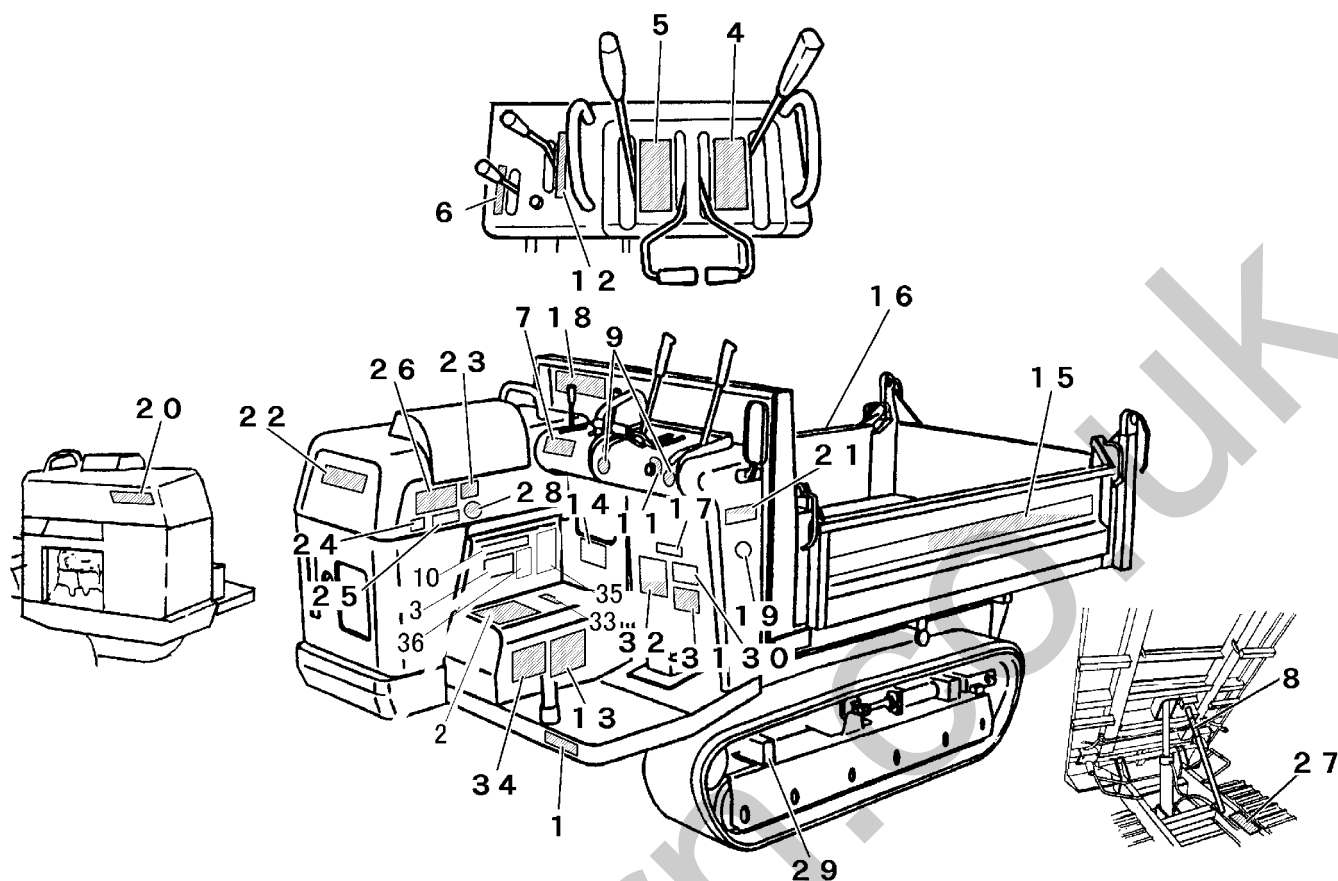
FIG 21 マーク (輸出仕様) MARK (OVERSEAS SPECS)
