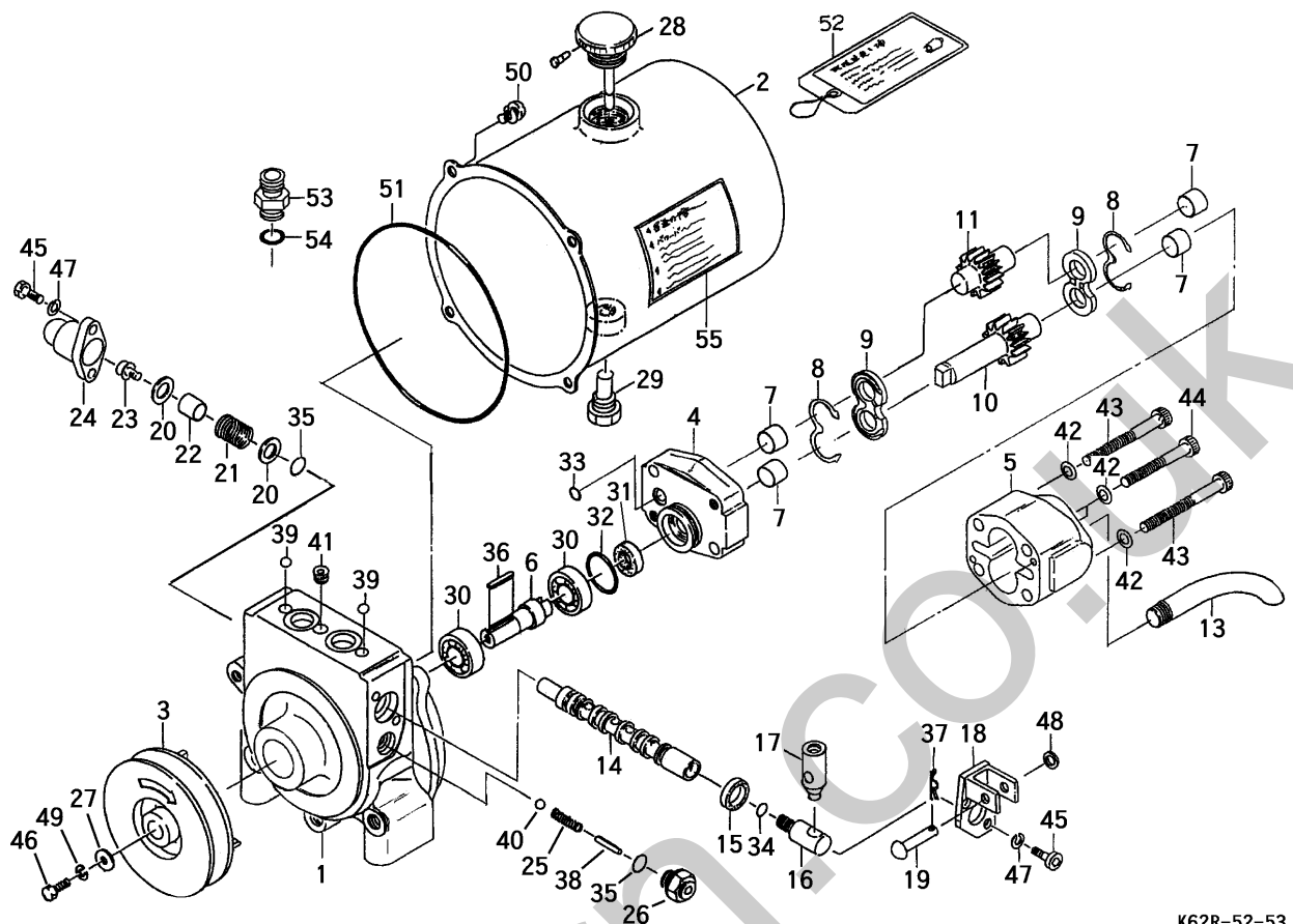
FIG 25 パッケージ HYDRAULIC PUMP NO.6260080～
