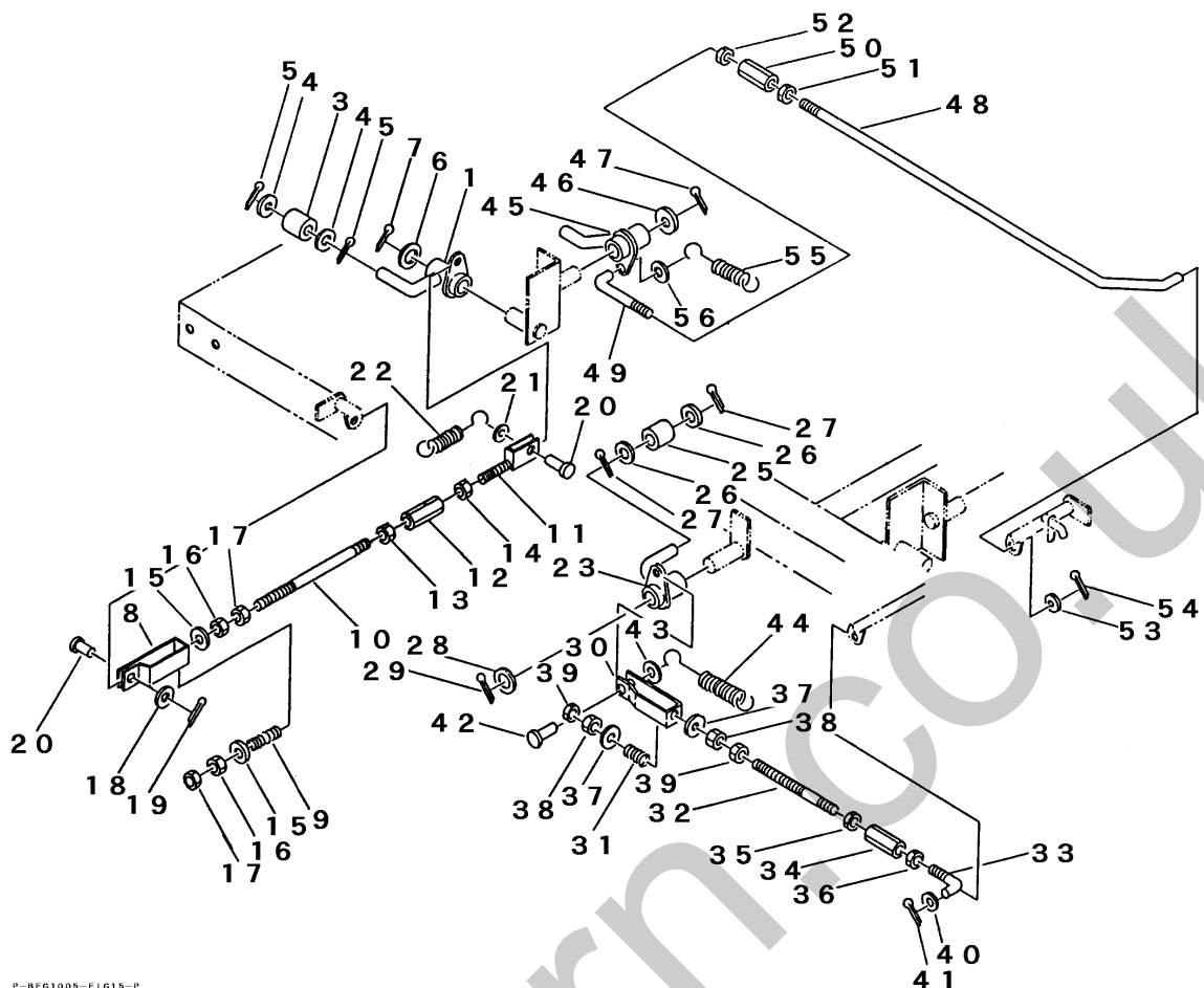
FIG 15 ゲートロック (三転ダンプ) GATE LOCK (3-WAY DUMPING)
