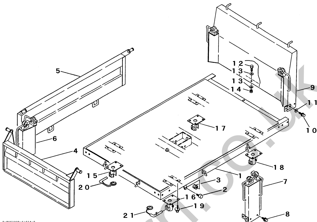
FIG 14 ニダイ &amp; ゲート (三転ダンプ)
