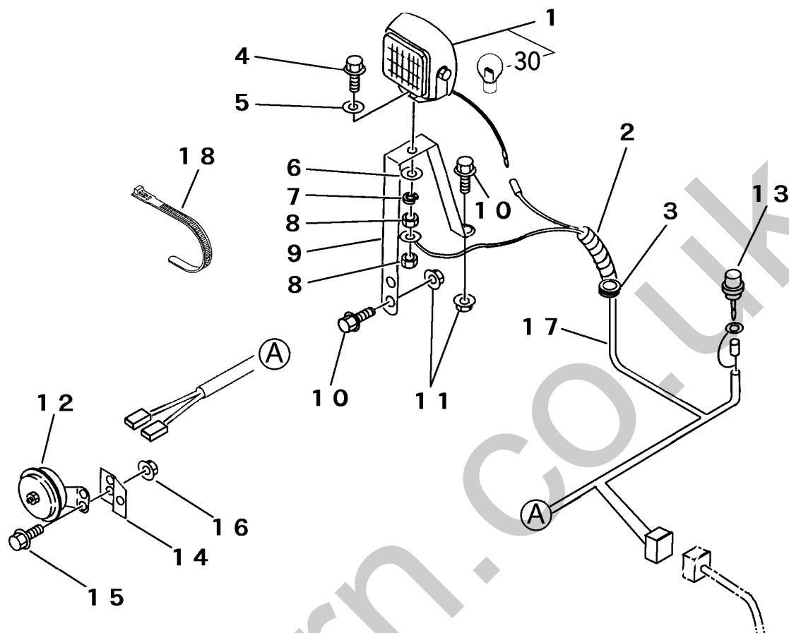
FIG 6 ワーキングランプ & ホーン (CE 対応) LIGHT & HORN (Parts for CE Marking)
