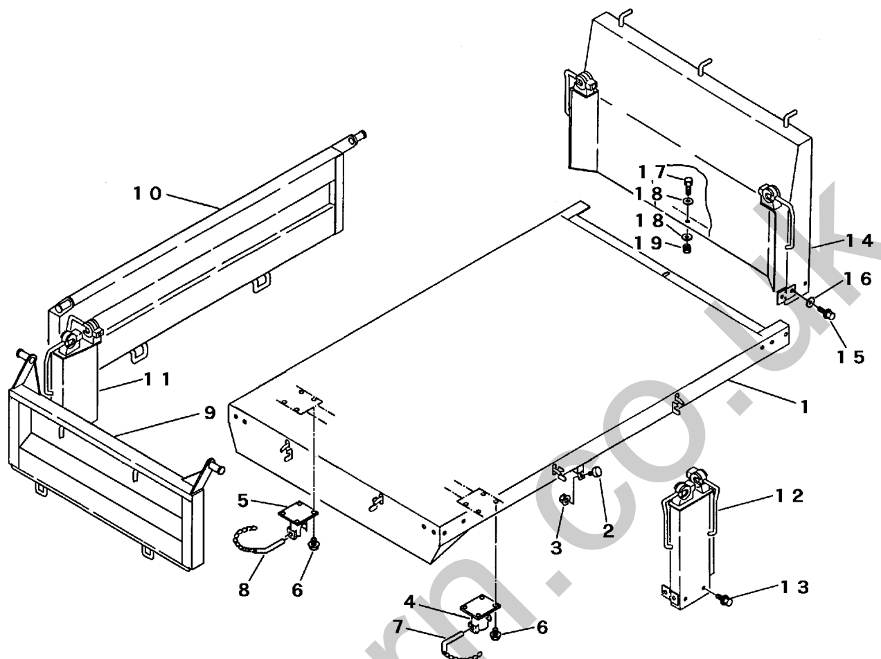
FIG 13 ニダイ &amp; ゲート (三転ダンプ)
